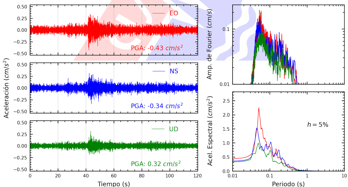
Figura A.4: Registros tiempo-historia, espectros de Fourier y de respuesta en las direcciones EO, NS y vertical de la estación UNTEL. Sismo de Matucana, Huarochiri - Lima del 2025-08-09, 22:08:34 (Hora local)
