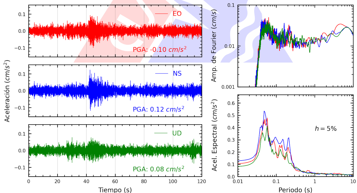
Figura A.16: Registros tiempo-historia, espectros de Fourier y de respuesta en las direcciones EO, NS y vertical de la estación IMCA. Sismo de Matucana, Huarochiri - Lima del 2025-08-09, 22:08:34 (Hora local)
