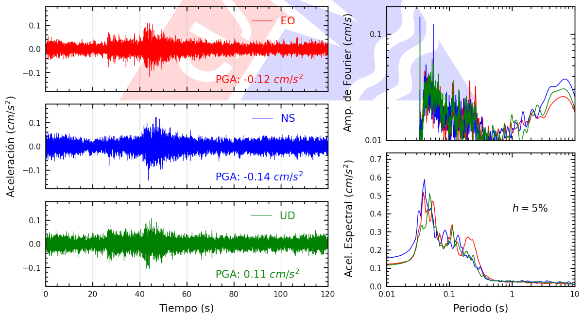
Figura A.14: Registros tiempo-historia, espectros de Fourier y de respuesta en las direcciones EO, NS y vertical de la estación USMP. Sismo de Matucana, Huarochiri - Lima del 2025-08-09, 22:08:34 (Hora local)
