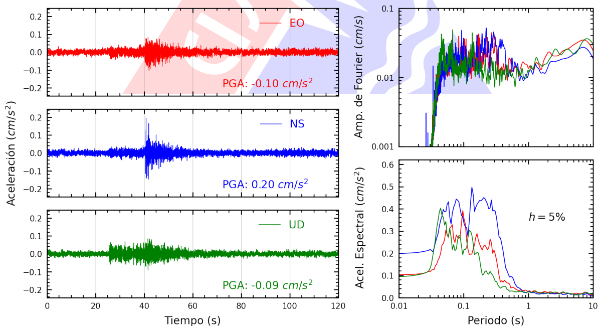
Figura A.8: Registros tiempo-historia, espectros de Fourier y de respuesta en las direcciones EO, NS y vertical de la estación USILP. Sismo de Matucana, Huarochiri - Lima del 2025-08-09, 22:08:34 (Hora local)
