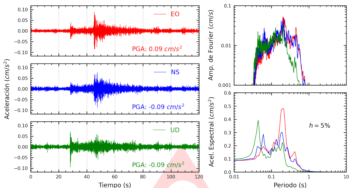
Figura A.19: Registros tiempo-historia, espectros de Fourier y de respuesta en las direcciones EO, NS y vertical de la estación VHAYA. Sismo de Matucana, Huarochiri - Lima del 2025-08-09, 22:08:34 (Hora local)
