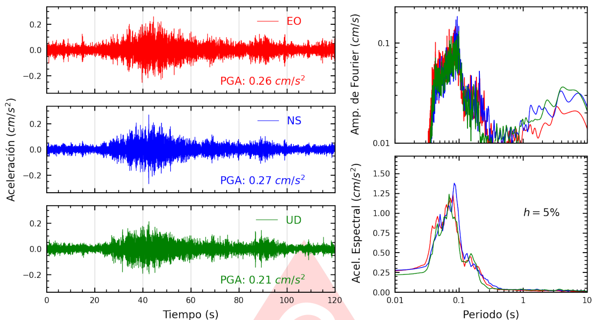
Figura A.7: Registros tiempo-historia, espectros de Fourier y de respuesta en las direcciones EO, NS y vertical de la estación INDEP. Sismo de Matucana, Huarochiri - Lima del 2025-08-09, 22:08:34 (Hora local)
