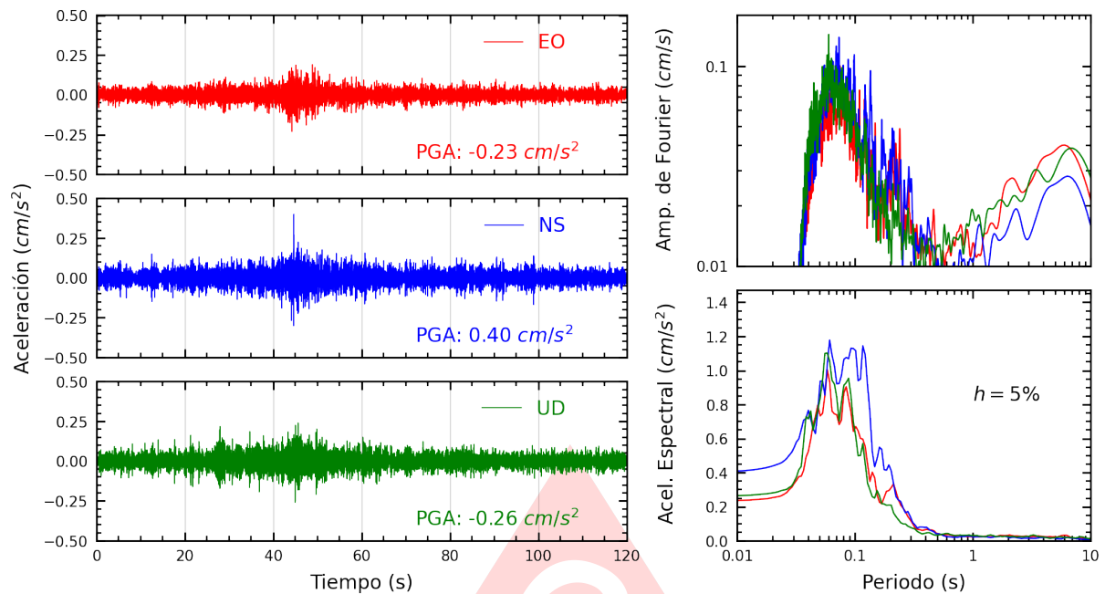
Figura A.5: Registros tiempo-historia, espectros de Fourier y de respuesta en las direcciones EO, NS y vertical de la estación SJLSC. Sismo de Matucana, Huarochiri - Lima del 2025-08-09, 22:08:34 (Hora local)
