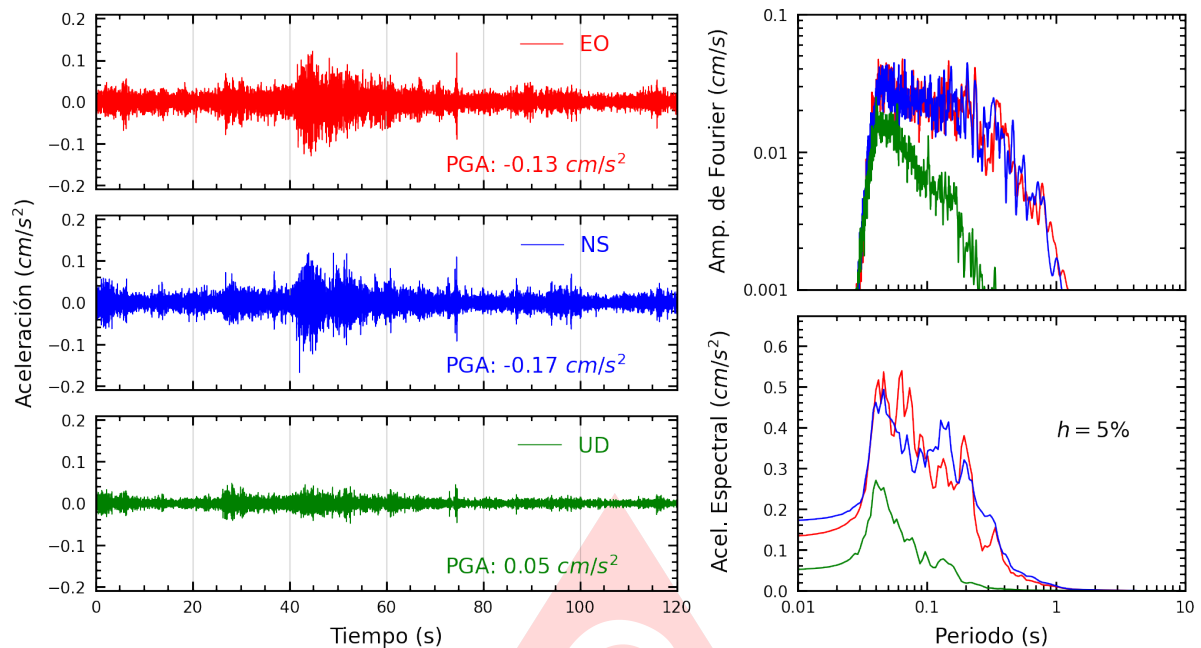
Figura A.11: Registros tiempo-historia, espectros de Fourier y de respuesta en las direcciones EO, NS y vertical de la estación UCVAT. Sismo de Matucana, Huarochiri - Lima del 2025-08-09, 22:08:34 (Hora local)
