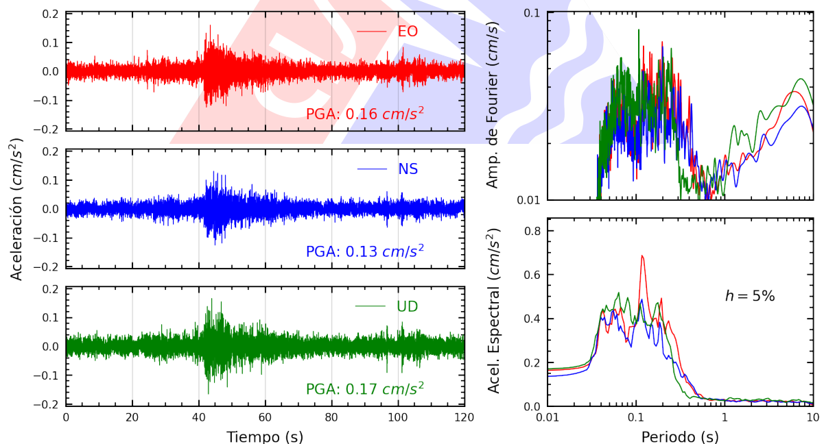
Figura A.12: Registros tiempo-historia, espectros de Fourier y de respuesta en las direcciones EO, NS y vertical de la estación SOVES. Sismo de Matucana, Huarochiri - Lima del 2025-08-09, 22:08:34 (Hora local)
