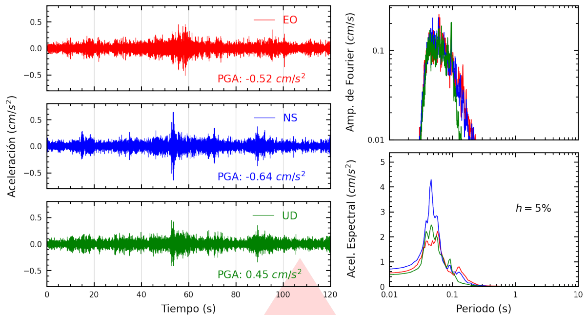
Figura A.1: Registros tiempo-historia, espectros de Fourier y de respuesta en las direcciones EO, NS y vertical de la estación SROSA. Sismo de Matucana, Huarochiri - Lima del 2025-08-09, 22:08:34 (Hora local)
