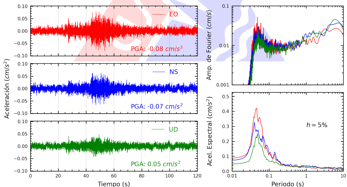
Figura A.20: Registros tiempo-historia, espectros de Fourier y de respuesta en las direcciones EO, NS y vertical de la estación UCSS. Sismo de Matucana, Huarochiri - Lima del 2025-08-09, 22:08:34 (Hora local)
