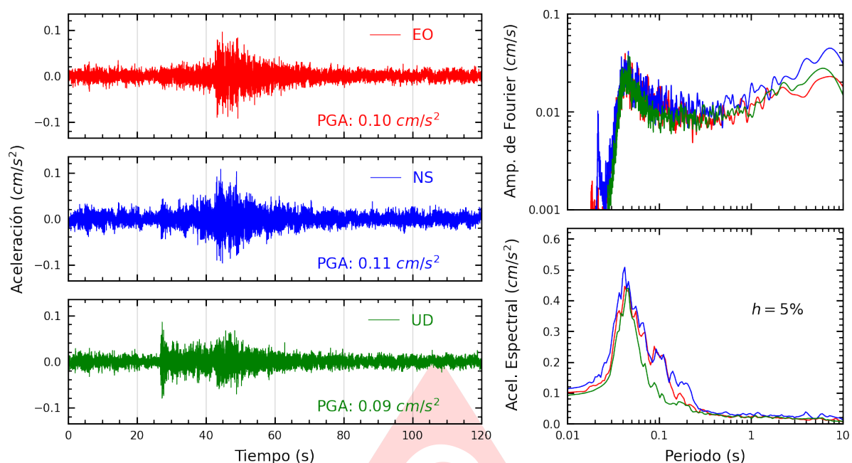
Figura A.17: Registros tiempo-historia, espectros de Fourier y de respuesta en las direcciones EO, NS y vertical de la estación SJLCE. Sismo de Matucana, Huarochiri - Lima del 2025-08-09, 22:08:34 (Hora local)
