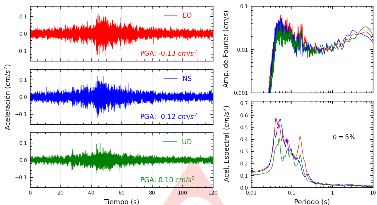
Figura A.15: Registros tiempo-historia, espectros de Fourier y de respuesta en las direcciones EO, NS y vertical de la estación FICPE. Sismo de Matucana, Huarochiri - Lima del 2025-08-09, 22:08:34 (Hora local)
