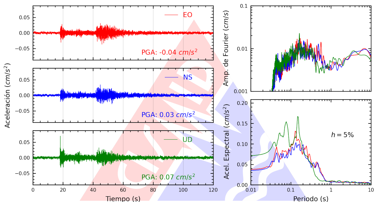
Figura A.21: Registros tiempo-historia, espectros de Fourier y de respuesta en las direcciones EO, NS y vertical de la estación CARAL. Sismo de Matucana, Huarochiri - Lima del 2025-08-09, 22:08:34 (Hora local)
