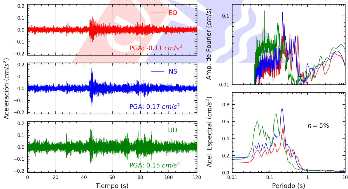
Figura A.10: Registros tiempo-historia, espectros de Fourier y de respuesta en las direcciones EO, NS y vertical de la estación MDPP. Sismo de Matucana, Huarochiri - Lima del 2025-08-09, 22:08:34 (Hora local)
