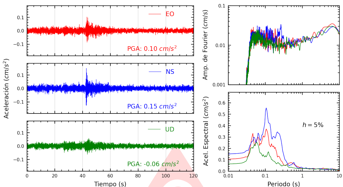
Figura A.13: Registros tiempo-historia, espectros de Fourier y de respuesta en las direcciones EO, NS y vertical de la estación SERVI. Sismo de Matucana, Huarochiri - Lima del 2025-08-09, 22:08:34 (Hora local)
