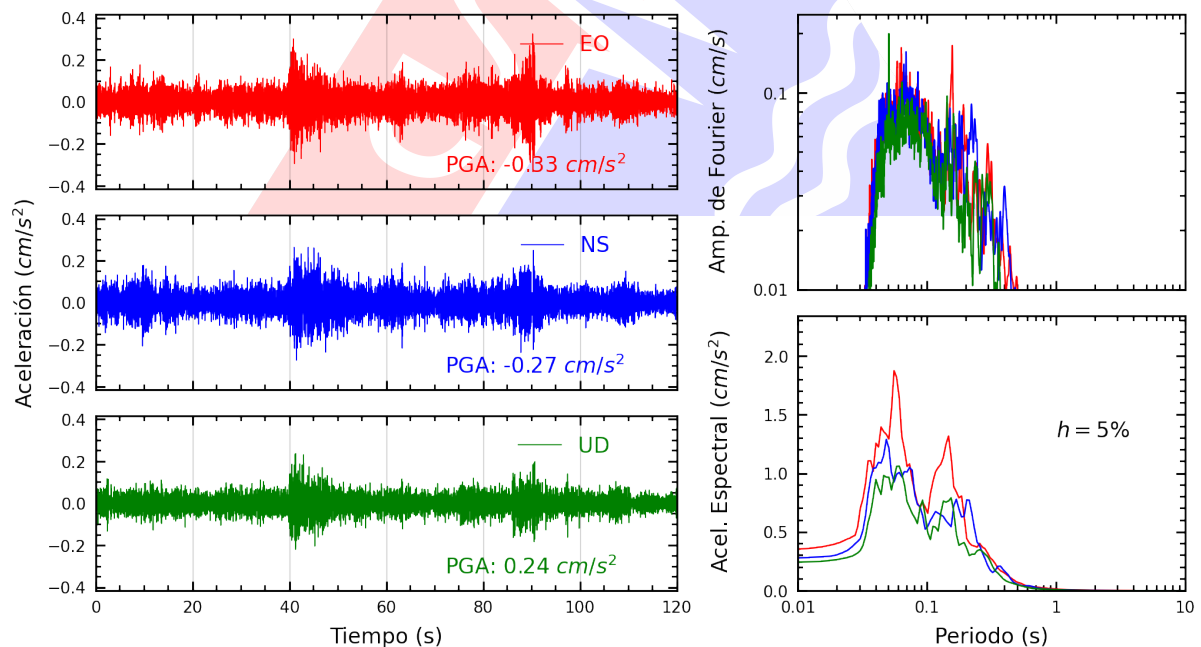
Figura A.6: Registros tiempo-historia, espectros de Fourier y de respuesta en las direcciones EO, NS y vertical de la estación PHERM. Sismo de Matucana, Huarochiri - Lima del 2025-08-09, 22:08:34 (Hora local)
