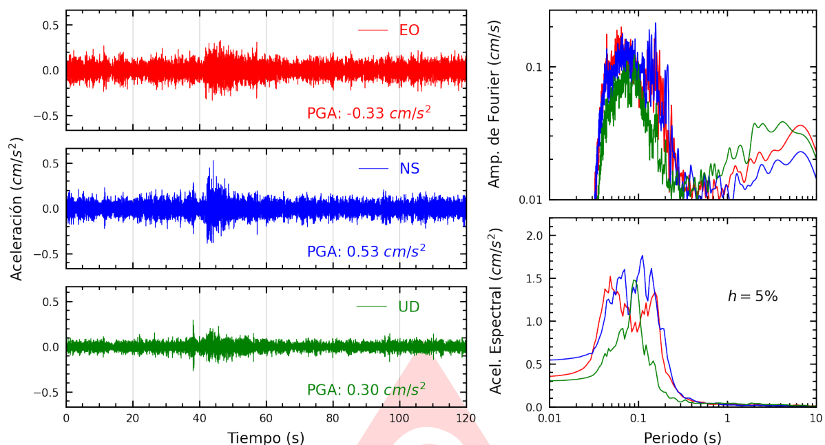
Figura A.3: Registros tiempo-historia, espectros de Fourier y de respuesta en las direcciones EO, NS y vertical de la estación USILM. Sismo de Matucana, Huarochiri - Lima del 2025-08-09, 22:08:34 (Hora local)
