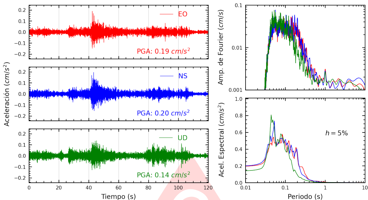
Figura A.9: Registros tiempo-historia, espectros de Fourier y de respuesta en las direcciones EO, NS y vertical de la estación ASIA. Sismo de Matucana, Huarochiri - Lima del 2025-08-09, 22:08:34 (Hora local)
