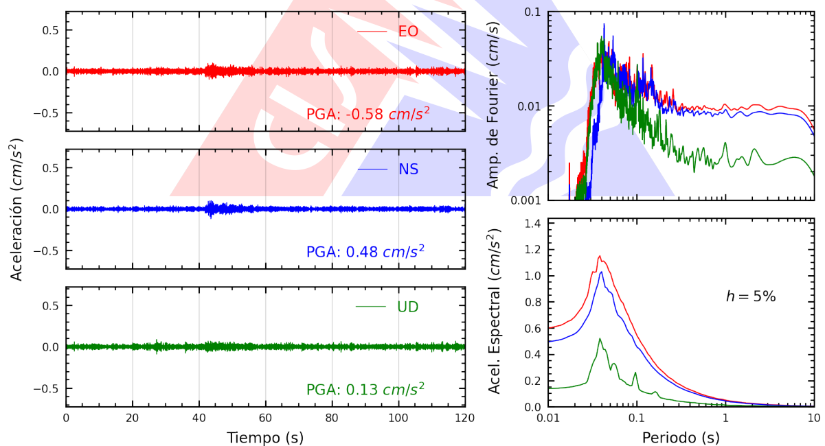
Figura A.2: Registros tiempo-historia, espectros de Fourier y de respuesta en las direcciones EO, NS y vertical de la estación ATARJ. Sismo de Matucana, Huarochiri - Lima del 2025-08-09, 22:08:34 (Hora local)
