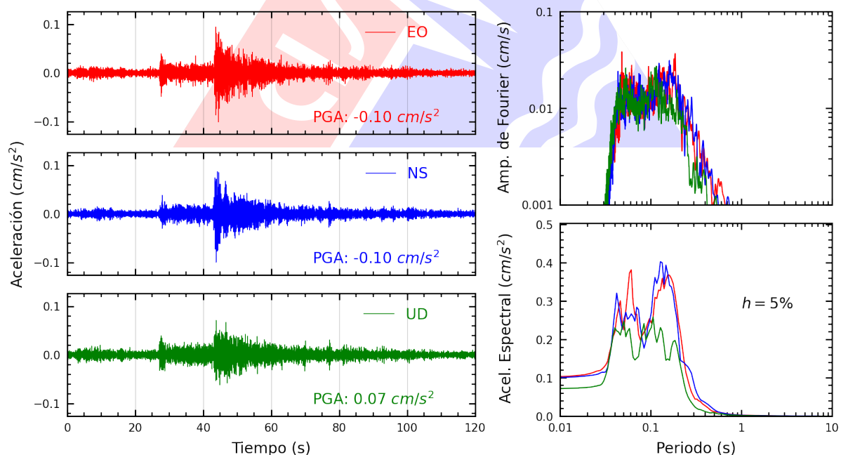
Figura A.18: Registros tiempo-historia, espectros de Fourier y de respuesta en las direcciones EO, NS y vertical de la estación JALV2. Sismo de Matucana, Huarochiri - Lima del 2025-08-09, 22:08:34 (Hora local)
