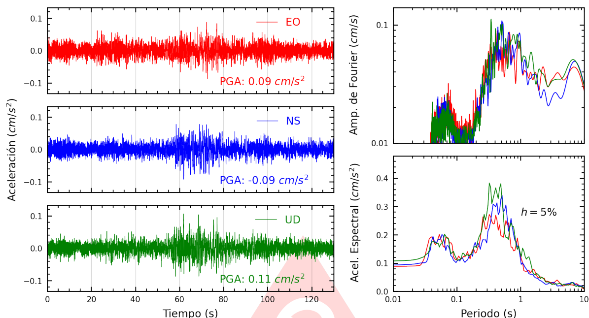
Figura A.25: Registros tiempo-historia, espectros de Fourier y de respuesta en las direcciones EO, NS y vertical de la estación UNSCH. Sismo de Pisco, Pisco - Ica del 2025-08-11, 06:41:24 (Hora local)
