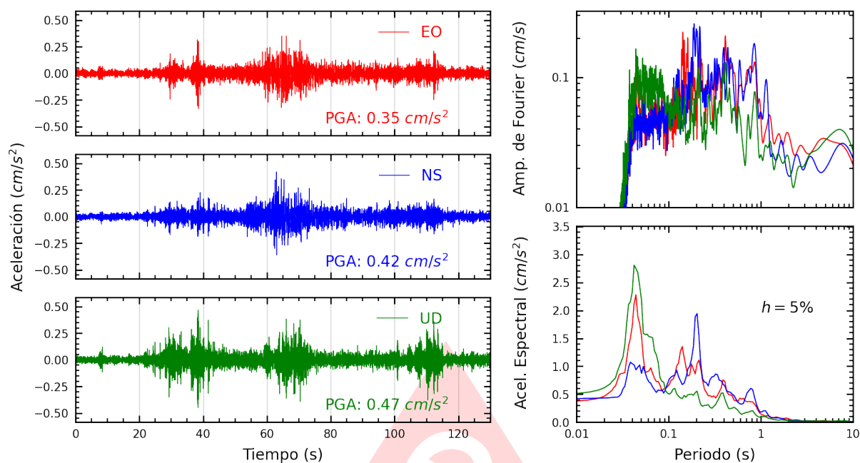
Figura A.5: Registros tiempo-historia, espectros de Fourier y de respuesta en las direcciones EO, NS y vertical de la estación SOCHO. Sismo de Pisco, Pisco - Ica del 2025-08-11, 06:41:24 (Hora local)
