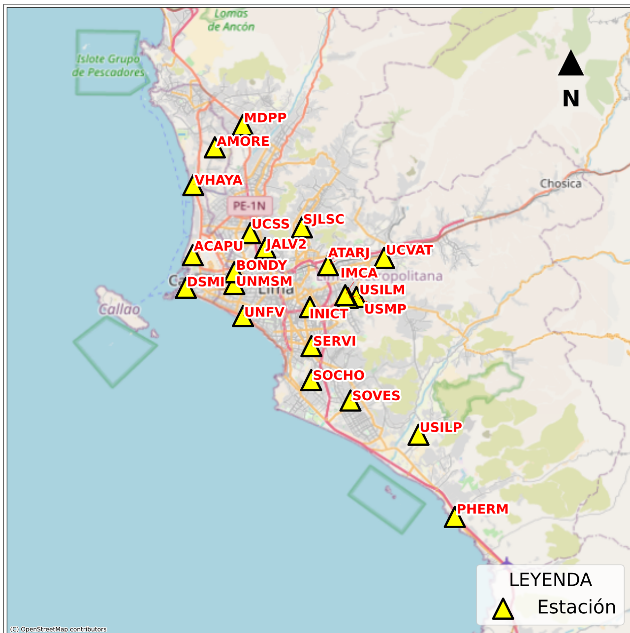
Figura 3: Mapa de ubicación de la(s) estación(es) acelerográfica(s) en Lima Metropolitana correspondiente(s) al Sismo de Pisco, Pisco - Ica del 11 de agosto de 2025 a las 06:41:24 (hora local)
