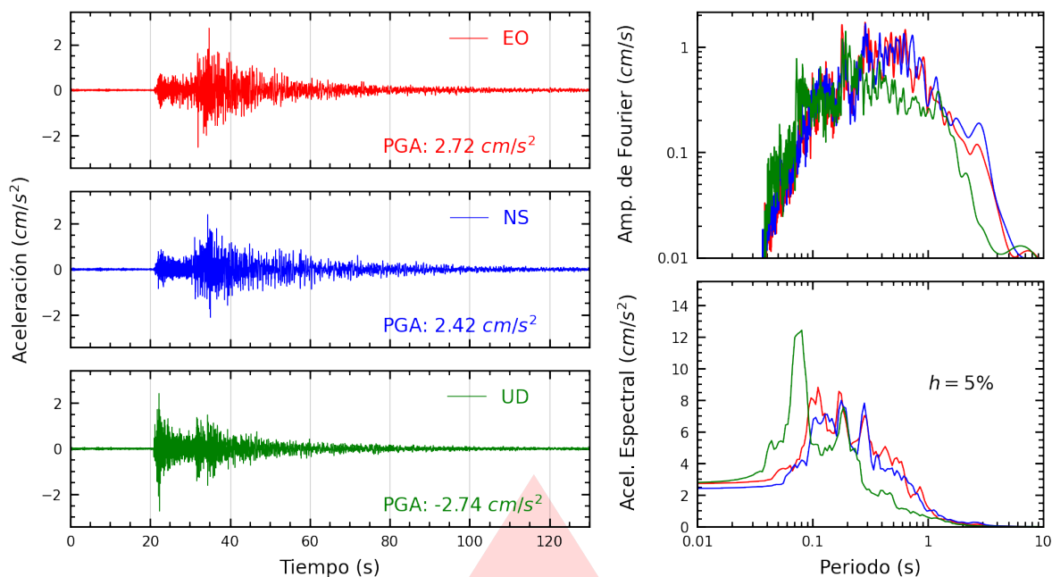
Figura A.1: Registros tiempo-historia, espectros de Fourier y de respuesta en las direcciones EO, NS y vertical de la estación UNICA. Sismo de Pisco, Pisco - Ica del 2025-08-11, 06:41:24 (Hora local)
