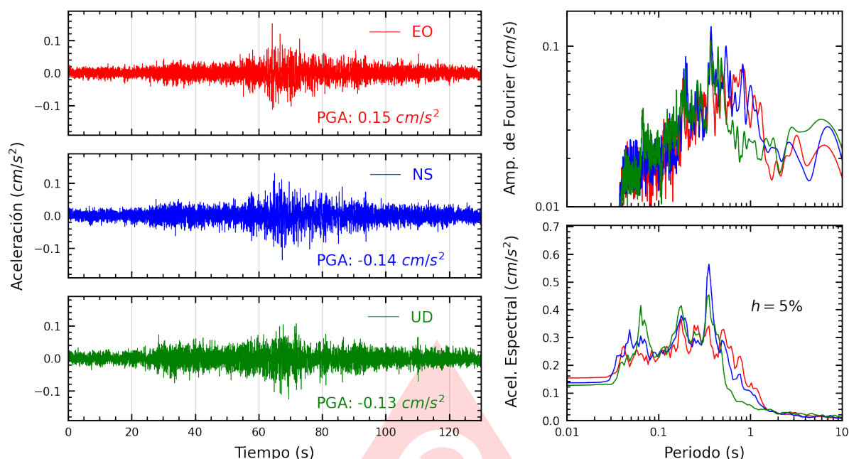
Figura A.19: Registros tiempo-historia, espectros de Fourier y de respuesta en las direcciones EO, NS y vertical de la estación UNFV. Sismo de Pisco, Pisco - Ica del 2025-08-11, 06:41:24 (Hora local)
