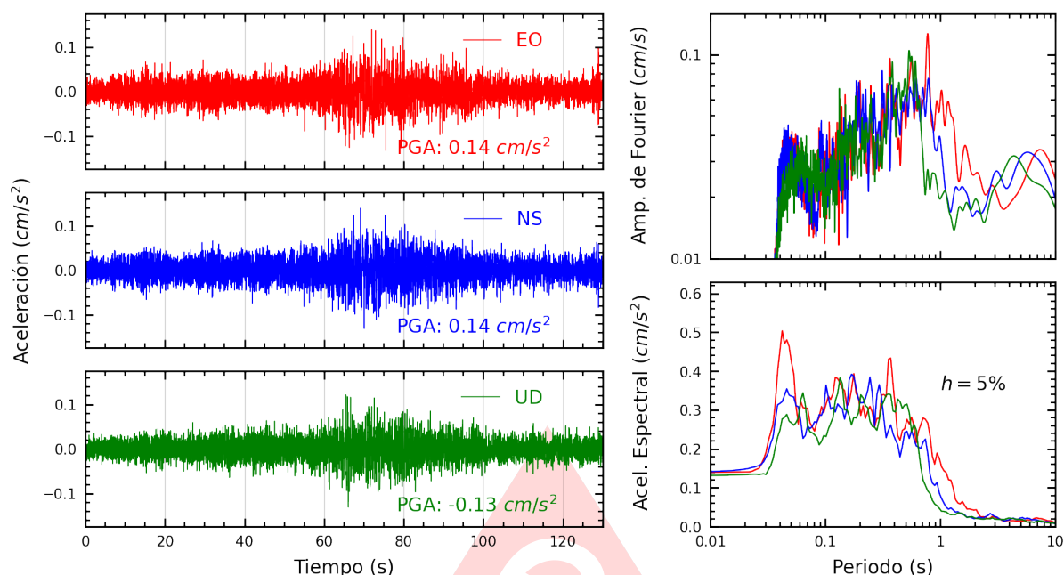
Figura A.21: Registros tiempo-historia, espectros de Fourier y de respuesta en las direcciones EO, NS y vertical de la estación IMCA. Sismo de Pisco, Pisco - Ica del 2025-08-11, 06:41:24 (Hora local)
