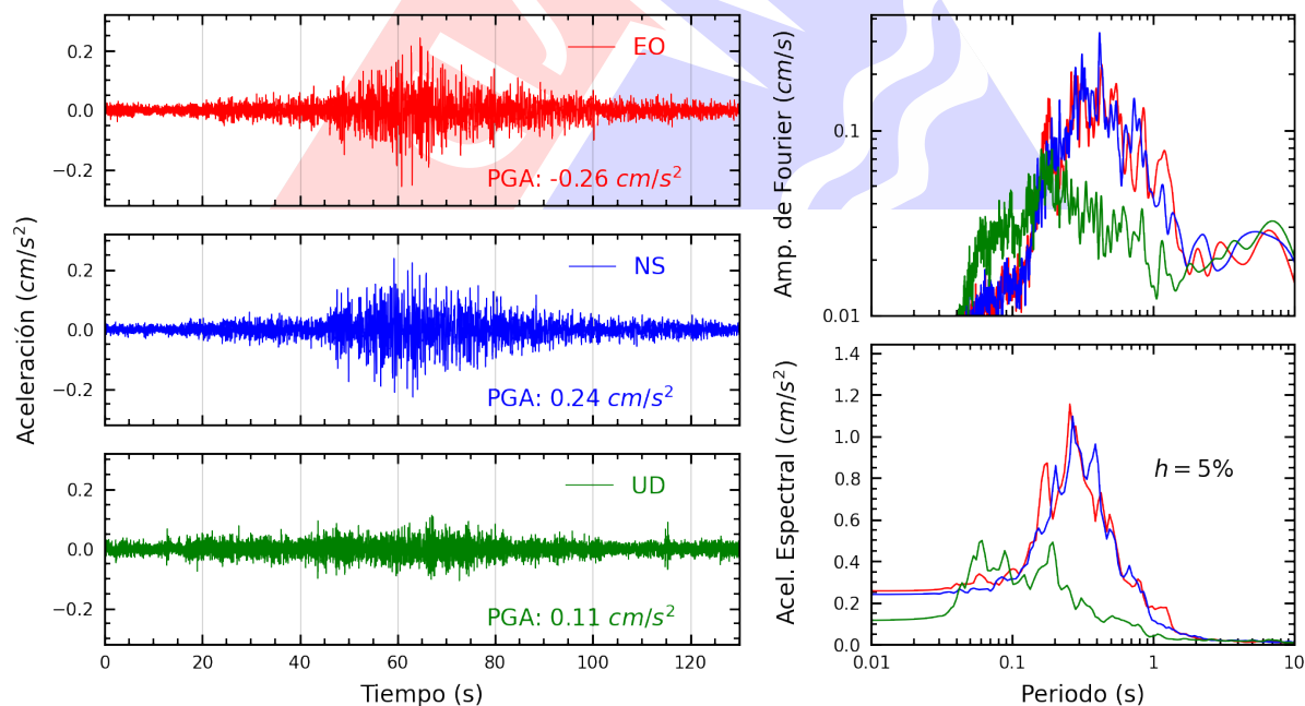
Figura A.12: Registros tiempo-historia, espectros de Fourier y de respuesta en las direcciones EO, NS y vertical de la estación ACAPU. Sismo de Pisco, Pisco - Ica del 2025-08-11, 06:41:24 (Hora local)
