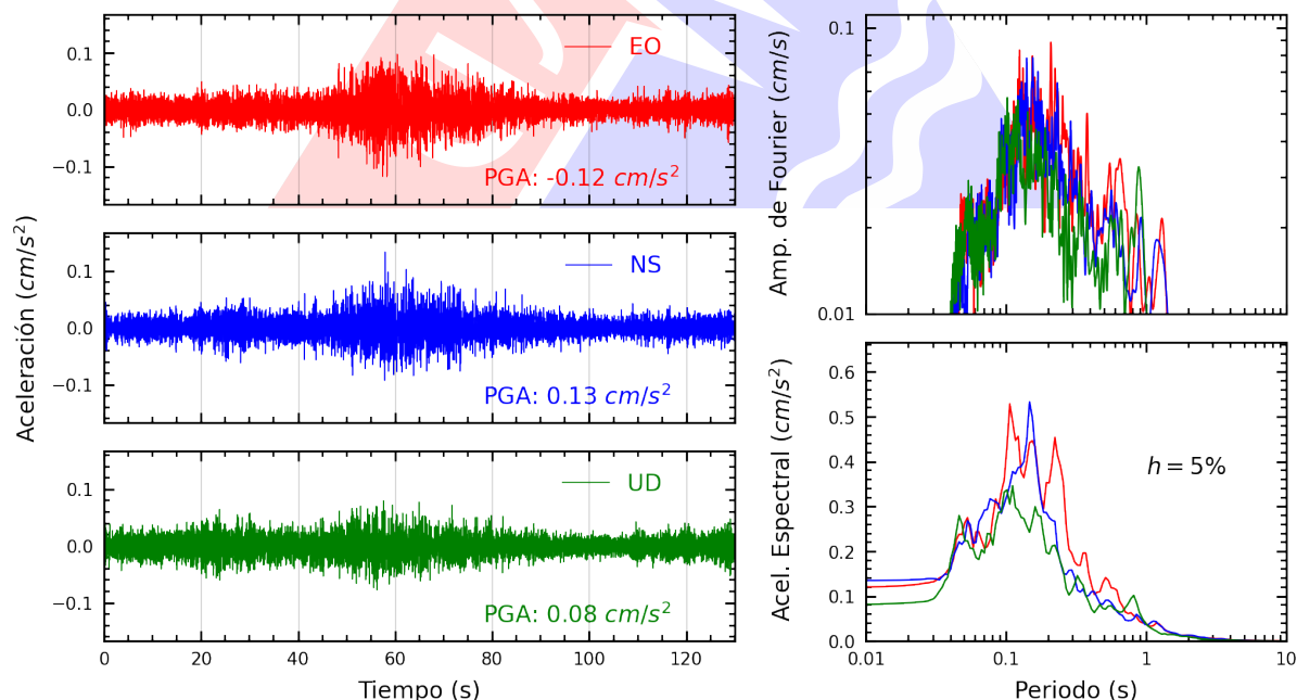
Figura A.22: Registros tiempo-historia, espectros de Fourier y de respuesta en las direcciones EO, NS y vertical de la estación JALV2. Sismo de Pisco, Pisco - Ica del 2025-08-11, 06:41:24 (Hora local)
