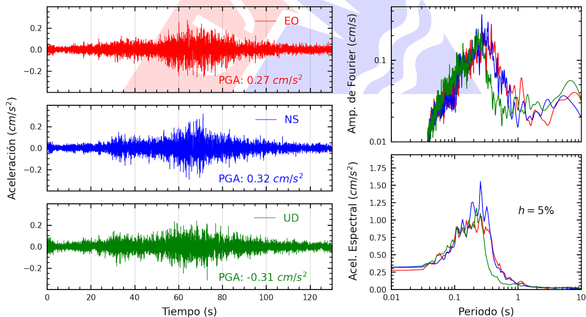
Figura A.10: Registros tiempo-historia, espectros de Fourier y de respuesta en las direcciones EO, NS y vertical de la estación SOVES. Sismo de Pisco, Pisco - Ica del 2025-08-11, 06:41:24 (Hora local)
