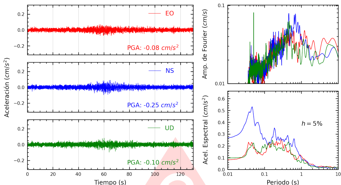
Figura A.13: Registros tiempo-historia, espectros de Fourier y de respuesta en las direcciones EO, NS y vertical de la estación BONDY. Sismo de Pisco, Pisco - Ica del 2025-08-11, 06:41:24 (Hora local)
