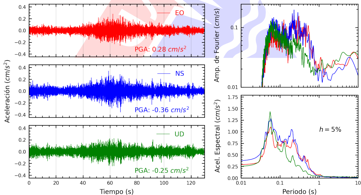
Figura A.6: Registros tiempo-historia, espectros de Fourier y de respuesta en las direcciones EO, NS y vertical de la estación SJLSC. Sismo de Pisco, Pisco - Ica del 2025-08-11, 06:41:24 (Hora local)
