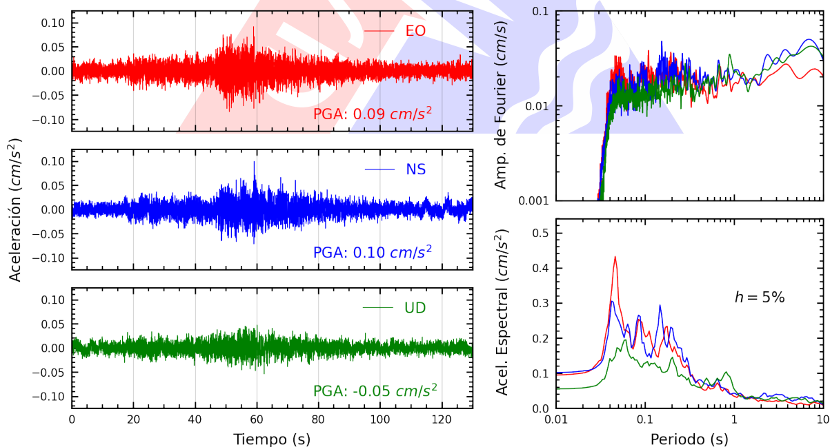
Figura A.26: Registros tiempo-historia, espectros de Fourier y de respuesta en las direcciones EO, NS y vertical de la estación UCSS. Sismo de Pisco, Pisco - Ica del 2025-08-11, 06:41:24 (Hora local)
