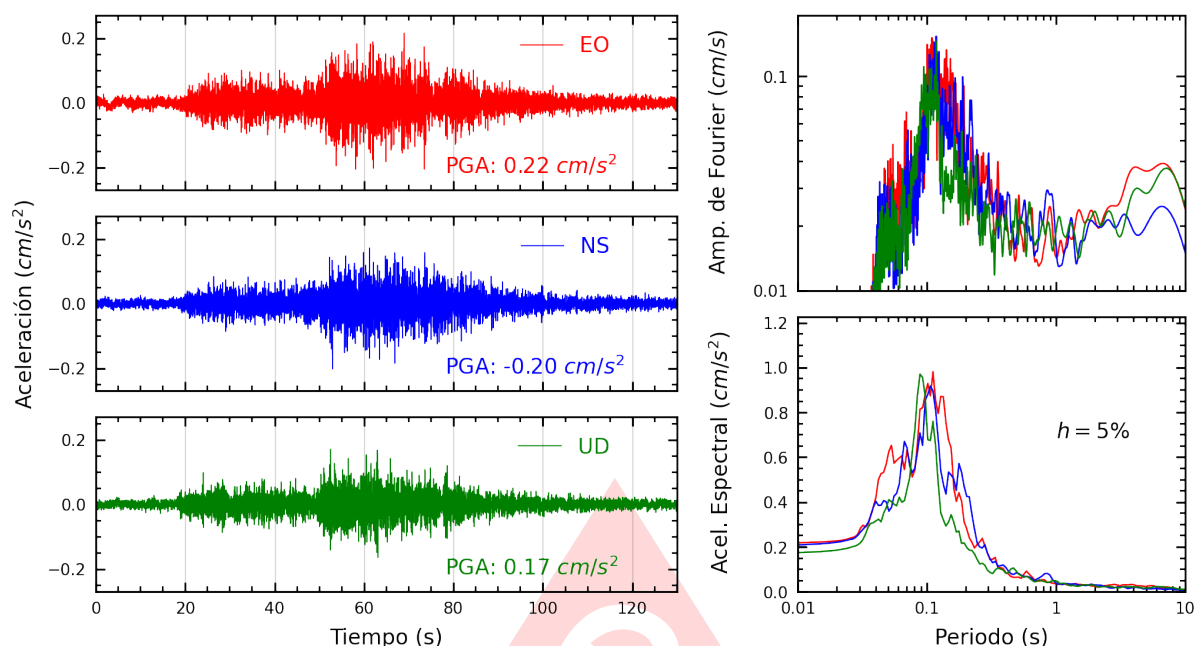
Figura A.15: Registros tiempo-historia, espectros de Fourier y de respuesta en las direcciones EO, NS y vertical de la estación AMORE. Sismo de Pisco, Pisco - Ica del 2025-08-11, 06:41:24 (Hora local)
