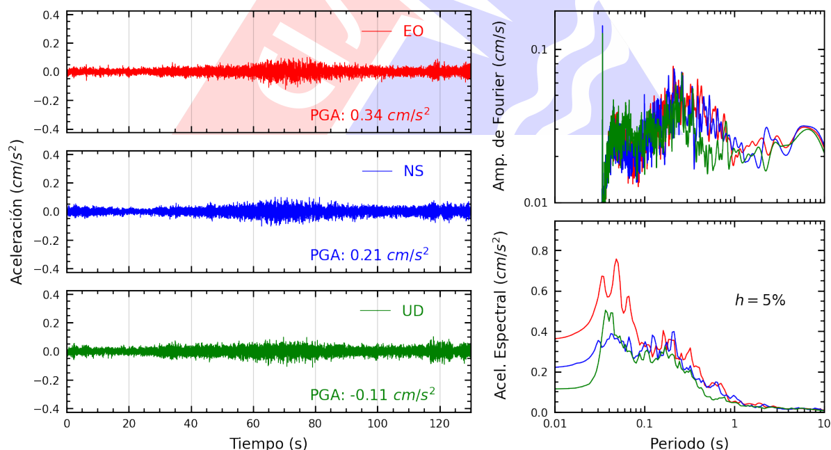
Figura A.8: Registros tiempo-historia, espectros de Fourier y de respuesta en las direcciones EO, NS y vertical de la estación USMP. Sismo de Pisco, Pisco - Ica del 2025-08-11, 06:41:24 (Hora local)
