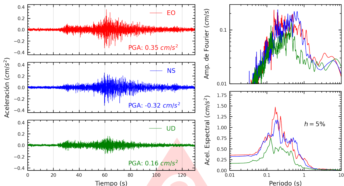
Figura A.7: Registros tiempo-historia, espectros de Fourier y de respuesta en las direcciones EO, NS y vertical de la estación USILP. Sismo de Pisco, Pisco - Ica del 2025-08-11, 06:41:24 (Hora local)
