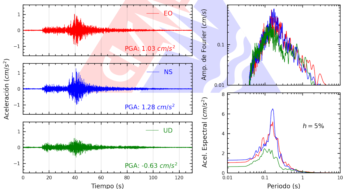
Figura A.2: Registros tiempo-historia, espectros de Fourier y de respuesta en las direcciones EO, NS y vertical de la estación ASIA. Sismo de Pisco, Pisco - Ica del 2025-08-11, 06:41:24 (Hora local)
