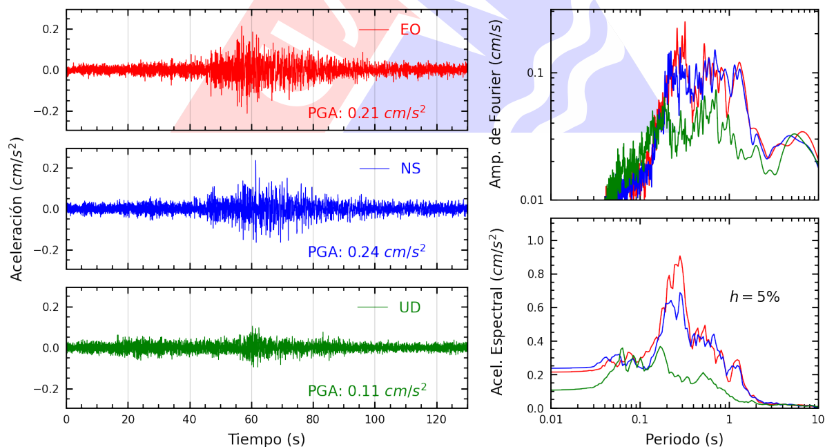
Figura A.14: Registros tiempo-historia, espectros de Fourier y de respuesta en las direcciones EO, NS y vertical de la estación DSMI. Sismo de Pisco, Pisco - Ica del 2025-08-11, 06:41:24 (Hora local)
