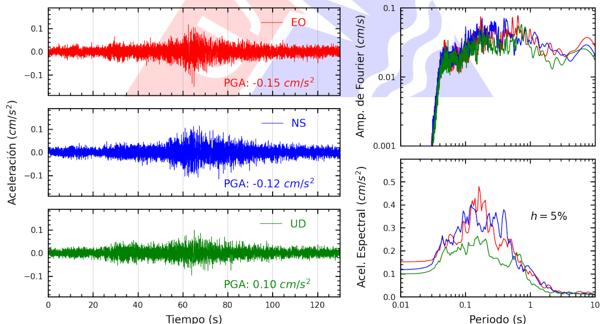
Figura A.20: Registros tiempo-historia, espectros de Fourier y de respuesta en las direcciones EO, NS y vertical de la estación SERVI. Sismo de Pisco, Pisco - Ica del 2025-08-11, 06:41:24 (Hora local)
