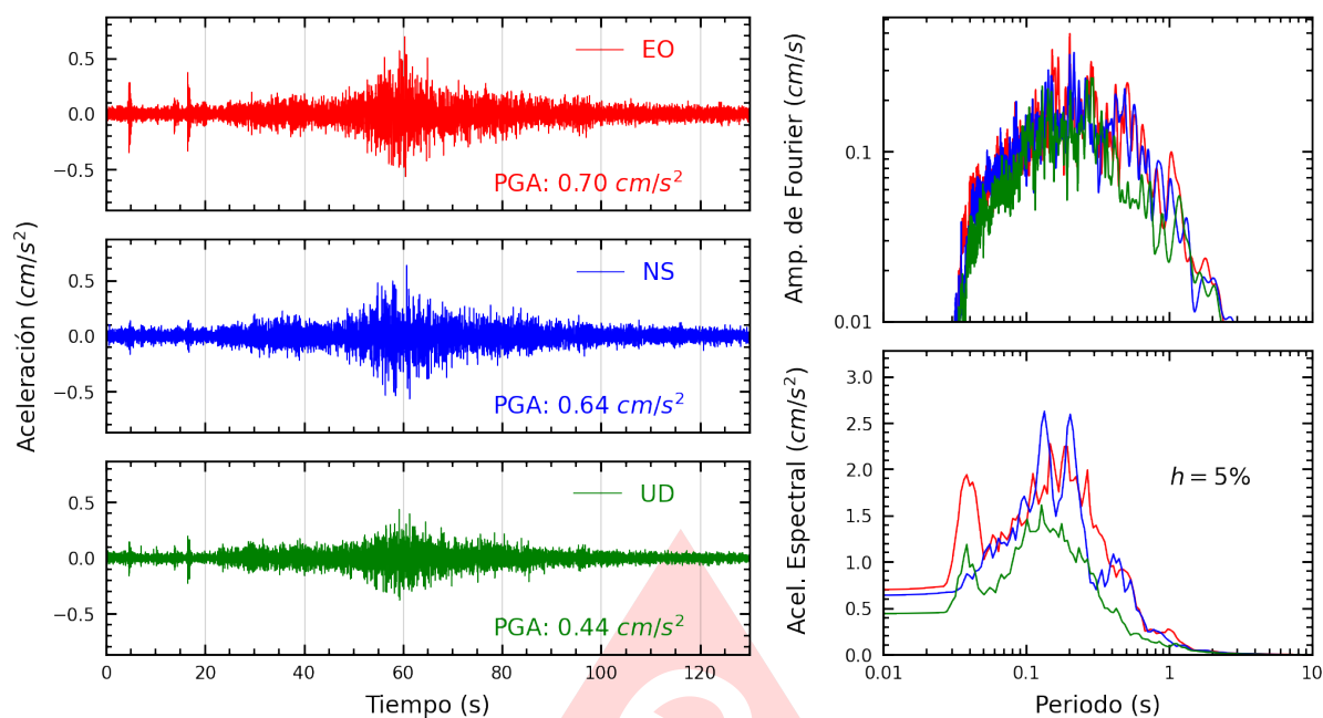
Figura A.3: Registros tiempo-historia, espectros de Fourier y de respuesta en las direcciones EO, NS y vertical de la estación PHERM. Sismo de Pisco, Pisco - Ica del 2025-08-11, 06:41:24 (Hora local)
