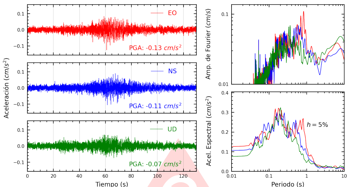
Figura A.23: Registros tiempo-historia, espectros de Fourier y de respuesta en las direcciones EO, NS y vertical de la estación UNMSM. Sismo de Pisco, Pisco - Ica del 2025-08-11, 06:41:24 (Hora local)
