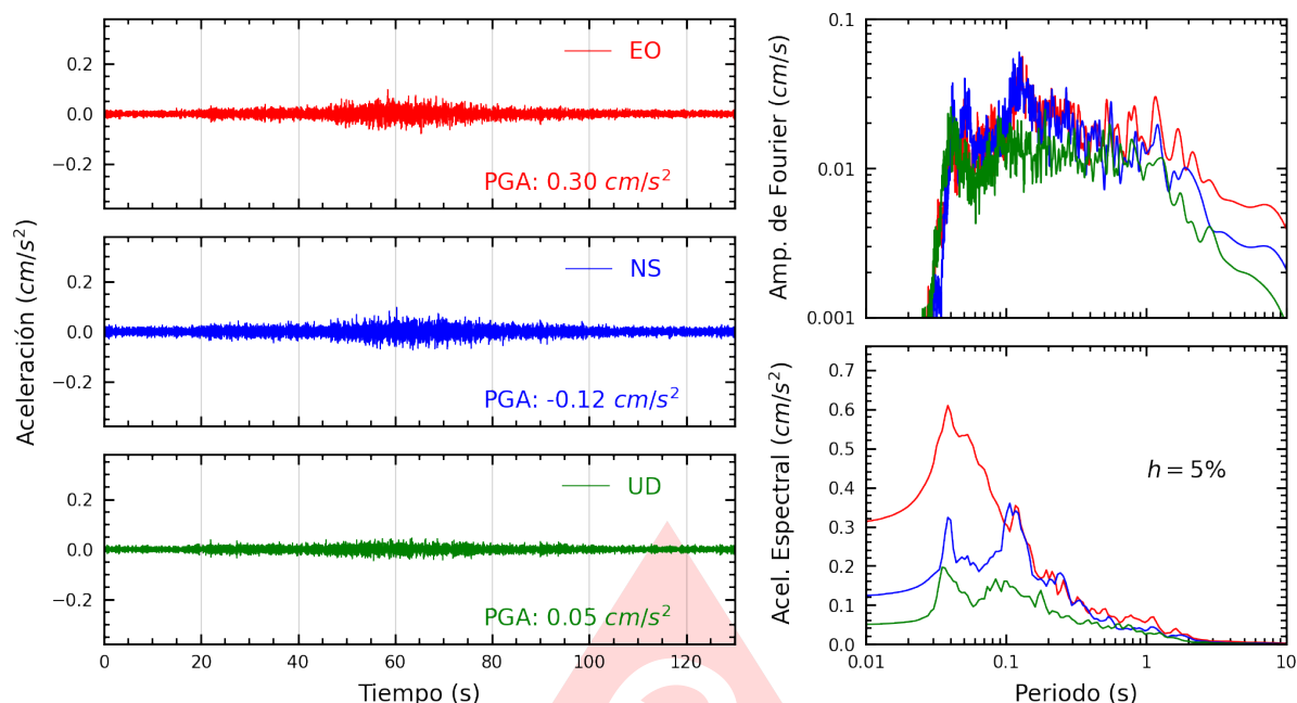
Figura A.11: Registros tiempo-historia, espectros de Fourier y de respuesta en las direcciones EO, NS y vertical de la estación ATARJ. Sismo de Pisco, Pisco - Ica del 2025-08-11, 06:41:24 (Hora local)
