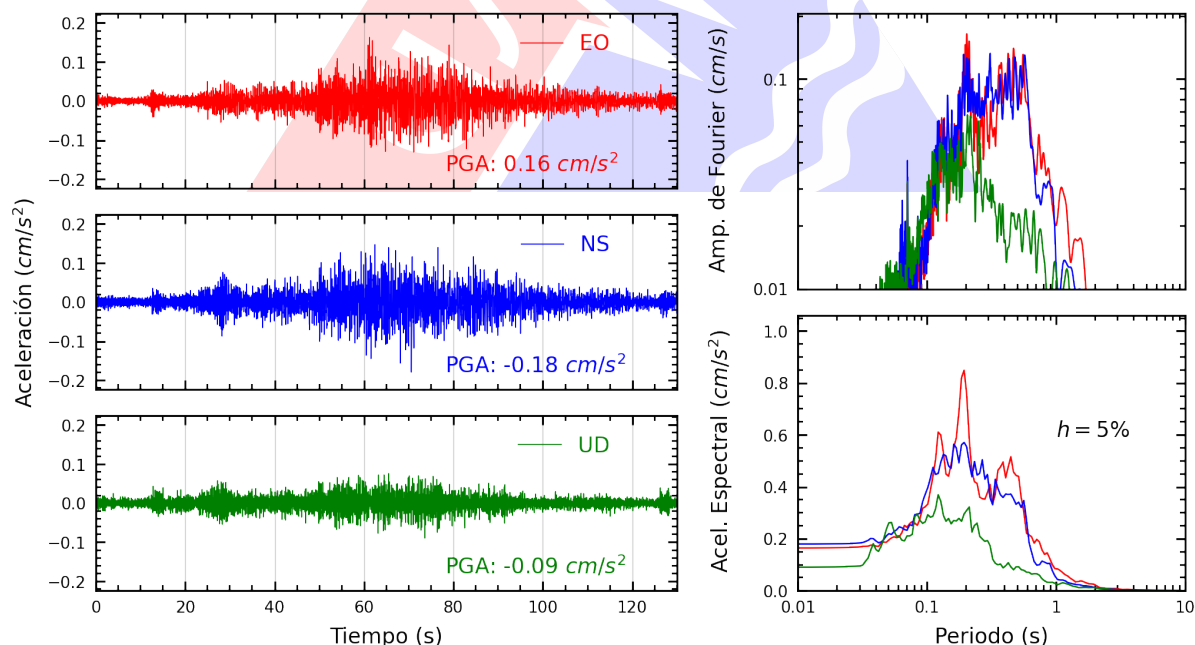
Figura A.18: Registros tiempo-historia, espectros de Fourier y de respuesta en las direcciones EO, NS y vertical de la estación VHAYA. Sismo de Pisco, Pisco - Ica del 2025-08-11, 06:41:24 (Hora local)
