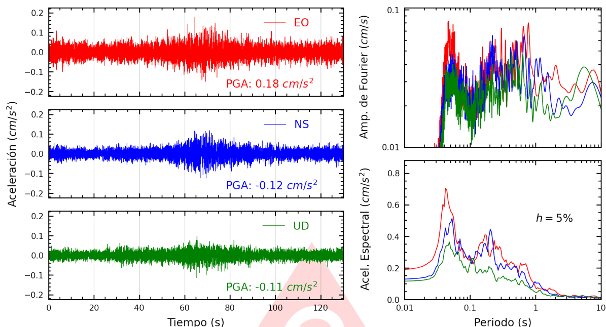
Figura A.17: Registros tiempo-historia, espectros de Fourier y de respuesta en las direcciones EO, NS y vertical de la estación INICT. Sismo de Pisco, Pisco - Ica del 2025-08-11, 06:41:24 (Hora local)
