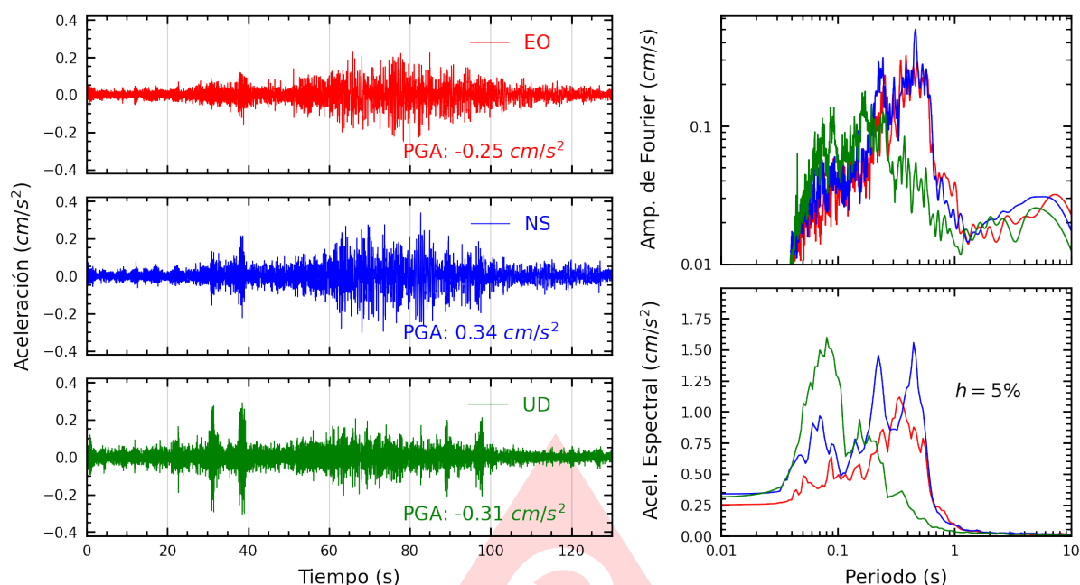
Figura A.9: Registros tiempo-historia, espectros de Fourier y de respuesta en las direcciones EO, NS y vertical de la estación MDPP. Sismo de Pisco, Pisco - Ica del 2025-08-11, 06:41:24 (Hora local)
