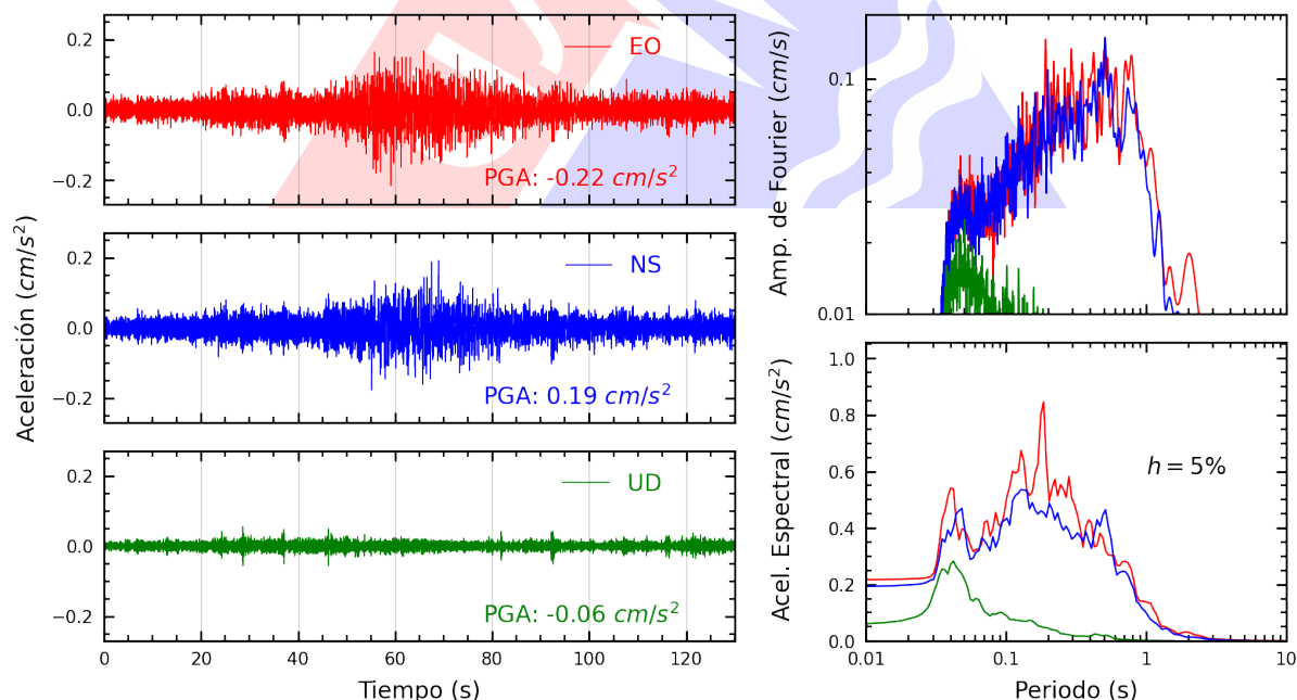
Figura A.16: Registros tiempo-historia, espectros de Fourier y de respuesta en las direcciones EO, NS y vertical de la estación UCVAT. Sismo de Pisco, Pisco - Ica del 2025-08-11, 06:41:24 (Hora local)
