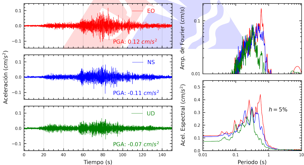
Figura A.24: Registros tiempo-historia, espectros de Fourier y de respuesta en las direcciones EO, NS y vertical de la estación CARAL. Sismo de Pisco, Pisco - Ica del 2025-08-11, 06:41:24 (Hora local)
