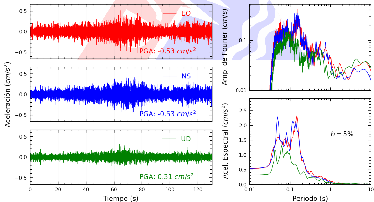
Figura A.4: Registros tiempo-historia, espectros de Fourier y de respuesta en las direcciones EO, NS y vertical de la estación USILM. Sismo de Pisco, Pisco - Ica del 2025-08-11, 06:41:24 (Hora local)
