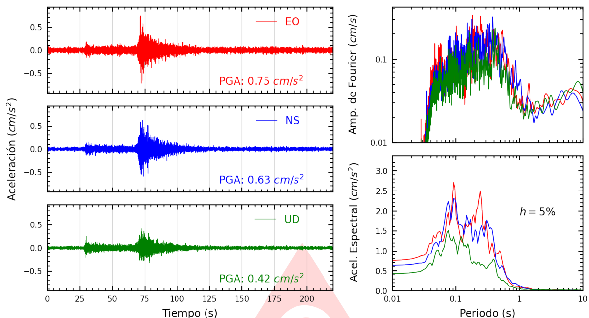
Figura A.45: Registros tiempo-historia, espectros de Fourier y de respuesta en las direcciones EO, NS y vertical de la estación INICT. Sismo de Chimbote, Santa - Ancash del 2025-08-12, 19:54:30 (Hora local)
