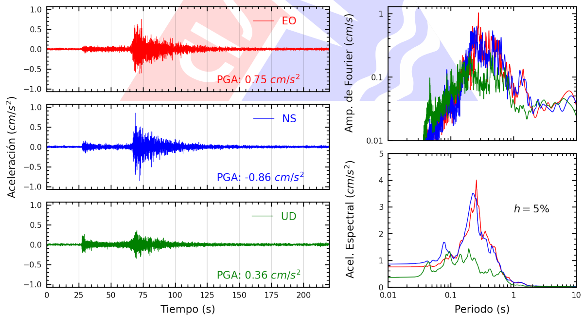
Figura A.40: Registros tiempo-historia, espectros de Fourier y de respuesta en las direcciones EO, NS y vertical de la estación DSMI. Sismo de Chimbote, Santa - Ancash del 2025-08-12, 19:54:30 (Hora local)
