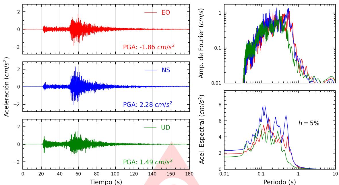
Figura A.11: Registros tiempo-historia, espectros de Fourier y de respuesta en las direcciones EO, NS y vertical de la estación CARAL. Sismo de Chimbote, Santa - Ancash del 2025-08-12, 19:54:30 (Hora local)
