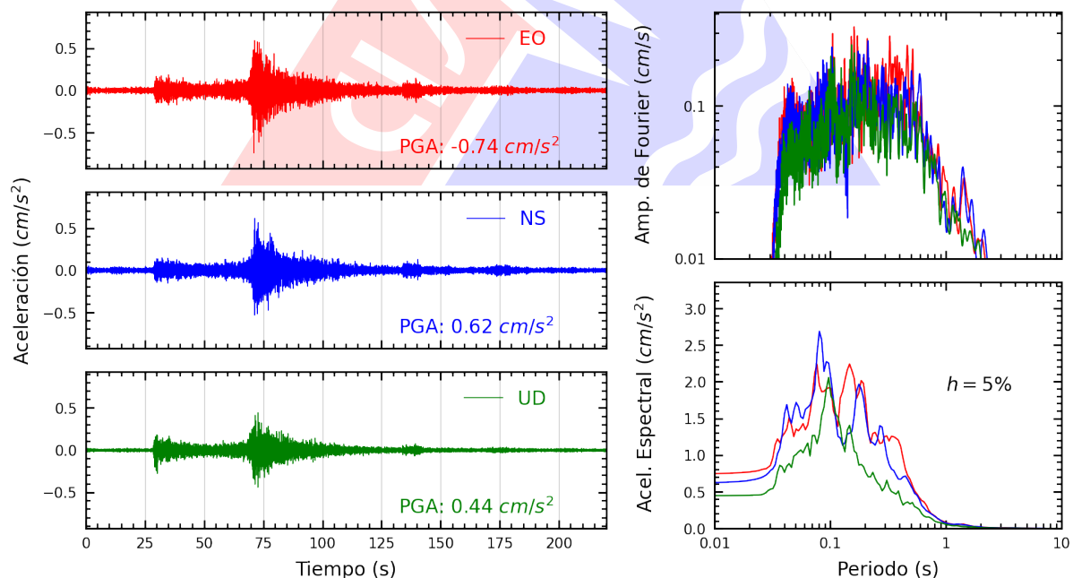
Figura A.46: Registros tiempo-historia, espectros de Fourier y de respuesta en las direcciones EO, NS y vertical de la estación BORJA. Sismo de Chimbote, Santa - Ancash del 2025-08-12, 19:54:30 (Hora local)
