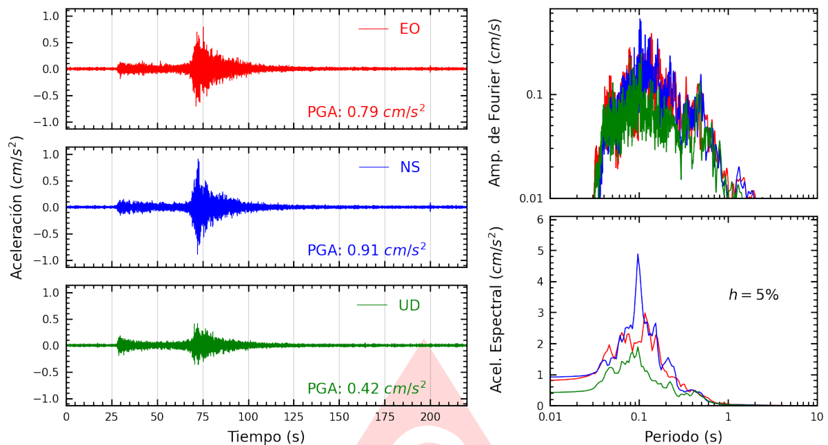
Figura A.39: Registros tiempo-historia, espectros de Fourier y de respuesta en las direcciones EO, NS y vertical de la estación ATARJ. Sismo de Chimbote, Santa - Ancash del 2025-08-12, 19:54:30 (Hora local)
