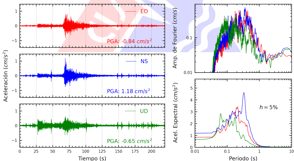
Figura A.30: Registros tiempo-historia, espectros de Fourier y de respuesta en las direcciones EO, NS y vertical de la estación RAMON. Sismo de Chimbote, Santa - Ancash del 2025-08-12, 19:54:30 (Hora local)
