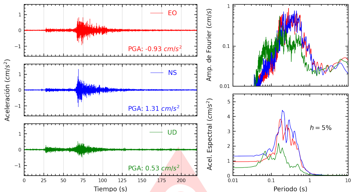
Figura A.27: Registros tiempo-historia, espectros de Fourier y de respuesta en las direcciones EO, NS y vertical de la estación ACAPU. Sismo de Chimbote, Santa - Ancash del 2025-08-12, 19:54:30 (Hora local)
