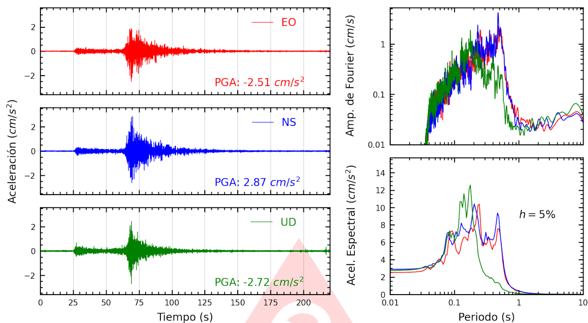
Figura A.7: Registros tiempo-historia, espectros de Fourier y de respuesta en las direcciones EO, NS y vertical de la estación MDPP. Sismo de Chimbote, Santa - Ancash del 2025-08-12, 19:54:30 (Hora local)
