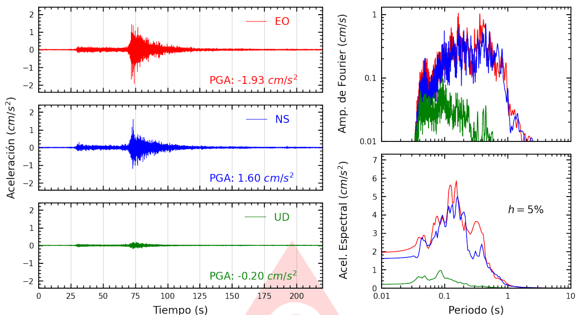
Figura A.17: Registros tiempo-historia, espectros de Fourier y de respuesta en las direcciones EO, NS y vertical de la estación UCVAT. Sismo de Chimbote, Santa - Ancash del 2025-08-12, 19:54:30 (Hora local)
