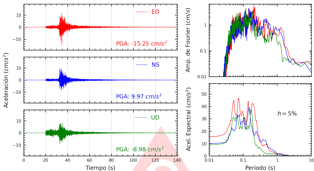
Figura A.3: Registros tiempo-historia, espectros de Fourier y de respuesta en las direcciones EO, NS y vertical de la estación UPAOT. Sismo de Chimbote, Santa - Ancash del 2025-08-12, 19:54:30 (Hora local)
