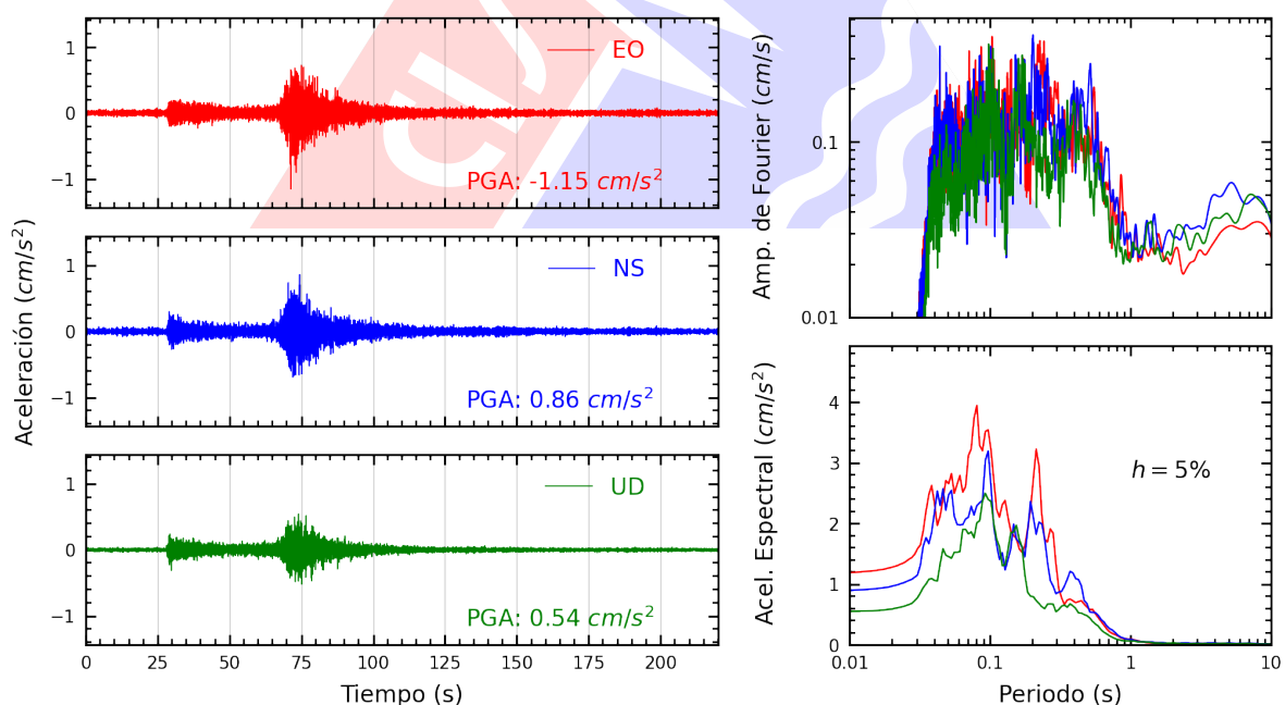
Figura A.32: Registros tiempo-historia, espectros de Fourier y de respuesta en las direcciones EO, NS y vertical de la estación CEPRE. Sismo de Chimbote, Santa - Ancash del 2025-08-12, 19:54:30 (Hora local)
