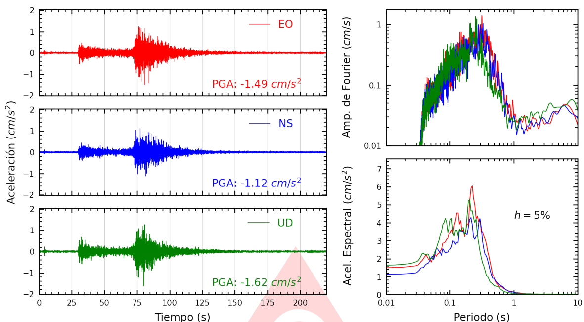
Figura A.21: Registros tiempo-historia, espectros de Fourier y de respuesta en las direcciones EO, NS y vertical de la estación SOVES. Sismo de Chimbote, Santa - Ancash del 2025-08-12, 19:54:30 (Hora local)
