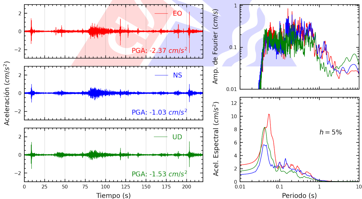
Figura A.10: Registros tiempo-historia, espectros de Fourier y de respuesta en las direcciones EO, NS y vertical de la estación PRADO. Sismo de Chimbote, Santa - Ancash del 2025-08-12, 19:54:30 (Hora local)
