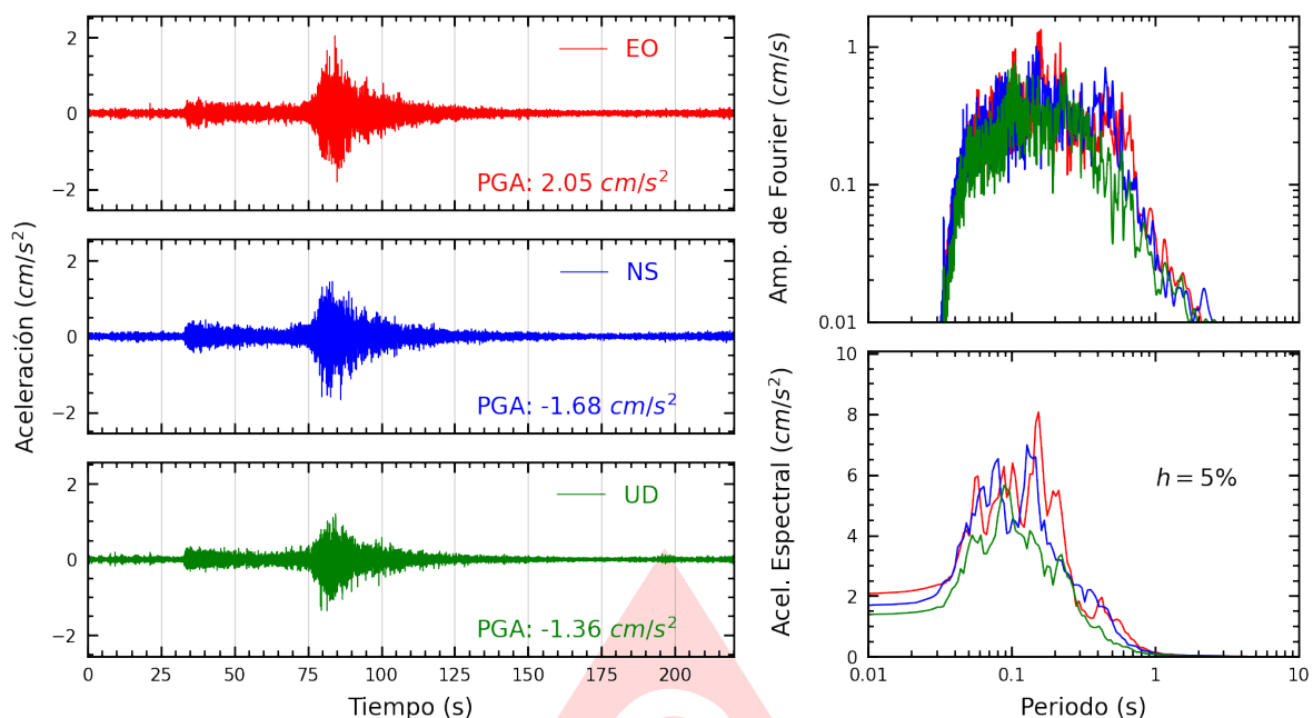
Figura A.15: Registros tiempo-historia, espectros de Fourier y de respuesta en las direcciones EO, NS y vertical de la estación PHERM. Sismo de Chimbote, Santa - Ancash del 2025-08-12, 19:54:30 (Hora local)
