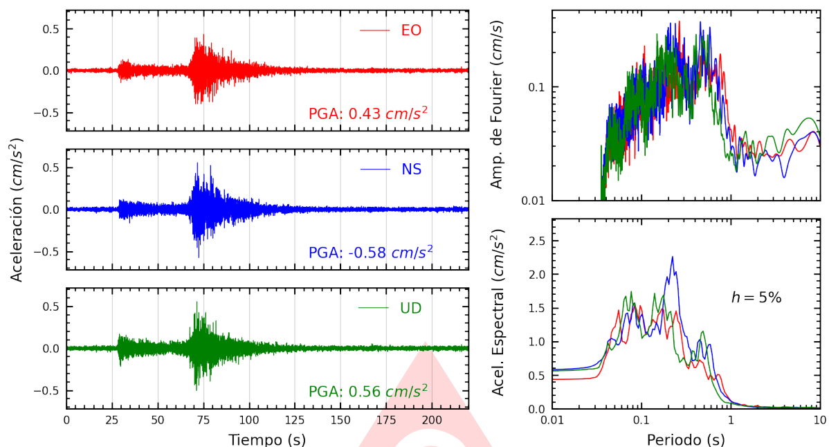
Figura A.51: Registros tiempo-historia, espectros de Fourier y de respuesta en las direcciones EO, NS y vertical de la estación UNFV. Sismo de Chimbote, Santa - Ancash del 2025-08-12, 19:54:30 (Hora local)
