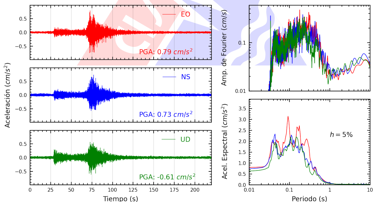
Figura A.42: Registros tiempo-historia, espectros de Fourier y de respuesta en las direcciones EO, NS y vertical de la estación USMP. Sismo de Chimbote, Santa - Ancash del 2025-08-12, 19:54:30 (Hora local)
