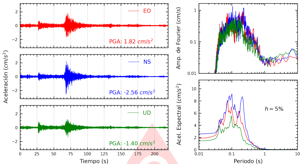
Figura A.9: Registros tiempo-historia, espectros de Fourier y de respuesta en las direcciones EO, NS y vertical de la estación INDEP. Sismo de Chimbote, Santa - Ancash del 2025-08-12, 19:54:30 (Hora local)
