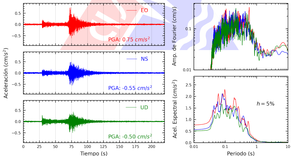
Figura A.44: Registros tiempo-historia, espectros de Fourier y de respuesta en las direcciones EO, NS y vertical de la estación SERVI. Sismo de Chimbote, Santa - Ancash del 2025-08-12, 19:54:30 (Hora local)
