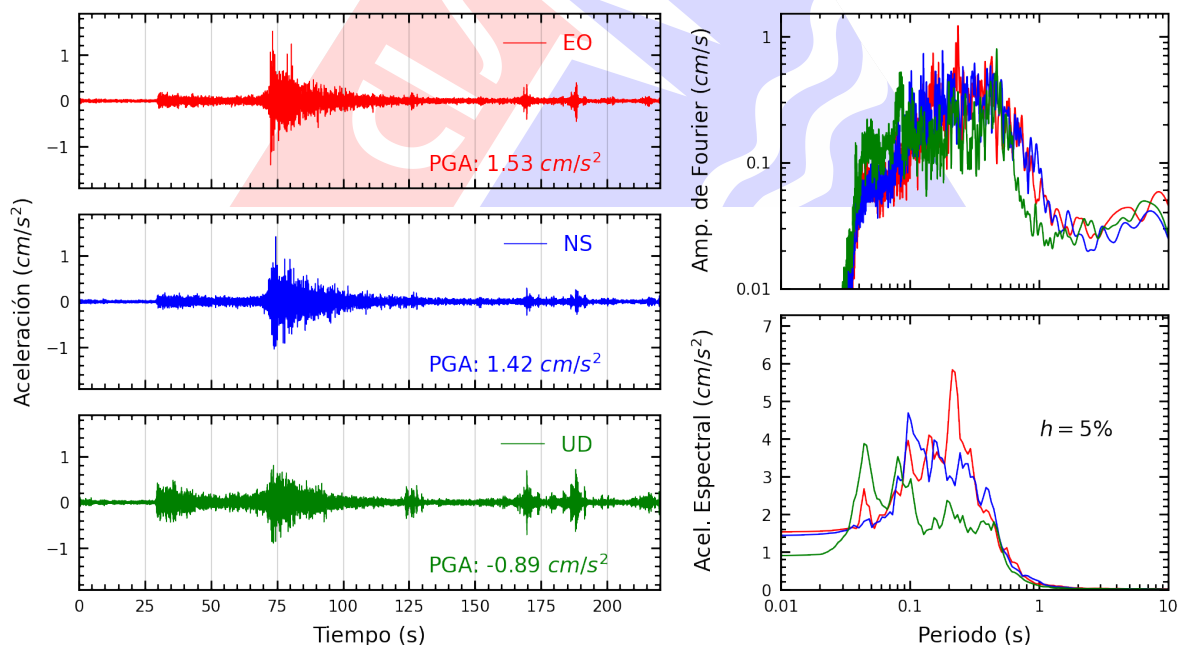
Figura A.22: Registros tiempo-historia, espectros de Fourier y de respuesta en las direcciones EO, NS y vertical de la estación SOCHO. Sismo de Chimbote, Santa - Ancash del 2025-08-12, 19:54:30 (Hora local)
