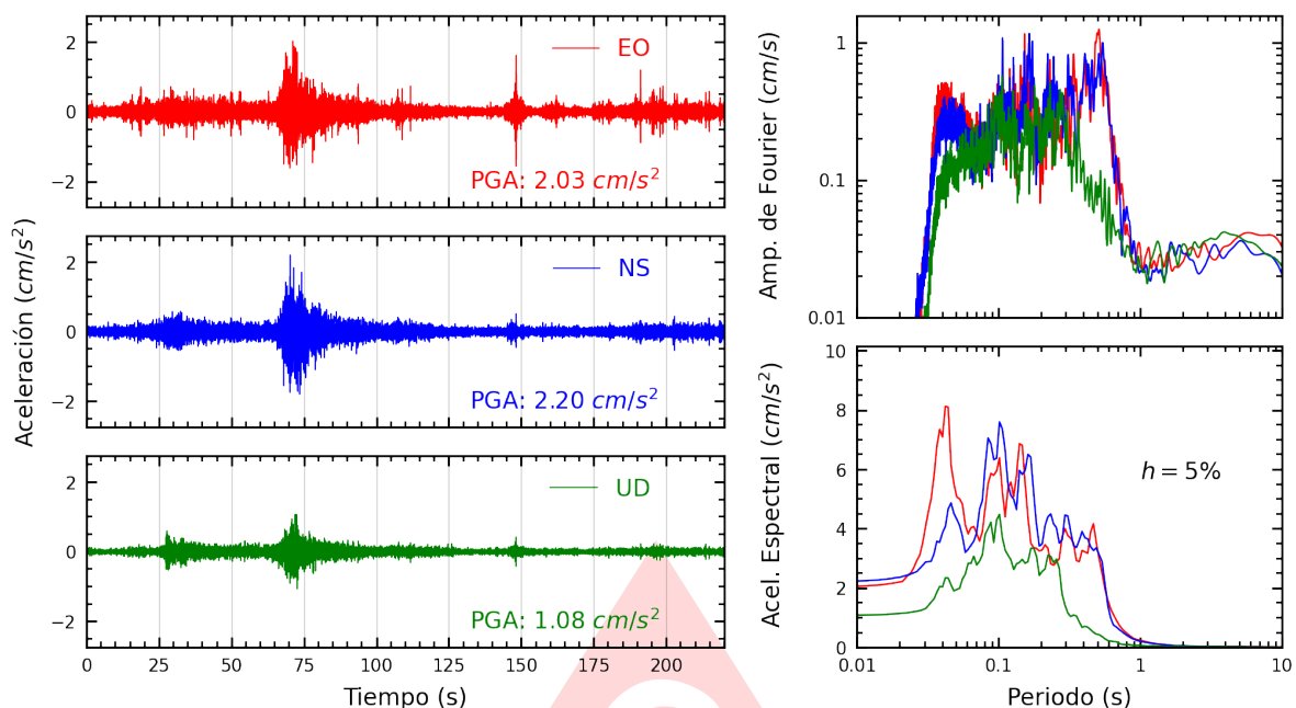
Figura A.13: Registros tiempo-historia, espectros de Fourier y de respuesta en las direcciones EO, NS y vertical de la estación OLIVO. Sismo de Chimbote, Santa - Ancash del 2025-08-12, 19:54:30 (Hora local)
