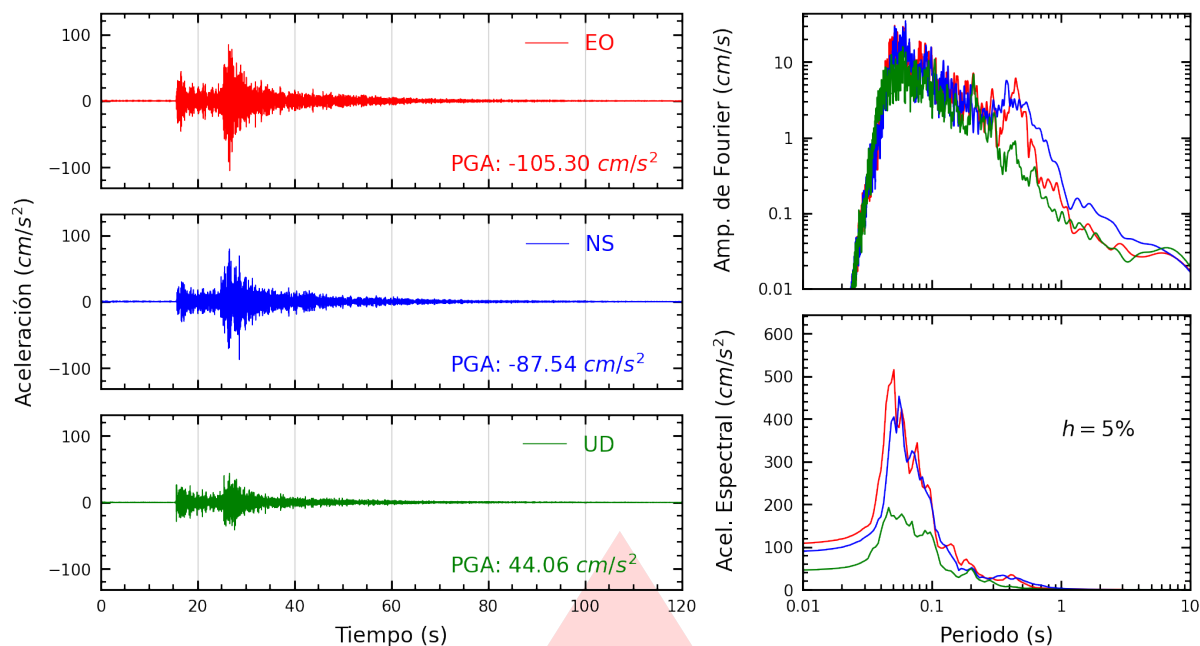
Figura A.1: Registros tiempo-historia, espectros de Fourier y de respuesta en las direcciones EO, NS y vertical de la estación USP. Sismo de Chimbote, Santa - Ancash del 2025-08-12, 19:54:30 (Hora local)
