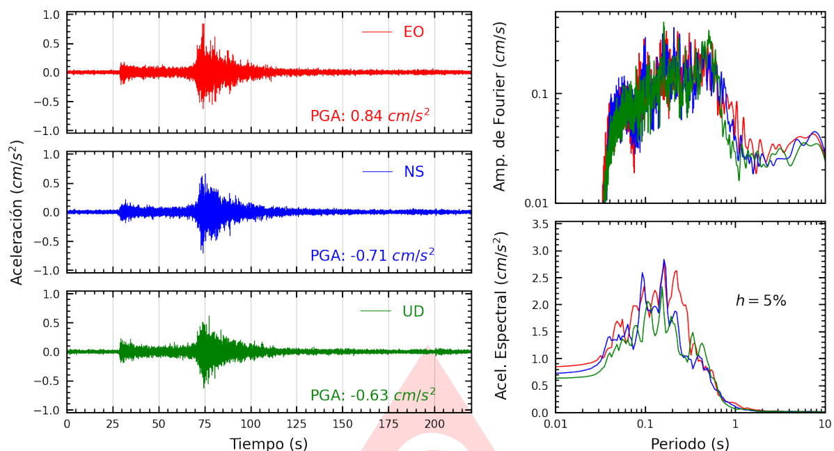
Figura A.41: Registros tiempo-historia, espectros de Fourier y de respuesta en las direcciones EO, NS y vertical de la estación IMCA. Sismo de Chimbote, Santa - Ancash del 2025-08-12, 19:54:30 (Hora local)
