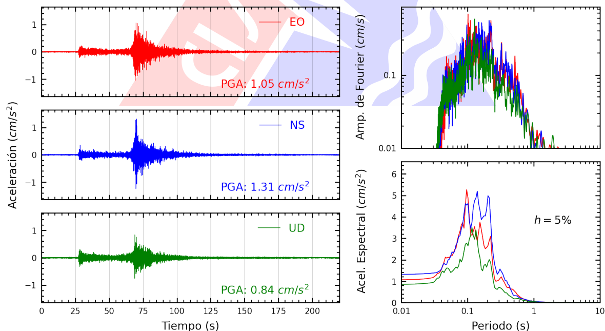
Figura A.28: Registros tiempo-historia, espectros de Fourier y de respuesta en las direcciones EO, NS y vertical de la estación JALV2. Sismo de Chimbote, Santa - Ancash del 2025-08-12, 19:54:30 (Hora local)
