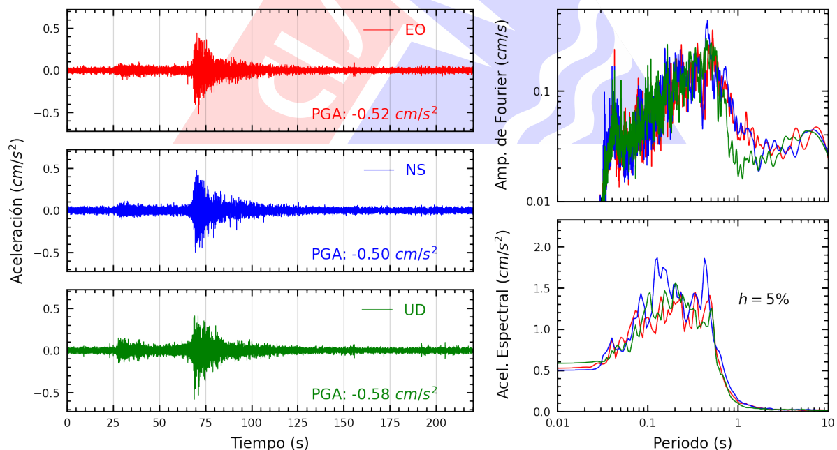
Figura A.50: Registros tiempo-historia, espectros de Fourier y de respuesta en las direcciones EO, NS y vertical de la estación BONDY. Sismo de Chimbote, Santa - Ancash del 2025-08-12, 19:54:30 (Hora local)
