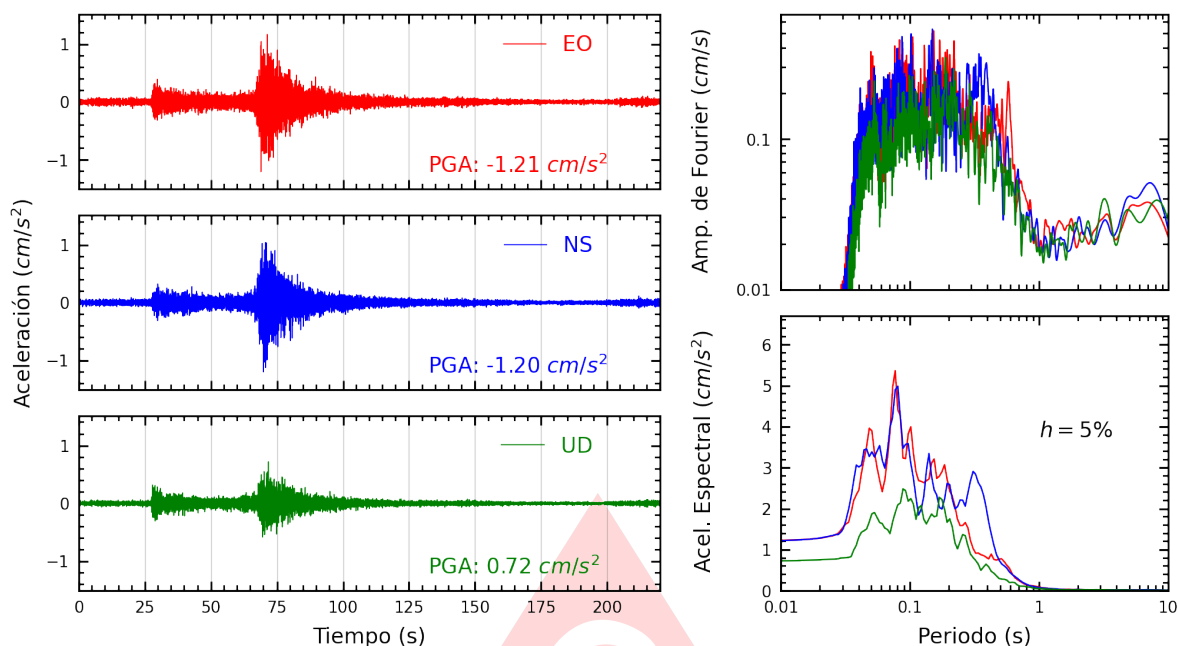
Figura A.29: Registros tiempo-historia, espectros de Fourier y de respuesta en las direcciones EO, NS y vertical de la estación FICPE. Sismo de Chimbote, Santa - Ancash del 2025-08-12, 19:54:30 (Hora local)
