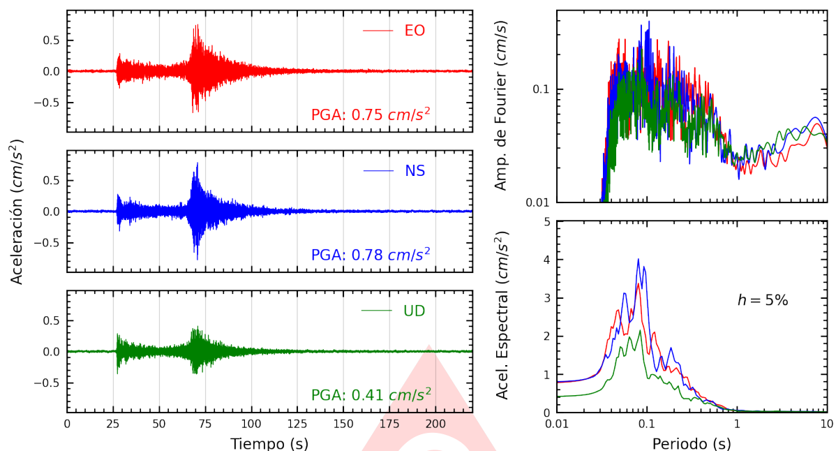
Figura A.43: Registros tiempo-historia, espectros de Fourier y de respuesta en las direcciones EO, NS y vertical de la estación UCSS. Sismo de Chimbote, Santa - Ancash del 2025-08-12, 19:54:30 (Hora local)
