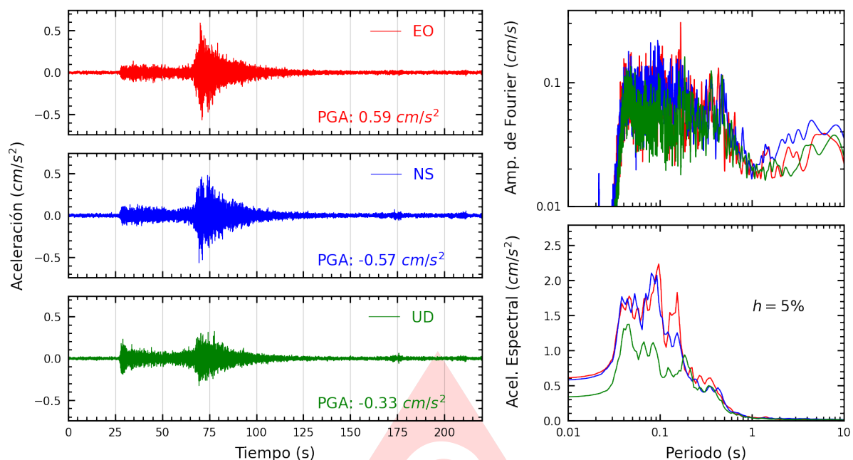
Figura A.49: Registros tiempo-historia, espectros de Fourier y de respuesta en las direcciones EO, NS y vertical de la estación SJLCE. Sismo de Chimbote, Santa - Ancash del 2025-08-12, 19:54:30 (Hora local)
