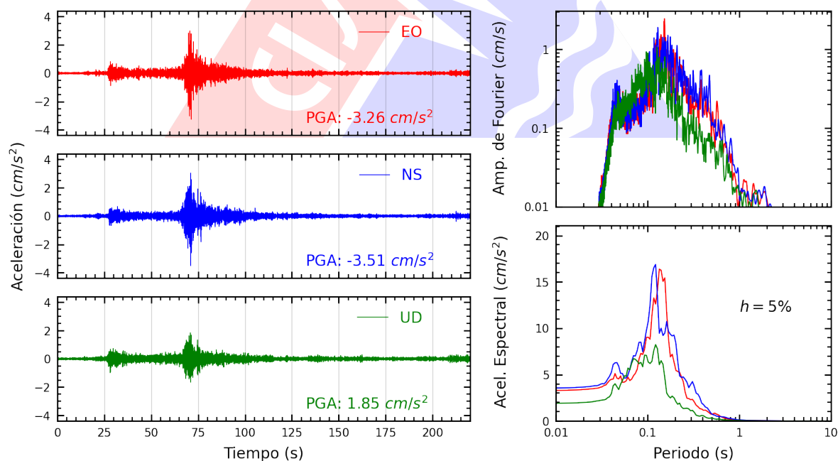
Figura A.4: Registros tiempo-historia, espectros de Fourier y de respuesta en las direcciones EO, NS y vertical de la estación CARAB. Sismo de Chimbote, Santa - Ancash del 2025-08-12, 19:54:30 (Hora local)
