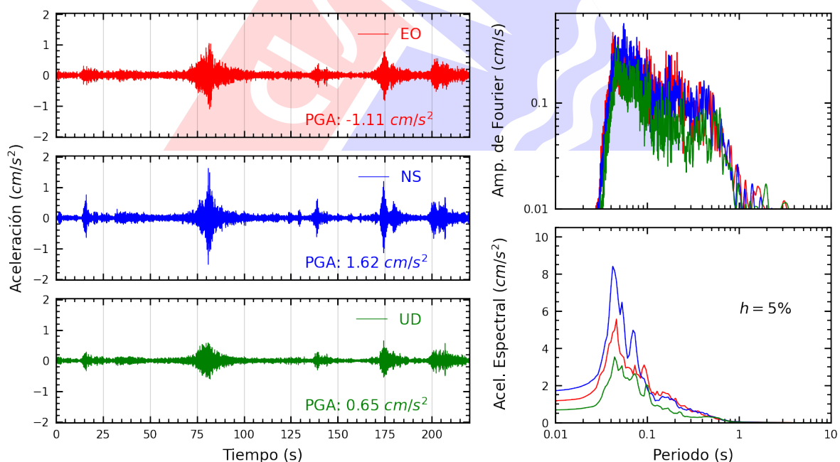
Figura A.20: Registros tiempo-historia, espectros de Fourier y de respuesta en las direcciones EO, NS y vertical de la estación PACHA. Sismo de Chimbote, Santa - Ancash del 2025-08-12, 19:54:30 (Hora local)
