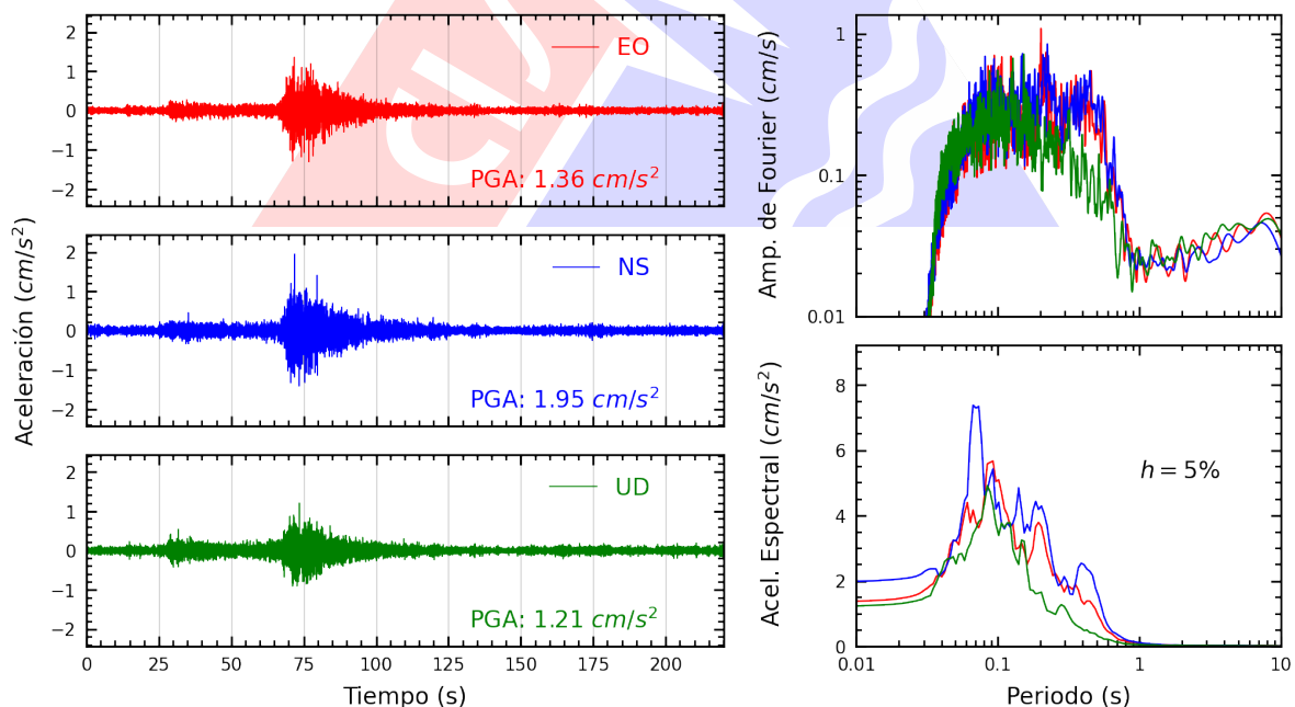
Figura A.16: Registros tiempo-historia, espectros de Fourier y de respuesta en las direcciones EO, NS y vertical de la estación SJLSC. Sismo de Chimbote, Santa - Ancash del 2025-08-12, 19:54:30 (Hora local)
