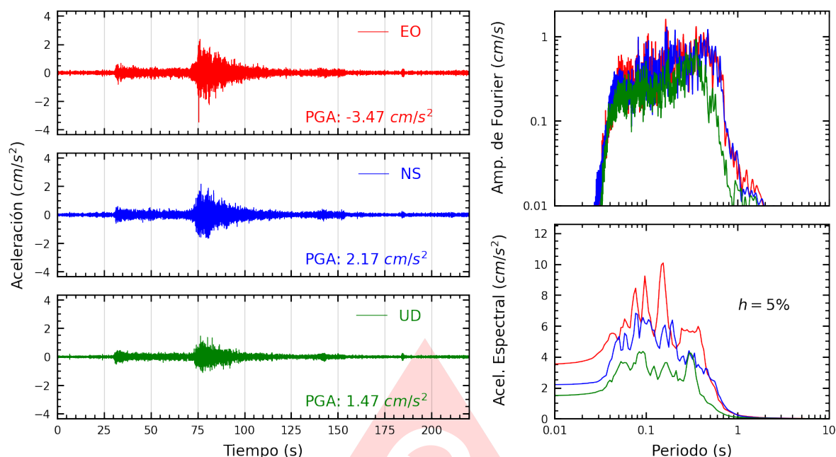
Figura A.5: Registros tiempo-historia, espectros de Fourier y de respuesta en las direcciones EO, NS y vertical de la estación UNTEL. Sismo de Chimbote, Santa - Ancash del 2025-08-12, 19:54:30 (Hora local)
