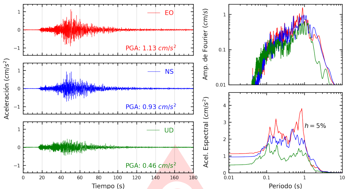
Figura A.33: Registros tiempo-historia, espectros de Fourier y de respuesta en las direcciones EO, NS y vertical de la estación UNC. Sismo de Chimbote, Santa - Ancash del 2025-08-12, 19:54:30 (Hora local)
