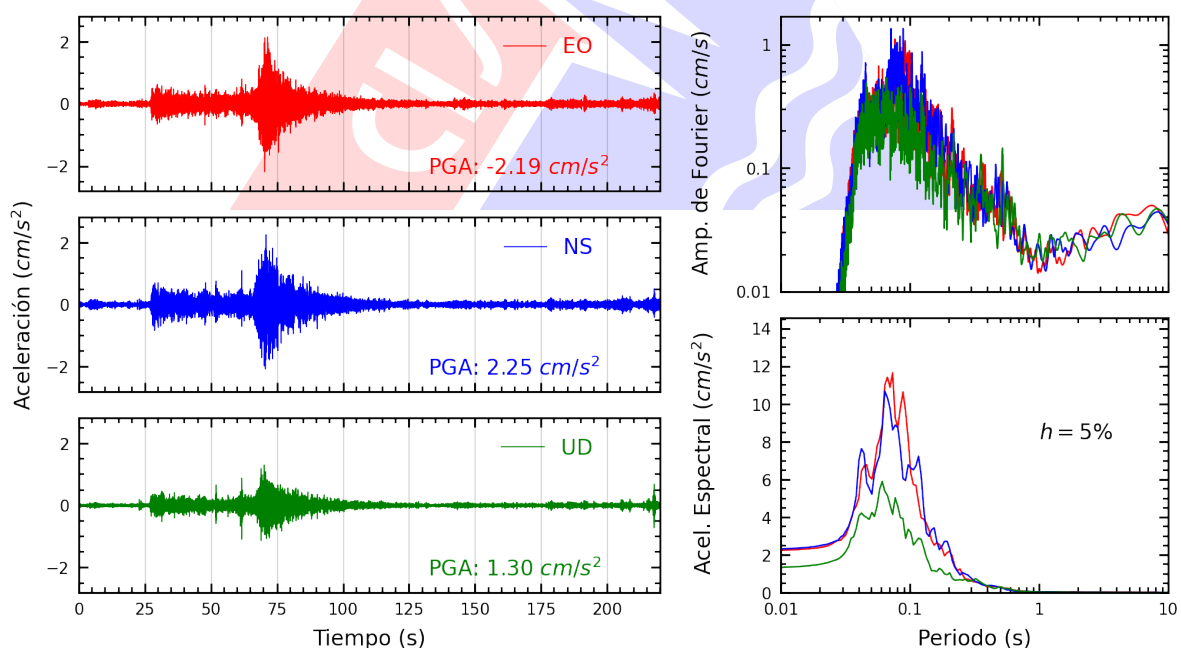
Figura A.12: Registros tiempo-historia, espectros de Fourier y de respuesta en las direcciones EO, NS y vertical de la estación JOSEO. Sismo de Chimbote, Santa - Ancash del 2025-08-12, 19:54:30 (Hora local)
