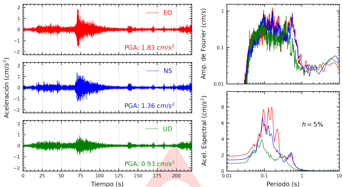
Figura A.19: Registros tiempo-historia, espectros de Fourier y de respuesta en las direcciones EO, NS y vertical de la estación SJLSV. Sismo de Chimbote, Santa - Ancash del 2025-08-12, 19:54:30 (Hora local)
