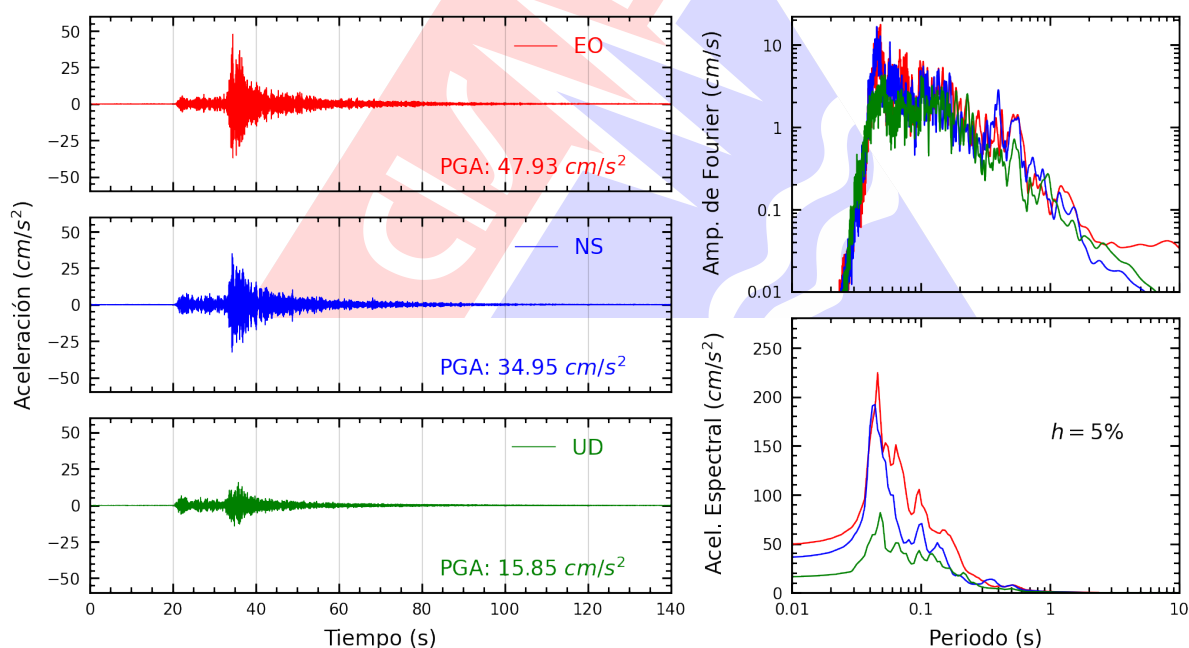
Figura A.2: Registros tiempo-historia, espectros de Fourier y de respuesta en las direcciones EO, NS y vertical de la estación SCTRU. Sismo de Chimbote, Santa - Ancash del 2025-08-12, 19:54:30 (Hora local)
