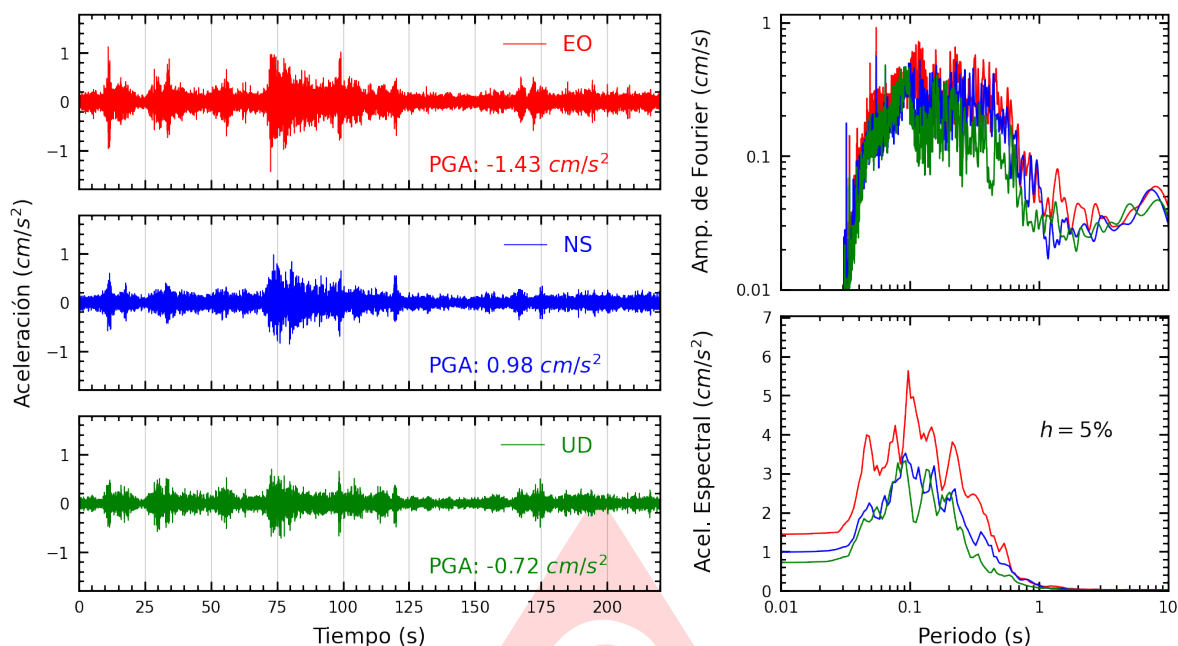
Figura A.25: Registros tiempo-historia, espectros de Fourier y de respuesta en las direcciones EO, NS y vertical de la estación SOBAR. Sismo de Chimbote, Santa - Ancash del 2025-08-12, 19:54:30 (Hora local)
