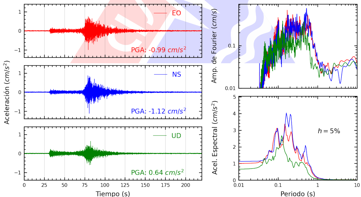
Figura A.34: Registros tiempo-historia, espectros de Fourier y de respuesta en las direcciones EO, NS y vertical de la estación USILP. Sismo de Chimbote, Santa - Ancash del 2025-08-12, 19:54:30 (Hora local)
