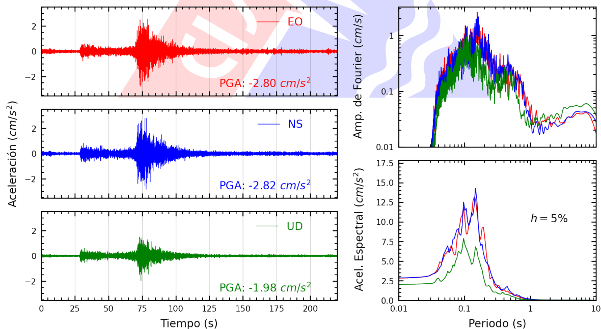
Figura A.8: Registros tiempo-historia, espectros de Fourier y de respuesta en las direcciones EO, NS y vertical de la estación USILM. Sismo de Chimbote, Santa - Ancash del 2025-08-12, 19:54:30 (Hora local)
