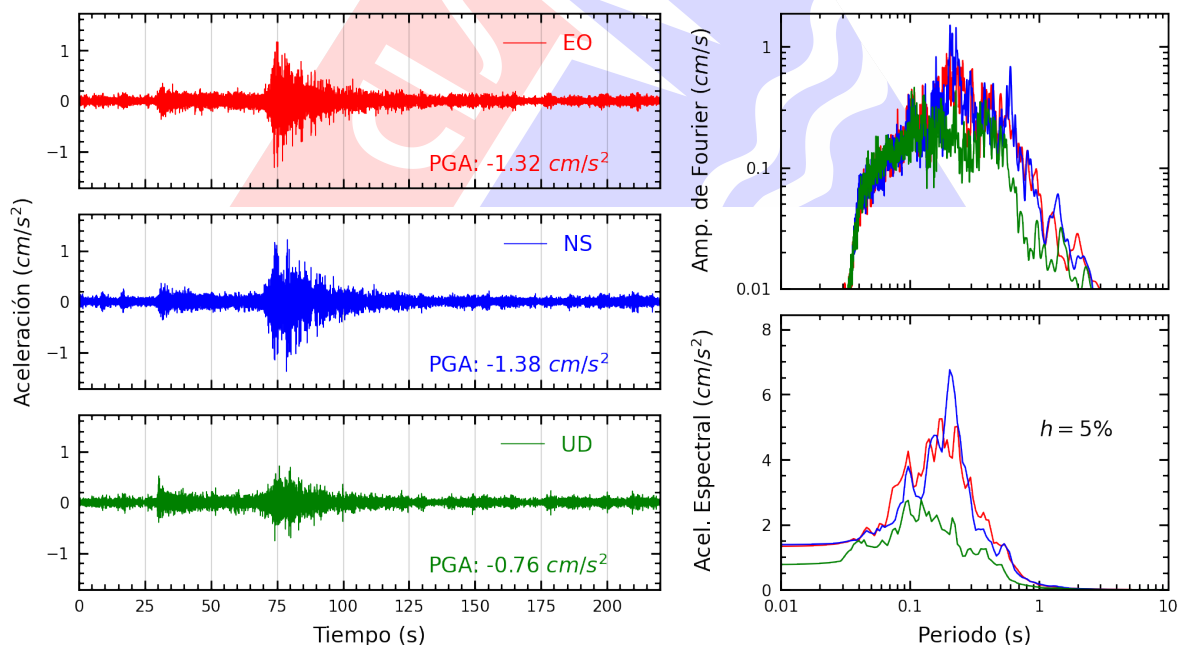
Figura A.26: Registros tiempo-historia, espectros de Fourier y de respuesta en las direcciones EO, NS y vertical de la estación SCCHO. Sismo de Chimbote, Santa - Ancash del 2025-08-12, 19:54:30 (Hora local)
