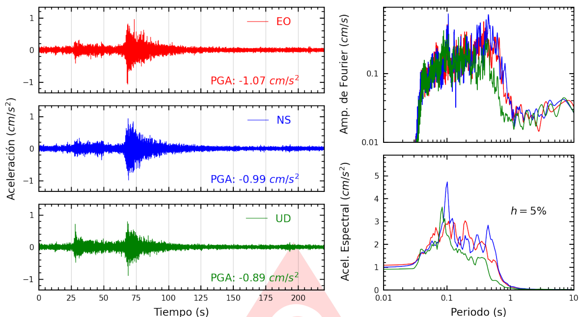
Figura A.35: Registros tiempo-historia, espectros de Fourier y de respuesta en las direcciones EO, NS y vertical de la estación MADRE. Sismo de Chimbote, Santa - Ancash del 2025-08-12, 19:54:30 (Hora local)
