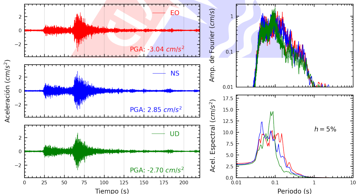
Figura A.6: Registros tiempo-historia, espectros de Fourier y de respuesta en las direcciones EO, NS y vertical de la estación SROSA. Sismo de Chimbote, Santa - Ancash del 2025-08-12, 19:54:30 (Hora local)
