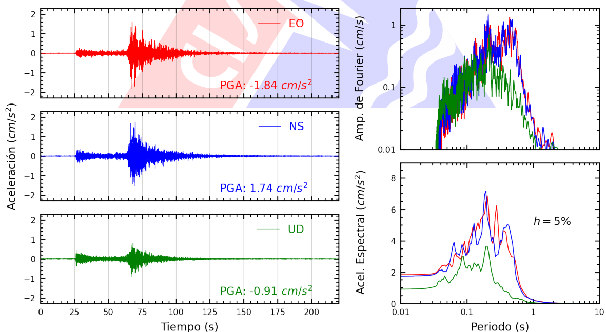
Figura A.18: Registros tiempo-historia, espectros de Fourier y de respuesta en las direcciones EO, NS y vertical de la estación VHAYA. Sismo de Chimbote, Santa - Ancash del 2025-08-12, 19:54:30 (Hora local)
