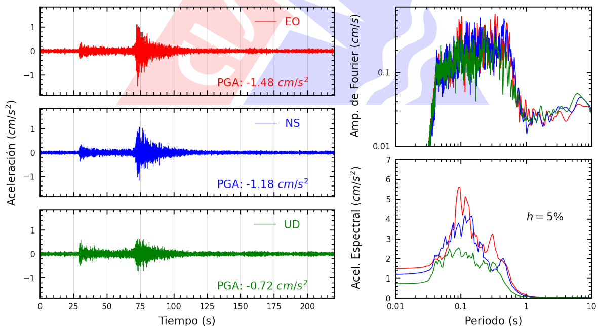
Figura A.24: Registros tiempo-historia, espectros de Fourier y de respuesta en las direcciones EO, NS y vertical de la estación URPE. Sismo de Chimbote, Santa - Ancash del 2025-08-12, 19:54:30 (Hora local)
