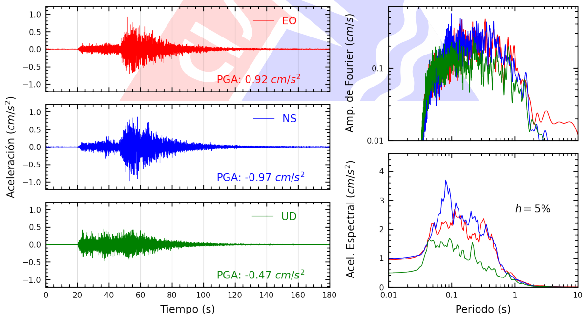
Figura A.36: Registros tiempo-historia, espectros de Fourier y de respuesta en las direcciones EO, NS y vertical de la estación SCCHI. Sismo de Chimbote, Santa - Ancash del 2025-08-12, 19:54:30 (Hora local)
