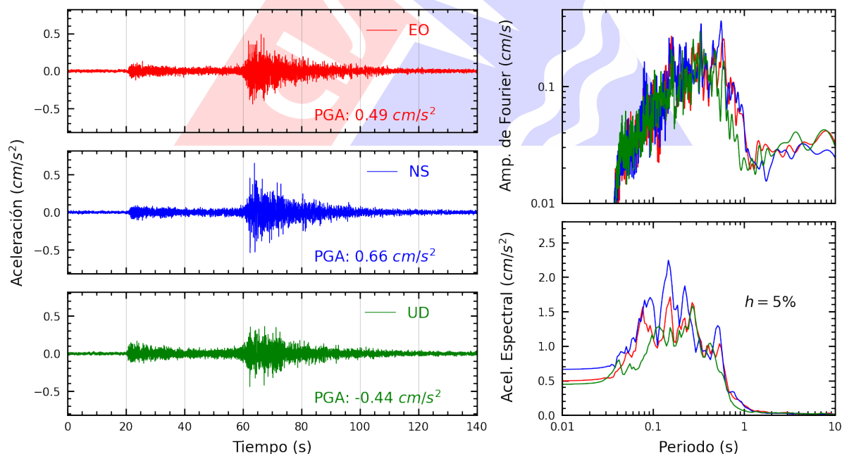
Figura A.48: Registros tiempo-historia, espectros de Fourier y de respuesta en las direcciones EO, NS y vertical de la estación UNMSM. Sismo de Chimbote, Santa - Ancash del 2025-08-12, 19:54:30 (Hora local)
