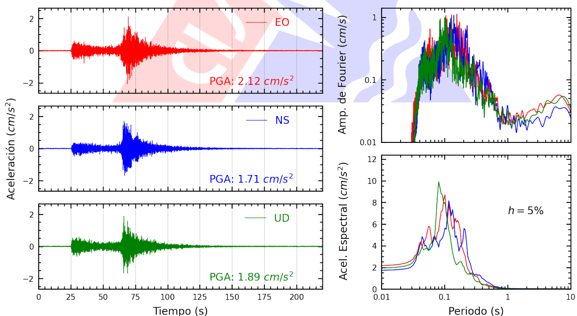
Figura A.14: Registros tiempo-historia, espectros de Fourier y de respuesta en las direcciones EO, NS y vertical de la estación AMORE. Sismo de Chimbote, Santa - Ancash del 2025-08-12, 19:54:30 (Hora local)
