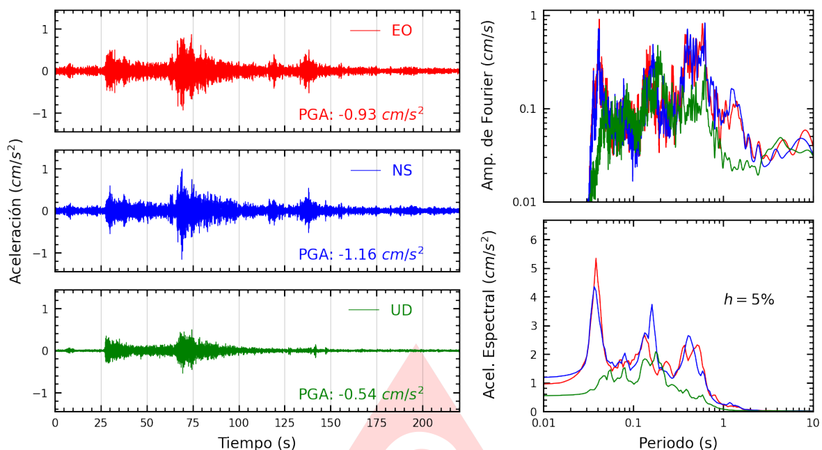
Figura A.31: Registros tiempo-historia, espectros de Fourier y de respuesta en las direcciones EO, NS y vertical de la estación DHNPE. Sismo de Chimbote, Santa - Ancash del 2025-08-12, 19:54:30 (Hora local)
