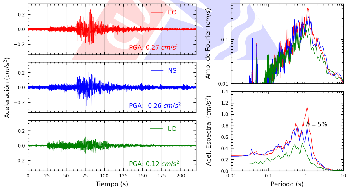
Figura A.52: Registros tiempo-historia, espectros de Fourier y de respuesta en las direcciones EO, NS y vertical de la estación UNJ. Sismo de Chimbote, Santa - Ancash del 2025-08-12, 19:54:30 (Hora local)
