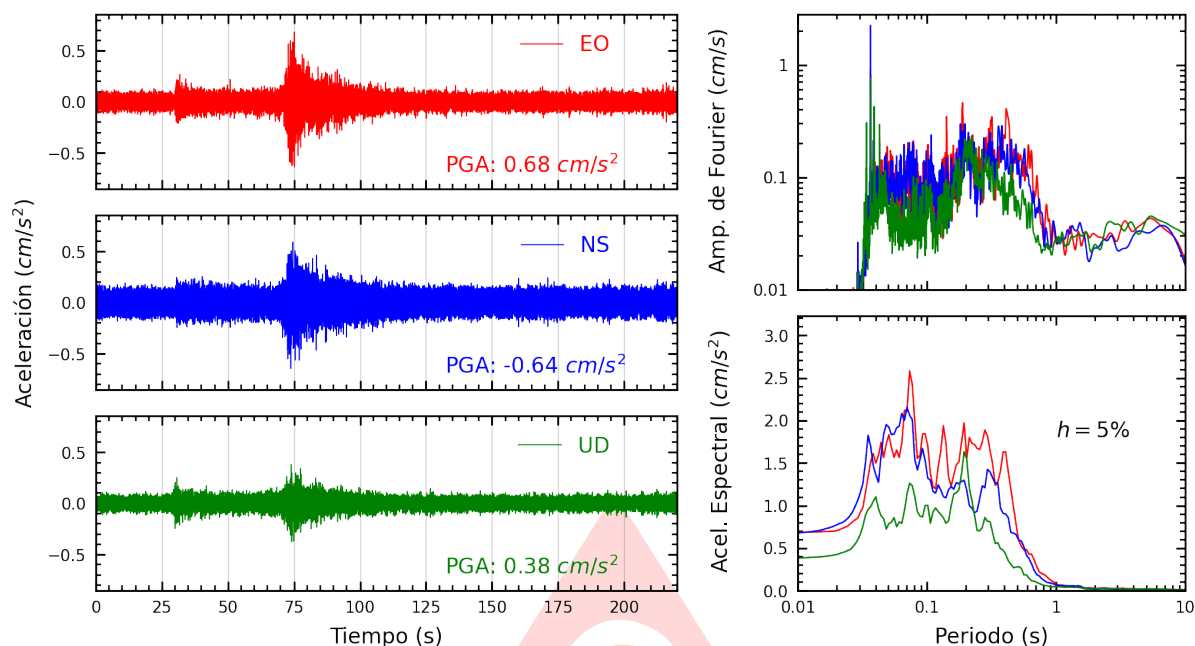
Figura A.47: Registros tiempo-historia, espectros de Fourier y de respuesta en las direcciones EO, NS y vertical de la estación UPCVI. Sismo de Chimbote, Santa - Ancash del 2025-08-12, 19:54:30 (Hora local)
