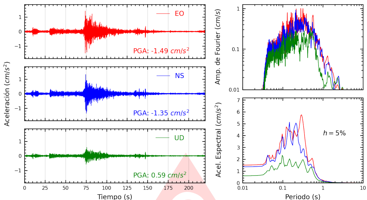
Figura A.23: Registros tiempo-historia, espectros de Fourier y de respuesta en las direcciones EO, NS y vertical de la estación BRISA. Sismo de Chimbote, Santa - Ancash del 2025-08-12, 19:54:30 (Hora local)
