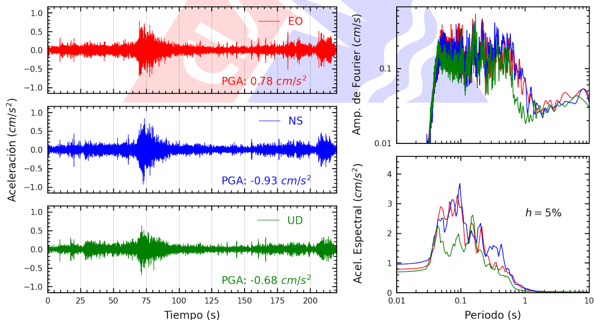
Figura A.38: Registros tiempo-historia, espectros de Fourier y de respuesta en las direcciones EO, NS y vertical de la estación UPCSM. Sismo de Chimbote, Santa - Ancash del 2025-08-12, 19:54:30 (Hora local)
