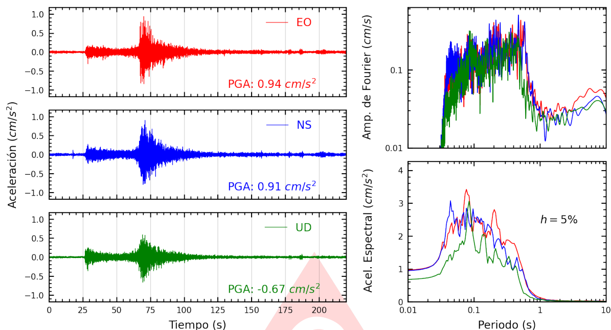
Figura A.37: Registros tiempo-historia, espectros de Fourier y de respuesta en las direcciones EO, NS y vertical de la estación COMAS. Sismo de Chimbote, Santa - Ancash del 2025-08-12, 19:54:30 (Hora local)
