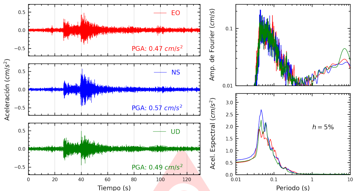
Figura A.25: Registros tiempo-historia, espectros de Fourier y de respuesta en las direcciones EO, NS y vertical de la estación URPPE. Sismo de Yungas, Canta - Lima del 2025-08-17, 08:33:57 (Hora local)
