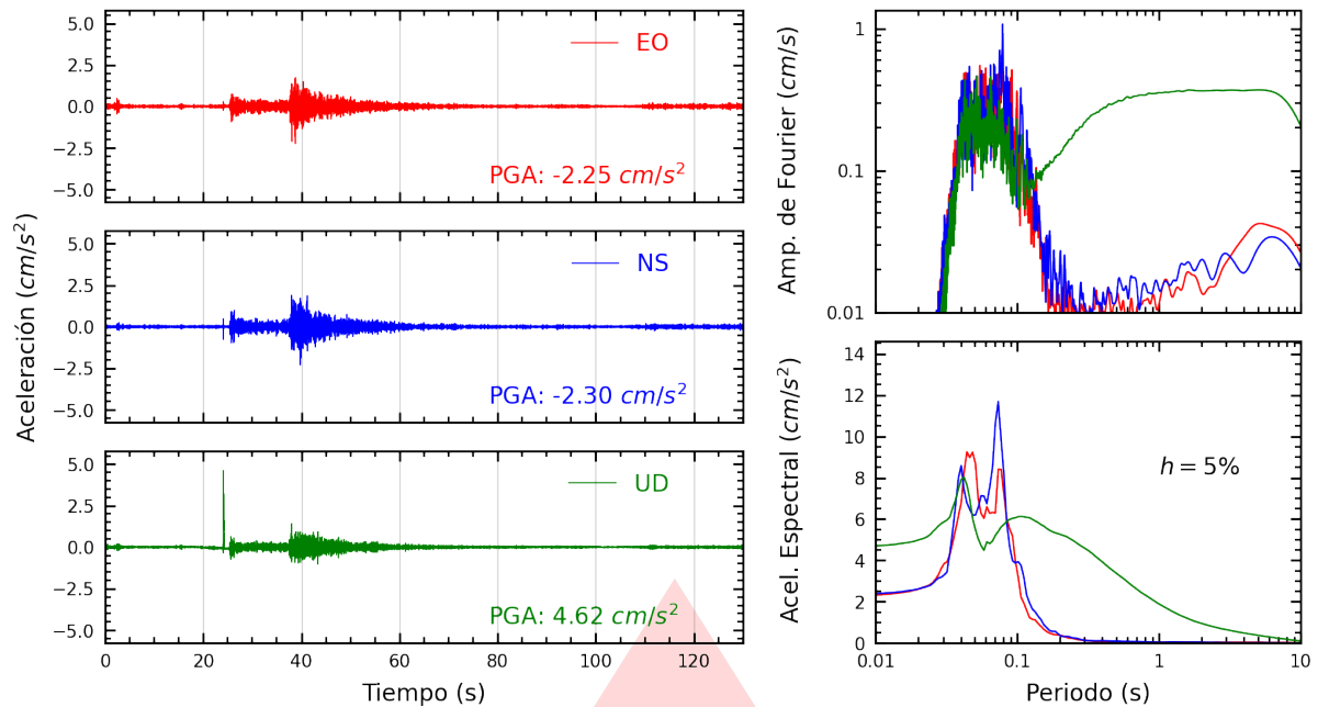
Figura A.1: Registros tiempo-historia, espectros de Fourier y de respuesta en las direcciones EO, NS y vertical de la estación JOSEO. Sismo de Yangas, Canta - Lima del 2025-08-17, 08:33:57 (Hora local)
