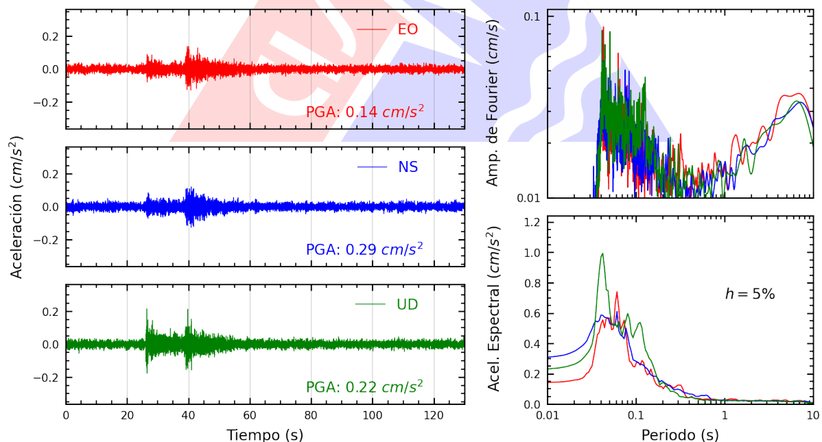
Figura A.40: Registros tiempo-historia, espectros de Fourier y de respuesta en las direcciones EO, NS y vertical de la estación BONDY. Sismo de Yungas, Canta - Lima del 2025-08-17, 08:33:57 (Hora local)
