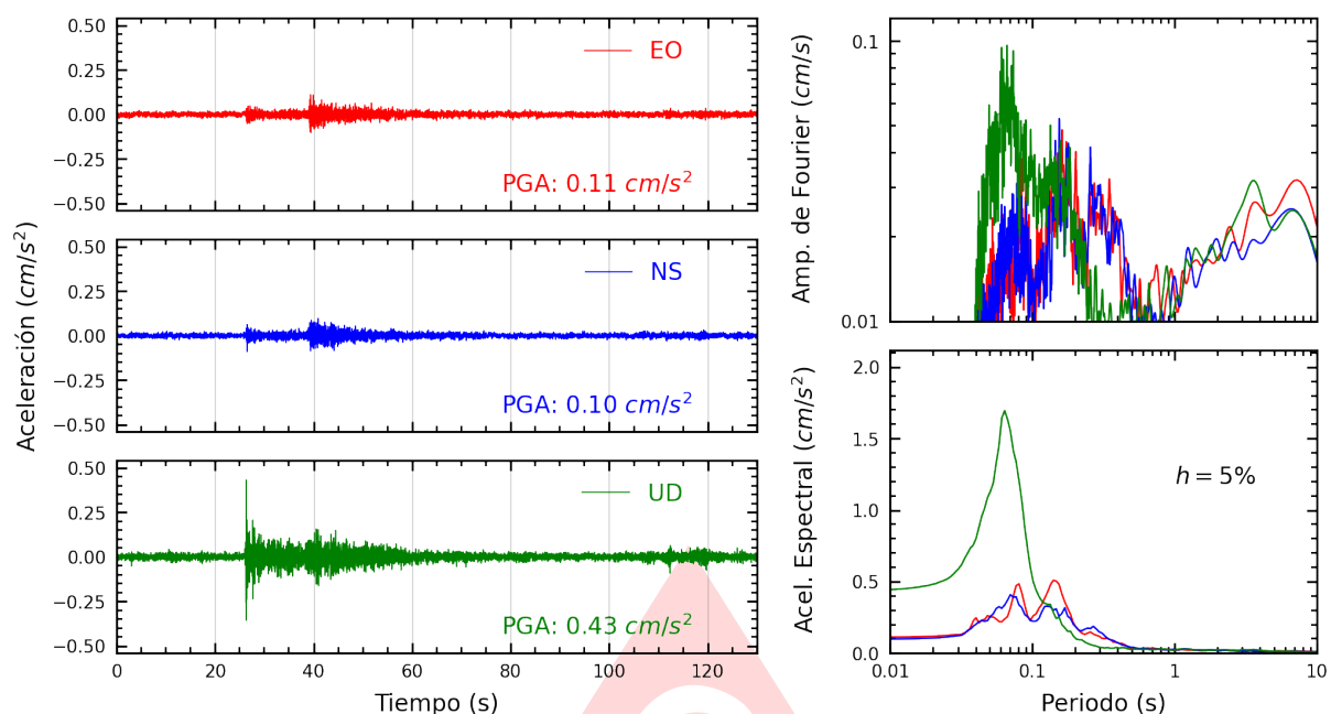
Figura A.33: Registros tiempo-historia, espectros de Fourier y de respuesta en las direcciones EO, NS y vertical de la estación ACAPU. Sismo de Yungas, Canta - Lima del 2025-08-17, 08:33:57 (Hora local)
