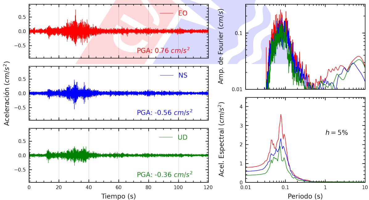
Figura A.20: Registros tiempo-historia, espectros de Fourier y de respuesta en las direcciones EO, NS y vertical de la estación SOBAR. Sismo de Yungas, Canta - Lima del 2025-08-17, 08:33:57 (Hora local)
