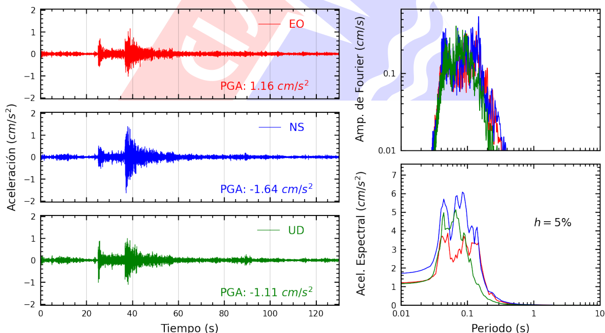
Figura A.8: Registros tiempo-historia, espectros de Fourier y de respuesta en las direcciones EO, NS y vertical de la estación CARAB. Sismo de Yungas, Canta - Lima del 2025-08-17, 08:33:57 (Hora local)
