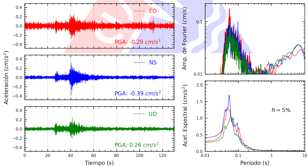
Figura A.36: Registros tiempo-historia, espectros de Fourier y de respuesta en las direcciones EO, NS y vertical de la estación INICT. Sismo de Yungas, Canta - Lima del 2025-08-17, 08:33:57 (Hora local)
