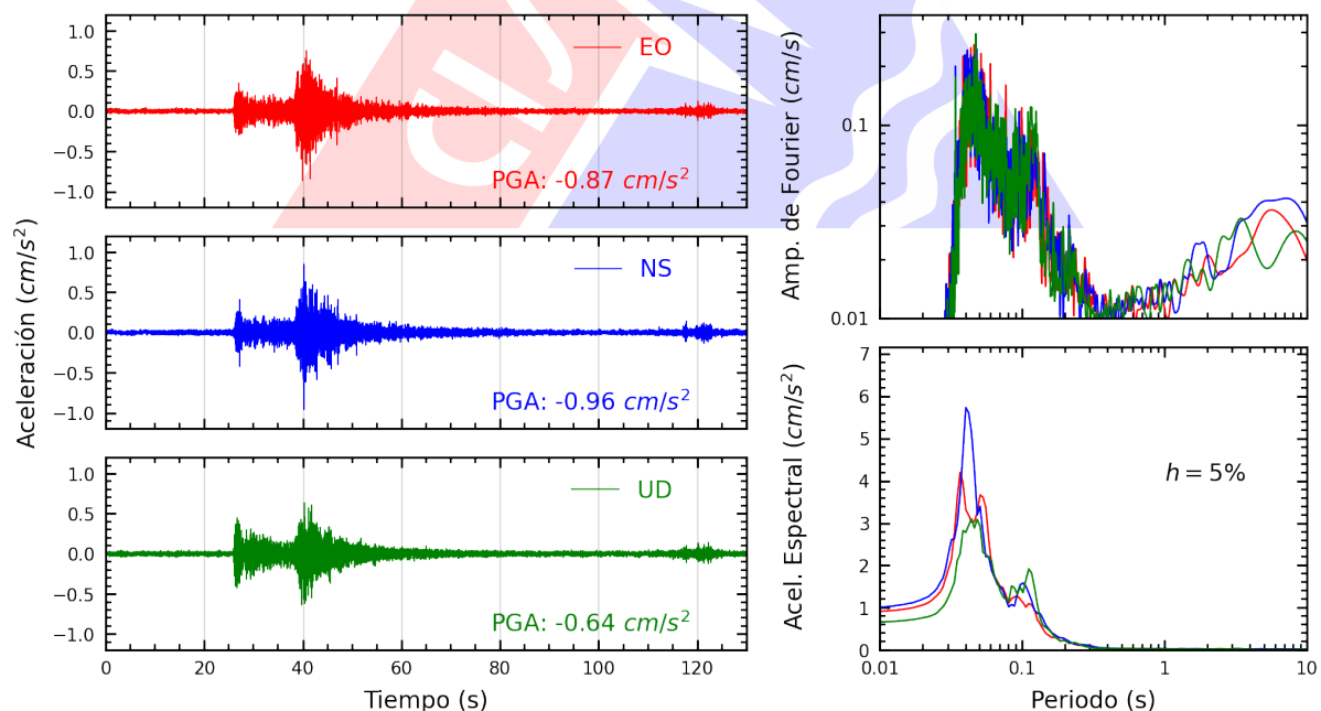
Figura A.16: Registros tiempo-historia, espectros de Fourier y de respuesta en las direcciones EO, NS y vertical de la estación USMP. Sismo de Yungas, Canta - Lima del 2025-08-17, 08:33:57 (Hora local)
