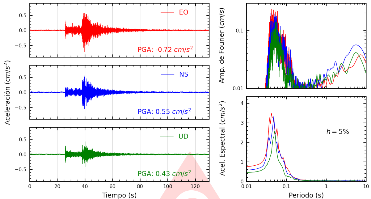
Figura A.21: Registros tiempo-historia, espectros de Fourier y de respuesta en las direcciones EO, NS y vertical de la estación UCSS. Sismo de Yungas, Canta - Lima del 2025-08-17, 08:33:57 (Hora local)
