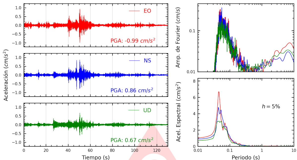
Figura A.15: Registros tiempo-historia, espectros de Fourier y de respuesta en las direcciones EO, NS y vertical de la estación UPCS. Sismo de Yungas, Canta - Lima del 2025-08-17, 08:33:57 (Hora local)
