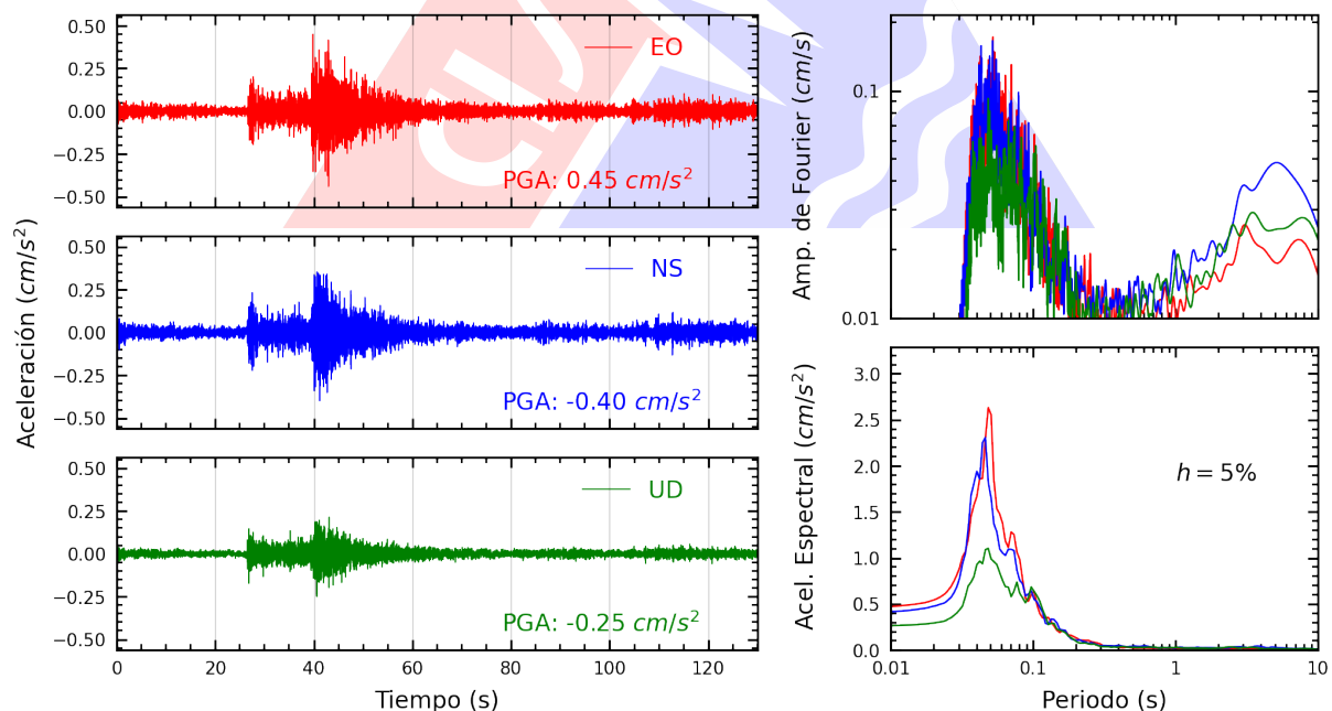
Figura A.30: Registros tiempo-historia, espectros de Fourier y de respuesta en las direcciones EO, NS y vertical de la estación CEPRE. Sismo de Yungas, Canta - Lima del 2025-08-17, 08:33:57 (Hora local)
