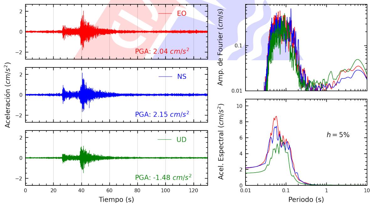
Figura A.4: Registros tiempo-historia, espectros de Fourier y de respuesta en las direcciones EO, NS y vertical de la estación USILM. Sismo de Yangas, Canta - Lima del 2025-08-17, 08:33:57 (Hora local)
