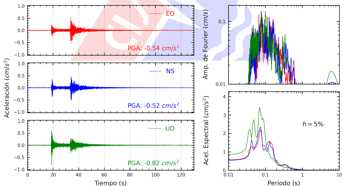
Figura A.18: Registros tiempo-historia, espectros de Fourier y de respuesta en las direcciones EO, NS y vertical de la estación CARAL. Sismo de Yungas, Canta - Lima del 2025-08-17, 08:33:57 (Hora local)
