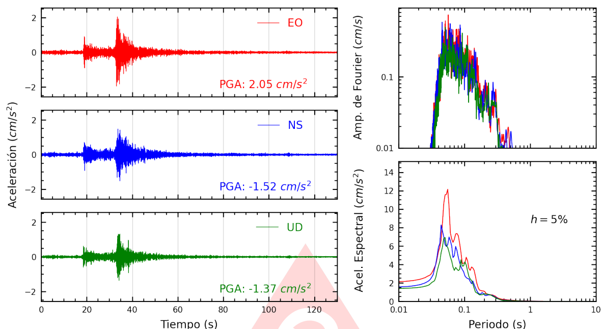
Figura A.5: Registros tiempo-historia, espectros de Fourier y de respuesta en las direcciones EO, NS y vertical de la estación PHERM. Sismo de Yungas, Canta - Lima del 2025-08-17, 08:33:57 (Hora local)
