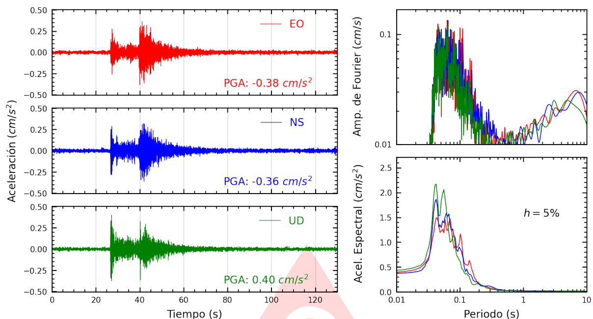
Figura A.35: Registros tiempo-historia, espectros de Fourier y de respuesta en las direcciones EO, NS y vertical de la estación SERVI. Sismo de Yungas, Canta - Lima del 2025-08-17, 08:33:57 (Hora local)
