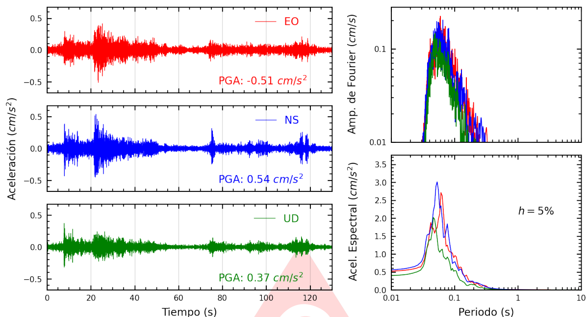
Figura A.27: Registros tiempo-historia, espectros de Fourier y de respuesta en las direcciones EO, NS y vertical de la estación PACHA. Sismo de Yungas, Canta - Lima del 2025-08-17, 08:33:57 (Hora local)
