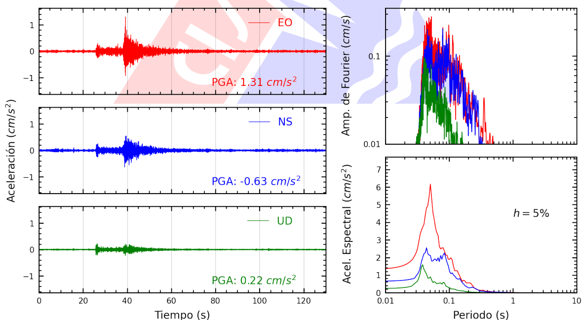
Figura A.12: Registros tiempo-historia, espectros de Fourier y de respuesta en las direcciones EO, NS y vertical de la estación UCVAT. Sismo de Yungas, Canta - Lima del 2025-08-17, 08:33:57 (Hora local)
