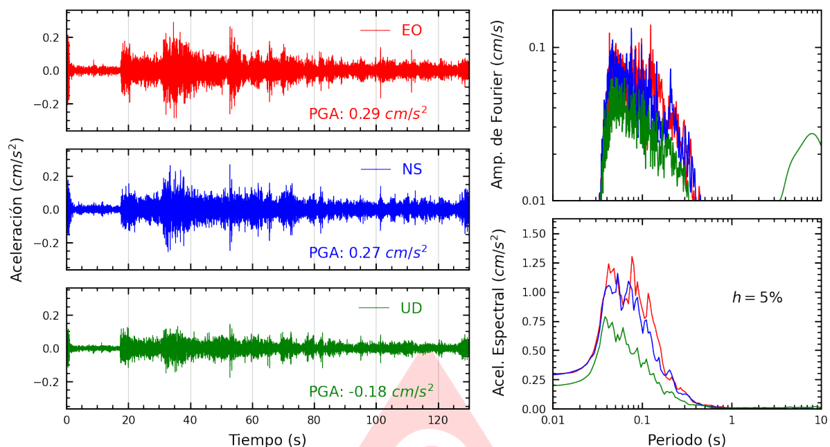
Figura A.39: Registros tiempo-historia, espectros de Fourier y de respuesta en las direcciones EO, NS y vertical de la estación BRISA. Sismo de Yungas, Canta - Lima del 2025-08-17, 08:33:57 (Hora local)
