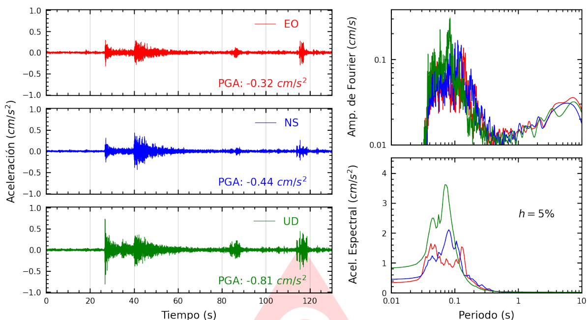
Figura A.19: Registros tiempo-historia, espectros de Fourier y de respuesta en las direcciones EO, NS y vertical de la estación SOCHO. Sismo de Yungas, Canta - Lima del 2025-08-17, 08:33:57 (Hora local)
