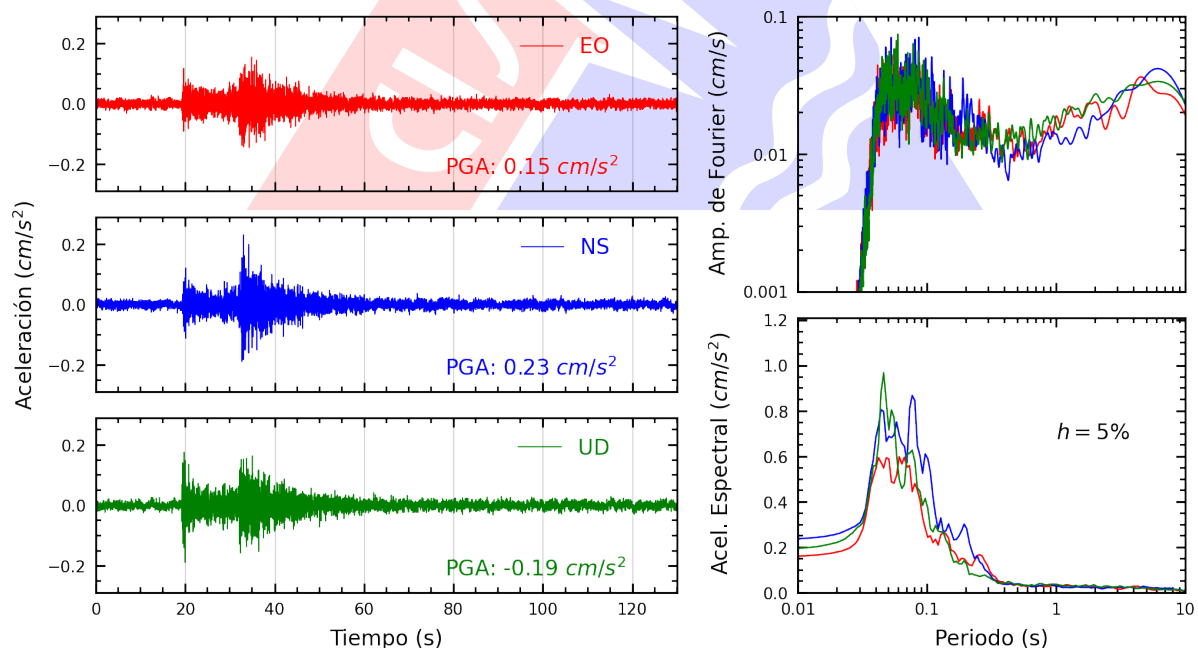
Figura A.42: Registros tiempo-historia, espectros de Fourier y de respuesta en las direcciones EO, NS y vertical de la estación UNMSM. Sismo de Yungas, Canta - Lima del 2025-08-17, 08:33:57 (Hora local)
