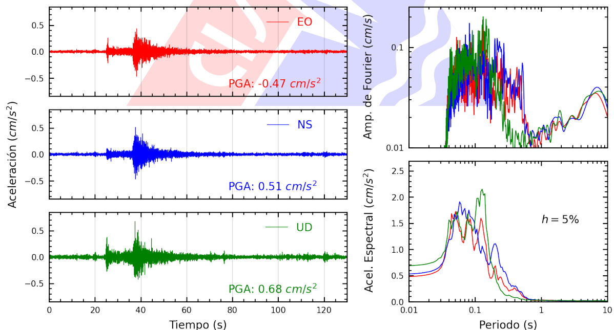
Figura A.24: Registros tiempo-historia, espectros de Fourier y de respuesta en las direcciones EO, NS y vertical de la estación MDPP. Sismo de Yungas, Canta - Lima del 2025-08-17, 08:33:57 (Hora local)
