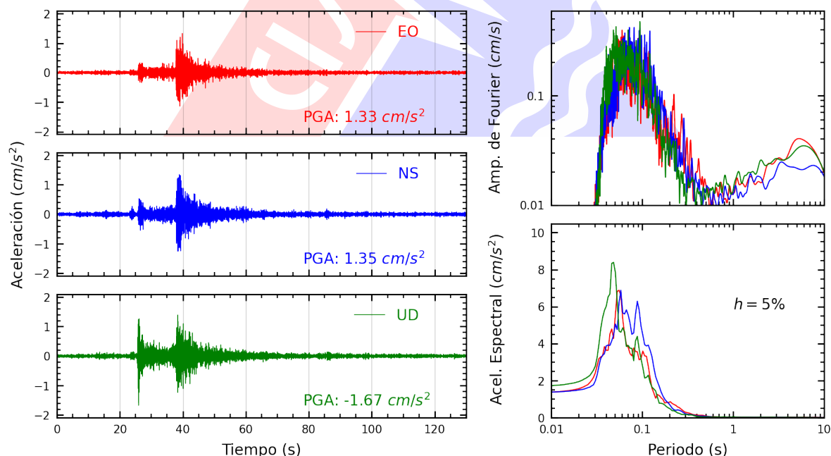
Figura A.6: Registros tiempo-historia, espectros de Fourier y de respuesta en las direcciones EO, NS y vertical de la estación SJLSC. Sismo de Yungas, Canta - Lima del 2025-08-17, 08:33:57 (Hora local)
