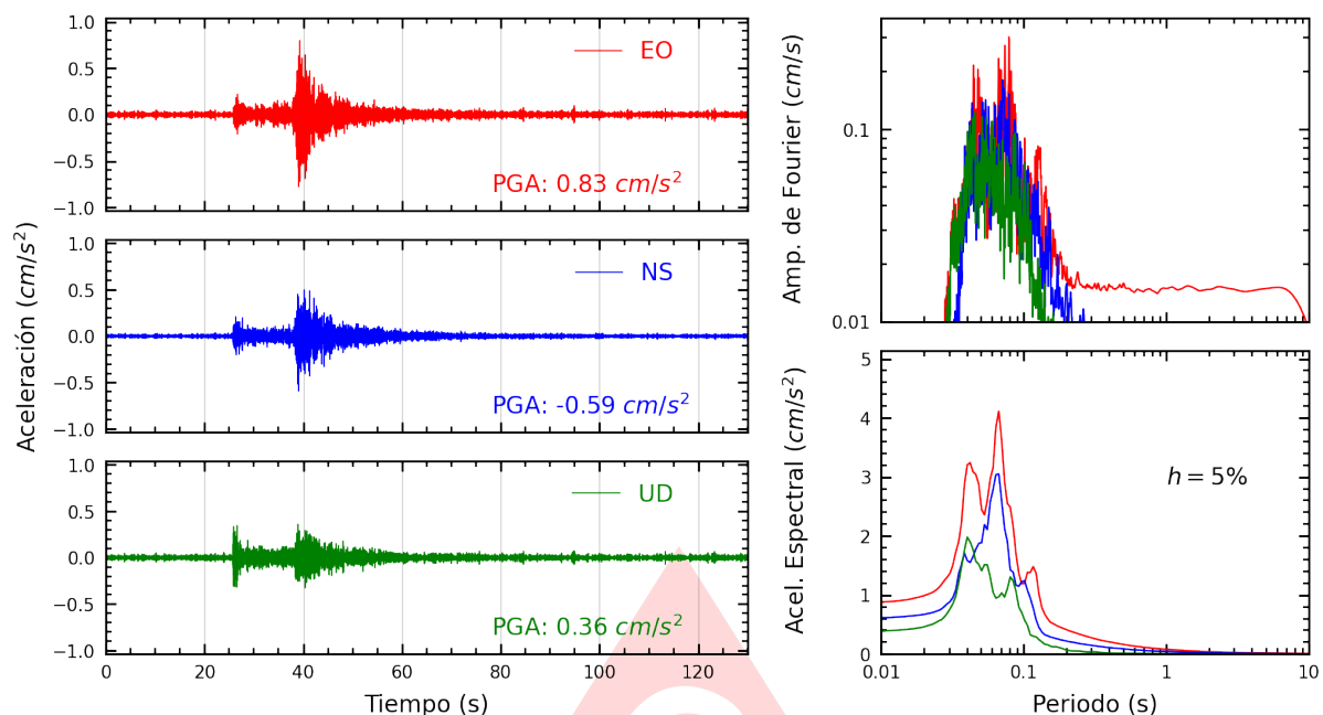
Figura A.17: Registros tiempo-historia, espectros de Fourier y de respuesta en las direcciones EO, NS y vertical de la estación ATARJ. Sismo de Yungas, Canta - Lima del 2025-08-17, 08:33:57 (Hora local)
