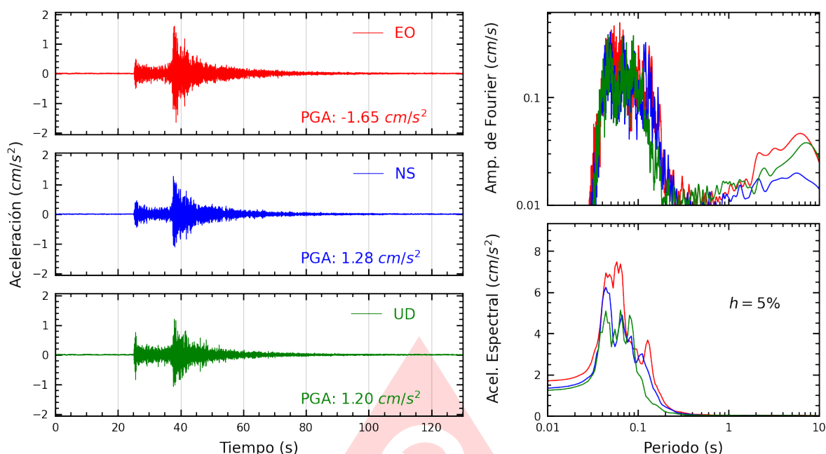
Figura A.7: Registros tiempo-historia, espectros de Fourier y de respuesta en las direcciones EO, NS y vertical de la estación AMORE. Sismo de Yungas, Canta - Lima del 2025-08-17, 08:33:57 (Hora local)
