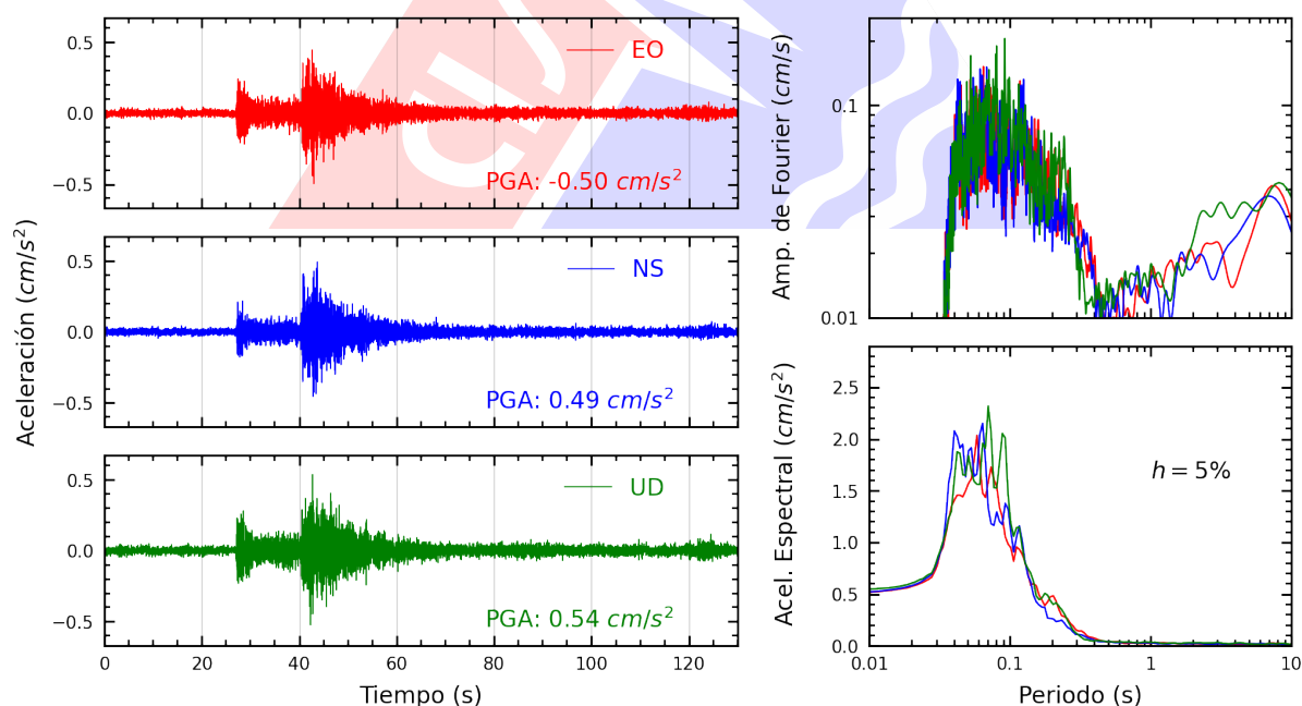
Figura A.28: Registros tiempo-historia, espectros de Fourier y de respuesta en las direcciones EO, NS y vertical de la estación SOVES. Sismo de Yungas, Canta - Lima del 2025-08-17, 08:33:57 (Hora local)
