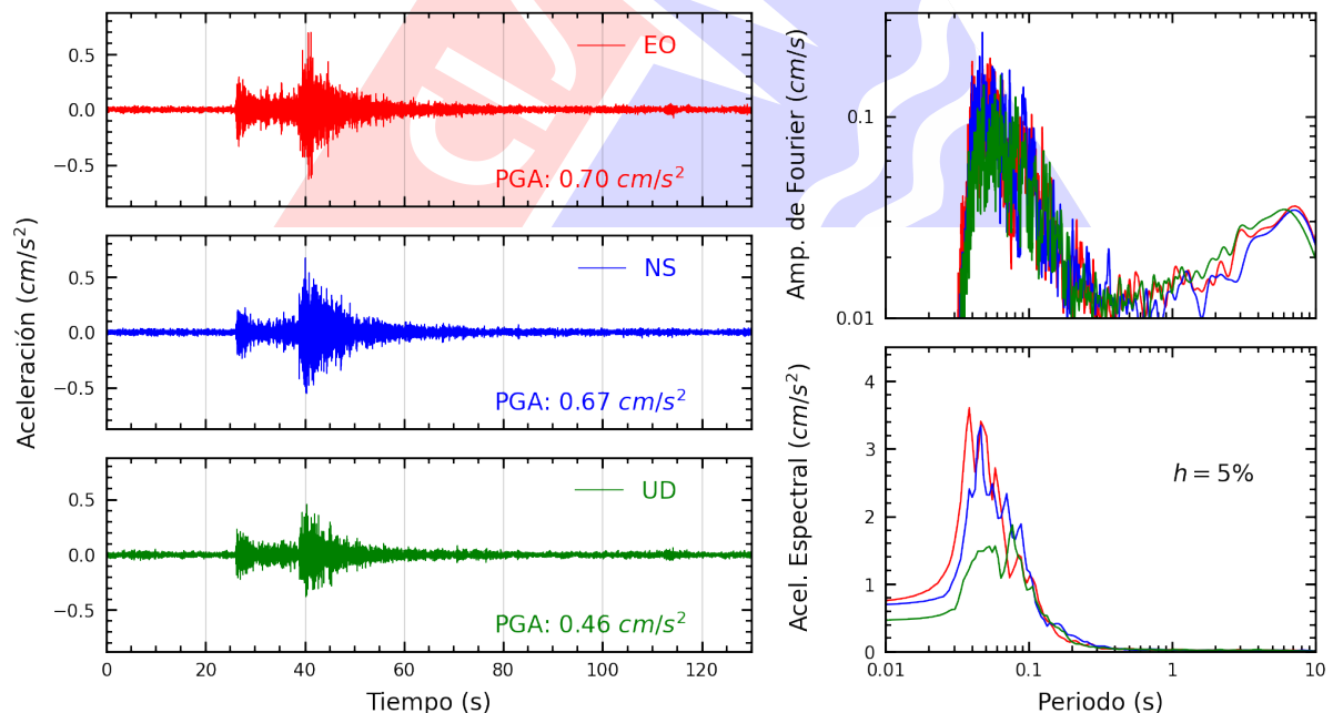
Figura A.22: Registros tiempo-historia, espectros de Fourier y de respuesta en las direcciones EO, NS y vertical de la estación IMCA. Sismo de Yungas, Canta - Lima del 2025-08-17, 08:33:57 (Hora local)
