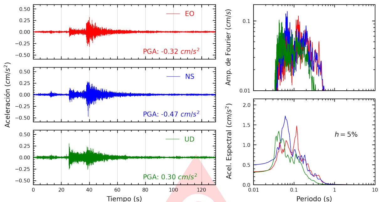
Figura A.29: Registros tiempo-historia, espectros de Fourier y de respuesta en las direcciones EO, NS y vertical de la estación VHAYA. Sismo de Yungas, Canta - Lima del 2025-08-17, 08:33:57 (Hora local)
