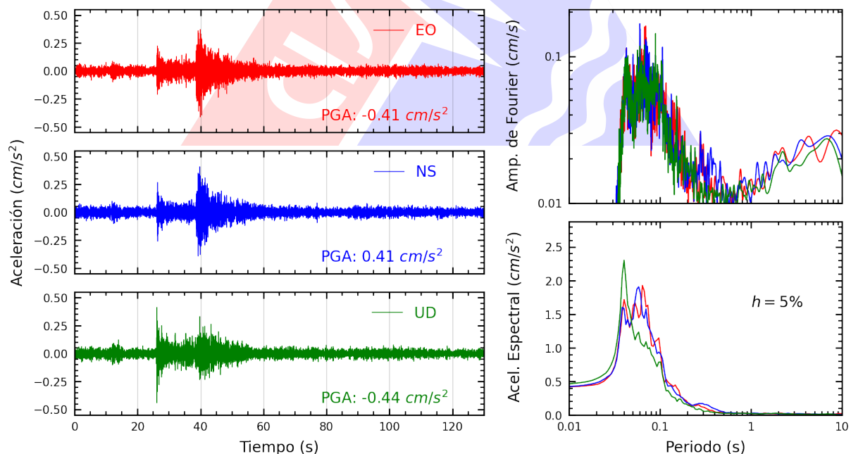
Figura A.32: Registros tiempo-historia, espectros de Fourier y de respuesta en las direcciones EO, NS y vertical de la estación MADRE. Sismo de Yungas, Canta - Lima del 2025-08-17, 08:33:57 (Hora local)
