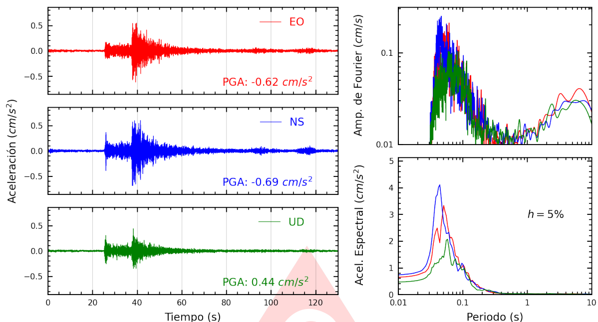
Figura A.23: Registros tiempo-historia, espectros de Fourier y de respuesta en las direcciones EO, NS y vertical de la estación COMAS. Sismo de Yungas, Canta - Lima del 2025-08-17, 08:33:57 (Hora local)
