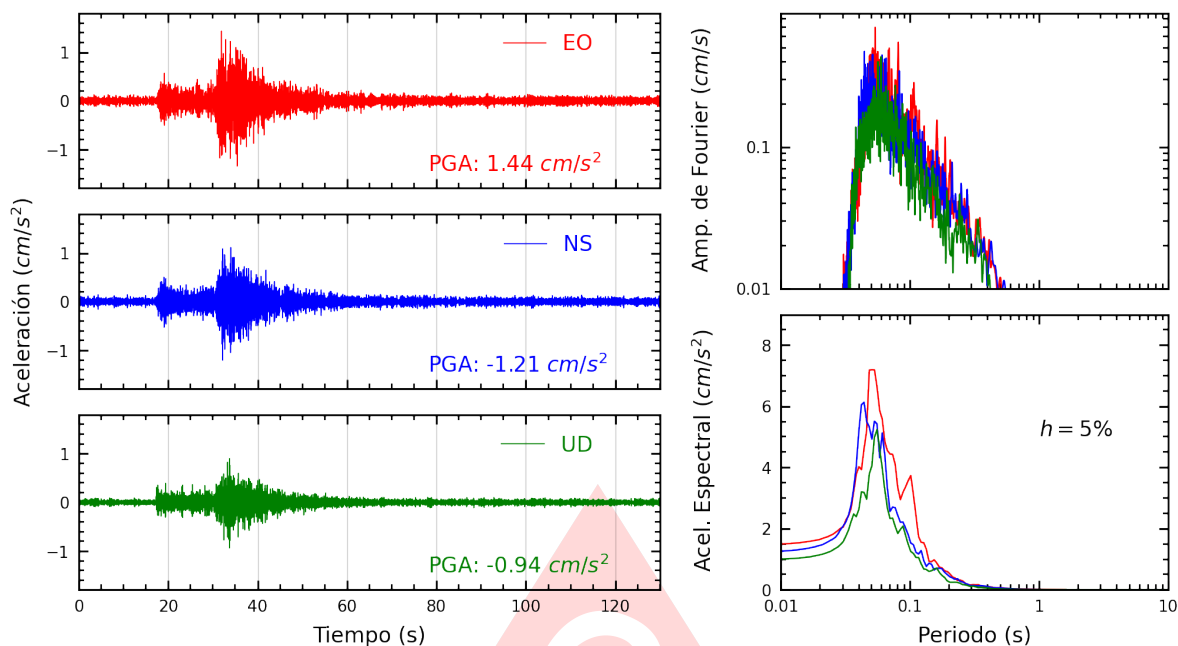
Figura A.9: Registros tiempo-historia, espectros de Fourier y de respuesta en las direcciones EO, NS y vertical de la estación UNTEL. Sismo de Yangas, Canta - Lima del 2025-08-17, 08:33:57 (Hora local)
