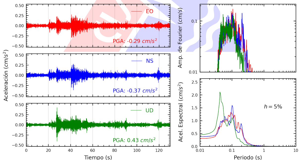
Figura A.34: Registros tiempo-historia, espectros de Fourier y de respuesta en las direcciones EO, NS y vertical de la estación SCCHO. Sismo de Yungas, Canta - Lima del 2025-08-17, 08:33:57 (Hora local)
