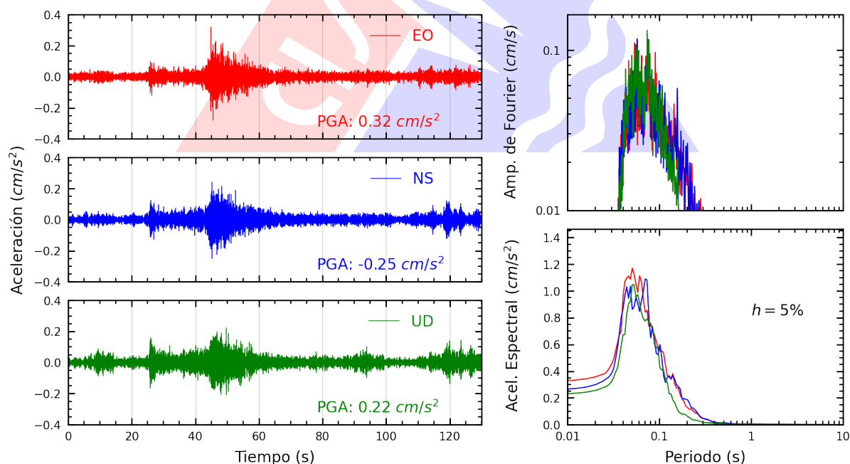
Figura A.38: Registros tiempo-historia, espectros de Fourier y de respuesta en las direcciones EO, NS y vertical de la estación ASIA. Sismo de Yangas, Canta - Lima del 2025-08-17, 08:33:57 (Hora local)
