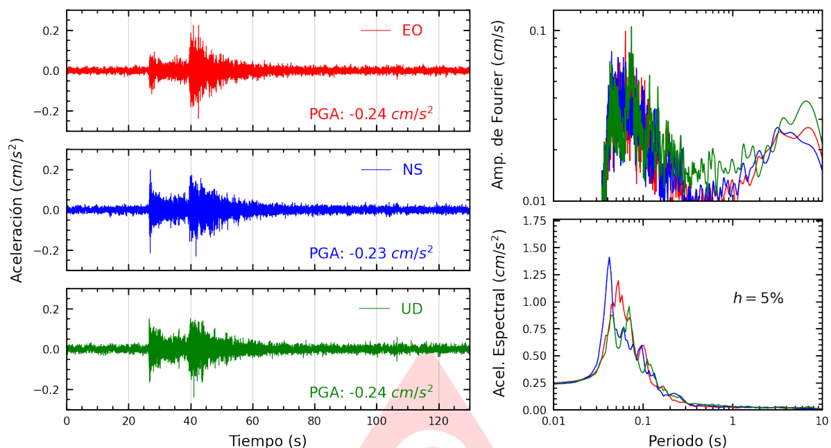
Figura A.41: Registros tiempo-historia, espectros de Fourier y de respuesta en las direcciones EO, NS y vertical de la estación UNFV. Sismo de Yungas, Canta - Lima del 2025-08-17, 08:33:57 (Hora local)
