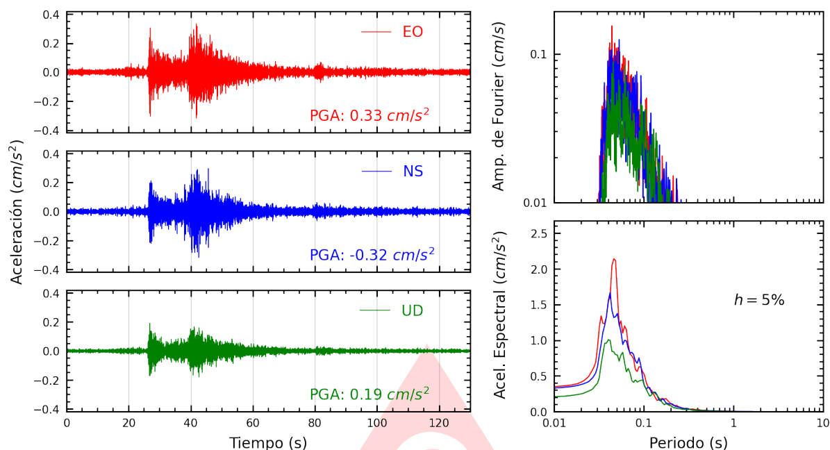
Figura A.37: Registros tiempo-historia, espectros de Fourier y de respuesta en las direcciones EO, NS y vertical de la estación BORJA. Sismo de Yangas, Canta - Lima del 2025-08-17, 08:33:57 (Hora local)
