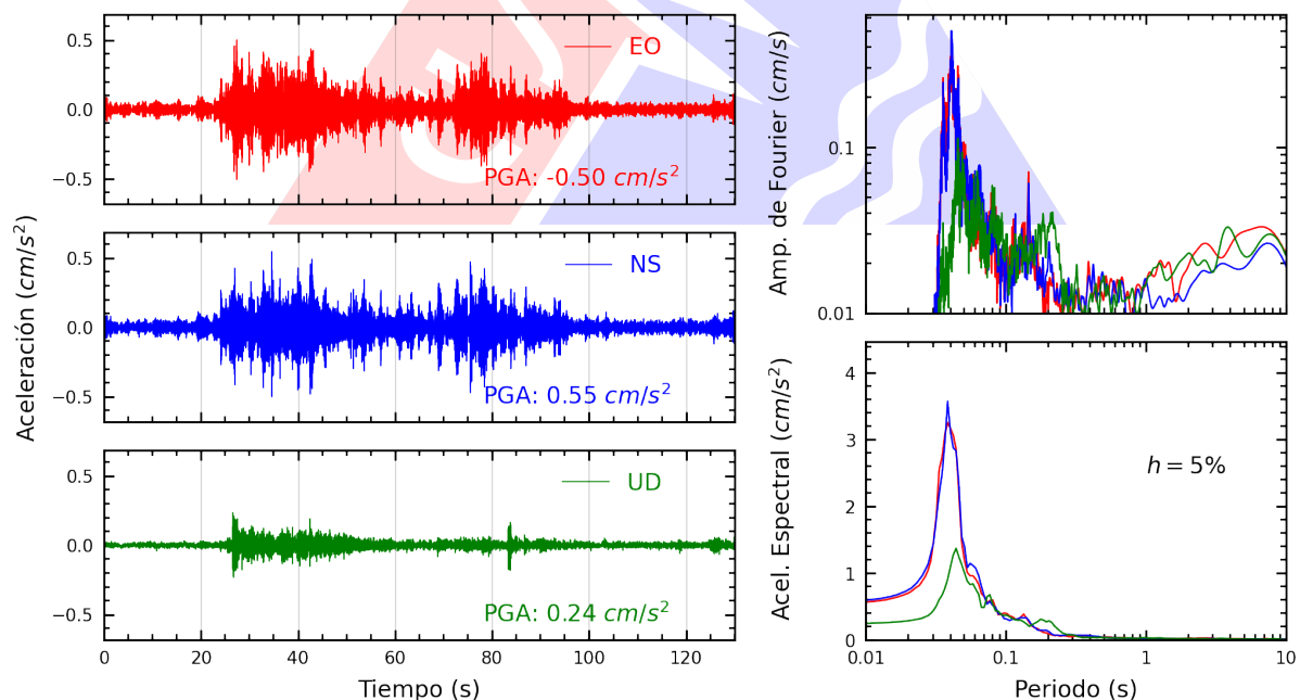
Figura A.26: Registros tiempo-historia, espectros de Fourier y de respuesta en las direcciones EO, NS y vertical de la estación DHNPE. Sismo de Yungas, Canta - Lima del 2025-08-17, 08:33:57 (Hora local)
