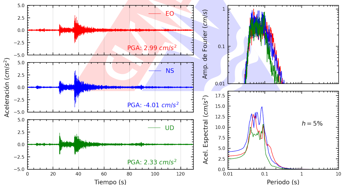
Figura A.2: Registros tiempo-historia, espectros de Fourier y de respuesta en las direcciones EO, NS y vertical de la estación SROSA. Sismo de Yangas, Canta - Lima del 2025-08-17, 08:33:57 (Hora local)
