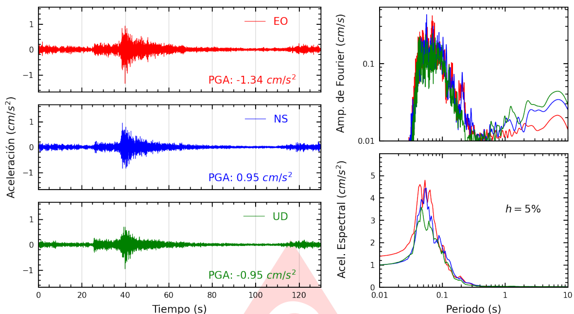
Figura A.11: Registros tiempo-historia, espectros de Fourier y de respuesta en las direcciones EO, NS y vertical de la estación INDEP. Sismo de Yungas, Canta - Lima del 2025-08-17, 08:33:57 (Hora local)
