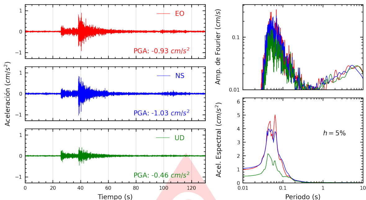
Figura A.13: Registros tiempo-historia, espectros de Fourier y de respuesta en las direcciones EO, NS y vertical de la estación FICPE. Sismo de Yungas, Canta - Lima del 2025-08-17, 08:33:57 (Hora local)
