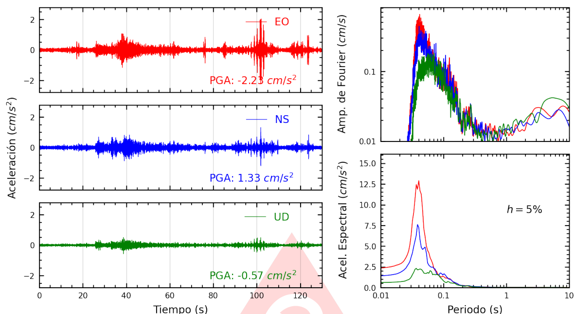
Figura A.3: Registros tiempo-historia, espectros de Fourier y de respuesta en las direcciones EO, NS y vertical de la estación OLIVO. Sismo de Yangas, Canta - Lima del 2025-08-17, 08:33:57 (Hora local)
