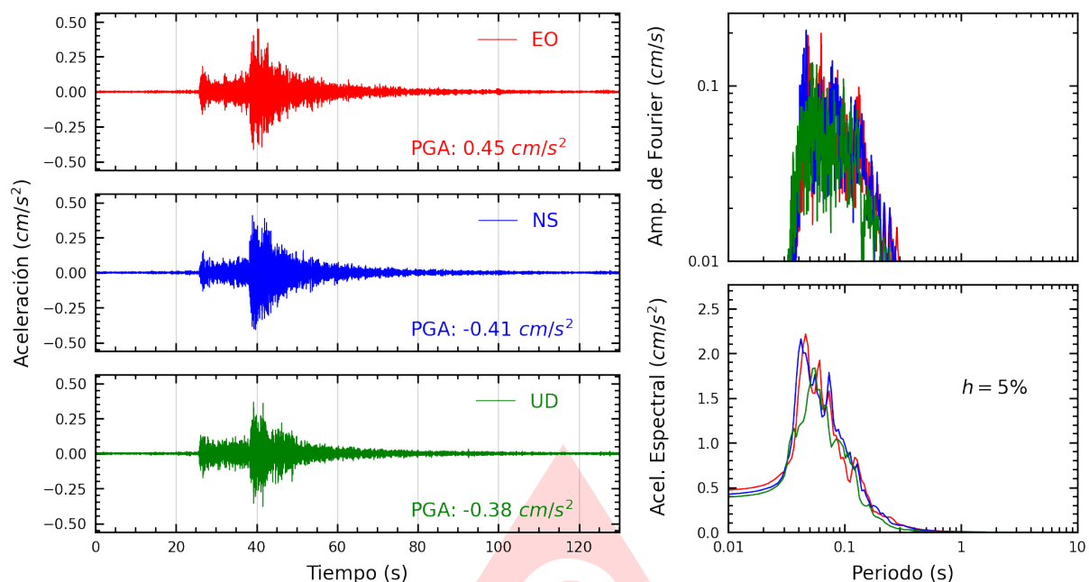
Figura A.31: Registros tiempo-historia, espectros de Fourier y de respuesta en las direcciones EO, NS y vertical de la estación JALV2. Sismo de Yungas, Canta - Lima del 2025-08-17, 08:33:57 (Hora local)
