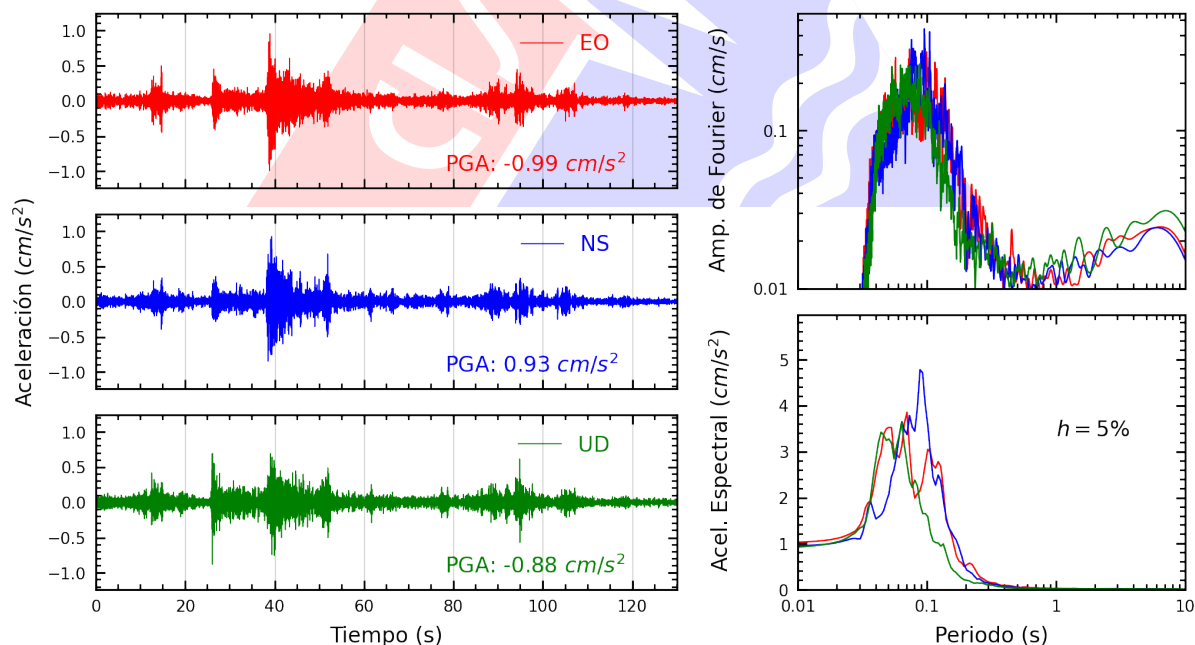
Figura A.14: Registros tiempo-historia, espectros de Fourier y de respuesta en las direcciones EO, NS y vertical de la estación SJLSV. Sismo de Yungas, Canta - Lima del 2025-08-17, 08:33:57 (Hora local)
