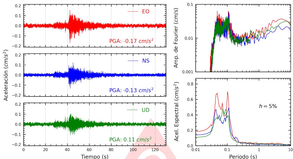
Figura A.3: Registros tiempo-historia, espectros de Fourier y de respuesta en las direcciones EO, NS y vertical de la estación AMORE. Sismo de Mala, Cañete - Lima del 2025-08-18, 21:52:07 (Hora local)
