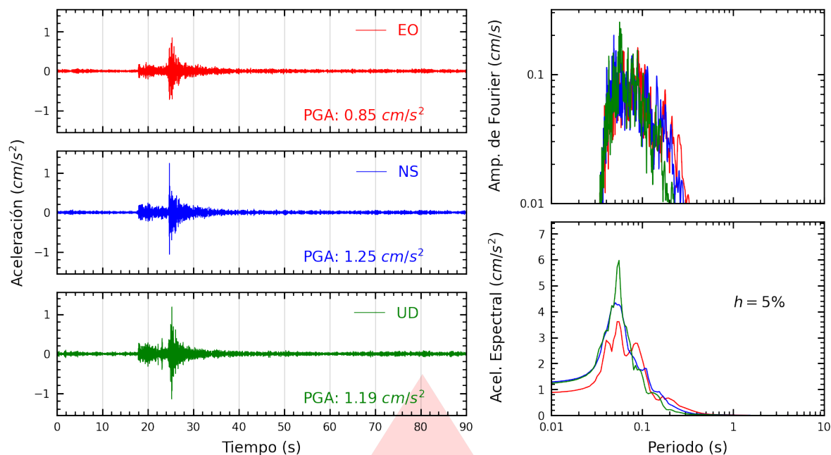
Figura A.1: Registros tiempo-historia, espectros de Fourier y de respuesta en las direcciones EO, NS y vertical de la estación ASIA. Sismo de Mala, Cañete - Lima del 2025-08-18, 21:52:07 (Hora local)
