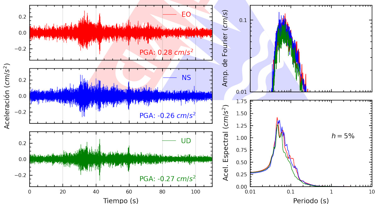
Figura A.2: Registros tiempo-historia, espectros de Fourier y de respuesta en las direcciones EO, NS y vertical de la estación PHERM. Sismo de Mala, Cañete - Lima del 2025-08-18, 21:52:07 (Hora local)
