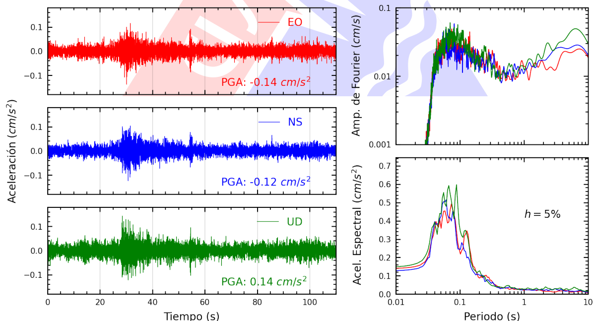
Figura A.4: Registros tiempo-historia, espectros de Fourier y de respuesta en las direcciones EO, NS y vertical de la estación SOVES. Sismo de Mala, Cañete - Lima del 2025-08-18, 21:52:07 (Hora local)
