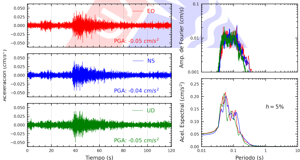
Figura A.8: Registros tiempo-historia, espectros de Fourier y de respuesta en las direcciones EO, NS y vertical de la estación JALV2. Sismo de Mala, Cañete - Lima del 2025-08-18, 21:52:07 (Hora local)
