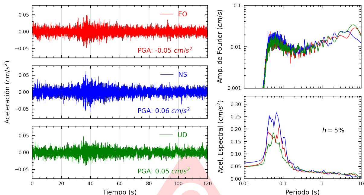
Figura A.7: Registros tiempo-historia, espectros de Fourier y de respuesta en las direcciones EO, NS y vertical de la estación SERVI. Sismo de Mala, Cañete - Lima del 2025-08-18, 21:52:07 (Hora local)
