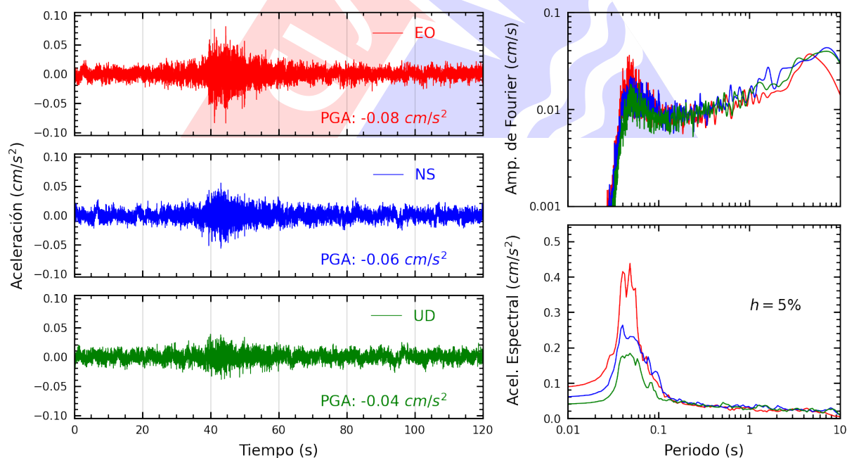
Figura A.6: Registros tiempo-historia, espectros de Fourier y de respuesta en las direcciones EO, NS y vertical de la estación UCSS. Sismo de Mala, Cañete - Lima del 2025-08-18, 21:52:07 (Hora local)
