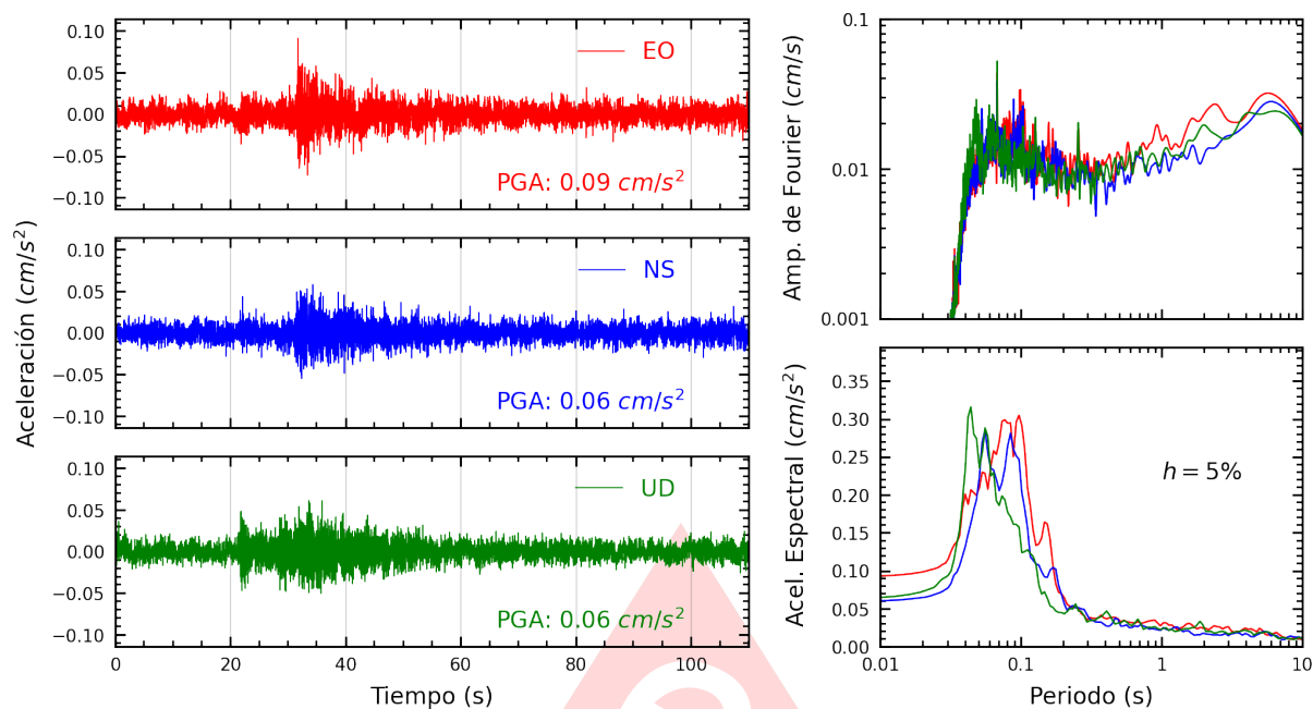
Figura A.5: Registros tiempo-historia, espectros de Fourier y de respuesta en las direcciones EO, NS y vertical de la estación USILP. Sismo de Mala, Cañete - Lima del 2025-08-18, 21:52:07 (Hora local)
