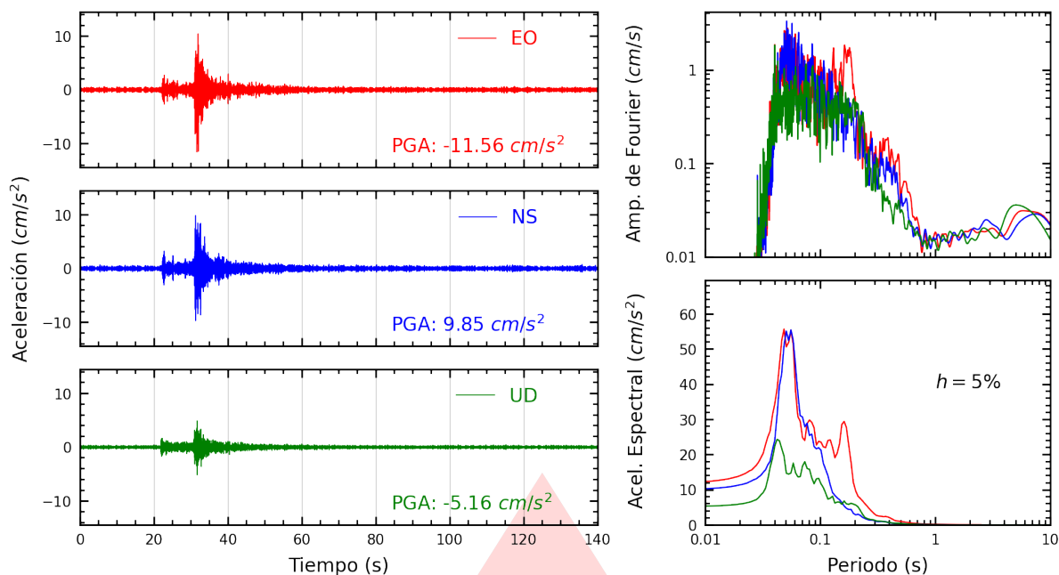
Figura A.1: Registros tiempo-historia, espectros de Fourier y de respuesta en las direcciones EO, NS y vertical de la estación USP. Sismo de Chimbote, Santa - Ancash del 2025-08-19, 04:15:46 (Hora local)
