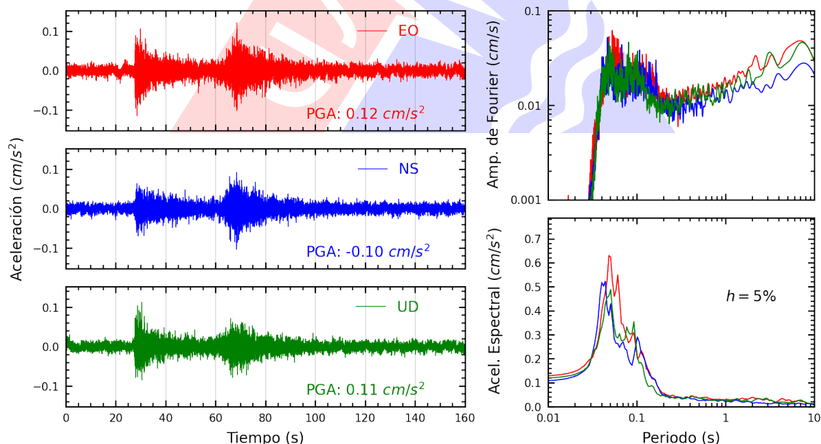
Figura A.4: Registros tiempo-historia, espectros de Fourier y de respuesta en las direcciones EO, NS y vertical de la estación AMORE. Sismo de Chimbote, Santa - Ancash del 2025-08-19, 04:15:46 (Hora local)
