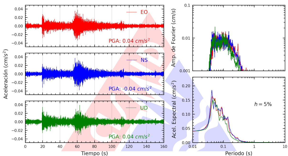
Figura A.7: Registros tiempo-historia, espectros de Fourier y de respuesta en las direcciones EO, NS y vertical de la estación JALV2. Sismo de Chimbote, Santa - Ancash del 2025-08-19, 04:15:46 (Hora local)
