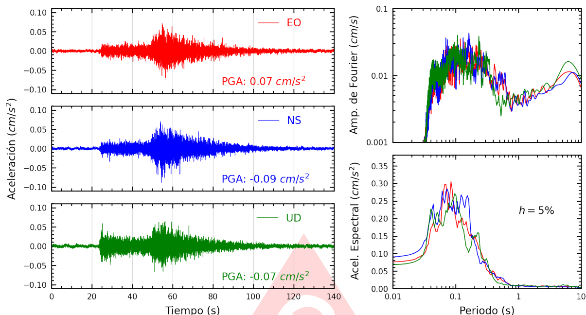
Figura A.5: Registros tiempo-historia, espectros de Fourier y de respuesta en las direcciones EO, NS y vertical de la estación CARAL. Sismo de Chimbote, Santa - Ancash del 2025-08-19, 04:15:46 (Hora local)
