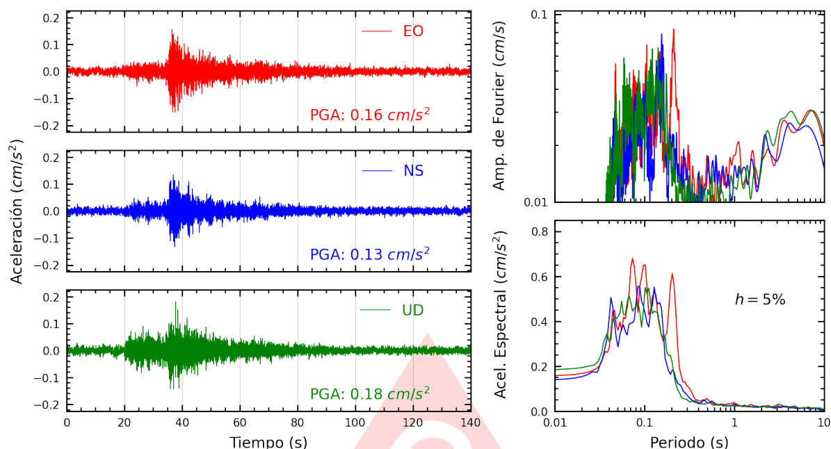
Figura A.3: Registros tiempo-historia, espectros de Fourier y de respuesta en las direcciones EO, NS y vertical de la estación UPAOT. Sismo de Chimbote, Santa - Ancash del 2025-08-19, 04:15:46 (Hora local)
