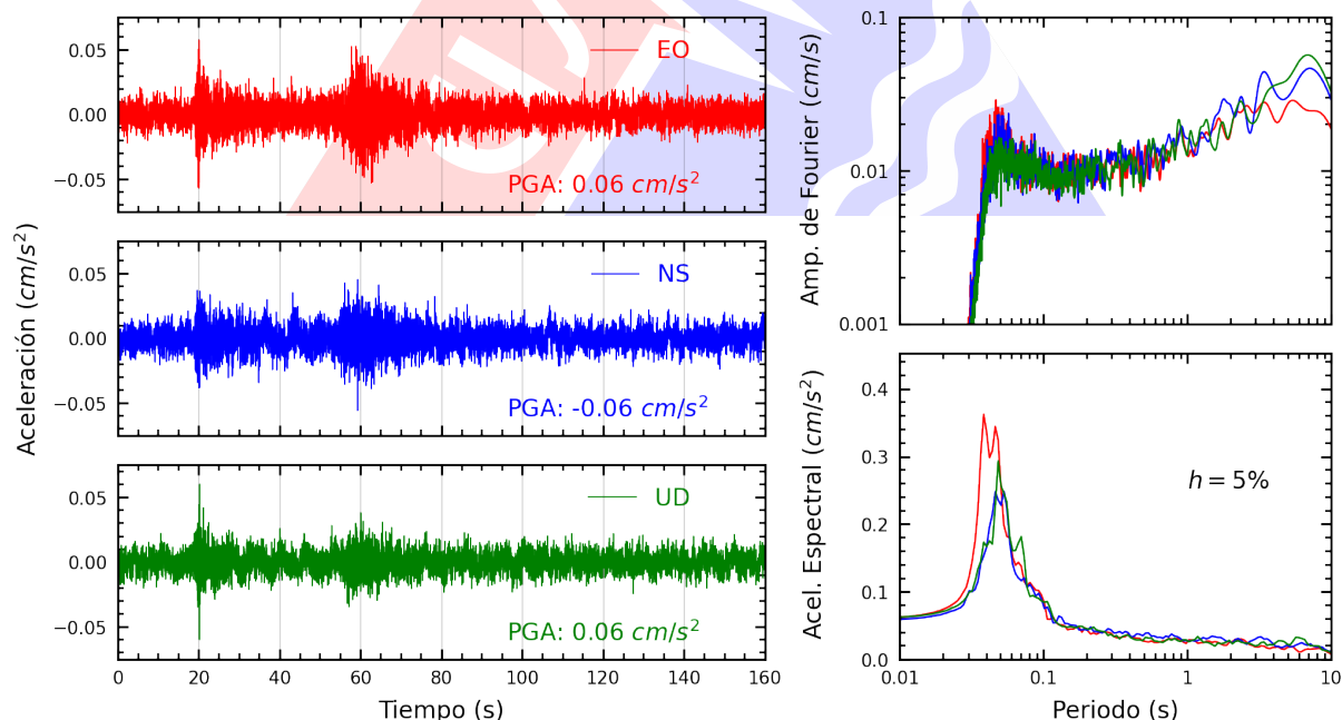
Figura A.6: Registros tiempo-historia, espectros de Fourier y de respuesta en las direcciones EO, NS y vertical de la estación UCSS. Sismo de Chimbote, Santa - Ancash del 2025-08-19, 04:15:46 (Hora local)
