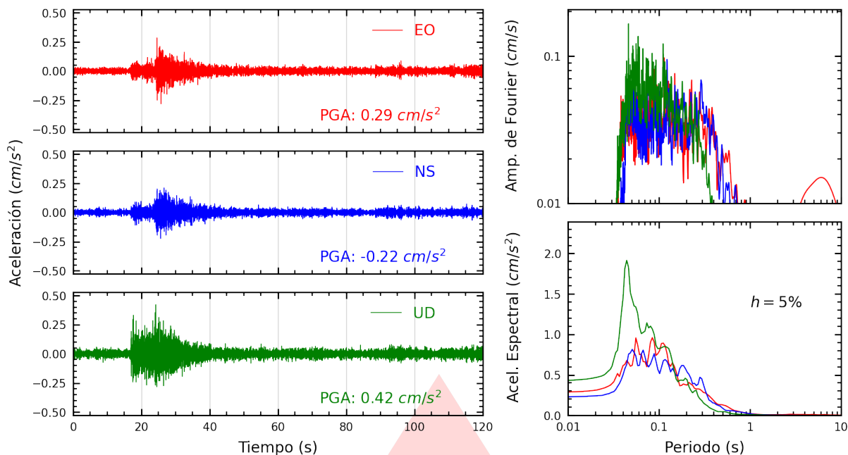
Figura A.1: Registros tiempo-historia, espectros de Fourier y de respuesta en las direcciones EO, NS y vertical de la estación SCPIU. Sismo de Sechura, Sechura - Piura del 2025-08-19, 14:49:36 (Hora local)
