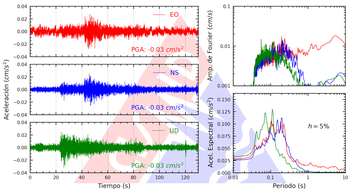
Figura A.3: Registros tiempo-historia, espectros de Fourier y de respuesta en las direcciones EO, NS y vertical de la estación SCCHI. Sismo de Sechura, Sechura - Piura del 2025-08-19, 14:49:36 (Hora local)
