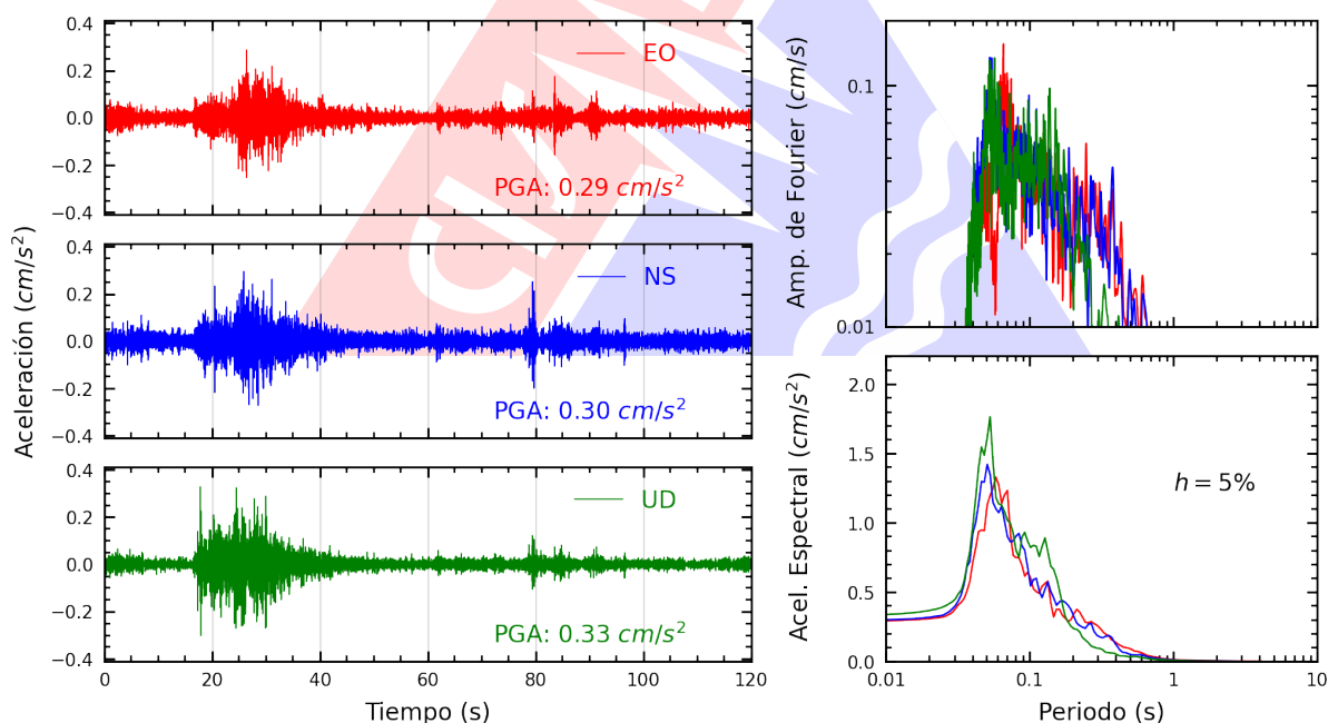
Figura A.2: Registros tiempo-historia, espectros de Fourier y de respuesta en las direcciones EO, NS y vertical de la estación UPAOP. Sismo de Sechura, Sechura - Piura del 2025-08-19, 14:49:36 (Hora local)
