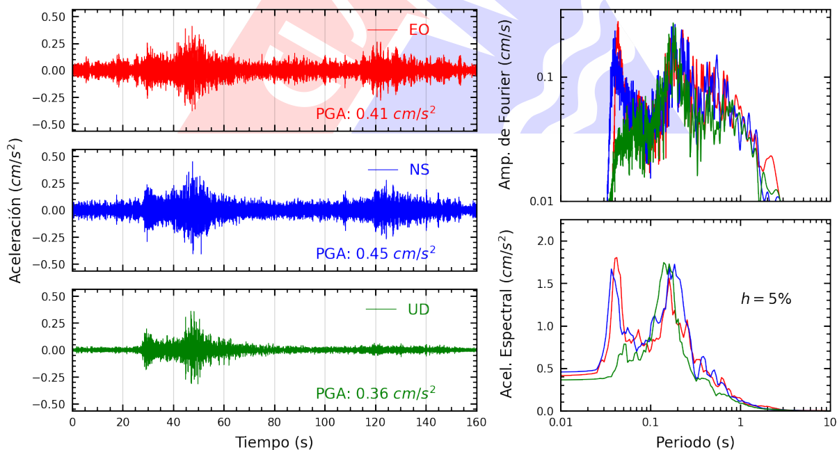
Figura A.4: Registros tiempo-historia, espectros de Fourier y de respuesta en las direcciones EO, NS y vertical de la estación UPTAC. Sismo de Ilo, Ilo - Moquegua del 2025-08-19, 17:49:25 (Hora local)
