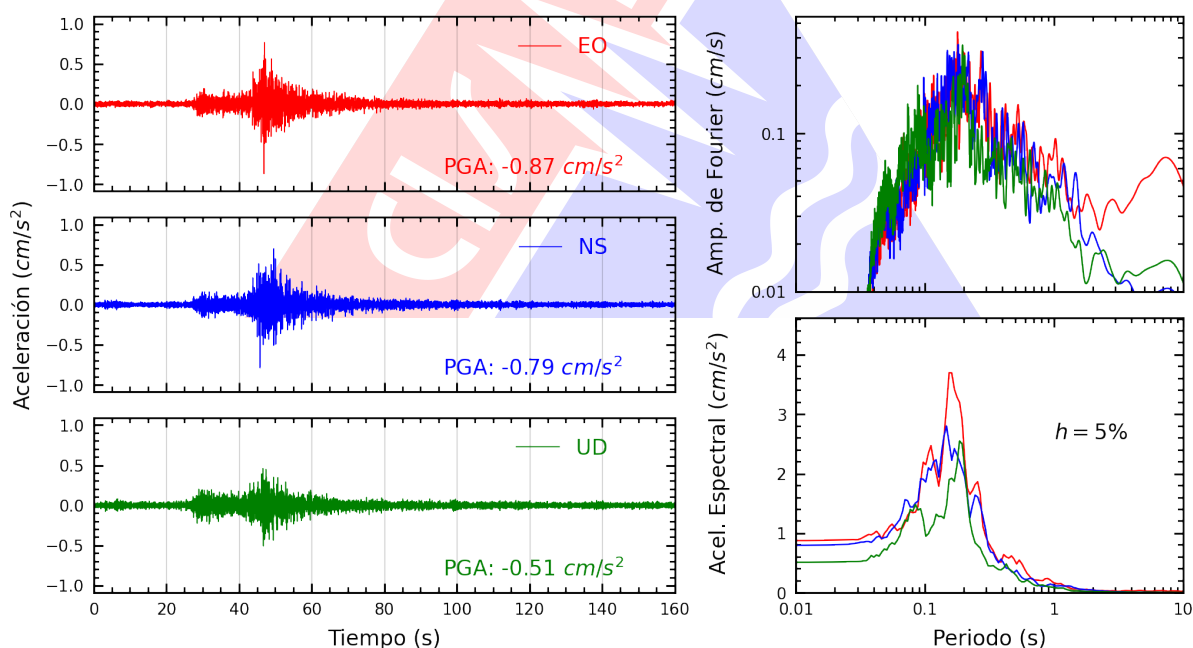
Figura A.2: Registros tiempo-historia, espectros de Fourier y de respuesta en las direcciones EO, NS y vertical de la estación UJBG3. Sismo de Ilo, Ilo - Moquegua del 2025-08-19, 17:49:25 (Hora local)
