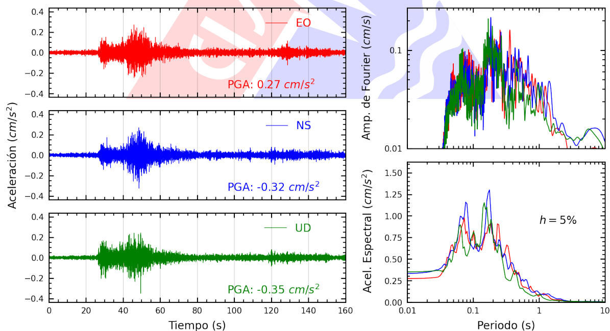
Figura A.6: Registros tiempo-historia, espectros de Fourier y de respuesta en las direcciones EO, NS y vertical de la estación CREY. Sismo de Ilo, Ilo - Moquegua del 2025-08-19, 17:49:25 (Hora local)
