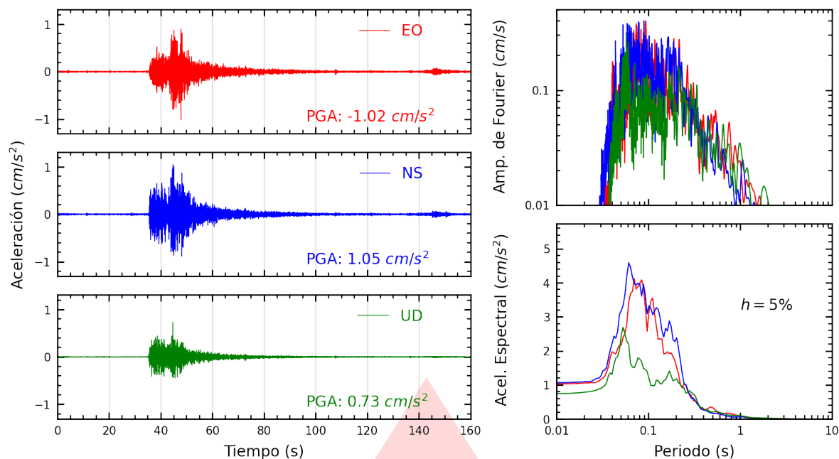
Figura A.1: Registros tiempo-historia, espectros de Fourier y de respuesta en las direcciones EO, NS y vertical de la estación UNAM. Sismo de Ilo, Ilo - Moquegua del 2025-08-19, 17:49:25 (Hora local)
