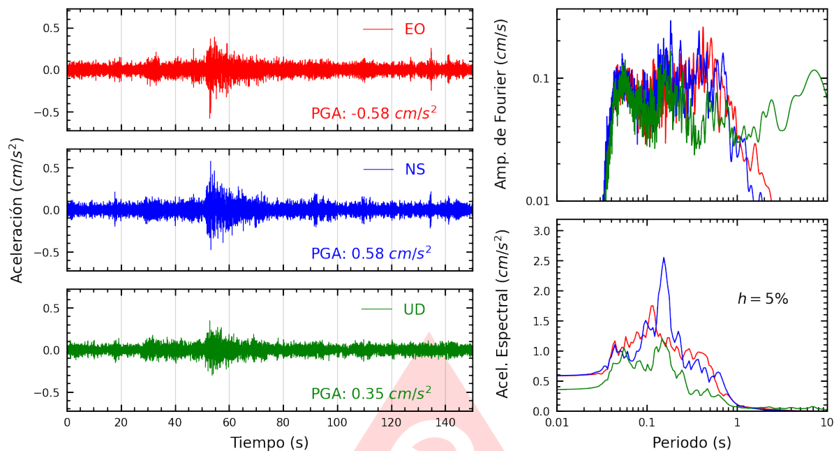
Figura A.3: Registros tiempo-historia, espectros de Fourier y de respuesta en las direcciones EO, NS y vertical de la estación SCARQ. Sismo de Ilo, Ilo - Moquegua del 2025-08-19, 17:49:25 (Hora local)
