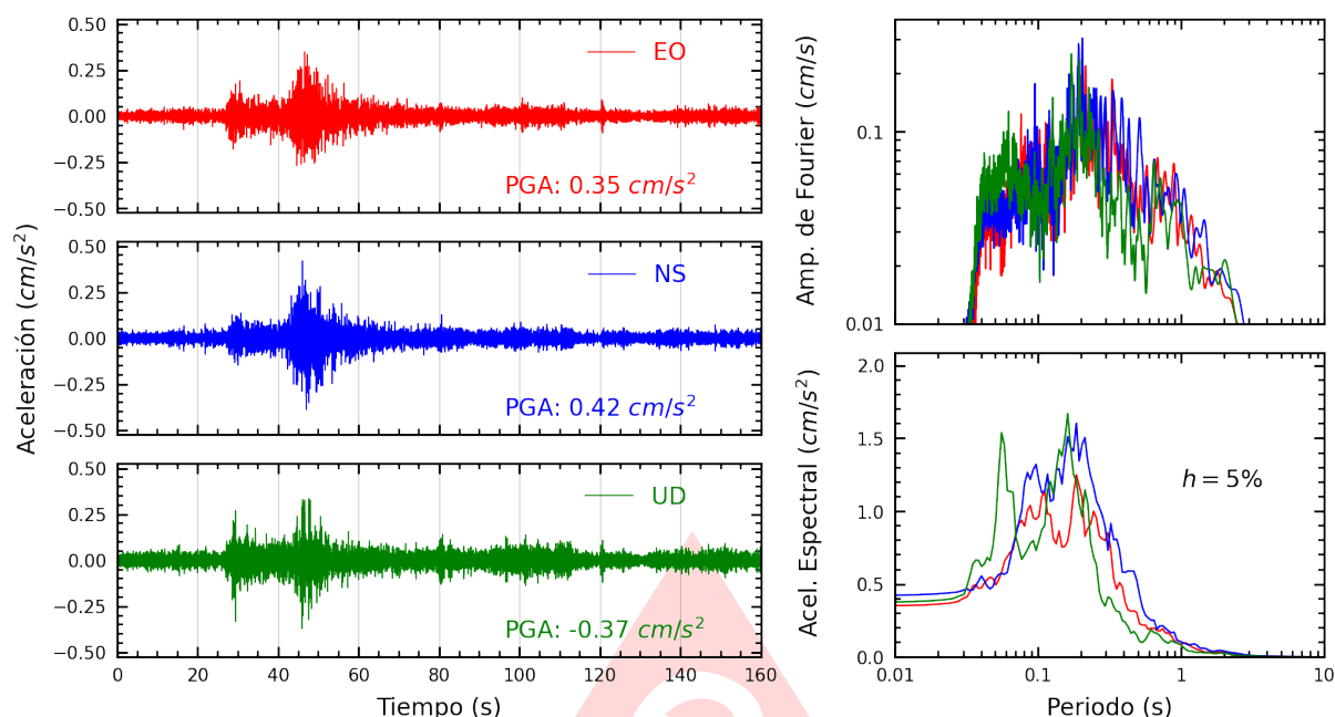
Figura A.5: Registros tiempo-historia, espectros de Fourier y de respuesta en las direcciones EO, NS y vertical de la estación UJBG2. Sismo de Ilo, Ilo - Moquegua del 2025-08-19, 17:49:25 (Hora local)
