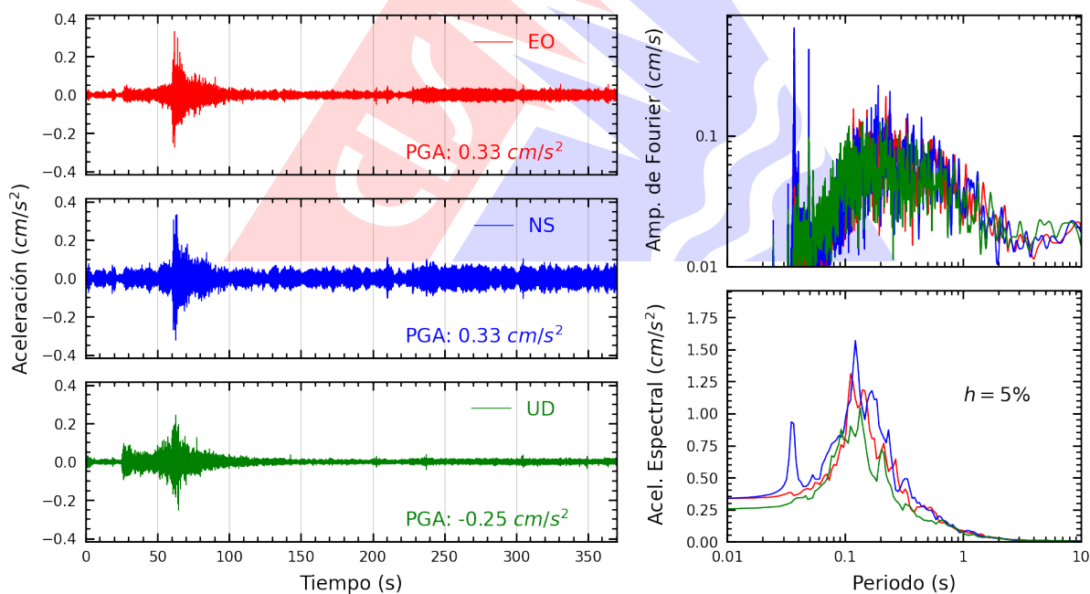
Figura A.2: Registros tiempo-historia, espectros de Fourier y de respuesta en las direcciones EO, NS y vertical de la estación UNJ. Sismo de Pastaza, Datem del Marañón - Loreto del 2025-08-20, 10:06:59 (Hora local)
