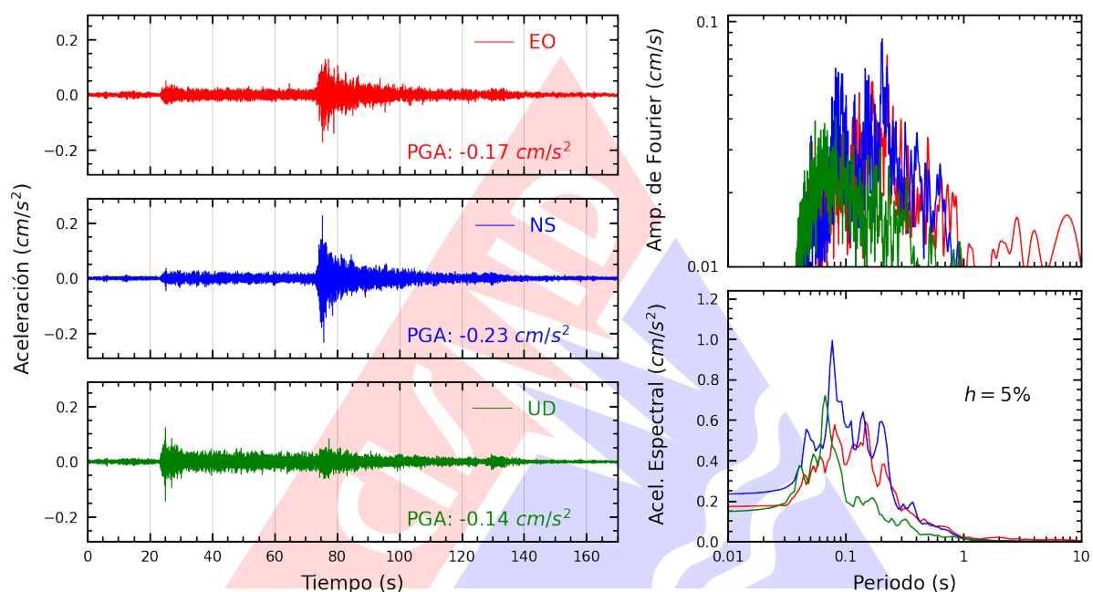
Figura A.3: Registros tiempo-historia, espectros de Fourier y de respuesta en las direcciones EO, NS y vertical de la estación SCCHI. Sismo de Pastaza, Datem del Marañón - Loreto del 2025-08-20, 10:06:59 (Hora local)
