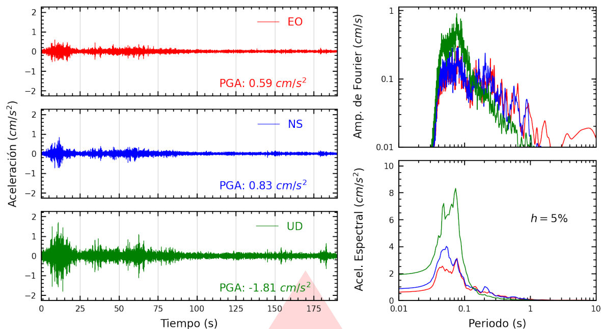
Figura A.1: Registros tiempo-historia, espectros de Fourier y de respuesta en las direcciones EO, NS y vertical de la estación SCIQU. Sismo de Pastaza, Datem del Marañón - Loreto del 2025-08-20, 10:06:59 (Hora local)
