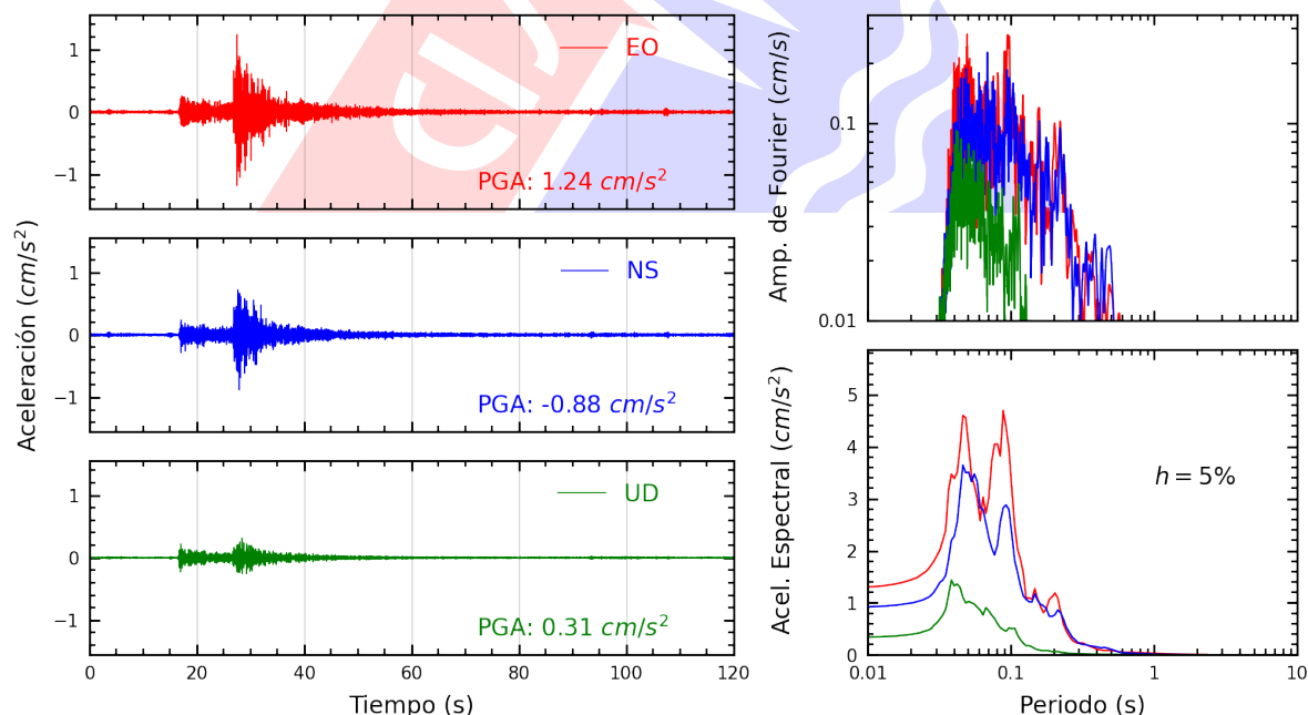
Figura A.8: Registros tiempo-historia, espectros de Fourier y de respuesta en las direcciones EO, NS y vertical de la estación UCVAT. Sismo de Chilca, Cañete - Lima del 2025-08-23, 21:10:22 (Hora local)
