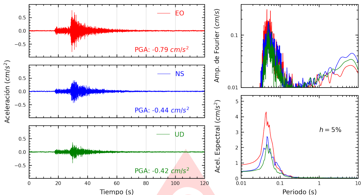
Figura A.13: Registros tiempo-historia, espectros de Fourier y de respuesta en las direcciones EO, NS y vertical de la estación UCSS. Sismo de Chilca, Cañete - Lima del 2025-08-23, 21:10:22 (Hora local)
