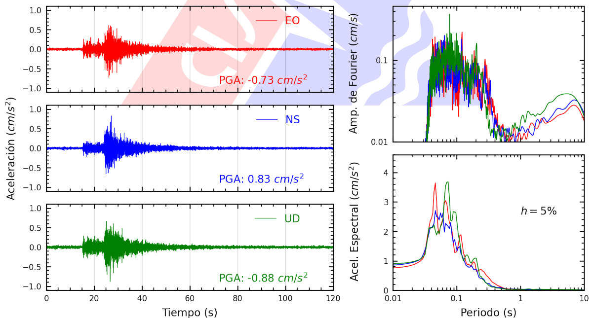
Figura A.10: Registros tiempo-historia, espectros de Fourier y de respuesta en las direcciones EO, NS y vertical de la estación SOVES. Sismo de Chilca, Cañete - Lima del 2025-08-23, 21:10:22 (Hora local)
