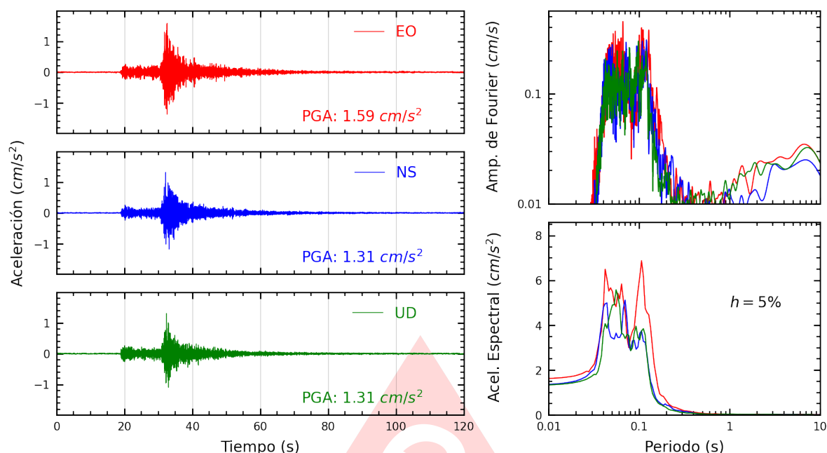
Figura A.5: Registros tiempo-historia, espectros de Fourier y de respuesta en las direcciones EO, NS y vertical de la estación AMORE. Sismo de Chilca, Cañete - Lima del 2025-08-23, 21:10:22 (Hora local)
