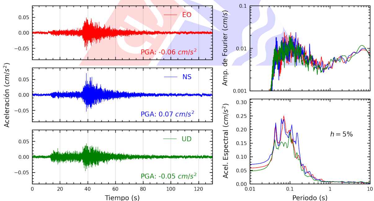
Figura A.26: Registros tiempo-historia, espectros de Fourier y de respuesta en las direcciones EO, NS y vertical de la estación CARAL. Sismo de Chilca, Cañete - Lima del 2025-08-23, 21:10:22 (Hora local)
