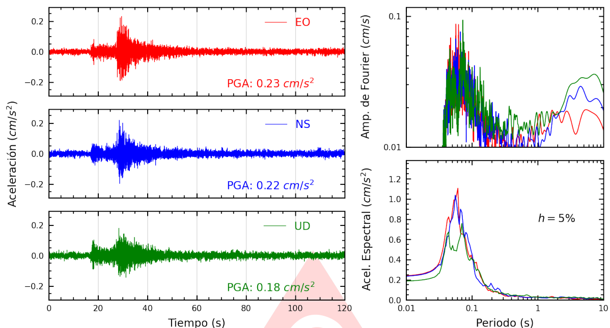
Figura A.25: Registros tiempo-historia, espectros de Fourier y de respuesta en las direcciones EO, NS y vertical de la estación UNFV. Sismo de Chilca, Cañete - Lima del 2025-08-23, 21:10:22 (Hora local)
