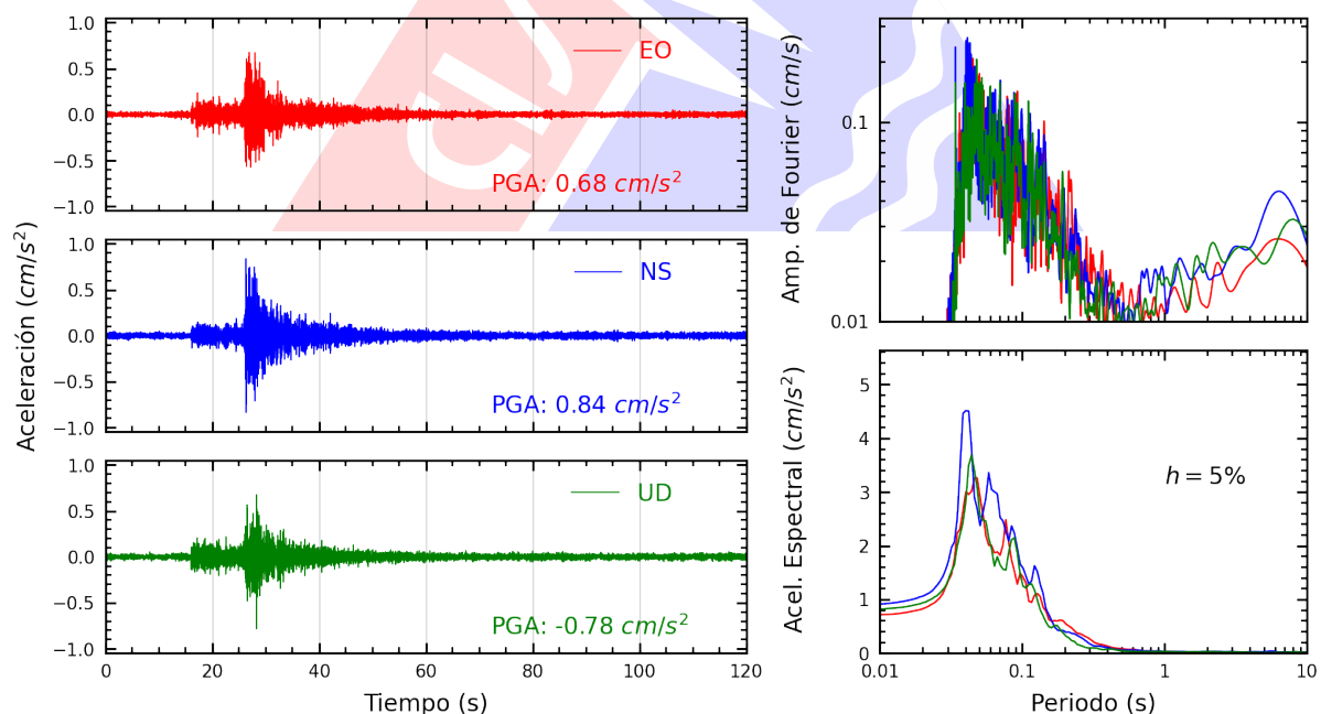
Figura A.12: Registros tiempo-historia, espectros de Fourier y de respuesta en las direcciones EO, NS y vertical de la estación USMP. Sismo de Chilca, Cañete - Lima del 2025-08-23, 21:10:22 (Hora local)
