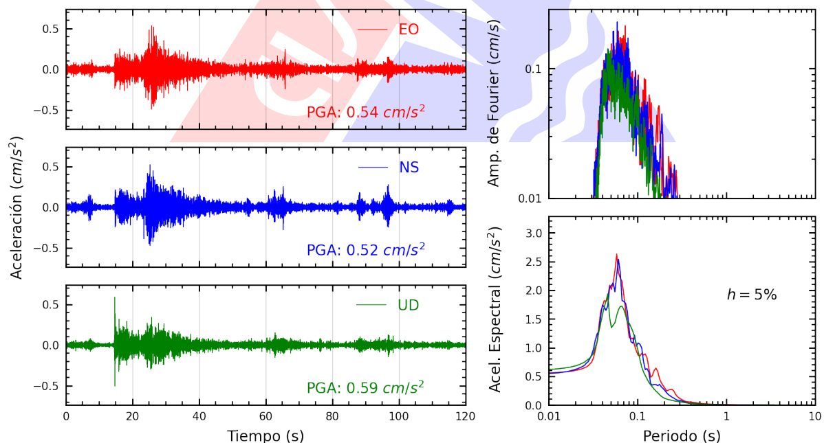
Figura A.22: Registros tiempo-historia, espectros de Fourier y de respuesta en las direcciones EO, NS y vertical de la estación PACHA. Sismo de Chilca, Cañete - Lima del 2025-08-23, 21:10:22 (Hora local)
