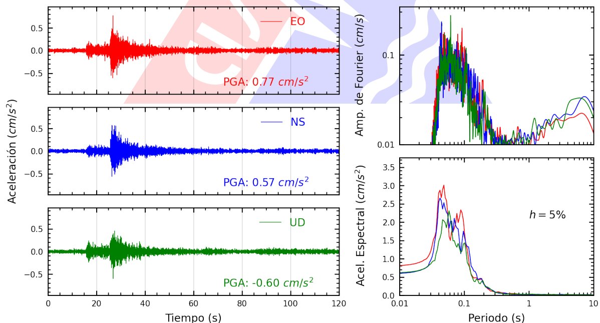
Figura A.18: Registros tiempo-historia, espectros de Fourier y de respuesta en las direcciones EO, NS y vertical de la estación URPPE. Sismo de Chilca, Cañete - Lima del 2025-08-23, 21:10:22 (Hora local)
