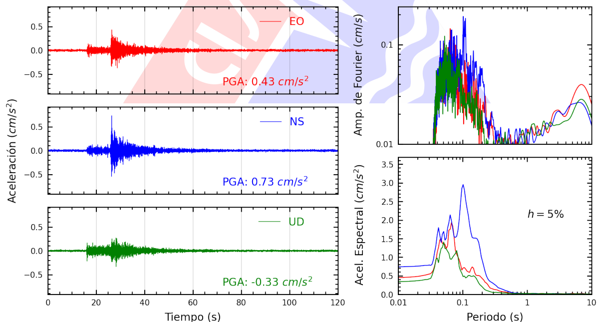
Figura A.20: Registros tiempo-historia, espectros de Fourier y de respuesta en las direcciones EO, NS y vertical de la estación SERVI. Sismo de Chilca, Cañete - Lima del 2025-08-23, 21:10:22 (Hora local)
