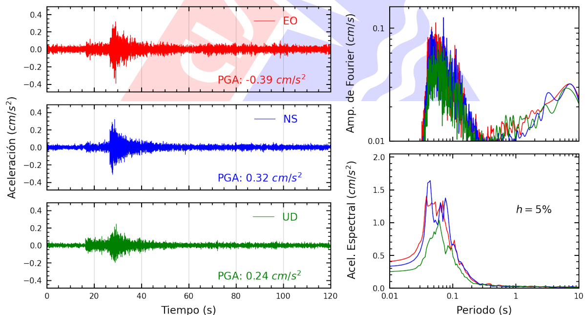
Figura A.24: Registros tiempo-historia, espectros de Fourier y de respuesta en las direcciones EO, NS y vertical de la estación INICT. Sismo de Chilca, Cañete - Lima del 2025-08-23, 21:10:22 (Hora local)
