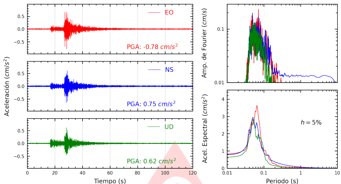
Figura A.15: Registros tiempo-historia, espectros de Fourier y de respuesta en las direcciones EO, NS y vertical de la estación ATARJ. Sismo de Chilca, Cañete - Lima del 2025-08-23, 21:10:22 (Hora local)
