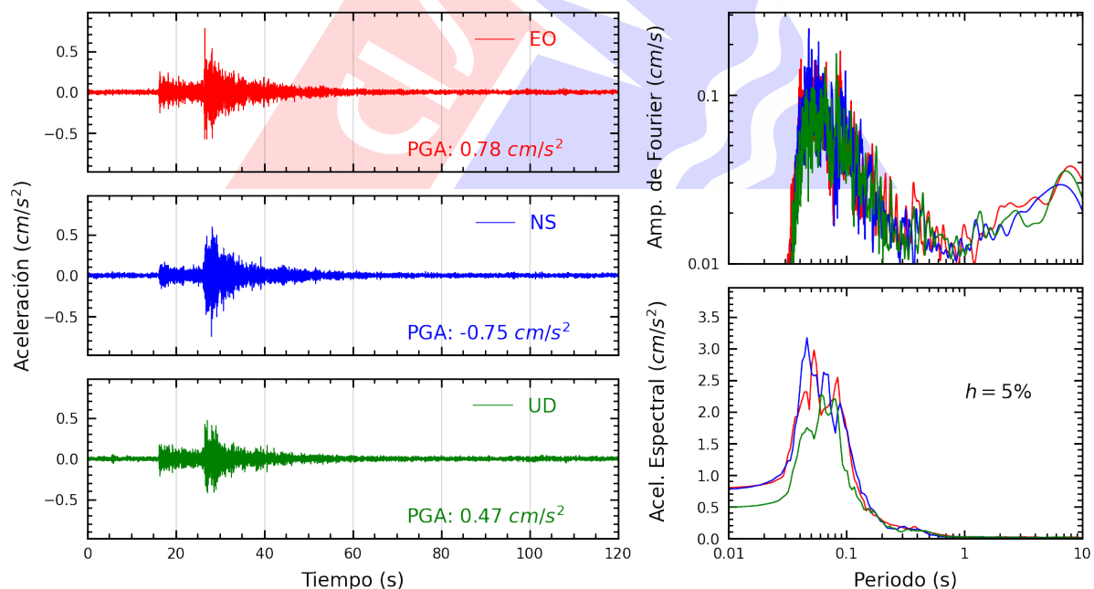
Figura A.14: Registros tiempo-historia, espectros de Fourier y de respuesta en las direcciones EO, NS y vertical de la estación IMCA. Sismo de Chilca, Cañete - Lima del 2025-08-23, 21:10:22 (Hora local)
