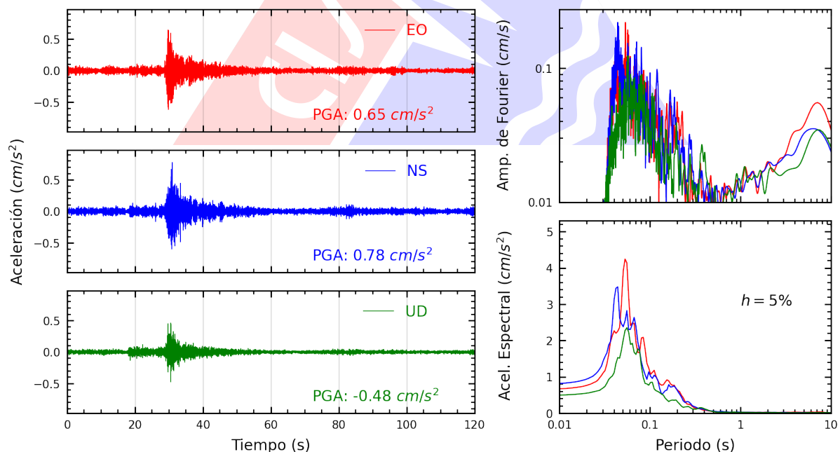
Figura A.16: Registros tiempo-historia, espectros de Fourier y de respuesta en las direcciones EO, NS y vertical de la estación COMAS. Sismo de Chilca, Cañete - Lima del 2025-08-23, 21:10:22 (Hora local)
