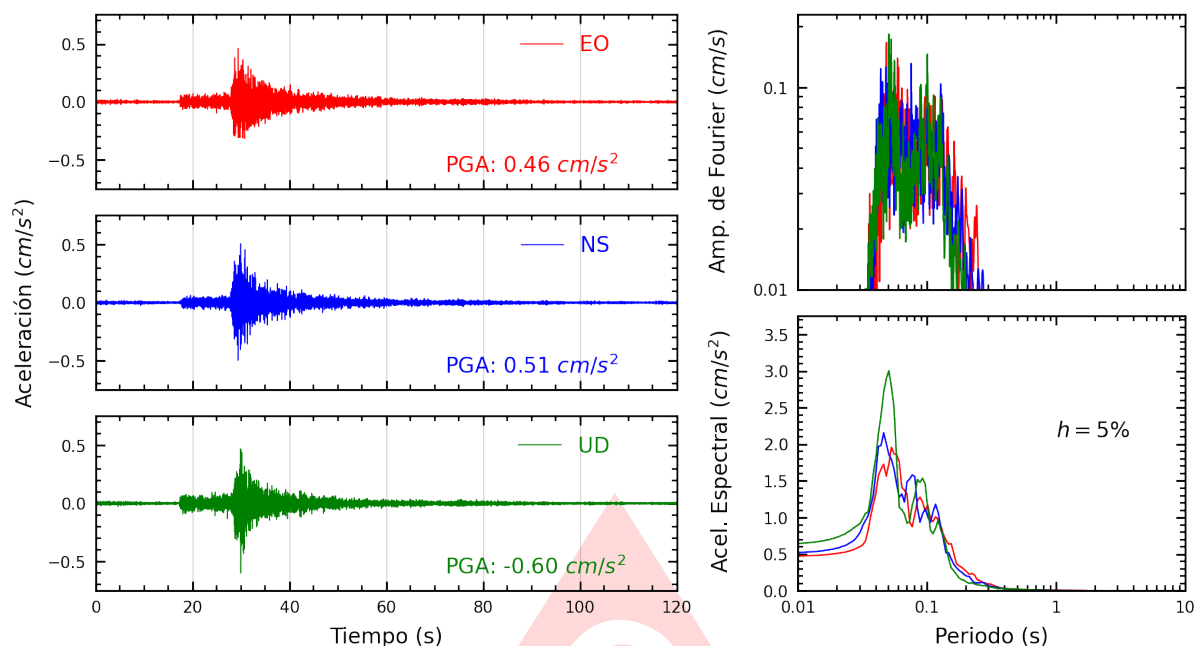
Figura A.21: Registros tiempo-historia, espectros de Fourier y de respuesta en las direcciones EO, NS y vertical de la estación JALV2. Sismo de Chilca, Cañete - Lima del 2025-08-23, 21:10:22 (Hora local)
