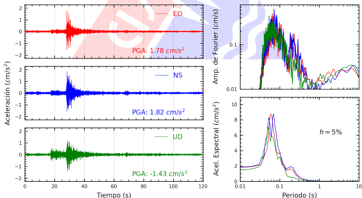
Figura A.4: Registros tiempo-historia, espectros de Fourier y de respuesta en las direcciones EO, NS y vertical de la estación SJLSC. Sismo de Chilca, Cañete - Lima del 2025-08-23, 21:10:22 (Hora local)
