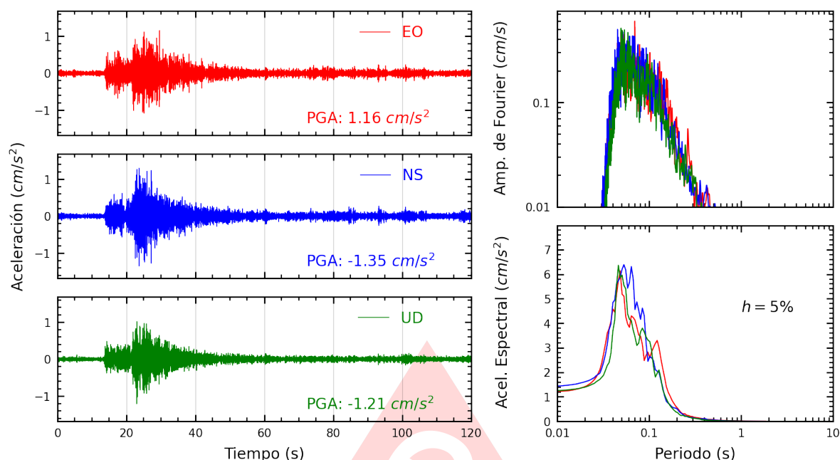
Figura A.7: Registros tiempo-historia, espectros de Fourier y de respuesta en las direcciones EO, NS y vertical de la estación PHERM. Sismo de Chilca, Cañete - Lima del 2025-08-23, 21:10:22 (Hora local)
