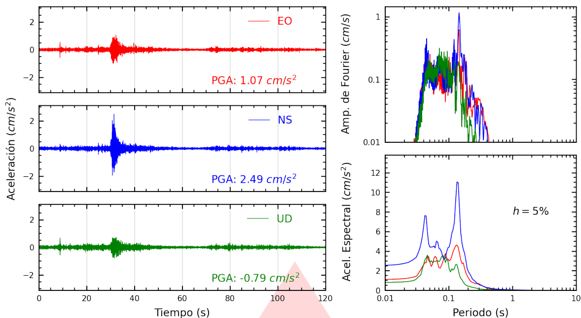
Figura A.1: Registros tiempo-historia, espectros de Fourier y de respuesta en las direcciones EO, NS y vertical de la estación CARAB. Sismo de Chilca, Cañete - Lima del 2025-08-23, 21:10:22 (Hora local)
