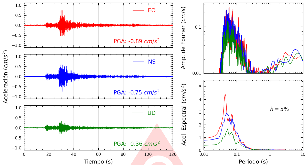
Figura A.9: Registros tiempo-historia, espectros de Fourier y de respuesta en las direcciones EO, NS y vertical de la estación FICPE. Sismo de Chilca, Cañete - Lima del 2025-08-23, 21:10:22 (Hora local)
