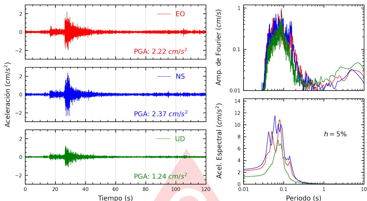
Figura A.3: Registros tiempo-historia, espectros de Fourier y de respuesta en las direcciones EO, NS y vertical de la estación USILM. Sismo de Chilca, Cañete - Lima del 2025-08-23, 21:10:22 (Hora local)
