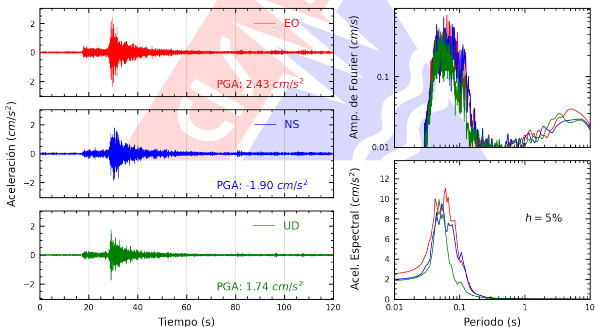
Figura A.2: Registros tiempo-historia, espectros de Fourier y de respuesta en las direcciones EO, NS y vertical de la estación JOSEO. Sismo de Chilca, Cañete - Lima del 2025-08-23, 21:10:22 (Hora local)
