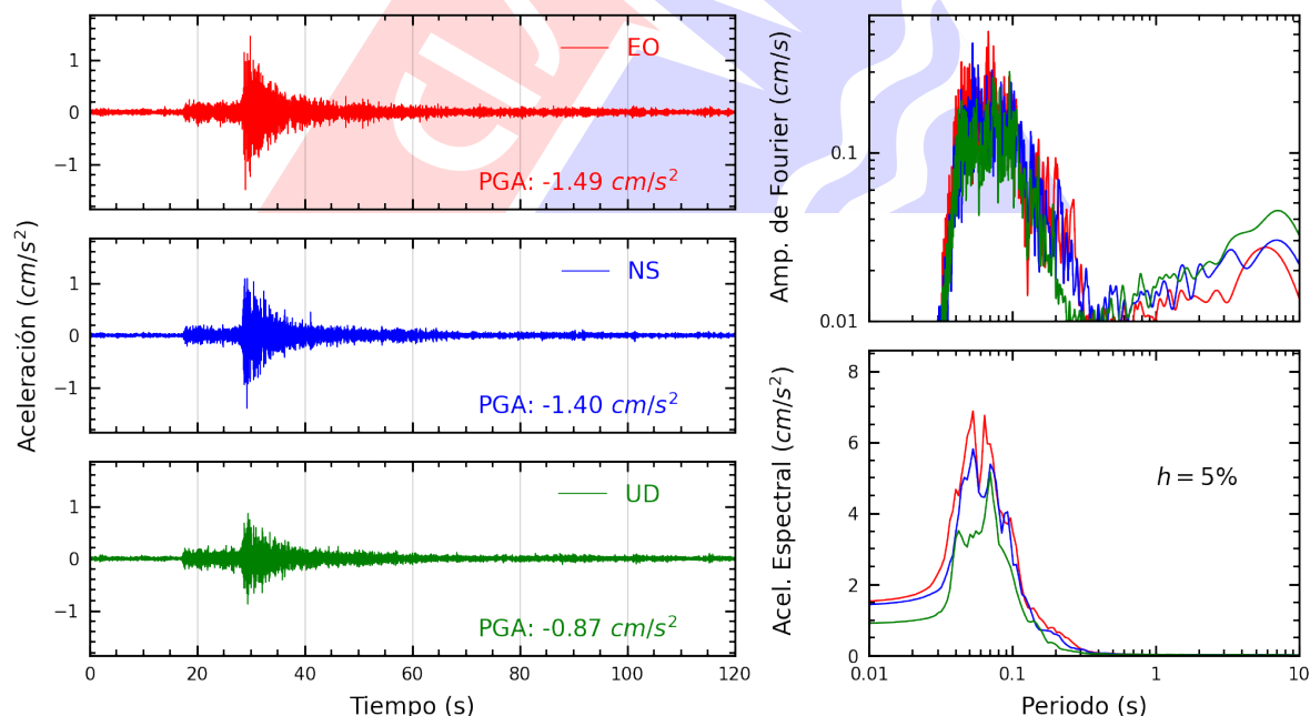
Figura A.6: Registros tiempo-historia, espectros de Fourier y de respuesta en las direcciones EO, NS y vertical de la estación INDEP. Sismo de Chilca, Cañete - Lima del 2025-08-23, 21:10:22 (Hora local)
