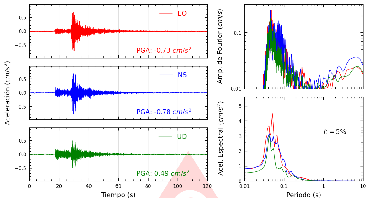
Figura A.17: Registros tiempo-historia, espectros de Fourier y de respuesta en las direcciones EO, NS y vertical de la estación SJLCE. Sismo de Chilca, Cañete - Lima del 2025-08-23, 21:10:22 (Hora local)
