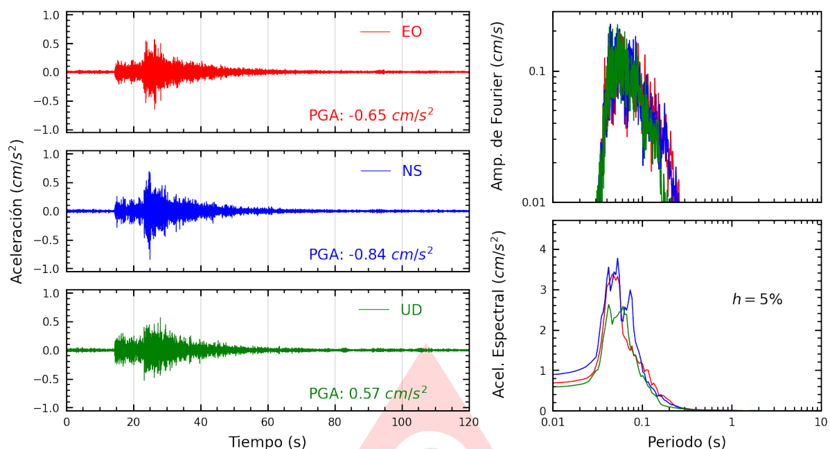
Figura A.11: Registros tiempo-historia, espectros de Fourier y de respuesta en las direcciones EO, NS y vertical de la estación ASIA. Sismo de Chilca, Cañete - Lima del 2025-08-23, 21:10:22 (Hora local)
