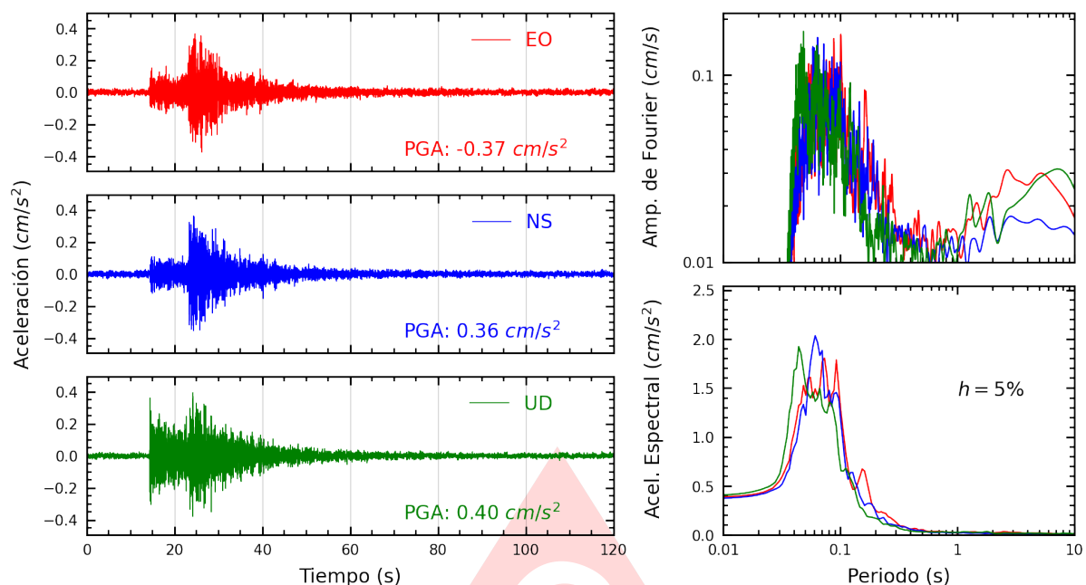
Figura A.23: Registros tiempo-historia, espectros de Fourier y de respuesta en las direcciones EO, NS y vertical de la estación USILP. Sismo de Chilca, Cañete - Lima del 2025-08-23, 21:10:22 (Hora local)
