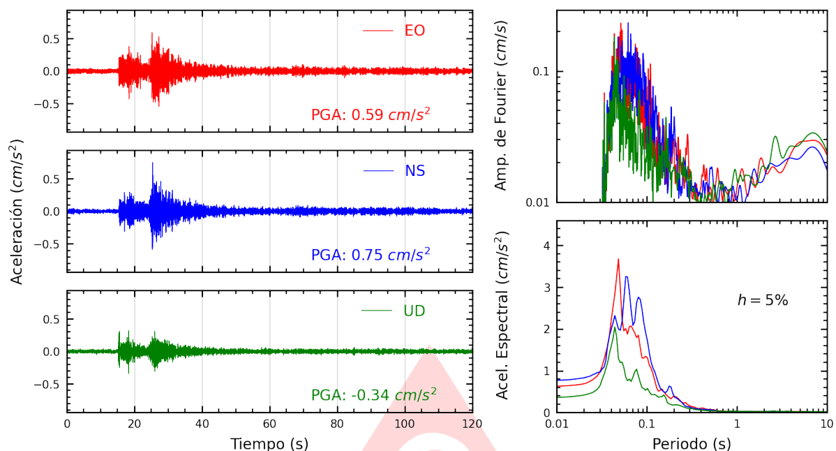
Figura A.19: Registros tiempo-historia, espectros de Fourier y de respuesta en las direcciones EO, NS y vertical de la estación UPCVI. Sismo de Chilca, Cañete - Lima del 2025-08-23, 21:10:22 (Hora local)
