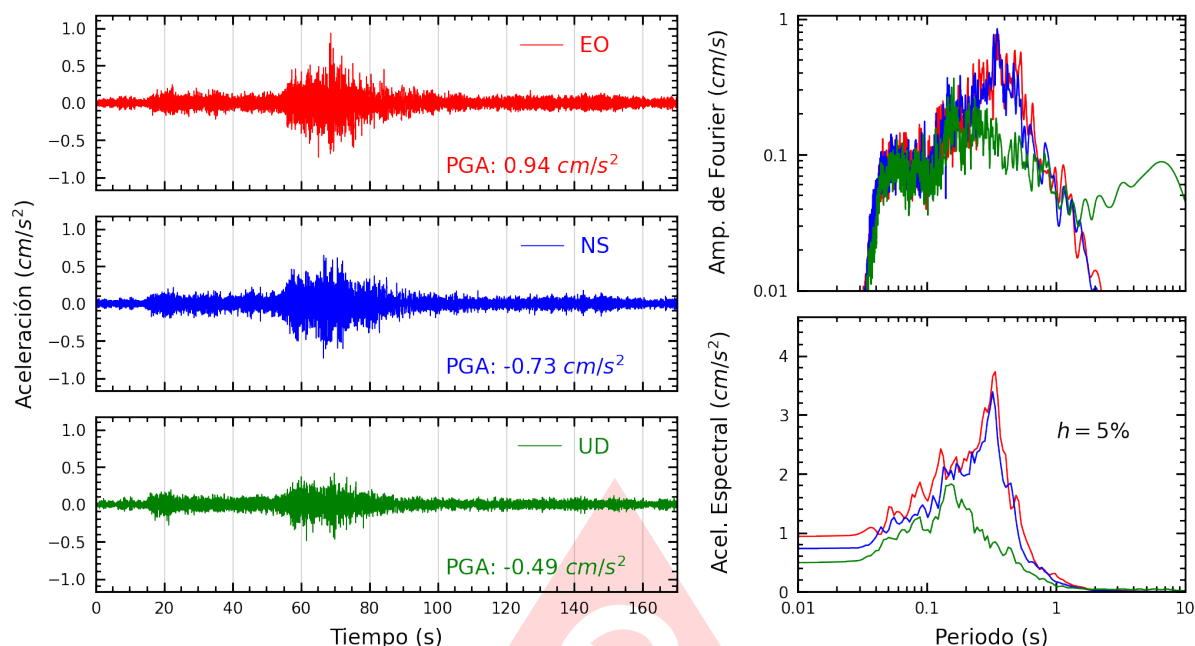
Figura A.5: Registros tiempo-historia, espectros de Fourier y de respuesta en las direcciones EO, NS y vertical de la estación SCARQ. Sismo de Tacna, Tacna - Tacna del 2025-08-23, 22:44:07 (Hora local)
