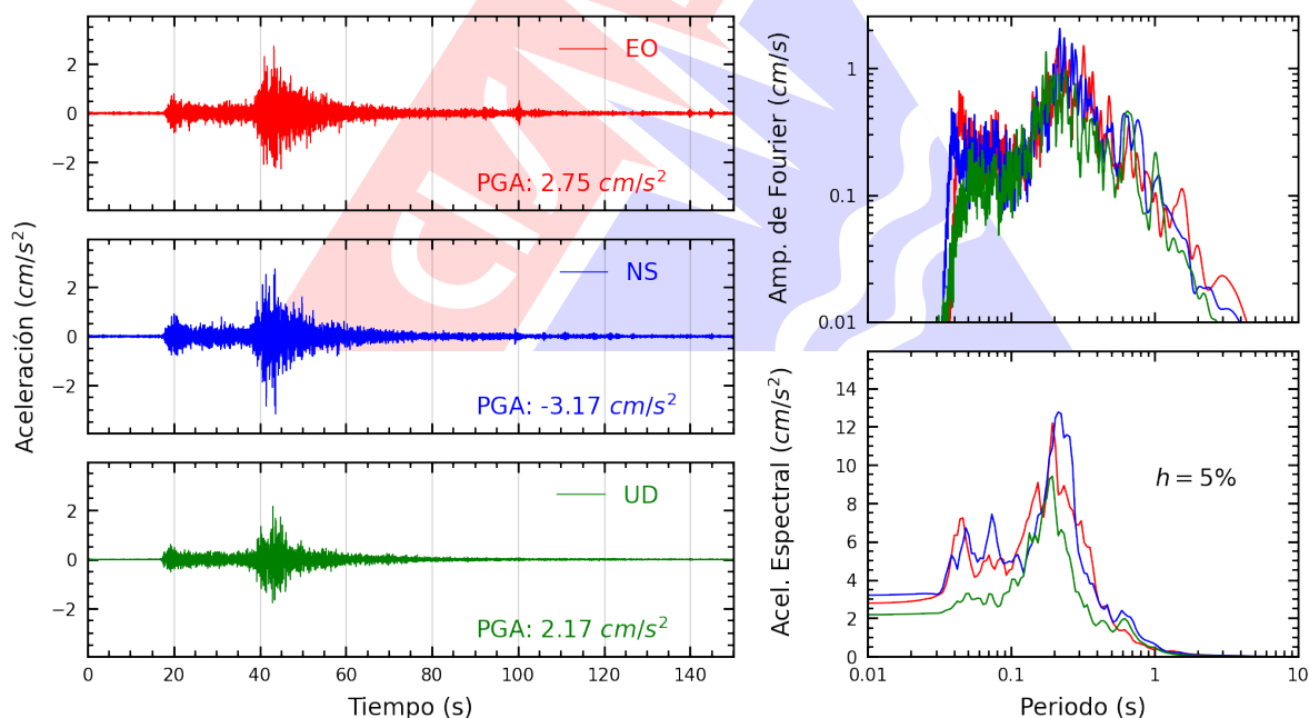
Figura A.2: Registros tiempo-historia, espectros de Fourier y de respuesta en las direcciones EO, NS y vertical de la estación UPTAC. Sismo de Tacna, Tacna - Tacna del 2025-08-23, 22:44:07 (Hora local)
