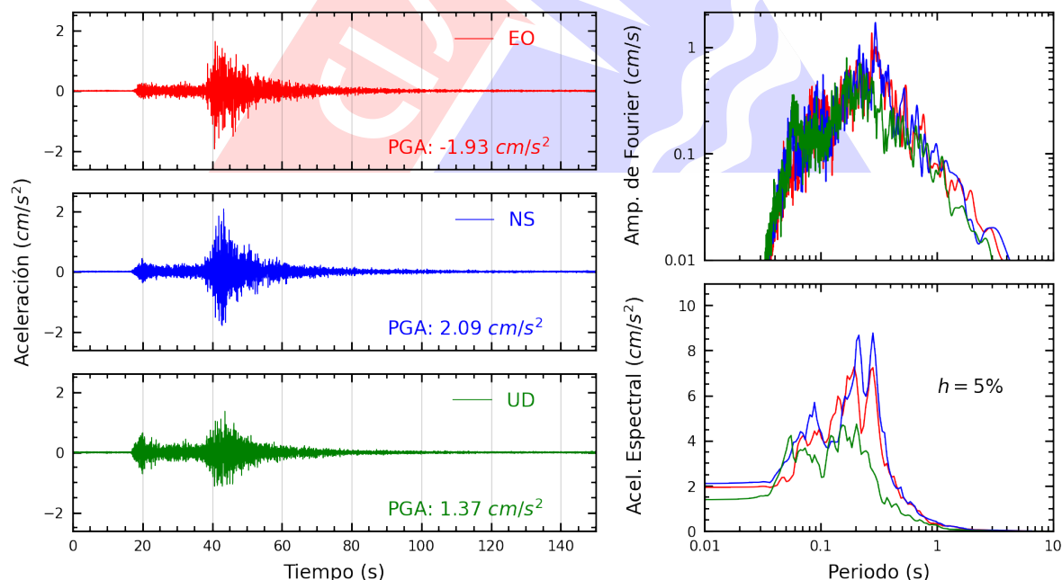
Figura A.4: Registros tiempo-historia, espectros de Fourier y de respuesta en las direcciones EO, NS y vertical de la estación UJBG2. Sismo de Tacna, Tacna - Tacna del 2025-08-23, 22:44:07 (Hora local)
