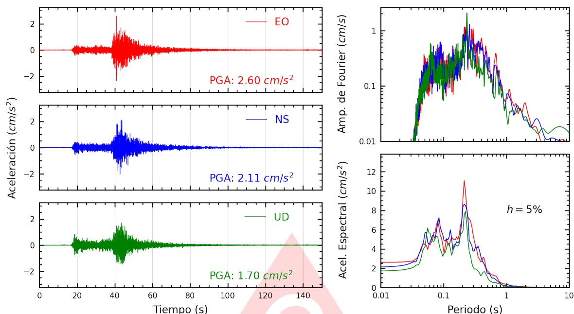
Figura A.3: Registros tiempo-historia, espectros de Fourier y de respuesta en las direcciones EO, NS y vertical de la estación CREY. Sismo de Tacna, Tacna - Tacna del 2025-08-23, 22:44:07 (Hora local)
