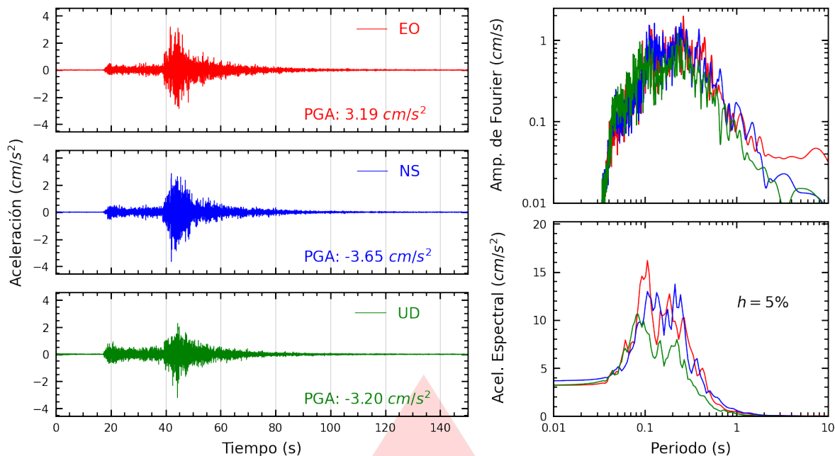
Figura A.1: Registros tiempo-historia, espectros de Fourier y de respuesta en las direcciones EO, NS y vertical de la estación UJBG3. Sismo de Tacna, Tacna - Tacna del 2025-08-23, 22:44:07 (Hora local)
