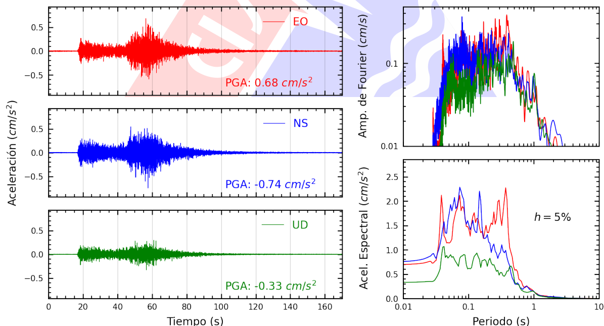
Figura A.6: Registros tiempo-historia, espectros de Fourier y de respuesta en las direcciones EO, NS y vertical de la estación UNAM. Sismo de Tacna, Tacna - Tacna del 2025-08-23, 22:44:07 (Hora local)
