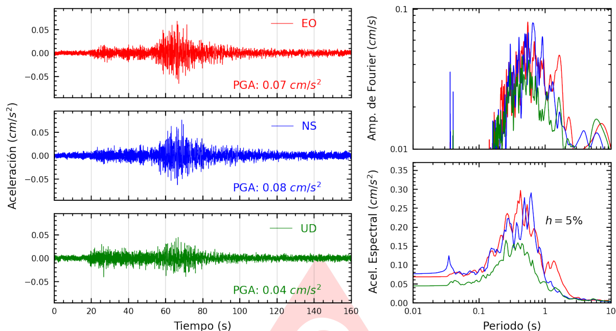
Figura A.3: Registros tiempo-historia, espectros de Fourier y de respuesta en las direcciones EO, NS y vertical de la estación UNJ. Sismo de Zorritos, Contralmirante Villar - Tumbes del 2025-08-26, 02:30:27 (Hora local)
