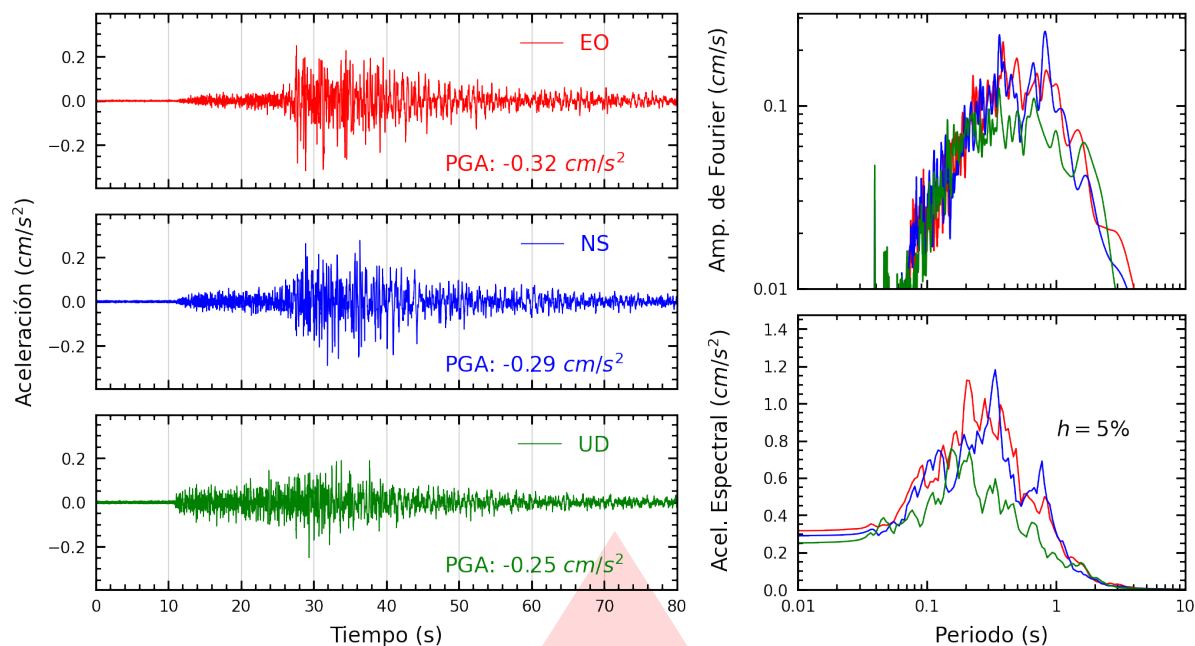
Figura A.1: Registros tiempo-historia, espectros de Fourier y de respuesta en las direcciones EO, NS y vertical de la estación UNF. Sismo de Zorritos, Contralmirante Villar - Tumbes del 2025-08-26, 02:30:27 (Hora local)
