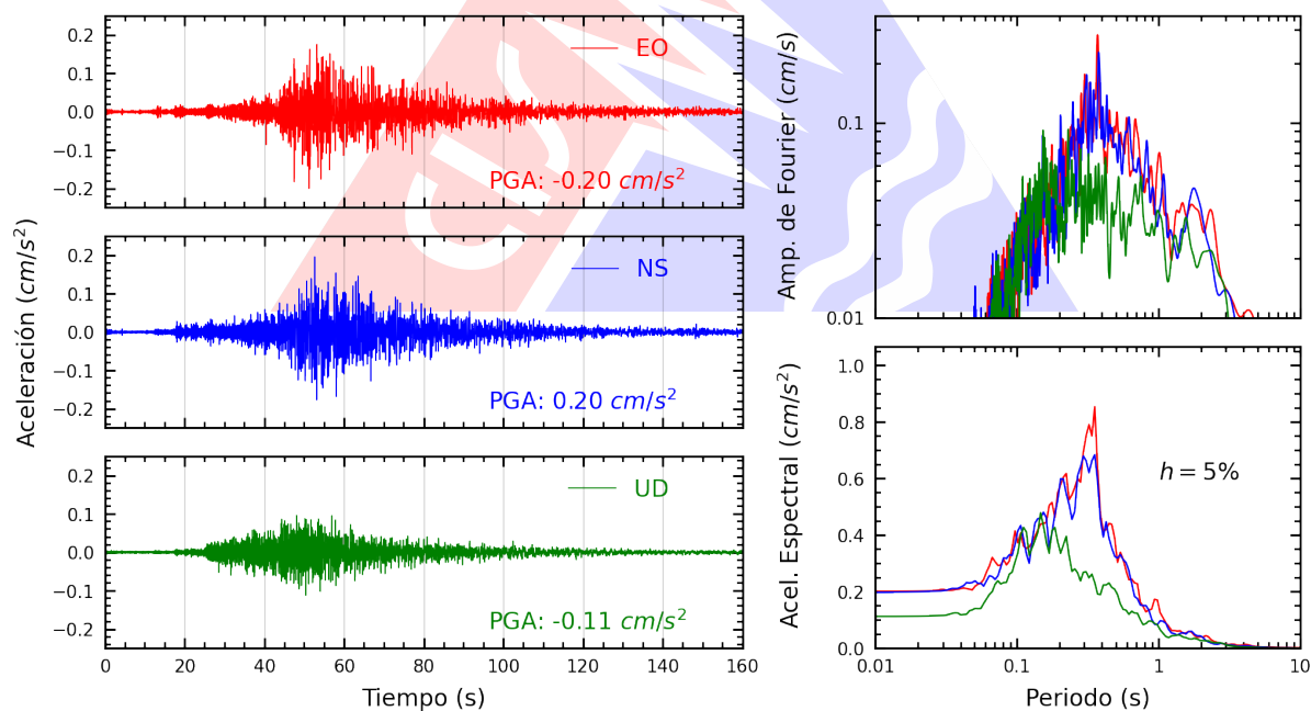
Figura A.2: Registros tiempo-historia, espectros de Fourier y de respuesta en las direcciones EO, NS y vertical de la estación UPAOP. Sismo de Zorritos, Contralmirante Villar - Tumbes del 2025-08-26, 02:30:27 (Hora local)
