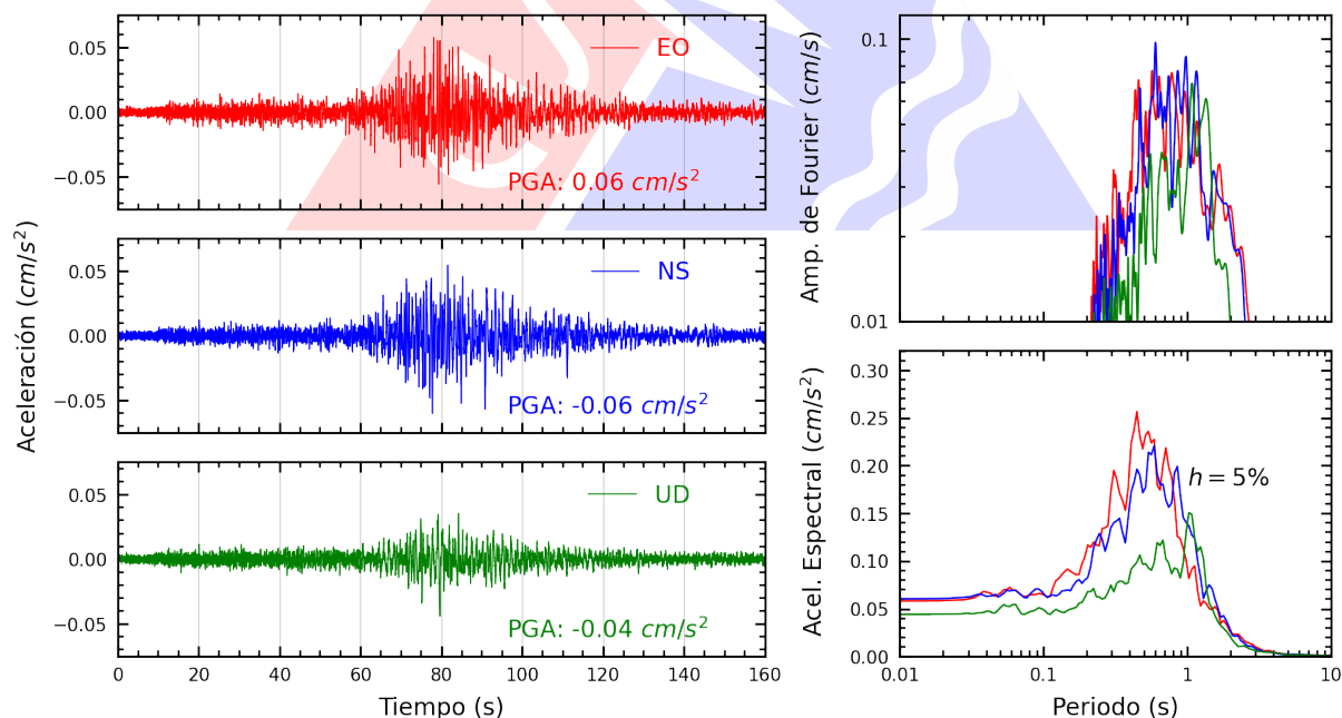
Figura A.4: Registros tiempo-historia, espectros de Fourier y de respuesta en las direcciones EO, NS y vertical de la estación UNC. Sismo de Zorritos, Contralmirante Villar - Tumbes del 2025-08-26, 02:30:27 (Hora local)
