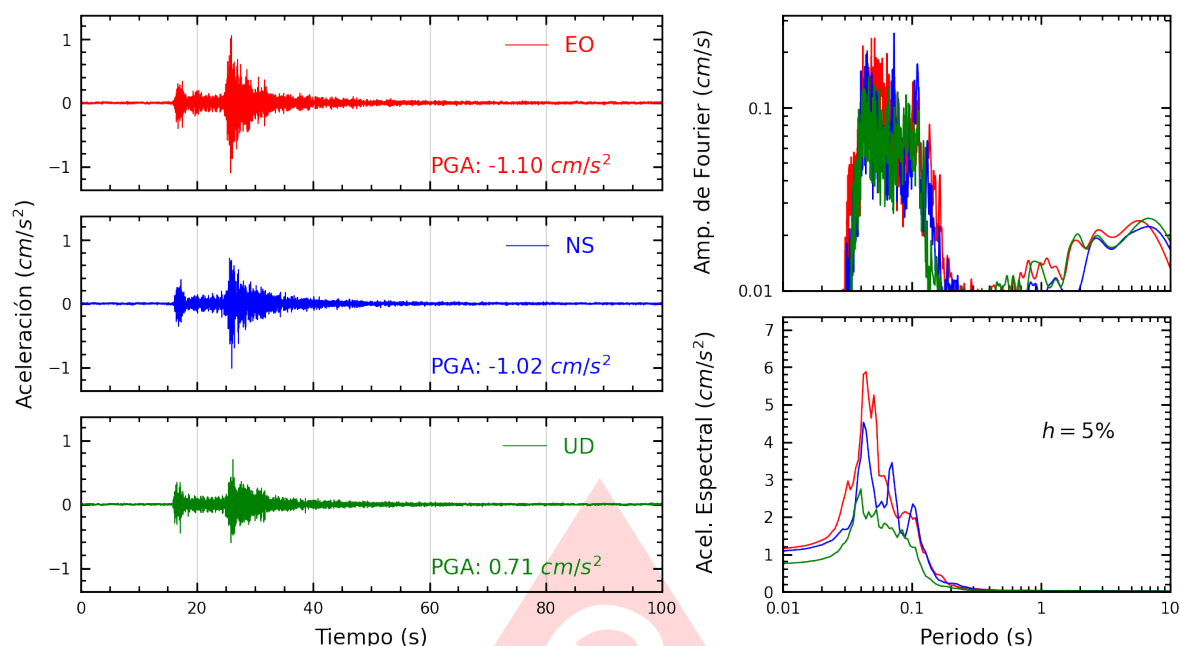
Figura A.7: Registros tiempo-historia, espectros de Fourier y de respuesta en las direcciones EO, NS y vertical de la estación AMORE. Sismo de Chilca, Cañete - Lima del 2025-08-26, 05:52:43 (Hora local)
