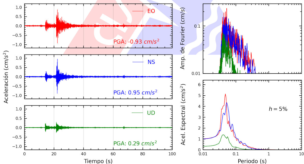
Figura A.10: Registros tiempo-historia, espectros de Fourier y de respuesta en las direcciones EO, NS y vertical de la estación UCVAT. Sismo de Chilca, Cañete - Lima del 2025-08-26, 05:52:43 (Hora local)
