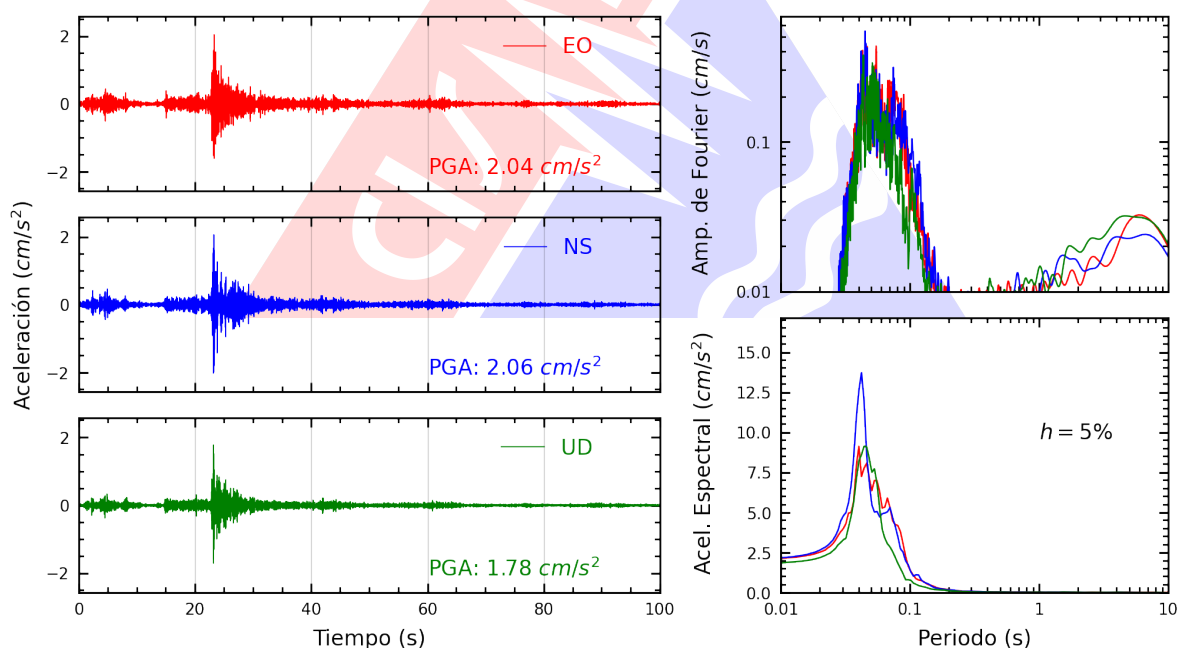
Figura A.2: Registros tiempo-historia, espectros de Fourier y de respuesta en las direcciones EO, NS y vertical de la estación JOSEO. Sismo de Chilca, Cañete - Lima del 2025-08-26, 05:52:43 (Hora local)
