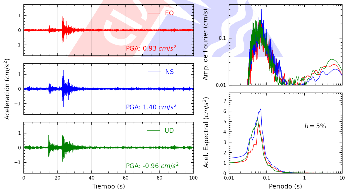
Figura A.6: Registros tiempo-historia, espectros de Fourier y de respuesta en las direcciones EO, NS y vertical de la estación SJLSC. Sismo de Chilca, Cañete - Lima del 2025-08-26, 05:52:43 (Hora local)
