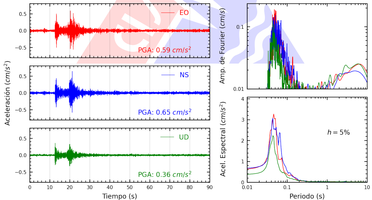
Figura A.16: Registros tiempo-historia, espectros de Fourier y de respuesta en las direcciones EO, NS y vertical de la estación UPCVI. Sismo de Chilca, Cañete - Lima del 2025-08-26, 05:52:43 (Hora local)
