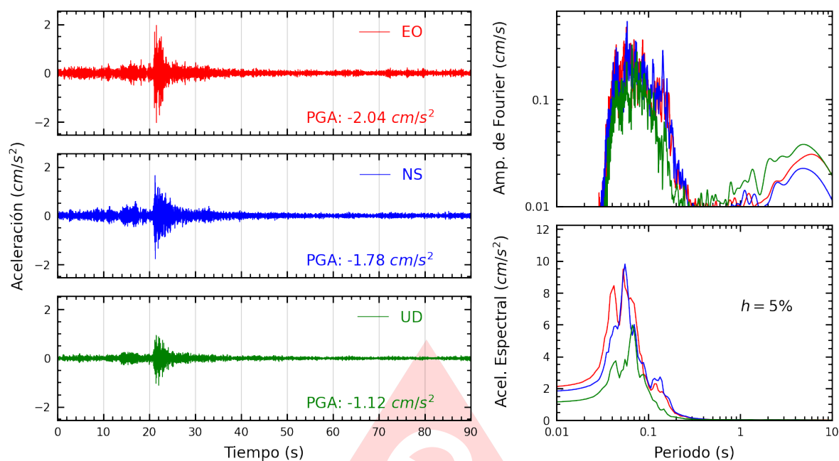
Figura A.3: Registros tiempo-historia, espectros de Fourier y de respuesta en las direcciones EO, NS y vertical de la estación USILM. Sismo de Chilca, Cañete - Lima del 2025-08-26, 05:52:43 (Hora local)
