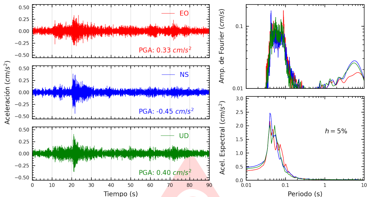
Figura A.21: Registros tiempo-historia, espectros de Fourier y de respuesta en las direcciones EO, NS y vertical de la estación URPPE. Sismo de Chilca, Cañete - Lima del 2025-08-26, 05:52:43 (Hora local)
