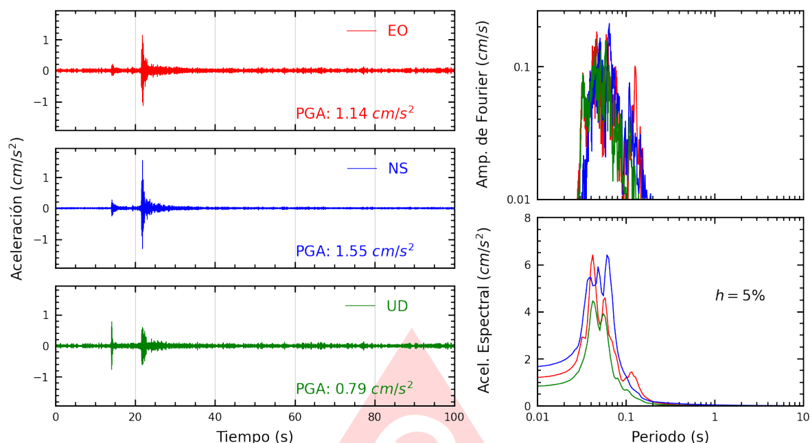
Figura A.5: Registros tiempo-historia, espectros de Fourier y de respuesta en las direcciones EO, NS y vertical de la estación ATARJ. Sismo de Chilca, Cañete - Lima del 2025-08-26, 05:52:43 (Hora local)
