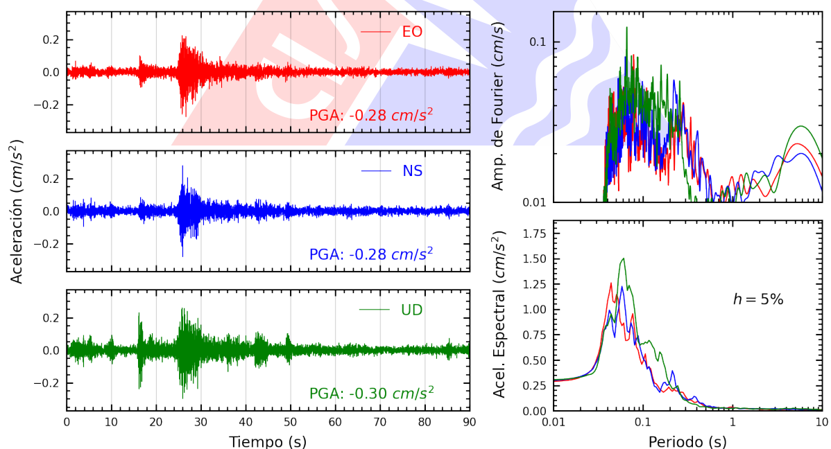
Figura A.24: Registros tiempo-historia, espectros de Fourier y de respuesta en las direcciones EO, NS y vertical de la estación MDPP. Sismo de Chilca, Cañete - Lima del 2025-08-26, 05:52:43 (Hora local)
