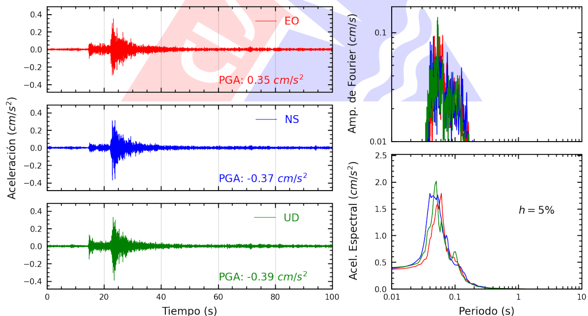
Figura A.22: Registros tiempo-historia, espectros de Fourier y de respuesta en las direcciones EO, NS y vertical de la estación JALV2. Sismo de Chilca, Cañete - Lima del 2025-08-26, 05:52:43 (Hora local)
