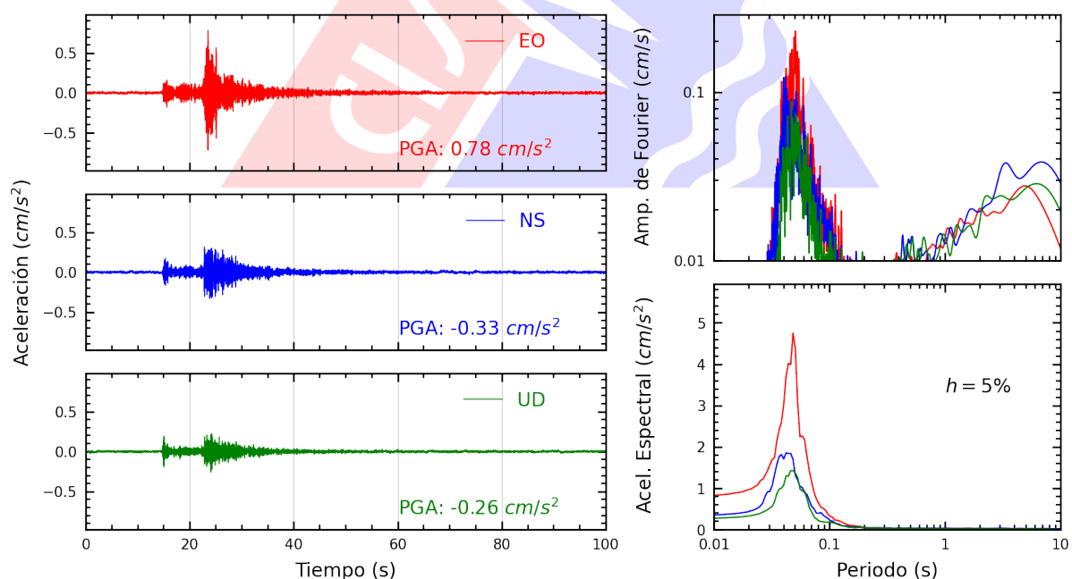
Figura A.12: Registros tiempo-historia, espectros de Fourier y de respuesta en las direcciones EO, NS y vertical de la estación UCSS. Sismo de Chilca, Cañete - Lima del 2025-08-26, 05:52:43 (Hora local)
