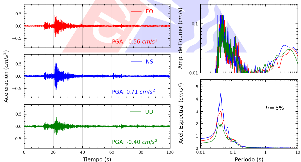
Figura A.14: Registros tiempo-historia, espectros de Fourier y de respuesta en las direcciones EO, NS y vertical de la estación USMP. Sismo de Chilca, Cañete - Lima del 2025-08-26, 05:52:43 (Hora local)
