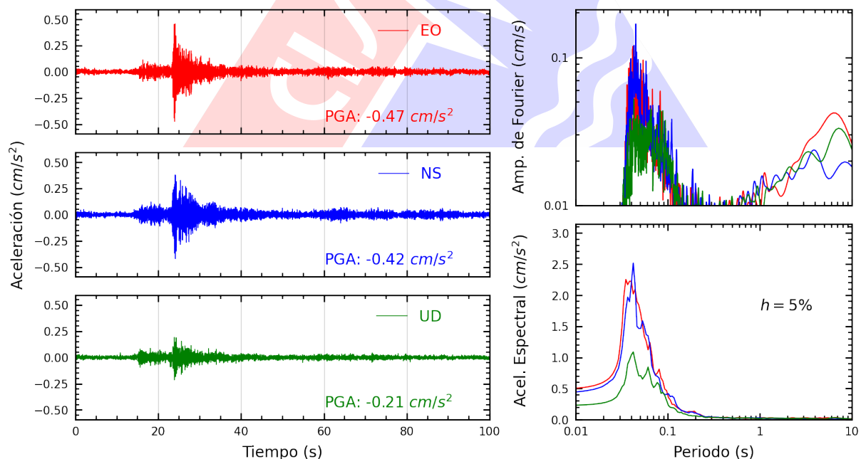
Figura A.20: Registros tiempo-historia, espectros de Fourier y de respuesta en las direcciones EO, NS y vertical de la estación COMAS. Sismo de Chilca, Cañete - Lima del 2025-08-26, 05:52:43 (Hora local)
