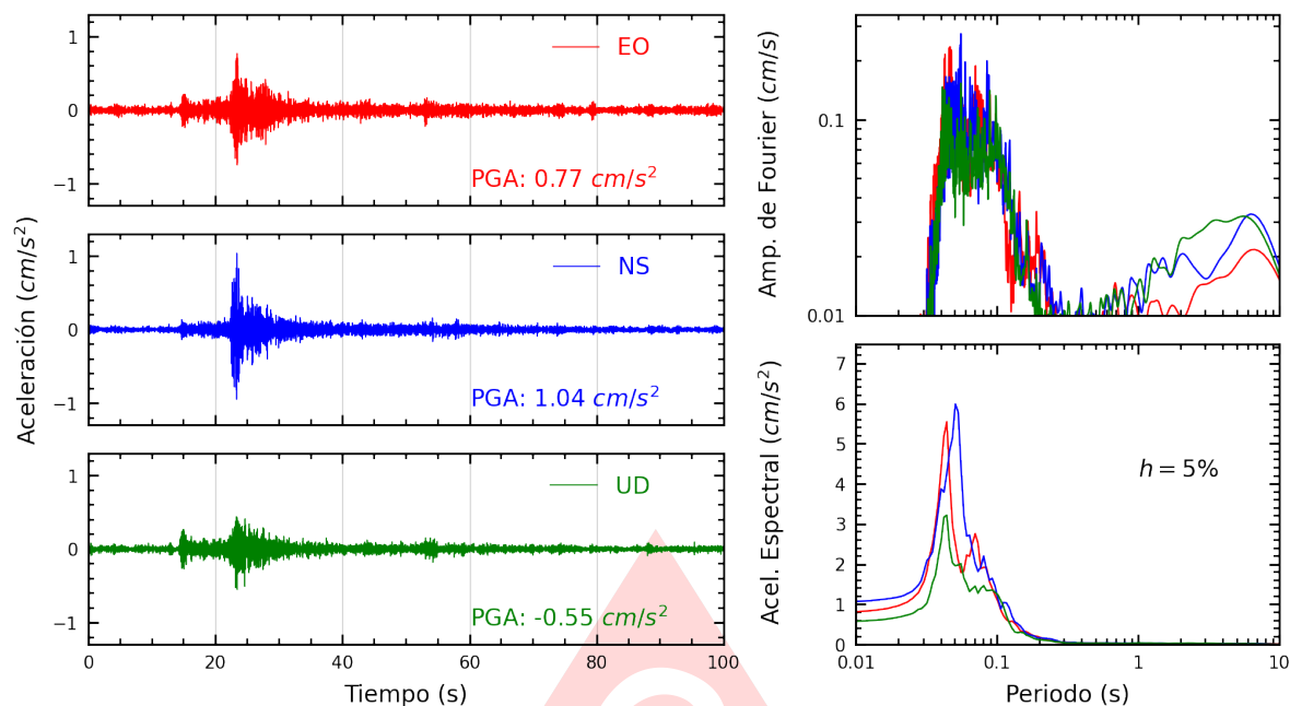
Figura A.9: Registros tiempo-historia, espectros de Fourier y de respuesta en las direcciones EO, NS y vertical de la estación INDEP. Sismo de Chilca, Cañete - Lima del 2025-08-26, 05:52:43 (Hora local)
