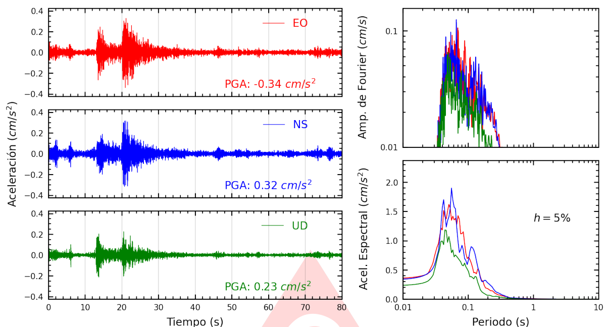
Figura A.23: Registros tiempo-historia, espectros de Fourier y de respuesta en las direcciones EO, NS y vertical de la estación BRIS2. Sismo de Chilca, Cañete - Lima del 2025-08-26, 05:52:43 (Hora local)
