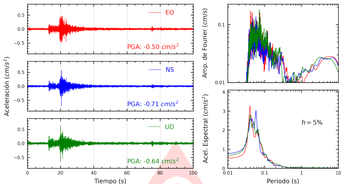
Figura A.13: Registros tiempo-historia, espectros de Fourier y de respuesta en las direcciones EO, NS y vertical de la estación SOVES. Sismo de Chilca, Cañete - Lima del 2025-08-26, 05:52:43 (Hora local)
