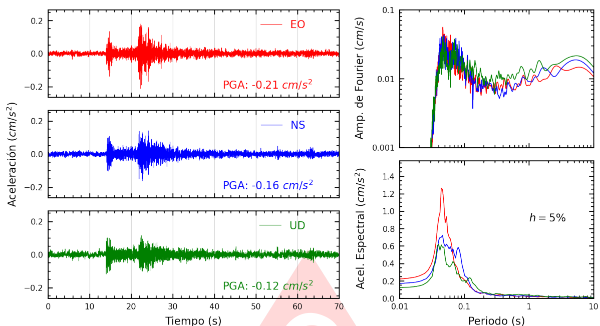
Figura A.25: Registros tiempo-historia, espectros de Fourier y de respuesta en las direcciones EO, NS y vertical de la estación UNFV. Sismo de Chilca, Cañete - Lima del 2025-08-26, 05:52:43 (Hora local)
