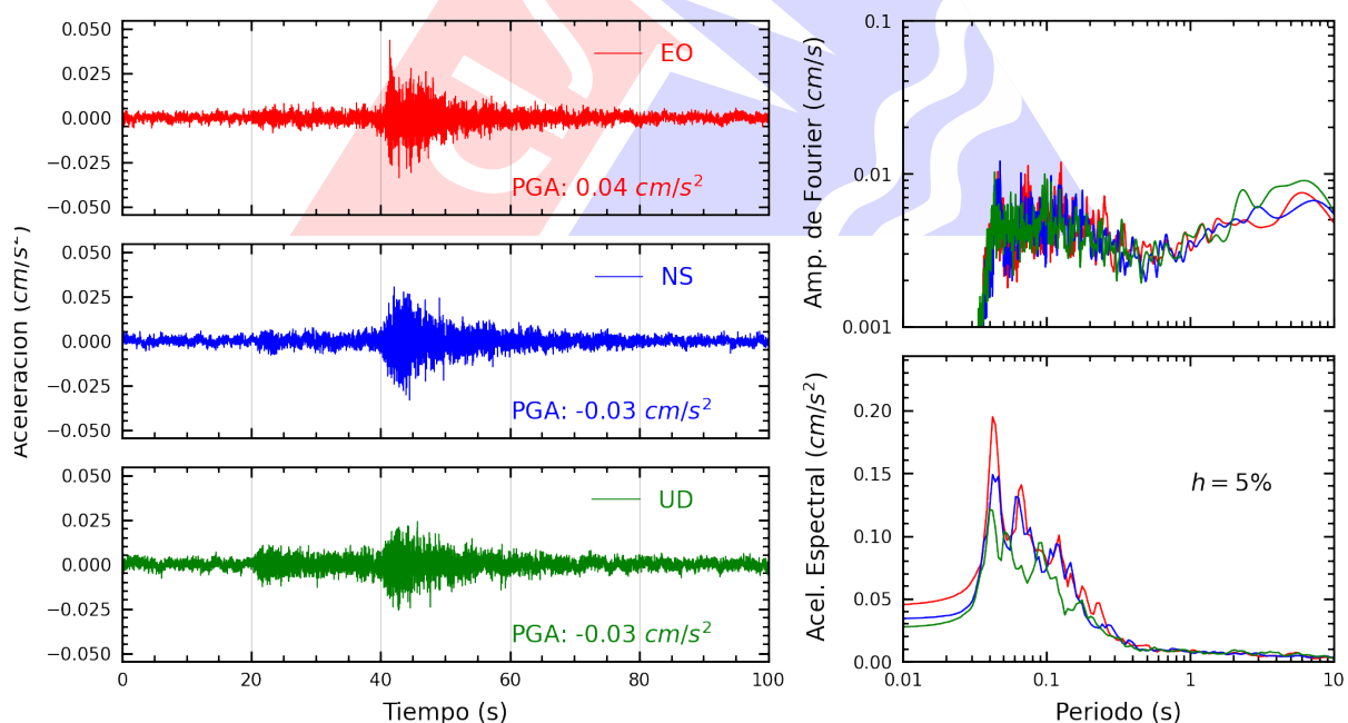
Figura A.26: Registros tiempo-historia, espectros de Fourier y de respuesta en las direcciones EO, NS y vertical de la estación CARAL. Sismo de Chilca, Cañete - Lima del 2025-08-26, 05:52:43 (Hora local)
