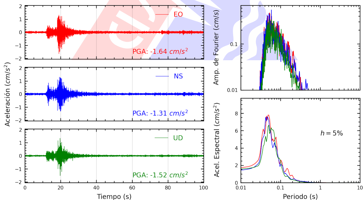
Figura A.4: Registros tiempo-historia, espectros de Fourier y de respuesta en las direcciones EO, NS y vertical de la estación PHERM. Sismo de Chilca, Cañete - Lima del 2025-08-26, 05:52:43 (Hora local)
