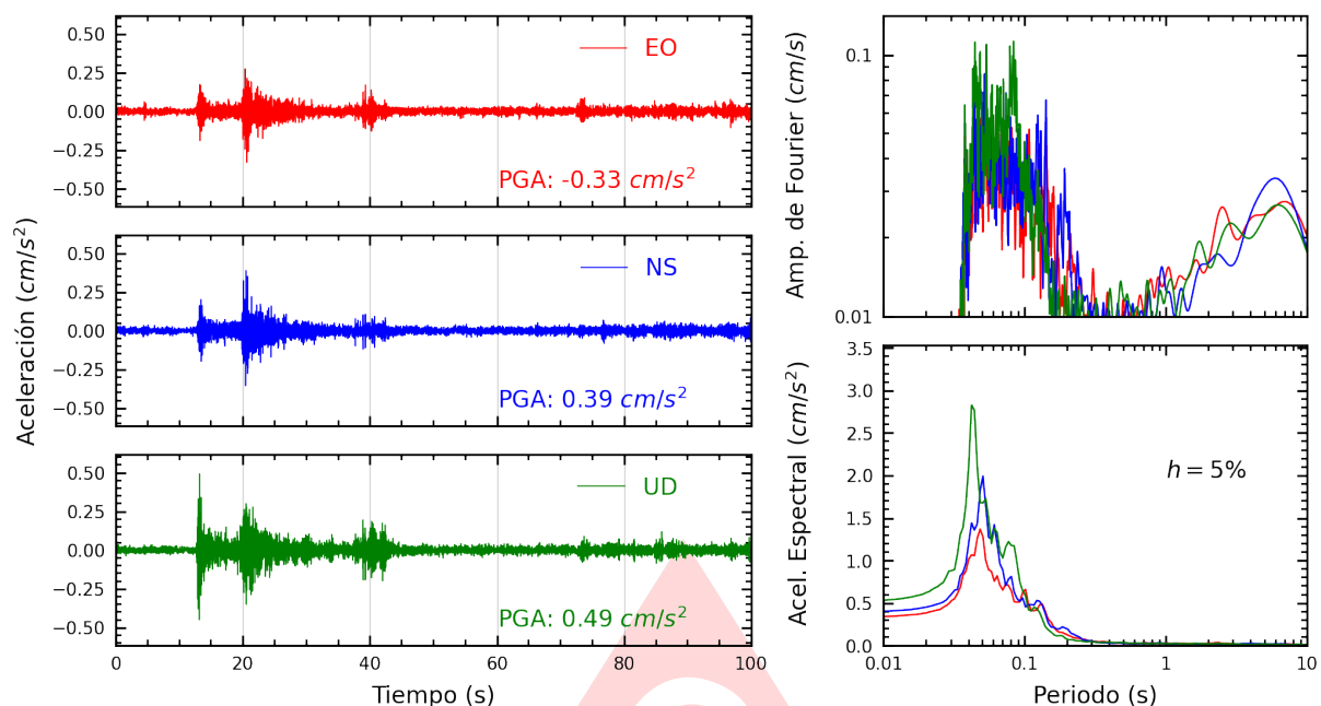
Figura A.19: Registros tiempo-historia, espectros de Fourier y de respuesta en las direcciones EO, NS y vertical de la estación SOCHO. Sismo de Chilca, Cañete - Lima del 2025-08-26, 05:52:43 (Hora local)
