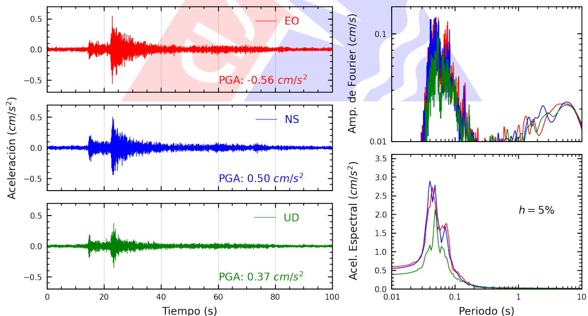
Figura A.18: Registros tiempo-historia, espectros de Fourier y de respuesta en las direcciones EO, NS y vertical de la estación FICPE. Sismo de Chilca, Cañete - Lima del 2025-08-26, 05:52:43 (Hora local)
