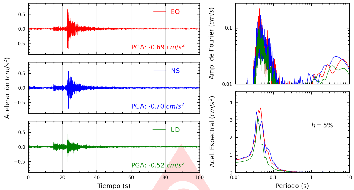
Figura A.15: Registros tiempo-historia, espectros de Fourier y de respuesta en las direcciones EO, NS y vertical de la estación SJLCE. Sismo de Chilca, Cañete - Lima del 2025-08-26, 05:52:43 (Hora local)
