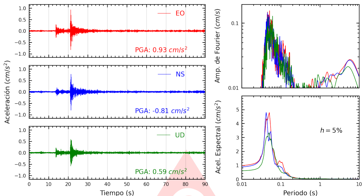
Figura A.11: Registros tiempo-historia, espectros de Fourier y de respuesta en las direcciones EO, NS y vertical de la estación IMCA. Sismo de Chilca, Cañete - Lima del 2025-08-26, 05:52:43 (Hora local)
