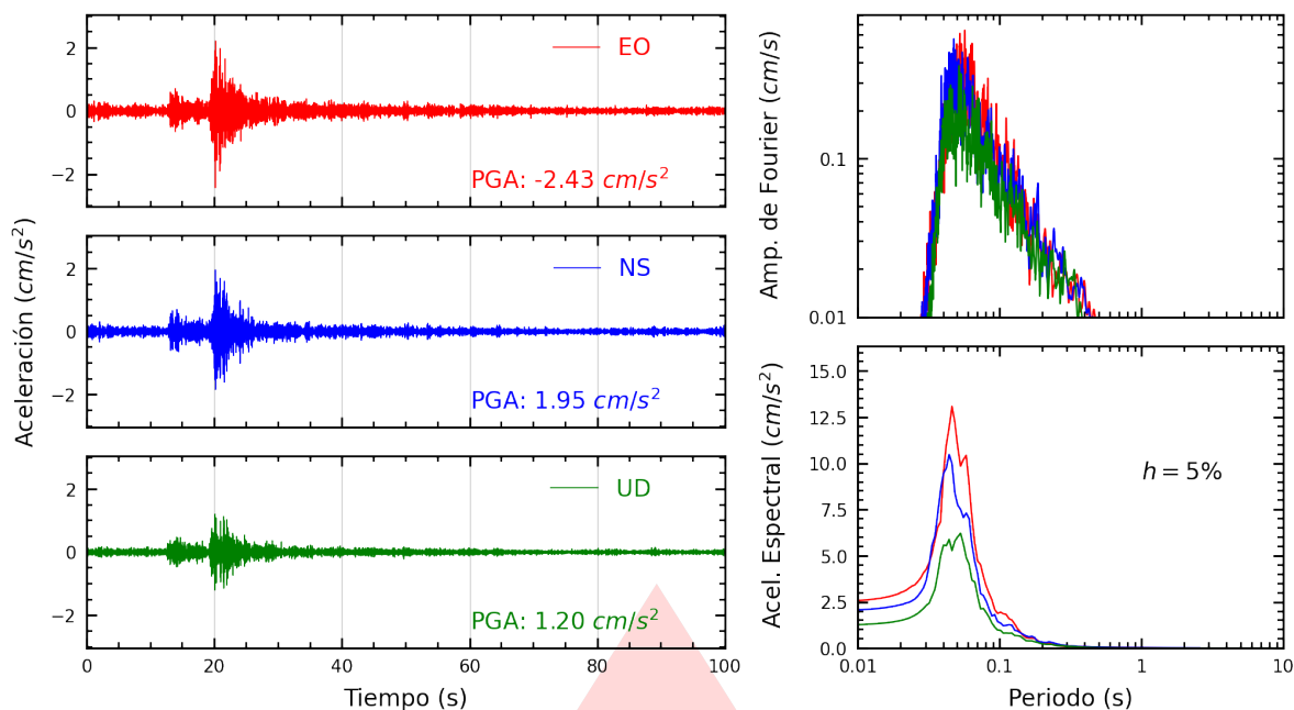
Figura A.1: Registros tiempo-historia, espectros de Fourier y de respuesta en las direcciones EO, NS y vertical de la estación UNTEL. Sismo de Chilca, Cañete - Lima del 2025-08-26, 05:52:43 (Hora local)
