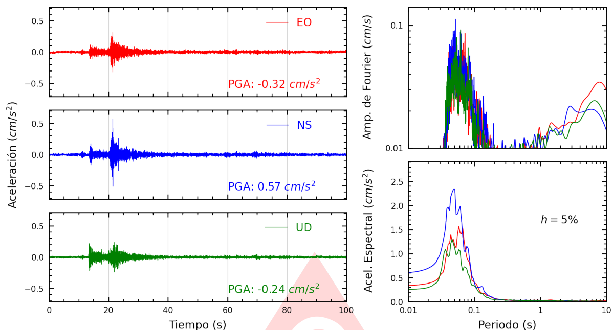
Figura A.17: Registros tiempo-historia, espectros de Fourier y de respuesta en las direcciones EO, NS y vertical de la estación SERVI. Sismo de Chilca, Cañete - Lima del 2025-08-26, 05:52:43 (Hora local)
