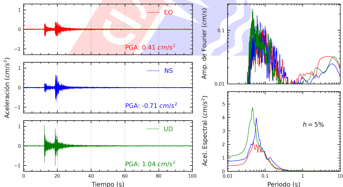
Figura A.8: Registros tiempo-historia, espectros de Fourier y de respuesta en las direcciones EO, NS y vertical de la estación USILP. Sismo de Chilca, Cañete - Lima del 2025-08-26, 05:52:43 (Hora local)
