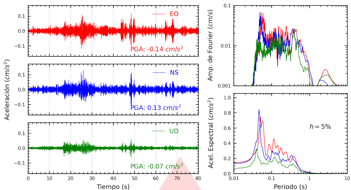
Figura A.1: Registros tiempo-historia, espectros de Fourier y de respuesta en las direcciones EO, NS y vertical de la estación UNMBA. Sismo de Limatambo, Anta - Cusco del 2025-08-26, 19:53:56 (Hora local)
