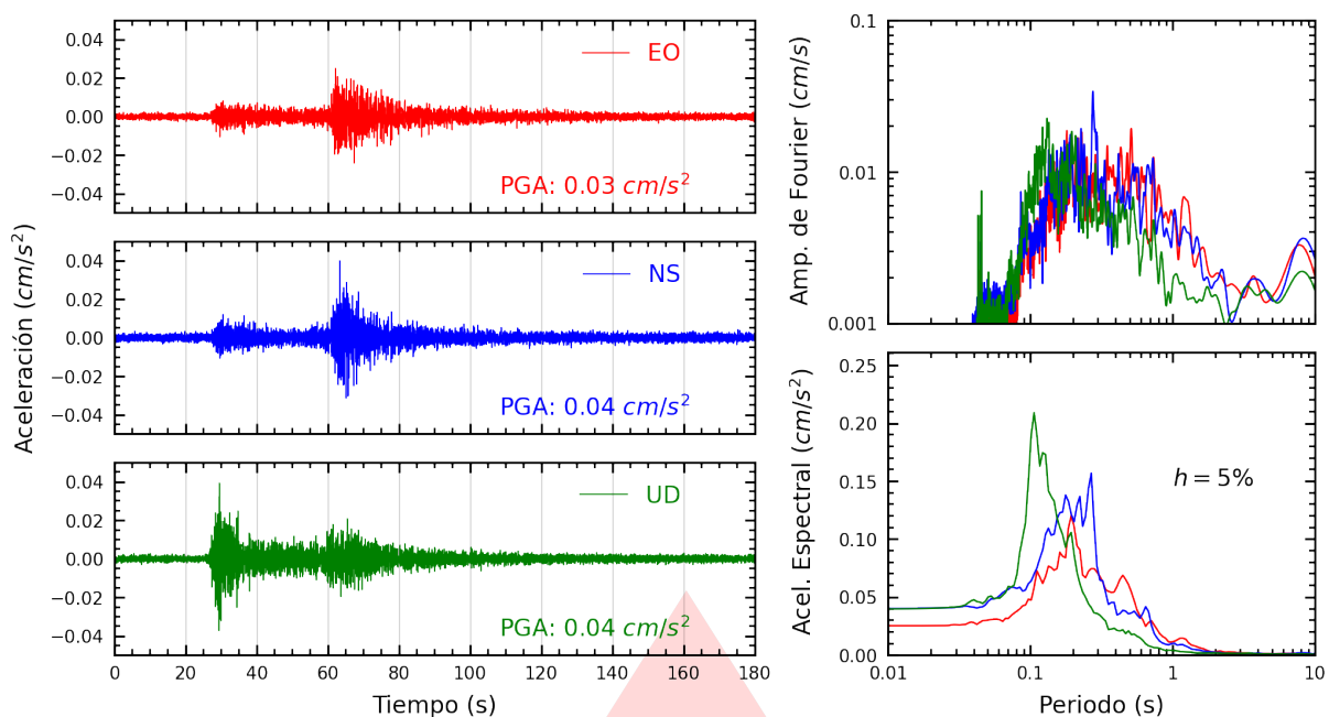
Figura A.1: Registros tiempo-historia, espectros de Fourier y de respuesta en las direcciones EO, NS y vertical de la estación UNIA. Sismo de Villa Rica, Oxapampa - Pasco del 2025-08-29, 23:40:33 (Hora local)
