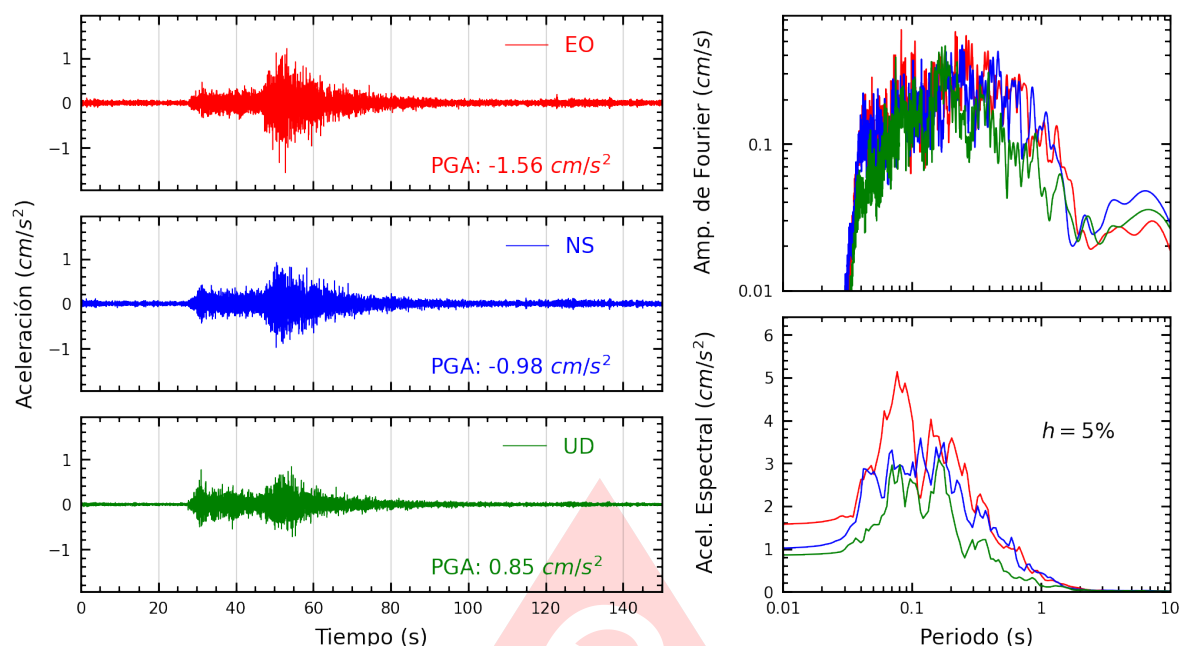
Figura A.31: Registros tiempo-historia, espectros de Fourier y de respuesta en las direcciones EO, NS y vertical de la estación CEPRE. Sismo de Pisco, Pisco - Ica del 2025-09-02, 14:50:09 (Hora local)
