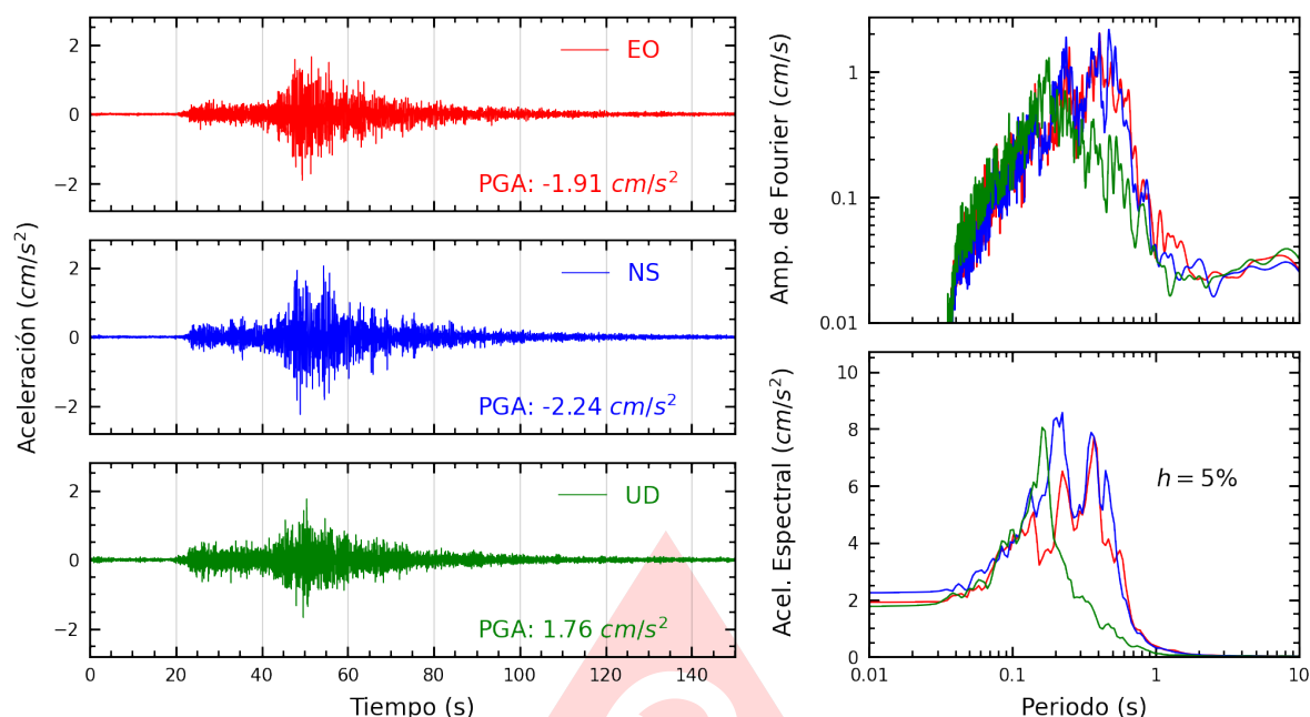
Figura A.21: Registros tiempo-historia, espectros de Fourier y de respuesta en las direcciones EO, NS y vertical de la estación MDPP. Sismo de Pisco, Pisco - Ica del 2025-09-02, 14:50:09 (Hora local)
