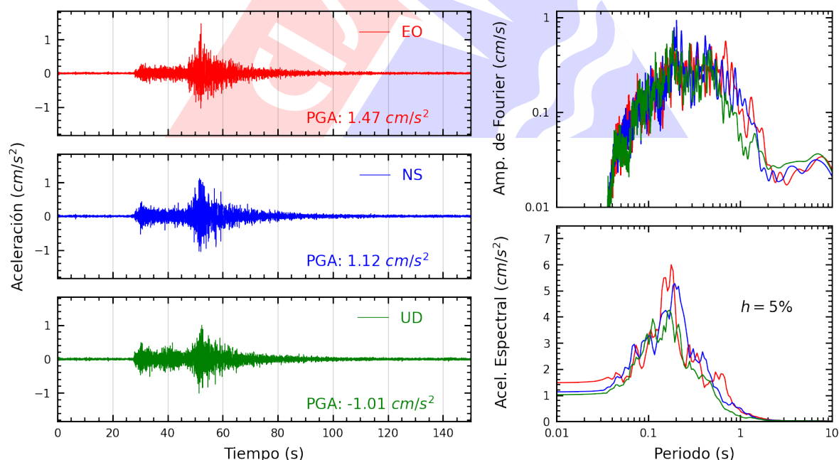
Figura A.34: Registros tiempo-historia, espectros de Fourier y de respuesta en las direcciones EO, NS y vertical de la estación UNFV. Sismo de Pisco, Pisco - Ica del 2025-09-02, 14:50:09 (Hora local)
