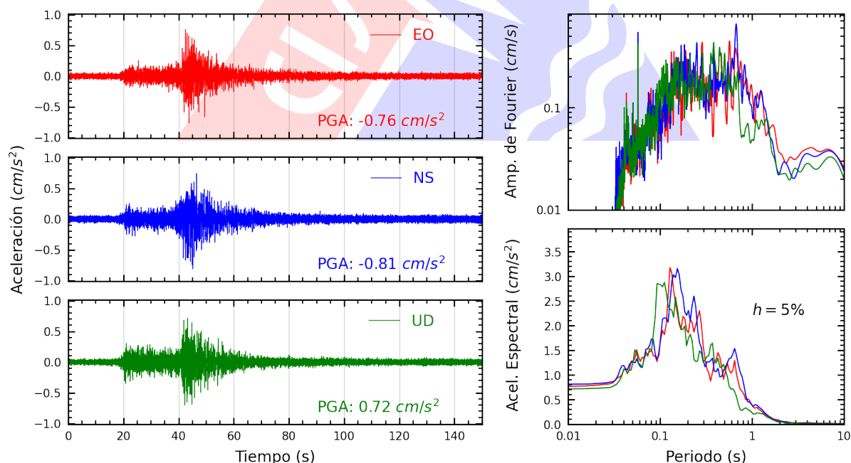
Figura A.42: Registros tiempo-historia, espectros de Fourier y de respuesta en las direcciones EO, NS y vertical de la estación BONDY. Sismo de Pisco, Pisco - Ica del 2025-09-02, 14:50:09 (Hora local)
