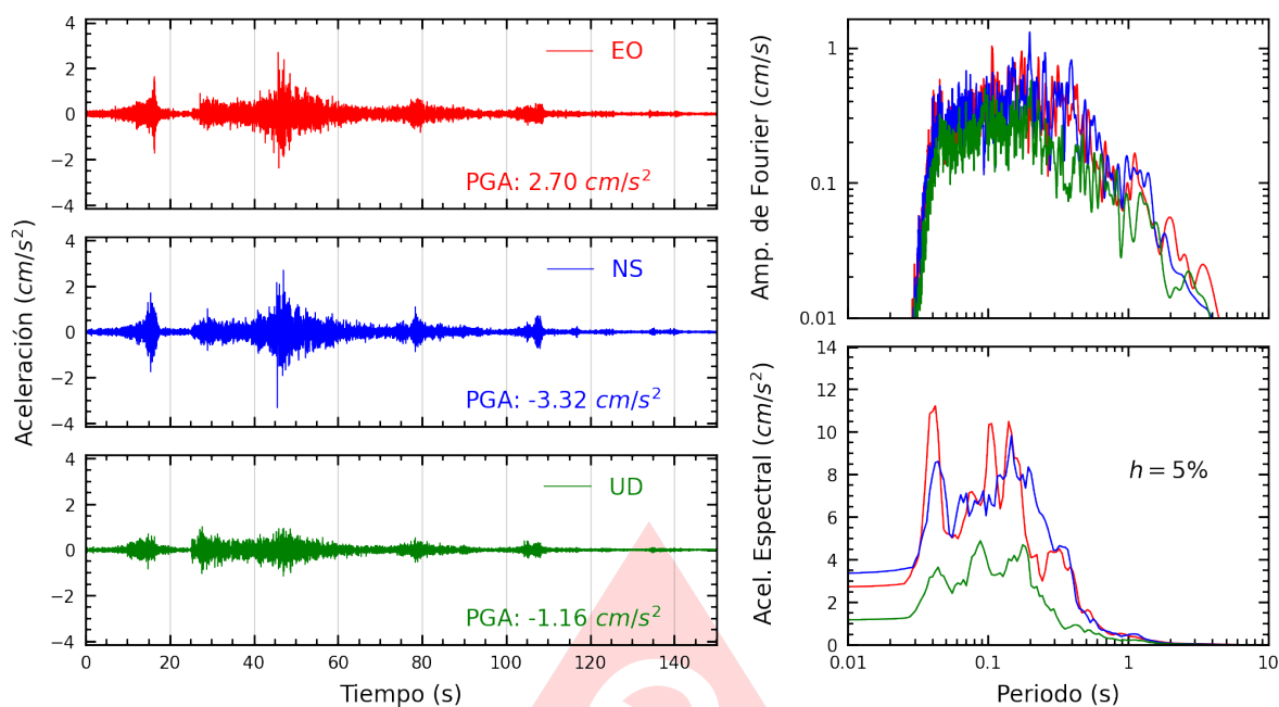
Figura A.9: Registros tiempo-historia, espectros de Fourier y de respuesta en las direcciones EO, NS y vertical de la estación PACHA. Sismo de Pisco, Pisco - Ica del 2025-09-02, 14:50:09 (Hora local)
