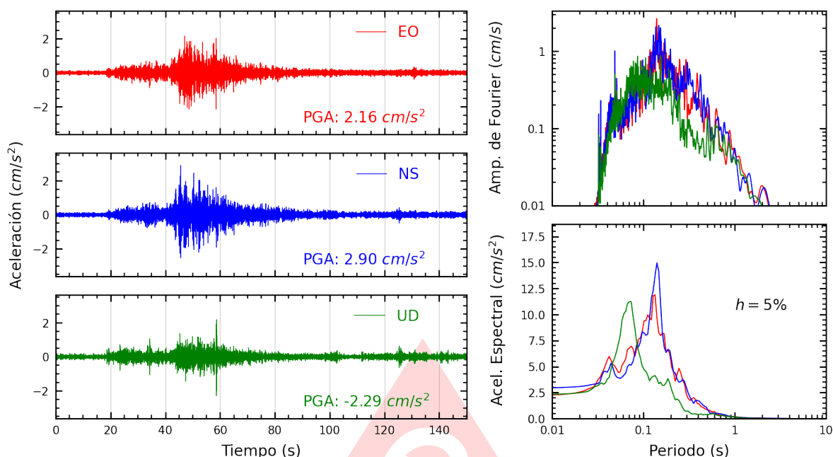
Figura A.13: Registros tiempo-historia, espectros de Fourier y de respuesta en las direcciones EO, NS y vertical de la estación CARAB. Sismo de Pisco, Pisco - Ica del 2025-09-02, 14:50:09 (Hora local)
