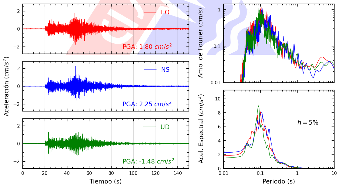
Figura A.20: Registros tiempo-historia, espectros de Fourier y de respuesta en las direcciones EO, NS y vertical de la estación AMORE. Sismo de Pisco, Pisco - Ica del 2025-09-02, 14:50:09 (Hora local)
