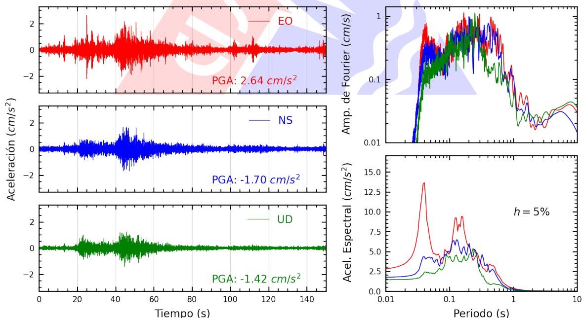
Figura A.16: Registros tiempo-historia, espectros de Fourier y de respuesta en las direcciones EO, NS y vertical de la estación OLIVO. Sismo de Pisco, Pisco - Ica del 2025-09-02, 14:50:09 (Hora local)
