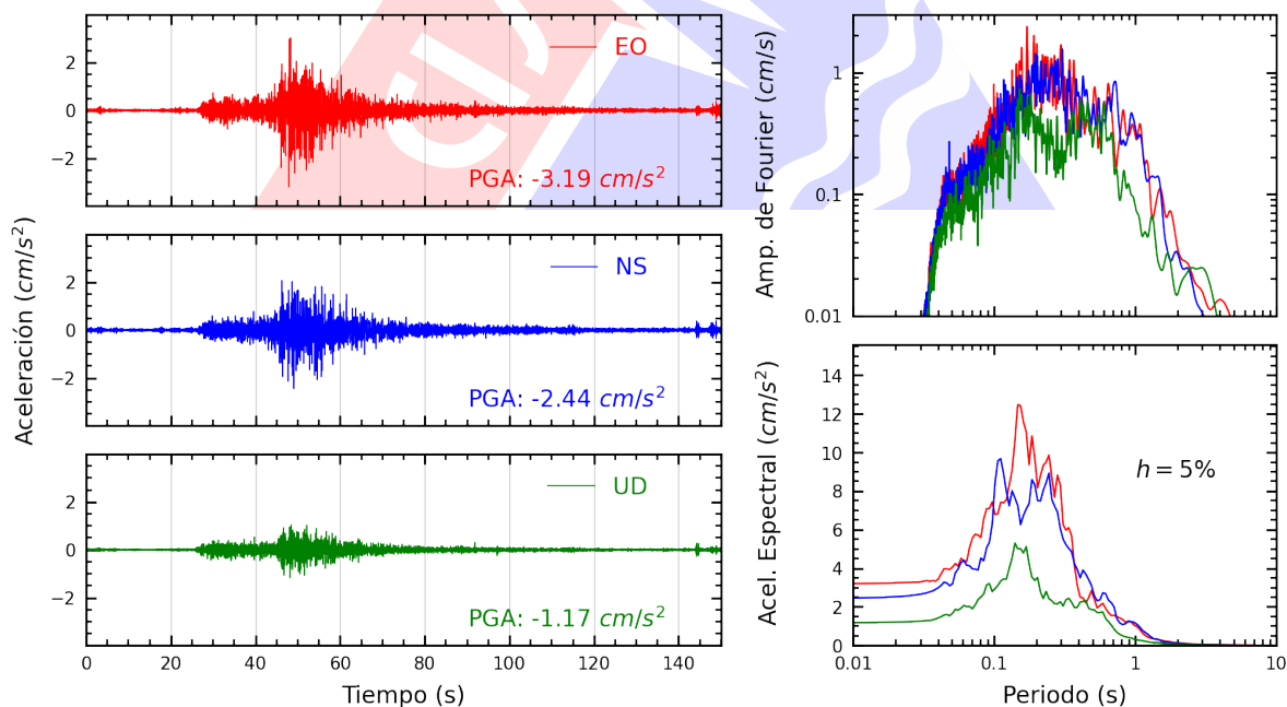
Figura A.10: Registros tiempo-historia, espectros de Fourier y de respuesta en las direcciones EO, NS y vertical de la estación BRIS2. Sismo de Pisco, Pisco - Ica del 2025-09-02, 14:50:09 (Hora local)
