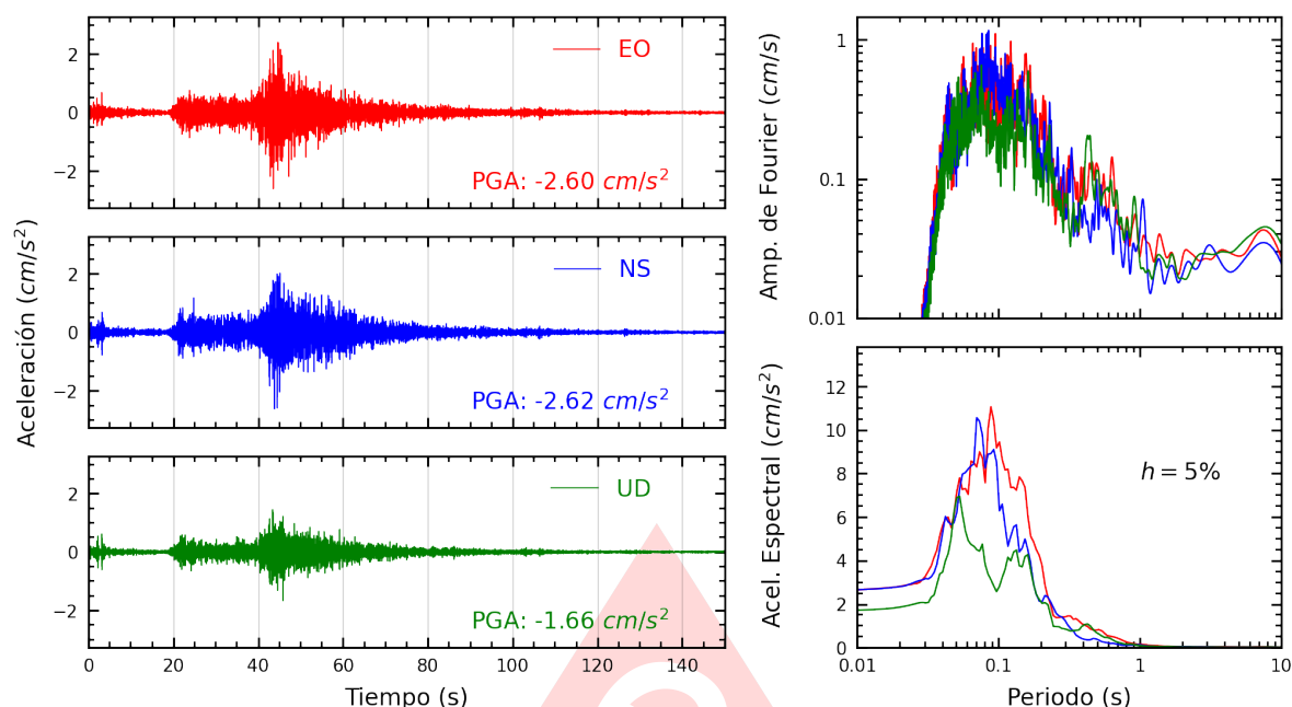
Figura A.17: Registros tiempo-historia, espectros de Fourier y de respuesta en las direcciones EO, NS y vertical de la estación JOSEO. Sismo de Pisco, Pisco - Ica del 2025-09-02, 14:50:09 (Hora local)
