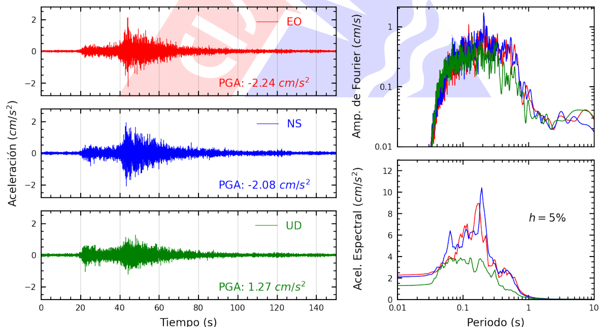
Figura A.22: Registros tiempo-historia, espectros de Fourier y de respuesta en las direcciones EO, NS y vertical de la estación SJLSC. Sismo de Pisco, Pisco - Ica del 2025-09-02, 14:50:09 (Hora local)
