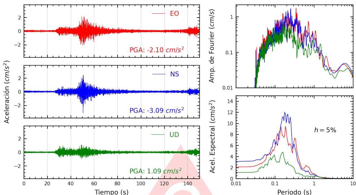
Figura A.11: Registros tiempo-historia, espectros de Fourier y de respuesta en las direcciones EO, NS y vertical de la estación SOBAR. Sismo de Pisco, Pisco - Ica del 2025-09-02, 14:50:09 (Hora local)
