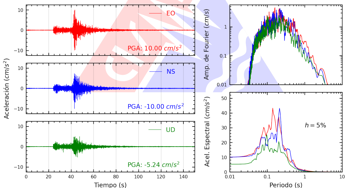
Figura A.2: Registros tiempo-historia, espectros de Fourier y de respuesta en las direcciones EO, NS y vertical de la estación PHERM. Sismo de Pisco, Pisco - Ica del 2025-09-02, 14:50:09 (Hora local)
