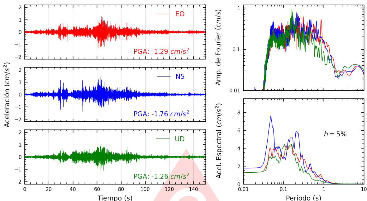
Figura A.27: Registros tiempo-historia, espectros de Fourier y de respuesta en las direcciones EO, NS y vertical de la estación UPCSM. Sismo de Pisco, Pisco - Ica del 2025-09-02, 14:50:09 (Hora local)
