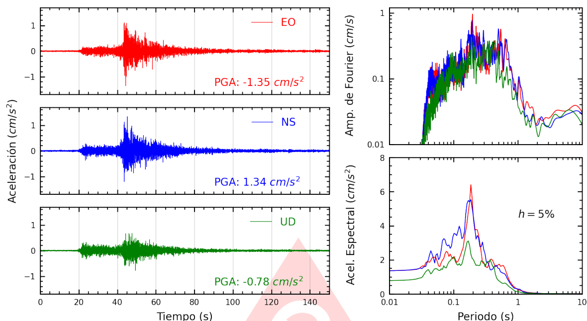
Figura A.35: Registros tiempo-historia, espectros de Fourier y de respuesta en las direcciones EO, NS y vertical de la estación COMAS. Sismo de Pisco, Pisco - Ica del 2025-09-02, 14:50:09 (Hora local)
