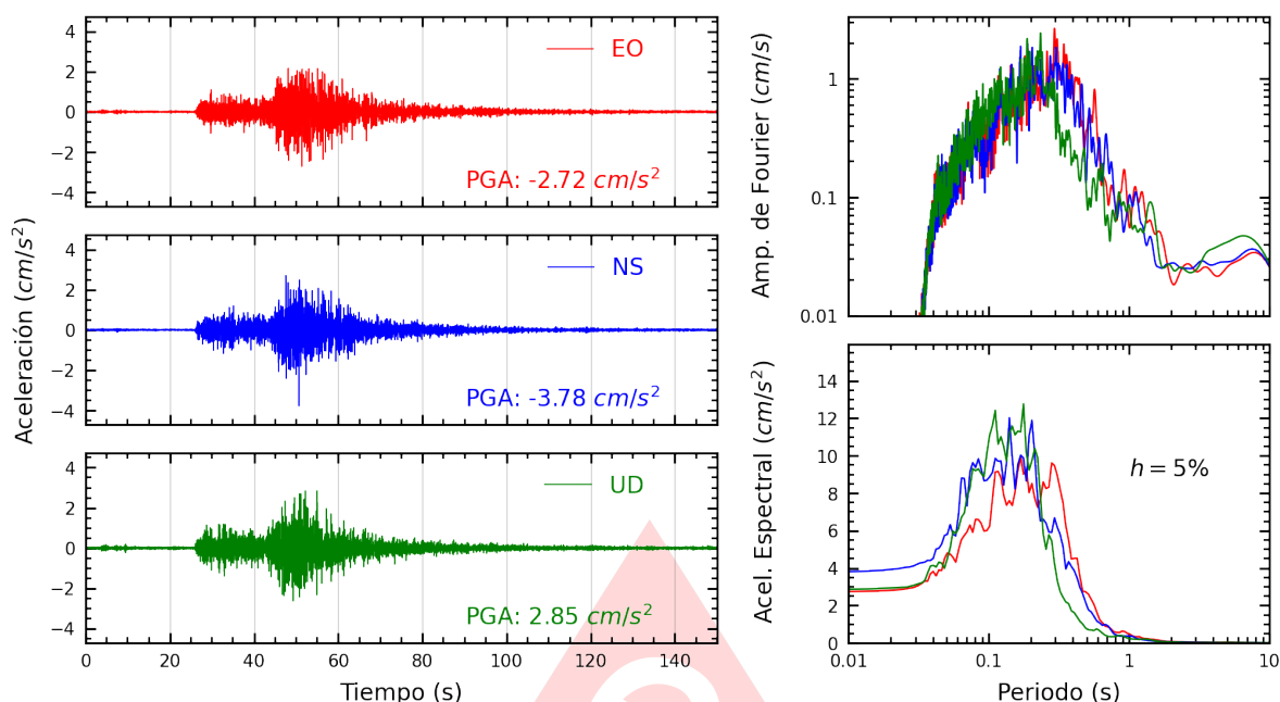
Figura A.7: Registros tiempo-historia, espectros de Fourier y de respuesta en las direcciones EO, NS y vertical de la estación SOVES. Sismo de Pisco, Pisco - Ica del 2025-09-02, 14:50:09 (Hora local)
