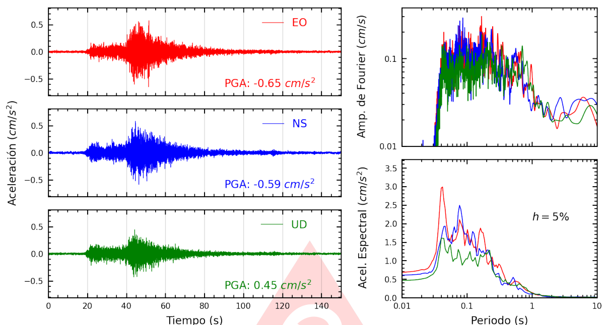
Figura A.43: Registros tiempo-historia, espectros de Fourier y de respuesta en las direcciones EO, NS y vertical de la estación SJLCE. Sismo de Pisco, Pisco - Ica del 2025-09-02, 14:50:09 (Hora local)
