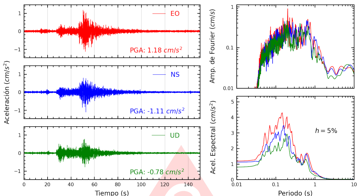
Figura A.37: Registros tiempo-historia, espectros de Fourier y de respuesta en las direcciones EO, NS y vertical de la estación INICT. Sismo de Pisco, Pisco - Ica del 2025-09-02, 14:50:09 (Hora local)
