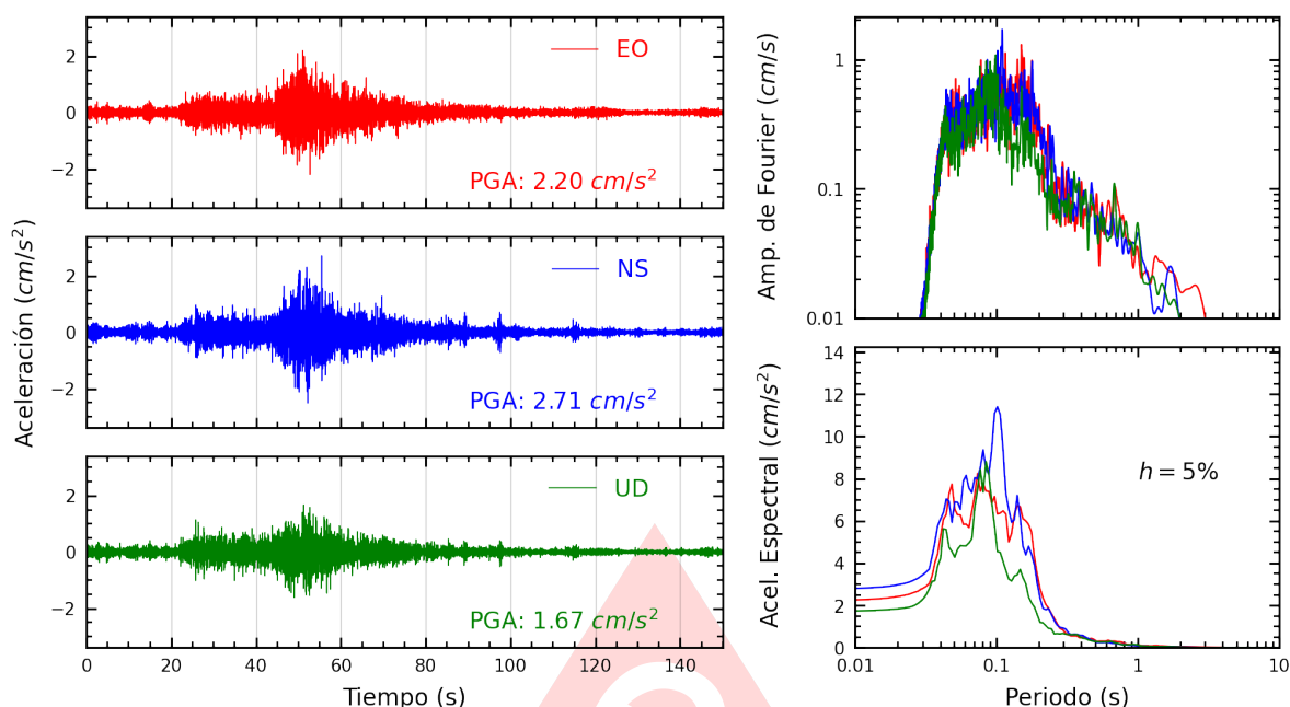
Figura A.15: Registros tiempo-historia, espectros de Fourier y de respuesta en las direcciones EO, NS y vertical de la estación SROSA. Sismo de Pisco, Pisco - Ica del 2025-09-02, 14:50:09 (Hora local)
