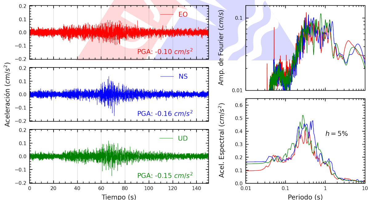
Figura A.44: Registros tiempo-historia, espectros de Fourier y de respuesta en las direcciones EO, NS y vertical de la estación UNSCH. Sismo de Pisco, Pisco - Ica del 2025-09-02, 14:50:09 (Hora local)
