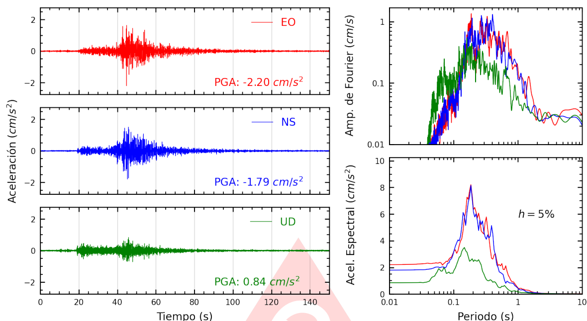
Figura A.23: Registros tiempo-historia, espectros de Fourier y de respuesta en las direcciones EO, NS y vertical de la estación ACAPU. Sismo de Pisco, Pisco - Ica del 2025-09-02, 14:50:09 (Hora local)
