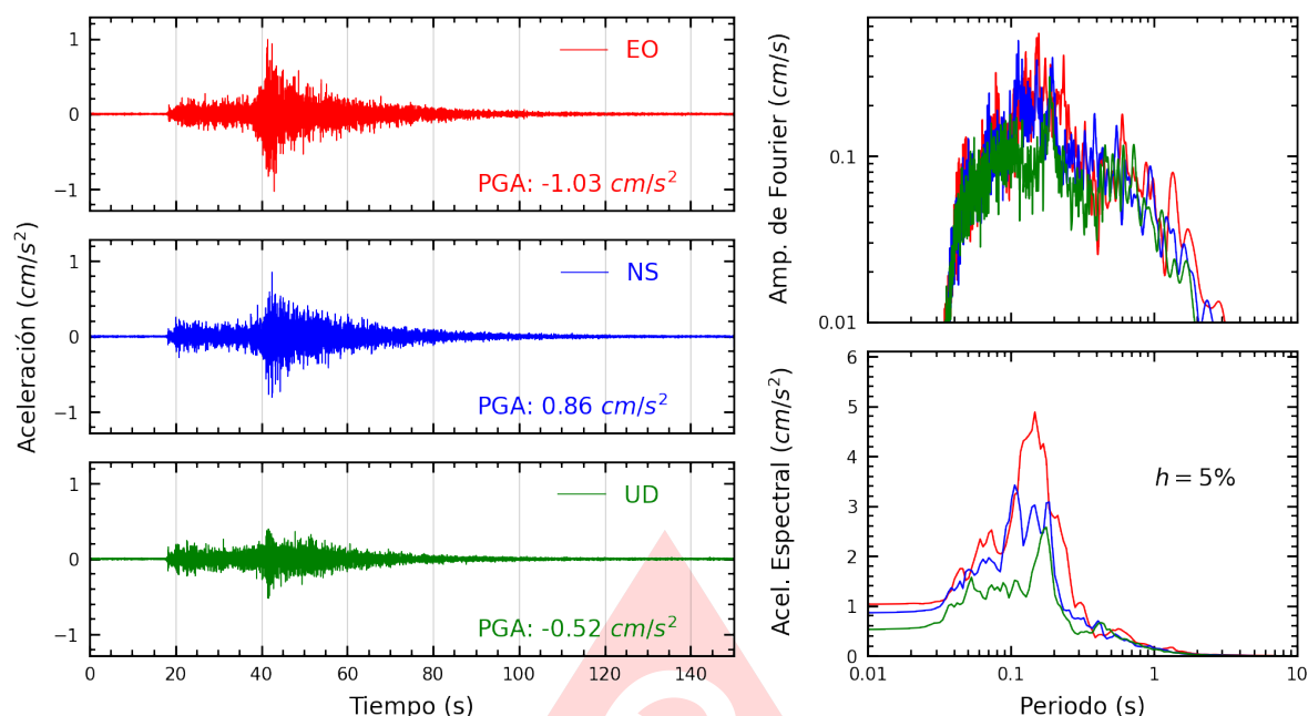
Figura A.41: Registros tiempo-historia, espectros de Fourier y de respuesta en las direcciones EO, NS y vertical de la estación ATARJ. Sismo de Pisco, Pisco - Ica del 2025-09-02, 14:50:09 (Hora local)
