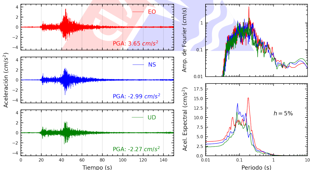
Figura A.8: Registros tiempo-historia, espectros de Fourier y de respuesta en las direcciones EO, NS y vertical de la estación INDEP. Sismo de Pisco, Pisco - Ica del 2025-09-02, 14:50:09 (Hora local)
