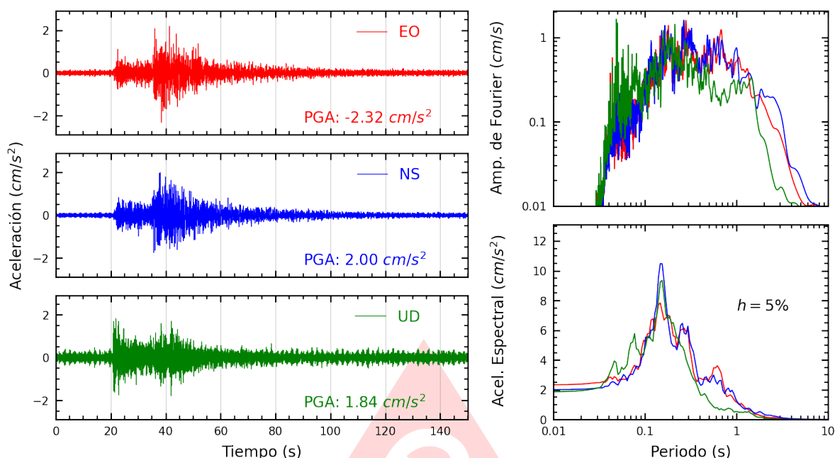
Figura A.19: Registros tiempo-historia, espectros de Fourier y de respuesta en las direcciones EO, NS y vertical de la estación UNICA. Sismo de Pisco, Pisco - Ica del 2025-09-02, 14:50:09 (Hora local)
