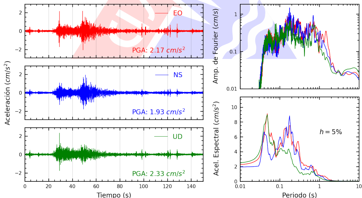
Figura A.18: Registros tiempo-historia, espectros de Fourier y de respuesta en las direcciones EO, NS y vertical de la estación PRADO. Sismo de Pisco, Pisco - Ica del 2025-09-02, 14:50:09 (Hora local)
