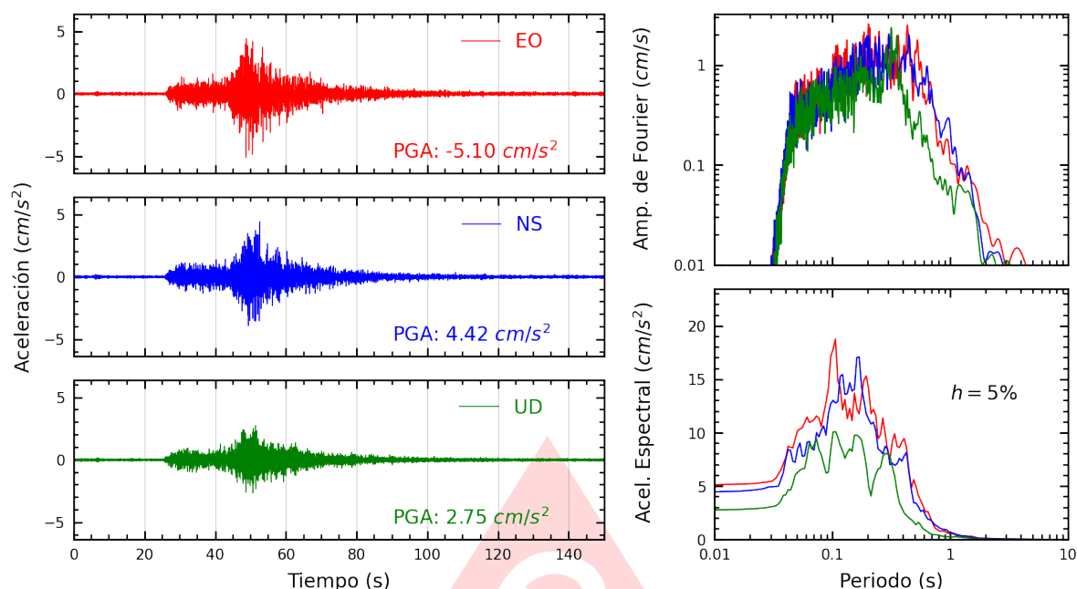
Figura A.5: Registros tiempo-historia, espectros de Fourier y de respuesta en las direcciones EO, NS y vertical de la estación UNTEL. Sismo de Pisco, Pisco - Ica del 2025-09-02, 14:50:09 (Hora local)
