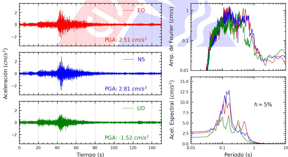
Figura A.14: Registros tiempo-historia, espectros de Fourier y de respuesta en las direcciones EO, NS y vertical de la estación SJLSV. Sismo de Pisco, Pisco - Ica del 2025-09-02, 14:50:09 (Hora local)
