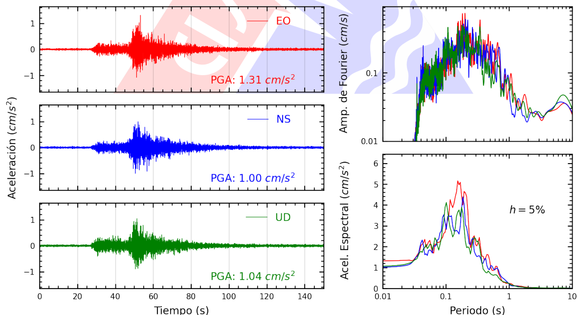
Figura A.36: Registros tiempo-historia, espectros de Fourier y de respuesta en las direcciones EO, NS y vertical de la estación USMP. Sismo de Pisco, Pisco - Ica del 2025-09-02, 14:50:09 (Hora local)
