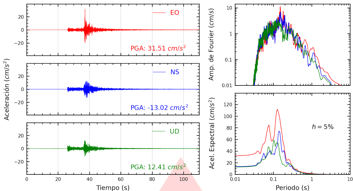
Figura A.1: Registros tiempo-historia, espectros de Fourier y de respuesta en las direcciones EO, NS y vertical de la estación ASIA. Sismo de Pisco, Pisco - Ica del 2025-09-02, 14:50:09 (Hora local)
