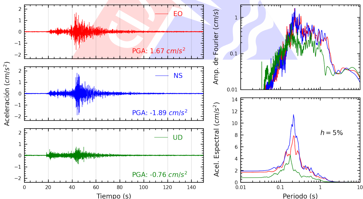
Figura A.26: Registros tiempo-historia, espectros de Fourier y de respuesta en las direcciones EO, NS y vertical de la estación DSMI. Sismo de Pisco, Pisco - Ica del 2025-09-02, 14:50:09 (Hora local)
