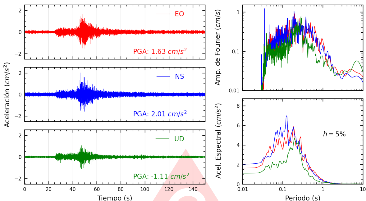
Figura A.25: Registros tiempo-historia, espectros de Fourier y de respuesta en las direcciones EO, NS y vertical de la estación UPCVI. Sismo de Pisco, Pisco - Ica del 2025-09-02, 14:50:09 (Hora local)
