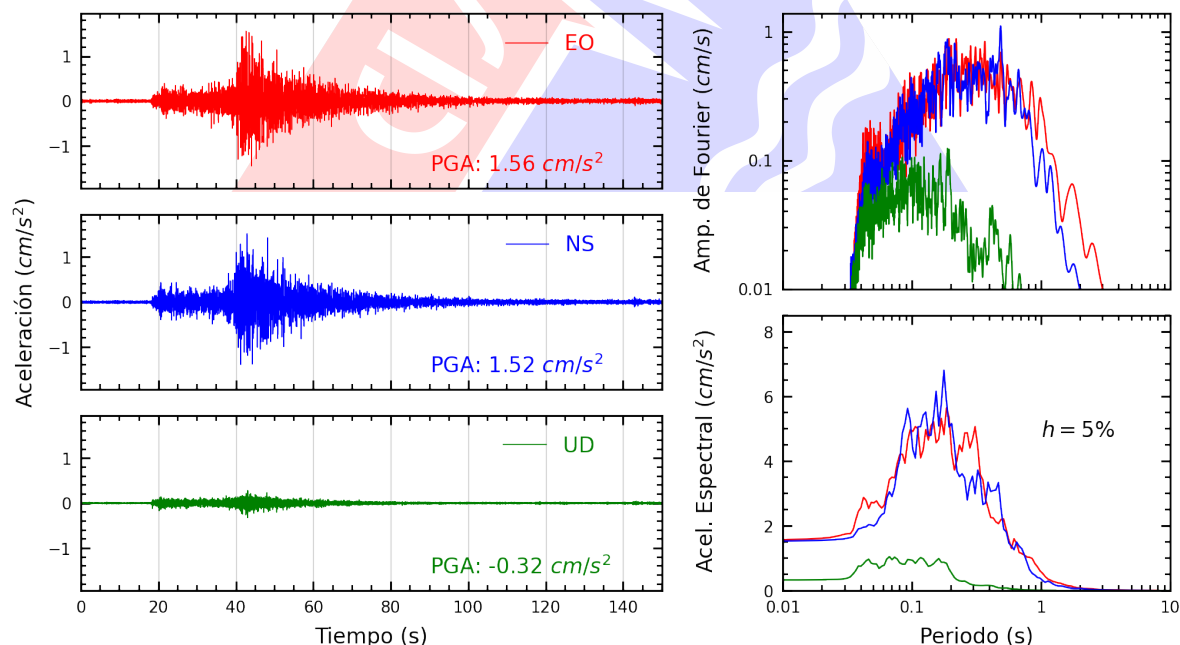
Figura A.32: Registros tiempo-historia, espectros de Fourier y de respuesta en las direcciones EO, NS y vertical de la estación UCVAT. Sismo de Pisco, Pisco - Ica del 2025-09-02, 14:50:09 (Hora local)
