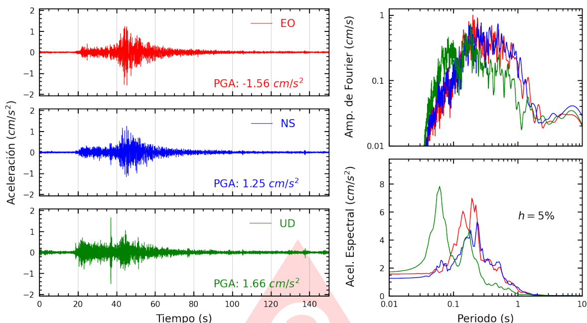
Figura A.29: Registros tiempo-historia, espectros de Fourier y de respuesta en las direcciones EO, NS y vertical de la estación RAMON. Sismo de Pisco, Pisco - Ica del 2025-09-02, 14:50:09 (Hora local)
