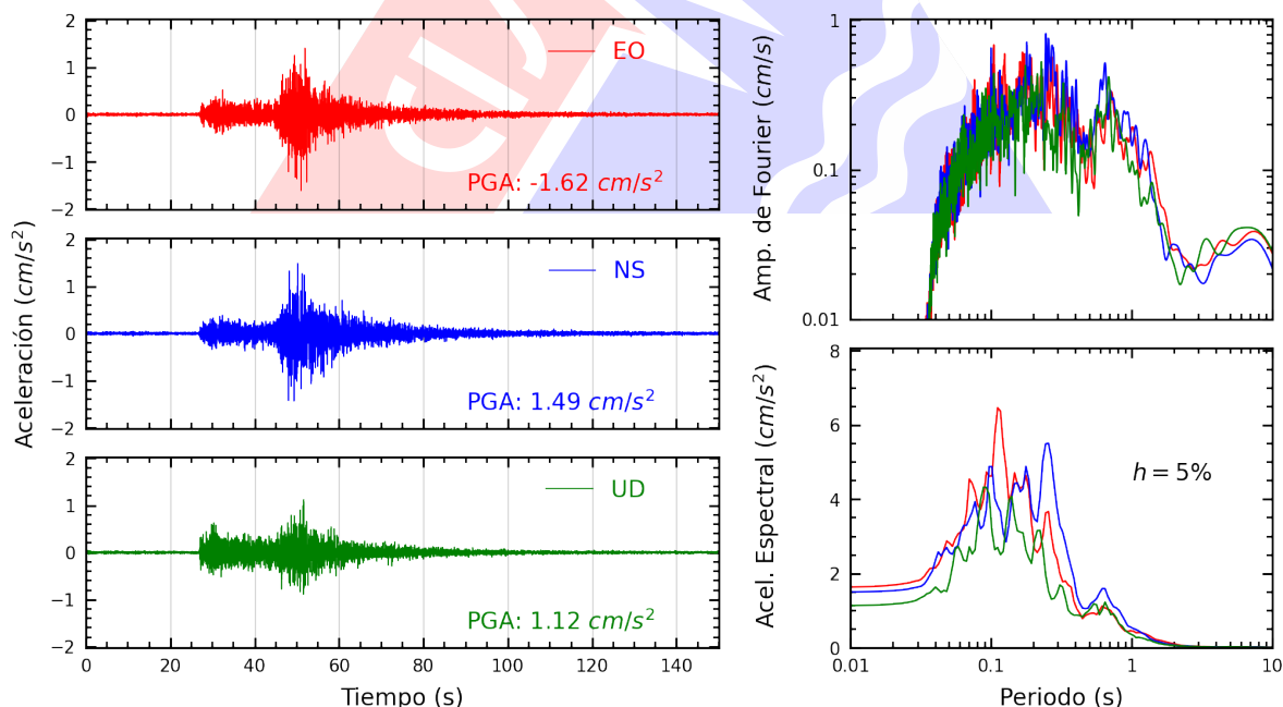
Figura A.30: Registros tiempo-historia, espectros de Fourier y de respuesta en las direcciones EO, NS y vertical de la estación SERVI. Sismo de Pisco, Pisco - Ica del 2025-09-02, 14:50:09 (Hora local)
