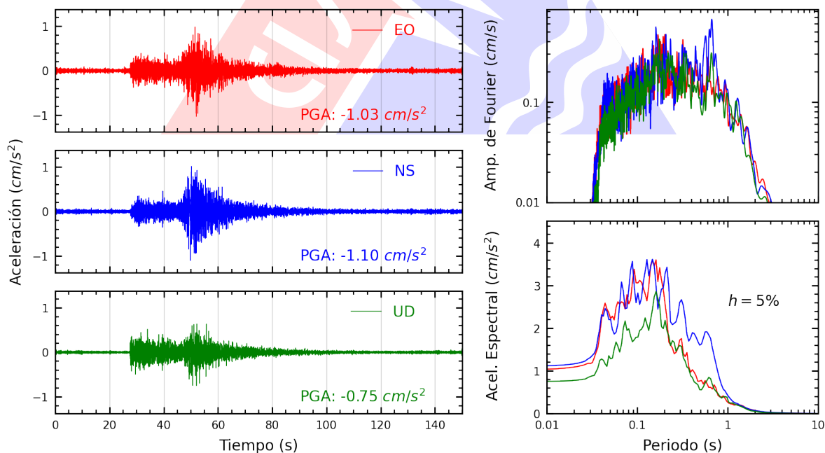
Figura A.38: Registros tiempo-historia, espectros de Fourier y de respuesta en las direcciones EO, NS y vertical de la estación BORJA. Sismo de Pisco, Pisco - Ica del 2025-09-02, 14:50:09 (Hora local)
