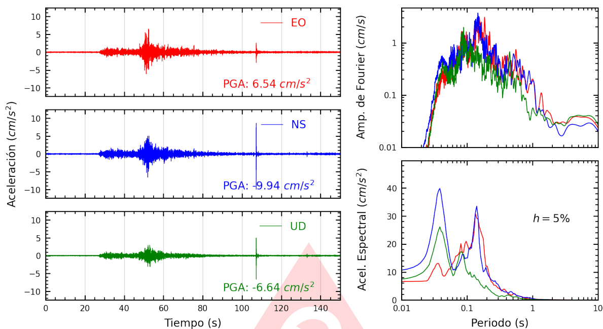
Figura A.3: Registros tiempo-historia, espectros de Fourier y de respuesta en las direcciones EO, NS y vertical de la estación USILM. Sismo de Pisco, Pisco - Ica del 2025-09-02, 14:50:09 (Hora local)
