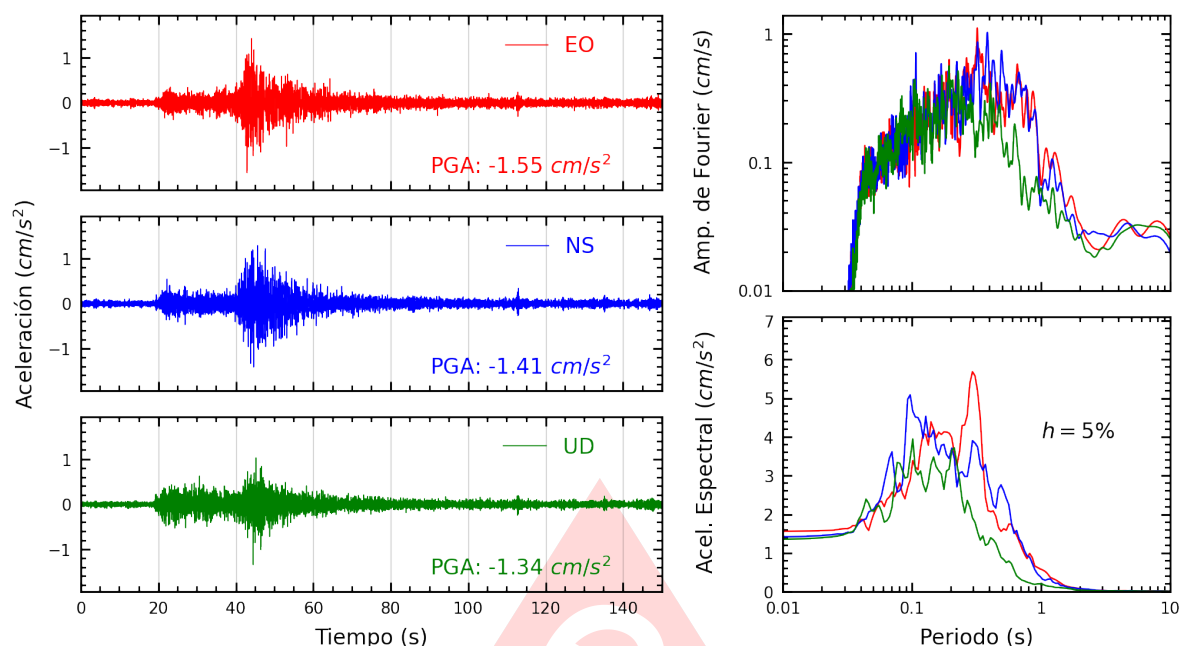
Figura A.33: Registros tiempo-historia, espectros de Fourier y de respuesta en las direcciones EO, NS y vertical de la estación MADRE. Sismo de Pisco, Pisco - Ica del 2025-09-02, 14:50:09 (Hora local)
