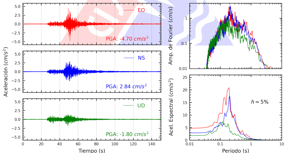
Figura A.6: Registros tiempo-historia, espectros de Fourier y de respuesta en las direcciones EO, NS y vertical de la estación SCCHO. Sismo de Pisco, Pisco - Ica del 2025-09-02, 14:50:09 (Hora local)
