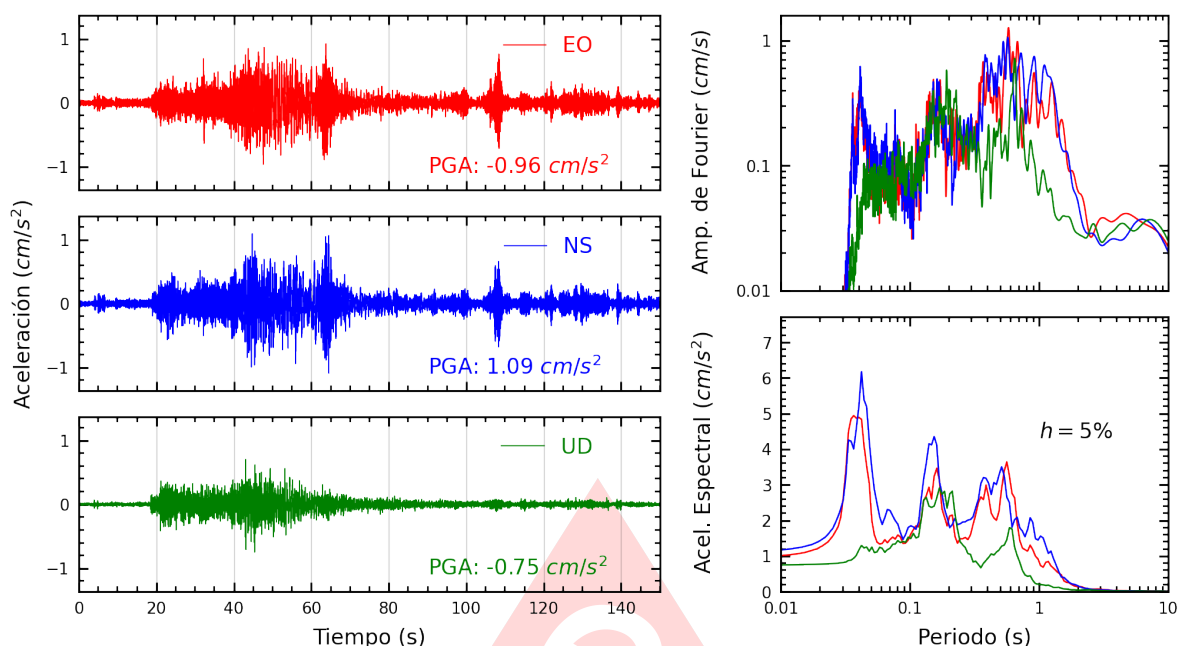
Figura A.39: Registros tiempo-historia, espectros de Fourier y de respuesta en las direcciones EO, NS y vertical de la estación DHNPE. Sismo de Pisco, Pisco - Ica del 2025-09-02, 14:50:09 (Hora local)
