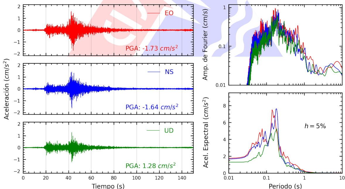
Figura A.28: Registros tiempo-historia, espectros de Fourier y de respuesta en las direcciones EO, NS y vertical de la estación FICPE. Sismo de Pisco, Pisco - Ica del 2025-09-02, 14:50:09 (Hora local)
