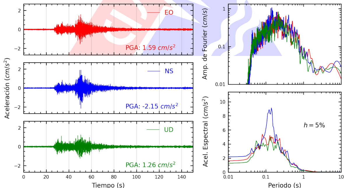
Figura A.24: Registros tiempo-historia, espectros de Fourier y de respuesta en las direcciones EO, NS y vertical de la estación URPPE. Sismo de Pisco, Pisco - Ica del 2025-09-02, 14:50:09 (Hora local)
