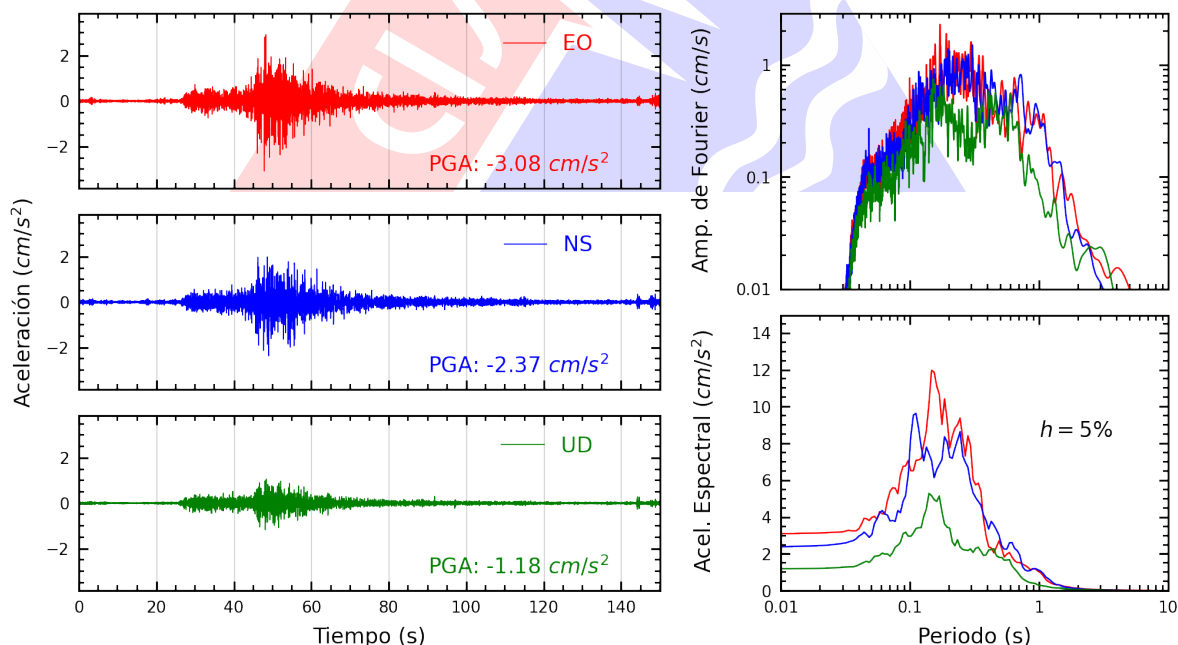
Figura A.12: Registros tiempo-historia, espectros de Fourier y de respuesta en las direcciones EO, NS y vertical de la estación BRISA. Sismo de Pisco, Pisco - Ica del 2025-09-02, 14:50:09 (Hora local)
