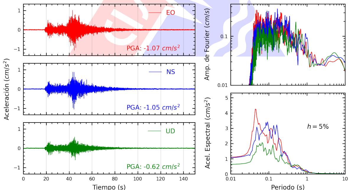
Figura A.40: Registros tiempo-historia, espectros de Fourier y de respuesta en las direcciones EO, NS y vertical de la estación UCSS. Sismo de Pisco, Pisco - Ica del 2025-09-02, 14:50:09 (Hora local)
