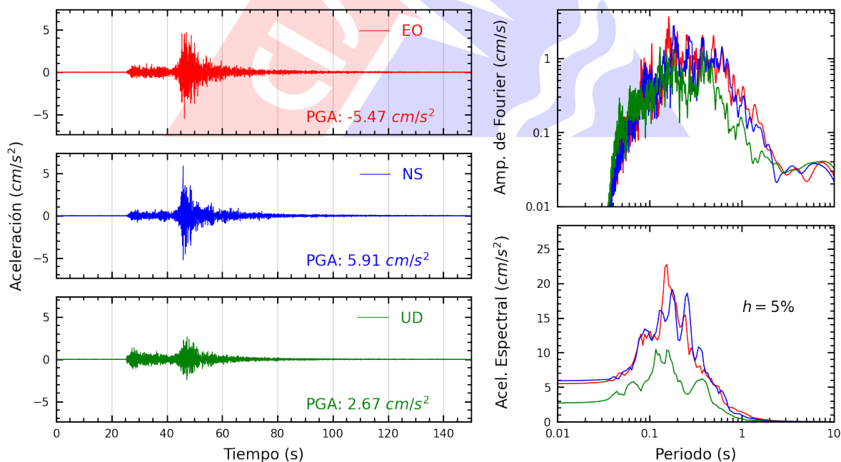
Figura A.4: Registros tiempo-historia, espectros de Fourier y de respuesta en las direcciones EO, NS y vertical de la estación USILP. Sismo de Pisco, Pisco - Ica del 2025-09-02, 14:50:09 (Hora local)
