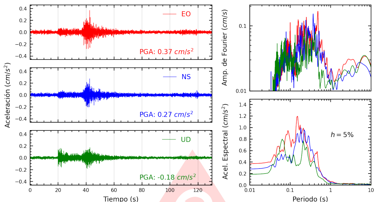
Figura A.3: Registros tiempo-historia, espectros de Fourier y de respuesta en las direcciones EO, NS y vertical de la estación USILP. Sismo de Pisco, Pisco - Ica del 2025-09-03, 10:16:33 (Hora local)
