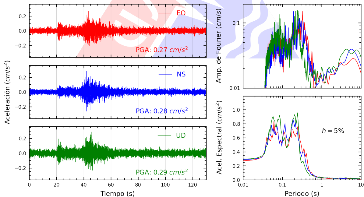
Figura A.4: Registros tiempo-historia, espectros de Fourier y de respuesta en las direcciones EO, NS y vertical de la estación SOVES. Sismo de Pisco, Pisco - Ica del 2025-09-03, 10:16:33 (Hora local)
