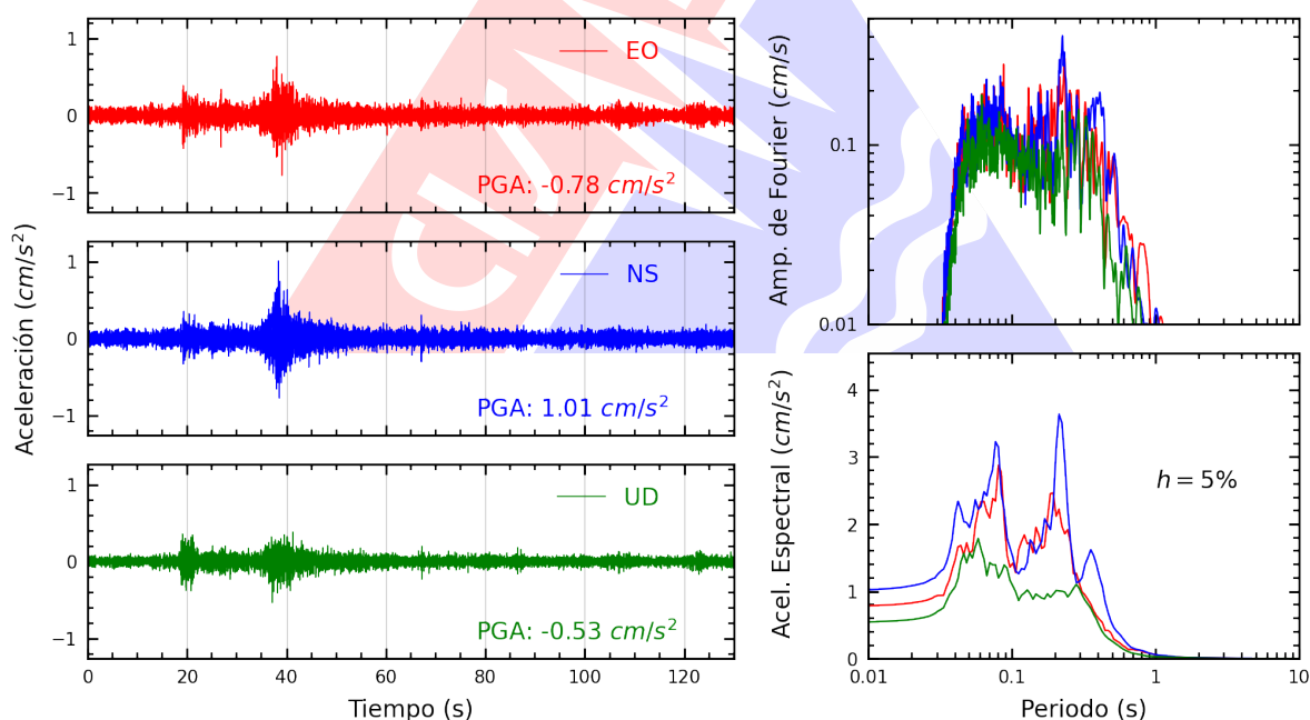
Figura A.2: Registros tiempo-historia, espectros de Fourier y de respuesta en las direcciones EO, NS y vertical de la estación PHERM. Sismo de Pisco, Pisco - Ica del 2025-09-03, 10:16:33 (Hora local)
