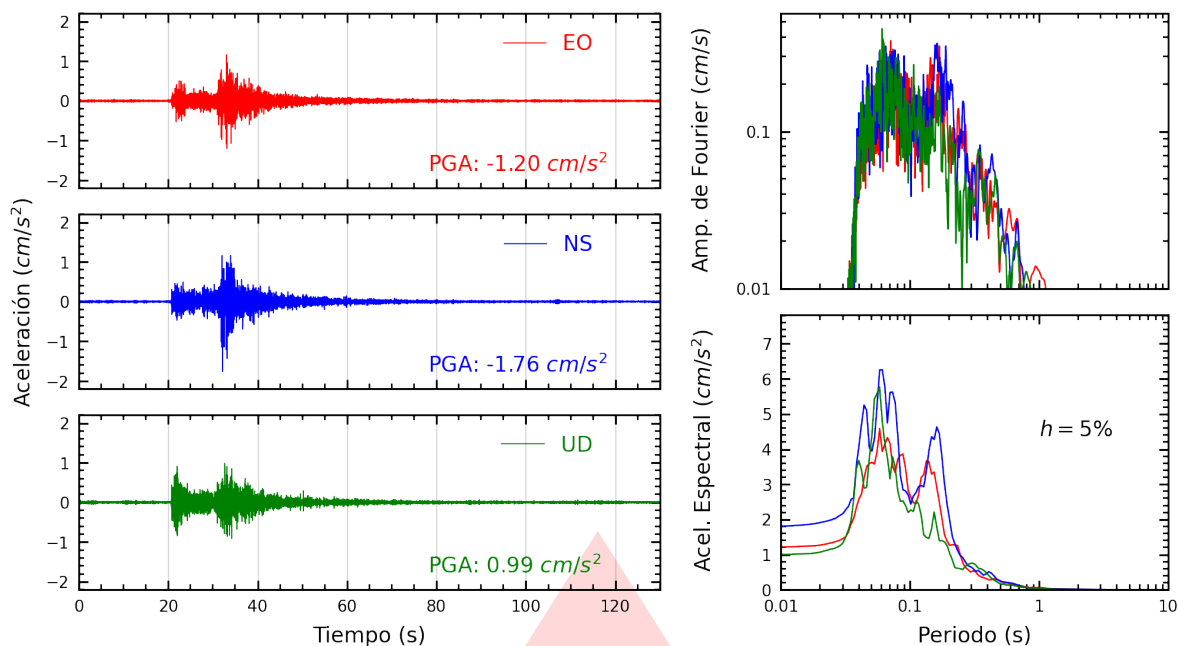
Figura A.1: Registros tiempo-historia, espectros de Fourier y de respuesta en las direcciones EO, NS y vertical de la estación ASIA. Sismo de Pisco, Pisco - Ica del 2025-09-03, 10:16:33 (Hora local)
