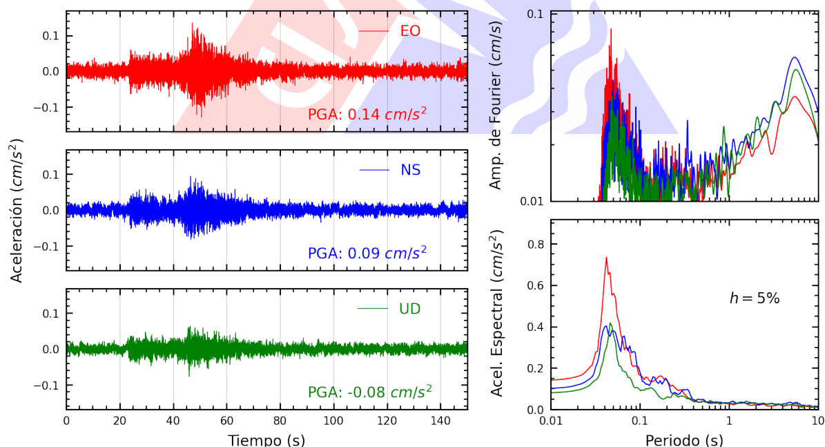
Figura A.6: Registros tiempo-historia, espectros de Fourier y de respuesta en las direcciones EO, NS y vertical de la estación UCSS. Sismo de Pisco, Pisco - Ica del 2025-09-03, 10:16:33 (Hora local)
