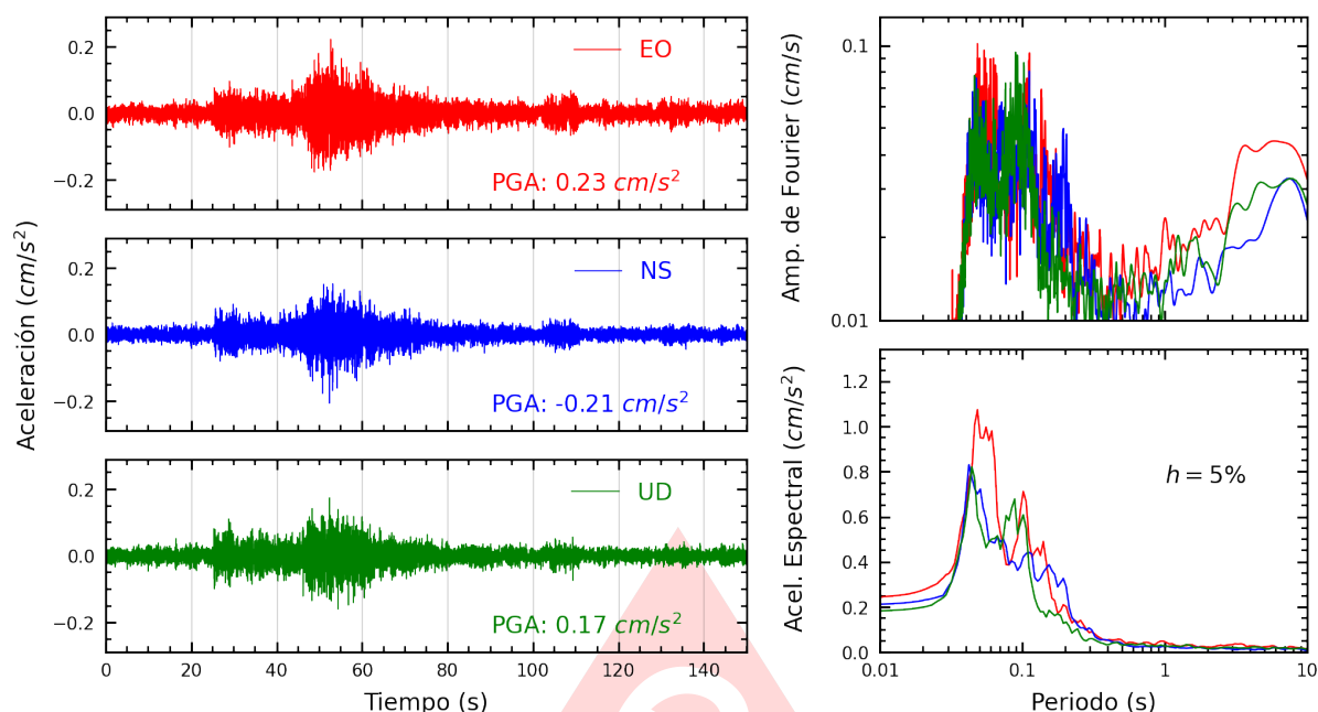
Figura A.5: Registros tiempo-historia, espectros de Fourier y de respuesta en las direcciones EO, NS y vertical de la estación AMORE. Sismo de Pisco, Pisco - Ica del 2025-09-03, 10:16:33 (Hora local)
