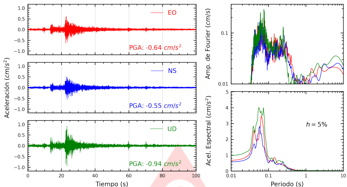
Figura A.15: Registros tiempo-historia, espectros de Fourier y de respuesta en las direcciones EO, NS y vertical de la estación SOVES. Sismo de Chilca, Cañete - Lima del 2025-09-04, 11:32:10 (Hora local)
