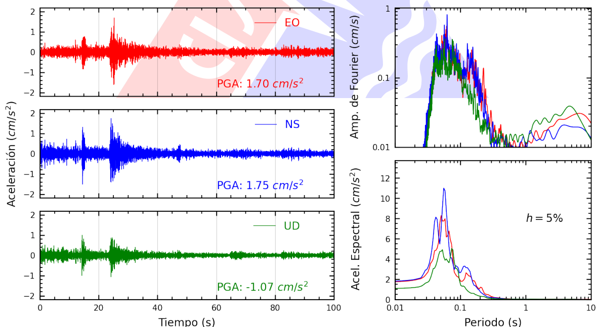
Figura A.6: Registros tiempo-historia, espectros de Fourier y de respuesta en las direcciones EO, NS y vertical de la estación USILM. Sismo de Chilca, Cañete - Lima del 2025-09-04, 11:32:10 (Hora local)
