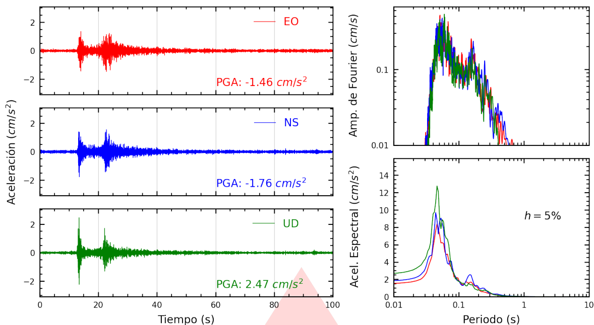
Figura A.1: Registros tiempo-historia, espectros de Fourier y de respuesta en las direcciones EO, NS y vertical de la estación PHERM. Sismo de Chilca, Cañete - Lima del 2025-09-04, 11:32:10 (Hora local)
