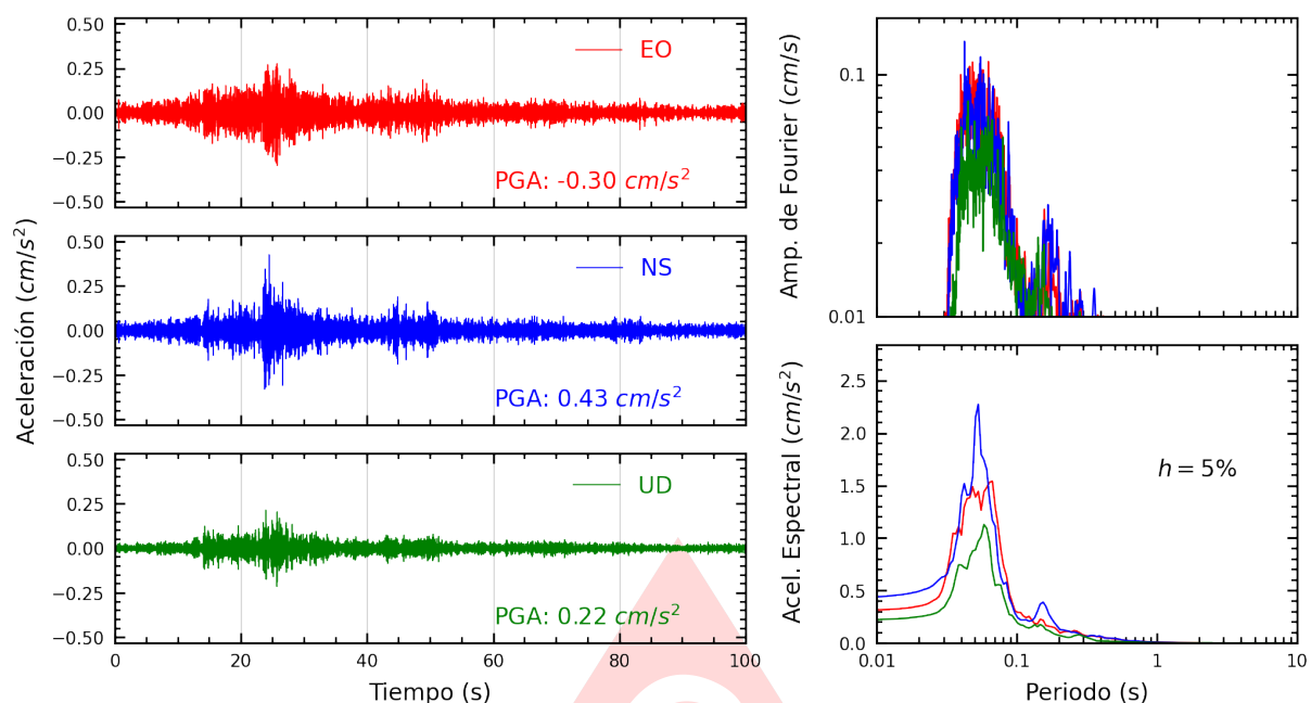
Figura A.33: Registros tiempo-historia, espectros de Fourier y de respuesta en las direcciones EO, NS y vertical de la estación BORJA. Sismo de Chilca, Cañete - Lima del 2025-09-04, 11:32:10 (Hora local)
