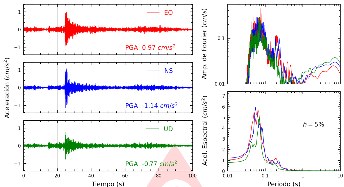
Figura A.13: Registros tiempo-historia, espectros de Fourier y de respuesta en las direcciones EO, NS y vertical de la estación INDEP. Sismo de Chilca, Cañete - Lima del 2025-09-04, 11:32:10 (Hora local)
