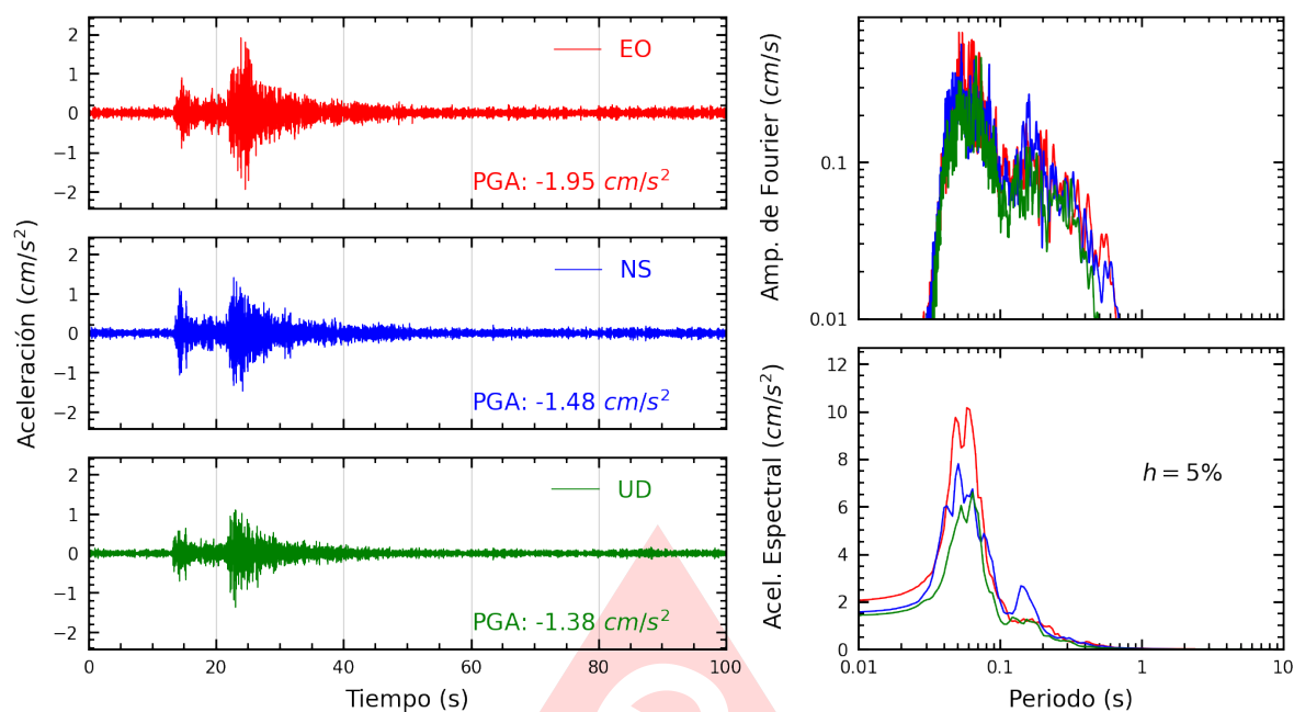
Figura A.3: Registros tiempo-historia, espectros de Fourier y de respuesta en las direcciones EO, NS y vertical de la estación UNTEL. Sismo de Chilca, Cañete - Lima del 2025-09-04, 11:32:10 (Hora local)
