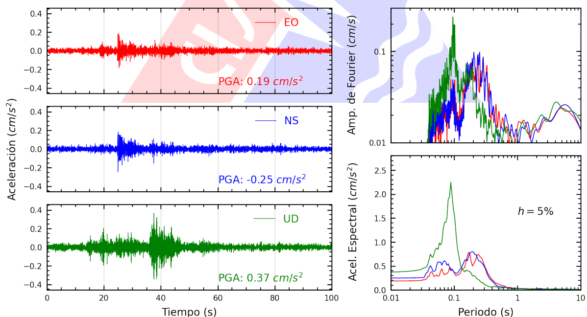
Figura A.34: Registros tiempo-historia, espectros de Fourier y de respuesta en las direcciones EO, NS y vertical de la estación DSMI. Sismo de Chilca, Cañete - Lima del 2025-09-04, 11:32:10 (Hora local)
