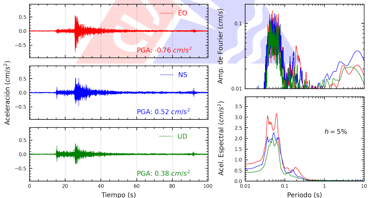
Figura A.18: Registros tiempo-historia, espectros de Fourier y de respuesta en las direcciones EO, NS y vertical de la estación SJLCE. Sismo de Chilca, Cañete - Lima del 2025-09-04, 11:32:10 (Hora local)
