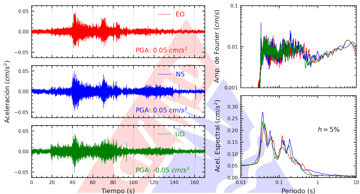
Figura A.37: Registros tiempo-historia, espectros de Fourier y de respuesta en las direcciones EO, NS y vertical de la estación CARAL. Sismo de Chilca, Cañete - Lima del 2025-09-04, 11:32:10 (Hora local)
