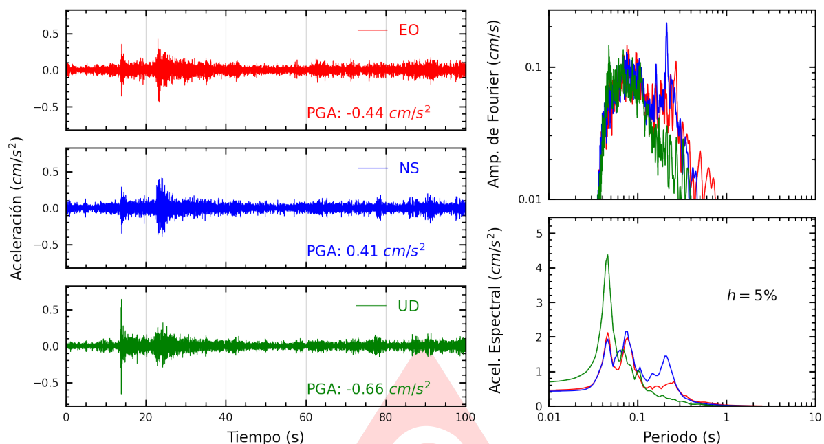
Figura A.19: Registros tiempo-historia, espectros de Fourier y de respuesta en las direcciones EO, NS y vertical de la estación SCCHO. Sismo de Chilca, Cañete - Lima del 2025-09-04, 11:32:10 (Hora local)
