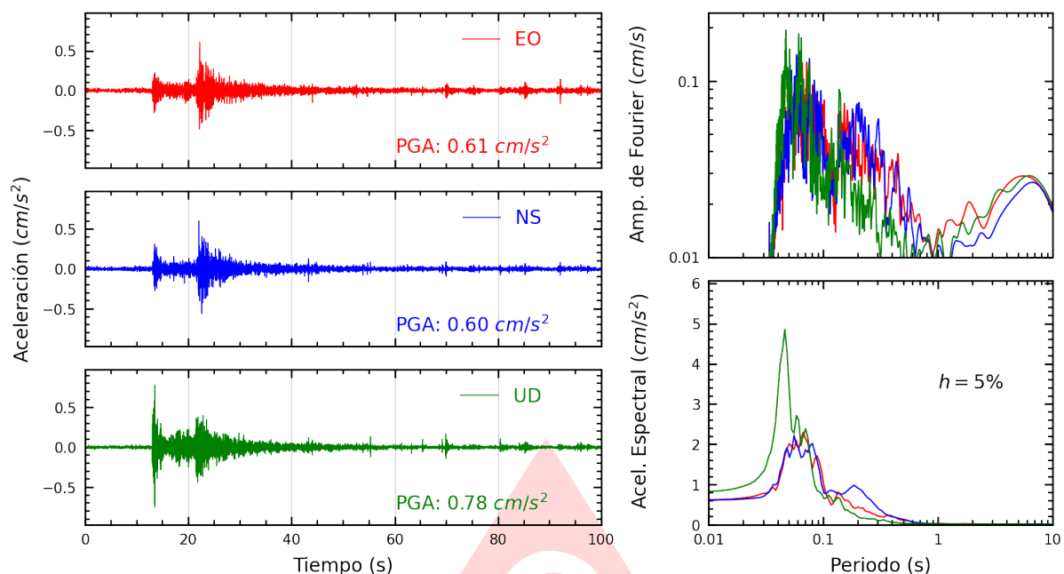
Figura A.17: Registros tiempo-historia, espectros de Fourier y de respuesta en las direcciones EO, NS y vertical de la estación USILP. Sismo de Chilca, Cañete - Lima del 2025-09-04, 11:32:10 (Hora local)
