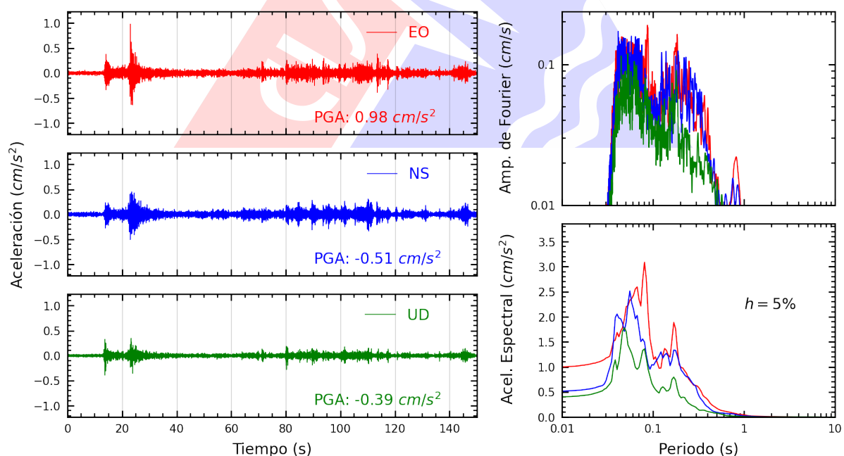
Figura A.14: Registros tiempo-historia, espectros de Fourier y de respuesta en las direcciones EO, NS y vertical de la estación BRISA. Sismo de Chilca, Cañete - Lima del 2025-09-04, 11:32:10 (Hora local)
