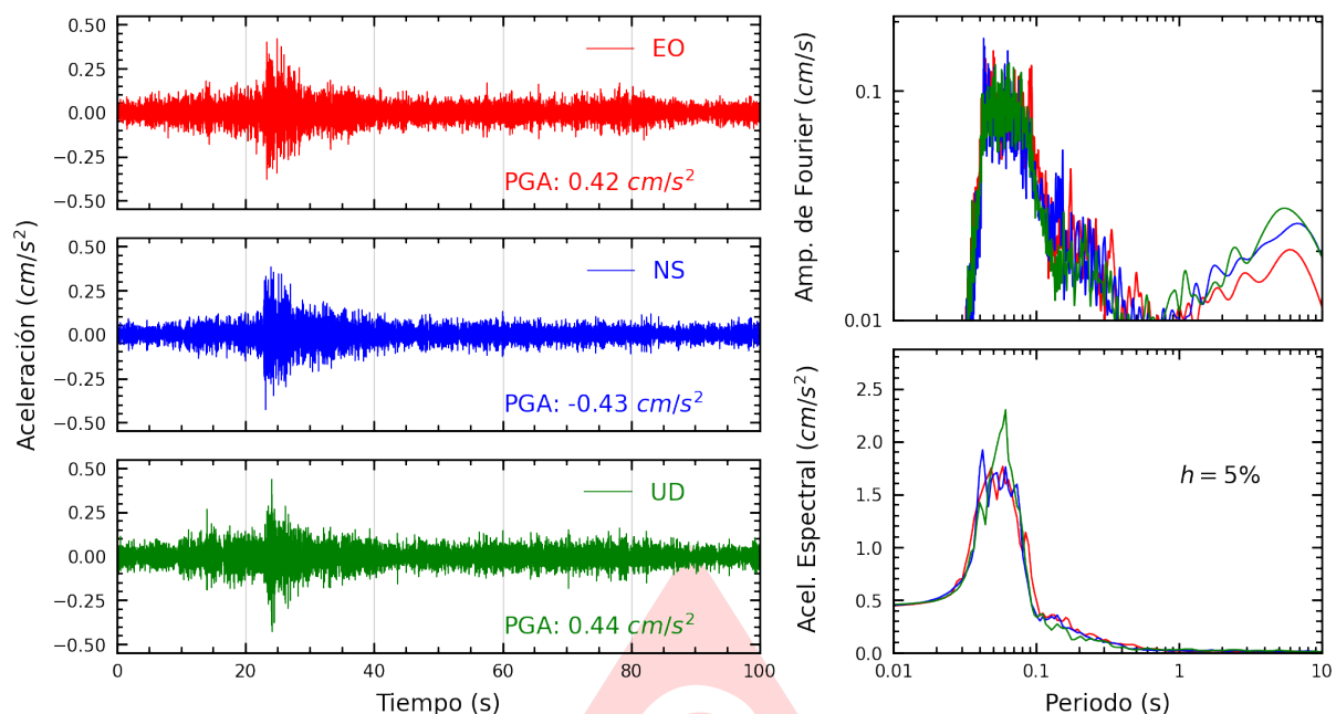
Figura A.31: Registros tiempo-historia, espectros de Fourier y de respuesta en las direcciones EO, NS y vertical de la estación URPPE. Sismo de Chilca, Cañete - Lima del 2025-09-04, 11:32:10 (Hora local)
