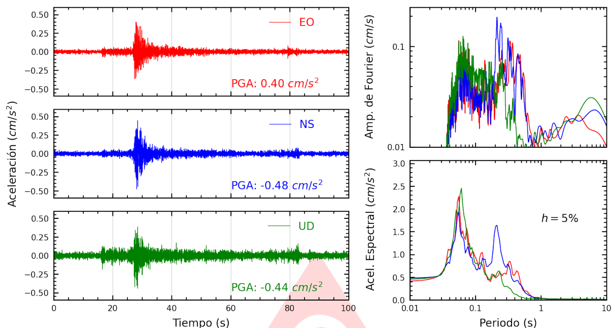
Figura A.29: Registros tiempo-historia, espectros de Fourier y de respuesta en las direcciones EO, NS y vertical de la estación MDPP. Sismo de Chilca, Cañete - Lima del 2025-09-04, 11:32:10 (Hora local)
