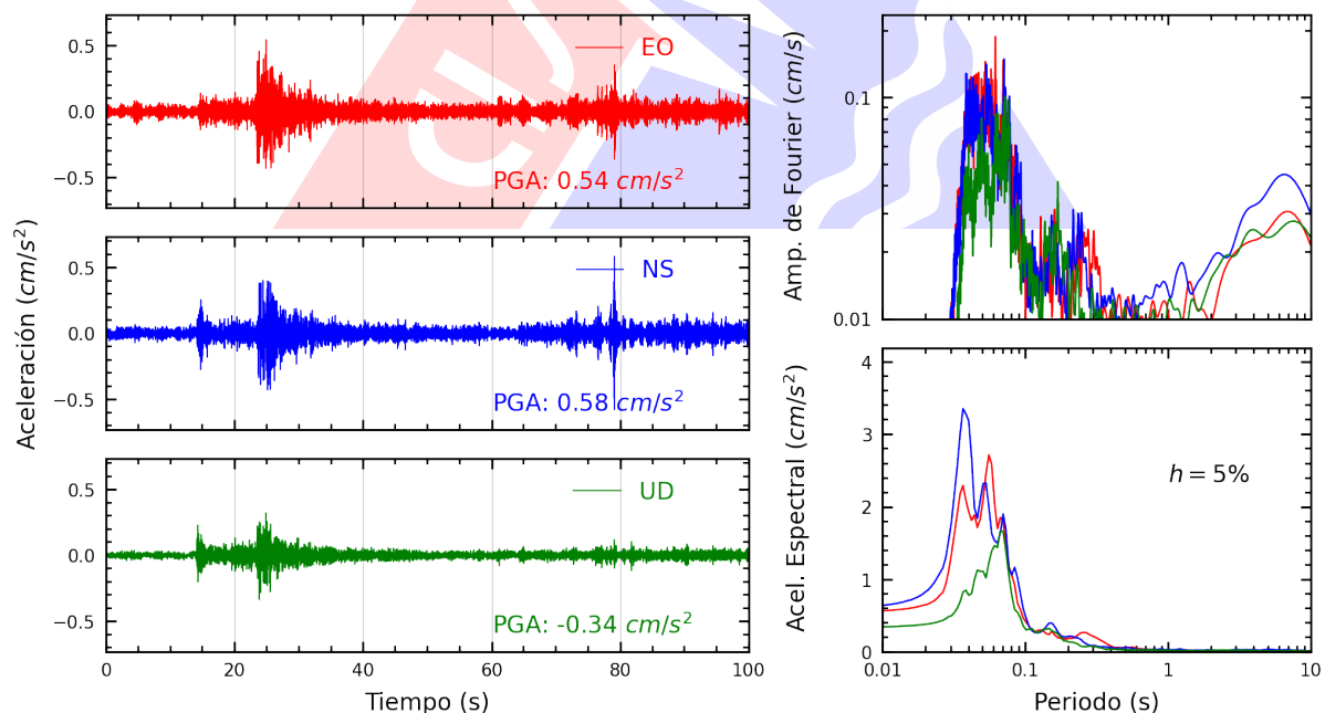
Figura A.24: Registros tiempo-historia, espectros de Fourier y de respuesta en las direcciones EO, NS y vertical de la estación CEPRE. Sismo de Chilca, Cañete - Lima del 2025-09-04, 11:32:10 (Hora local)
