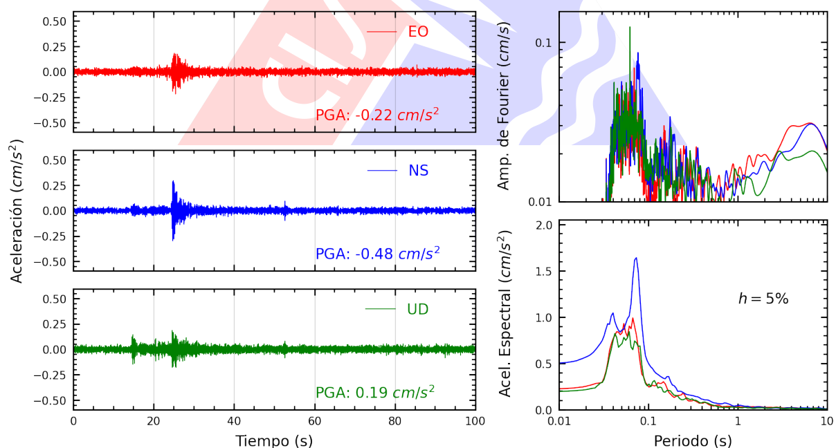
Figura A.30: Registros tiempo-historia, espectros de Fourier y de respuesta en las direcciones EO, NS y vertical de la estación BONDY. Sismo de Chilca, Cañete - Lima del 2025-09-04, 11:32:10 (Hora local)
