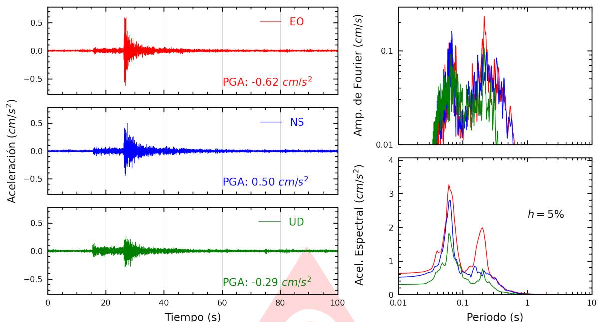
Figura A.23: Registros tiempo-historia, espectros de Fourier y de respuesta en las direcciones EO, NS y vertical de la estación VHAYA. Sismo de Chilca, Cañete - Lima del 2025-09-04, 11:32:10 (Hora local)
