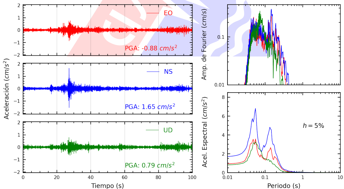
Figura A.8: Registros tiempo-historia, espectros de Fourier y de respuesta en las direcciones EO, NS y vertical de la estación CARAB. Sismo de Chilca, Cañete - Lima del 2025-09-04, 11:32:10 (Hora local)
