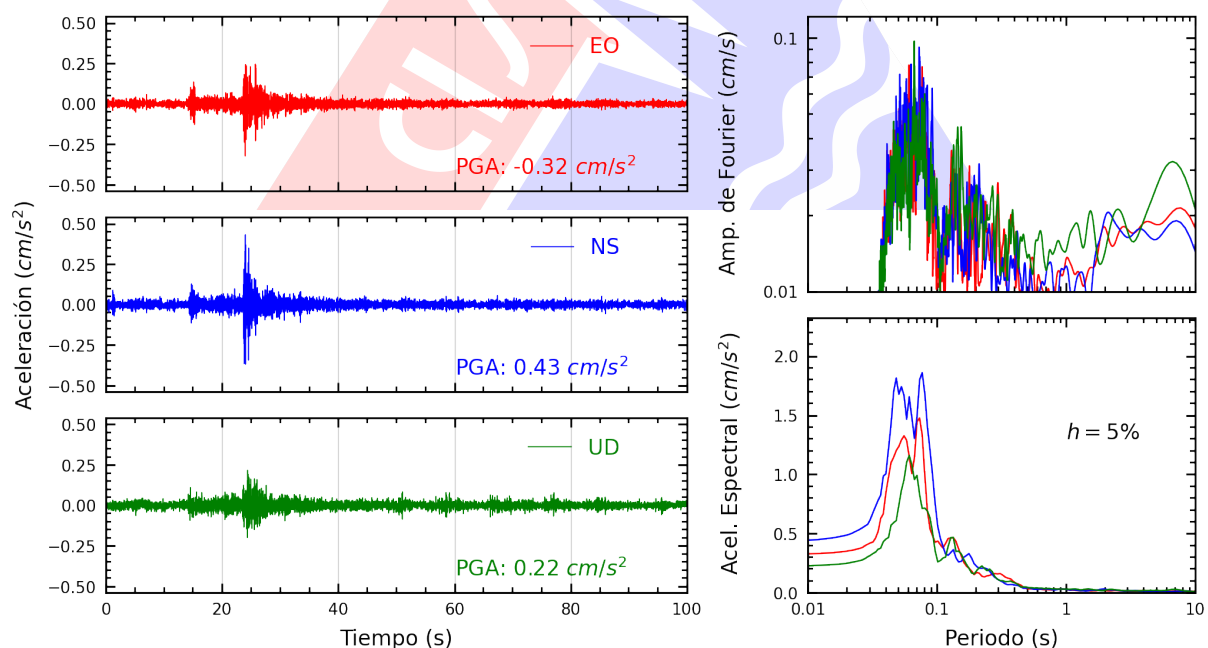
Figura A.32: Registros tiempo-historia, espectros de Fourier y de respuesta en las direcciones EO, NS y vertical de la estación UNFV. Sismo de Chilca, Cañete - Lima del 2025-09-04, 11:32:10 (Hora local)
