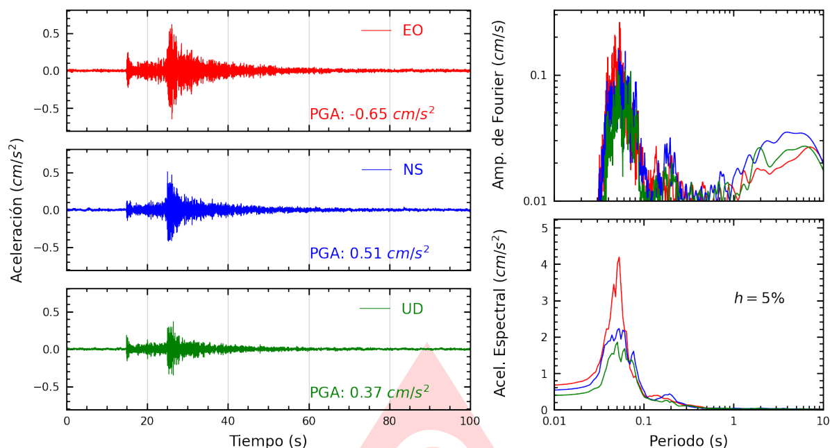
Figura A.21: Registros tiempo-historia, espectros de Fourier y de respuesta en las direcciones EO, NS y vertical de la estación UCSS. Sismo de Chilca, Cañete - Lima del 2025-09-04, 11:32:10 (Hora local)
