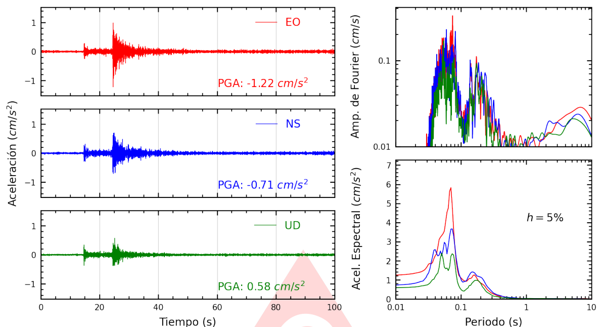
Figura A.11: Registros tiempo-historia, espectros de Fourier y de respuesta en las direcciones EO, NS y vertical de la estación FICPE. Sismo de Chilca, Cañete - Lima del 2025-09-04, 11:32:10 (Hora local)
