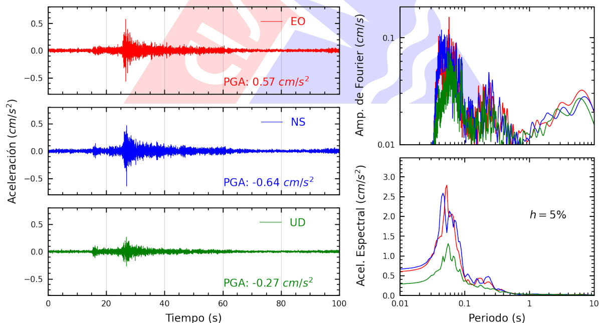
Figura A.22: Registros tiempo-historia, espectros de Fourier y de respuesta en las direcciones EO, NS y vertical de la estación COMAS. Sismo de Chilca, Cañete - Lima del 2025-09-04, 11:32:10 (Hora local)
