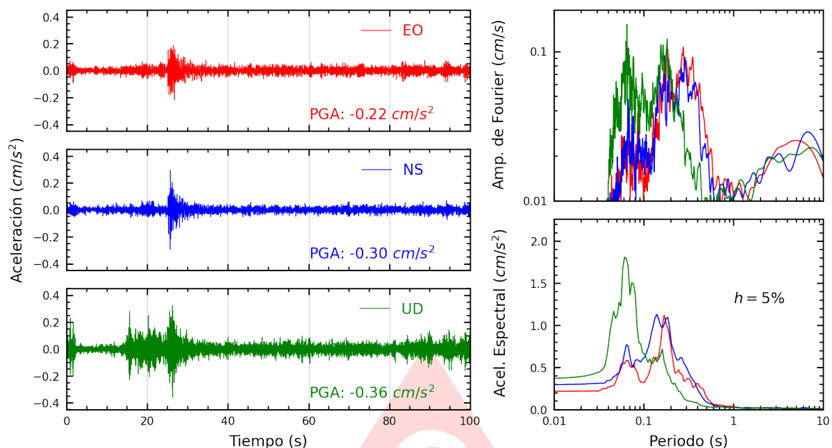
Figura A.35: Registros tiempo-historia, espectros de Fourier y de respuesta en las direcciones EO, NS y vertical de la estación ACAPU. Sismo de Chilca, Cañete - Lima del 2025-09-04, 11:32:10 (Hora local)
