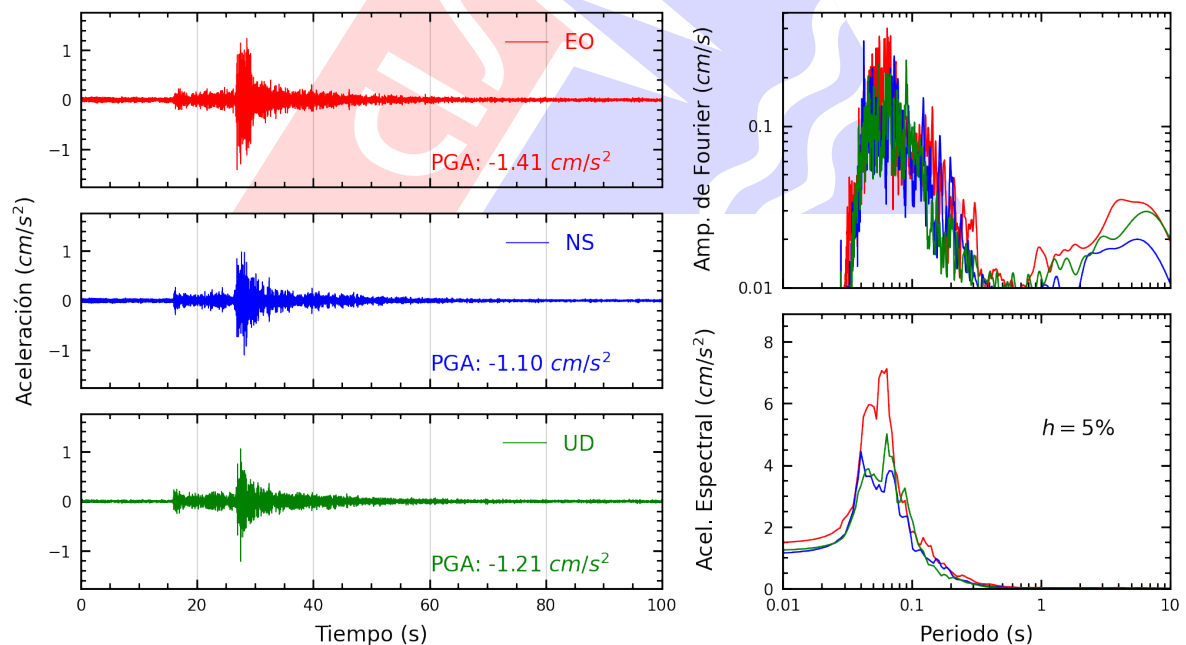
Figura A.10: Registros tiempo-historia, espectros de Fourier y de respuesta en las direcciones EO, NS y vertical de la estación AMORE. Sismo de Chilca, Cañete - Lima del 2025-09-04, 11:32:10 (Hora local)
