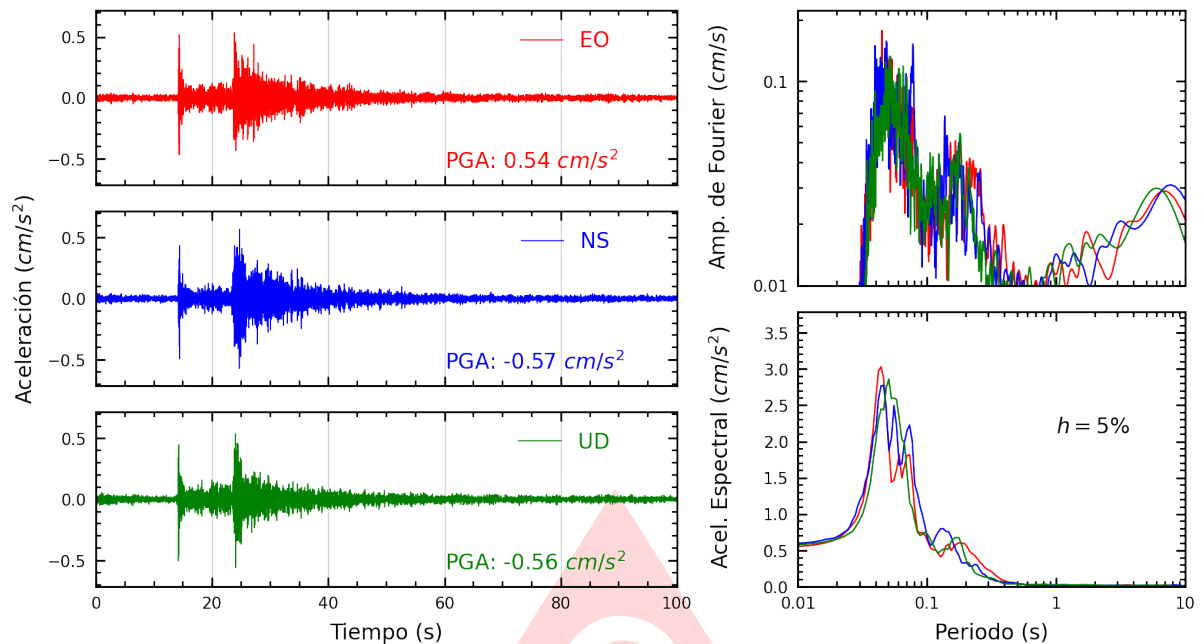
Figura A.25: Registros tiempo-historia, espectros de Fourier y de respuesta en las direcciones EO, NS y vertical de la estación USMP. Sismo de Chilca, Cañete - Lima del 2025-09-04, 11:32:10 (Hora local)
