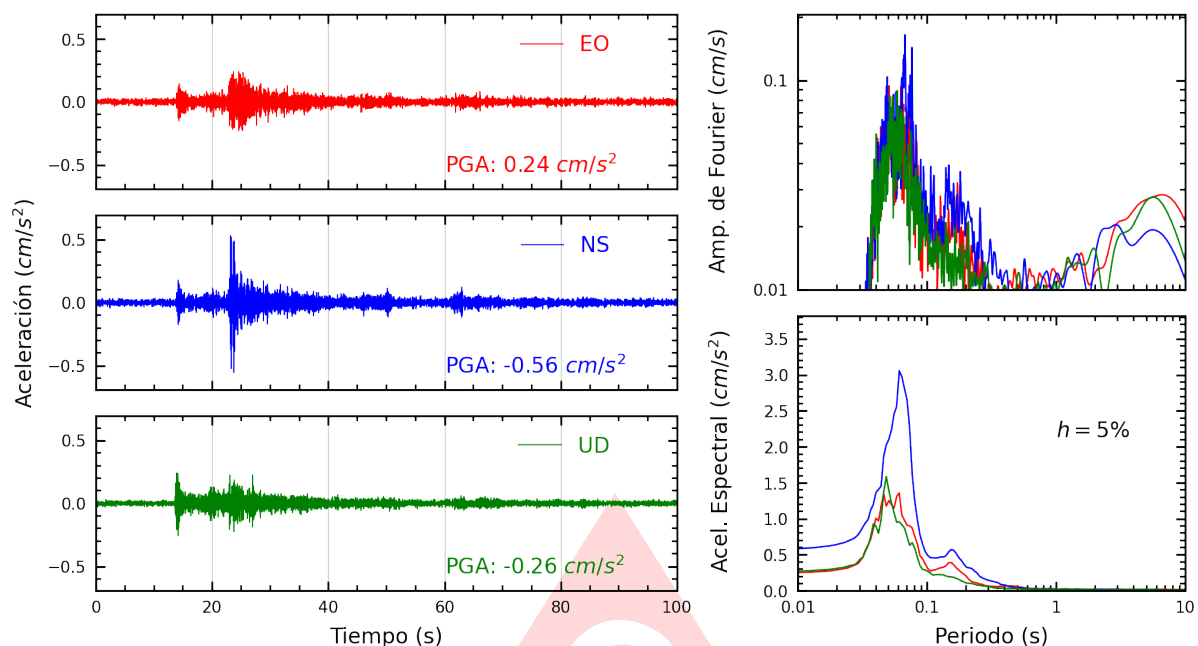
Figura A.27: Registros tiempo-historia, espectros de Fourier y de respuesta en las direcciones EO, NS y vertical de la estación SERVI. Sismo de Chilca, Cañete - Lima del 2025-09-04, 11:32:10 (Hora local)
