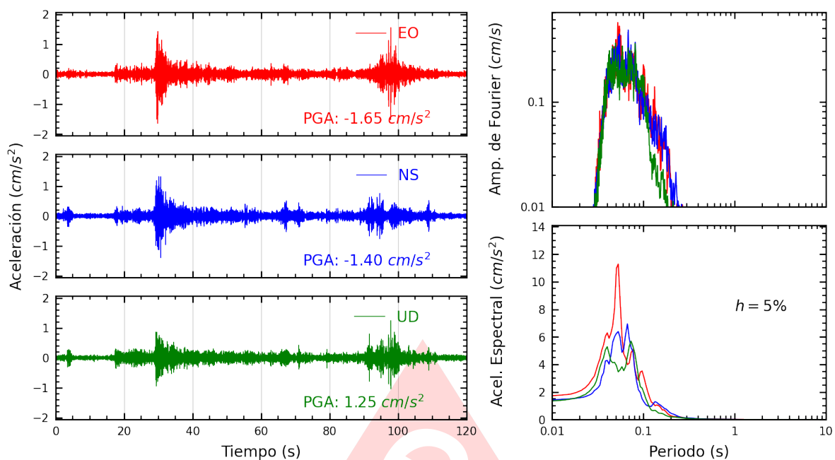
Figura A.7: Registros tiempo-historia, espectros de Fourier y de respuesta en las direcciones EO, NS y vertical de la estación SROSA. Sismo de Chilca, Cañete - Lima del 2025-09-04, 11:32:10 (Hora local)
