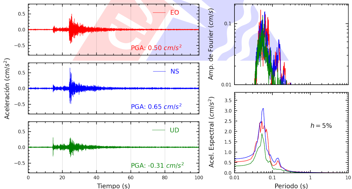
Figura A.20: Registros tiempo-historia, espectros de Fourier y de respuesta en las direcciones EO, NS y vertical de la estación ATARJ. Sismo de Chilca, Cañete - Lima del 2025-09-04, 11:32:10 (Hora local)
