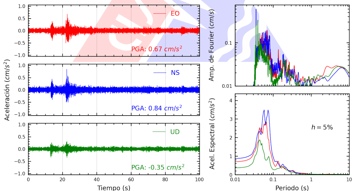
Figura A.16: Registros tiempo-historia, espectros de Fourier y de respuesta en las direcciones EO, NS y vertical de la estación UPCVI. Sismo de Chilca, Cañete - Lima del 2025-09-04, 11:32:10 (Hora local)
