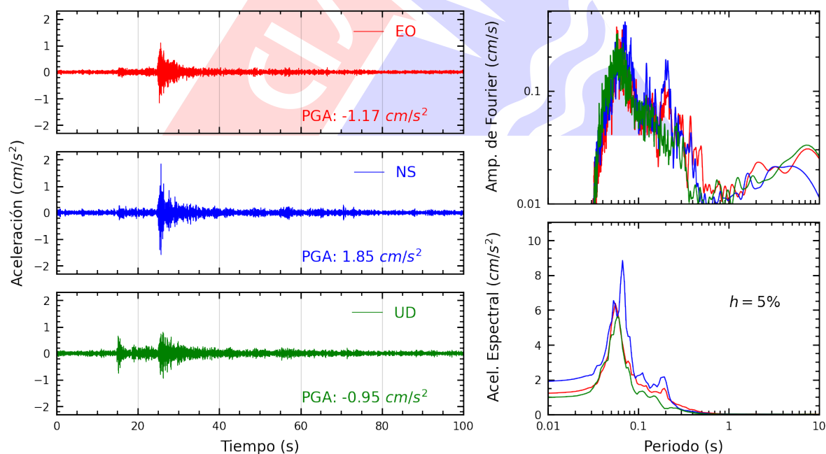
Figura A.4: Registros tiempo-historia, espectros de Fourier y de respuesta en las direcciones EO, NS y vertical de la estación SJLSC. Sismo de Chilca, Cañete - Lima del 2025-09-04, 11:32:10 (Hora local)
