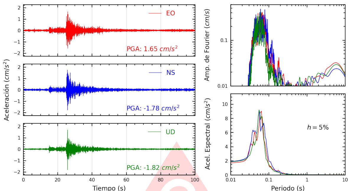
Figura A.5: Registros tiempo-historia, espectros de Fourier y de respuesta en las direcciones EO, NS y vertical de la estación JOSEO. Sismo de Chilca, Cañete - Lima del 2025-09-04, 11:32:10 (Hora local)
