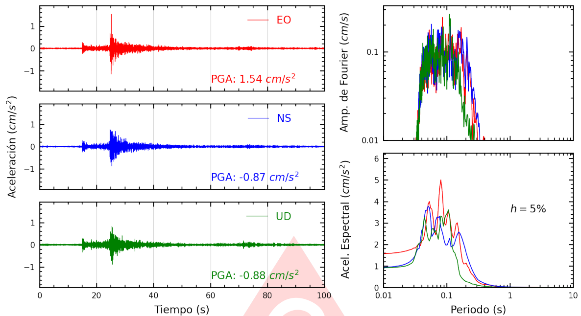
Figura A.9: Registros tiempo-historia, espectros de Fourier y de respuesta en las direcciones EO, NS y vertical de la estación ASIA. Sismo de Chilca, Cañete - Lima del 2025-09-04, 11:32:10 (Hora local)
