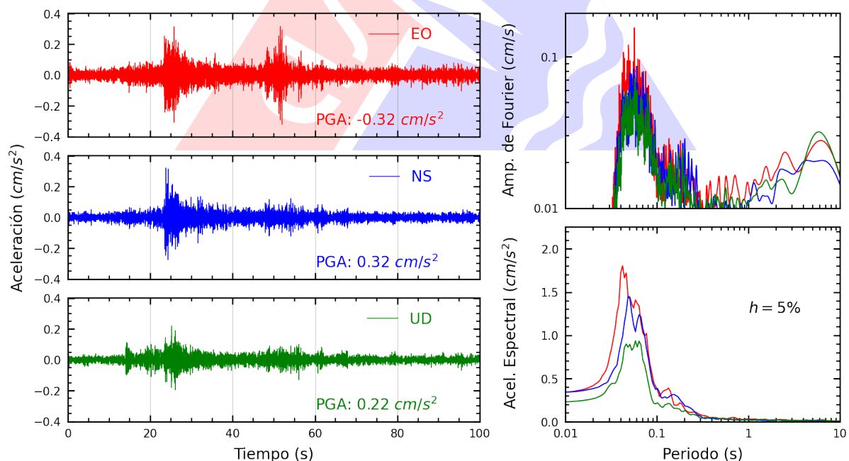
Figura A.36: Registros tiempo-historia, espectros de Fourier y de respuesta en las direcciones EO, NS y vertical de la estación INICT. Sismo de Chilca, Cañete - Lima del 2025-09-04, 11:32:10 (Hora local)
