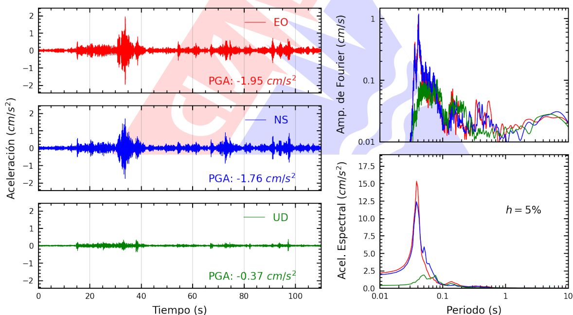
Figura A.2: Registros tiempo-historia, espectros de Fourier y de respuesta en las direcciones EO, NS y vertical de la estación DHNPE. Sismo de Chilca, Cañete - Lima del 2025-09-04, 11:32:10 (Hora local)
