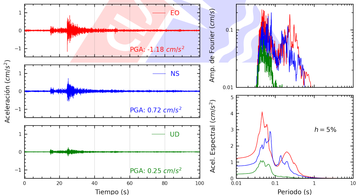
Figura A.12: Registros tiempo-historia, espectros de Fourier y de respuesta en las direcciones EO, NS y vertical de la estación UCVAT. Sismo de Chilca, Cañete - Lima del 2025-09-04, 11:32:10 (Hora local)
