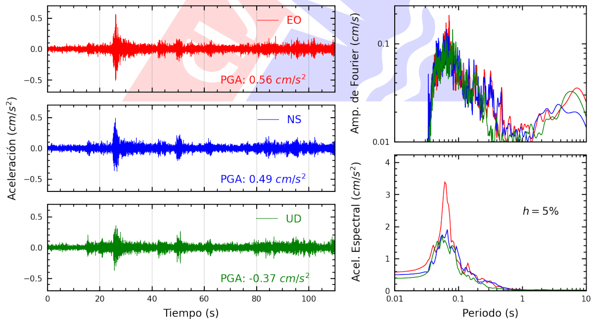
Figura A.26: Registros tiempo-historia, espectros de Fourier y de respuesta en las direcciones EO, NS y vertical de la estación MADRE. Sismo de Chilca, Cañete - Lima del 2025-09-04, 11:32:10 (Hora local)
