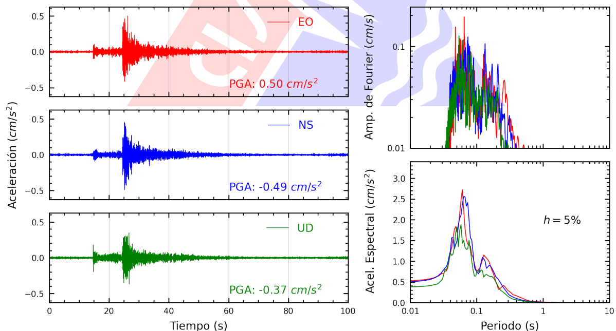
Figura A.28: Registros tiempo-historia, espectros de Fourier y de respuesta en las direcciones EO, NS y vertical de la estación JALV2. Sismo de Chilca, Cañete - Lima del 2025-09-04, 11:32:10 (Hora local)
