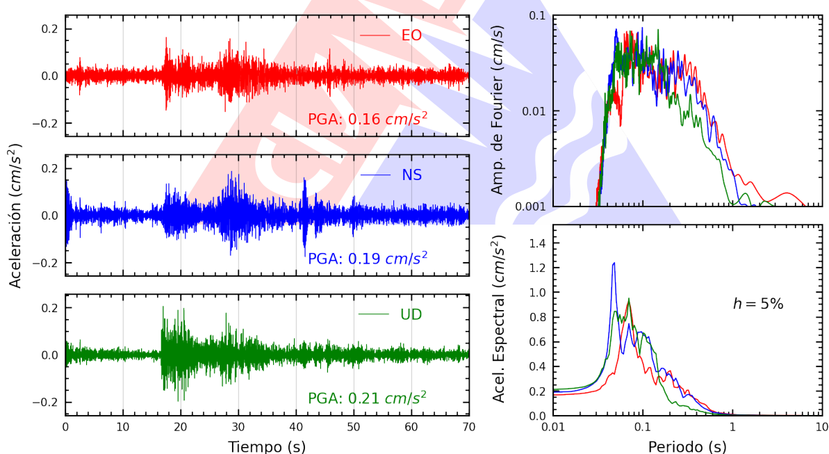
Figura A.2: Registros tiempo-historia, espectros de Fourier y de respuesta en las direcciones EO, NS y vertical de la estación UPAOP. Sismo de Sechura, Sechura - Piura del 2025-09-09, 08:10:13 (Hora local)
