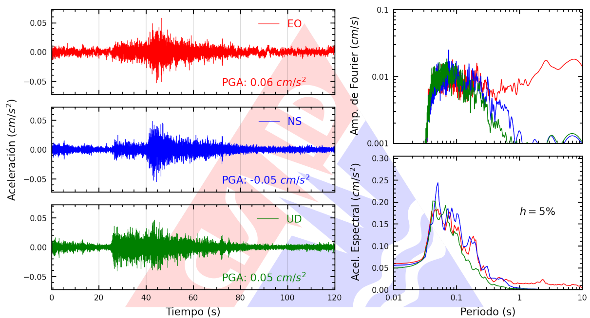
Figura A.3: Registros tiempo-historia, espectros de Fourier y de respuesta en las direcciones EO, NS y vertical de la estación SCCHI. Sismo de Sechura, Sechura - Piura del 2025-09-09, 08:10:13 (Hora local)
