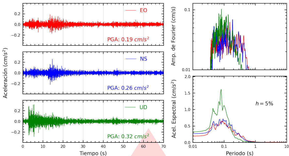
Figura A.1: Registros tiempo-historia, espectros de Fourier y de respuesta en las direcciones EO, NS y vertical de la estación SCPIU. Sismo de Sechura, Sechura - Piura del 2025-09-09, 08:10:13 (Hora local)
