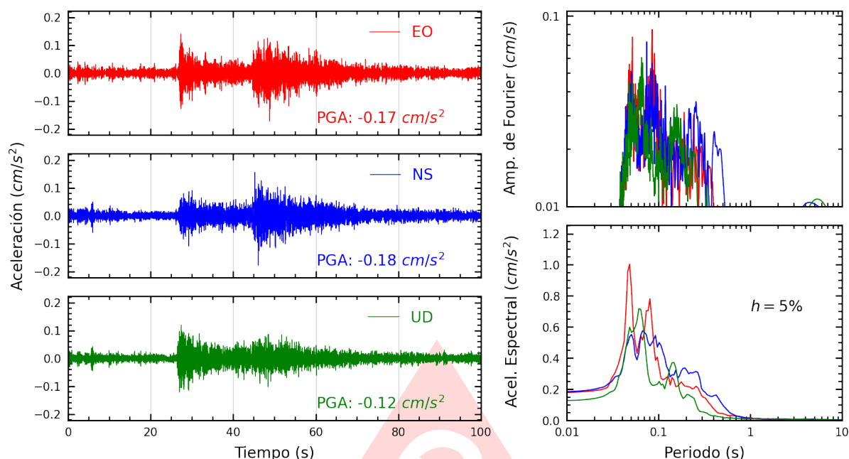
Figura A.3: Registros tiempo-historia, espectros de Fourier y de respuesta en las direcciones EO, NS y vertical de la estación CREY. Sismo de Calana, Tacna - Tacna del 2025-09-11, 19:16:21 (Hora local)
