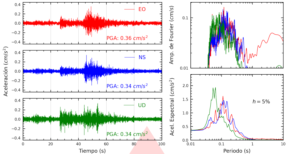
Figura A.1: Registros tiempo-historia, espectros de Fourier y de respuesta en las direcciones EO, NS y vertical de la estación UJB3. Sismo de Calana, Tacna - Tacna del 2025-09-11, 19:16:21 (Hora local)
