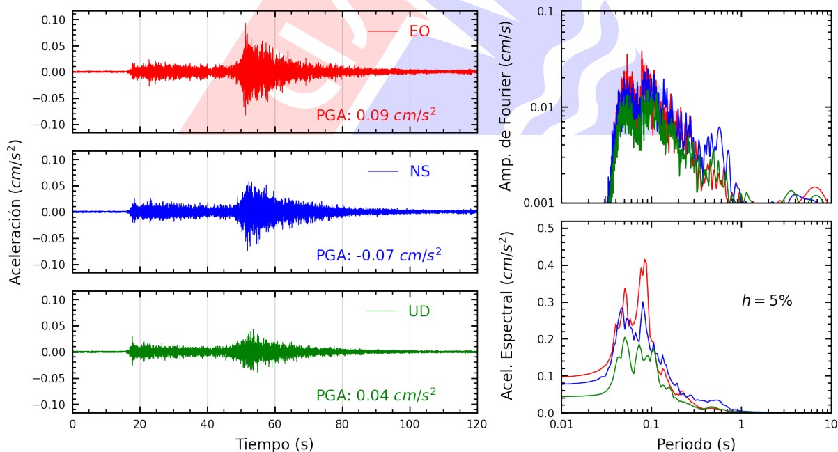
Figura A.4: Registros tiempo-historia, espectros de Fourier y de respuesta en las direcciones EO, NS y vertical de la estación UNSA2. Sismo de Calana, Tacna - Tacna del 2025-09-11, 19:16:21 (Hora local)
