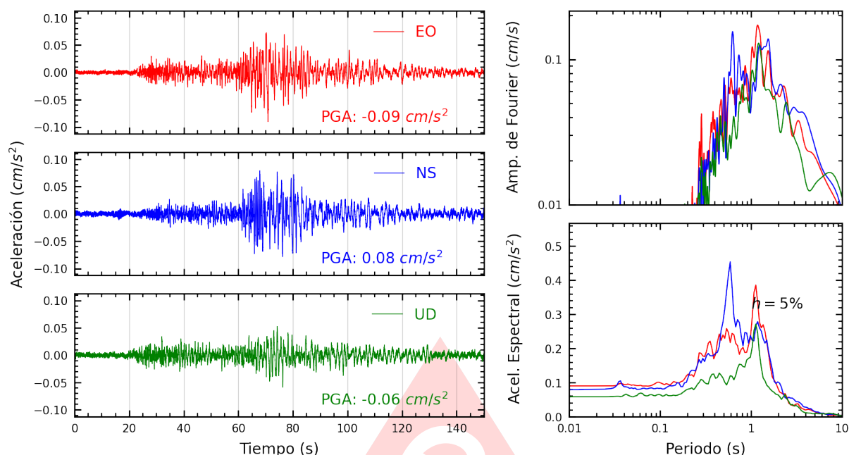
Figura A.3: Registros tiempo-historia, espectros de Fourier y de respuesta en las direcciones EO, NS y vertical de la estación UNJ. Sismo de Paita, Paita - Piura del 2025-09-15, 22:41:48 (Hora local)
