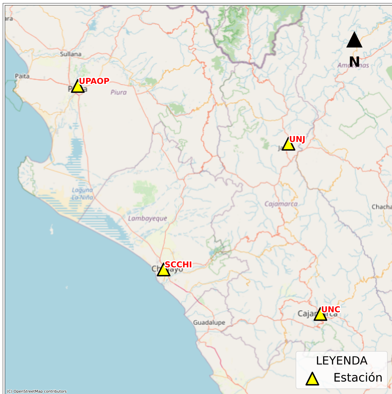
Figura 2: Mapa de ubicación de la(s) estación(es) acelerográfica(s) correspondiente(s) al Sismo de Paita, Paita - Piura del 15 de setiembre de 2025 a las 22:41:48 (hora local)
