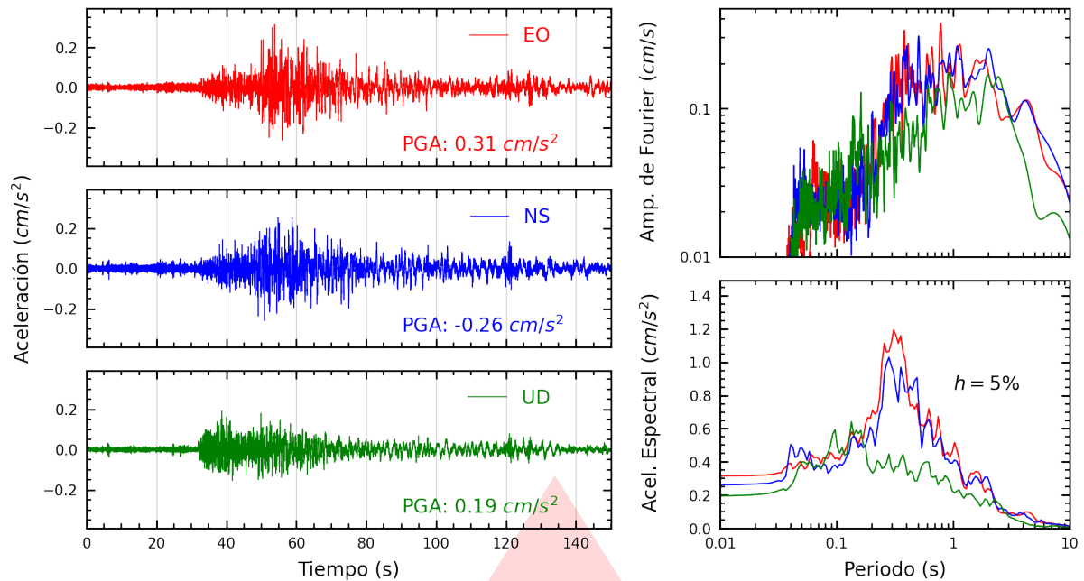
Figura A.1: Registros tiempo-historia, espectros de Fourier y de respuesta en las direcciones EO, NS y vertical de la estación UPAOP. Sismo de Paita, Paita - Piura del 2025-09-15, 22:41:48 (Hora local)
