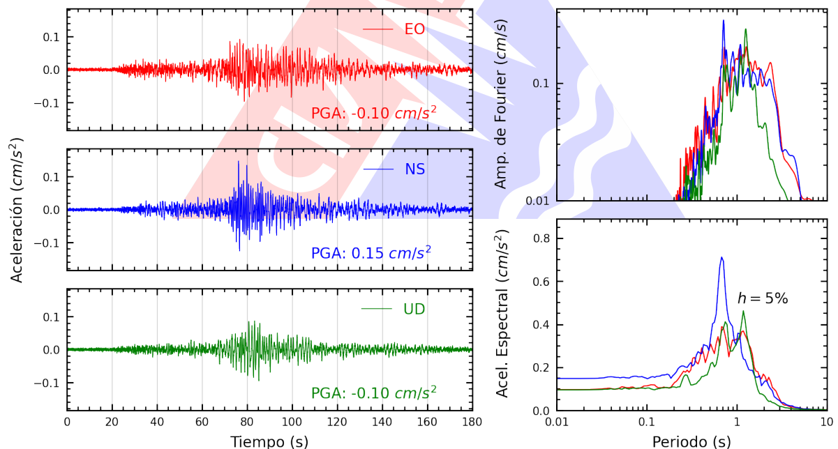
Figura A.2: Registros tiempo-historia, espectros de Fourier y de respuesta en las direcciones EO, NS y vertical de la estación UNC. Sismo de Paita, Paita - Piura del 2025-09-15, 22:41:48 (Hora local)
