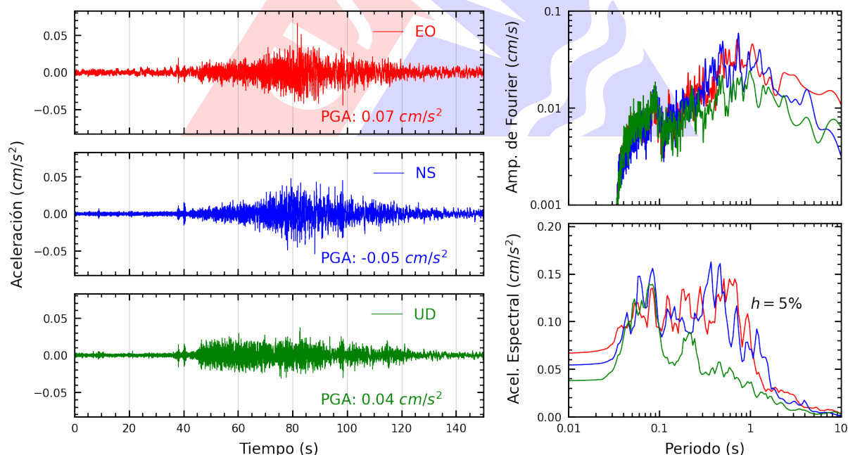
Figura A.4: Registros tiempo-historia, espectros de Fourier y de respuesta en las direcciones EO, NS y vertical de la estación SCCHI. Sismo de Paita, Paita - Piura del 2025-09-15, 22:41:48 (Hora local)
