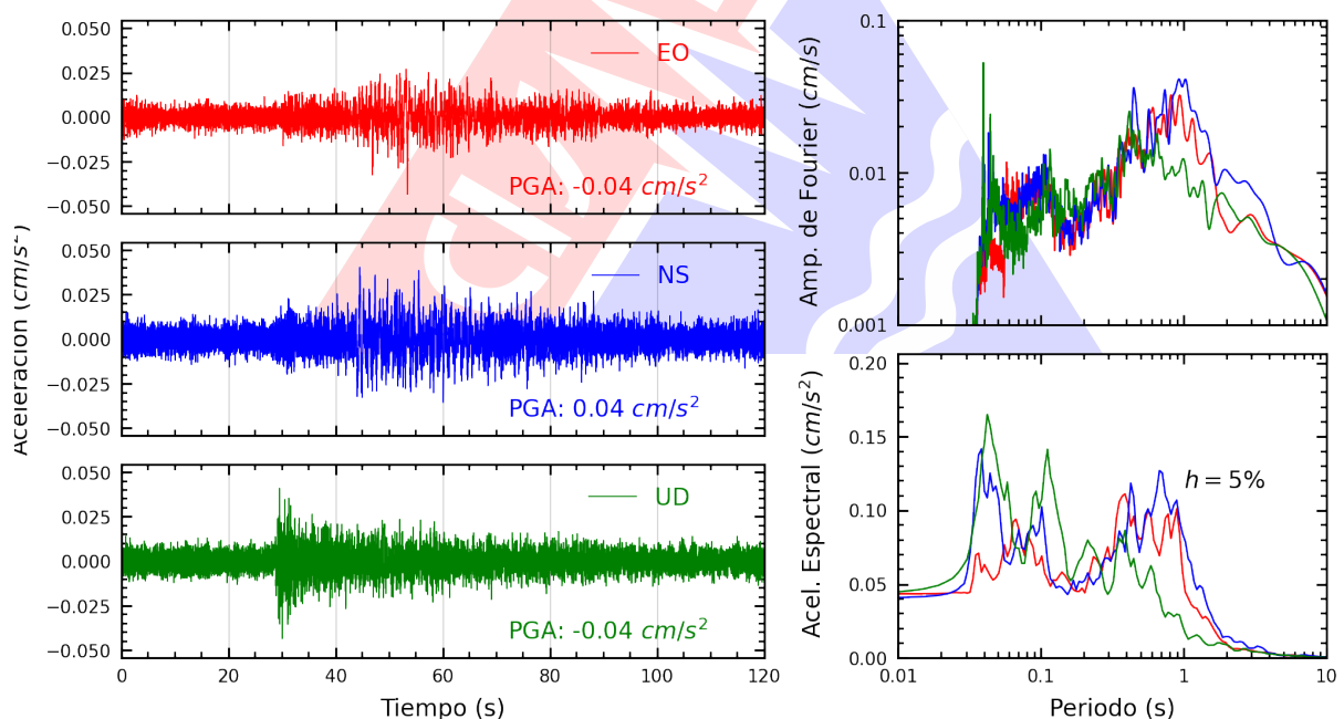
Figura A.2: Registros tiempo-historia, espectros de Fourier y de respuesta en las direcciones EO, NS y vertical de la estación UNF. Sismo de Paíta, Paíta - Piura del 2025-09-19, 05:58:58 (Hora local)
