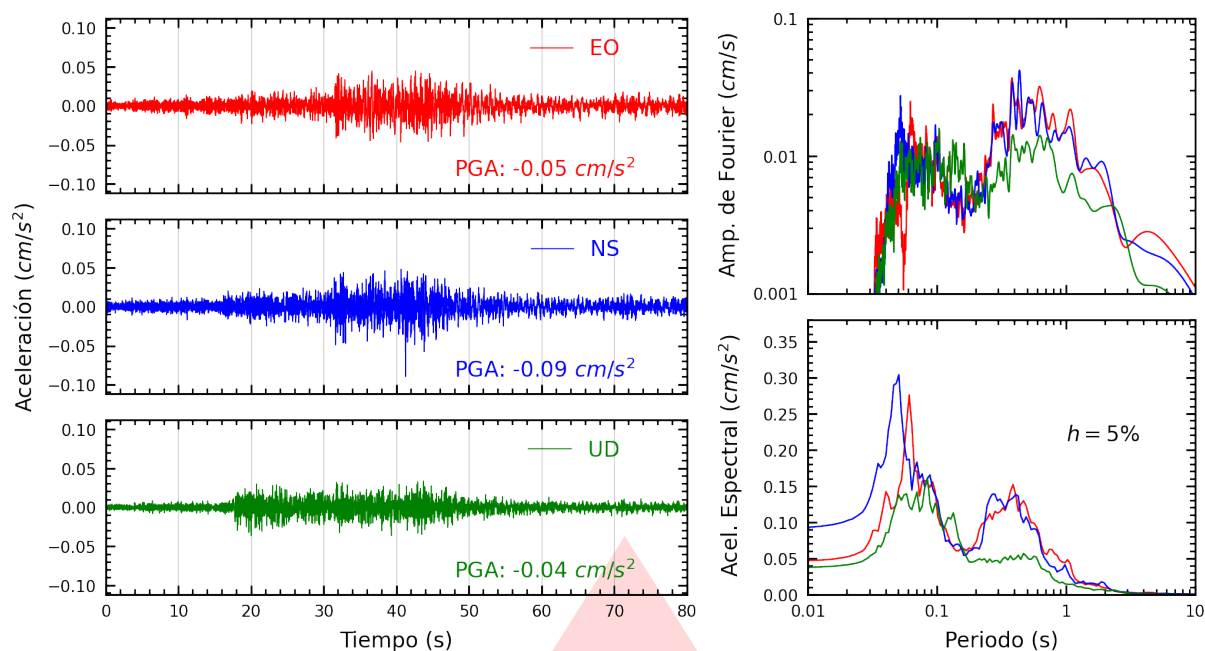
Figura A.1: Registros tiempo-historia, espectros de Fourier y de respuesta en las direcciones EO, NS y vertical de la estación UPAOP. Sismo de Paíta, Paíta - Piura del 2025-09-19, 05:58:58 (Hora local)
