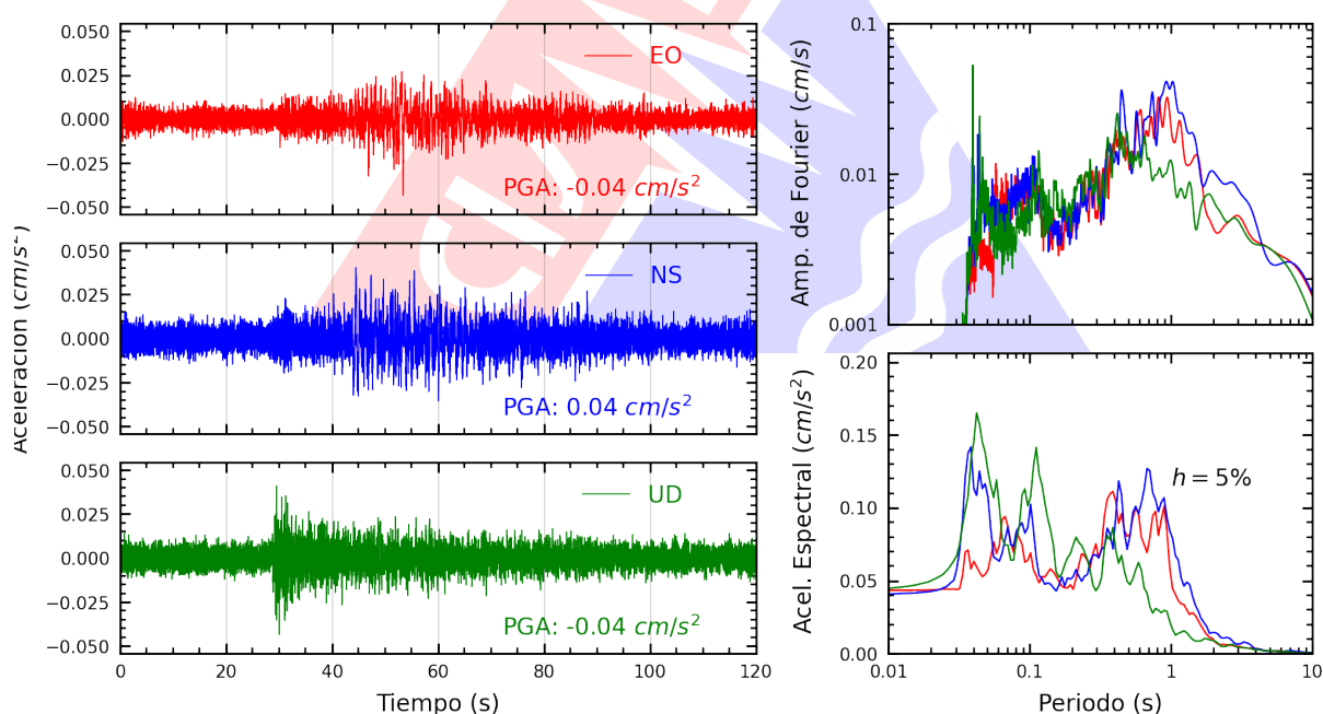
Figura A.2: Registros tiempo-historia, espectros de Fourier y de respuesta en las direcciones EO, NS y vertical de la estación UNF. Sismo de Paíta, Paíta - Piura del 2025-09-19, 05:58:58 (Hora local)
