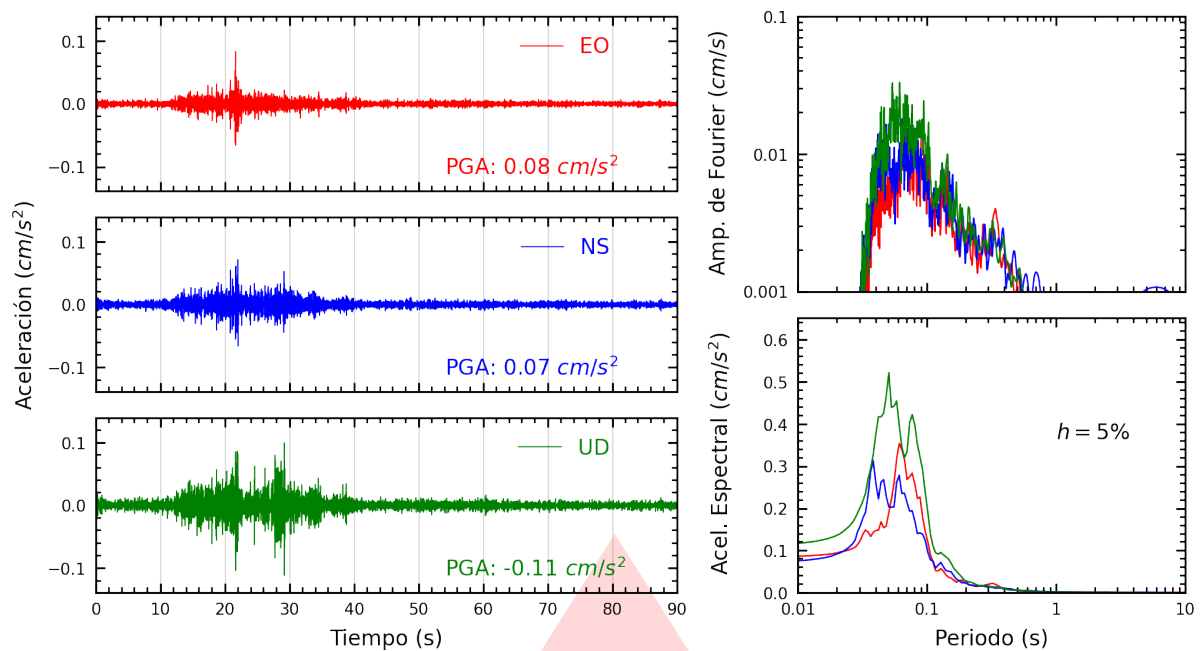
Figura A.1: Registros tiempo-historia, espectros de Fourier y de respuesta en las direcciones EO, NS y vertical de la estación SCHYO. Sismo de Colcabamba, Tayacaja - Huancavelica del 2025-09-20, 02:29:07 (Hora local)
