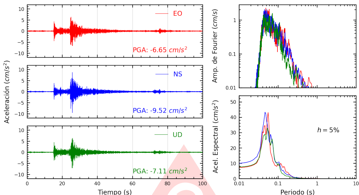
Figura A.5: Registros tiempo-historia, espectros de Fourier y de respuesta en las direcciones EO, NS y vertical de la estación SROSA. Sismo de Chilca, Cañete - Lima del 2025-09-22, 16:52:31 (Hora local)
