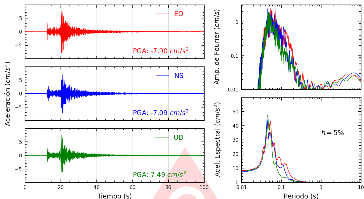
Figura A.7: Registros tiempo-historia, espectros de Fourier y de respuesta en las direcciones EO, NS y vertical de la estación JOSEO. Sismo de Chilca, Cañete - Lima del 2025-09-22, 16:52:31 (Hora local)
