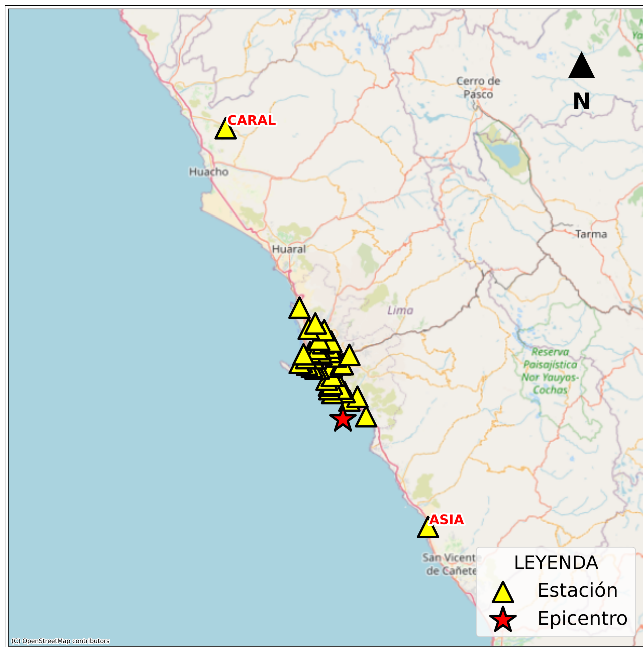
Figura 2: Mapa de ubicación de la(s) estación(es) acelerográfica(s) a nivel nacional correspondiente(s) al Sismo de Chilca, Cañete - Lima del 22 de setiembre de 2025 a las 16:52:31 (hora local)
