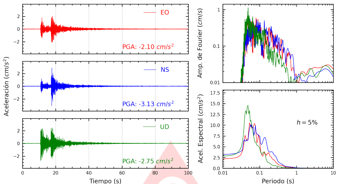
Figura A.29: Registros tiempo-historia, espectros de Fourier y de respuesta en las direcciones EO, NS y vertical de la estación USILP. Sismo de Chilca, Cañete - Lima del 2025-09-22, 16:52:31 (Hora local)
