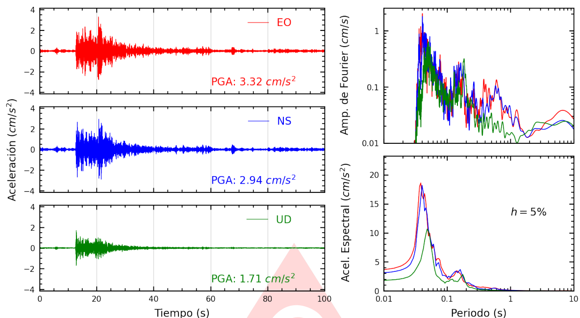
Figura A.25: Registros tiempo-historia, espectros de Fourier y de respuesta en las direcciones EO, NS y vertical de la estación DHNPE. Sismo de Chilca, Cañete - Lima del 2025-09-22, 16:52:31 (Hora local)
