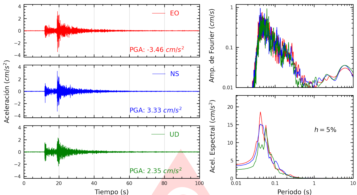
Figura A.23: Registros tiempo-historia, espectros de Fourier y de respuesta en las direcciones EO, NS y vertical de la estación USMP. Sismo de Chilca, Cañete - Lima del 2025-09-22, 16:52:31 (Hora local)
