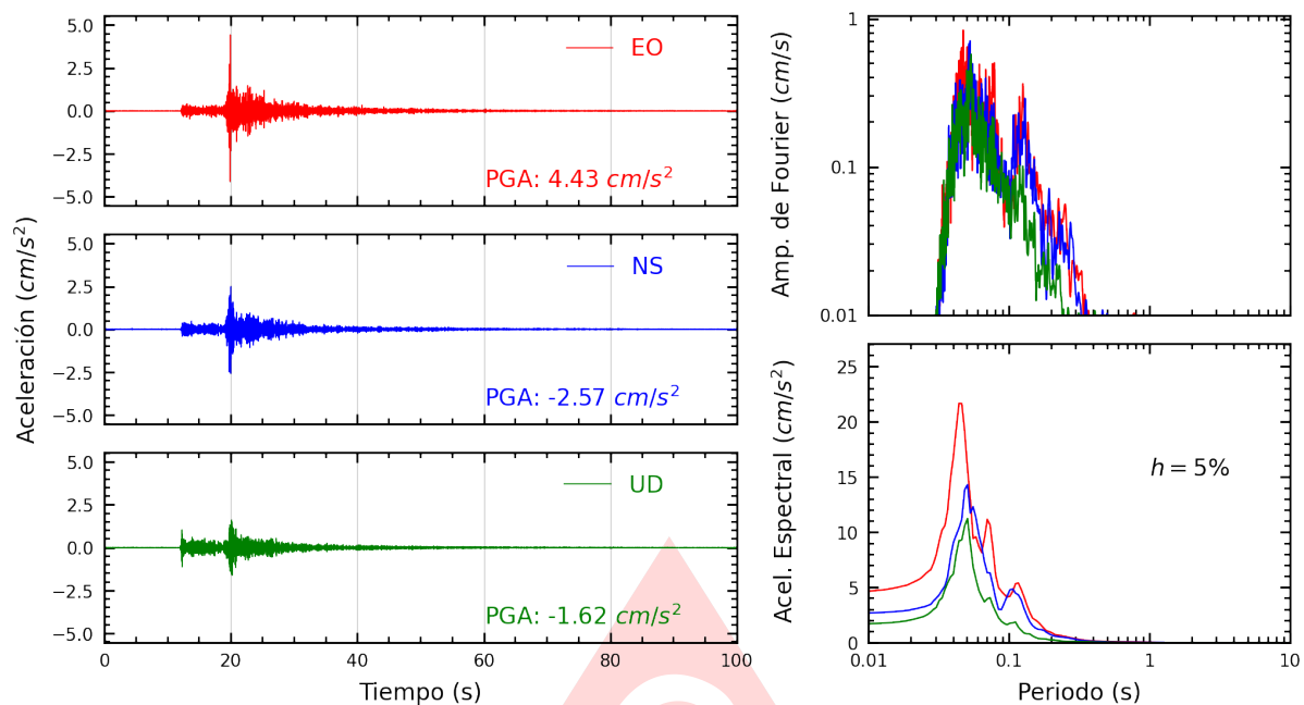
Figura A.15: Registros tiempo-historia, espectros de Fourier y de respuesta en las direcciones EO, NS y vertical de la estación ATARJ. Sismo de Chilca, Cañete - Lima del 2025-09-22, 16:52:31 (Hora local)
