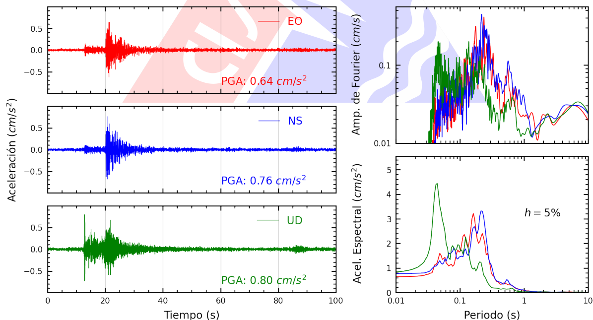
Figura A.42: Registros tiempo-historia, espectros de Fourier y de respuesta en las direcciones EO, NS y vertical de la estación DSMI. Sismo de Chilca, Cañete - Lima del 2025-09-22, 16:52:31 (Hora local)
