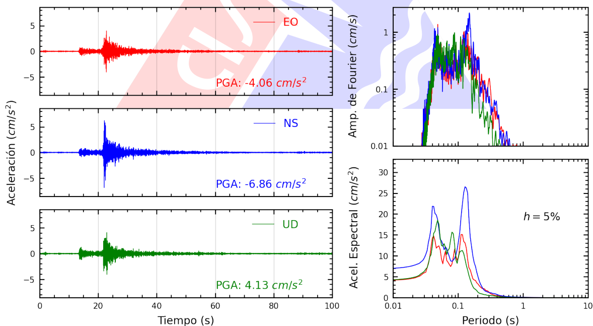
Figura A.10: Registros tiempo-historia, espectros de Fourier y de respuesta en las direcciones EO, NS y vertical de la estación CARAB. Sismo de Chilca, Cañete - Lima del 2025-09-22, 16:52:31 (Hora local)
