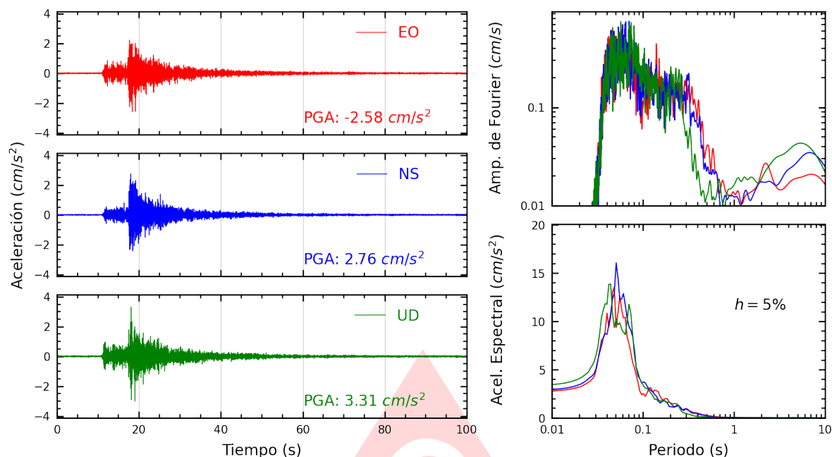
Figura A.27: Registros tiempo-historia, espectros de Fourier y de respuesta en las direcciones EO, NS y vertical de la estación SOVES. Sismo de Chilca, Cañete - Lima del 2025-09-22, 16:52:31 (Hora local)
