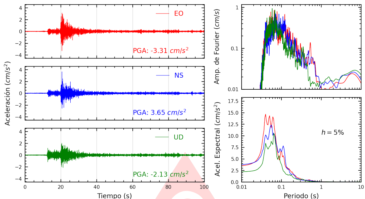
Figura A.19: Registros tiempo-historia, espectros de Fourier y de respuesta en las direcciones EO, NS y vertical de la estación SJLSV. Sismo de Chilca, Cañete - Lima del 2025-09-22, 16:52:31 (Hora local)
