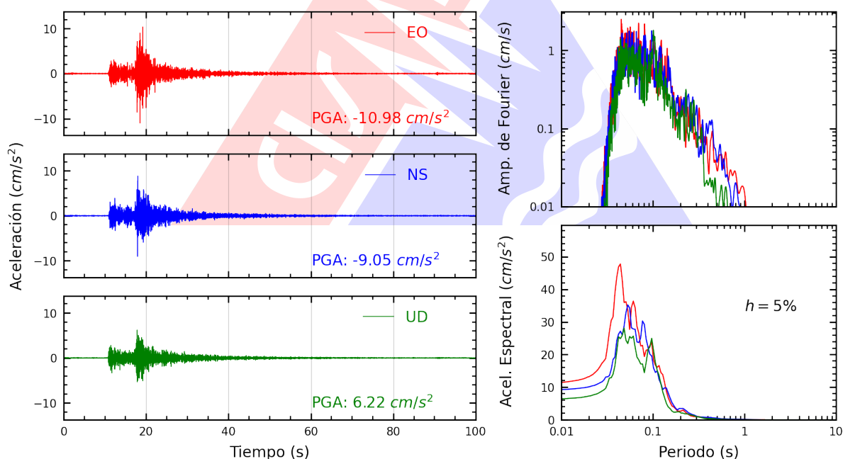
Figura A.2: Registros tiempo-historia, espectros de Fourier y de respuesta en las direcciones EO, NS y vertical de la estación PHERM. Sismo de Chilca, Cañete - Lima del 2025-09-22, 16:52:31 (Hora local)
