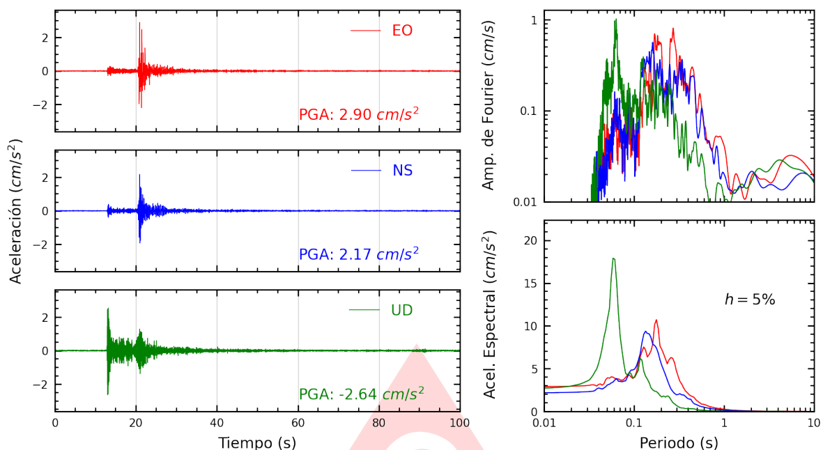
Figura A.33: Registros tiempo-historia, espectros de Fourier y de respuesta en las direcciones EO, NS y vertical de la estación ACAPU. Sismo de Chilca, Cañete - Lima del 2025-09-22, 16:52:31 (Hora local)
