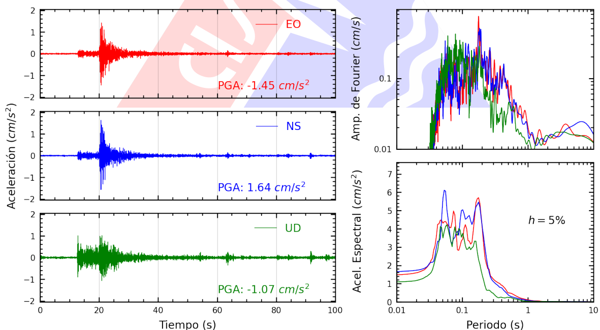
Figura A.40: Registros tiempo-historia, espectros de Fourier y de respuesta en las direcciones EO, NS y vertical de la estación RAMON. Sismo de Chilca, Cañete - Lima del 2025-09-22, 16:52:31 (Hora local)
