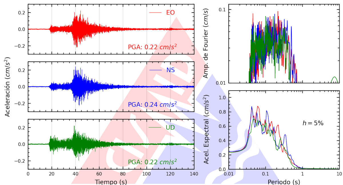
Figura A.43: Registros tiempo-historia, espectros de Fourier y de respuesta en las direcciones EO, NS y vertical de la estación CARAL. Sismo de Chilca, Cañete - Lima del 2025-09-22, 16:52:31 (Hora local)
