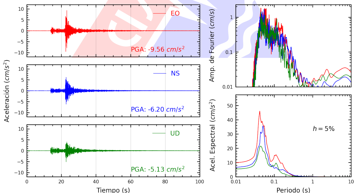
Figura A.4: Registros tiempo-historia, espectros de Fourier y de respuesta en las direcciones EO, NS y vertical de la estación AMORE. Sismo de Chilca, Cañete - Lima del 2025-09-22, 16:52:31 (Hora local)
