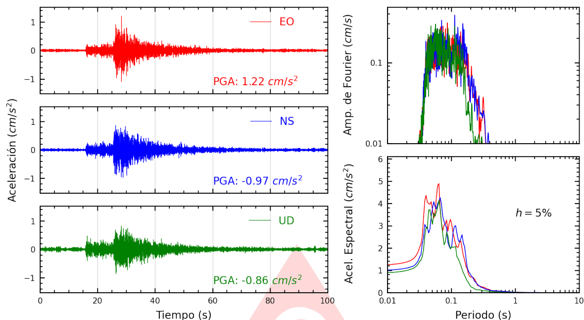
Figura A.41: Registros tiempo-historia, espectros de Fourier y de respuesta en las direcciones EO, NS y vertical de la estación ASIA. Sismo de Chilca, Cañete - Lima del 2025-09-22, 16:52:31 (Hora local)
