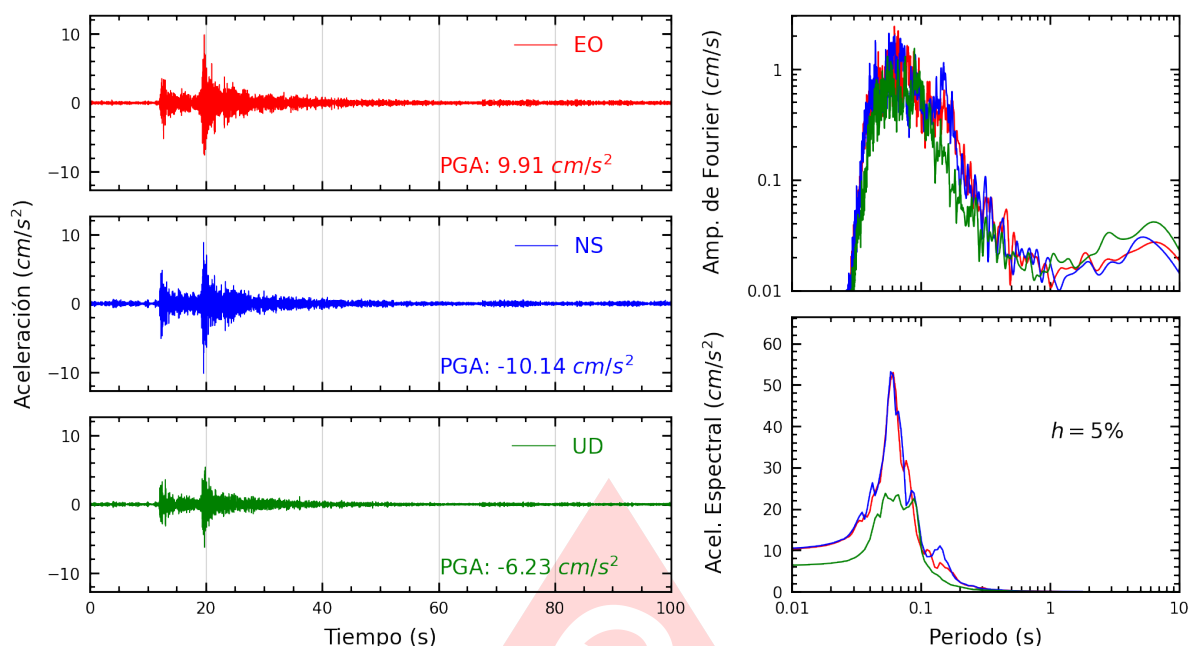
Figura A.3: Registros tiempo-historia, espectros de Fourier y de respuesta en las direcciones EO, NS y vertical de la estación USILM. Sismo de Chilca, Cañete - Lima del 2025-09-22, 16:52:31 (Hora local)
