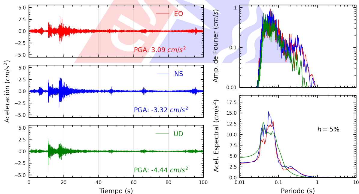
Figura A.14: Registros tiempo-historia, espectros de Fourier y de respuesta en las direcciones EO, NS y vertical de la estación PACHA. Sismo de Chilca, Cañete - Lima del 2025-09-22, 16:52:31 (Hora local)
