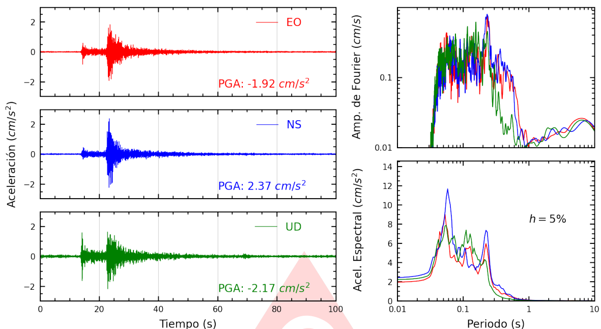
Figura A.35: Registros tiempo-historia, espectros de Fourier y de respuesta en las direcciones EO, NS y vertical de la estación MDPP. Sismo de Chilca, Cañete - Lima del 2025-09-22, 16:52:31 (Hora local)
