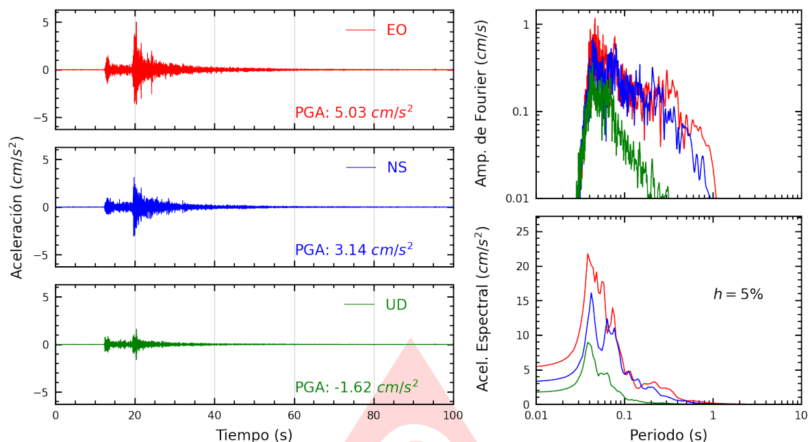
Figura A.13: Registros tiempo-historia, espectros de Fourier y de respuesta en las direcciones EO, NS y vertical de la estación UCVAT. Sismo de Chilca, Cañete - Lima del 2025-09-22, 16:52:31 (Hora local)
