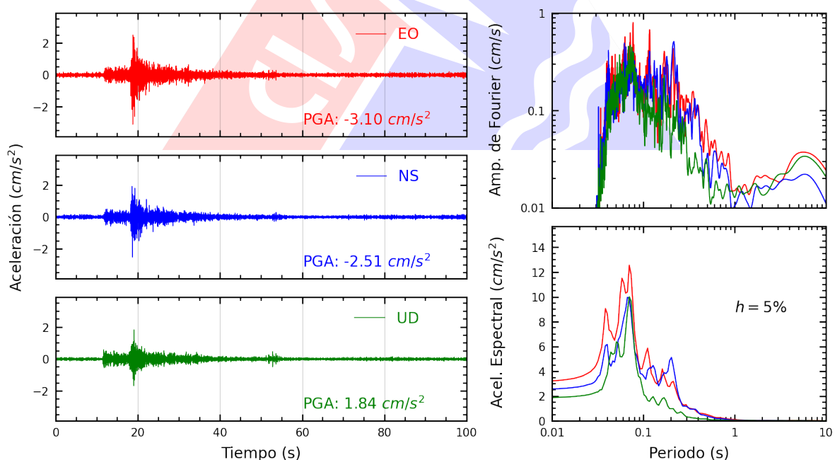
Figura A.30: Registros tiempo-historia, espectros de Fourier y de respuesta en las direcciones EO, NS y vertical de la estación SOBAR. Sismo de Chilca, Cañete - Lima del 2025-09-22, 16:52:31 (Hora local)
