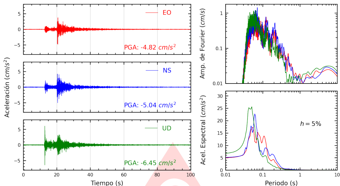
Figura A.11: Registros tiempo-historia, espectros de Fourier y de respuesta en las direcciones EO, NS y vertical de la estación SJLSC. Sismo de Chilca, Cañete - Lima del 2025-09-22, 16:52:31 (Hora local)
