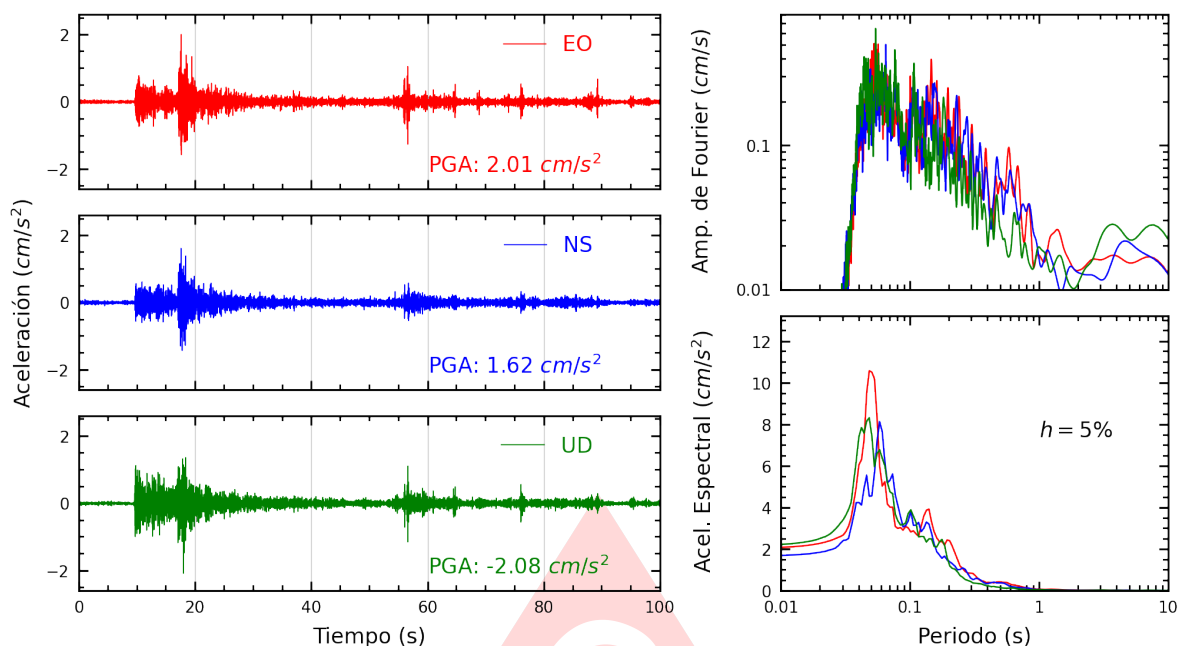
Figura A.39: Registros tiempo-historia, espectros de Fourier y de respuesta en las direcciones EO, NS y vertical de la estación PRADO. Sismo de Chilca, Cañete - Lima del 2025-09-22, 16:52:31 (Hora local)
