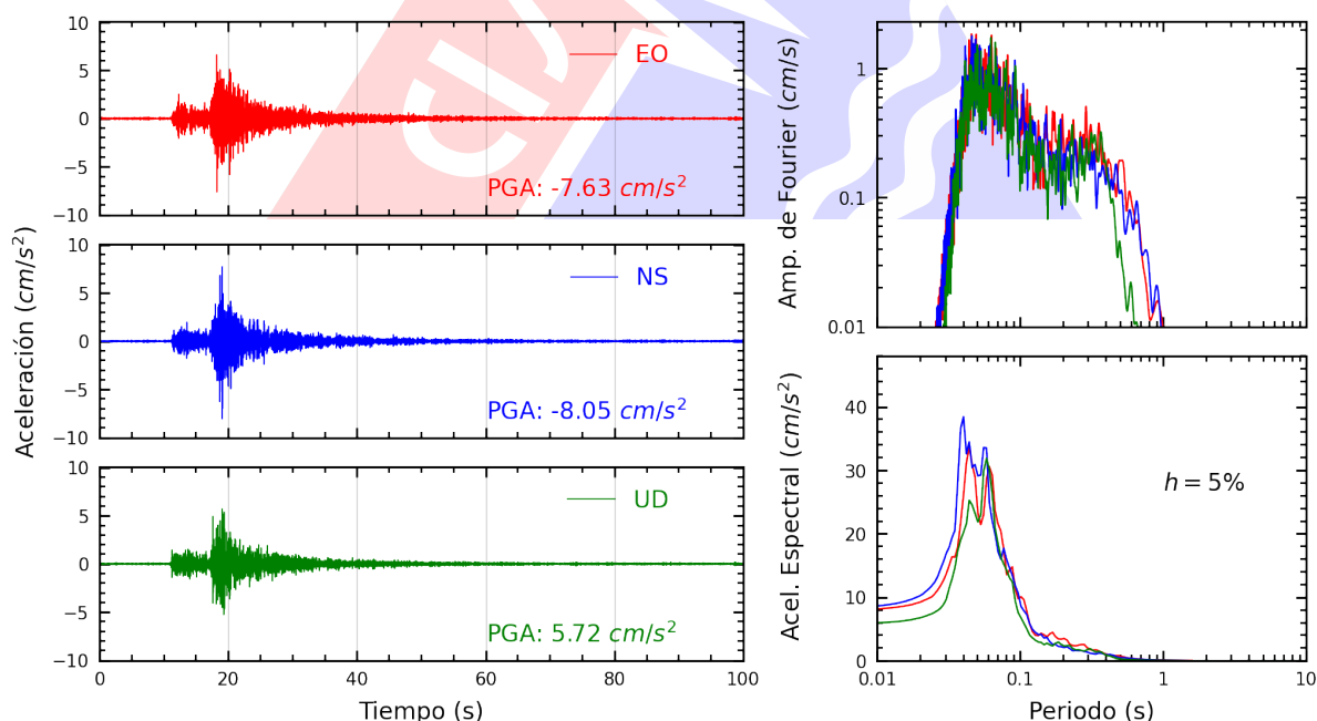
Figura A.6: Registros tiempo-historia, espectros de Fourier y de respuesta en las direcciones EO, NS y vertical de la estación UNTEL. Sismo de Chilca, Cañete - Lima del 2025-09-22, 16:52:31 (Hora local)
