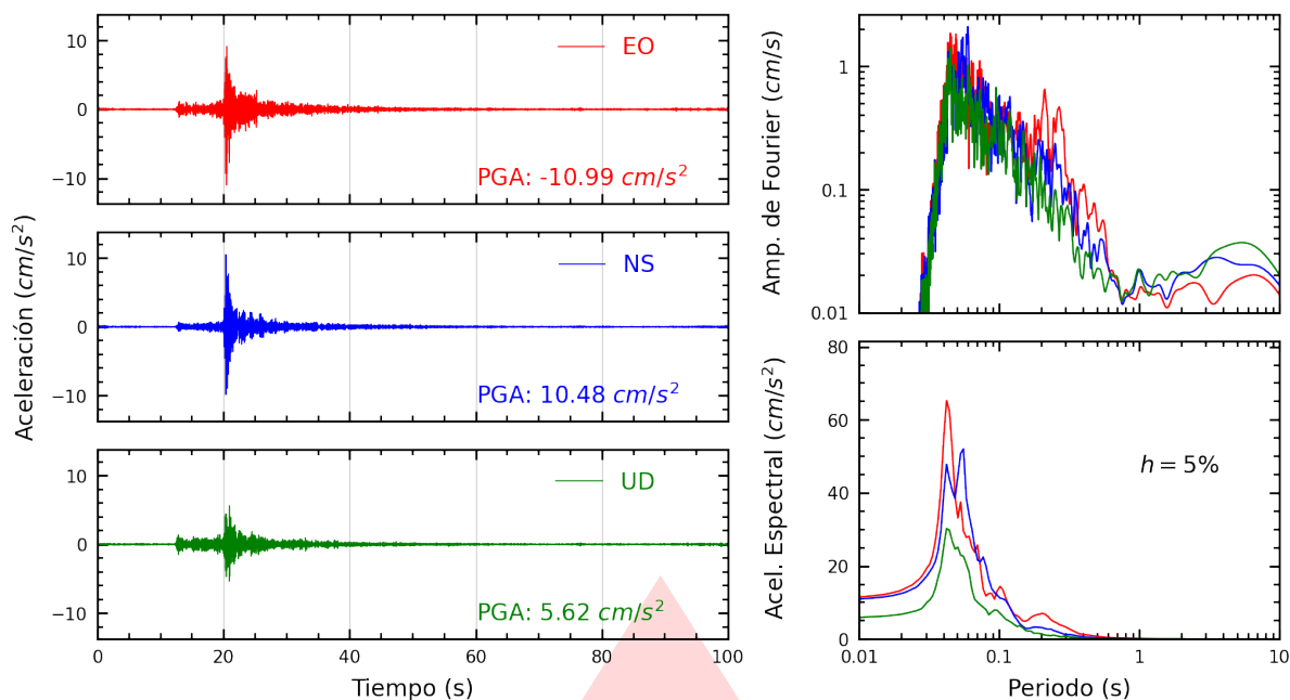
Figura A.1: Registros tiempo-historia, espectros de Fourier y de respuesta en las direcciones EO, NS y vertical de la estación INDEP. Sismo de Chilca, Cañete - Lima del 2025-09-22, 16:52:31 (Hora local)
