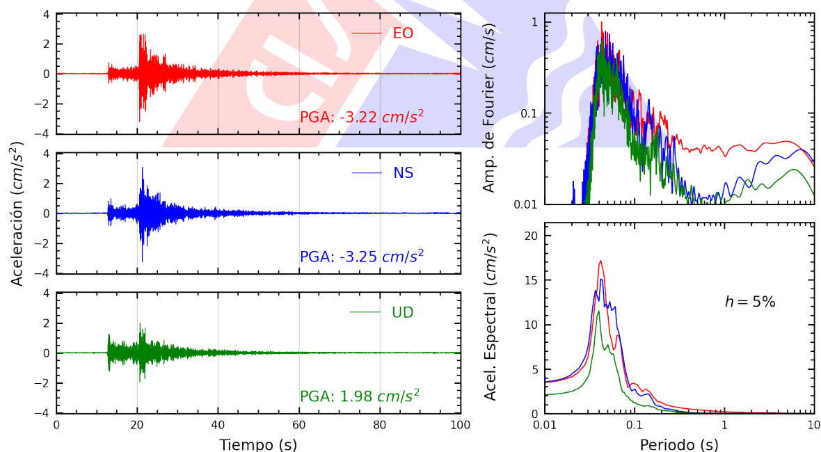
Figura A.28: Registros tiempo-historia, espectros de Fourier y de respuesta en las direcciones EO, NS y vertical de la estación SJLCE. Sismo de Chilca, Cañete - Lima del 2025-09-22, 16:52:31 (Hora local)
