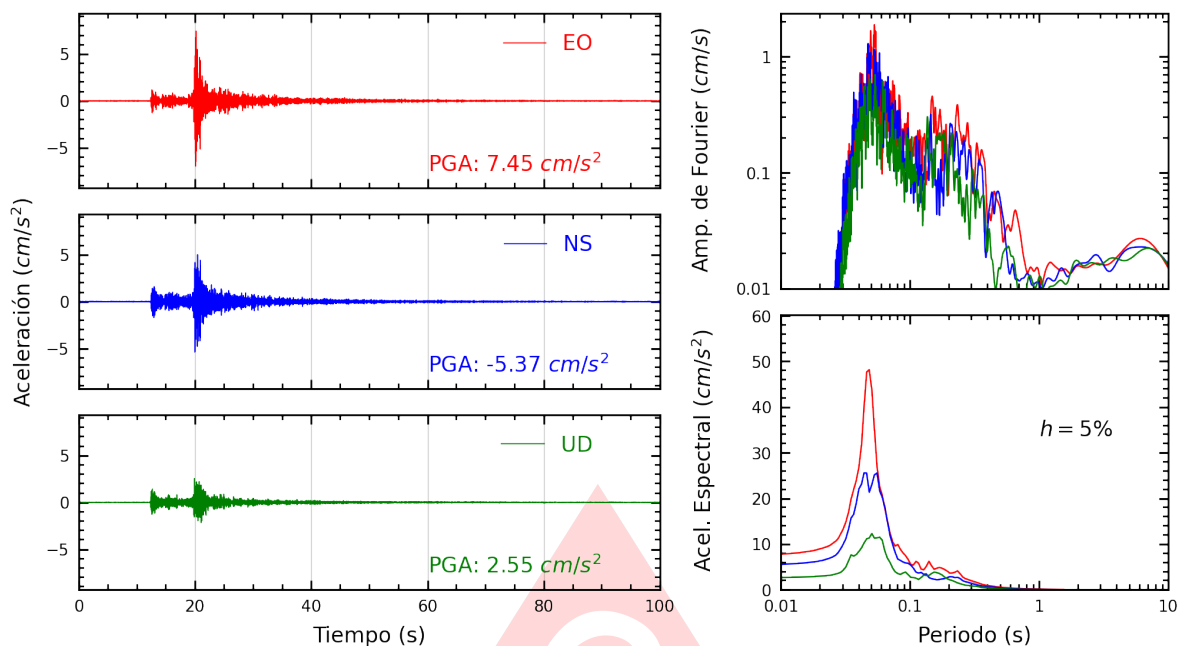
Figura A.9: Registros tiempo-historia, espectros de Fourier y de respuesta en las direcciones EO, NS y vertical de la estación FICPE. Sismo de Chilca, Cañete - Lima del 2025-09-22, 16:52:31 (Hora local)
