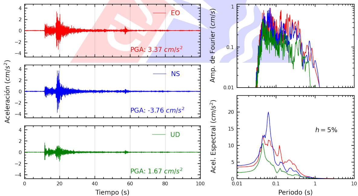
Figura A.16: Registros tiempo-historia, espectros de Fourier y de respuesta en las direcciones EO, NS y vertical de la estación BRIS2. Sismo de Chilca, Cañete - Lima del 2025-09-22, 16:52:31 (Hora local)
