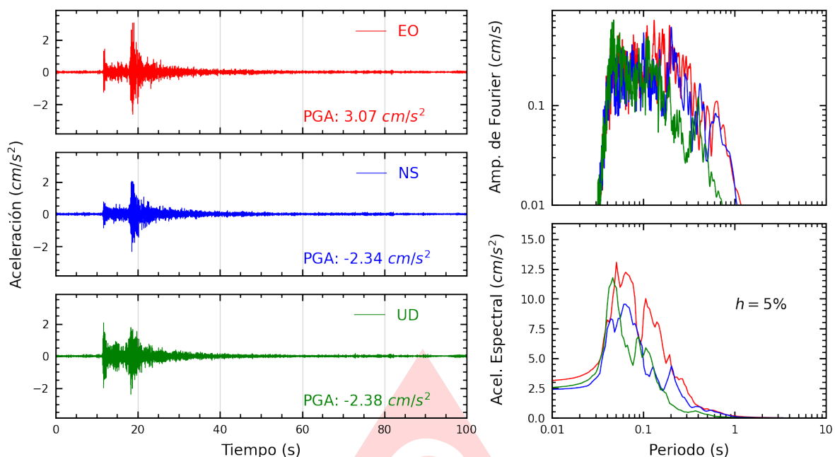
Figura A.31: Registros tiempo-historia, espectros de Fourier y de respuesta en las direcciones EO, NS y vertical de la estación SCCHO. Sismo de Chilca, Cañete - Lima del 2025-09-22, 16:52:31 (Hora local)
