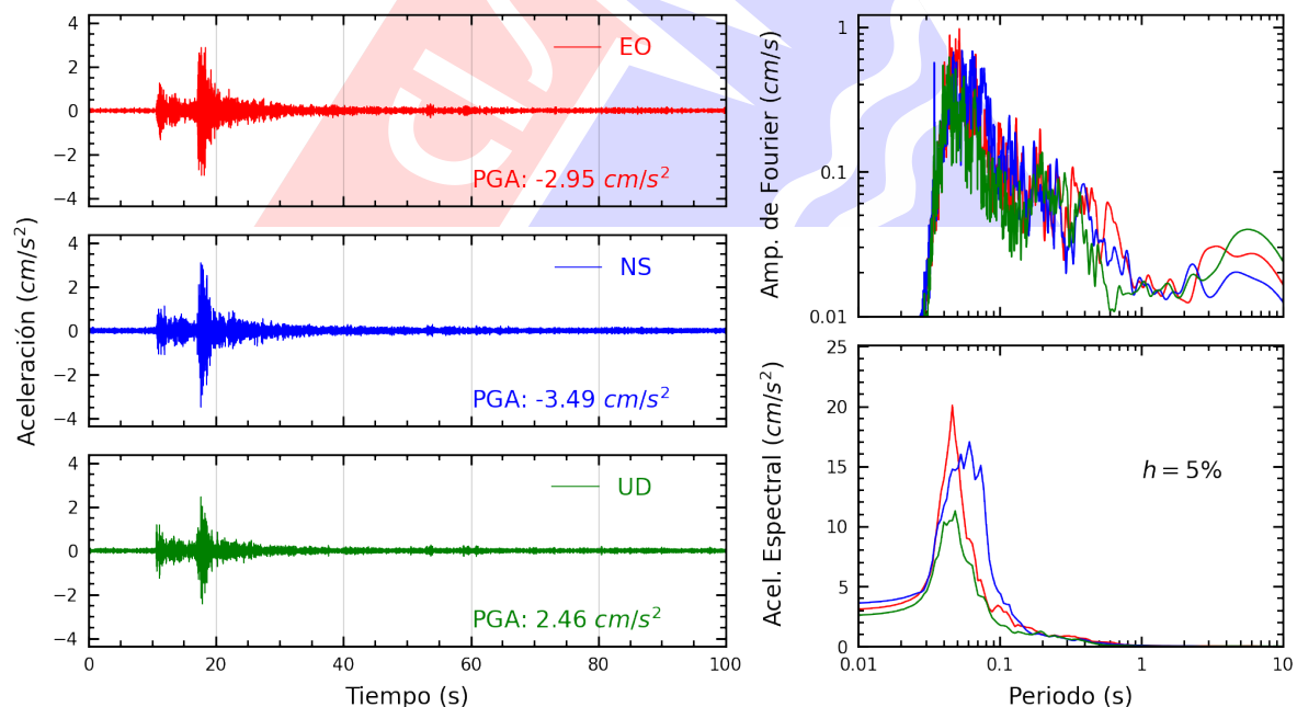
Figura A.22: Registros tiempo-historia, espectros de Fourier y de respuesta en las direcciones EO, NS y vertical de la estación UPCVI. Sismo de Chilca, Cañete - Lima del 2025-09-22, 16:52:31 (Hora local)
