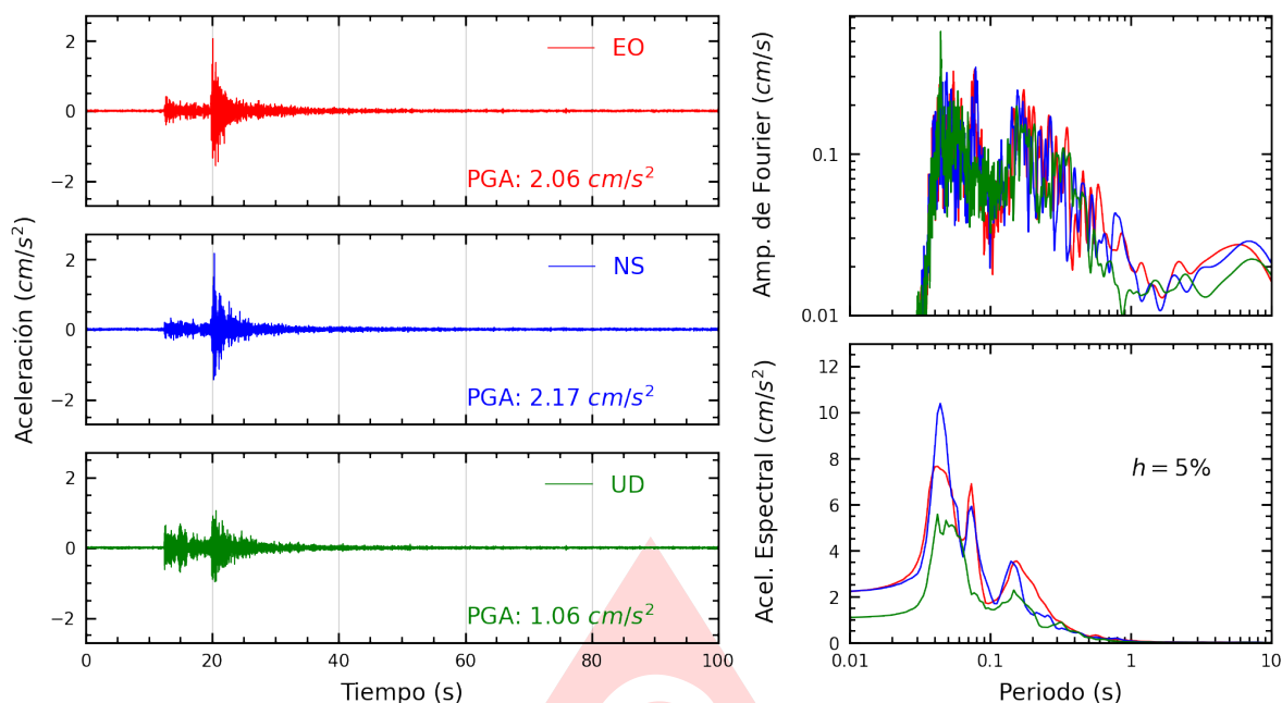
Figura A.37: Registros tiempo-historia, espectros de Fourier y de respuesta en las direcciones EO, NS y vertical de la estación BONDY. Sismo de Chilca, Cañete - Lima del 2025-09-22, 16:52:31 (Hora local)
