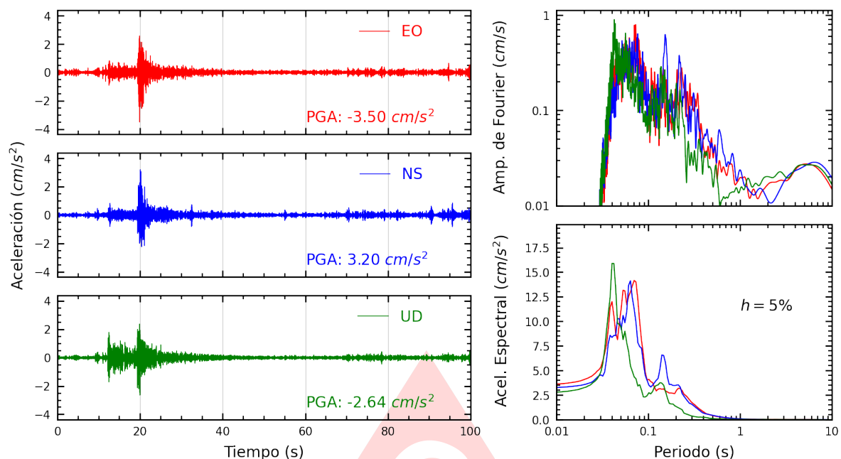
Figura A.21: Registros tiempo-historia, espectros de Fourier y de respuesta en las direcciones EO, NS y vertical de la estación UPCS. Sismo de Chilca, Cañete - Lima del 2025-09-22, 16:52:31 (Hora local)
