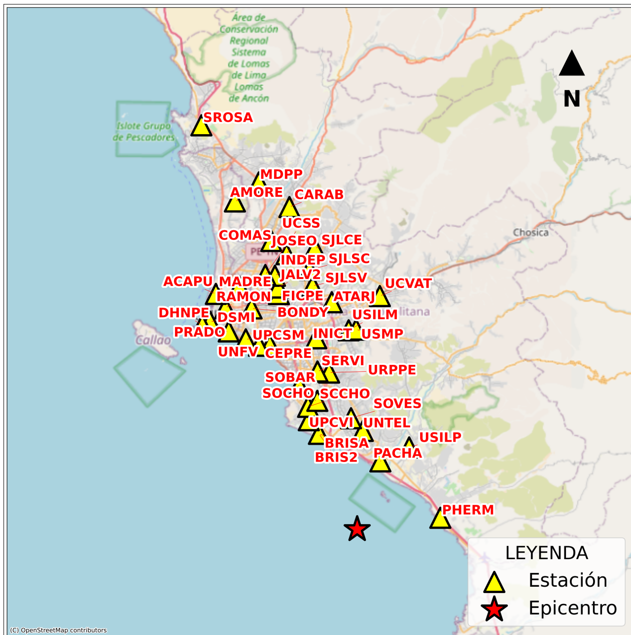
Figura 3: Mapa de ubicación de la(s) estación(es) acelerográfica(s) en Lima Metropolitana correspondiente(s) al Sismo de Chilca, Cañete - Lima del 22 de setiembre de 2025 a las 16:52:31 (hora local)
