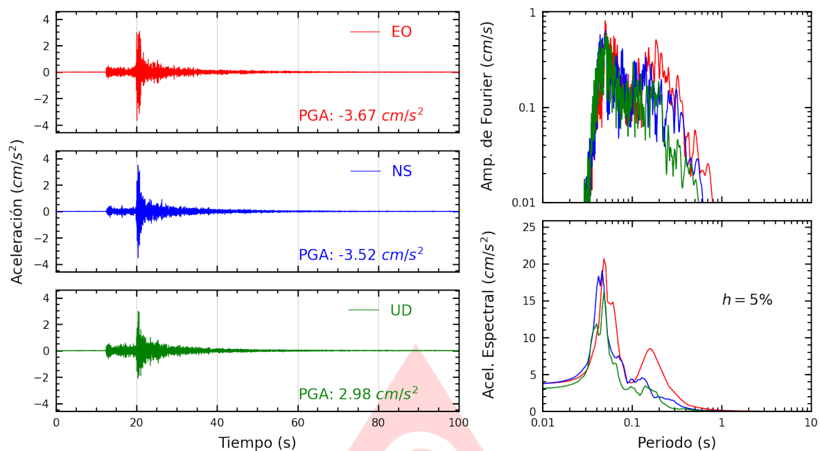
Figura A.17: Registros tiempo-historia, espectros de Fourier y de respuesta en las direcciones EO, NS y vertical de la estación JALV2. Sismo de Chilca, Cañete - Lima del 2025-09-22, 16:52:31 (Hora local)
