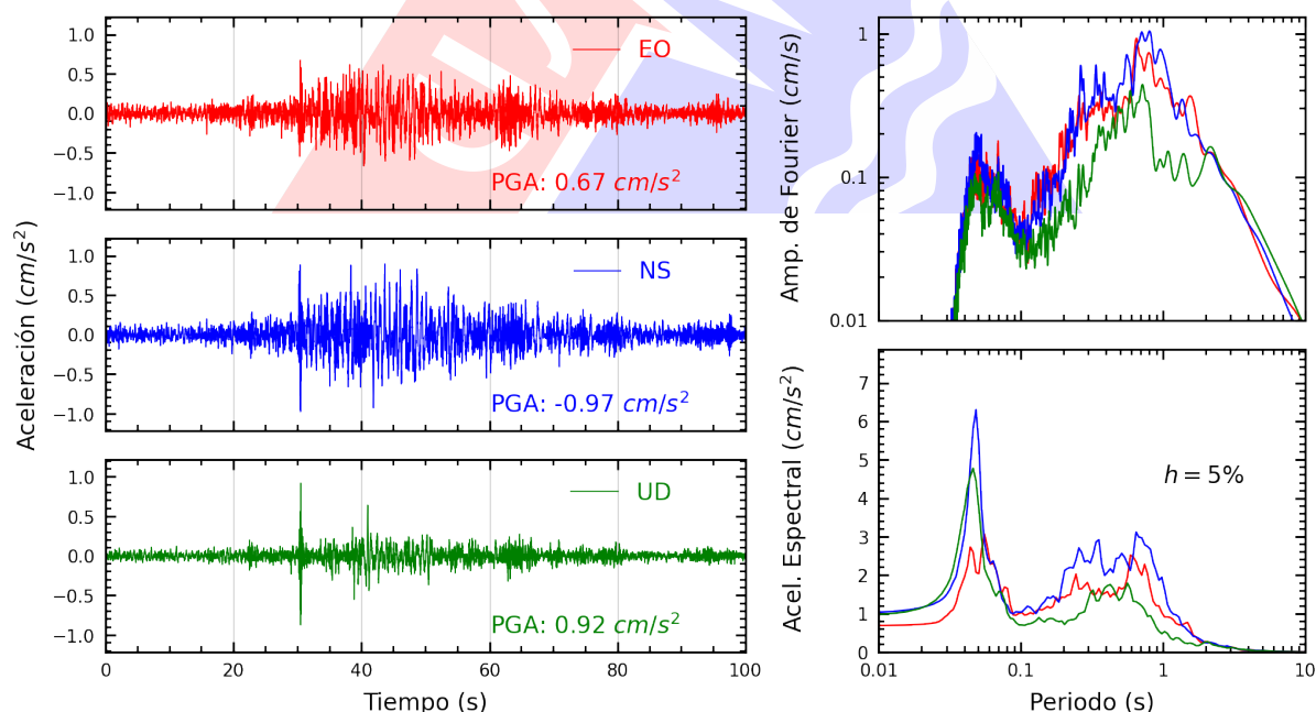
Figura A.4: Registros tiempo-historia, espectros de Fourier y de respuesta en las direcciones EO, NS y vertical de la estación BRIS2. Sismo de Lomas, Caraveli - Arequipa del 2025-09-23, 12:39:18 (Hora local)
