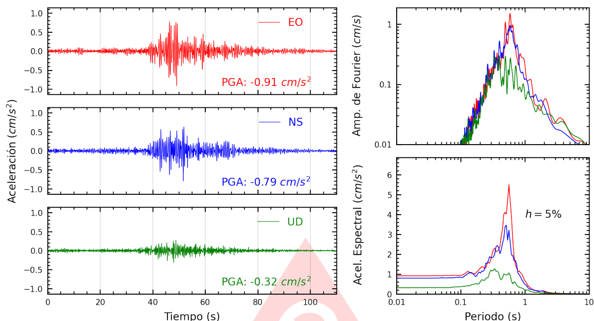
Figura A.5: Registros tiempo-historia, espectros de Fourier y de respuesta en las direcciones EO, NS y vertical de la estación CARAL. Sismo de Lomas, Caraveli - Arequipa del 2025-09-23, 12:39:18 (Hora local)
