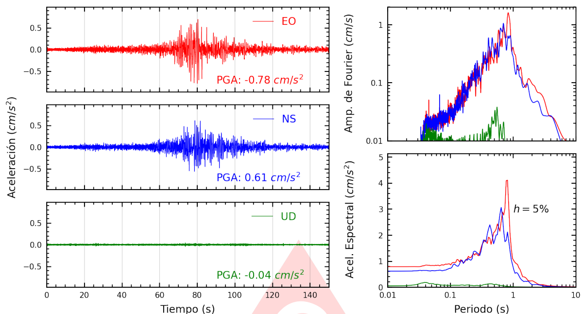
Figura A.11: Registros tiempo-historia, espectros de Fourier y de respuesta en las direcciones EO, NS y vertical de la estación UCVAT. Sismo de Lomas, Caraveli - Arequipa del 2025-09-23, 12:39:18 (Hora local)
