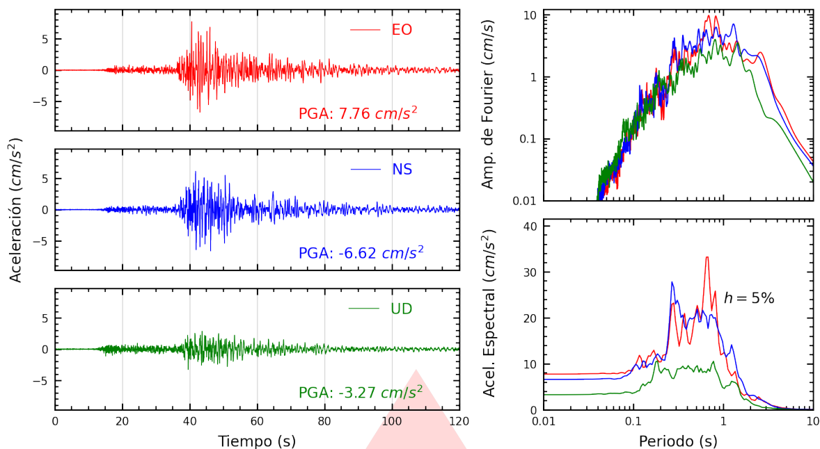
Figura A.1: Registros tiempo-historia, espectros de Fourier y de respuesta en las direcciones EO, NS y vertical de la estación UNICA. Sismo de Lomas, Caraveli - Arequipa del 2025-09-23, 12:39:18 (Hora local)
