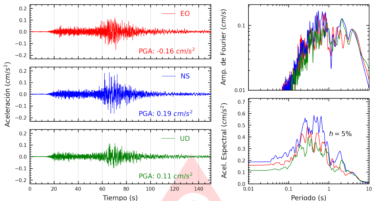
Figura A.39: Registros tiempo-historia, espectros de Fourier y de respuesta en las direcciones EO, NS y vertical de la estación UNSA2. Sismo de Lomas, Caraveli - Arequipa del 2025-09-23, 12:39:18 (Hora local)
