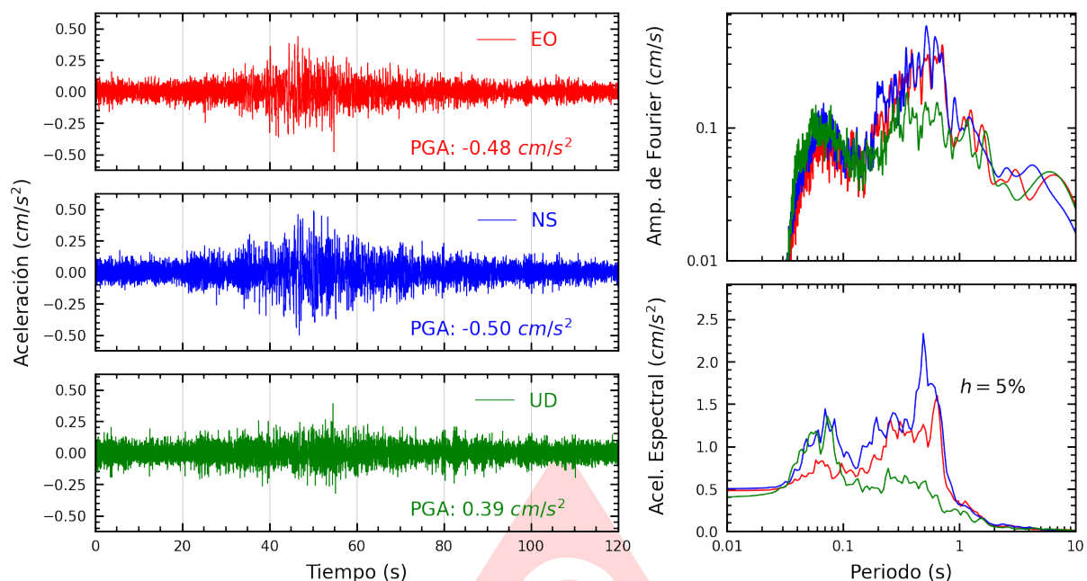
Figura A.23: Registros tiempo-historia, espectros de Fourier y de respuesta en las direcciones EO, NS y vertical de la estación SJLSC. Sismo de Lomas, Caraveli - Arequipa del 2025-09-23, 12:39:18 (Hora local)
