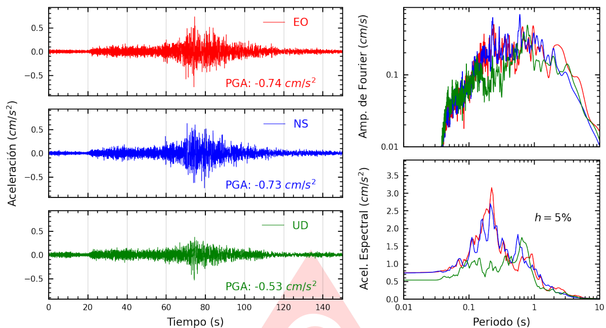
Figura A.13: Registros tiempo-historia, espectros de Fourier y de respuesta en las direcciones EO, NS y vertical de la estación ASIA. Sismo de Lomas, Caraveli - Arequipa del 2025-09-23, 12:39:18 (Hora local)
