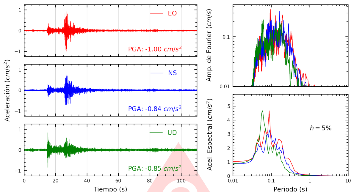
Figura A.3: Registros tiempo-historia, espectros de Fourier y de respuesta en las direcciones EO, NS y vertical de la estación UJBG2. Sismo de Tacna, Tacna - Tacna del 2025-09-26, 22:31:50 (Hora local)
