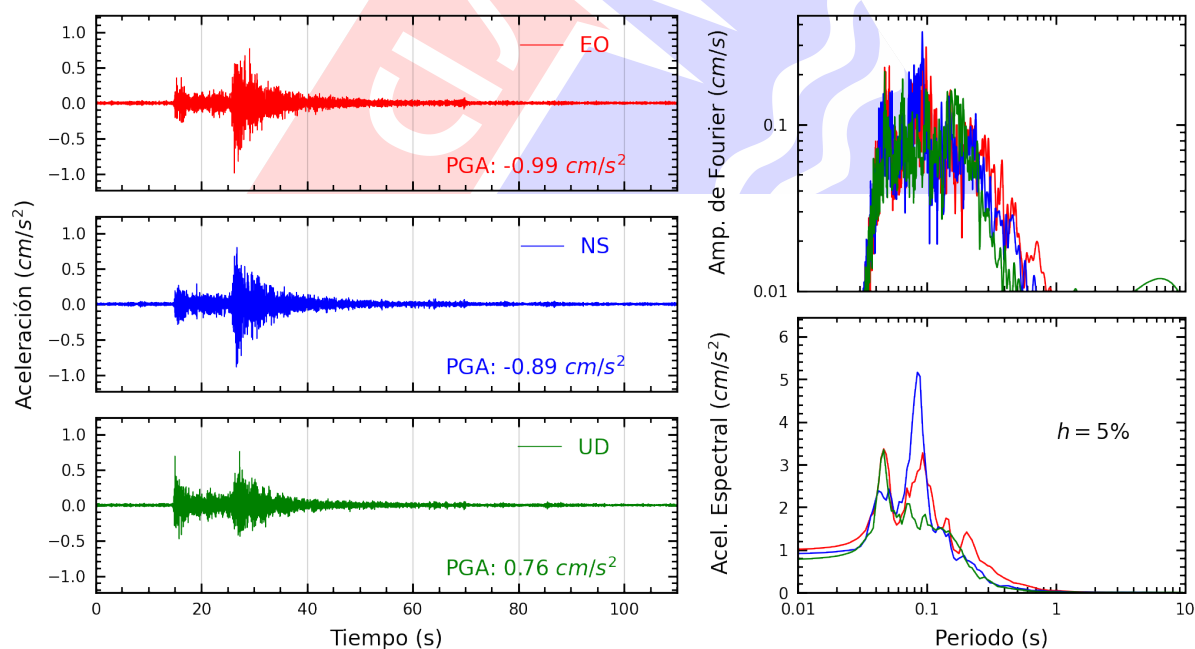
Figura A.4: Registros tiempo-historia, espectros de Fourier y de respuesta en las direcciones EO, NS y vertical de la estación CREY. Sismo de Tacna, Tacna - Tacna del 2025-09-26, 22:31:50 (Hora local)
