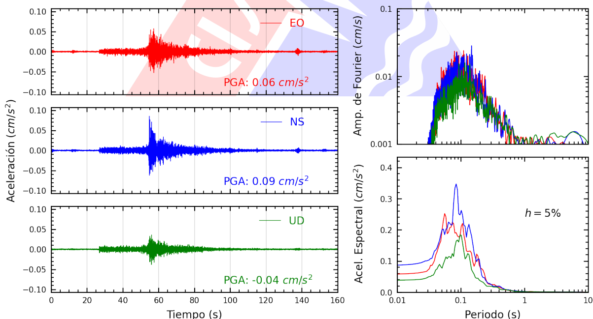
Figura A.6: Registros tiempo-historia, espectros de Fourier y de respuesta en las direcciones EO, NS y vertical de la estación UNSA2. Sismo de Tacna, Tacna - Tacna del 2025-09-26, 22:31:50 (Hora local)
