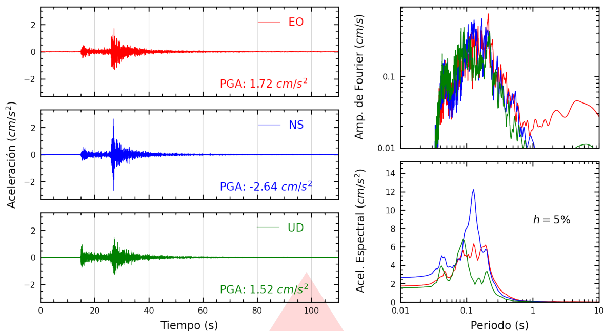
Figura A.1: Registros tiempo-historia, espectros de Fourier y de respuesta en las direcciones EO, NS y vertical de la estación UJBG3. Sismo de Tacna, Tacna - Tacna del 2025-09-26, 22:31:50 (Hora local)
