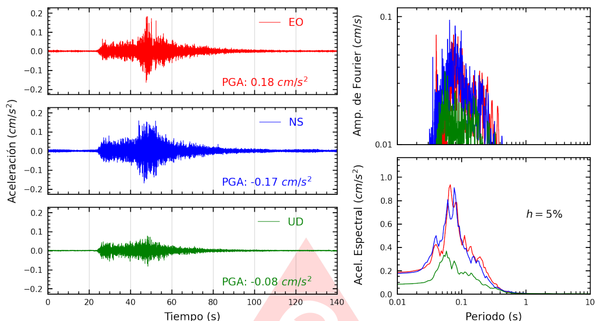
Figura A.5: Registros tiempo-historia, espectros de Fourier y de respuesta en las direcciones EO, NS y vertical de la estación UNAM. Sismo de Tacna, Tacna - Tacna del 2025-09-26, 22:31:50 (Hora local)
