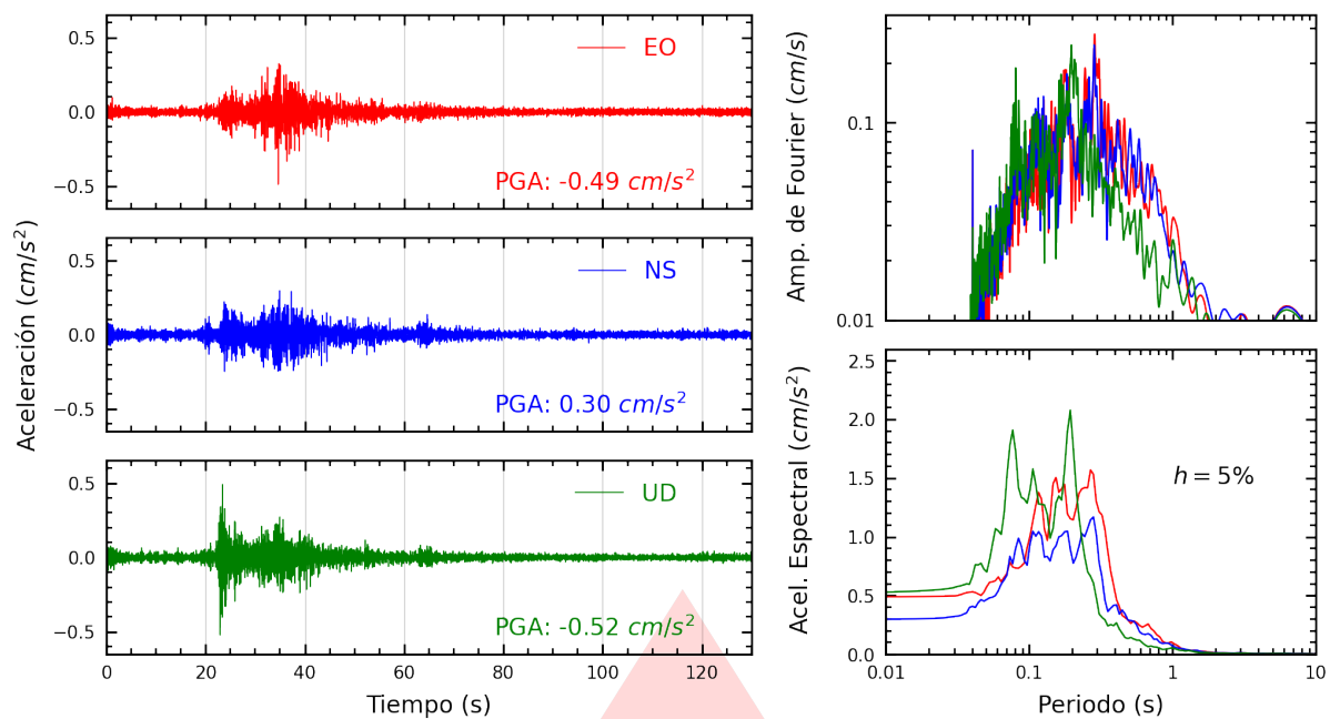
Figura A.1: Registros tiempo-historia, espectros de Fourier y de respuesta en las direcciones EO, NS y vertical de la estación UNICA. Sismo de Ica, Ica - Ica del 2025-10-12, 06:14:26 (Hora local)
