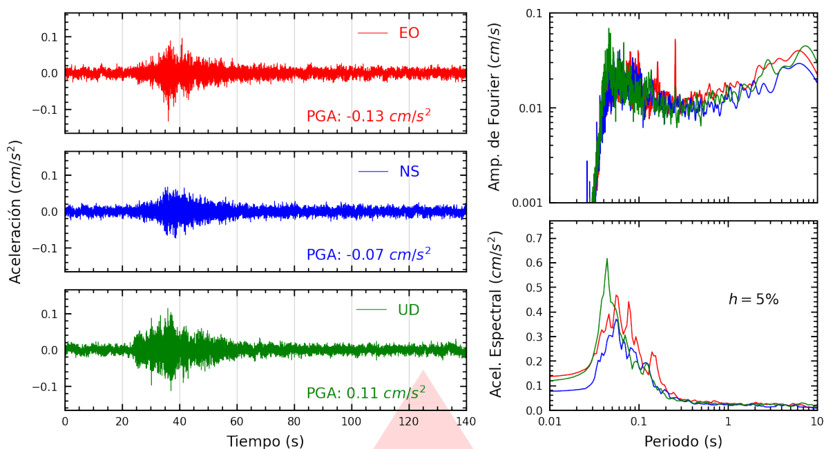
Figura A.17: Registros tiempo-historia, espectros de Fourier y de respuesta en las direcciones EO, NS y vertical de la estación USILP. Sismo de Mala, Cañete - Lima del 2025-10-15, 23:56:28 (Hora local)
