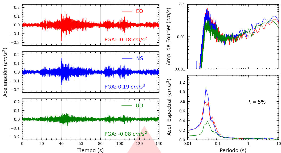
Figura A.13: Registros tiempo-historia, espectros de Fourier y de respuesta en las direcciones EO, NS y vertical de la estación CEPRE. Sismo de Mala, Cañete - Lima del 2025-10-15, 23:56:28 (Hora local)
