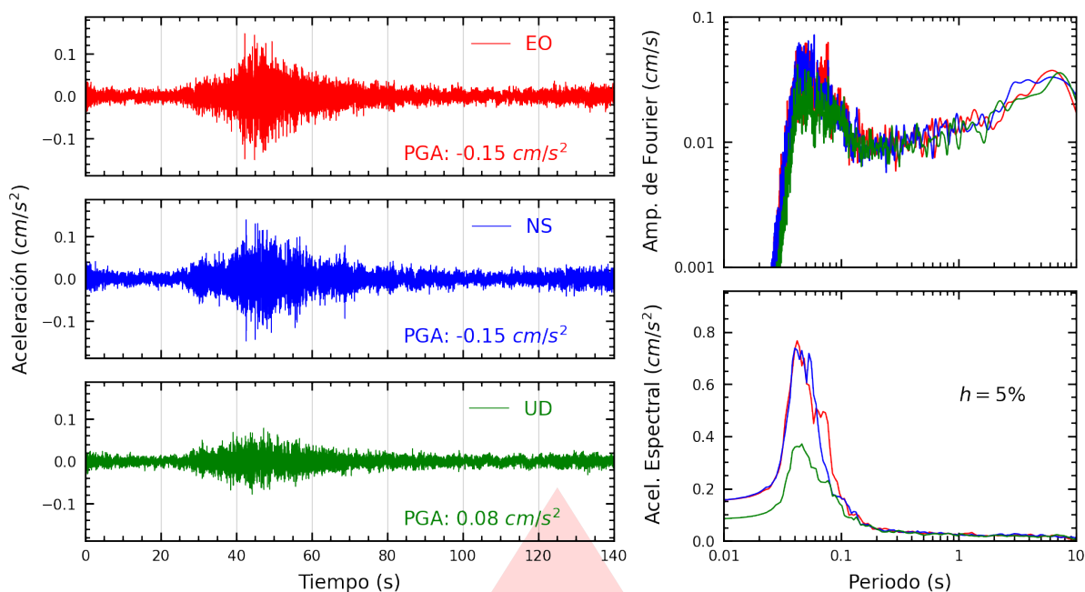
Figura A.15: Registros tiempo-historia, espectros de Fourier y de respuesta en las direcciones EO, NS y vertical de la estación FICPE. Sismo de Mala, Cañete - Lima del 2025-10-15, 23:56:28 (Hora local)
