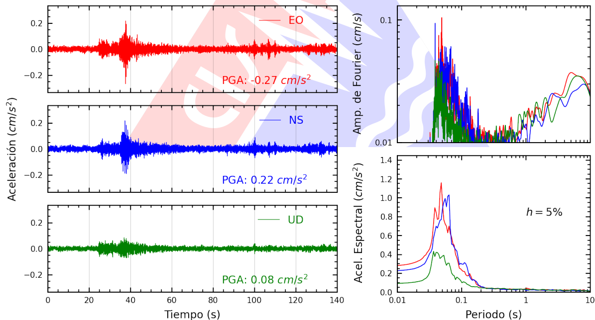
Figura A.8: Registros tiempo-historia, espectros de Fourier y de respuesta en las direcciones EO, NS y vertical de la estación UPCVI. Sismo de Mala, Cañete - Lima del 2025-10-15, 23:56:28 (Hora local)
