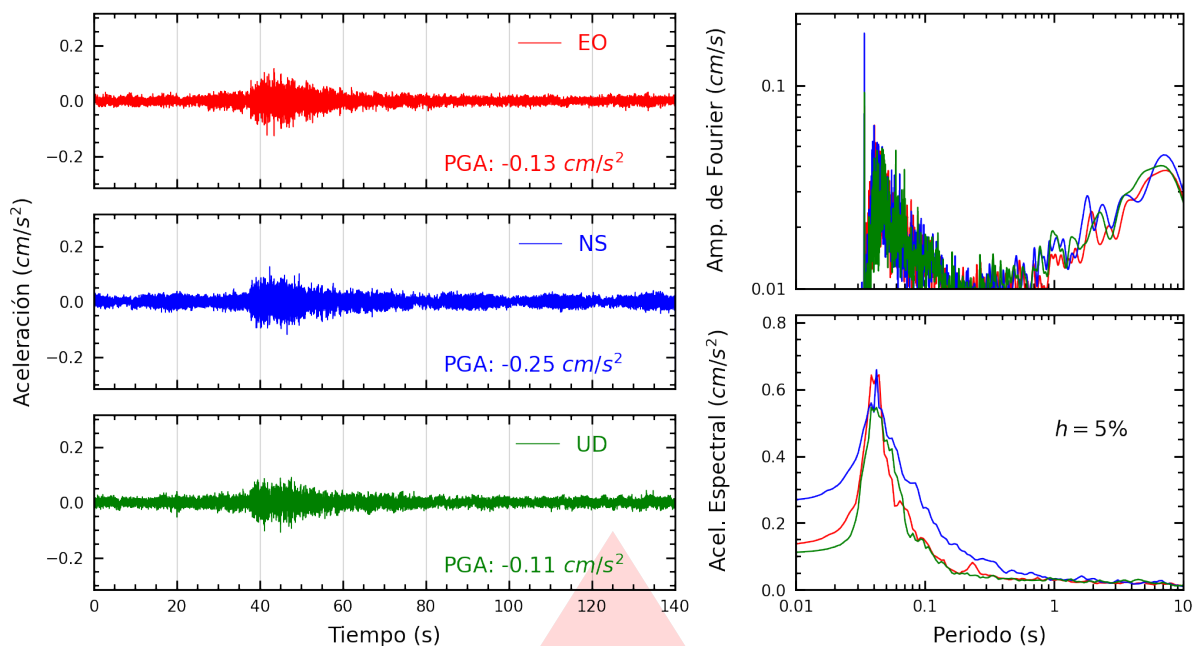
Figura A.9: Registros tiempo-historia, espectros de Fourier y de respuesta en las direcciones EO, NS y vertical de la estación USMP. Sismo de Mala, Cañete - Lima del 2025-10-15, 23:56:28 (Hora local)
