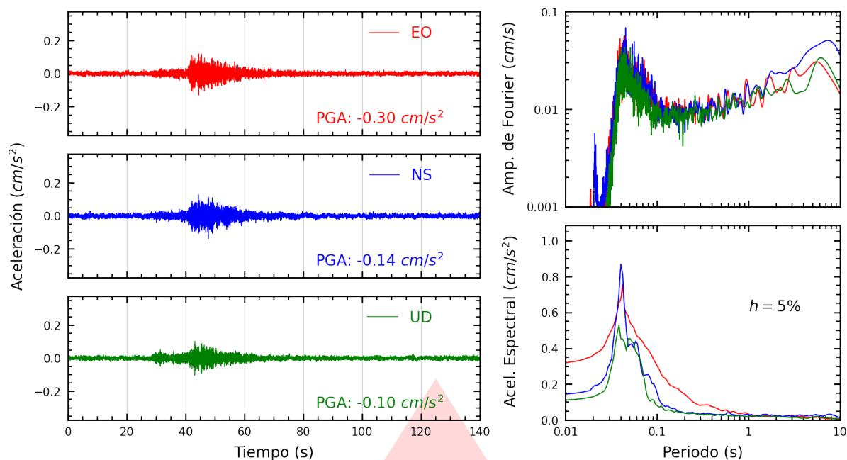
Figura A.5: Registros tiempo-historia, espectros de Fourier y de respuesta en las direcciones EO, NS y vertical de la estación SJLCE. Sismo de Mala, Cañete - Lima del 2025-10-15, 23:56:28 (Hora local)
