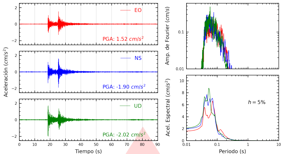
Figura A.1: Registros tiempo-historia, espectros de Fourier y de respuesta en las direcciones EO, NS y vertical de la estación ASIA. Sismo de Mala, Cañete - Lima del 2025-10-15, 23:56:28 (Hora local)
