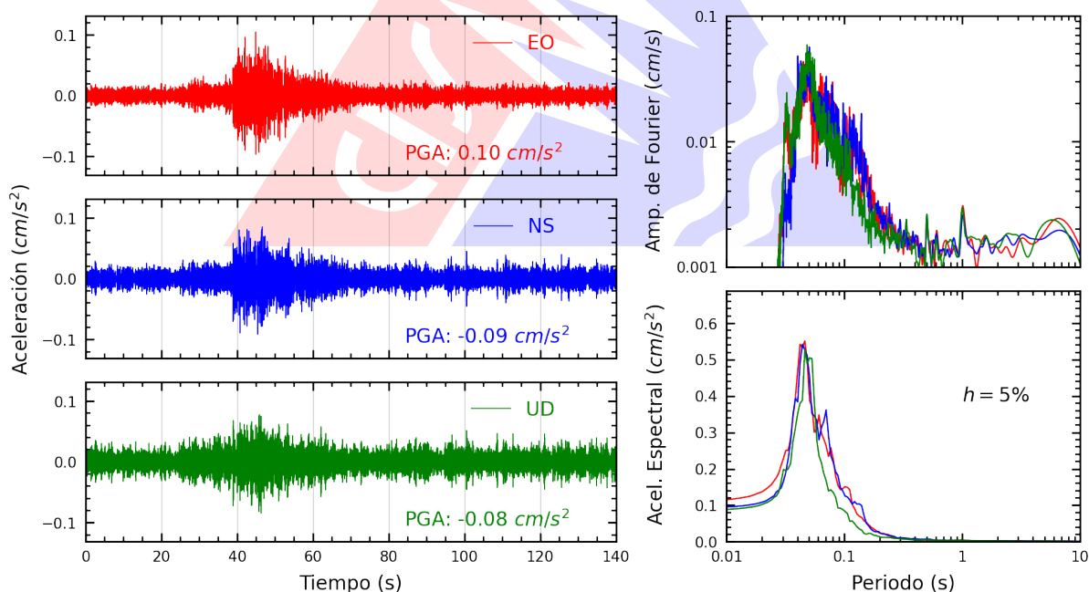
Figura A.18: Registros tiempo-historia, espectros de Fourier y de respuesta en las direcciones EO, NS y vertical de la estación ATARJ. Sismo de Mala, Cañete - Lima del 2025-10-15, 23:56:28 (Hora local)
