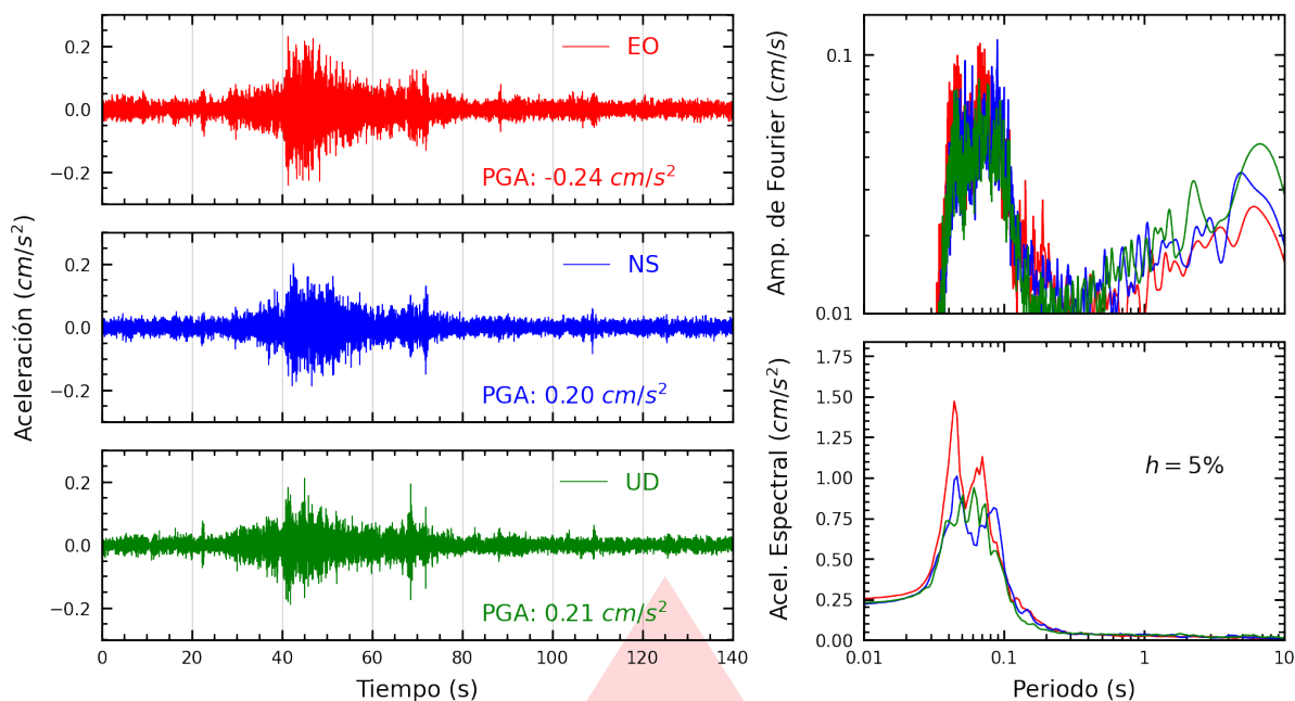
Figura A.11: Registros tiempo-historia, espectros de Fourier y de respuesta en las direcciones EO, NS y vertical de la estación INDEP. Sismo de Mala, Cañete - Lima del 2025-10-15, 23:56:28 (Hora local)
