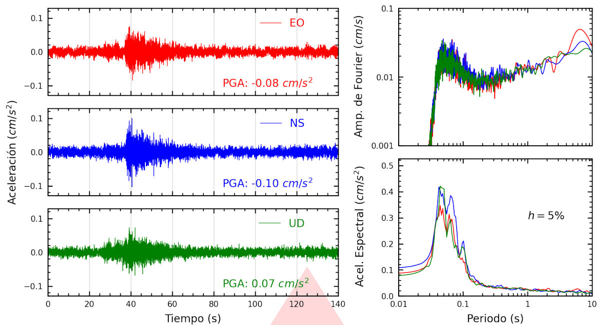
Figura A.19: Registros tiempo-historia, espectros de Fourier y de respuesta en las direcciones EO, NS y vertical de la estación SERVI. Sismo de Mala, Cañete - Lima del 2025-10-15, 23:56:28 (Hora local)
