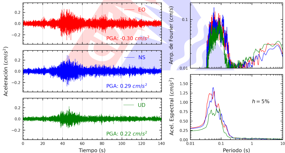
Figura A.6: Registros tiempo-historia, espectros de Fourier y de respuesta en las direcciones EO, NS y vertical de la estación USILM. Sismo de Mala, Cañete - Lima del 2025-10-15, 23:56:28 (Hora local)
