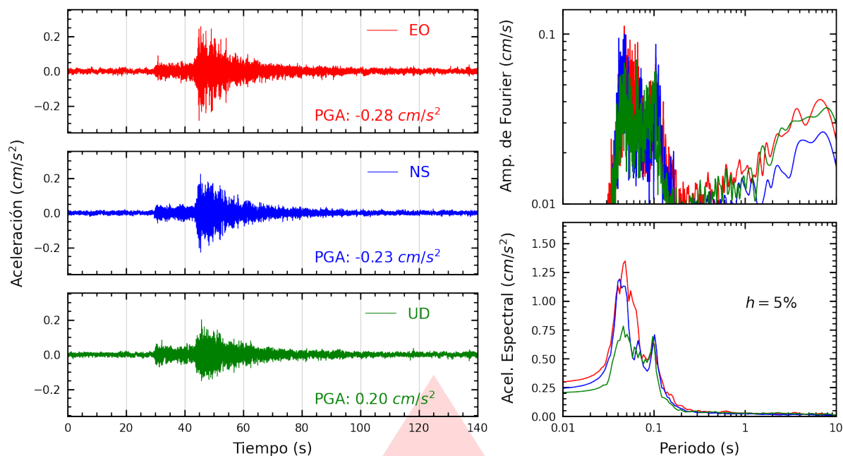
Figura A.7: Registros tiempo-historia, espectros de Fourier y de respuesta en las direcciones EO, NS y vertical de la estación AMORE. Sismo de Mala, Cañete - Lima del 2025-10-15, 23:56:28 (Hora local)
