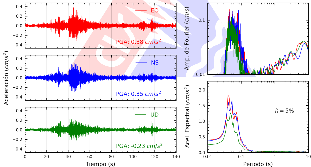
Figura A.4: Registros tiempo-historia, espectros de Fourier y de respuesta en las direcciones EO, NS y vertical de la estación JOSEO. Sismo de Mala, Cañete - Lima del 2025-10-15, 23:56:28 (Hora local)
