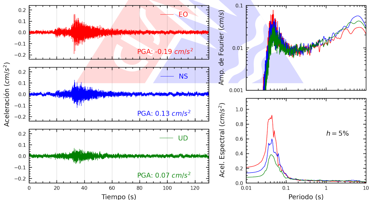
Figura A.12: Registros tiempo-historia, espectros de Fourier y de respuesta en las direcciones EO, NS y vertical de la estación UCSS. Sismo de Mala, Cañete - Lima del 2025-10-15, 23:56:28 (Hora local)
