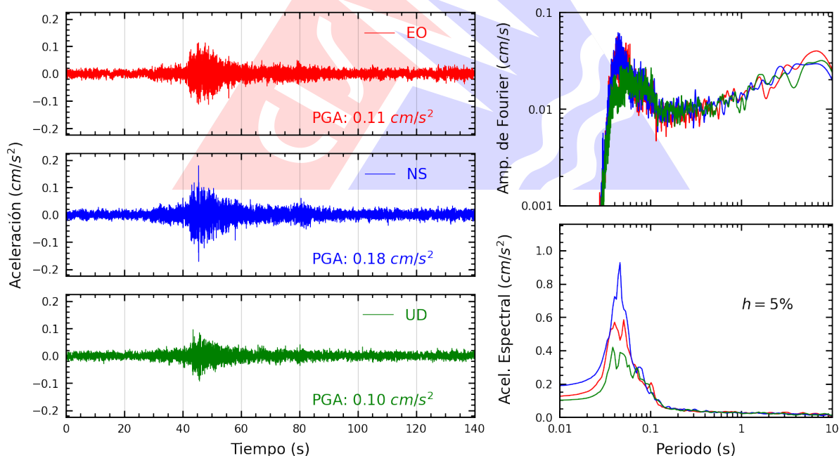
Figura A.14: Registros tiempo-historia, espectros de Fourier y de respuesta en las direcciones EO, NS y vertical de la estación COMAS. Sismo de Mala, Cañete - Lima del 2025-10-15, 23:56:28 (Hora local)
