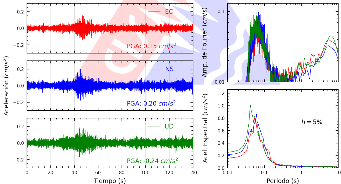
Figura A.10: Registros tiempo-historia, espectros de Fourier y de respuesta en las direcciones EO, NS y vertical de la estación SJLSC. Sismo de Mala, Cañete - Lima del 2025-10-15, 23:56:28 (Hora local)
