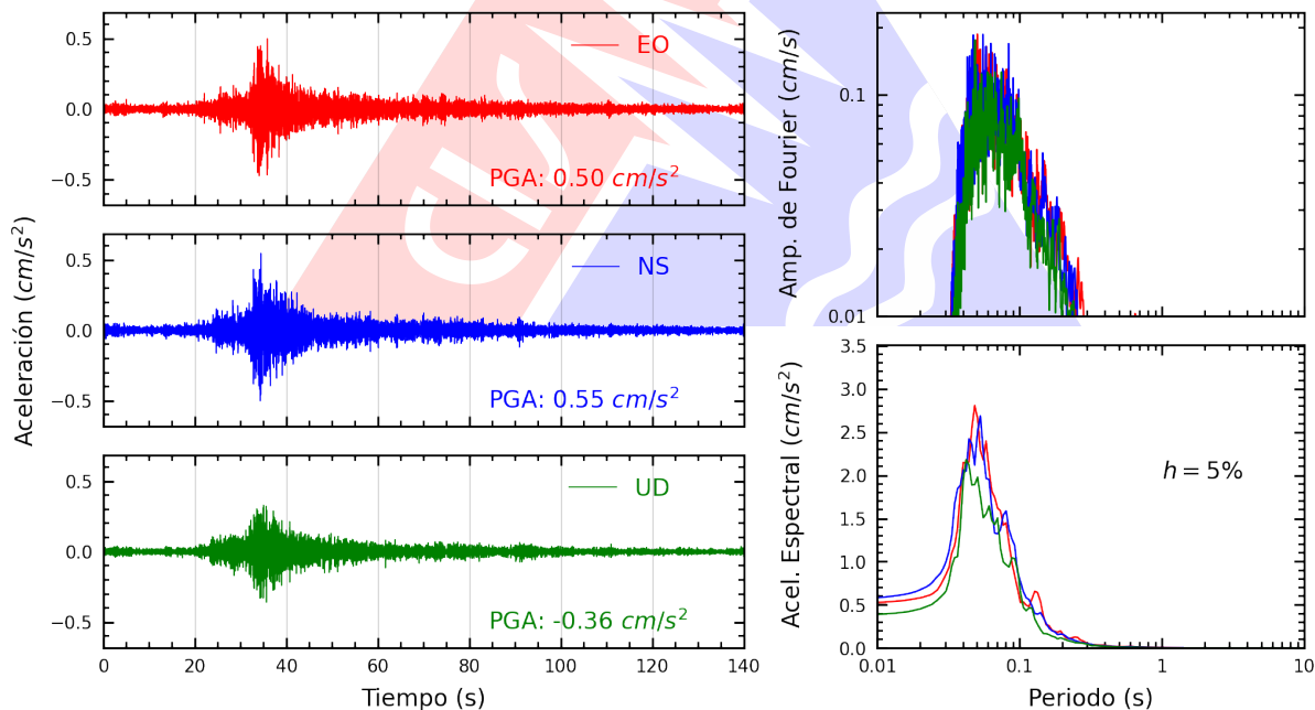
Figura A.2: Registros tiempo-historia, espectros de Fourier y de respuesta en las direcciones EO, NS y vertical de la estación PHERM. Sismo de Mala, Cañete - Lima del 2025-10-15, 23:56:28 (Hora local)
