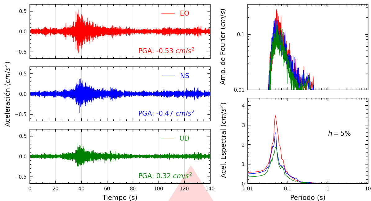
Figura A.3: Registros tiempo-historia, espectros de Fourier y de respuesta en las direcciones EO, NS y vertical de la estación UNTEL. Sismo de Mala, Cañete - Lima del 2025-10-15, 23:56:28 (Hora local)
