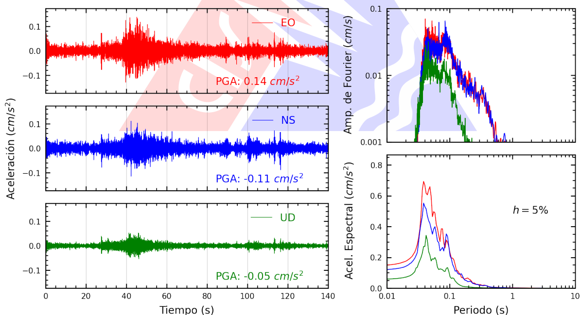
Figura A.16: Registros tiempo-historia, espectros de Fourier y de respuesta en las direcciones EO, NS y vertical de la estación UCVAT. Sismo de Mala, Cañete - Lima del 2025-10-15, 23:56:28 (Hora local)
