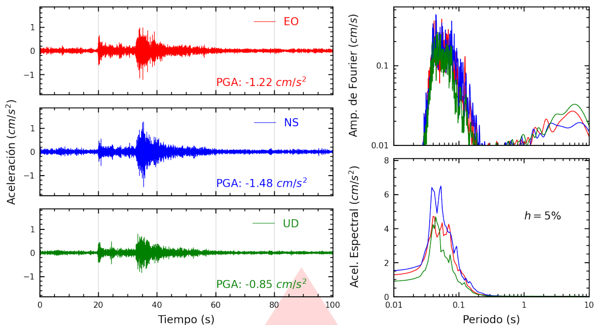
Figura A.1: Registros tiempo-historia, espectros de Fourier y de respuesta en las direcciones EO, NS y vertical de la estación JOSEO. Sismo de Calango, Cañete - Lima del 2025-10-16, 21:07:53 (Hora local)
