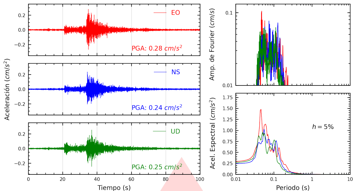
Figura A.25: Registros tiempo-historia, espectros de Fourier y de respuesta en las direcciones EO, NS y vertical de la estación JALV2. Sismo de Calango, Cañete - Lima del 2025-10-16, 21:07:53 (Hora local)
