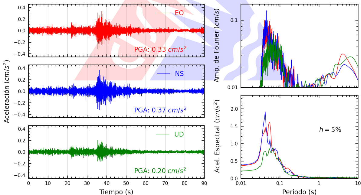
Figura A.20: Registros tiempo-historia, espectros de Fourier y de respuesta en las direcciones EO, NS y vertical de la estación COMAS. Sismo de Calango, Cañete - Lima del 2025-10-16, 21:07:53 (Hora local)
