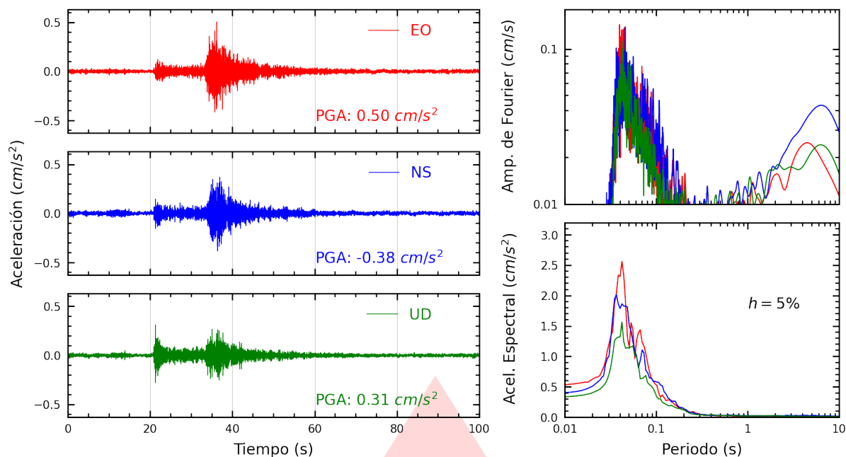
Figura A.13: Registros tiempo-historia, espectros de Fourier y de respuesta en las direcciones EO, NS y vertical de la estación SJLCE. Sismo de Calango, Cañete - Lima del 2025-10-16, 21:07:53 (Hora local)
