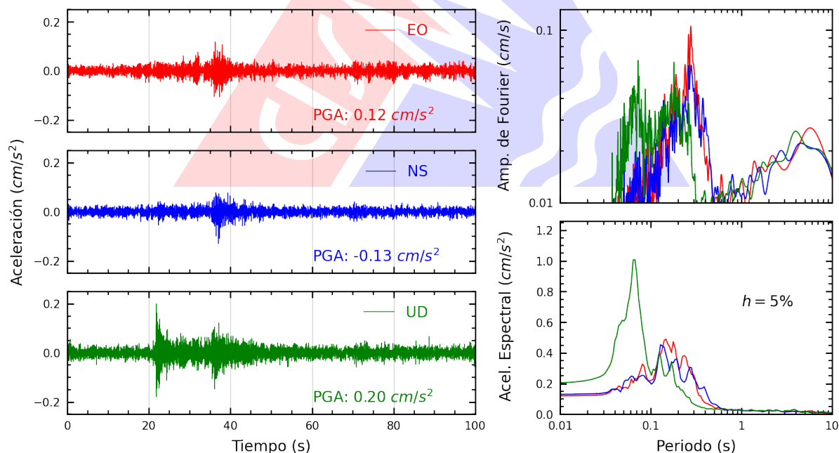
Figura A.26: Registros tiempo-historia, espectros de Fourier y de respuesta en las direcciones EO, NS y vertical de la estación ACAPU. Sismo de Calango, Cañete - Lima del 2025-10-16, 21:07:53 (Hora local)
