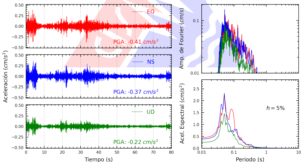
Figura A.16: Registros tiempo-historia, espectros de Fourier y de respuesta en las direcciones EO, NS y vertical de la estación BRIS2. Sismo de Calango, Cañete - Lima del 2025-10-16, 21:07:53 (Hora local)
