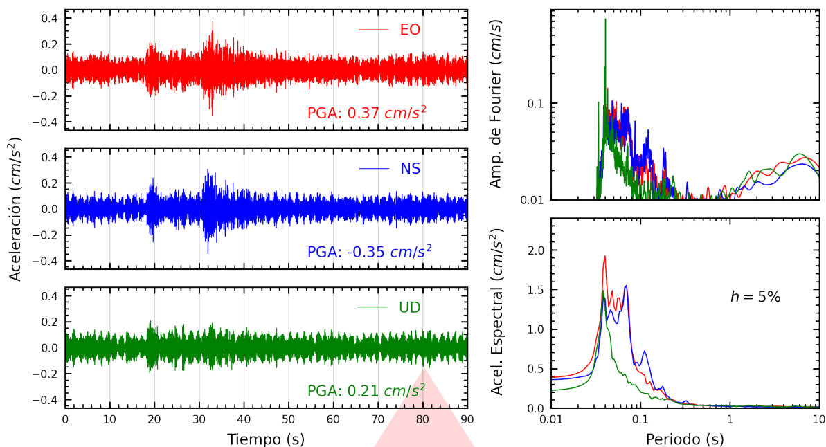
Figura A.19: Registros tiempo-historia, espectros de Fourier y de respuesta en las direcciones EO, NS y vertical de la estación UPCVI. Sismo de Calango, Cañete - Lima del 2025-10-16, 21:07:53 (Hora local)
