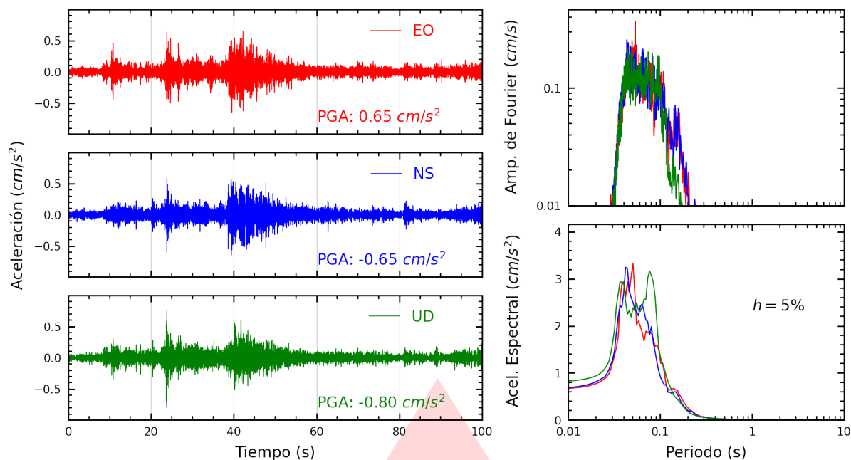
Figura A.7: Registros tiempo-historia, espectros de Fourier y de respuesta en las direcciones EO, NS y vertical de la estación SROSA. Sismo de Calango, Cañete - Lima del 2025-10-16, 21:07:53 (Hora local)
