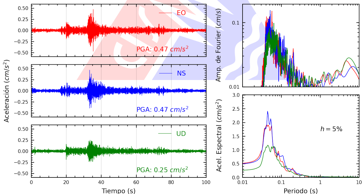
Figura A.14: Registros tiempo-historia, espectros de Fourier y de respuesta en las direcciones EO, NS y vertical de la estación IMCA. Sismo de Calango, Cañete - Lima del 2025-10-16, 21:07:53 (Hora local)
