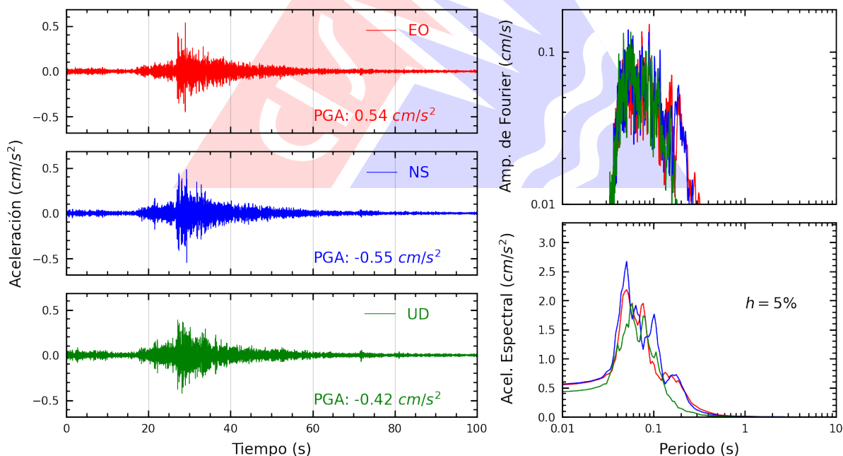
Figura A.12: Registros tiempo-historia, espectros de Fourier y de respuesta en las direcciones EO, NS y vertical de la estación ASIA. Sismo de Calango, Cañete - Lima del 2025-10-16, 21:07:53 (Hora local)
