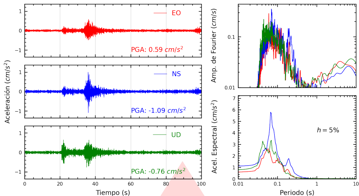
Figura A.5: Registros tiempo-historia, espectros de Fourier y de respuesta en las direcciones EO, NS y vertical de la estación SJLSC. Sismo de Calango, Cañete - Lima del 2025-10-16, 21:07:53 (Hora local)
