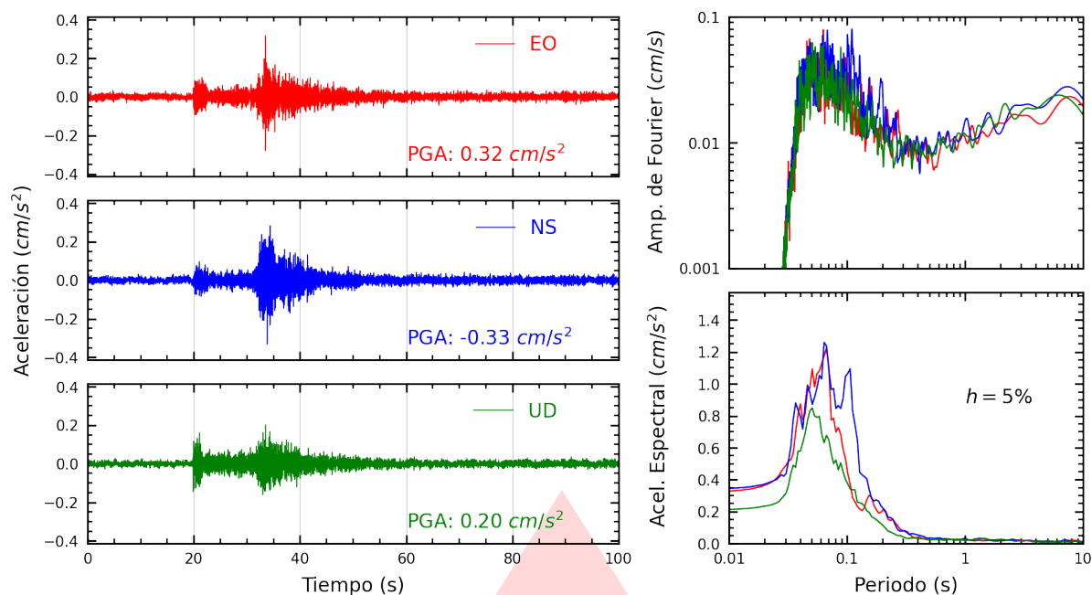
Figura A.23: Registros tiempo-historia, espectros de Fourier y de respuesta en las direcciones EO, NS y vertical de la estación SERVI. Sismo de Calango, Cañete - Lima del 2025-10-16, 21:07:53 (Hora local)
