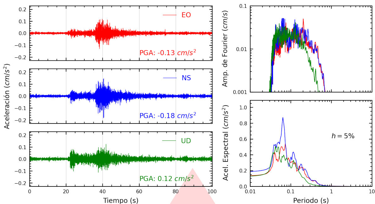
Figura A.27: Registros tiempo-historia, espectros de Fourier y de respuesta en las direcciones EO, NS y vertical de la estación VHAYA. Sismo de Calango, Cañete - Lima del 2025-10-16, 21:07:53 (Hora local)
