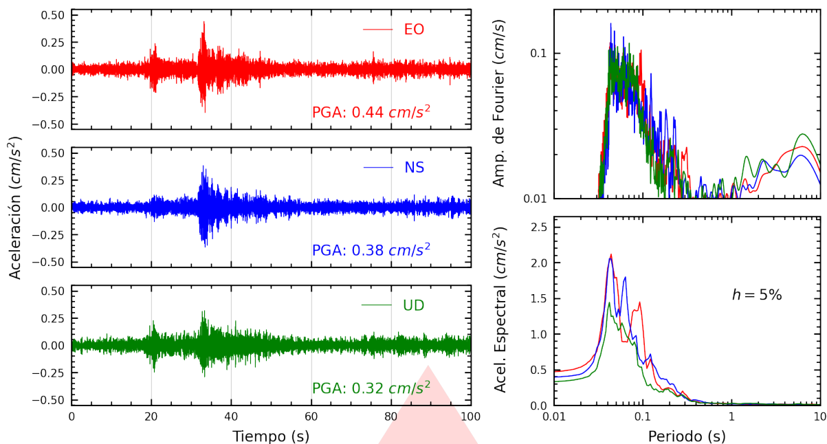
Figura A.15: Registros tiempo-historia, espectros de Fourier y de respuesta en las direcciones EO, NS y vertical de la estación URPE. Sismo de Calango, Cañete - Lima del 2025-10-16, 21:07:53 (Hora local)
