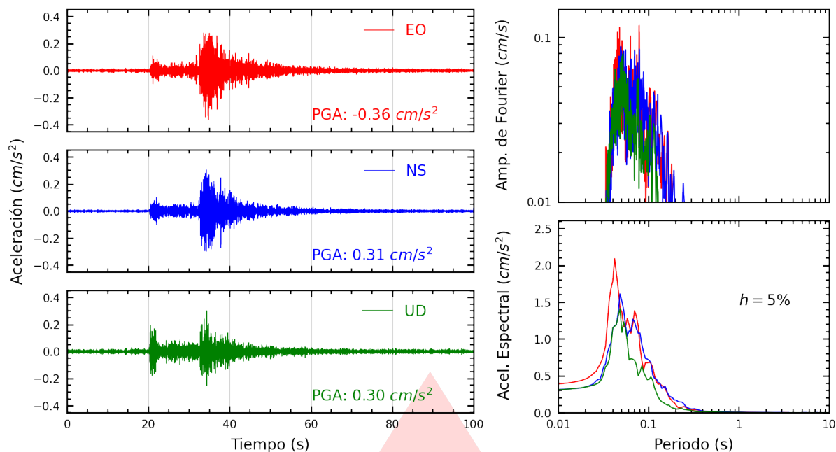
Figura A.21: Registros tiempo-historia, espectros de Fourier y de respuesta en las direcciones EO, NS y vertical de la estación ATARJ. Sismo de Calango, Cañete - Lima del 2025-10-16, 21:07:53 (Hora local)
