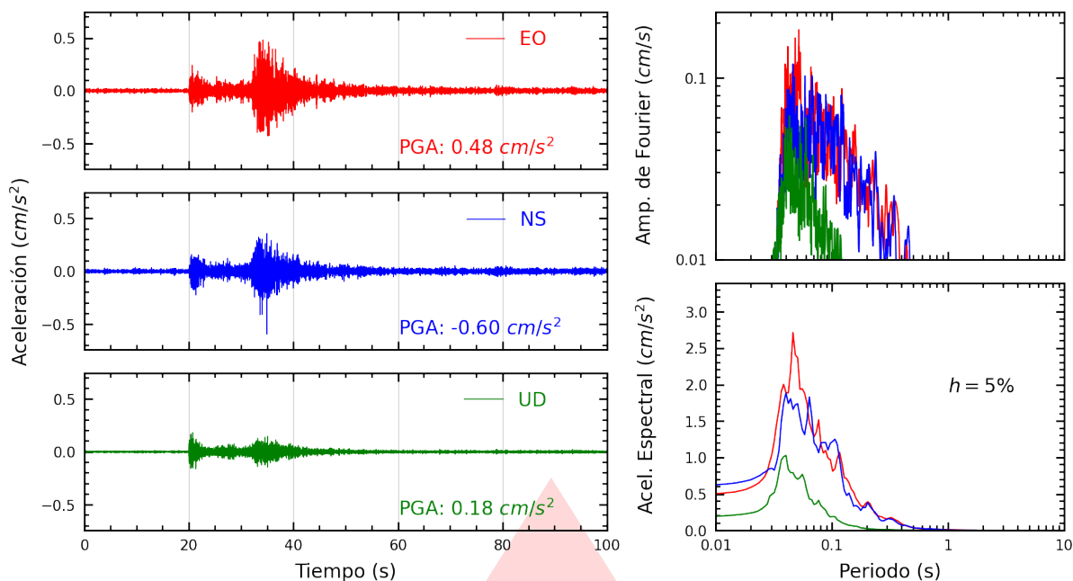
Figura A.11: Registros tiempo-historia, espectros de Fourier y de respuesta en las direcciones EO, NS y vertical de la estación UCVAT. Sismo de Calango, Cañete - Lima del 2025-10-16, 21:07:53 (Hora local)
