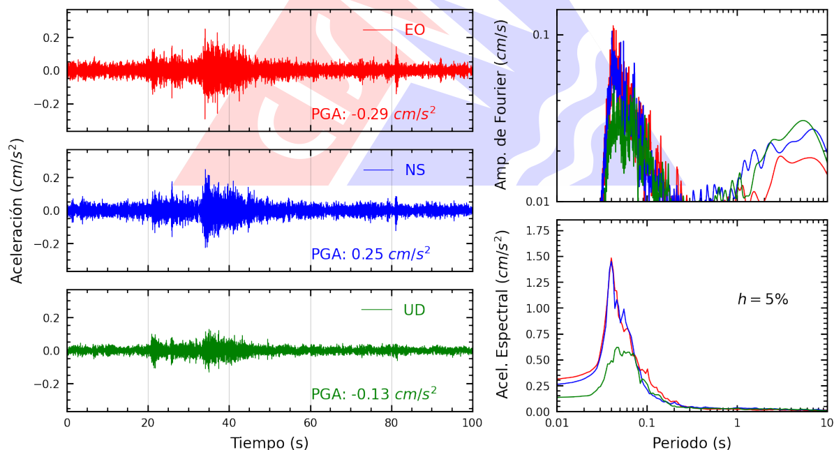
Figura A.24: Registros tiempo-historia, espectros de Fourier y de respuesta en las direcciones EO, NS y vertical de la estación CEPRE. Sismo de Calango, Cañete - Lima del 2025-10-16, 21:07:53 (Hora local)
