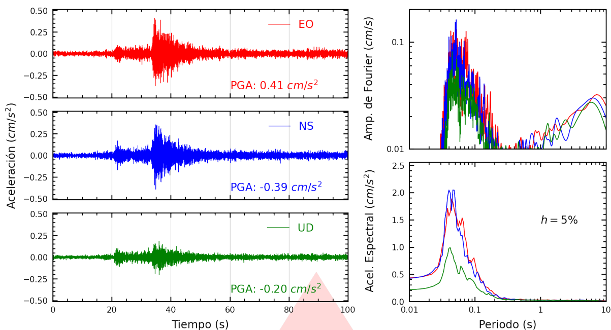
Figura A.17: Registros tiempo-historia, espectros de Fourier y de respuesta en las direcciones EO, NS y vertical de la estación FICPE. Sismo de Calango, Cañete - Lima del 2025-10-16, 21:07:53 (Hora local)
