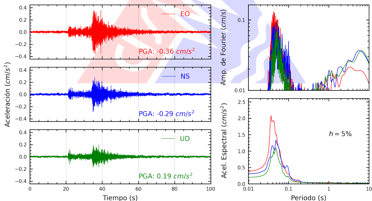
Figura A.22: Registros tiempo-historia, espectros de Fourier y de respuesta en las direcciones EO, NS y vertical de la estación UCSS. Sismo de Calango, Cañete - Lima del 2025-10-16, 21:07:53 (Hora local)
