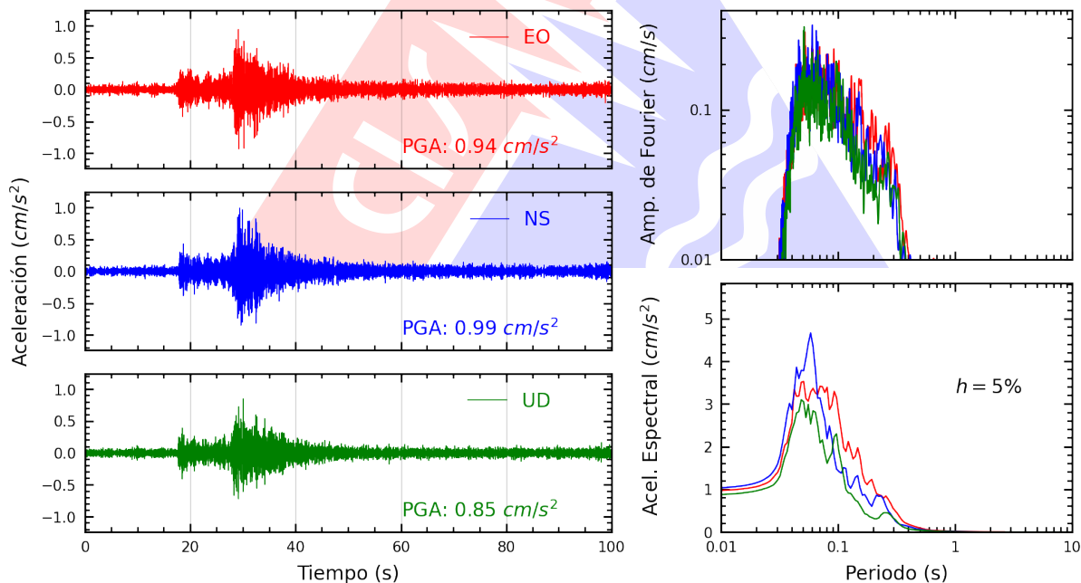
Figura A.6: Registros tiempo-historia, espectros de Fourier y de respuesta en las direcciones EO, NS y vertical de la estación PHERM. Sismo de Calango, Cañete - Lima del 2025-10-16, 21:07:53 (Hora local)
