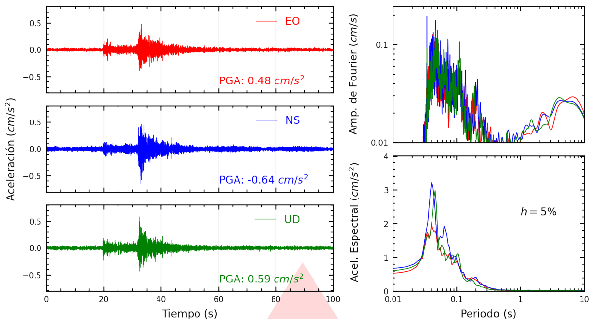
Figura A.9: Registros tiempo-historia, espectros de Fourier y de respuesta en las direcciones EO, NS y vertical de la estación USMP. Sismo de Calango, Cañete - Lima del 2025-10-16, 21:07:53 (Hora local)
