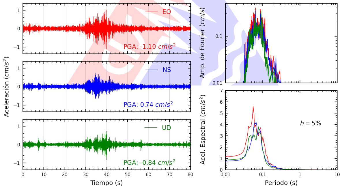
Figura A.4: Registros tiempo-historia, espectros de Fourier y de respuesta en las direcciones EO, NS y vertical de la estación SOBAR. Sismo de Calango, Cañete - Lima del 2025-10-16, 21:07:53 (Hora local)
