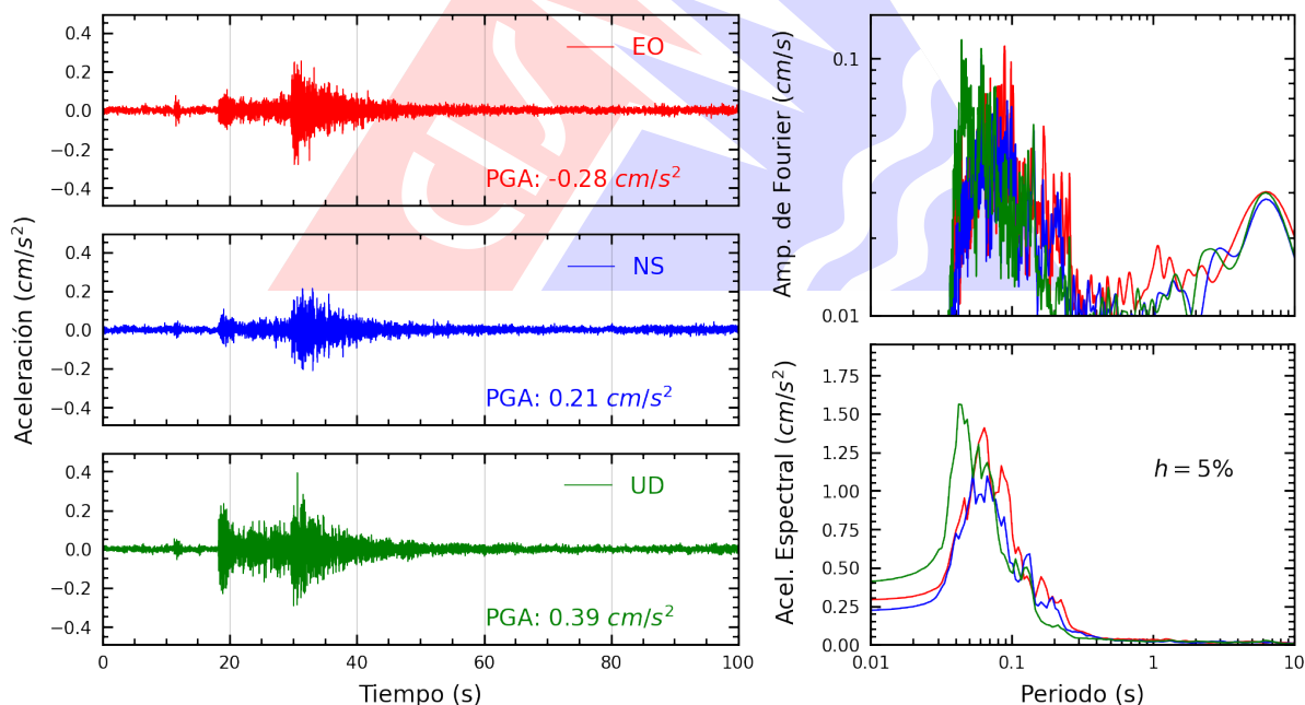
Figura A.18: Registros tiempo-historia, espectros de Fourier y de respuesta en las direcciones EO, NS y vertical de la estación USILP. Sismo de Calango, Cañete - Lima del 2025-10-16, 21:07:53 (Hora local)
