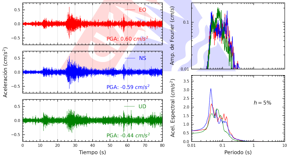
Figura A.10: Registros tiempo-historia, espectros de Fourier y de respuesta en las direcciones EO, NS y vertical de la estación CARAB. Sismo de Calango, Cañete - Lima del 2025-10-16, 21:07:53 (Hora local)
