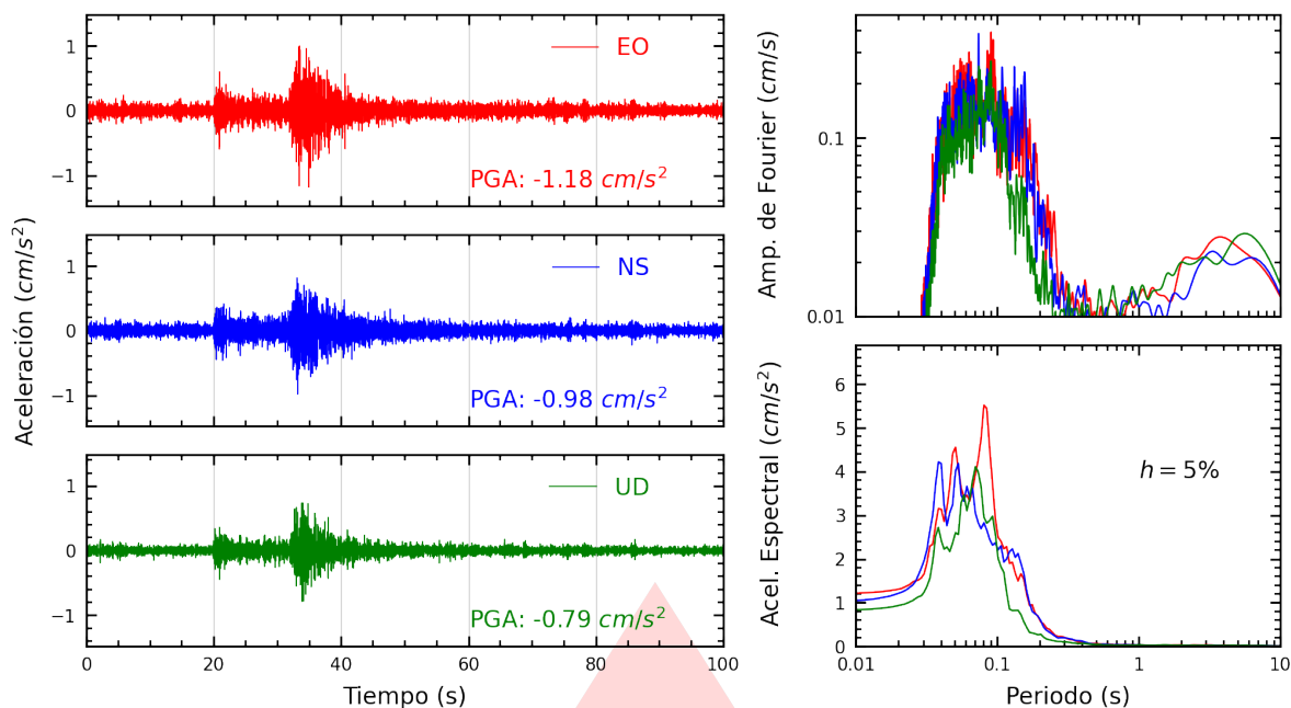
Figura A.3: Registros tiempo-historia, espectros de Fourier y de respuesta en las direcciones EO, NS y vertical de la estación USILM. Sismo de Calango, Cañete - Lima del 2025-10-16, 21:07:53 (Hora local)
