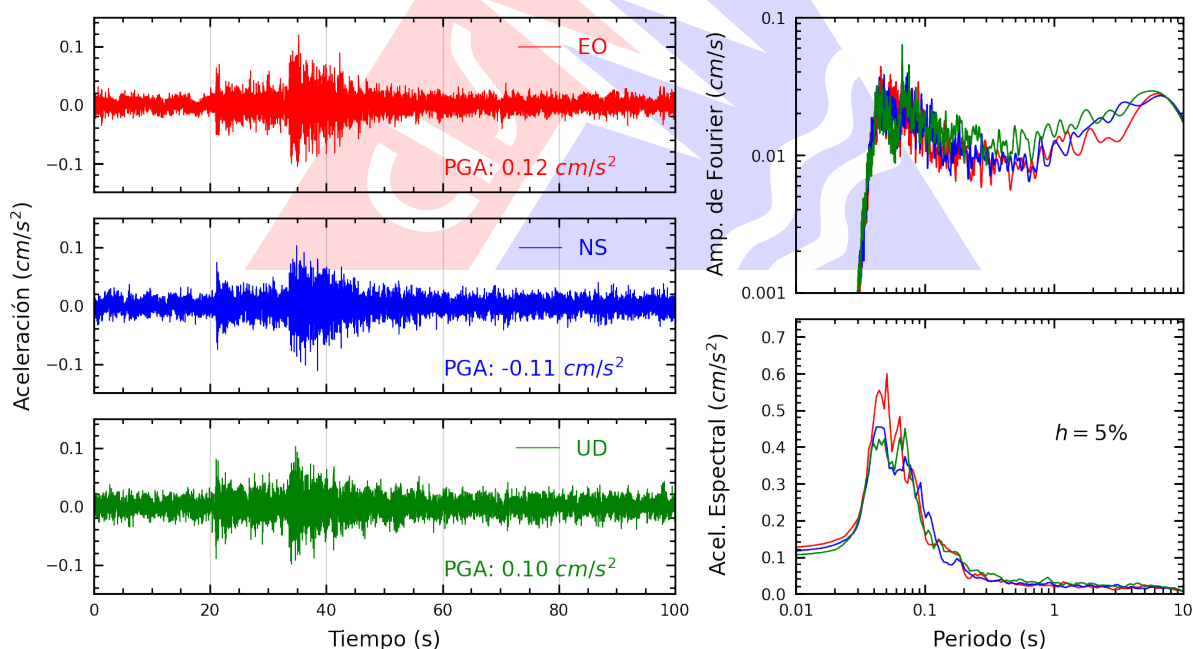
Figura A.28: Registros tiempo-historia, espectros de Fourier y de respuesta en las direcciones EO, NS y vertical de la estación UNFV. Sismo de Calango, Cañete - Lima del 2025-10-16, 21:07:53 (Hora local)
