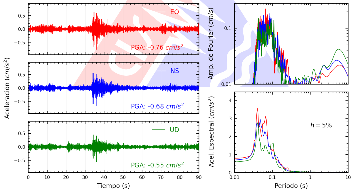
Figura A.8: Registros tiempo-historia, espectros de Fourier y de respuesta en las direcciones EO, NS y vertical de la estación INDEP. Sismo de Calango, Cañete - Lima del 2025-10-16, 21:07:53 (Hora local)
