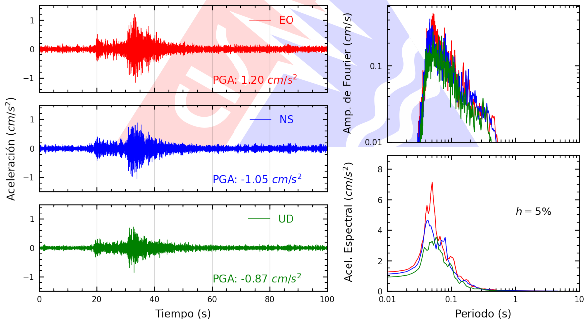
Figura A.2: Registros tiempo-historia, espectros de Fourier y de respuesta en las direcciones EO, NS y vertical de la estación UNTEL. Sismo de Calango, Cañete - Lima del 2025-10-16, 21:07:53 (Hora local)
