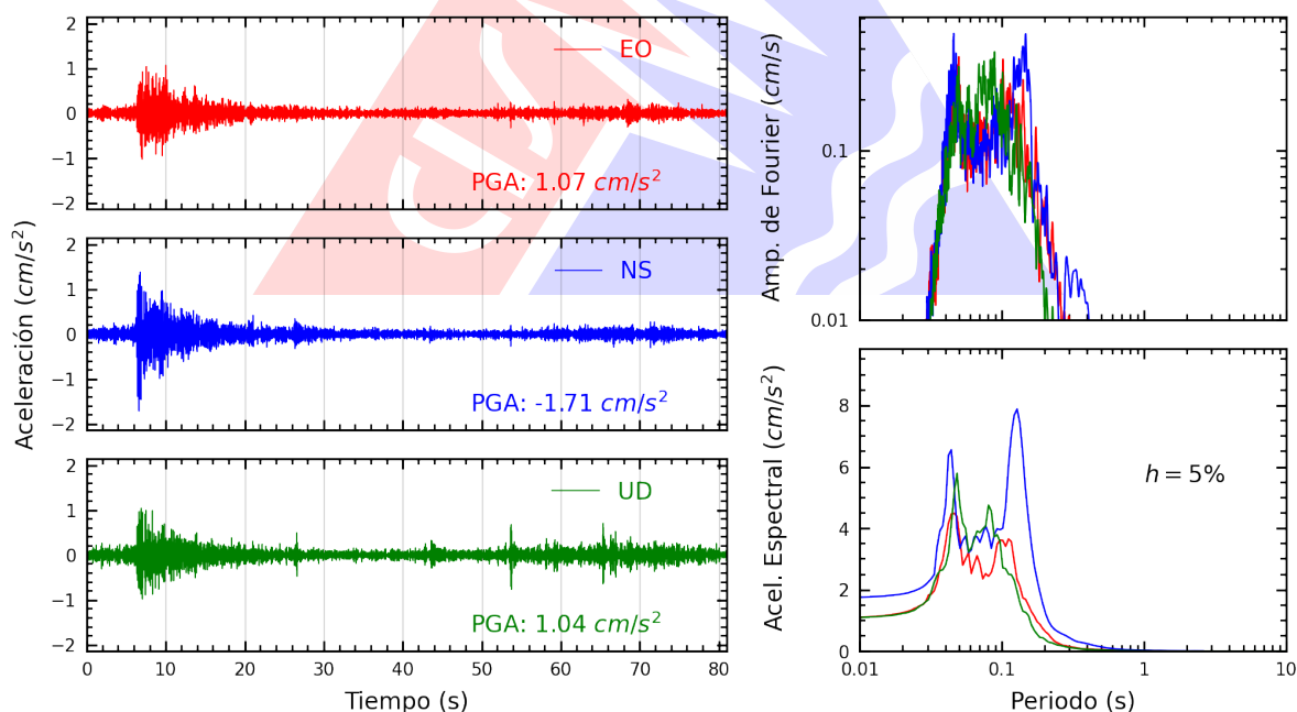
Figura A.22: Registros tiempo-historia, espectros de Fourier y de respuesta en las direcciones EO, NS y vertical de la estación CARAB. Sismo de Chilca, Cañete - Lima del 2025-10-20, 20:23:44 (Hora local)
