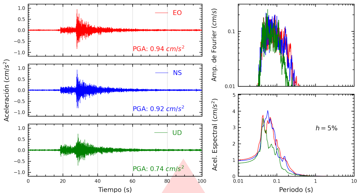
Figura A.29: Registros tiempo-historia, espectros de Fourier y de respuesta en las direcciones EO, NS y vertical de la estación ASIA. Sismo de Chilca, Cañete - Lima del 2025-10-20, 20:23:44 (Hora local)
