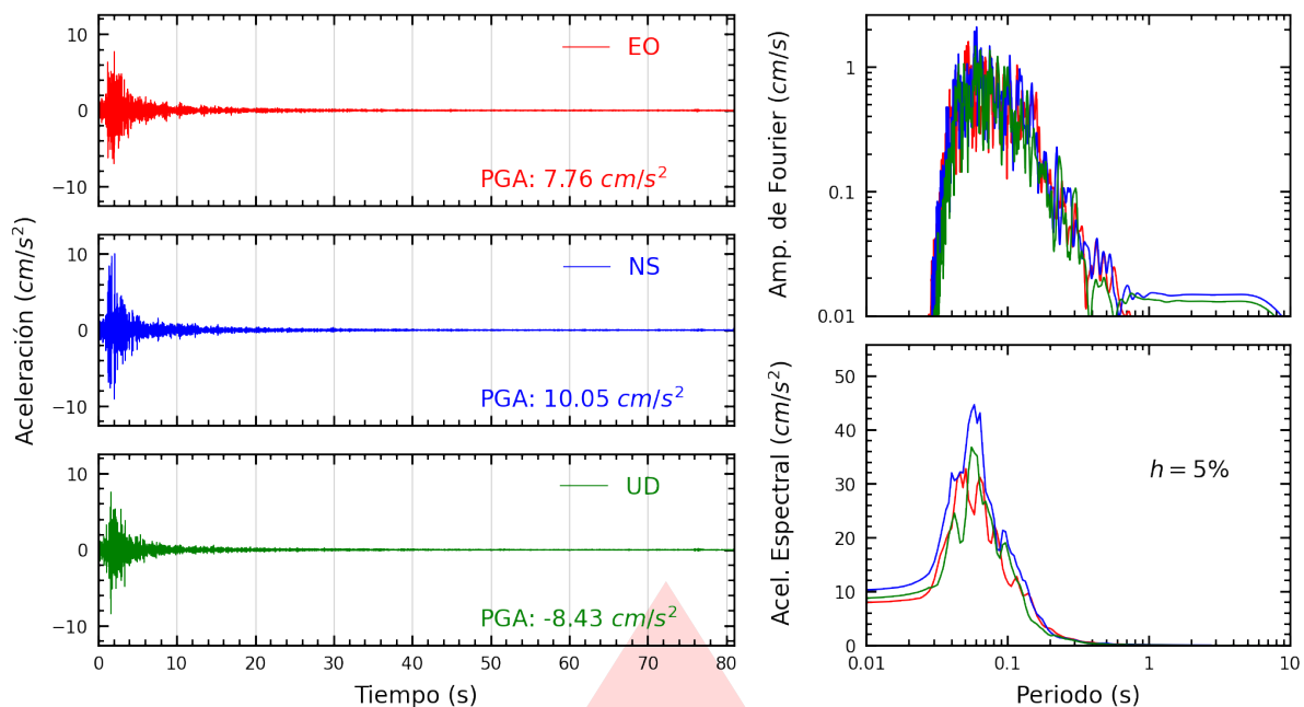
Figura A.1: Registros tiempo-historia, espectros de Fourier y de respuesta en las direcciones EO, NS y vertical de la estación PHERM. Sismo de Chilca, Cañete - Lima del 2025-10-20, 20:23:44 (Hora local)
