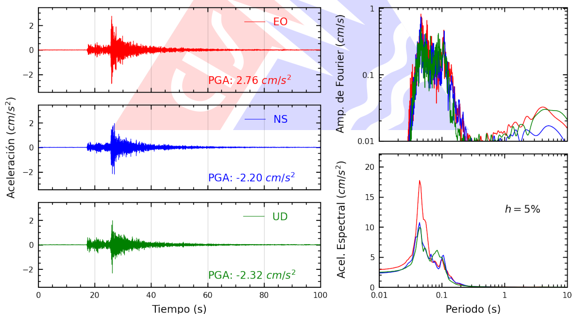
Figura A.12: Registros tiempo-historia, espectros de Fourier y de respuesta en las direcciones EO, NS y vertical de la estación AMORE. Sismo de Chilca, Cañete - Lima del 2025-10-20, 20:23:44 (Hora local)
