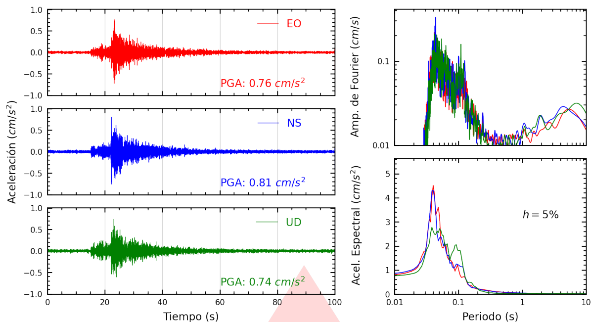
Figura A.33: Registros tiempo-historia, espectros de Fourier y de respuesta en las direcciones EO, NS y vertical de la estación USMP. Sismo de Chilca, Cañete - Lima del 2025-10-20, 20:23:44 (Hora local)
