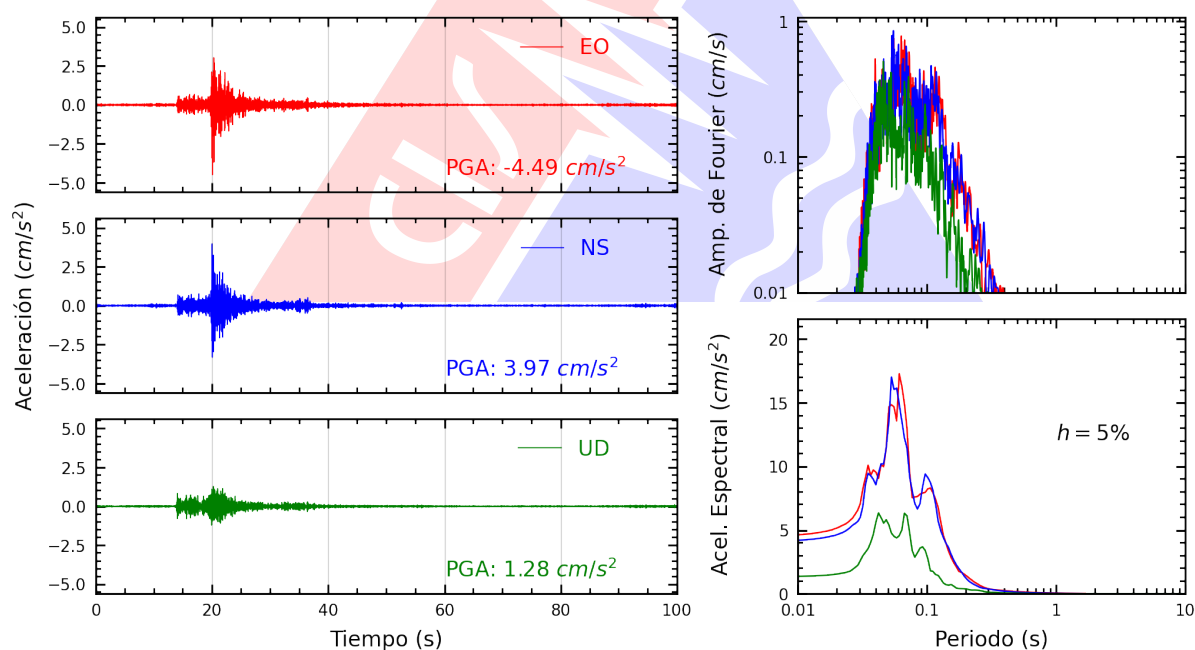
Figura A.4: Registros tiempo-historia, espectros de Fourier y de respuesta en las direcciones EO, NS y vertical de la estación PACHA. Sismo de Chilca, Cañete - Lima del 2025-10-20, 20:23:44 (Hora local)
