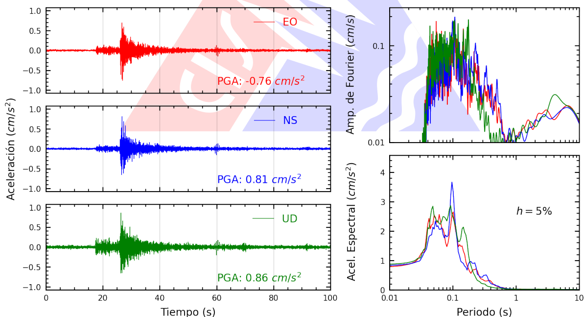
Figura A.32: Registros tiempo-historia, espectros de Fourier y de respuesta en las direcciones EO, NS y vertical de la estación MDPP. Sismo de Chilca, Cañete - Lima del 2025-10-20, 20:23:44 (Hora local)
