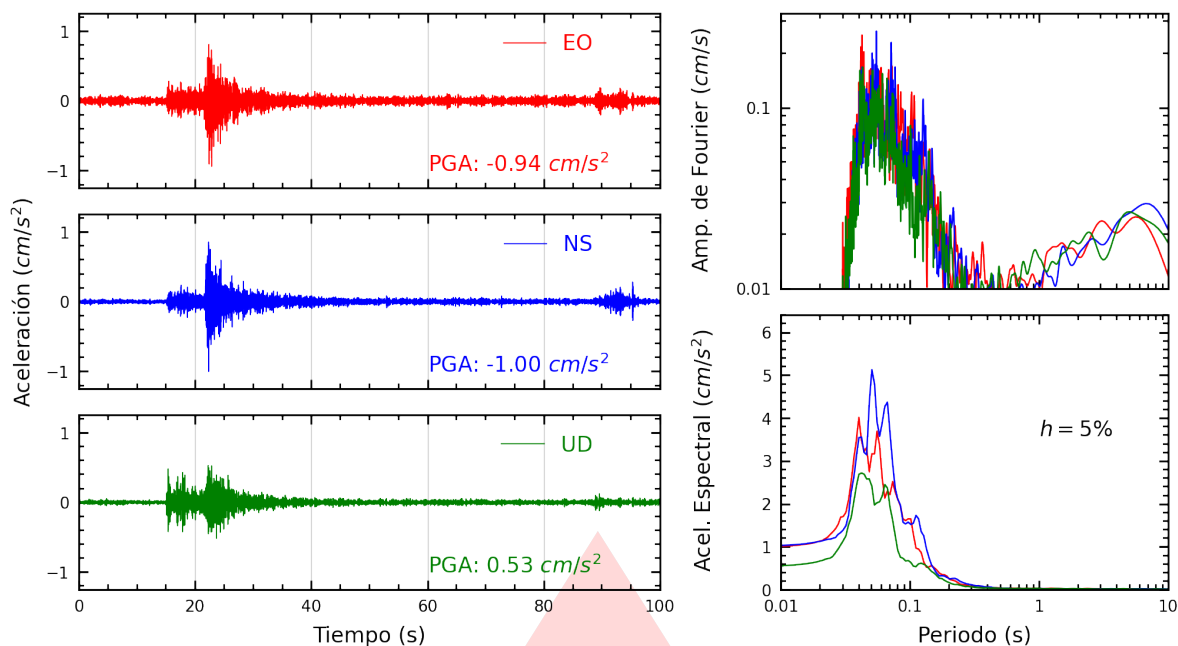
Figura A.27: Registros tiempo-historia, espectros de Fourier y de respuesta en las direcciones EO, NS y vertical de la estación INICT. Sismo de Chilca, Cañete - Lima del 2025-10-20, 20:23:44 (Hora local)
