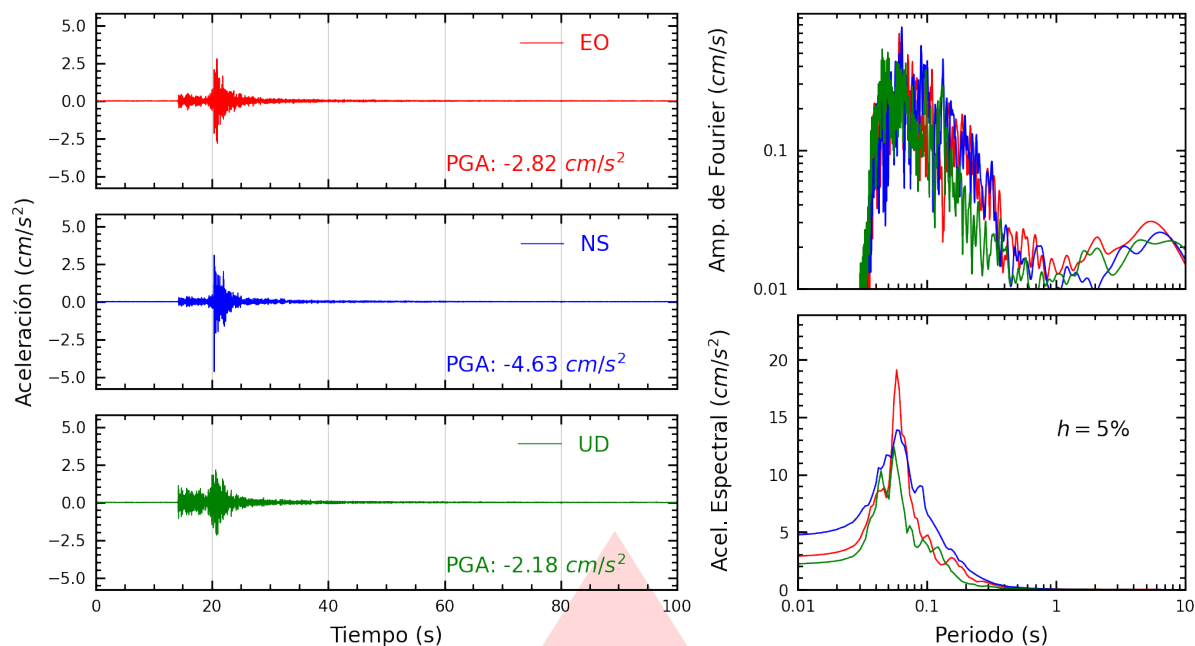
Figura A.3: Registros tiempo-historia, espectros de Fourier y de respuesta en las direcciones EO, NS y vertical de la estación USILP. Sismo de Chilca, Cañete - Lima del 2025-10-20, 20:23:44 (Hora local)
