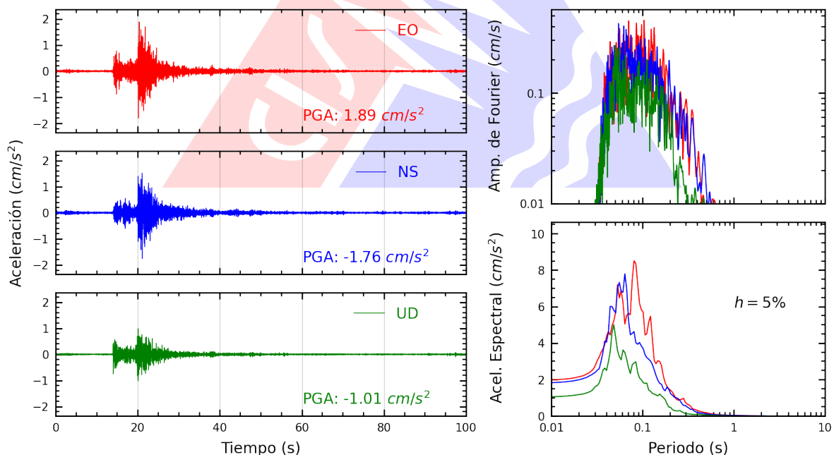
Figura A.18: Registros tiempo-historia, espectros de Fourier y de respuesta en las direcciones EO, NS y vertical de la estación BRISA. Sismo de Chilca, Cañete - Lima del 2025-10-20, 20:23:44 (Hora local)
