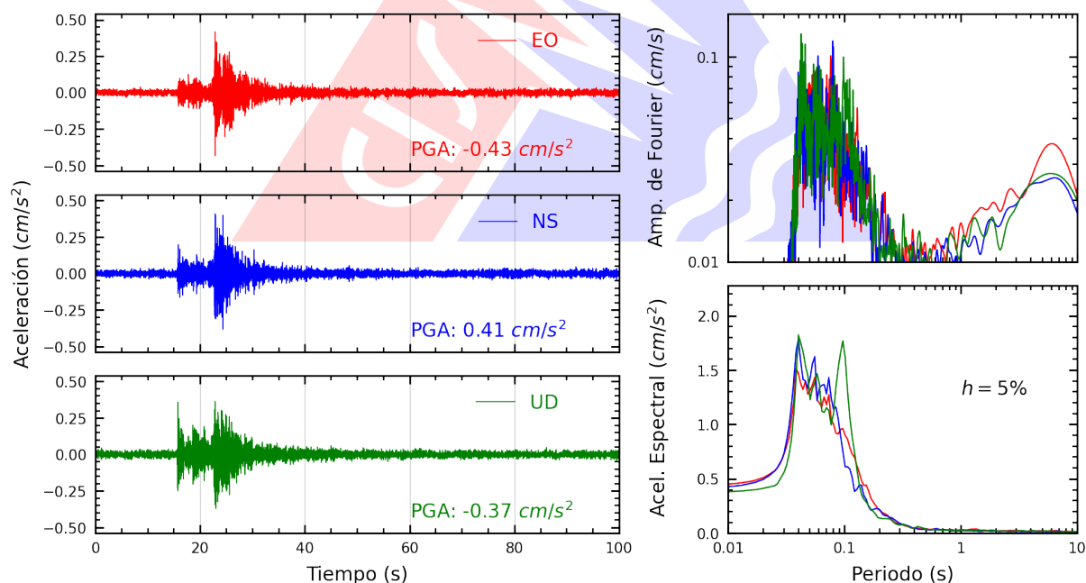
Figura A.40: Registros tiempo-historia, espectros de Fourier y de respuesta en las direcciones EO, NS y vertical de la estación BONDY. Sismo de Chilca, Cañete - Lima del 2025-10-20, 20:23:44 (Hora local)
