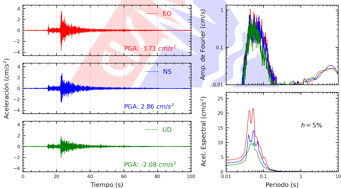
Figura A.6: Registros tiempo-historia, espectros de Fourier y de respuesta en las direcciones EO, NS y vertical de la estación JOSEO. Sismo de Chilca, Cañete - Lima del 2025-10-20, 20:23:44 (Hora local)
