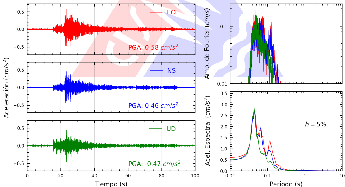
Figura A.38: Registros tiempo-historia, espectros de Fourier y de respuesta en las direcciones EO, NS y vertical de la estación ATARJ. Sismo de Chilca, Cañete - Lima del 2025-10-20, 20:23:44 (Hora local)
