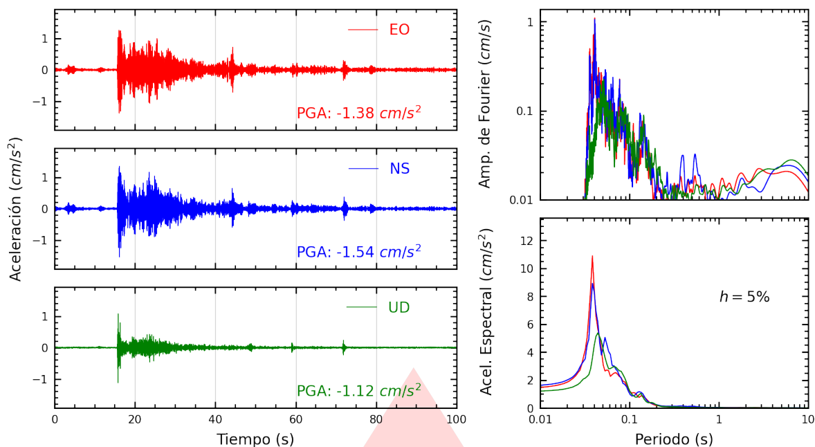
Figura A.23: Registros tiempo-historia, espectros de Fourier y de respuesta en las direcciones EO, NS y vertical de la estación DHNPE. Sismo de Chilca, Cañete - Lima del 2025-10-20, 20:23:44 (Hora local)
