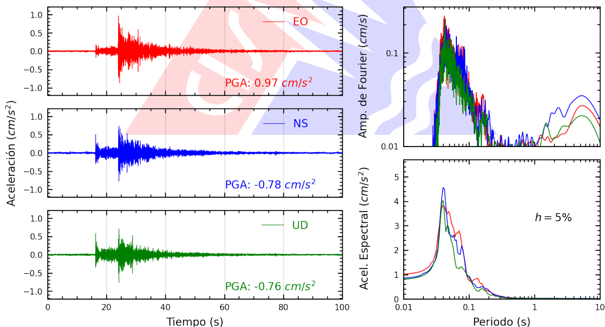
Figura A.28: Registros tiempo-historia, espectros de Fourier y de respuesta en las direcciones EO, NS y vertical de la estación SJLCE. Sismo de Chilca, Cañete - Lima del 2025-10-20, 20:23:44 (Hora local)
