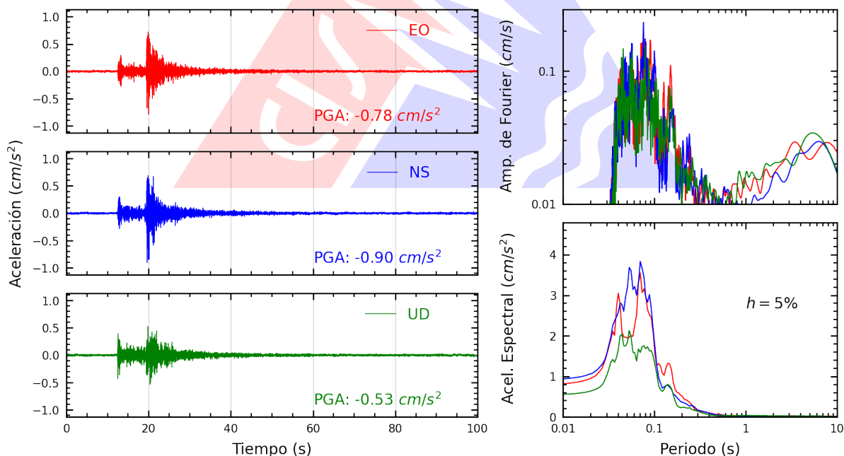
Figura A.30: Registros tiempo-historia, espectros de Fourier y de respuesta en las direcciones EO, NS y vertical de la estación UNMSM. Sismo de Chilca, Cañete - Lima del 2025-10-20, 20:23:44 (Hora local)
