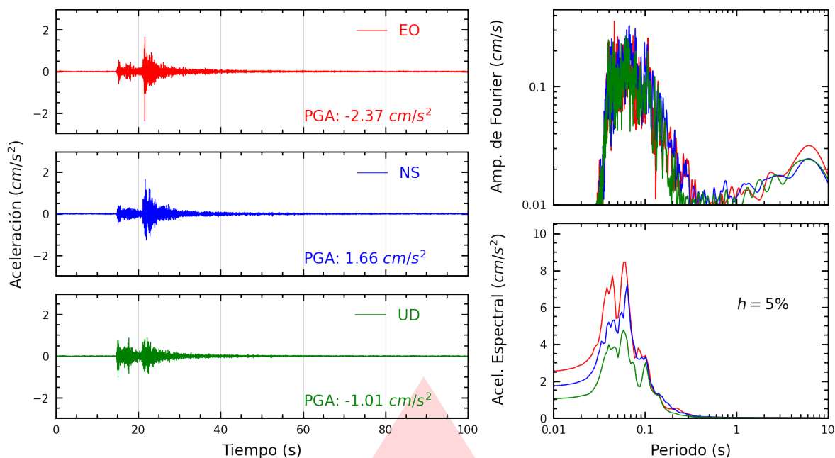
Figura A.13: Registros tiempo-historia, espectros de Fourier y de respuesta en las direcciones EO, NS y vertical de la estación SERVI. Sismo de Chilca, Cañete - Lima del 2025-10-20, 20:23:44 (Hora local)
