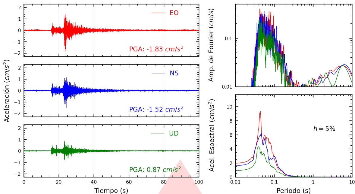
Figura A.19: Registros tiempo-historia, espectros de Fourier y de respuesta en las direcciones EO, NS y vertical de la estación FICPE. Sismo de Chilca, Cañete - Lima del 2025-10-20, 20:23:44 (Hora local)
