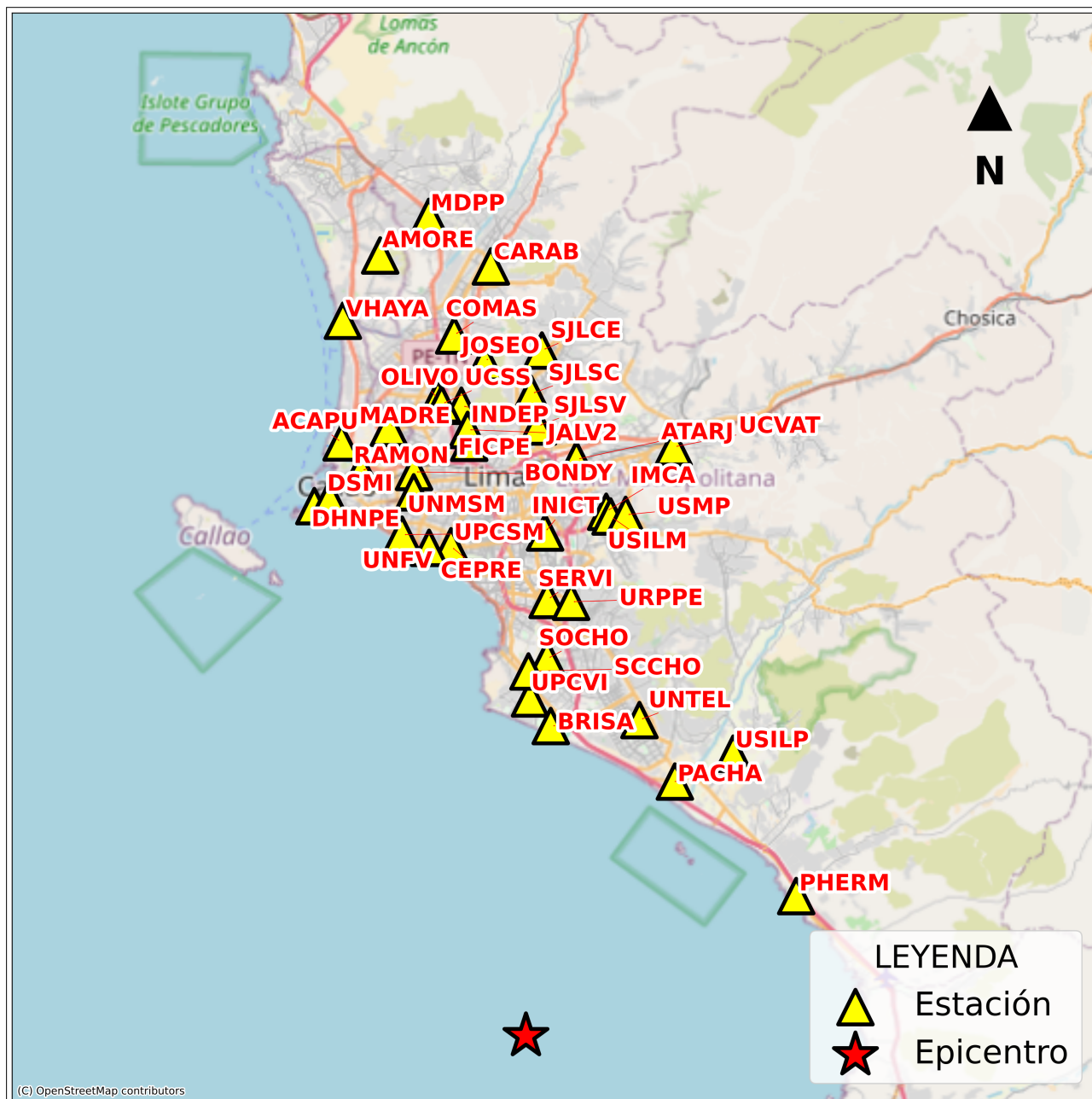
Figura 3: Mapa de ubicación de la(s) estación(es) acelerográfica(s) en Lima Metropolitana correspondiente(s) al Sismo de Chilca, Cañete - Lima del 20 de octubre de 2025 a las 20:23:44 (hora local)
