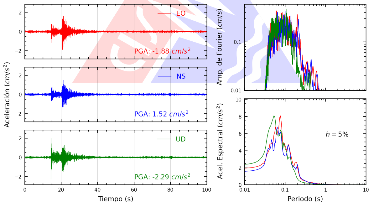
Figura A.14: Registros tiempo-historia, espectros de Fourier y de respuesta en las direcciones EO, NS y vertical de la estación SCCHO. Sismo de Chilca, Cañete - Lima del 2025-10-20, 20:23:44 (Hora local)
