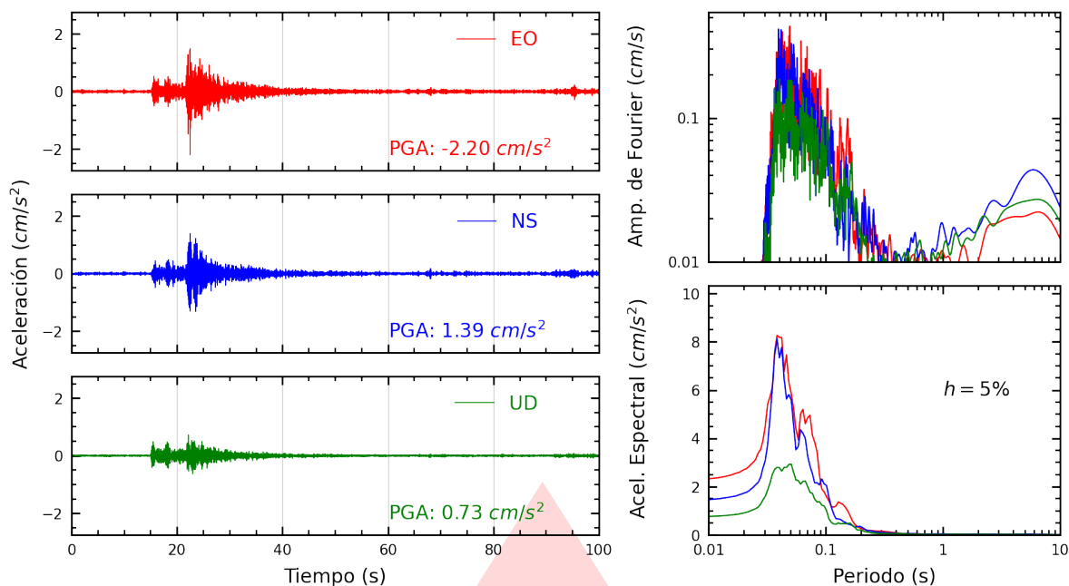
Figura A.15: Registros tiempo-historia, espectros de Fourier y de respuesta en las direcciones EO, NS y vertical de la estación CEPRE. Sismo de Chilca, Cañete - Lima del 2025-10-20, 20:23:44 (Hora local)
