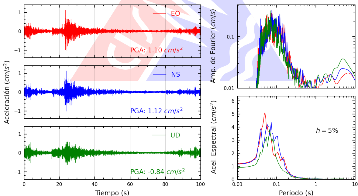
Figura A.26: Registros tiempo-historia, espectros de Fourier y de respuesta en las direcciones EO, NS y vertical de la estación SJLSV. Sismo de Chilca, Cañete - Lima del 2025-10-20, 20:23:44 (Hora local)
