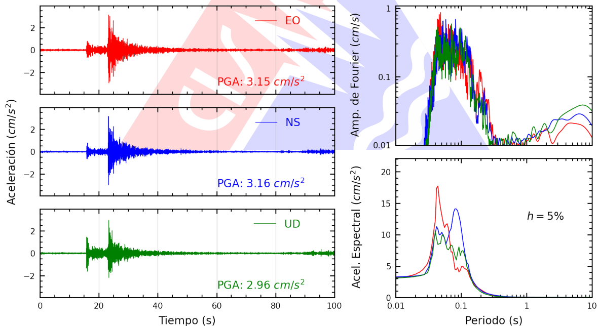
Figura A.10: Registros tiempo-historia, espectros de Fourier y de respuesta en las direcciones EO, NS y vertical de la estación INDEP. Sismo de Chilca, Cañete - Lima del 2025-10-20, 20:23:44 (Hora local)
