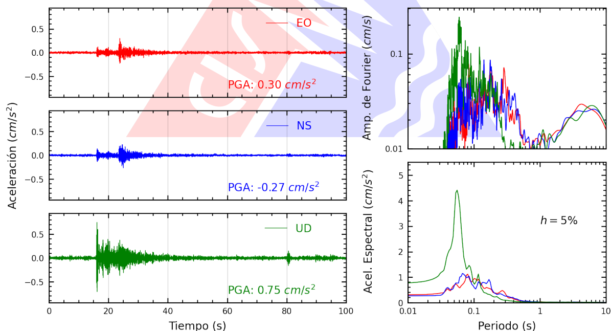
Figura A.36: Registros tiempo-historia, espectros de Fourier y de respuesta en las direcciones EO, NS y vertical de la estación ACAPU. Sismo de Chilca, Cañete - Lima del 2025-10-20, 20:23:44 (Hora local)
