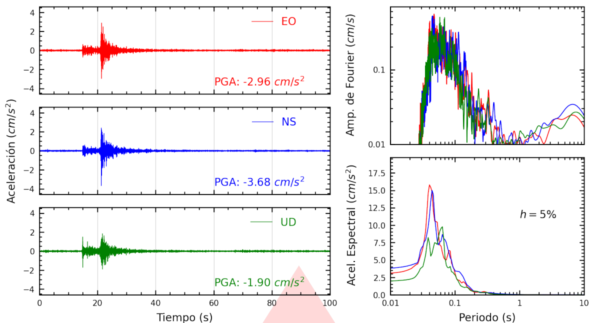
Figura A.7: Registros tiempo-historia, espectros de Fourier y de respuesta en las direcciones EO, NS y vertical de la estación URPE. Sismo de Chilca, Cañete - Lima del 2025-10-20, 20:23:44 (Hora local)
