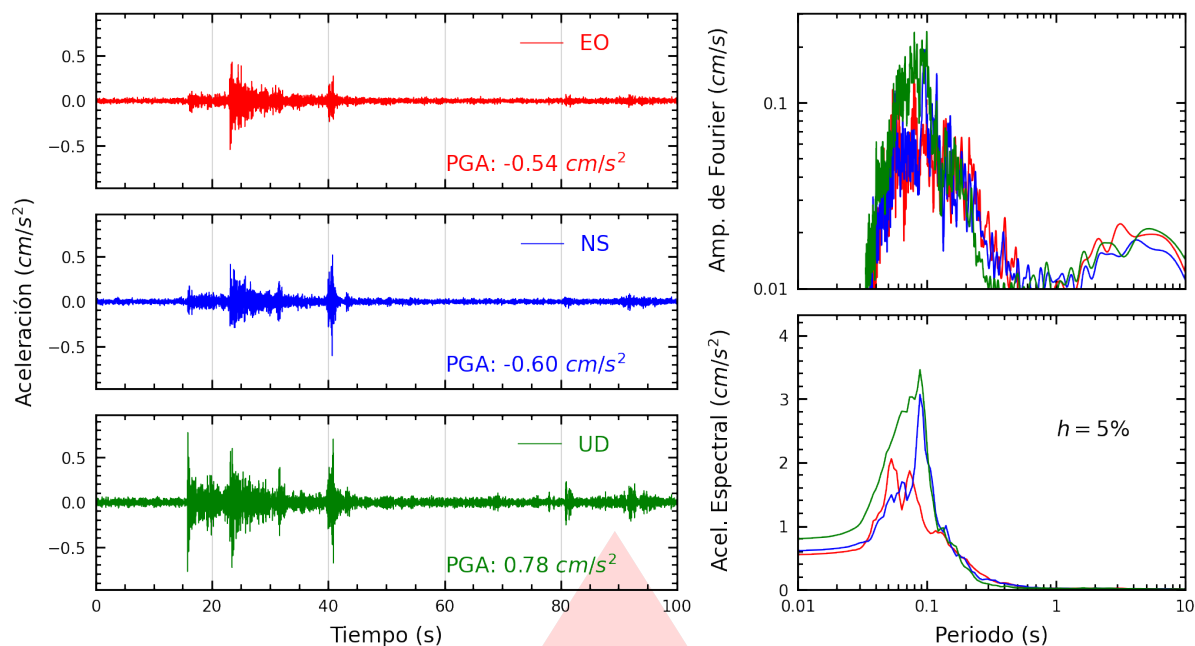
Figura A.35: Registros tiempo-historia, espectros de Fourier y de respuesta en las direcciones EO, NS y vertical de la estación RAMON. Sismo de Chilca, Cañete - Lima del 2025-10-20, 20:23:44 (Hora local)
