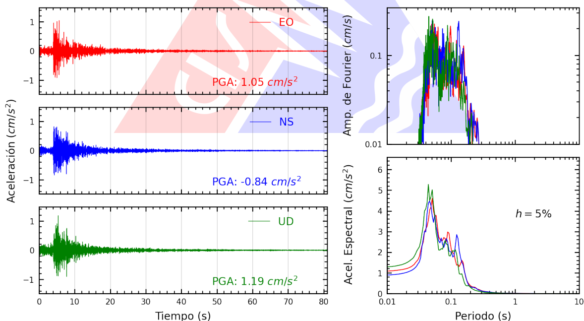
Figura A.24: Registros tiempo-historia, espectros de Fourier y de respuesta en las direcciones EO, NS y vertical de la estación JALV2. Sismo de Chilca, Cañete - Lima del 2025-10-20, 20:23:44 (Hora local)
