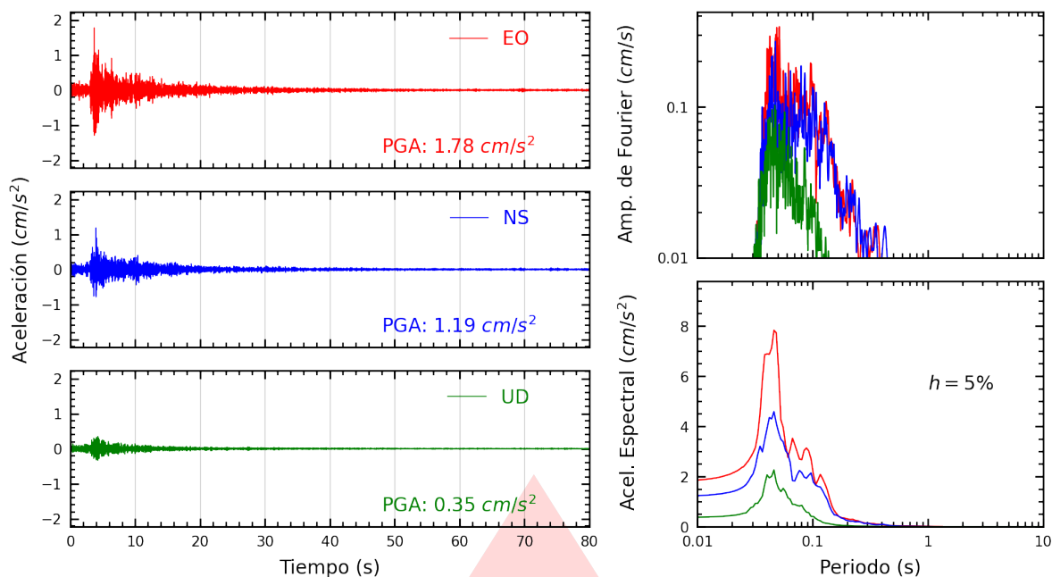
Figura A.21: Registros tiempo-historia, espectros de Fourier y de respuesta en las direcciones EO, NS y vertical de la estación UCVAT. Sismo de Chilca, Cañete - Lima del 2025-10-20, 20:23:44 (Hora local)
