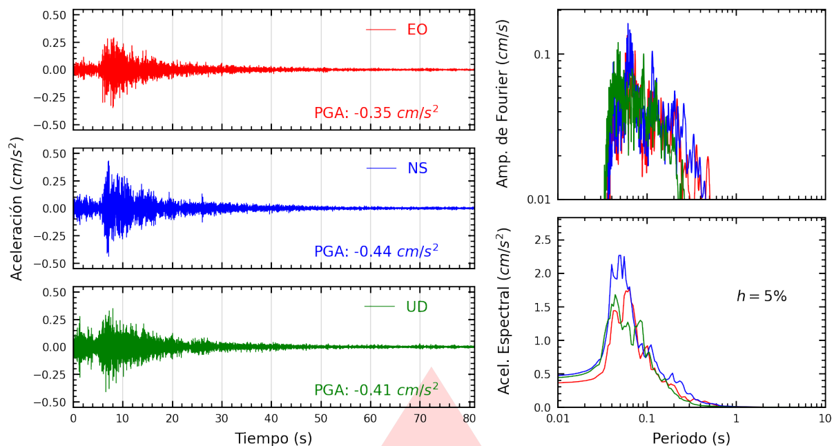
Figura A.39: Registros tiempo-historia, espectros de Fourier y de respuesta en las direcciones EO, NS y vertical de la estación VHAYA. Sismo de Chilca, Cañete - Lima del 2025-10-20, 20:23:44 (Hora local)
