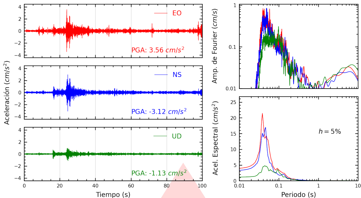
Figura A.9: Registros tiempo-historia, espectros de Fourier y de respuesta en las direcciones EO, NS y vertical de la estación OLIVO. Sismo de Chilca, Cañete - Lima del 2025-10-20, 20:23:44 (Hora local)
