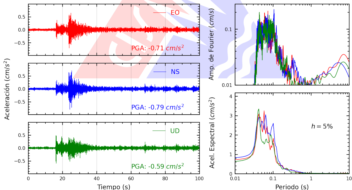
Figura A.34: Registros tiempo-historia, espectros de Fourier y de respuesta en las direcciones EO, NS y vertical de la estación MADRE. Sismo de Chilca, Cañete - Lima del 2025-10-20, 20:23:44 (Hora local)
