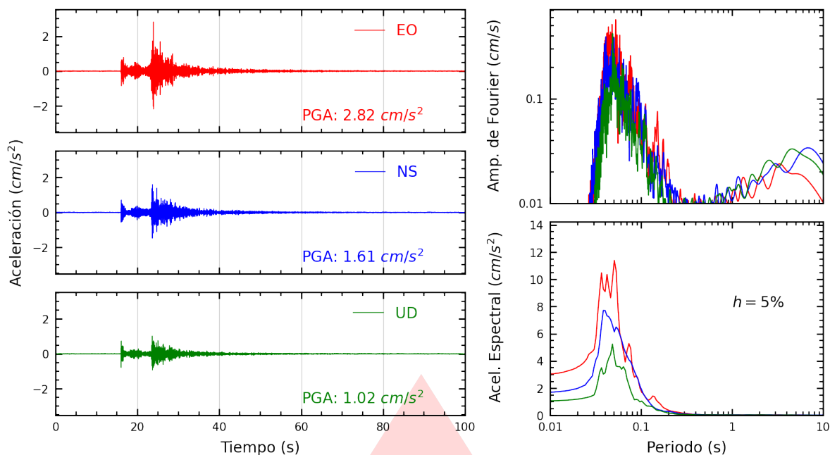
Figura A.11: Registros tiempo-historia, espectros de Fourier y de respuesta en las direcciones EO, NS y vertical de la estación UCSS. Sismo de Chilca, Cañete - Lima del 2025-10-20, 20:23:44 (Hora local)
