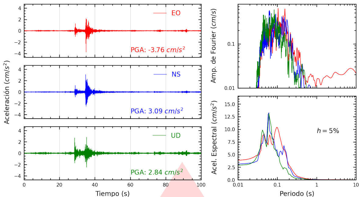
Figura A.5: Registros tiempo-historia, espectros de Fourier y de respuesta en las direcciones EO, NS y vertical de la estación SOCHO. Sismo de Chilca, Cañete - Lima del 2025-10-20, 20:23:44 (Hora local)
