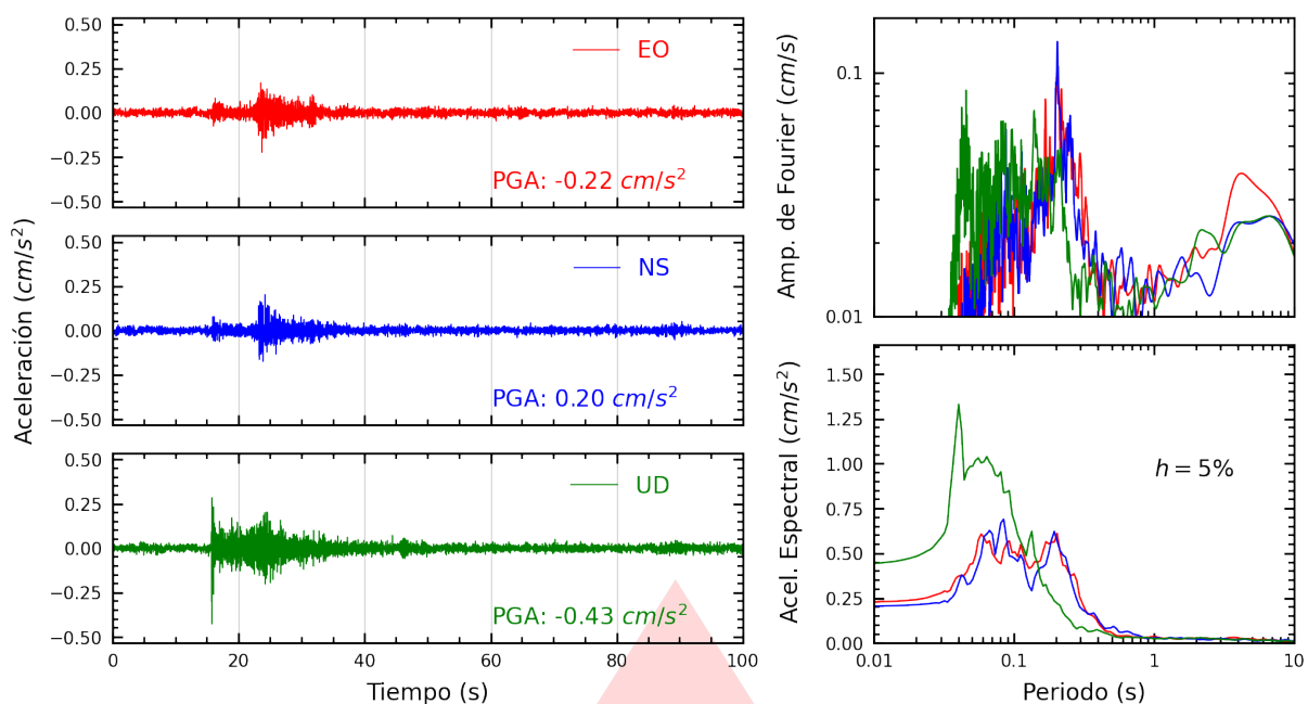
Figura A.41: Registros tiempo-historia, espectros de Fourier y de respuesta en las direcciones EO, NS y vertical de la estación DSML. Sismo de Chilca, Cañete - Lima del 2025-10-20, 20:23:44 (Hora local)
