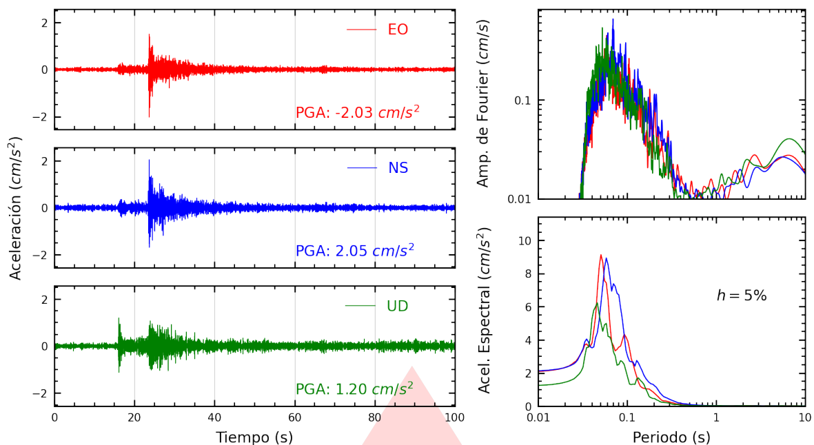
Figura A.17: Registros tiempo-historia, espectros de Fourier y de respuesta en las direcciones EO, NS y vertical de la estación SJLSC. Sismo de Chilca, Cañete - Lima del 2025-10-20, 20:23:44 (Hora local)
