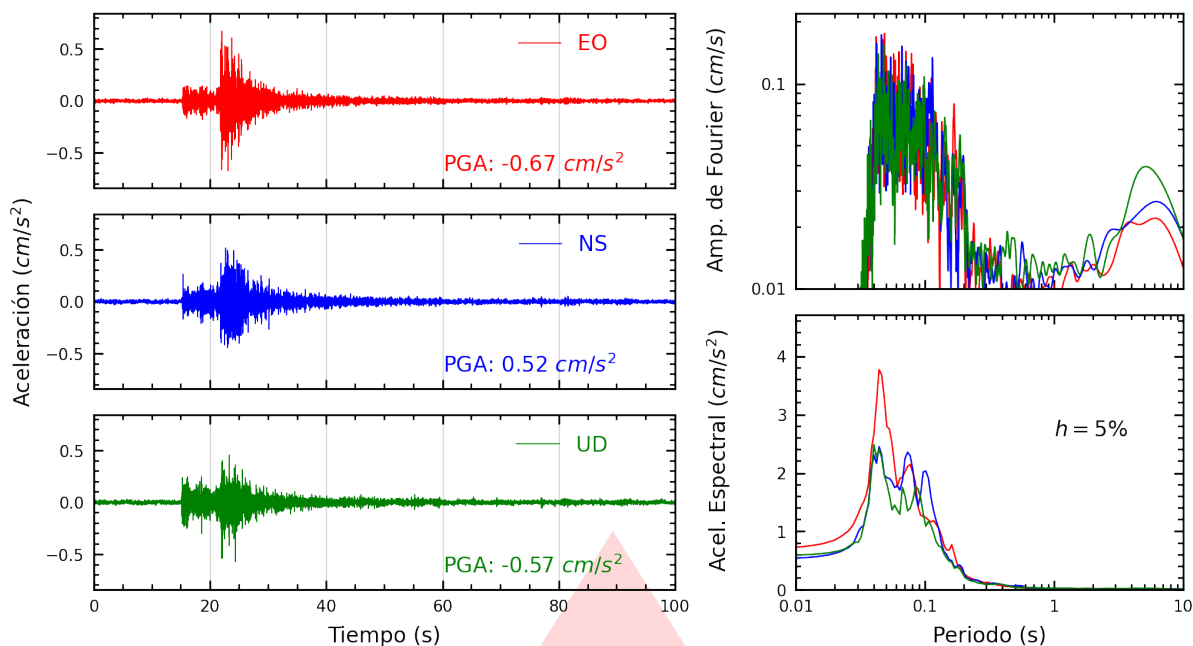
Figura A.37: Registros tiempo-historia, espectros de Fourier y de respuesta en las direcciones EO, NS y vertical de la estación UNFV. Sismo de Chilca, Cañete - Lima del 2025-10-20, 20:23:44 (Hora local)
