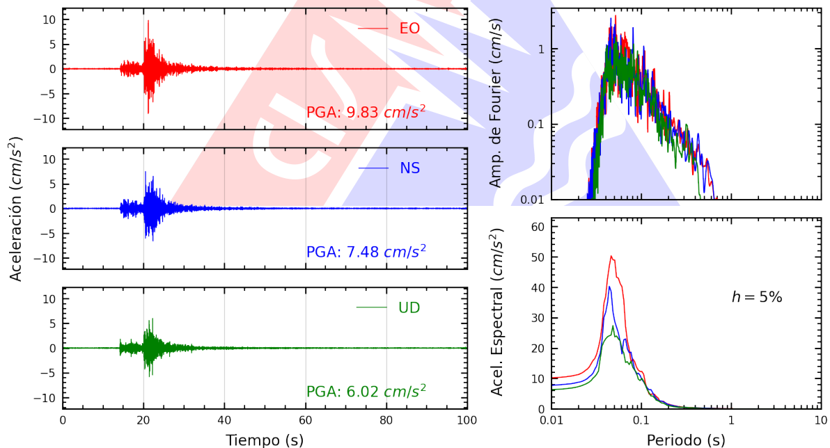
Figura A.2: Registros tiempo-historia, espectros de Fourier y de respuesta en las direcciones EO, NS y vertical de la estación UNTEL. Sismo de Chilca, Cañete - Lima del 2025-10-20, 20:23:44 (Hora local)
