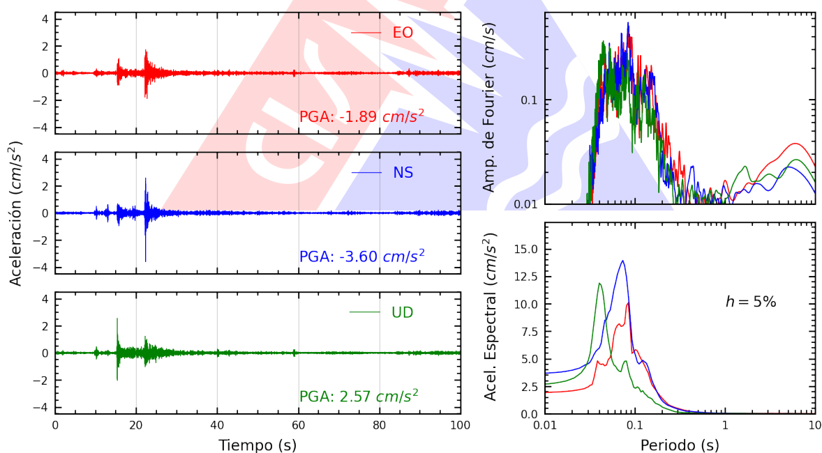
Figura A.8: Registros tiempo-historia, espectros de Fourier y de respuesta en las direcciones EO, NS y vertical de la estación UPCSM. Sismo de Chilca, Cañete - Lima del 2025-10-20, 20:23:44 (Hora local)
