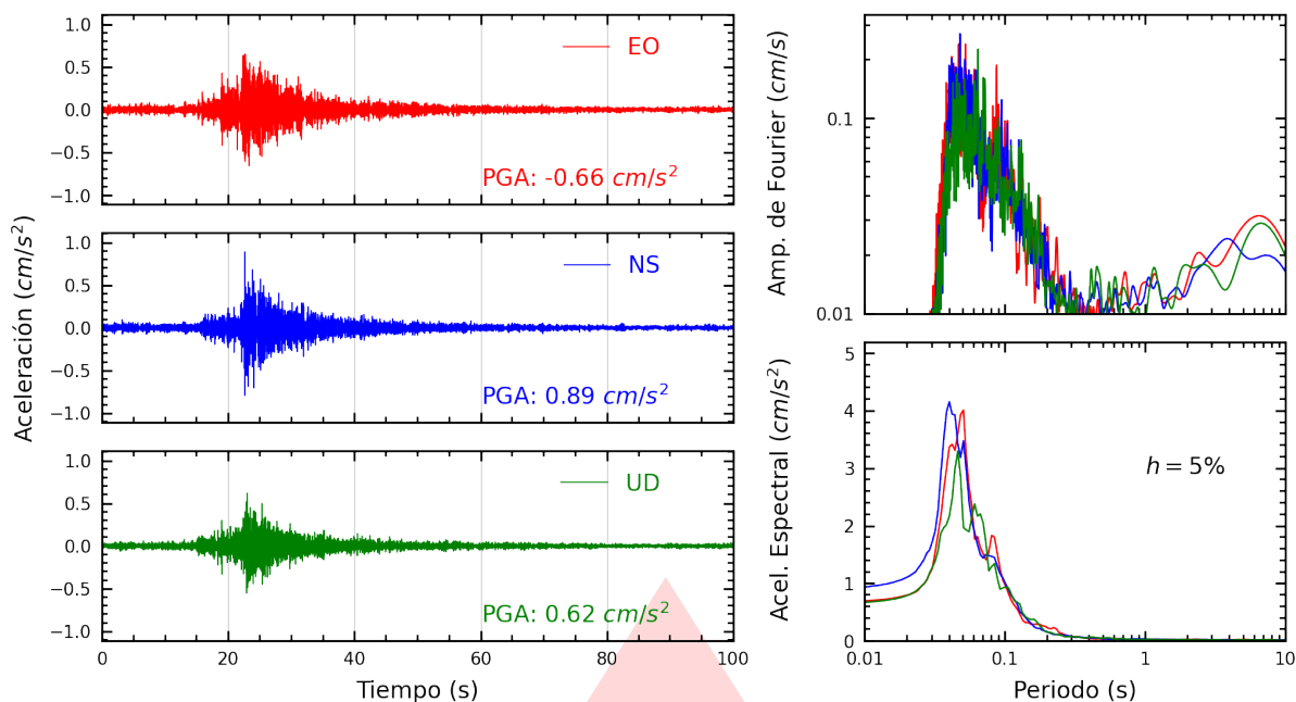
Figura A.31: Registros tiempo-historia, espectros de Fourier y de respuesta en las direcciones EO, NS y vertical de la estación IMCA. Sismo de Chilca, Cañete - Lima del 2025-10-20, 20:23:44 (Hora local)
