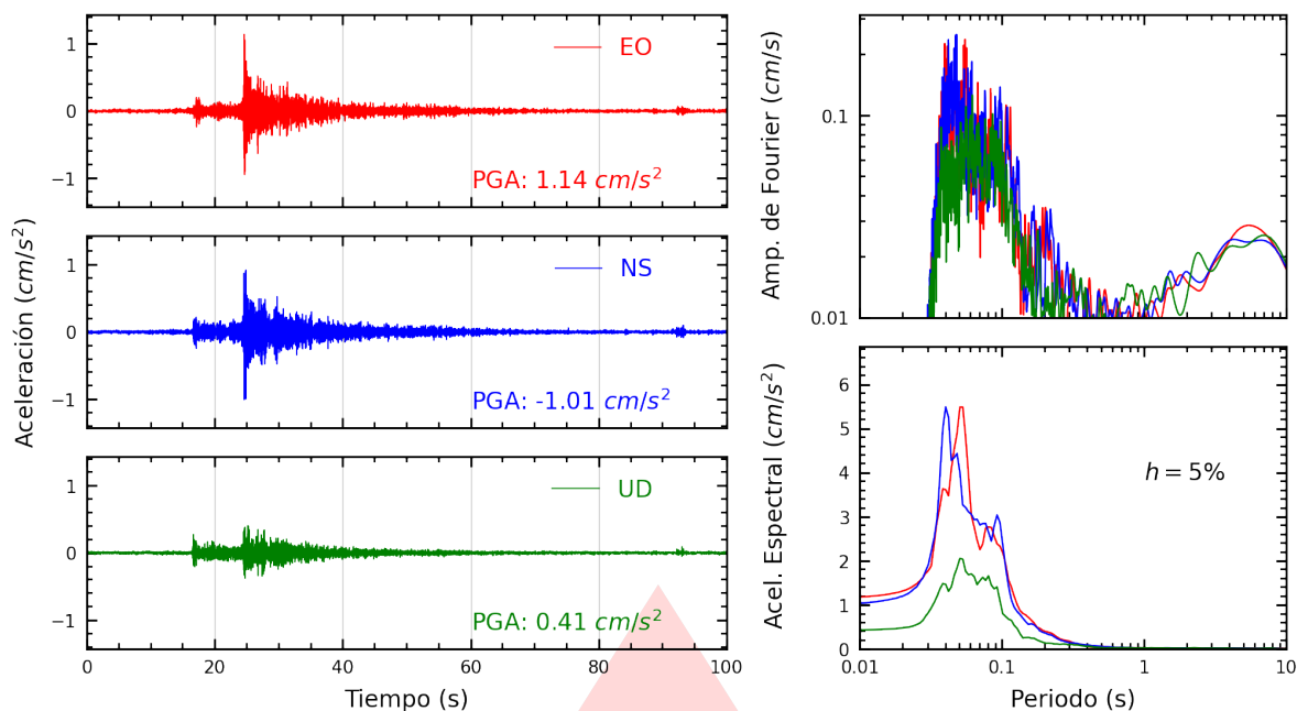
Figura A.25: Registros tiempo-historia, espectros de Fourier y de respuesta en las direcciones EO, NS y vertical de la estación COMAS. Sismo de Chilca, Cañete - Lima del 2025-10-20, 20:23:44 (Hora local)
