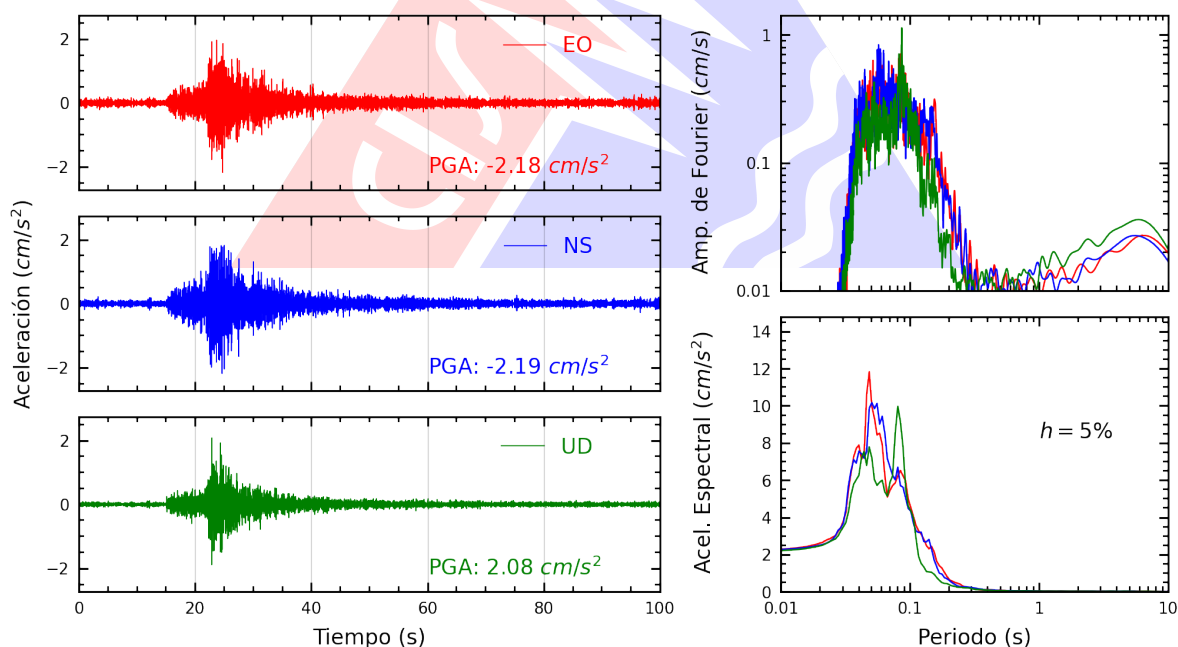
Figura A.16: Registros tiempo-historia, espectros de Fourier y de respuesta en las direcciones EO, NS y vertical de la estación USILM. Sismo de Chilca, Cañete - Lima del 2025-10-20, 20:23:44 (Hora local)
