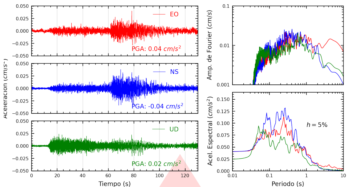
Figura A.15: Registros tiempo-historia, espectros de Fourier y de respuesta en las direcciones EO, NS y vertical de la estación SCCHI. Sismo de Uchiza, Tocache - San Martín del 2025-10-21, 00:24:09 (Hora local)
