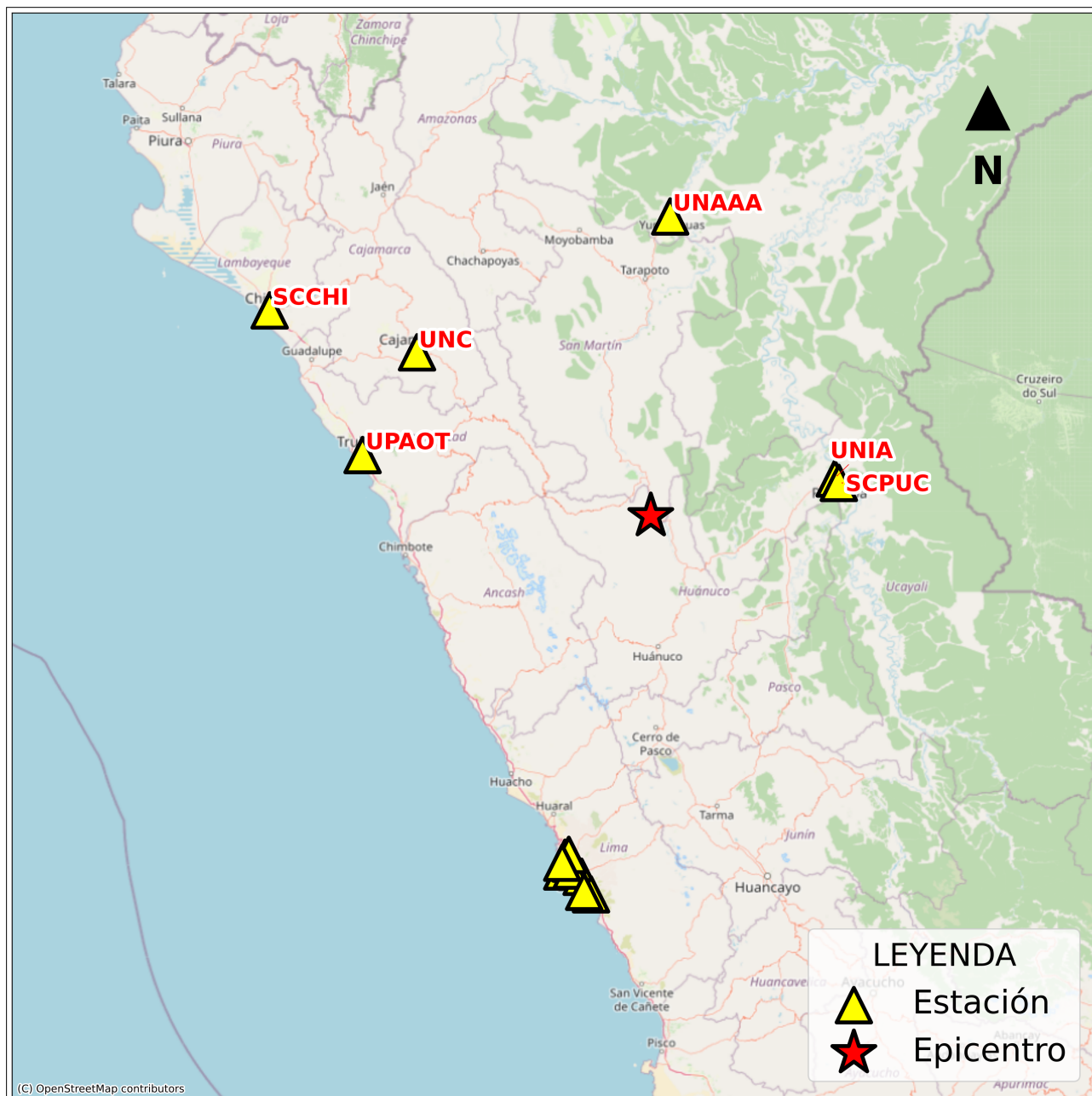
Figura 2: Mapa de ubicación de la(s) estación(es) acelerográfica(s) a nivel nacional correspondiente(s) al Sismo de Uchiza, Tocache - San Martín del 21 de octubre de 2025 a las 00:24:09 (hora local)
