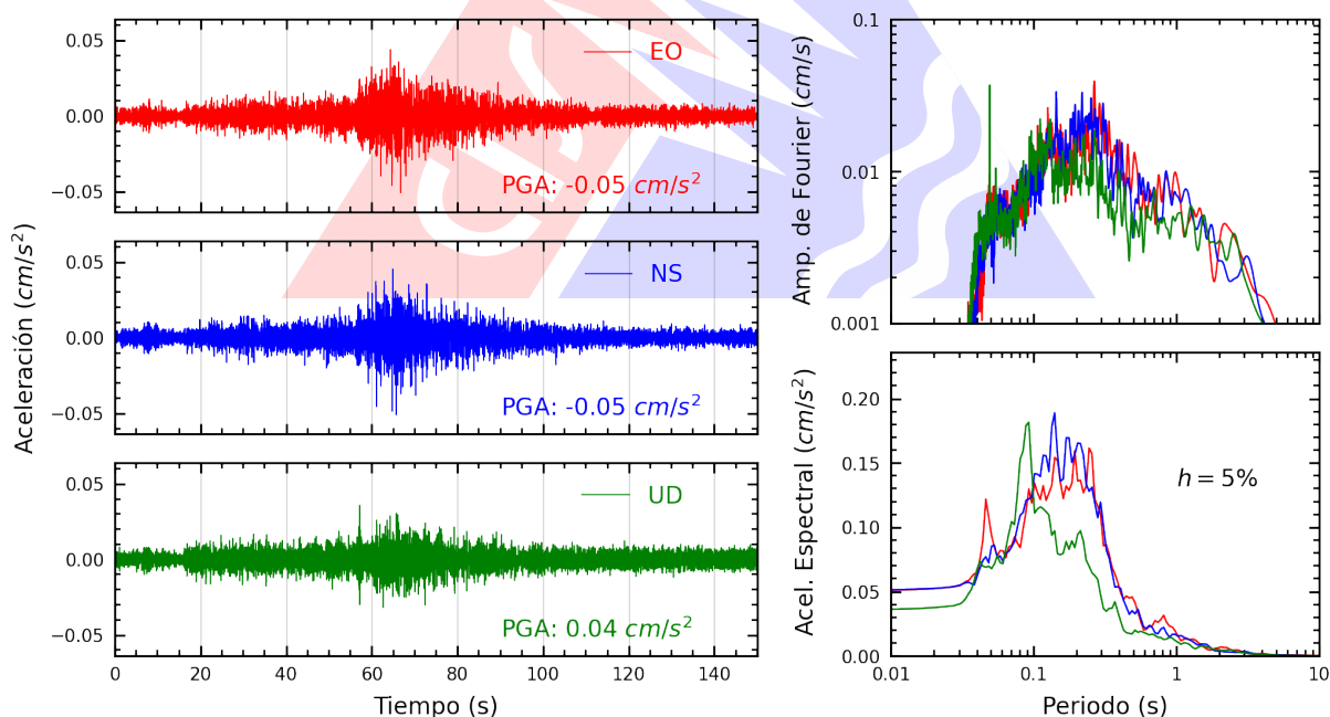
Figura A.14: Registros tiempo-historia, espectros de Fourier y de respuesta en las direcciones EO, NS y vertical de la estación JALV2. Sismo de Uchiza, Tocache - San Martín del 2025-10-21, 00:24:09 (Hora local)
