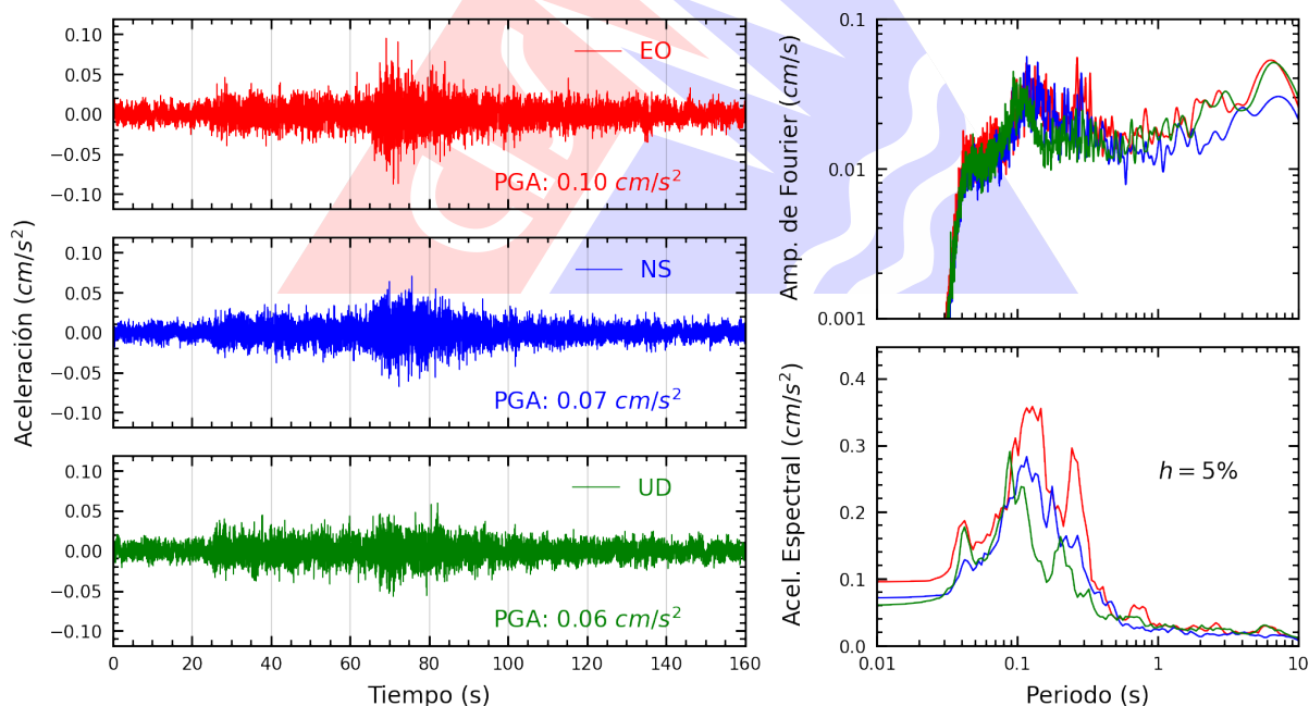
Figura A.12: Registros tiempo-historia, espectros de Fourier y de respuesta en las direcciones EO, NS y vertical de la estación AMORE. Sismo de Uchiza, Tocache - San Martín del 2025-10-21, 00:24:09 (Hora local)
