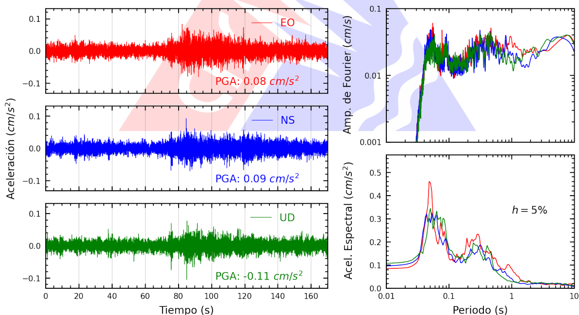
Figura A.10: Registros tiempo-historia, espectros de Fourier y de respuesta en las direcciones EO, NS y vertical de la estación IMCA. Sismo de Uchiza, Tocache - San Martín del 2025-10-21, 00:24:09 (Hora local)
