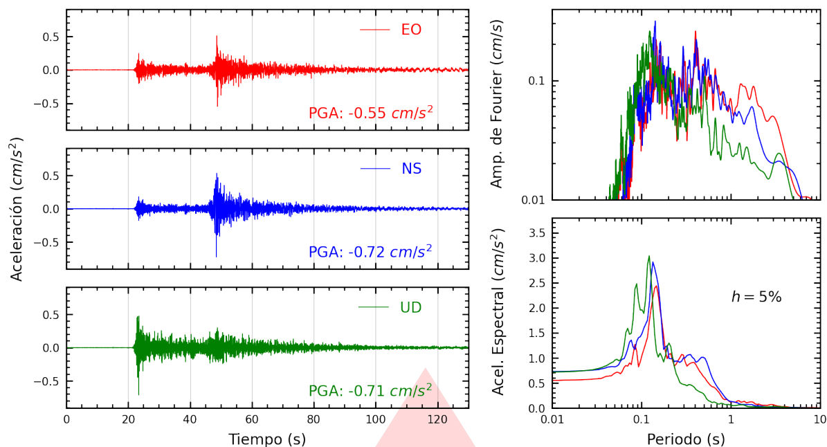
Figura A.1: Registros tiempo-historia, espectros de Fourier y de respuesta en las direcciones EO, NS y vertical de la estación UNIA. Sismo de Uchiza, Tocache - San Martín del 2025-10-21, 00:24:09 (Hora local)
