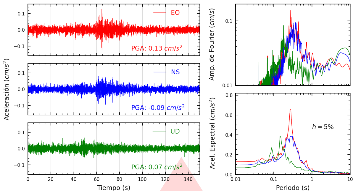
Figura A.9: Registros tiempo-historia, espectros de Fourier y de respuesta en las direcciones EO, NS y vertical de la estación ACAPU. Sismo de Uchiza, Tocache - San Martín del 2025-10-21, 00:24:09 (Hora local)
