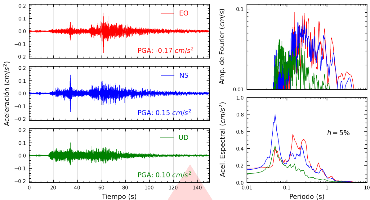
Figura A.7: Registros tiempo-historia, espectros de Fourier y de respuesta en las direcciones EO, NS y vertical de la estación UNAAA. Sismo de Uchiza, Tocache - San Martín del 2025-10-21, 00:24:09 (Hora local)
