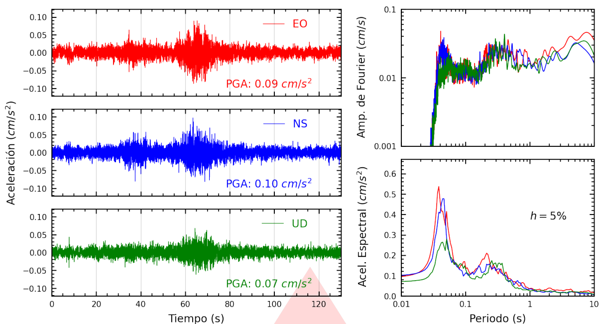
Figura A.11: Registros tiempo-historia, espectros de Fourier y de respuesta en las direcciones EO, NS y vertical de la estación COMAS. Sismo de Uchiza, Tocache - San Martín del 2025-10-21, 00:24:09 (Hora local)
