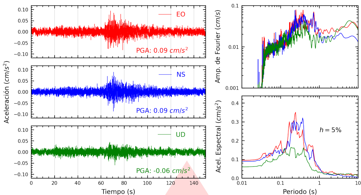
Figura A.13: Registros tiempo-historia, espectros de Fourier y de respuesta en las direcciones EO, NS y vertical de la estación USILP. Sismo de Uchiza, Tocache - San Martín del 2025-10-21, 00:24:09 (Hora local)
