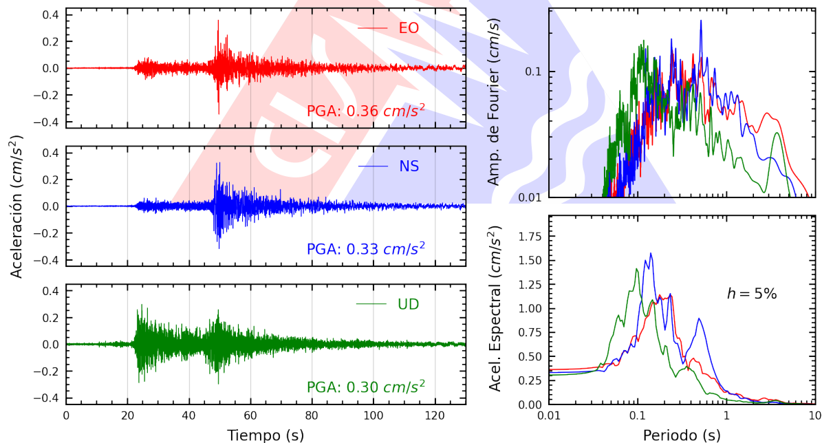
Figura A.2: Registros tiempo-historia, espectros de Fourier y de respuesta en las direcciones EO, NS y vertical de la estación SCPUC. Sismo de Uchiza, Tocache - San Martín del 2025-10-21, 00:24:09 (Hora local)
