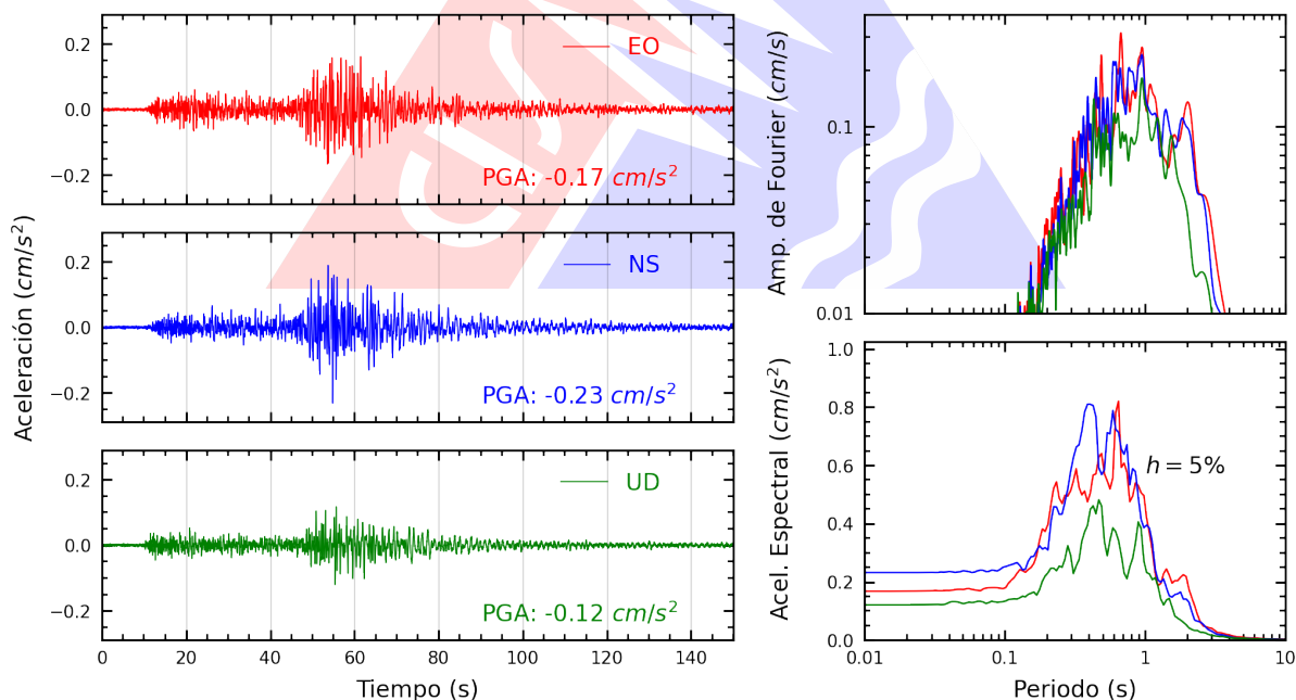
Figura A.4: Registros tiempo-historia, espectros de Fourier y de respuesta en las direcciones EO, NS y vertical de la estación UNC. Sismo de Uchiza, Tocache - San Martín del 2025-10-21, 00:24:09 (Hora local)
