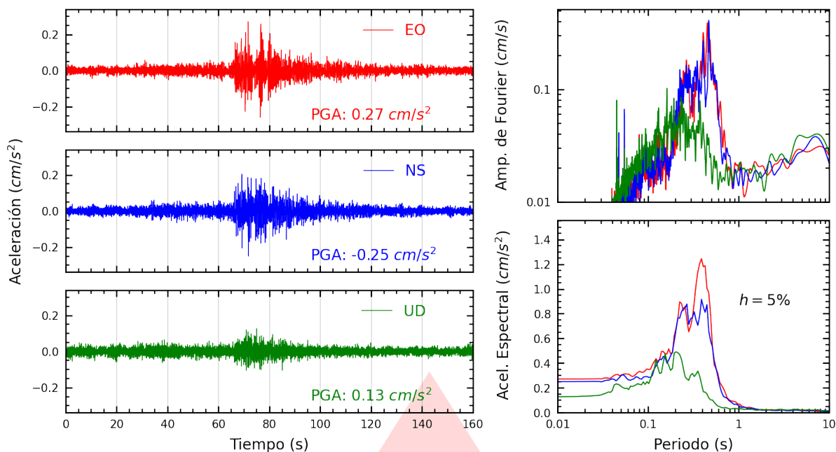
Figura A.3: Registros tiempo-historia, espectros de Fourier y de respuesta en las direcciones EO, NS y vertical de la estación MDPP. Sismo de Uchiza, Tocache - San Martín del 2025-10-21, 00:24:09 (Hora local)
