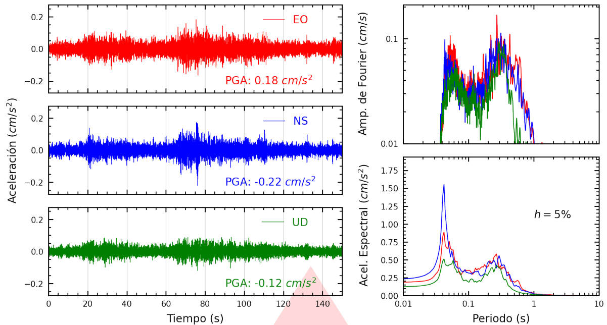
Figura A.5: Registros tiempo-historia, espectros de Fourier y de respuesta en las direcciones EO, NS y vertical de la estación UNTEL. Sismo de Uchiza, Tocache - San Martín del 2025-10-21, 00:24:09 (Hora local)
