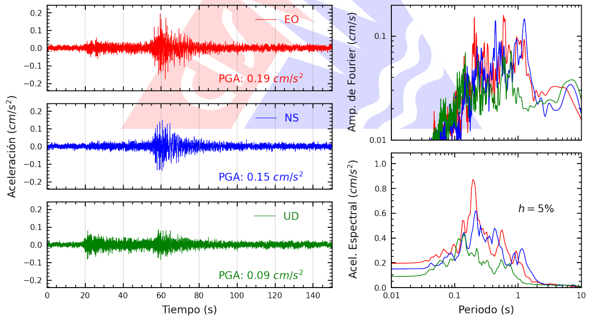
Figura A.6: Registros tiempo-historia, espectros de Fourier y de respuesta en las direcciones EO, NS y vertical de la estación UPAOT. Sismo de Uchiza, Tocache - San Martín del 2025-10-21, 00:24:09 (Hora local)
