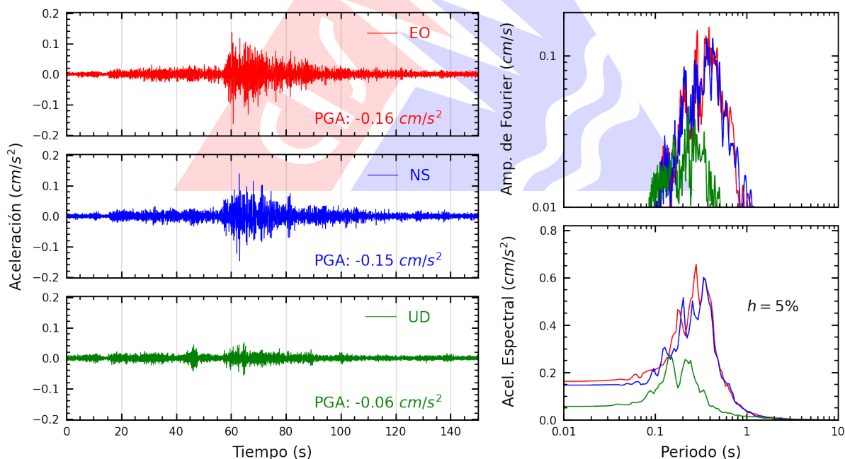
Figura A.8: Registros tiempo-historia, espectros de Fourier y de respuesta en las direcciones EO, NS y vertical de la estación VHAYA. Sismo de Uchiza, Tocache - San Martín del 2025-10-21, 00:24:09 (Hora local)
