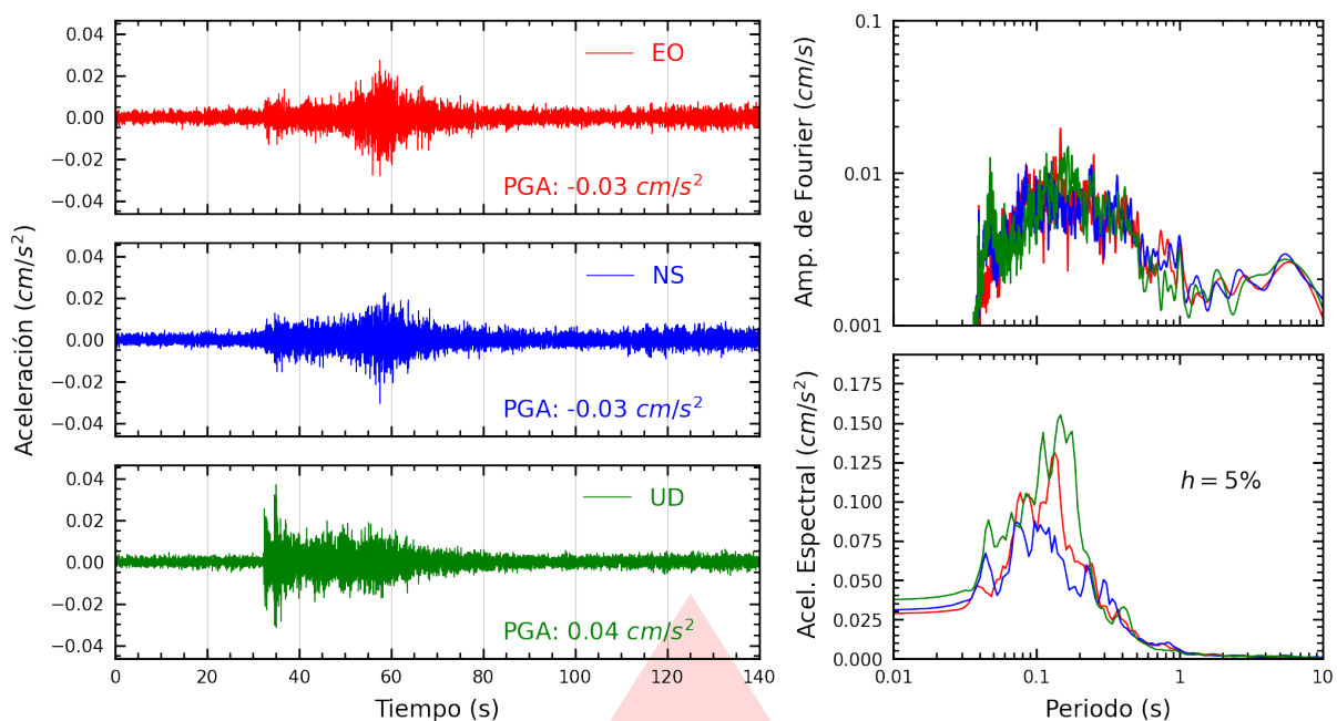
Figura A.1: Registros tiempo-historia, espectros de Fourier y de respuesta en las direcciones EO, NS y vertical de la estación UNF. Sismo de Zarumilla, Zarumilla - Tumbes del 2025-10-22, 23:18:56 (Hora local)
