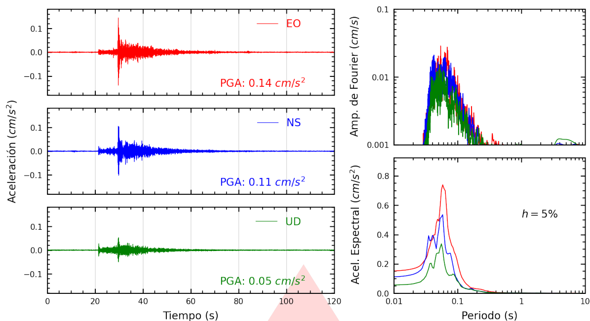
Figura A.1: Registros tiempo-historia, espectros de Fourier y de respuesta en las direcciones EO, NS y vertical de la estación UNSA2. Sismo de Arequipa, Arequipa - Arequipa del 2025-10-23, 00:46:39 (Hora local)
