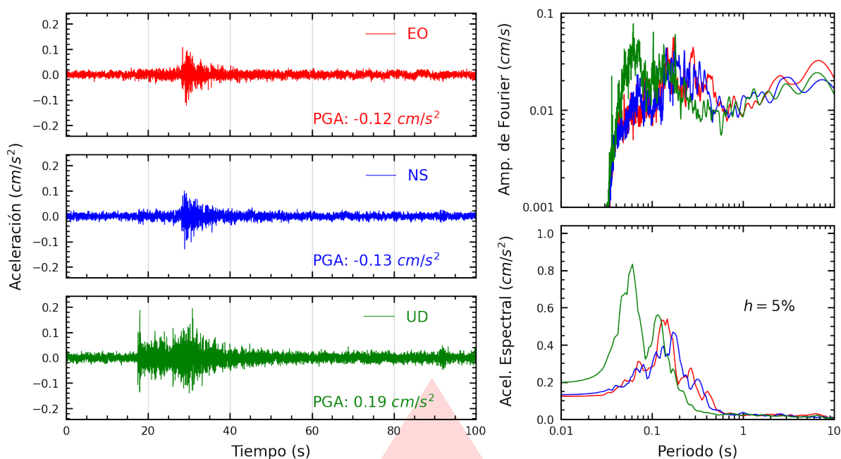
Figura A.29: Registros tiempo-historia, espectros de Fourier y de respuesta en las direcciones EO, NS y vertical de la estación ACAPU. Sismo de Chilca, Cañete - Lima del 2025-10-15, 03:30:51 (Hora local)
