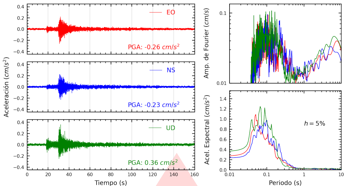
Figura A.23: Registros tiempo-historia, espectros de Fourier y de respuesta en las direcciones EO, NS y vertical de la estación MDPP. Sismo de Chilca, Cañete - Lima del 2025-10-15, 03:30:51 (Hora local)
