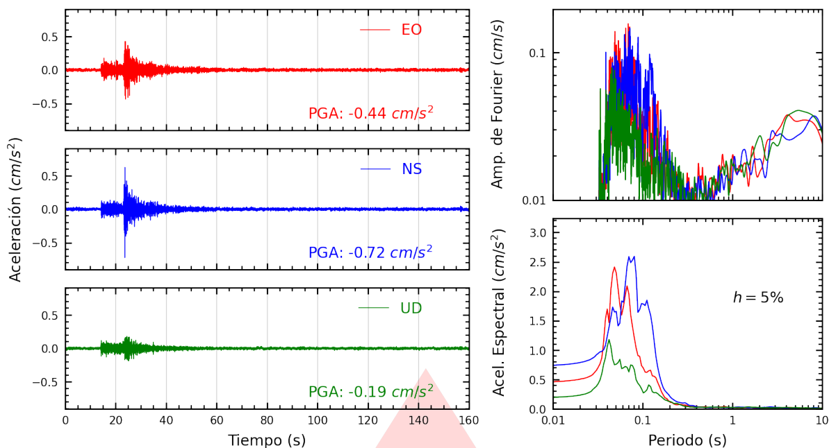
Figura A.11: Registros tiempo-historia, espectros de Fourier y de respuesta en las direcciones EO, NS y vertical de la estación UPCVI. Sismo de Chilca, Cañete - Lima del 2025-10-15, 03:30:51 (Hora local)
