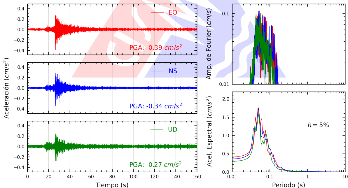
Figura A.20: Registros tiempo-historia, espectros de Fourier y de respuesta en las direcciones EO, NS y vertical de la estación ATARJ. Sismo de Chilca, Cañete - Lima del 2025-10-15, 03:30:51 (Hora local)
