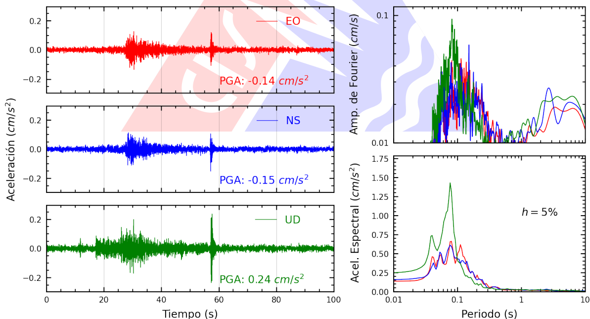
Figura A.28: Registros tiempo-historia, espectros de Fourier y de respuesta en las direcciones EO, NS y vertical de la estación RAMON. Sismo de Chilca, Cañete - Lima del 2025-10-15, 03:30:51 (Hora local)
