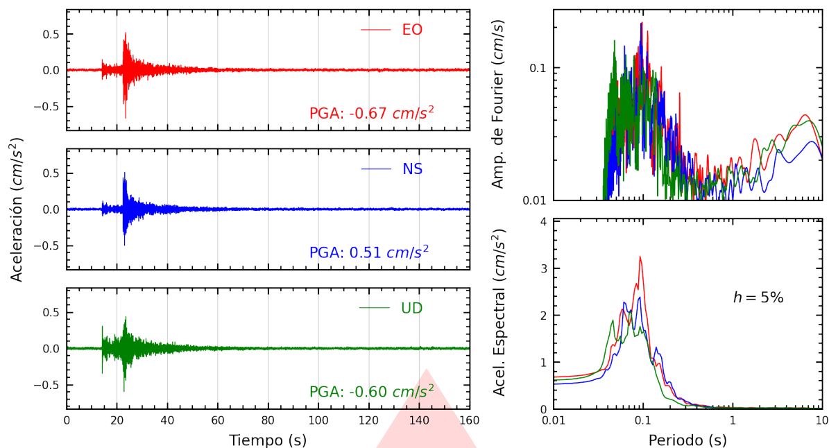
Figura A.13: Registros tiempo-historia, espectros de Fourier y de respuesta en las direcciones EO, NS y vertical de la estación USILP. Sismo de Chilca, Cañete - Lima del 2025-10-15, 03:30:51 (Hora local)
