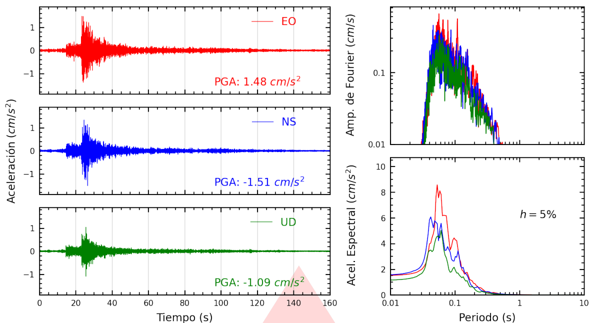
Figura A.1: Registros tiempo-historia, espectros de Fourier y de respuesta en las direcciones EO, NS y vertical de la estación UNTEL. Sismo de Chilca, Cañete - Lima del 2025-10-15, 03:30:51 (Hora local)
