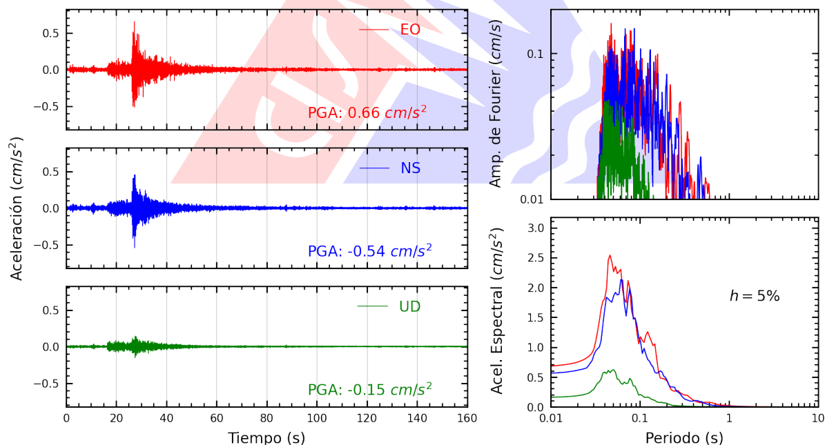
Figura A.14: Registros tiempo-historia, espectros de Fourier y de respuesta en las direcciones EO, NS y vertical de la estación UCVAT. Sismo de Chilca, Cañete - Lima del 2025-10-15, 03:30:51 (Hora local)
