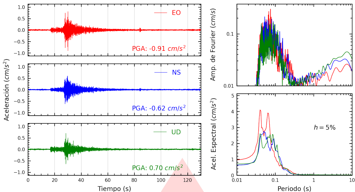
Figura A.7: Registros tiempo-historia, espectros de Fourier y de respuesta en las direcciones EO, NS y vertical de la estación INDEP. Sismo de Chilca, Cañete - Lima del 2025-10-15, 03:30:51 (Hora local)
