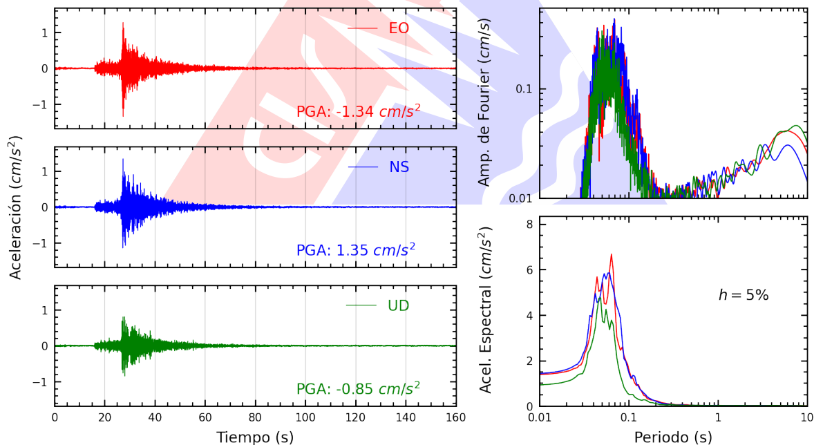
Figura A.4: Registros tiempo-historia, espectros de Fourier y de respuesta en las direcciones EO, NS y vertical de la estación JOSEO. Sismo de Chilca, Cañete - Lima del 2025-10-15, 03:30:51 (Hora local)
