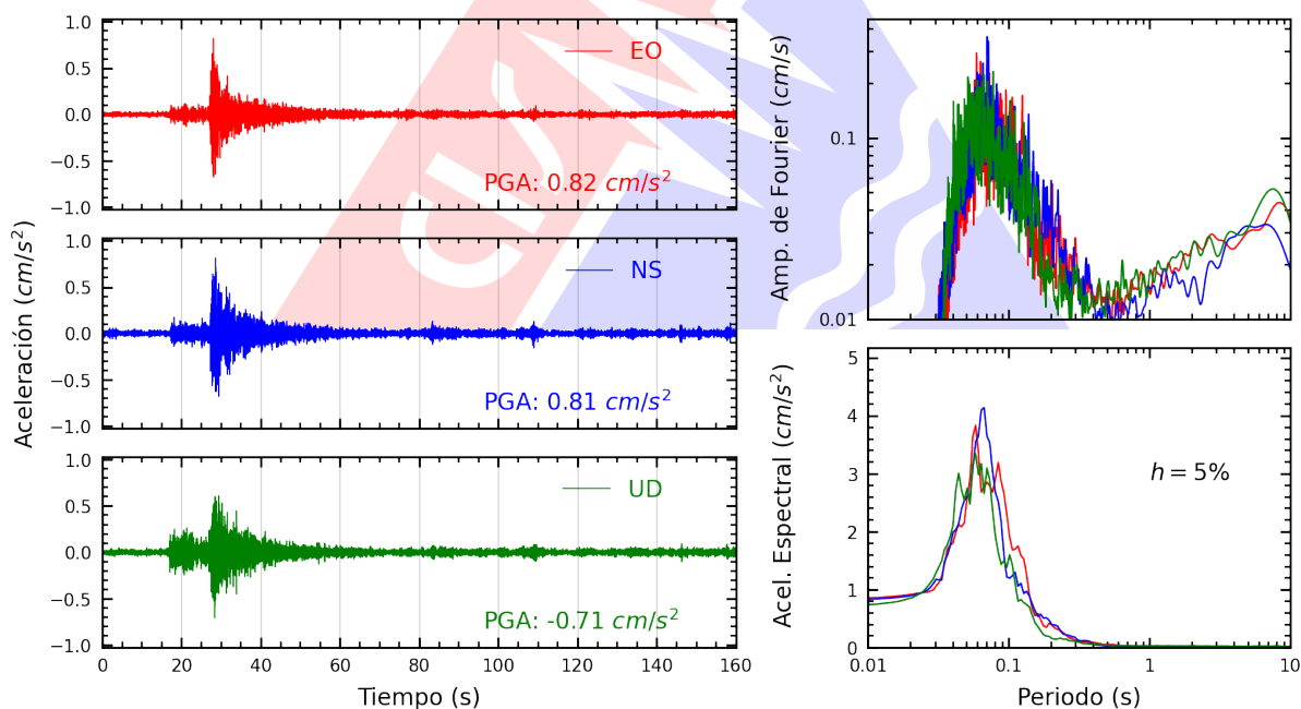
Figura A.8: Registros tiempo-historia, espectros de Fourier y de respuesta en las direcciones EO, NS y vertical de la estación SJLSC. Sismo de Chilca, Cañete - Lima del 2025-10-15, 03:30:51 (Hora local)
