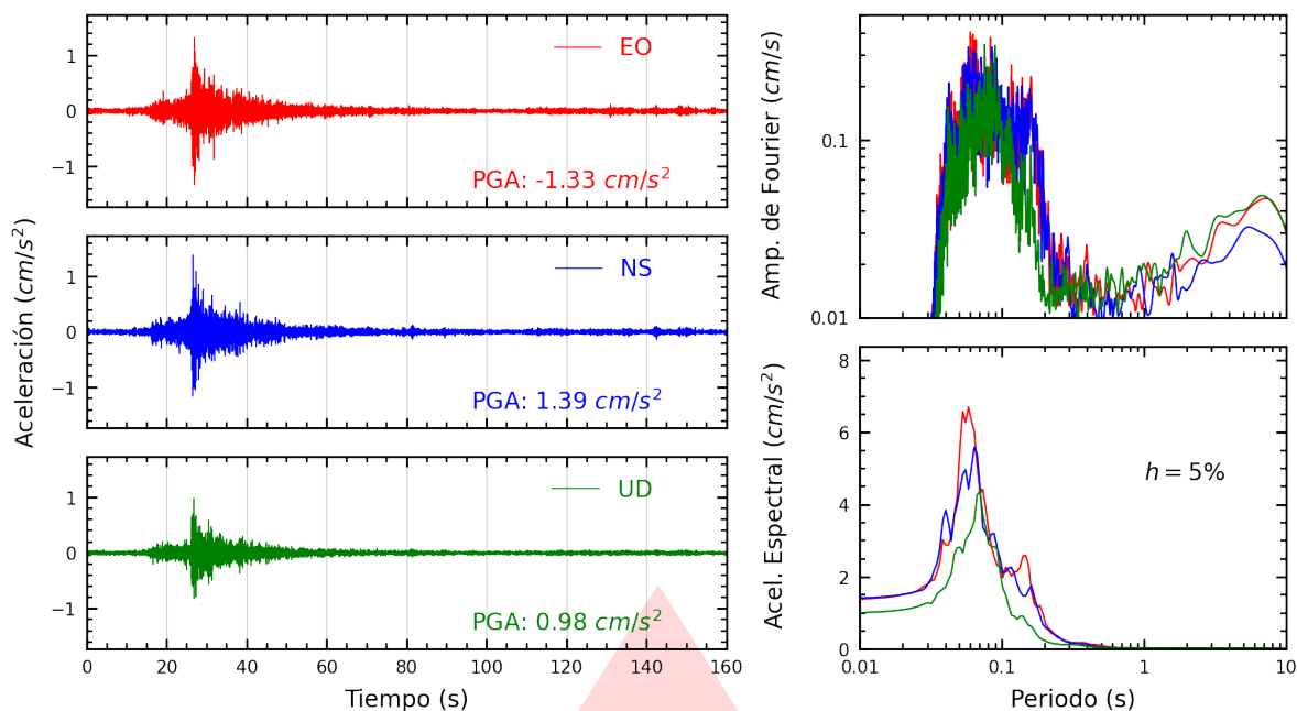
Figura A.3: Registros tiempo-historia, espectros de Fourier y de respuesta en las direcciones EO, NS y vertical de la estación USILM. Sismo de Chilca, Cañete - Lima del 2025-10-15, 03:30:51 (Hora local)
