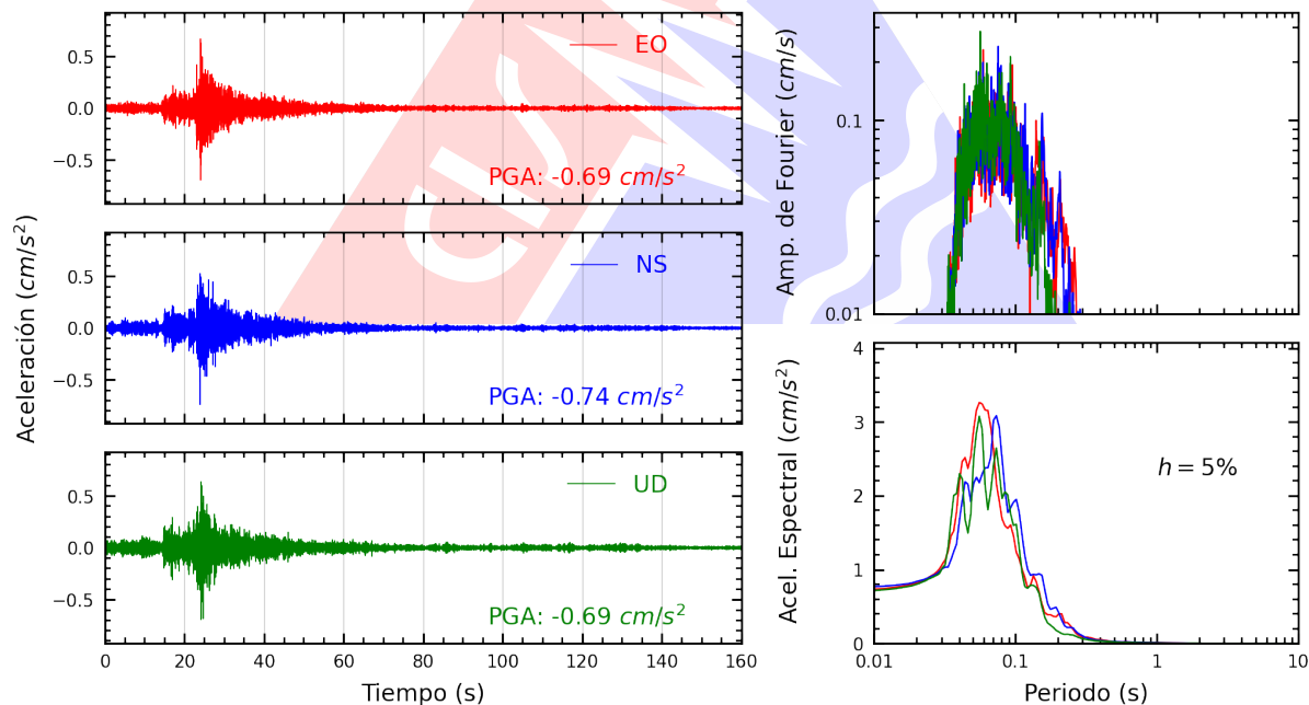
Figura A.10: Registros tiempo-historia, espectros de Fourier y de respuesta en las direcciones EO, NS y vertical de la estación ASIA. Sismo de Chilca, Cañete - Lima del 2025-10-15, 03:30:51 (Hora local)
