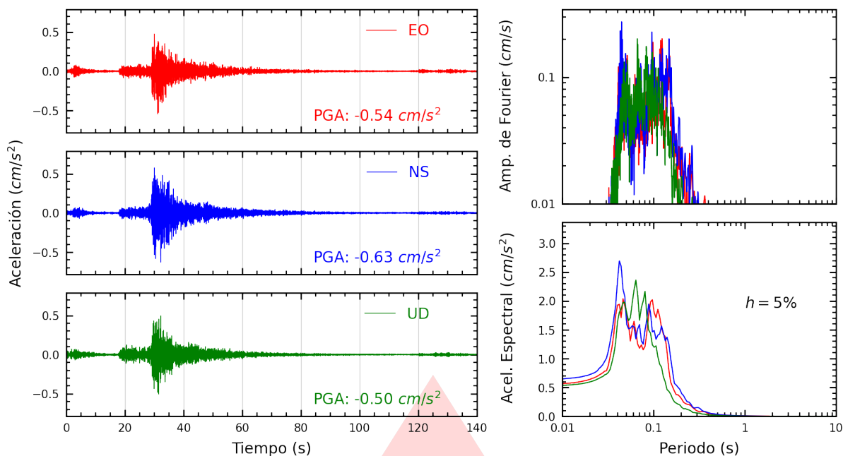
Figura A.15: Registros tiempo-historia, espectros de Fourier y de respuesta en las direcciones EO, NS y vertical de la estación CARAB. Sismo de Chilca, Cañete - Lima del 2025-10-15, 03:30:51 (Hora local)
