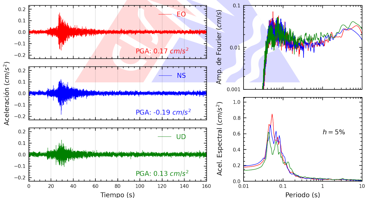
Figura A.30: Registros tiempo-historia, espectros de Fourier y de respuesta en las direcciones EO, NS y vertical de la estación UNFV. Sismo de Chilca, Cañete - Lima del 2025-10-15, 03:30:51 (Hora local)
