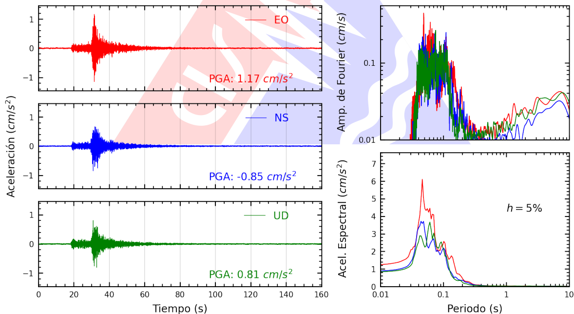
Figura A.6: Registros tiempo-historia, espectros de Fourier y de respuesta en las direcciones EO, NS y vertical de la estación AMORE. Sismo de Chilca, Cañete - Lima del 2025-10-15, 03:30:51 (Hora local)
