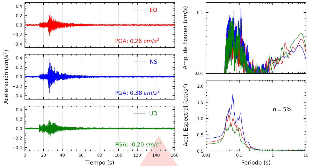
Figura A.21: Registros tiempo-historia, espectros de Fourier y de respuesta en las direcciones EO, NS y vertical de la estación SERVI. Sismo de Chilca, Cañete - Lima del 2025-10-15, 03:30:51 (Hora local)
