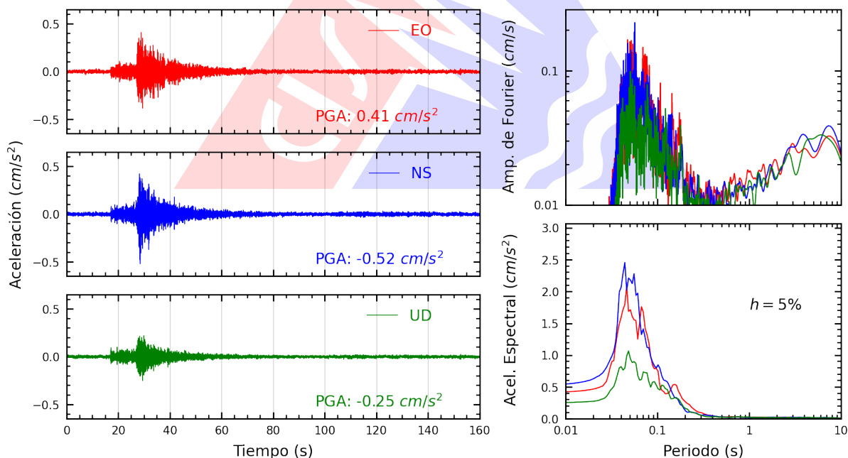
Figura A.16: Registros tiempo-historia, espectros de Fourier y de respuesta en las direcciones EO, NS y vertical de la estación FICPE. Sismo de Chilca, Cañete - Lima del 2025-10-15, 03:30:51 (Hora local)
