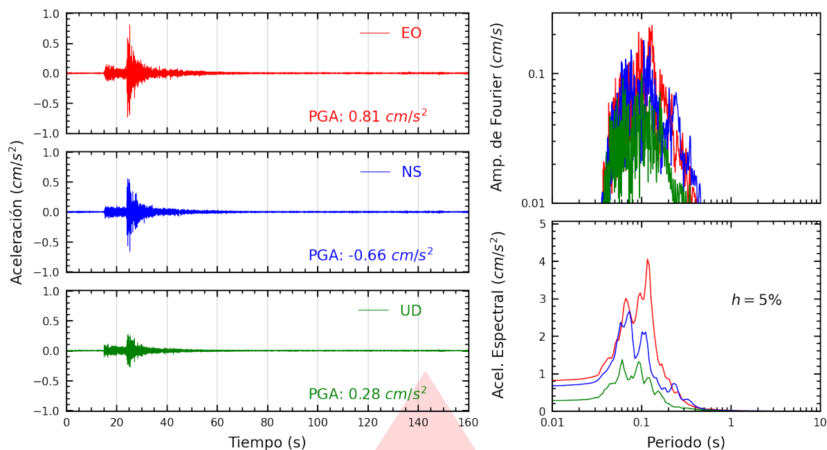
Figura A.9: Registros tiempo-historia, espectros de Fourier y de respuesta en las direcciones EO, NS y vertical de la estación BRISA. Sismo de Chilca, Cañete - Lima del 2025-10-15, 03:30:51 (Hora local)
