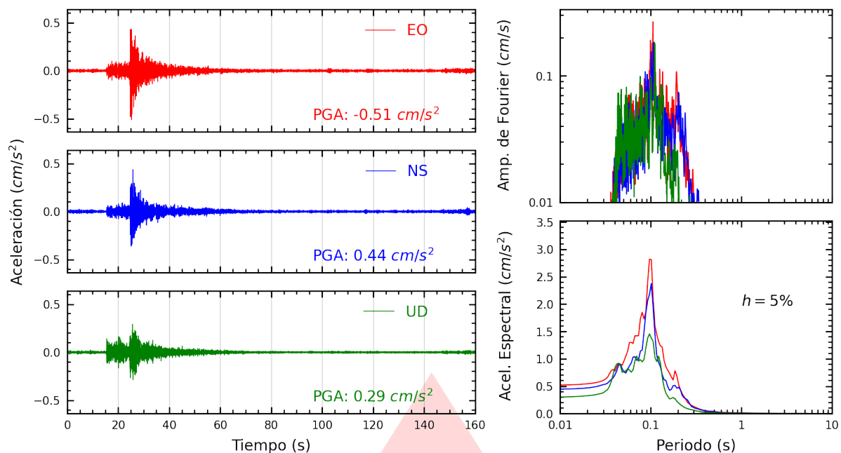
Figura A.17: Registros tiempo-historia, espectros de Fourier y de respuesta en las direcciones EO, NS y vertical de la estación SCCHO. Sismo de Chilca, Cañete - Lima del 2025-10-15, 03:30:51 (Hora local)
