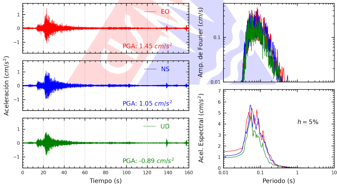
Figura A.2: Registros tiempo-historia, espectros de Fourier y de respuesta en las direcciones EO, NS y vertical de la estación PHERM. Sismo de Chilca, Cañete - Lima del 2025-10-15, 03:30:51 (Hora local)
