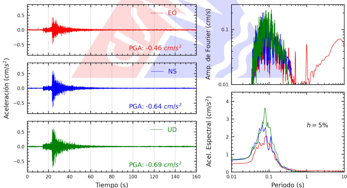
Figura A.12: Registros tiempo-historia, espectros de Fourier y de respuesta en las direcciones EO, NS y vertical de la estación SOVES. Sismo de Chilca, Cañete - Lima del 2025-10-15, 03:30:51 (Hora local)
