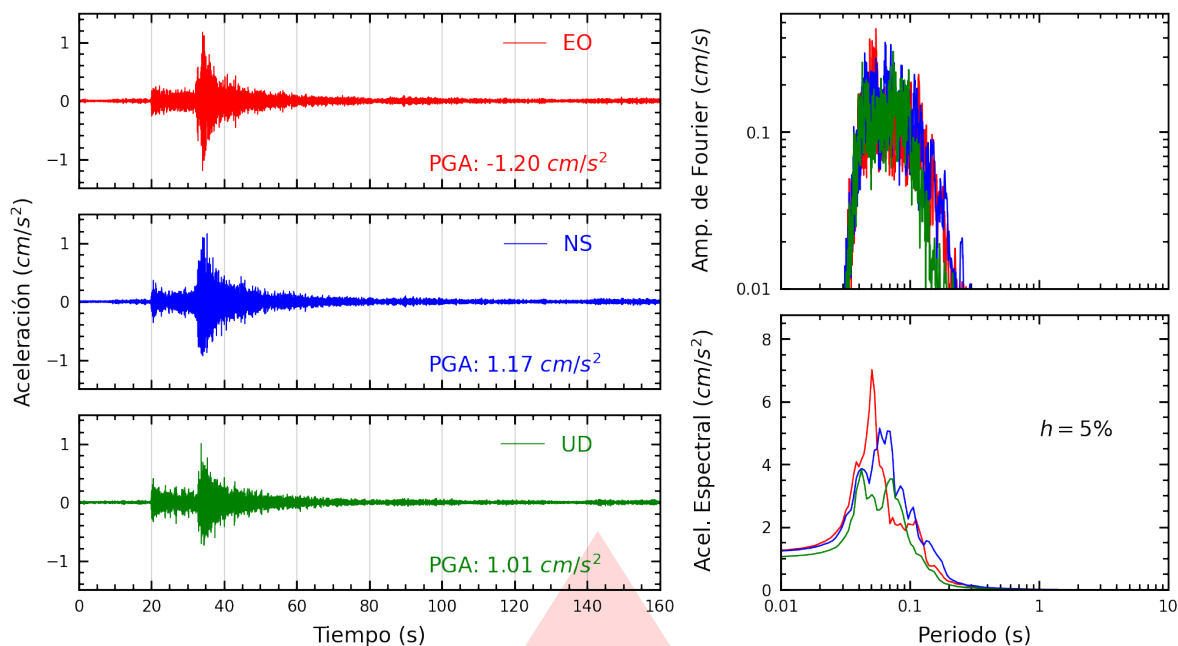
Figura A.5: Registros tiempo-historia, espectros de Fourier y de respuesta en las direcciones EO, NS y vertical de la estación SROSA. Sismo de Chilca, Cañete - Lima del 2025-10-15, 03:30:51 (Hora local)
