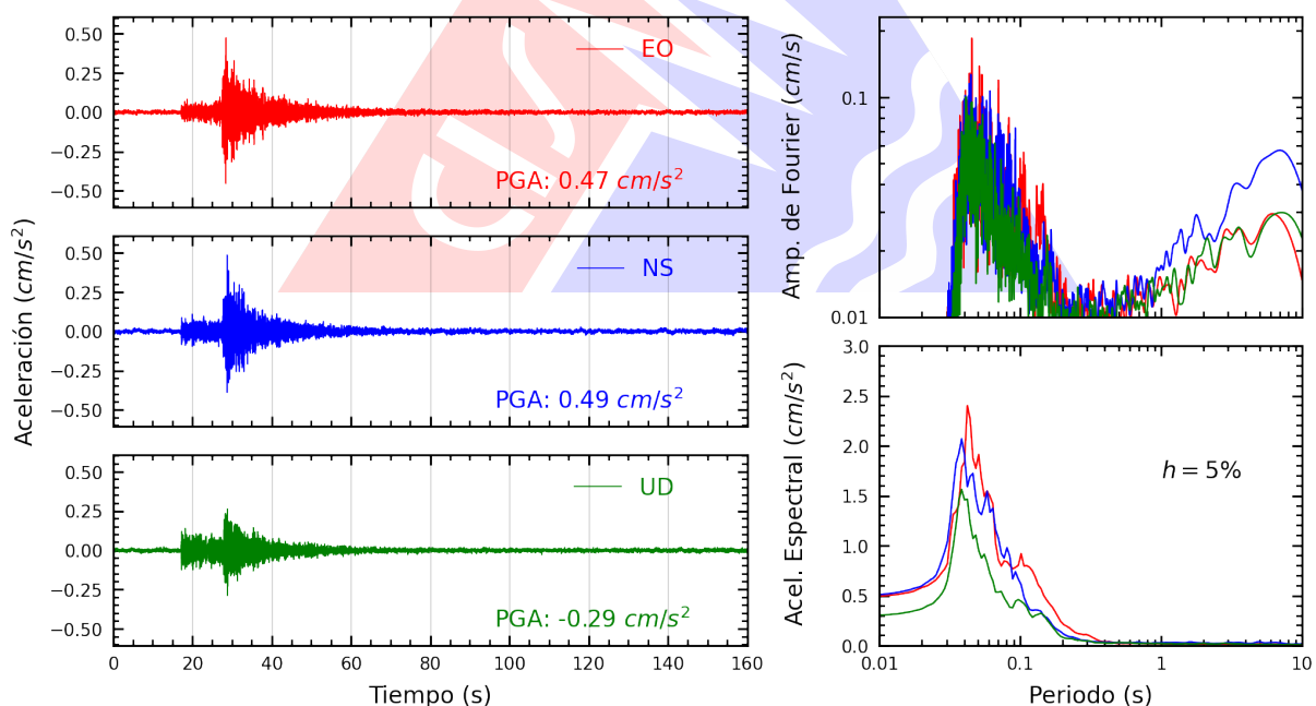
Figura A.18: Registros tiempo-historia, espectros de Fourier y de respuesta en las direcciones EO, NS y vertical de la estación SJLCE. Sismo de Chilca, Cañete - Lima del 2025-10-15, 03:30:51 (Hora local)
