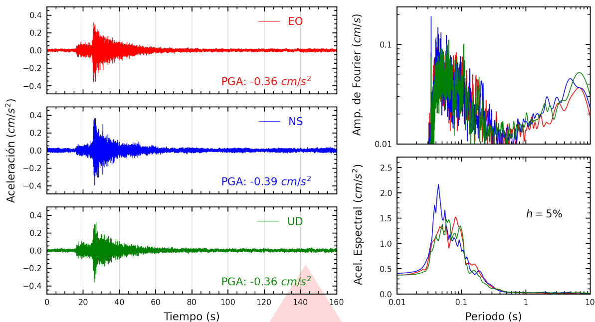
Figura A.19: Registros tiempo-historia, espectros de Fourier y de respuesta en las direcciones EO, NS y vertical de la estación USMP. Sismo de Chilca, Cañete - Lima del 2025-10-15, 03:30:51 (Hora local)
