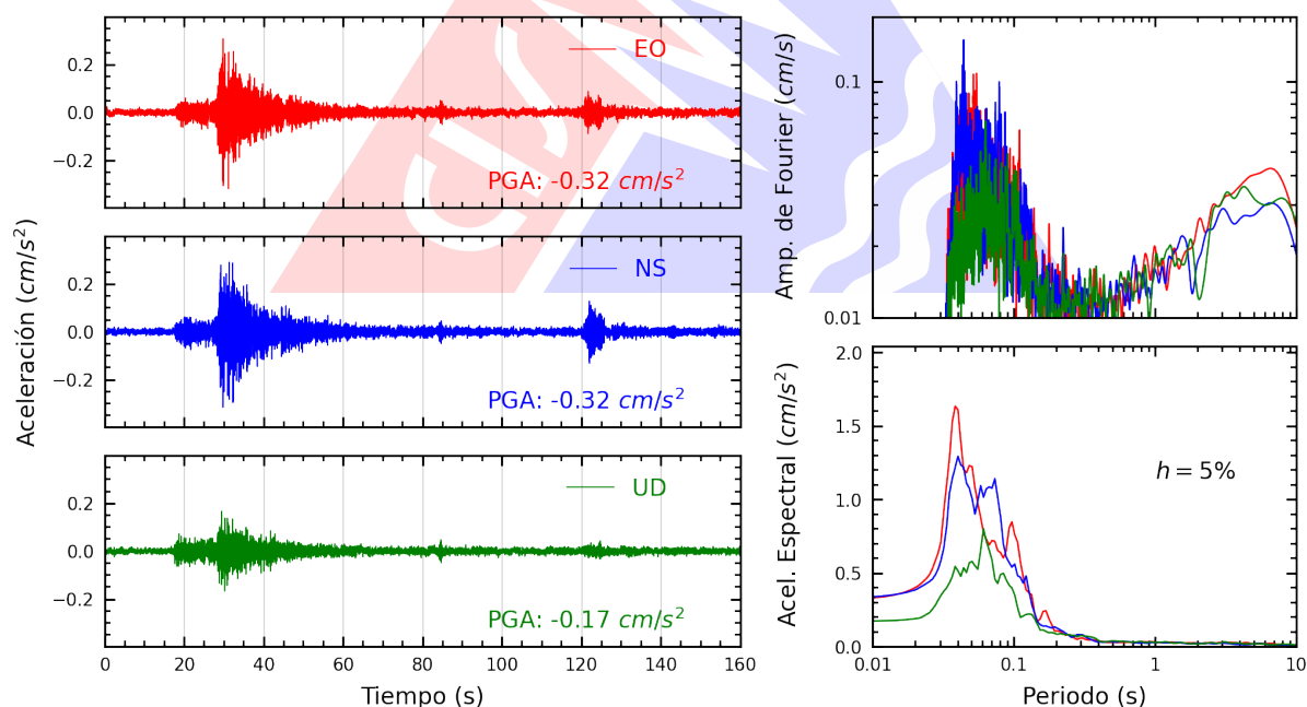
Figura A.26: Registros tiempo-historia, espectros de Fourier y de respuesta en las direcciones EO, NS y vertical de la estación COMAS. Sismo de Chilca, Cañete - Lima del 2025-10-15, 03:30:51 (Hora local)
