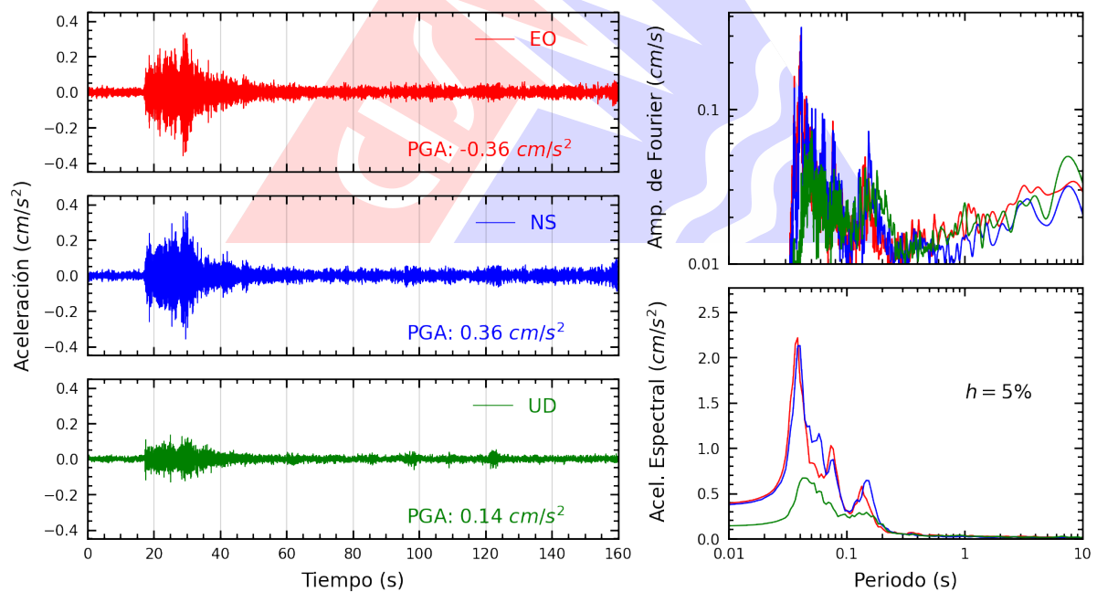
Figura A.22: Registros tiempo-historia, espectros de Fourier y de respuesta en las direcciones EO, NS y vertical de la estación DHNPE. Sismo de Chilca, Cañete - Lima del 2025-10-15, 03:30:51 (Hora local)
