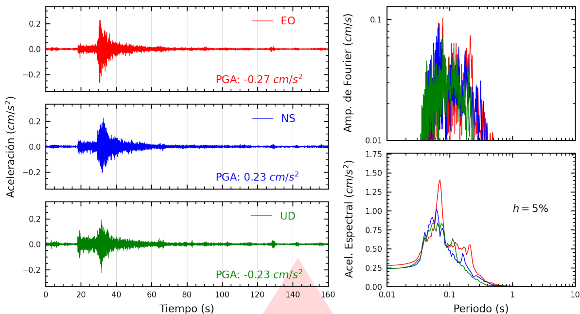
Figura A.27: Registros tiempo-historia, espectros de Fourier y de respuesta en las direcciones EO, NS y vertical de la estación VHAYA. Sismo de Chilca, Cañete - Lima del 2025-10-15, 03:30:51 (Hora local)
