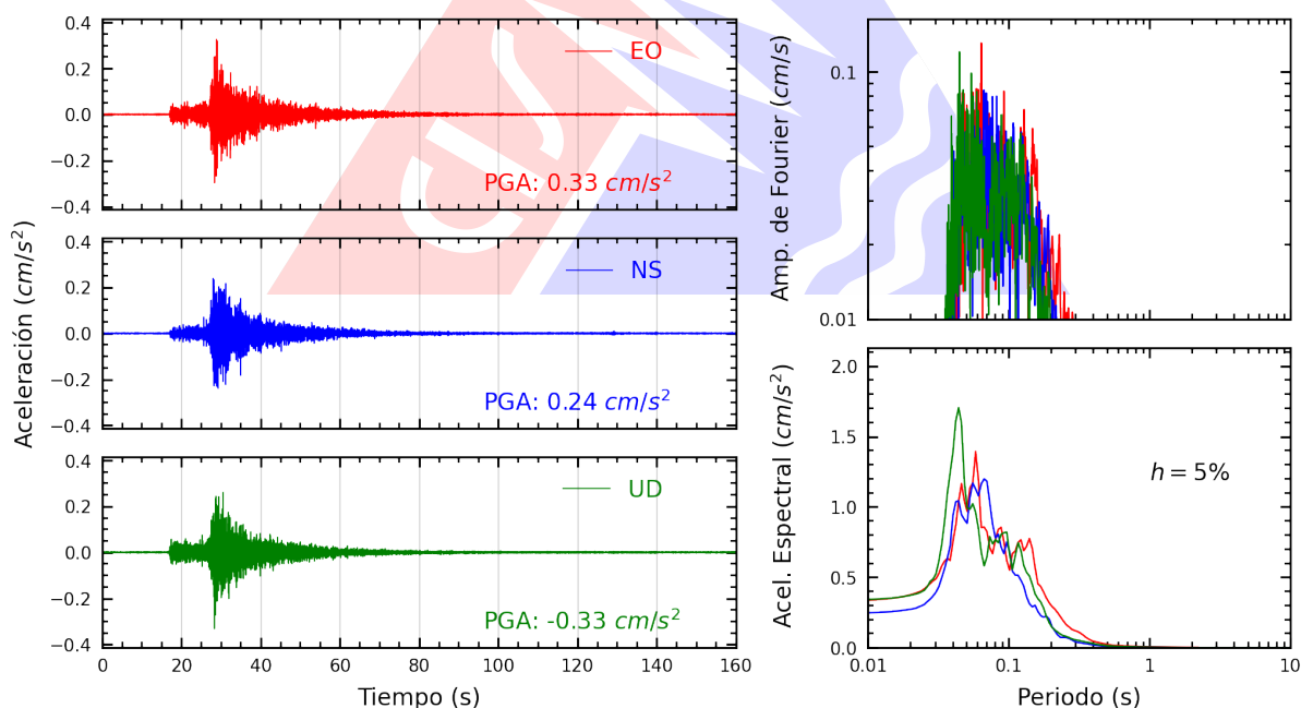
Figura A.24: Registros tiempo-historia, espectros de Fourier y de respuesta en las direcciones EO, NS y vertical de la estación JALV2. Sismo de Chilca, Cañete - Lima del 2025-10-15, 03:30:51 (Hora local)
