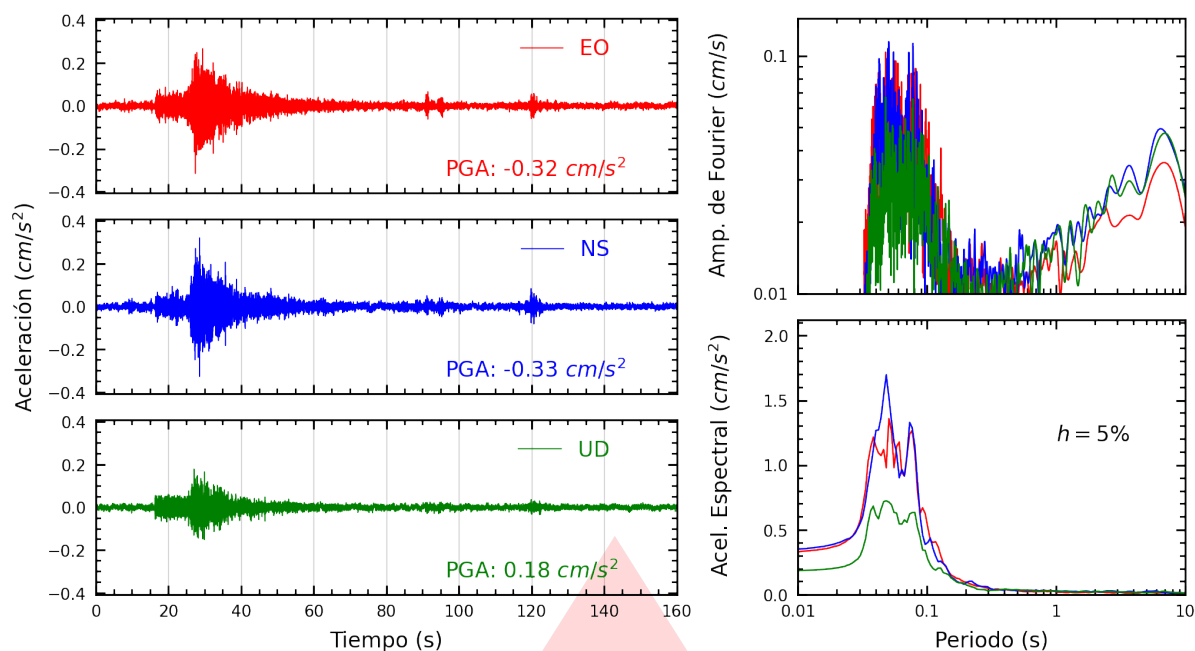
Figura A.25: Registros tiempo-historia, espectros de Fourier y de respuesta en las direcciones EO, NS y vertical de la estación CEPRE. Sismo de Chilca, Cañete - Lima del 2025-10-15, 03:30:51 (Hora local)
