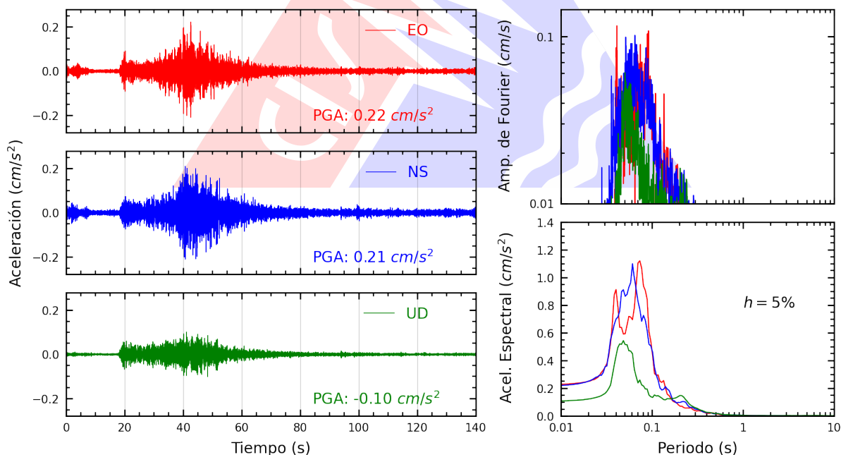
Figura A.2: Registros tiempo-historia, espectros de Fourier y de respuesta en las direcciones EO, NS y vertical de la estación UNAM. Sismo de Camaná, Camaná - Arequipa del 2025-10-22, 13:00:23 (Hora local)
