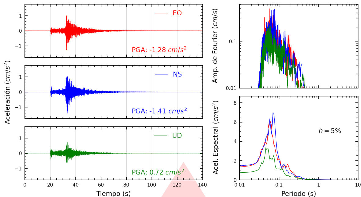
Figura A.1: Registros tiempo-historia, espectros de Fourier y de respuesta en las direcciones EO, NS y vertical de la estación UNSA2. Sismo de Camaná, Camaná - Arequipa del 2025-10-22, 13:00:23 (Hora local)
