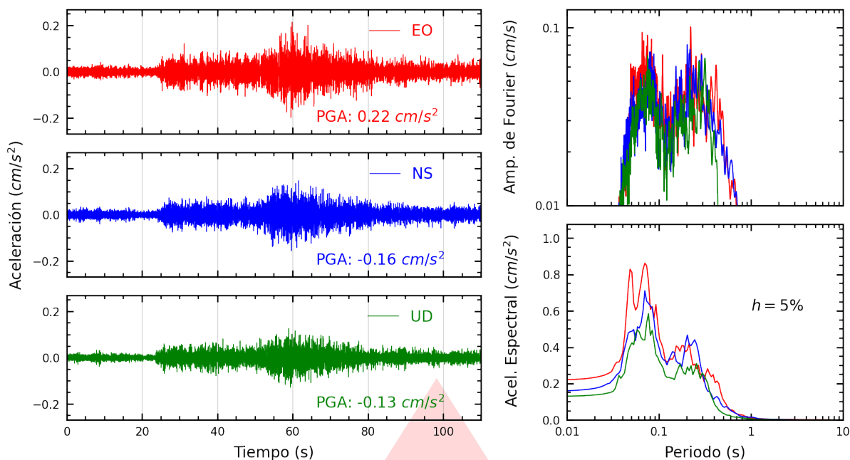
Figura A.5: Registros tiempo-historia, espectros de Fourier y de respuesta en las direcciones EO, NS y vertical de la estación UNTEL. Sismo de Colcabamba, Tayacaja - Huancavelica del 2025-11-04, 03:44:37 (Hora local)
