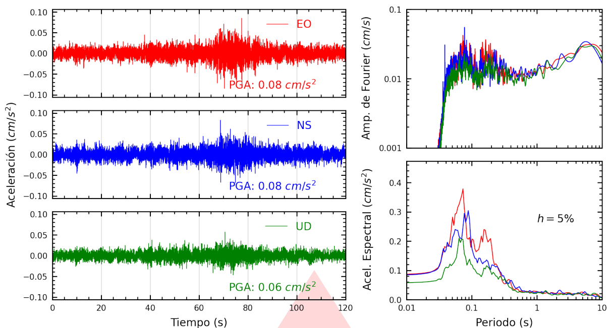
Figura A.21: Registros tiempo-historia, espectros de Fourier y de respuesta en las direcciones EO, NS y vertical de la estación FICPE. Sismo de Colcabamba, Tayacaja - Huancavelica del 2025-11-04, 03:44:37 (Hora local)
