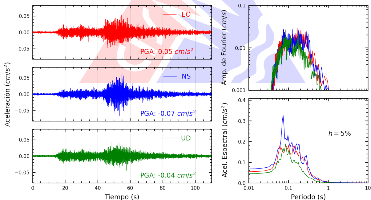
Figura A.24: Registros tiempo-historia, espectros de Fourier y de respuesta en las direcciones EO, NS y vertical de la estación JALV2. Sismo de Colcabamba, Tayacaja - Huancavelica del 2025-11-04, 03:44:37 (Hora local)
