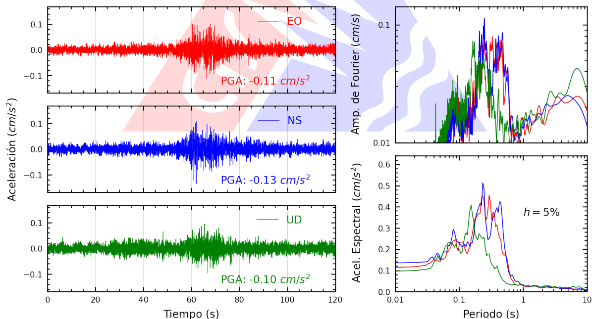
Figura A.12: Registros tiempo-historia, espectros de Fourier y de respuesta en las direcciones EO, NS y vertical de la estación MDPP. Sismo de Colcabamba, Tayacaja - Huancavelica del 2025-11-04, 03:44:37 (Hora local)
