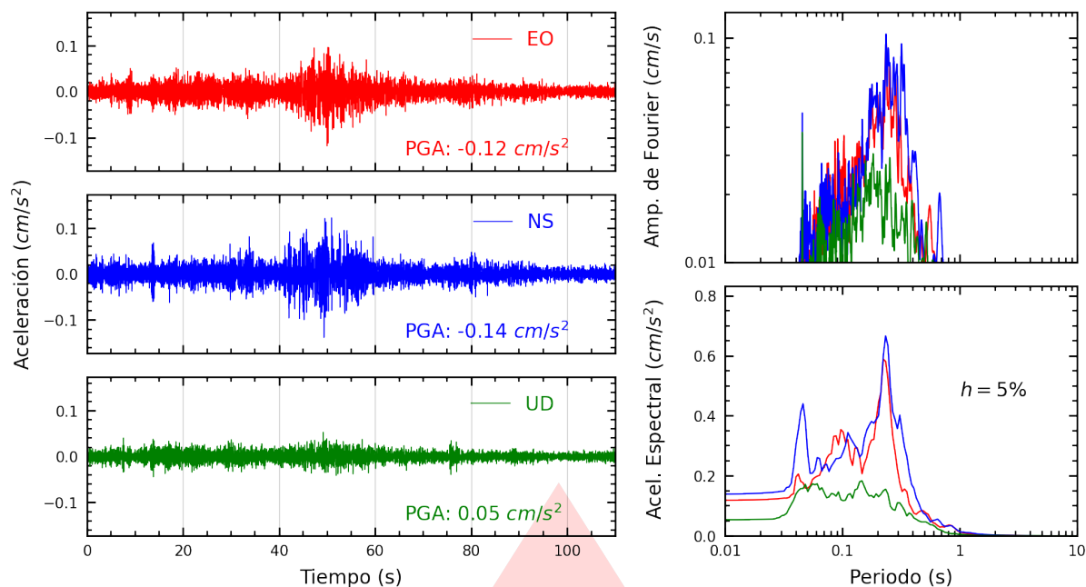
Figura A.11: Registros tiempo-historia, espectros de Fourier y de respuesta en las direcciones EO, NS y vertical de la estación BRIS2. Sismo de Colcabamba, Tayacaja - Huancavelica del 2025-11-04, 03:44:37 (Hora local)
