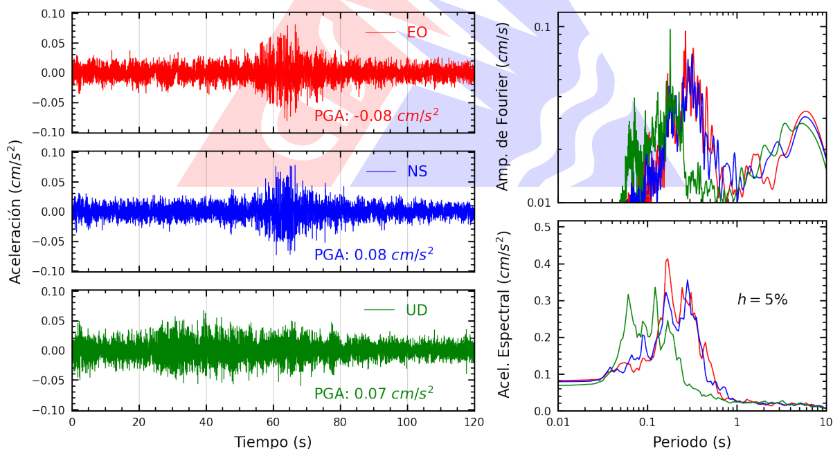
Figura A.22: Registros tiempo-historia, espectros de Fourier y de respuesta en las direcciones EO, NS y vertical de la estación ACAPU. Sismo de Colcabamba, Tayacaja - Huancavelica del 2025-11-04, 03:44:37 (Hora local)
