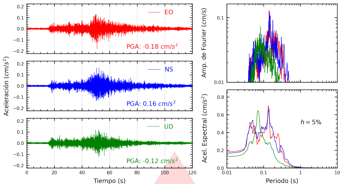
Figura A.7: Registros tiempo-historia, espectros de Fourier y de respuesta en las direcciones EO, NS y vertical de la estación CARAB. Sismo de Colcabamba, Tayacaja - Huancavelica del 2025-11-04, 03:44:37 (Hora local)
