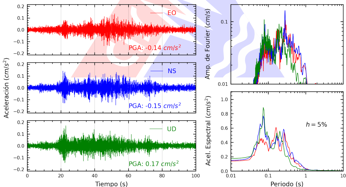
Figura A.8: Registros tiempo-historia, espectros de Fourier y de respuesta en las direcciones EO, NS y vertical de la estación UNICA. Sismo de Colcabamba, Tayacaja - Huancavelica del 2025-11-04, 03:44:37 (Hora local)
