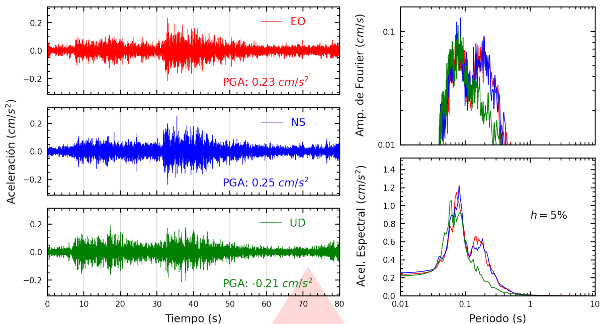
Figura A.3: Registros tiempo-historia, espectros de Fourier y de respuesta en las direcciones EO, NS y vertical de la estación ASIA. Sismo de Colcabamba, Tayacaja - Huancavelica del 2025-11-04, 03:44:37 (Hora local)
