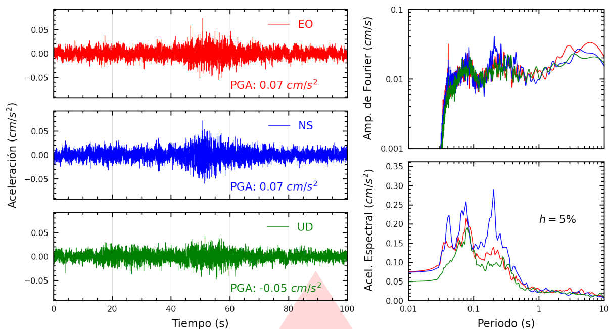
Figura A.23: Registros tiempo-historia, espectros de Fourier y de respuesta en las direcciones EO, NS y vertical de la estación COMAS. Sismo de Colcabamba, Tayacaja - Huancavelica del 2025-11-04, 03:44:37 (Hora local)
