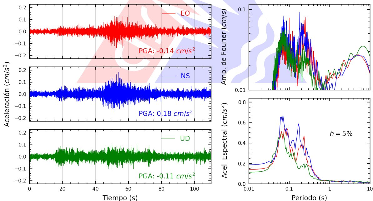
Figura A.6: Registros tiempo-historia, espectros de Fourier y de respuesta en las direcciones EO, NS y vertical de la estación SJLSC. Sismo de Colcabamba, Tayacaja - Huancavelica del 2025-11-04, 03:44:37 (Hora local)
