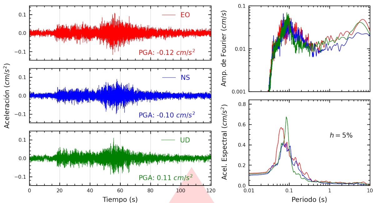
Figura A.15: Registros tiempo-historia, espectros de Fourier y de respuesta en las direcciones EO, NS y vertical de la estación AMORE. Sismo de Colcabamba, Tayacaja - Huancavelica del 2025-11-04, 03:44:37 (Hora local)
