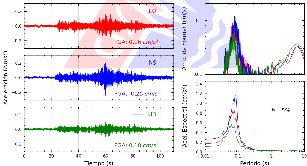
Figura A.4: Registros tiempo-historia, espectros de Fourier y de respuesta en las direcciones EO, NS y vertical de la estación JOSEO. Sismo de Colcabamba, Tayacaja - Huancavelica del 2025-11-04, 03:44:37 (Hora local)
