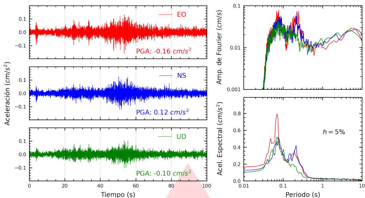
Figura A.9: Registros tiempo-historia, espectros de Fourier y de respuesta en las direcciones EO, NS y vertical de la estación INDEP. Sismo de Colcabamba, Tayacaja - Huancavelica del 2025-11-04, 03:44:37 (Hora local)
