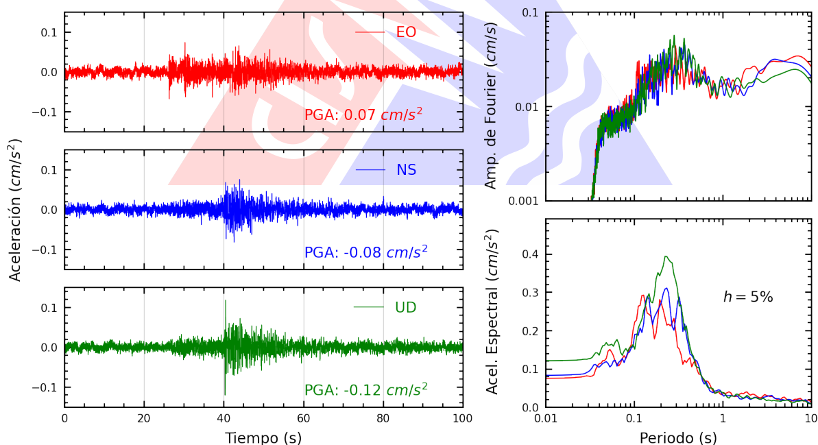
Figura A.14: Registros tiempo-historia, espectros de Fourier y de respuesta en las direcciones EO, NS y vertical de la estación UNSCH. Sismo de Colcabamba, Tayacaja - Huancavelica del 2025-11-04, 03:44:37 (Hora local)
