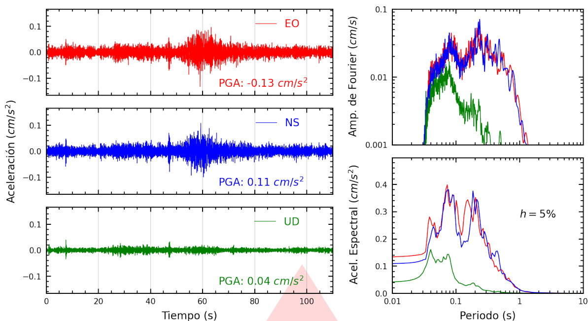
Figura A.13: Registros tiempo-historia, espectros de Fourier y de respuesta en las direcciones EO, NS y vertical de la estación UCVAT. Sismo de Colcabamba, Tayacaja - Huancavelica del 2025-11-04, 03:44:37 (Hora local)
