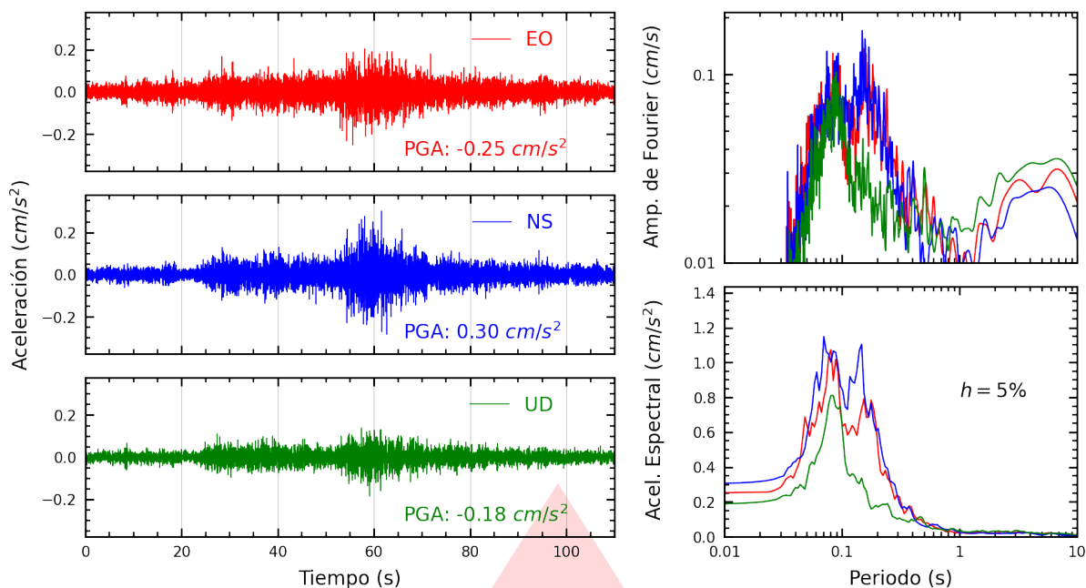
Figura A.1: Registros tiempo-historia, espectros de Fourier y de respuesta en las direcciones EO, NS y vertical de la estación USILM. Sismo de Colcabamba, Tayacaja - Huancavelica del 2025-11-04, 03:44:37 (Hora local)
