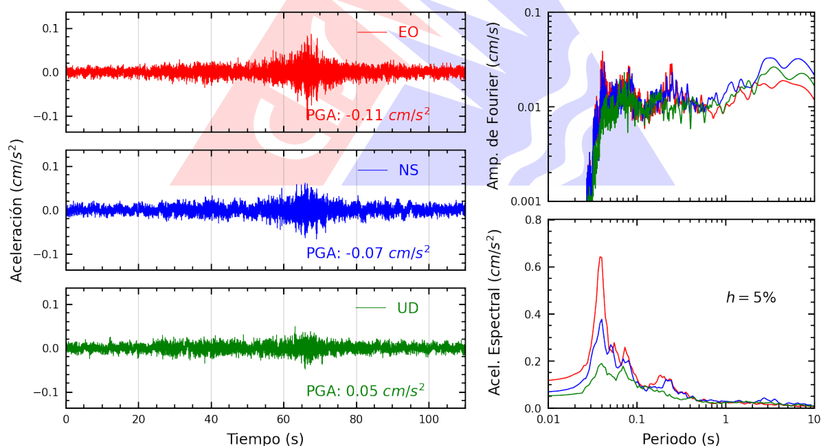
Figura A.18: Registros tiempo-historia, espectros de Fourier y de respuesta en las direcciones EO, NS y vertical de la estación CEPRE. Sismo de Colcabamba, Tayacaja - Huancavelica del 2025-11-04, 03:44:37 (Hora local)
