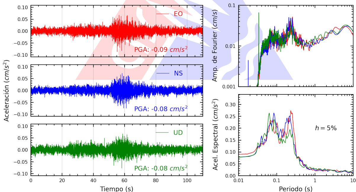
Figura A.20: Registros tiempo-historia, espectros de Fourier y de respuesta en las direcciones EO, NS y vertical de la estación USMP. Sismo de Colcabamba, Tayacaja - Huancavelica del 2025-11-04, 03:44:37 (Hora local)
