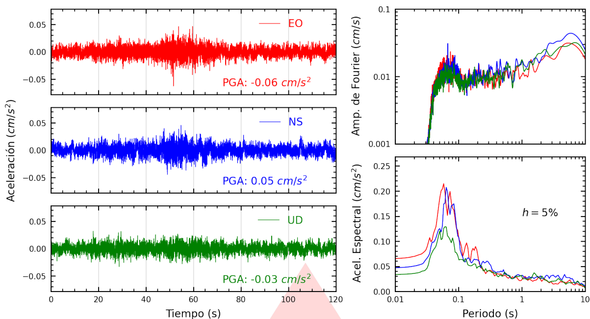
Figura A.25: Registros tiempo-historia, espectros de Fourier y de respuesta en las direcciones EO, NS y vertical de la estación UCSS. Sismo de Colcabamba, Tayacaja - Huancavelica del 2025-11-04, 03:44:37 (Hora local)
