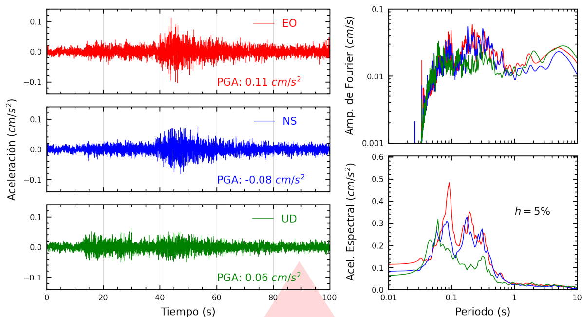
Figura A.17: Registros tiempo-historia, espectros de Fourier y de respuesta en las direcciones EO, NS y vertical de la estación USILP. Sismo de Colcabamba, Tayacaja - Huancavelica del 2025-11-04, 03:44:37 (Hora local)
