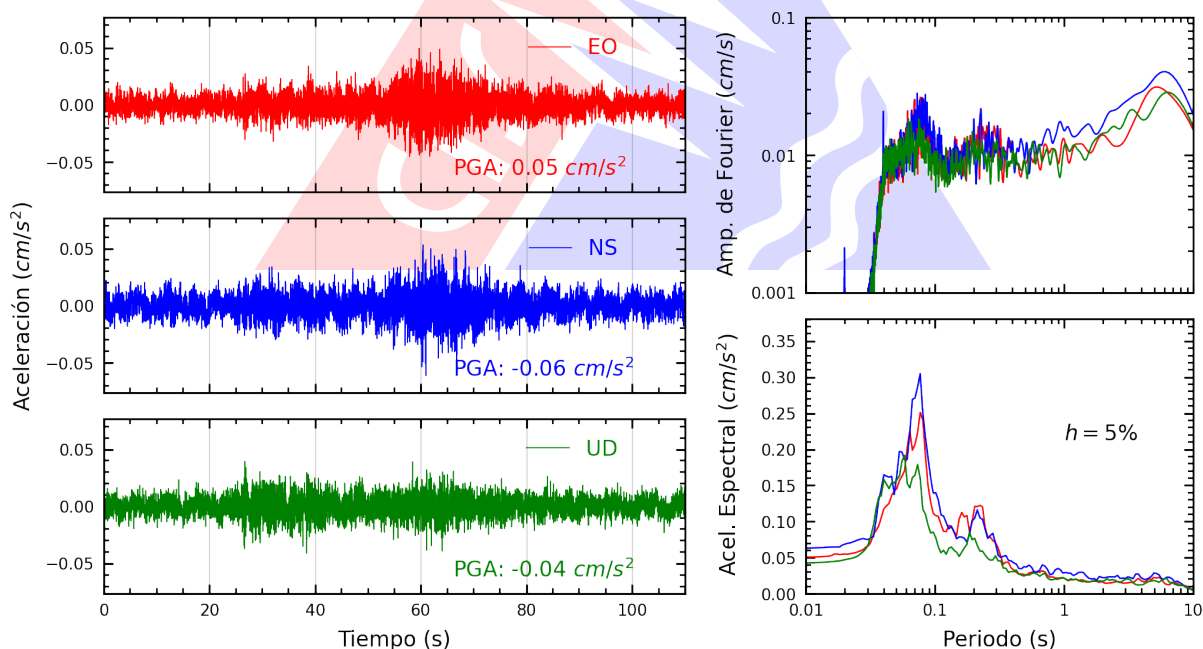
Figura A.26: Registros tiempo-historia, espectros de Fourier y de respuesta en las direcciones EO, NS y vertical de la estación SJLCE. Sismo de Colcabamba, Tayacaja - Huancavelica del 2025-11-04, 03:44:37 (Hora local)
