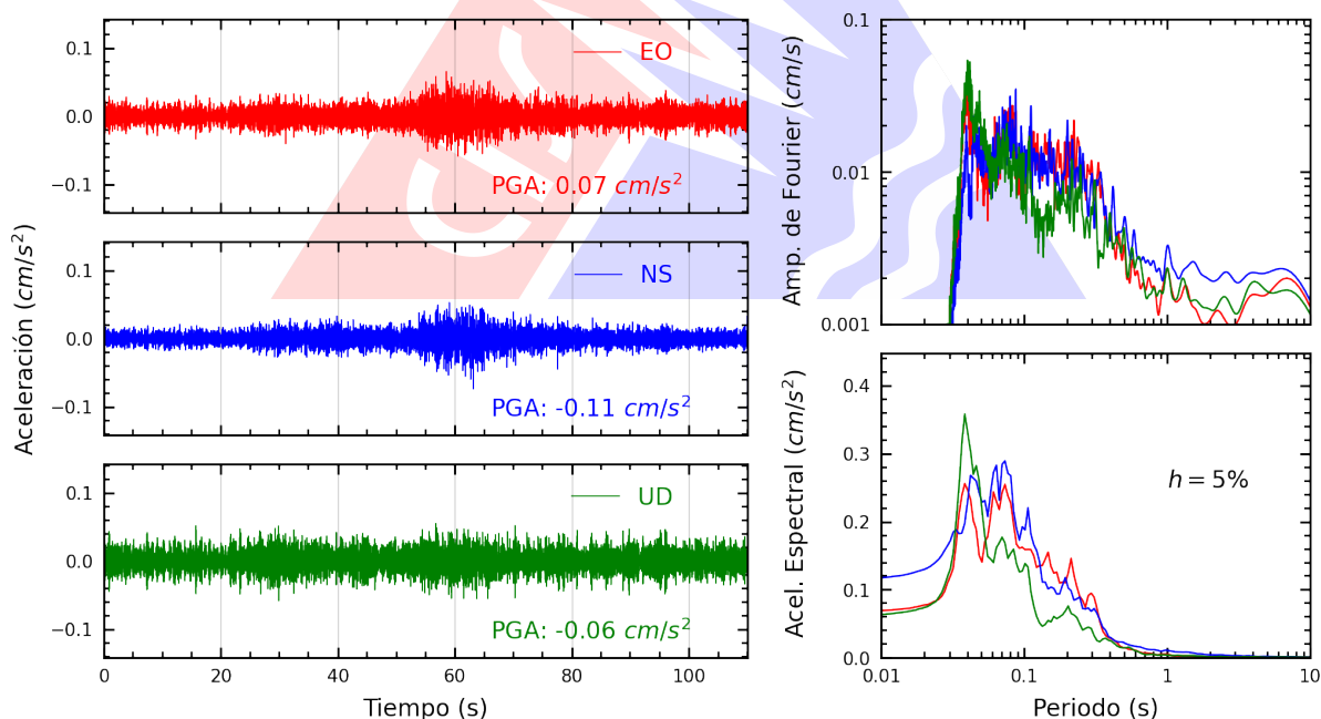
Figura A.16: Registros tiempo-historia, espectros de Fourier y de respuesta en las direcciones EO, NS y vertical de la estación ATARJ. Sismo de Colcabamba, Tayacaja - Huancavelica del 2025-11-04, 03:44:37 (Hora local)
