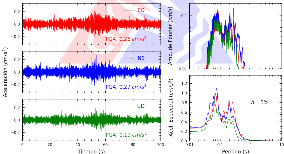
Figura A.2: Registros tiempo-historia, espectros de Fourier y de respuesta en las direcciones EO, NS y vertical de la estación PHERM. Sismo de Colcabamba, Tayacaja - Huancavelica del 2025-11-04, 03:44:37 (Hora local)
