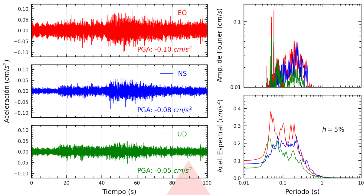
Figura A.19: Registros tiempo-historia, espectros de Fourier y de respuesta en las direcciones EO, NS y vertical de la estación SOBAR. Sismo de Colcabamba, Tayacaja - Huancavelica del 2025-11-04, 03:44:37 (Hora local)
