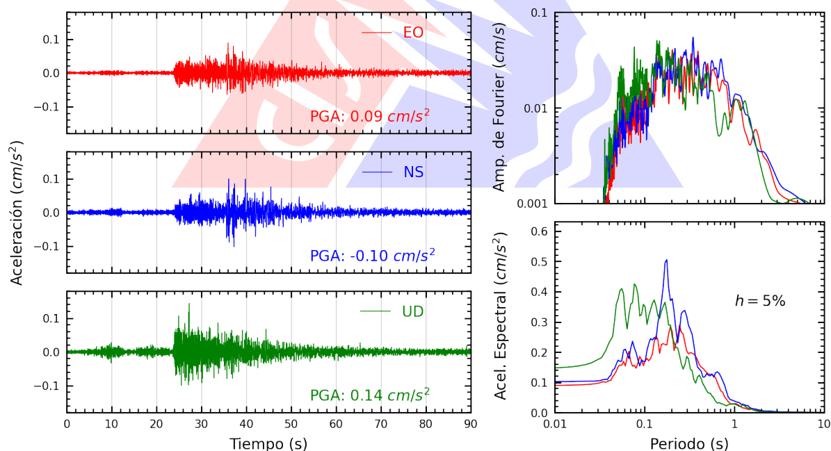
Figura A.10: Registros tiempo-historia, espectros de Fourier y de respuesta en las direcciones EO, NS y vertical de la estación SCHYO. Sismo de Colcabamba, Tayacaja - Huancavelica del 2025-11-04, 03:44:37 (Hora local)
