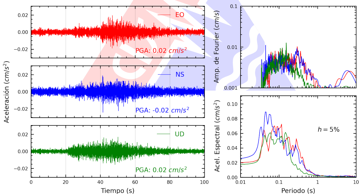
Figura A.2: Registros tiempo-historia, espectros de Fourier y de respuesta en las direcciones EO, NS y vertical de la estación UPAOP. Sismo de Tumbes, Tumbes - Tumbes del 2025-11-04, 03:49:35 (Hora local)
