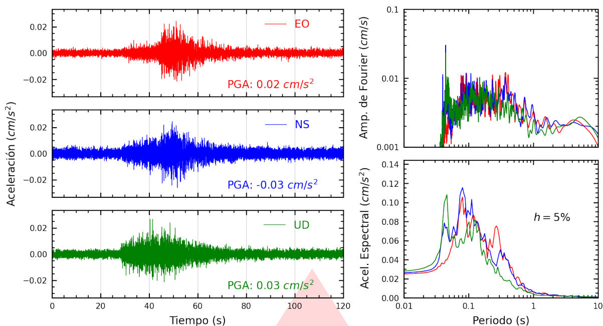
Figura A.1: Registros tiempo-historia, espectros de Fourier y de respuesta en las direcciones EO, NS y vertical de la estación UNF. Sismo de Tumbes, Tumbes - Tumbes del 2025-11-04, 03:49:35 (Hora local)
