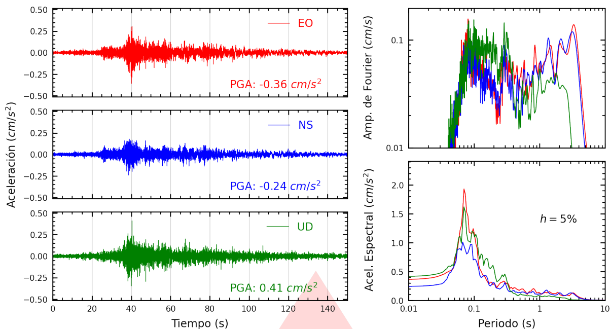
Figura A.5: Registros tiempo-historia, espectros de Fourier y de respuesta en las direcciones EO, NS y vertical de la estación UANCV. Sismo de Arequipa, Arequipa - Arequipa del 2025-11-11, 02:45:56 (Hora local)
