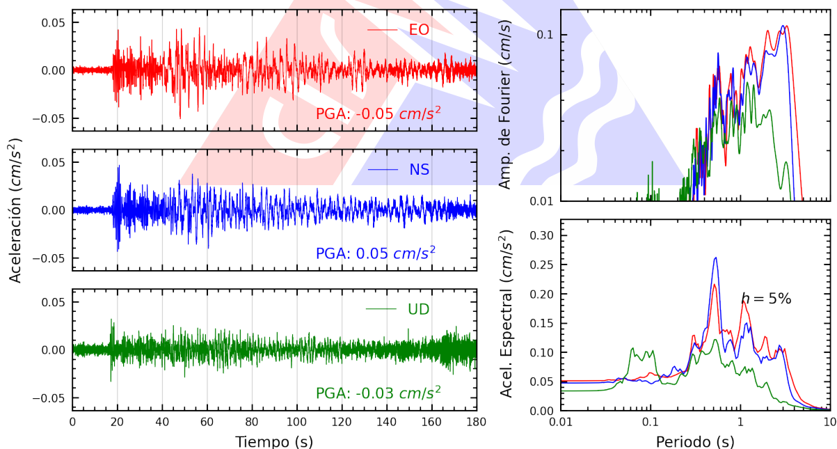
Figura A.8: Registros tiempo-historia, espectros de Fourier y de respuesta en las direcciones EO, NS y vertical de la estación UNAJ. Sismo de Arequipa, Arequipa - Arequipa del 2025-11-11, 02:45:56 (Hora local)
