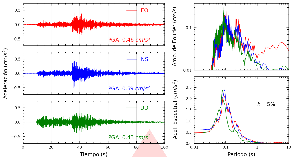
Figura A.3: Registros tiempo-historia, espectros de Fourier y de respuesta en las direcciones EO, NS y vertical de la estación UJBG3. Sismo de Arequipa, Arequipa - Arequipa del 2025-11-11, 02:45:56 (Hora local)
