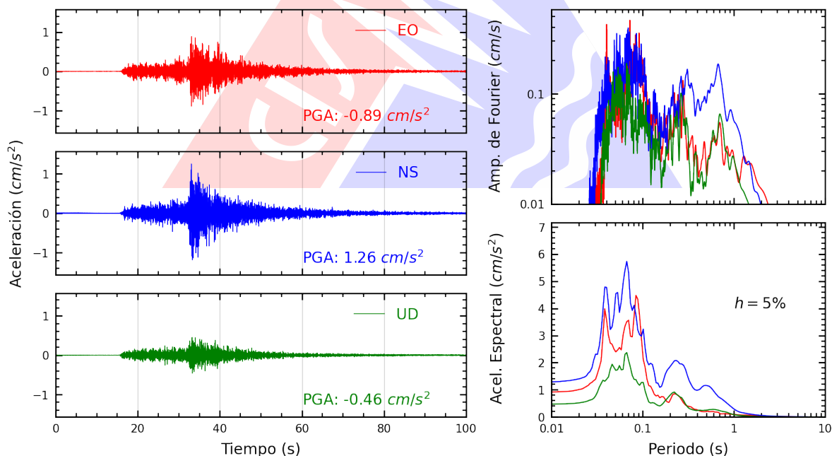
Figura A.2: Registros tiempo-historia, espectros de Fourier y de respuesta en las direcciones EO, NS y vertical de la estación UNAM. Sismo de Arequipa, Arequipa - Arequipa del 2025-11-11, 02:45:56 (Hora local)
