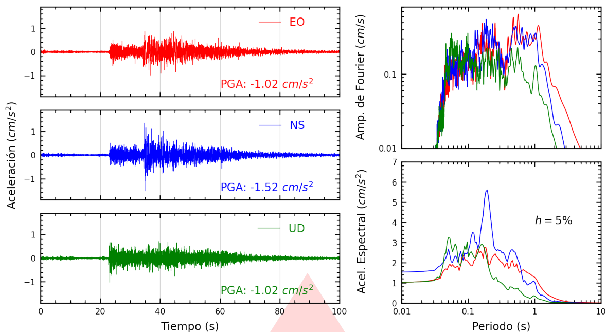
Figura A.1: Registros tiempo-historia, espectros de Fourier y de respuesta en las direcciones EO, NS y vertical de la estación SCAR2. Sismo de Arequipa, Arequipa - Arequipa del 2025-11-11, 02:45:56 (Hora local)
