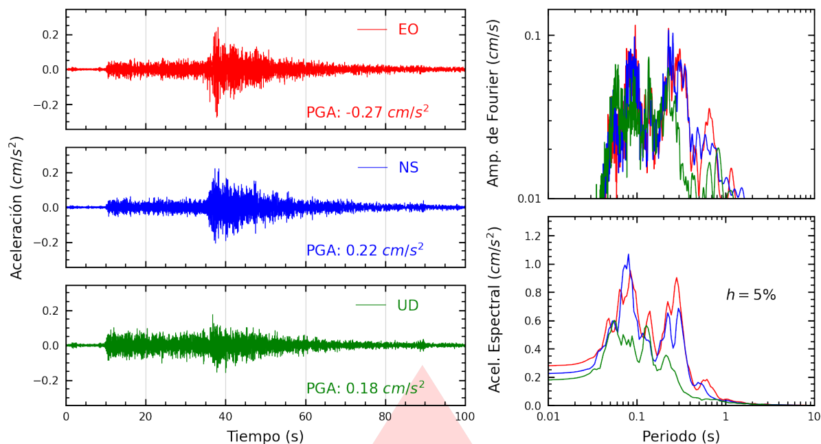
Figura A.7: Registros tiempo-historia, espectros de Fourier y de respuesta en las direcciones EO, NS y vertical de la estación UJBG2. Sismo de Arequipa, Arequipa - Arequipa del 2025-11-11, 02:45:56 (Hora local)
