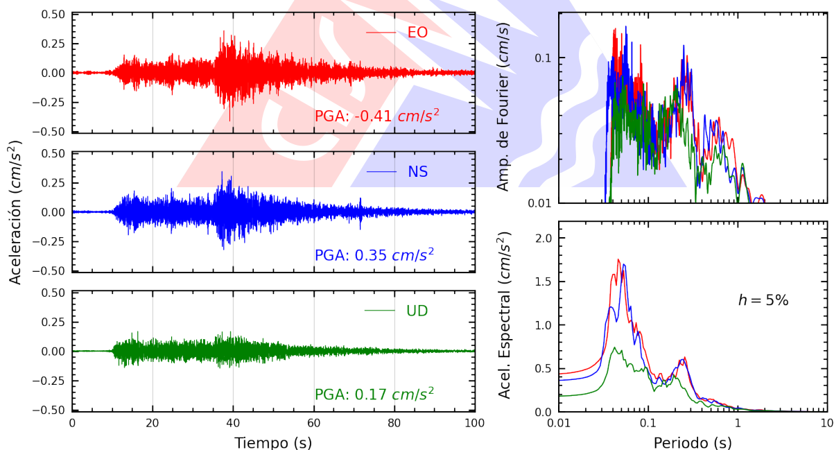
Figura A.4: Registros tiempo-historia, espectros de Fourier y de respuesta en las direcciones EO, NS y vertical de la estación UPTAC. Sismo de Arequipa, Arequipa - Arequipa del 2025-11-11, 02:45:56 (Hora local)
