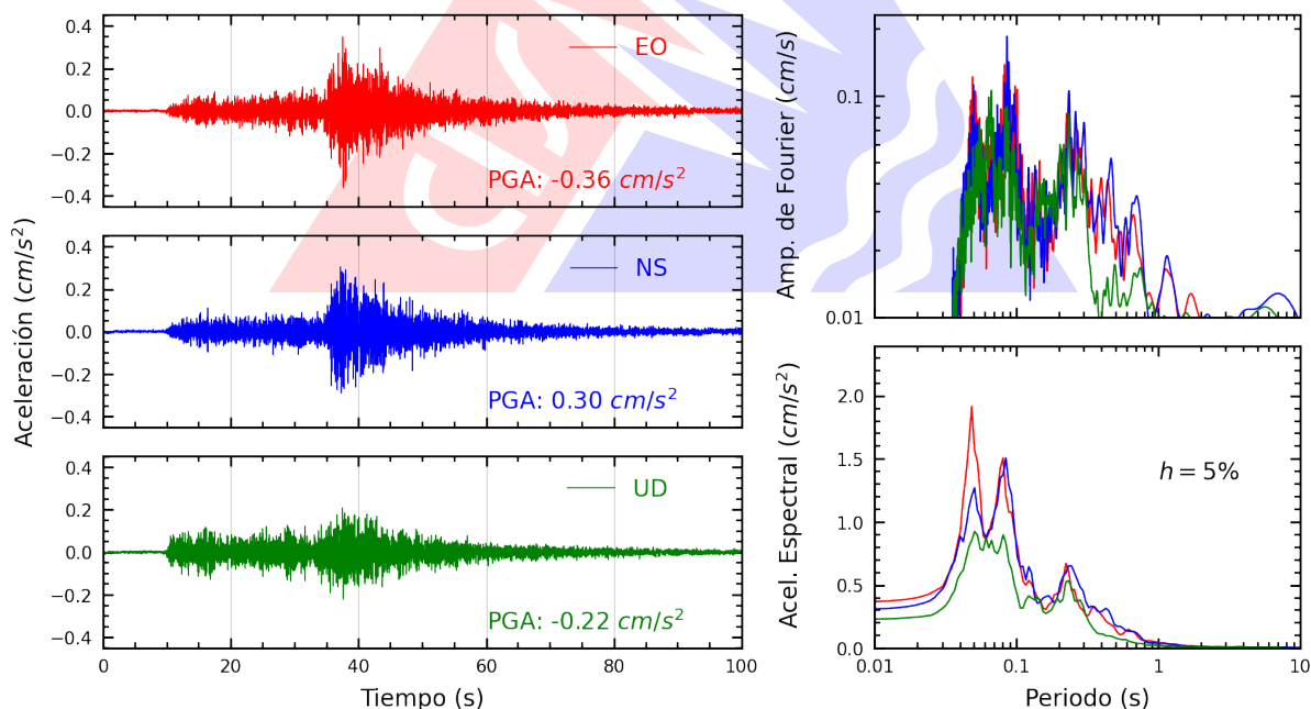
Figura A.6: Registros tiempo-historia, espectros de Fourier y de respuesta en las direcciones EO, NS y vertical de la estación CREY. Sismo de Arequipa, Arequipa - Arequipa del 2025-11-11, 02:45:56 (Hora local)
