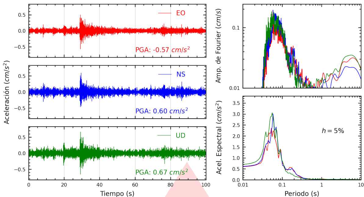
Figura A.7: Registros tiempo-historia, espectros de Fourier y de respuesta en las direcciones EO, NS y vertical de la estación SJLSC. Sismo de Bellavista, Provincia Constitucional del Callao del 2025-11-11, 09:20:16 (Hora local)
