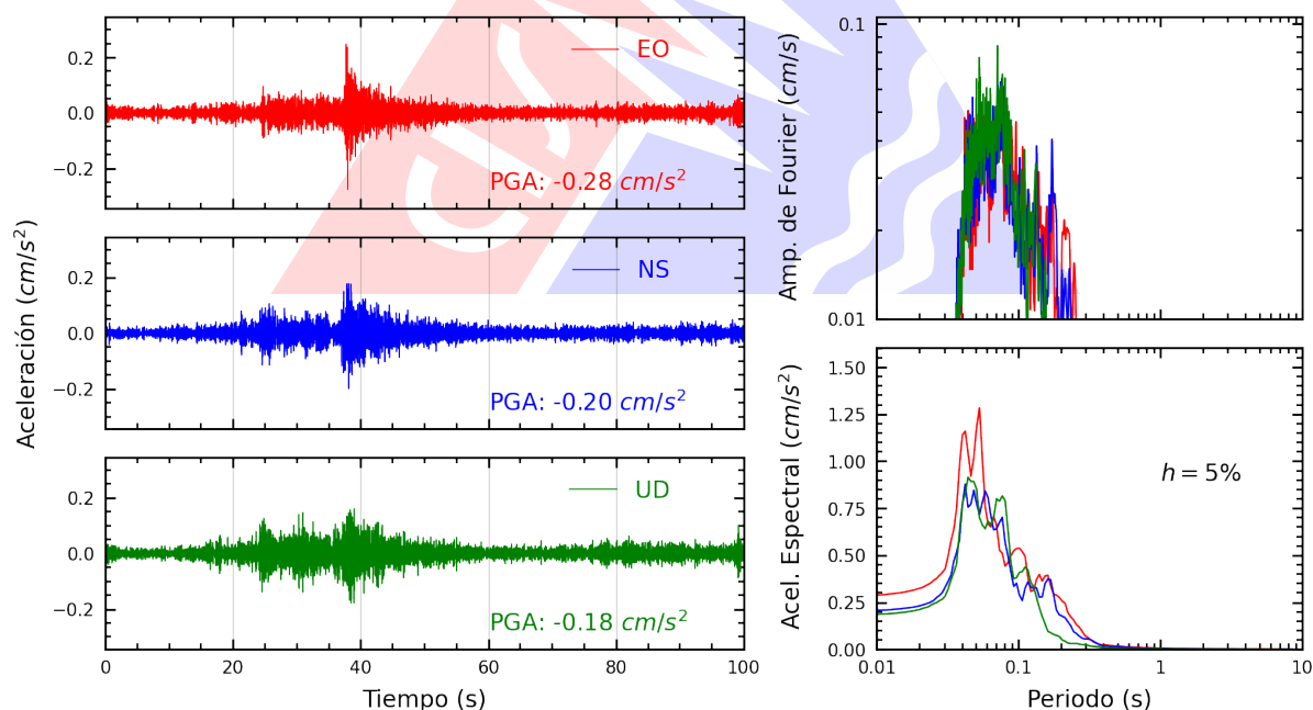
Figura A.20: Registros tiempo-historia, espectros de Fourier y de respuesta en las direcciones EO, NS y vertical de la estación ASIA. Sismo de Bellavista, Provincia Constitucional del Callao del 2025-11-11, 09:20:16 (Hora local)
