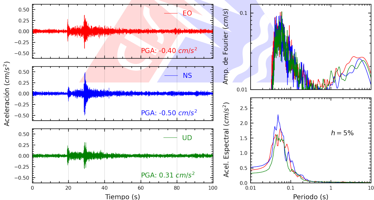
Figura A.10: Registros tiempo-historia, espectros de Fourier y de respuesta en las direcciones EO, NS y vertical de la estación IMCA. Sismo de Bellavista, Provincia Constitucional del Callao del 2025-11-11, 09:20:16 (Hora local)
