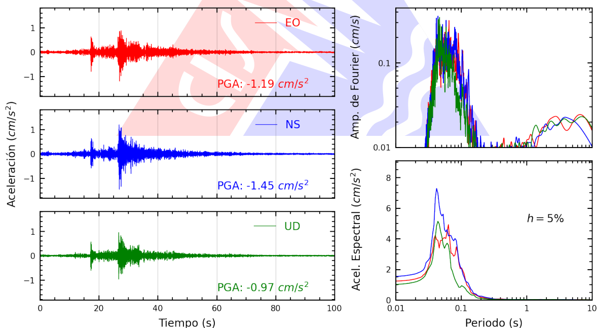
Figura A.2: Registros tiempo-historia, espectros de Fourier y de respuesta en las direcciones EO, NS y vertical de la estación JOSEO. Sismo de Bellavista, Provincia Constitucional del Callao del 2025-11-11, 09:20:16 (Hora local)
