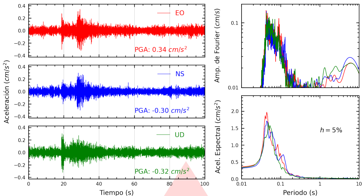
Figura A.17: Registros tiempo-historia, espectros de Fourier y de respuesta en las direcciones EO, NS y vertical de la estación URPE. Sismo de Bellavista, Provincia Constitucional del Callao del 2025-11-11, 09:20:16 (Hora local)
