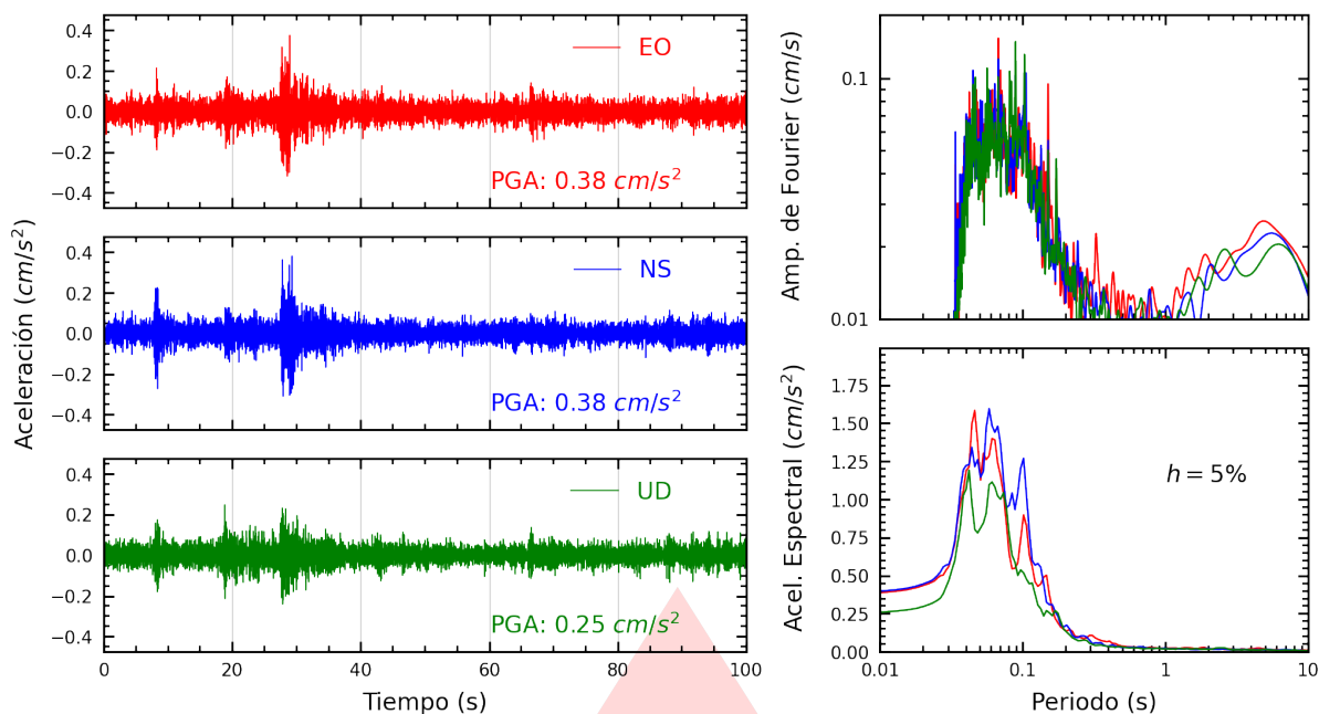
Figura A.15: Registros tiempo-historia, espectros de Fourier y de respuesta en las direcciones EO, NS y vertical de la estación MADRE. Sismo de Bellavista, Provincia Constitucional del Callao del 2025-11-11, 09:20:16 (Hora local)
