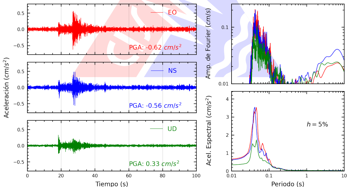
Figura A.8: Registros tiempo-historia, espectros de Fourier y de respuesta en las direcciones EO, NS y vertical de la estación CEPRE. Sismo de Bellavista, Provincia Constitucional del Callao del 2025-11-11, 09:20:16 (Hora local)
