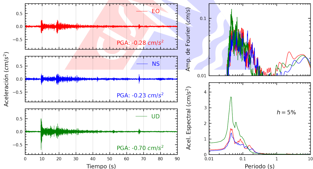
Figura A.6: Registros tiempo-historia, espectros de Fourier y de respuesta en las direcciones EO, NS y vertical de la estación USILP. Sismo de Bellavista, Provincia Constitucional del Callao del 2025-11-11, 09:20:16 (Hora local)
