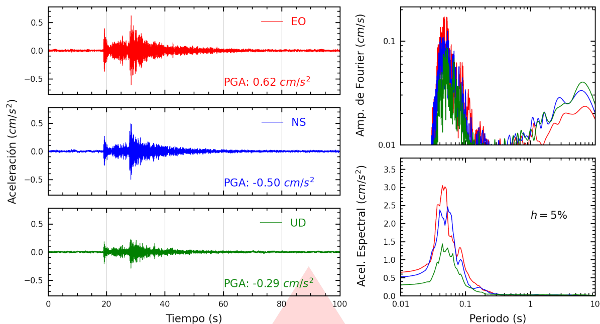
Figura A.9: Registros tiempo-historia, espectros de Fourier y de respuesta en las direcciones EO, NS y vertical de la estación UCSS. Sismo de Bellavista, Provincia Constitucional del Callao del 2025-11-11, 09:20:16 (Hora local)
