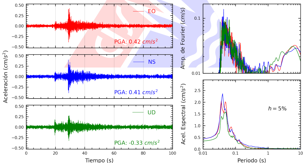
Figura A.14: Registros tiempo-historia, espectros de Fourier y de respuesta en las direcciones EO, NS y vertical de la estación USMP. Sismo de Bellavista, Provincia Constitucional del Callao del 2025-11-11, 09:20:16 (Hora local)
