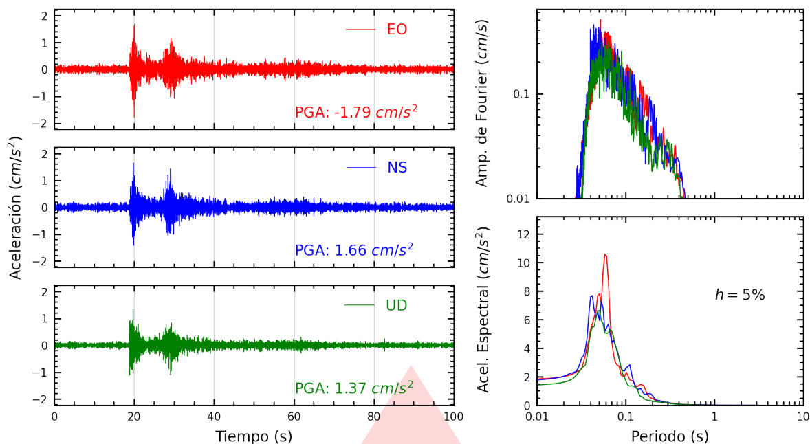
Figura A.1: Registros tiempo-historia, espectros de Fourier y de respuesta en las direcciones EO, NS y vertical de la estación UNTEL. Sismo de Bellavista, Provincia Constitucional del Callao del 2025-11-11, 09:20:16 (Hora local)
