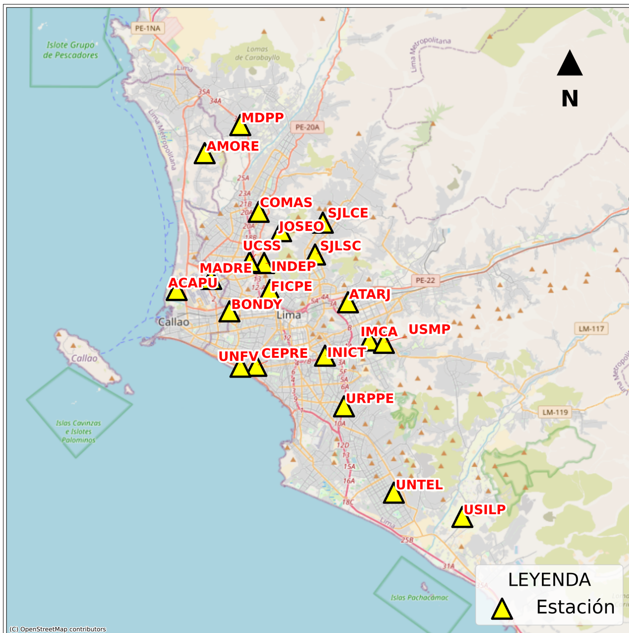
Figura 3: Mapa de ubicación de la(s) estación(es) acelerográfica(s) en Lima Metropolitana correspondiente(s) al Sismo de Bellavista, Provincia Constitucional del Callao del 11 de noviembre de 2025 a las 09:20:16 (hora local)
