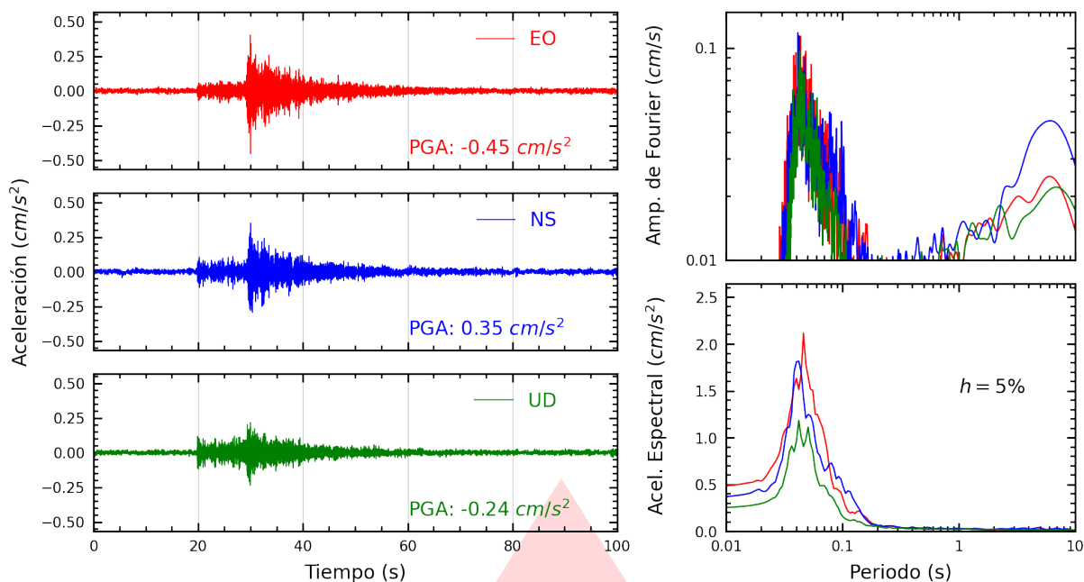
Figura A.11: Registros tiempo-historia, espectros de Fourier y de respuesta en las direcciones EO, NS y vertical de la estación SJLCE. Sismo de Bellavista, Provincia Constitucional del Callao del 2025-11-11, 09:20:16 (Hora local)
