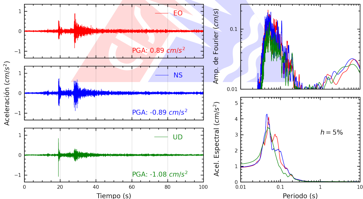
Figura A.4: Registros tiempo-historia, espectros de Fourier y de respuesta en las direcciones EO, NS y vertical de la estación FICPE. Sismo de Bellavista, Provincia Constitucional del Callao del 2025-11-11, 09:20:16 (Hora local)
