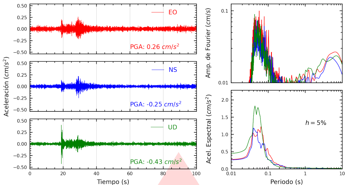
Figura A.13: Registros tiempo-historia, espectros de Fourier y de respuesta en las direcciones EO, NS y vertical de la estación INICT. Sismo de Bellavista, Provincia Constitucional del Callao del 2025-11-11, 09:20:16 (Hora local)
