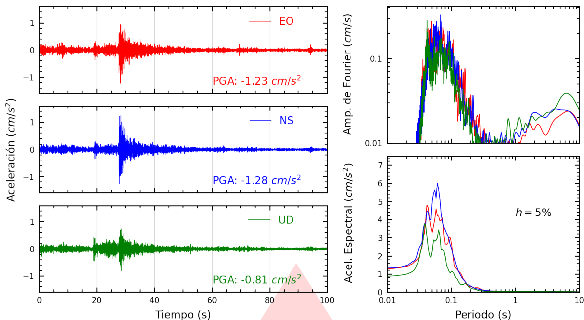
Figura A.3: Registros tiempo-historia, espectros de Fourier y de respuesta en las direcciones EO, NS y vertical de la estación INDEP. Sismo de Bellavista, Provincia Constitucional del Callao del 2025-11-11, 09:20:16 (Hora local)
