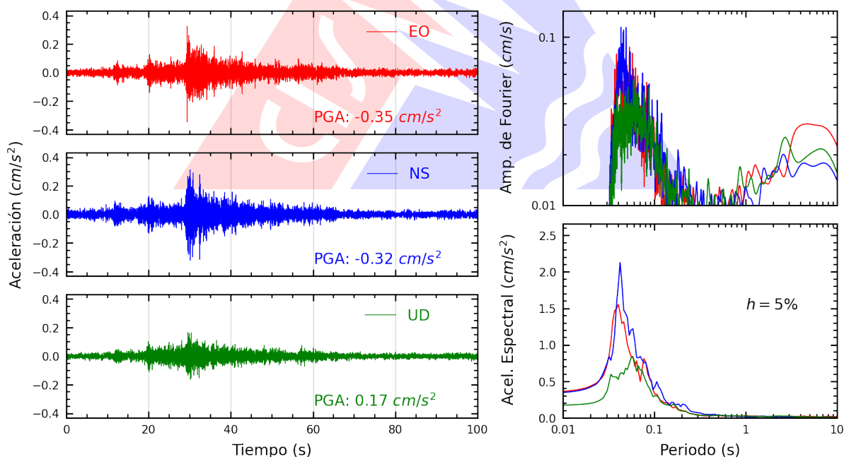
Figura A.16: Registros tiempo-historia, espectros de Fourier y de respuesta en las direcciones EO, NS y vertical de la estación COMAS. Sismo de Bellavista, Provincia Constitucional del Callao del 2025-11-11, 09:20:16 (Hora local)
