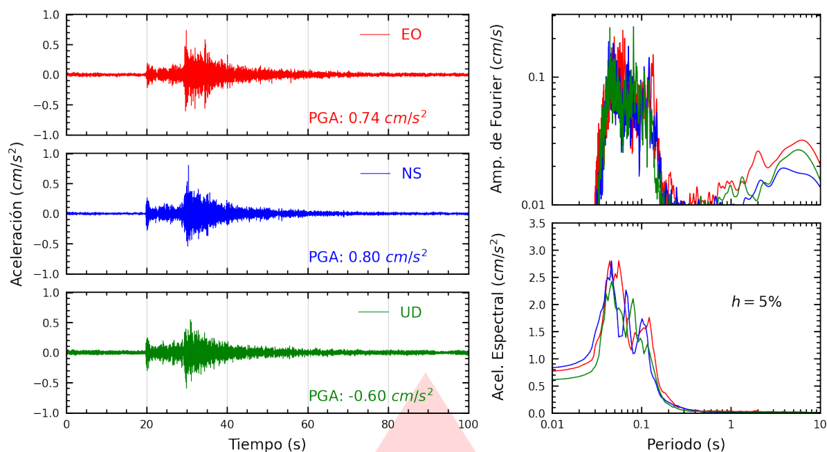
Figura A.5: Registros tiempo-historia, espectros de Fourier y de respuesta en las direcciones EO, NS y vertical de la estación AMORE. Sismo de Bellavista, Provincia Constitucional del Callao del 2025-11-11, 09:20:16 (Hora local)
