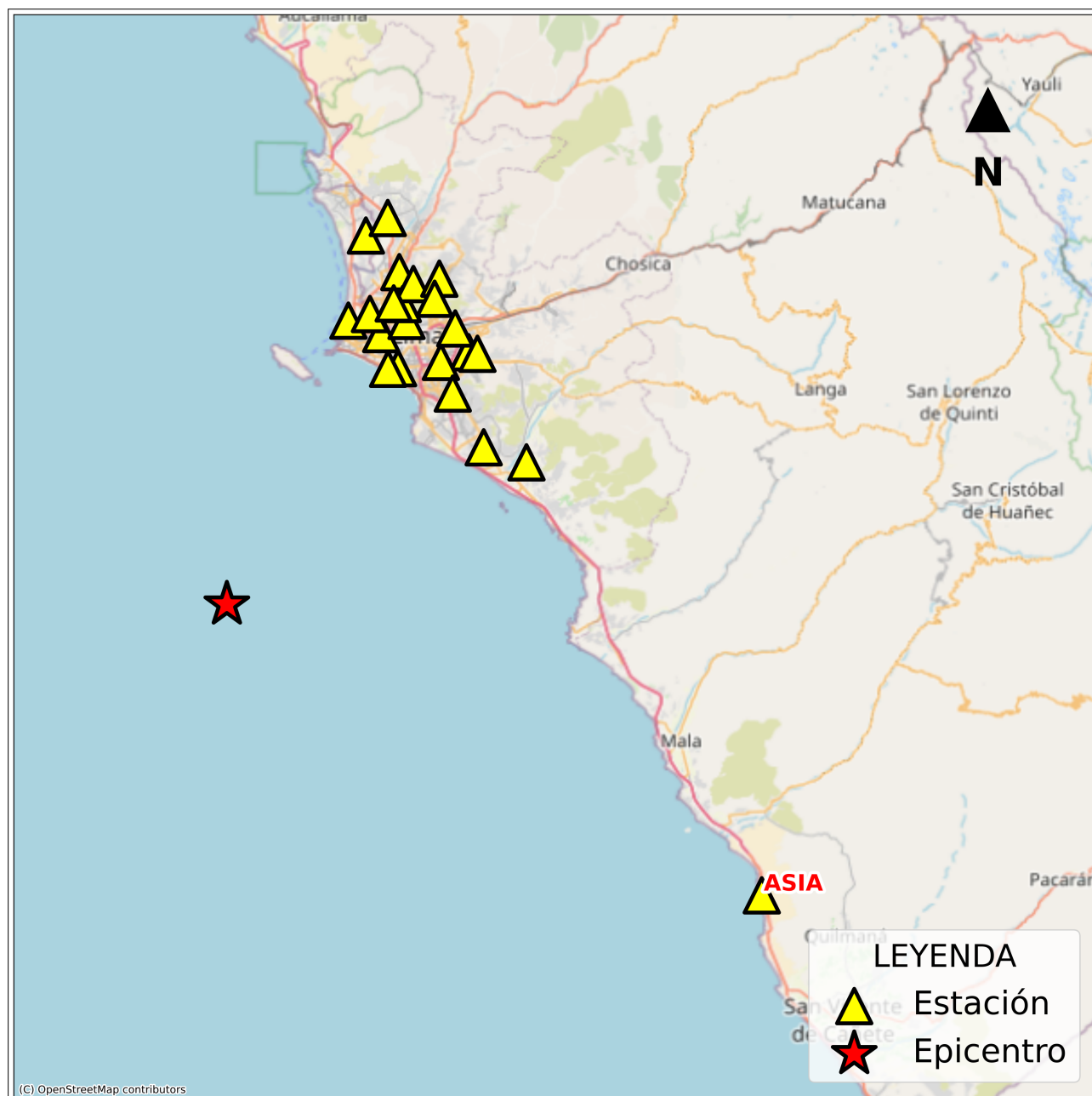
Figura 2: Mapa de ubicación de la(s) estación(es) acelerográfica(s) a nivel nacional correspondiente(s) al Sismo de Bellavista, Provincia Constitucional del Callao del 11 de noviembre de 2025 a las 09:20:16 (hora local)
