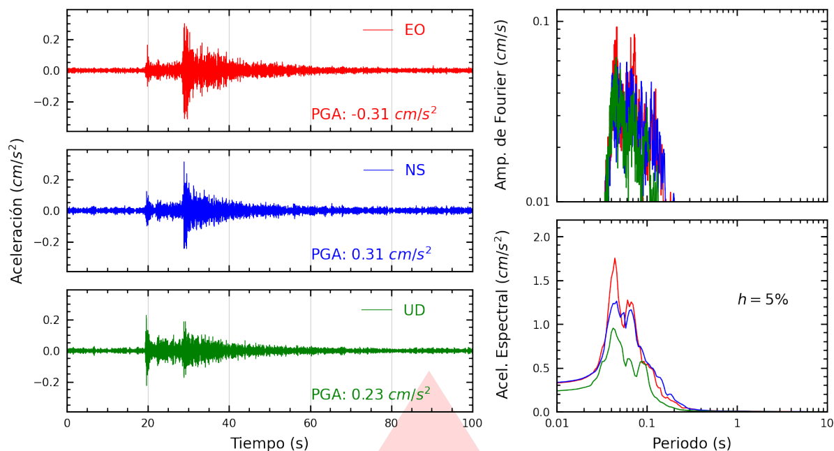
Figura A.19: Registros tiempo-historia, espectros de Fourier y de respuesta en las direcciones EO, NS y vertical de la estación ATARJ. Sismo de Bellavista, Provincia Constitucional del Callao del 2025-11-11, 09:20:16 (Hora local)
