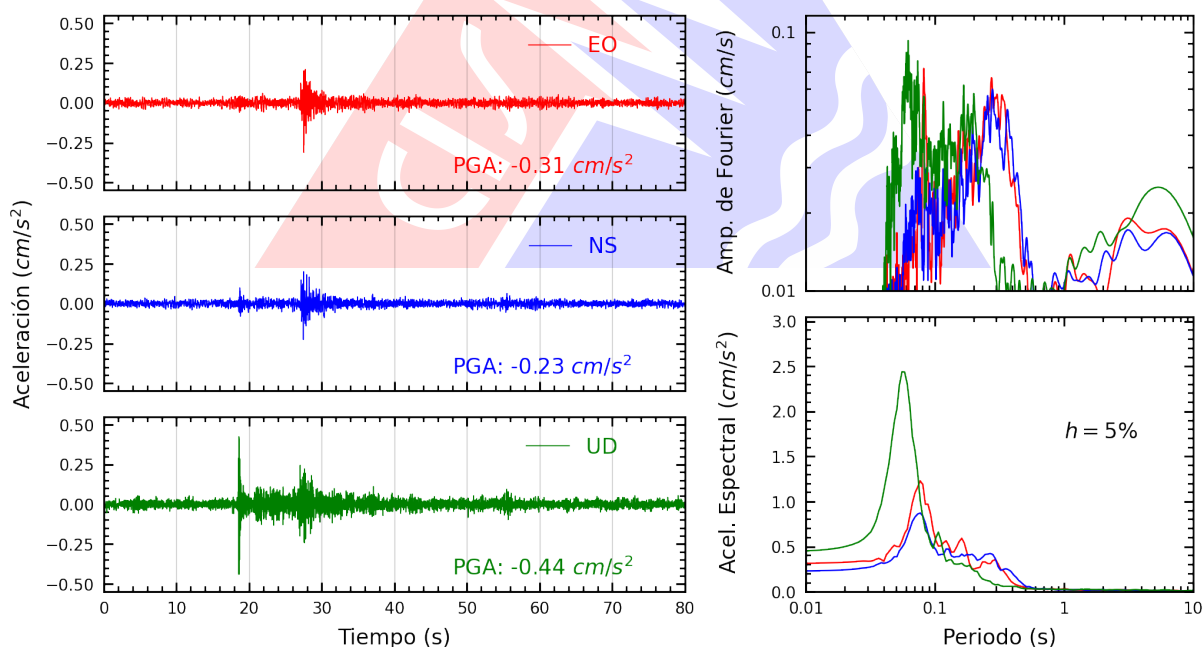
Figura A.12: Registros tiempo-historia, espectros de Fourier y de respuesta en las direcciones EO, NS y vertical de la estación ACAPU. Sismo de Bellavista, Provincia Constitucional del Callao del 2025-11-11, 09:20:16 (Hora local)
