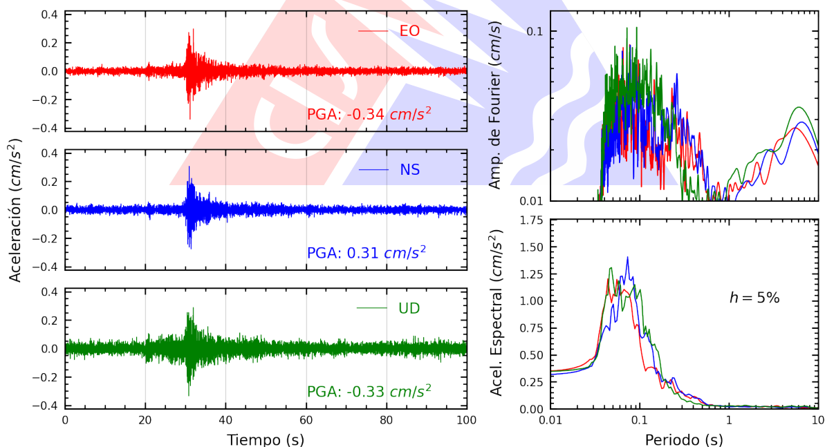
Figura A.18: Registros tiempo-historia, espectros de Fourier y de respuesta en las direcciones EO, NS y vertical de la estación MDPP. Sismo de Bellavista, Provincia Constitucional del Callao del 2025-11-11, 09:20:16 (Hora local)
