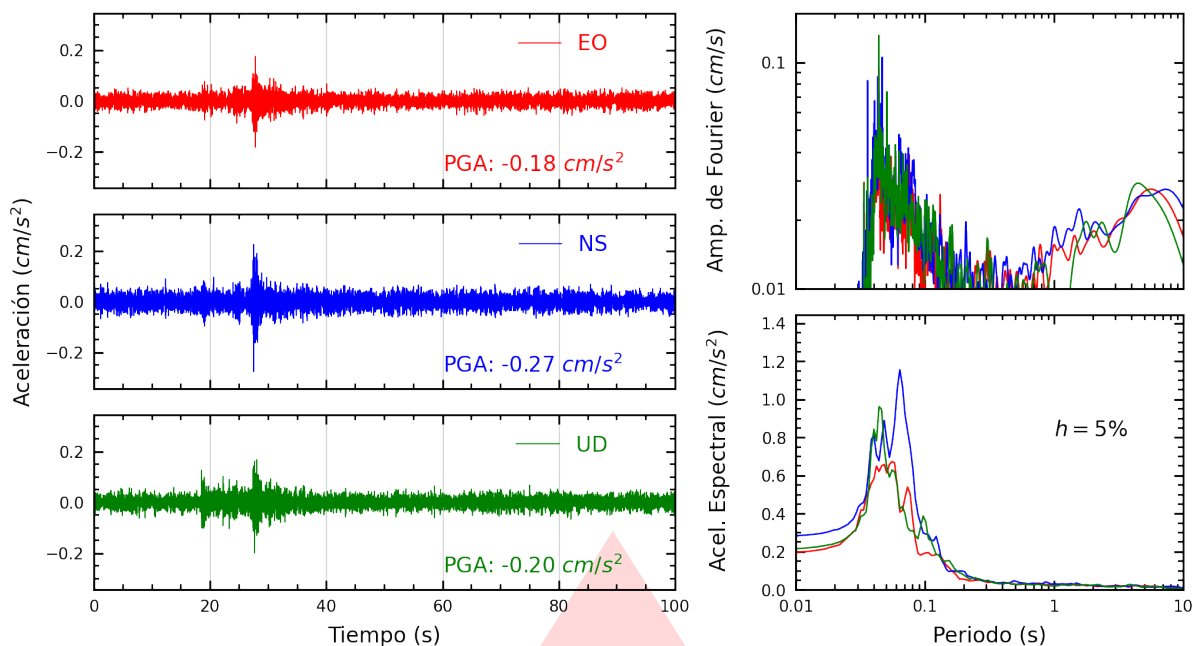
Figura A.21: Registros tiempo-historia, espectros de Fourier y de respuesta en las direcciones EO, NS y vertical de la estación BONDY. Sismo de Bellavista, Provincia Constitucional del Callao del 2025-11-11, 09:20:16 (Hora local)
