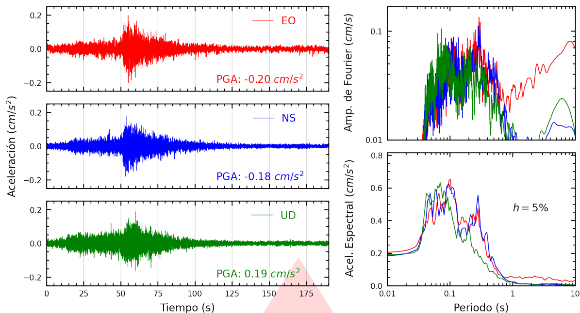
Figura A.5: Registros tiempo-historia, espectros de Fourier y de respuesta en las direcciones EO, NS y vertical de la estación UJBG3. Sismo de Ocoña, Camaná - Arequipa del 2025-11-13, 04:04:40 (Hora local)
