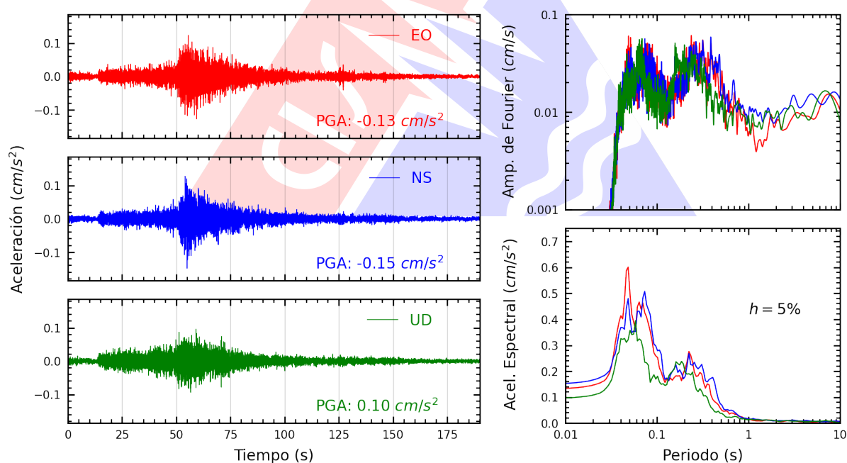
Figura A.6: Registros tiempo-historia, espectros de Fourier y de respuesta en las direcciones EO, NS y vertical de la estación CREY. Sismo de Ocoña, Camaná - Arequipa del 2025-11-13, 04:04:40 (Hora local)
