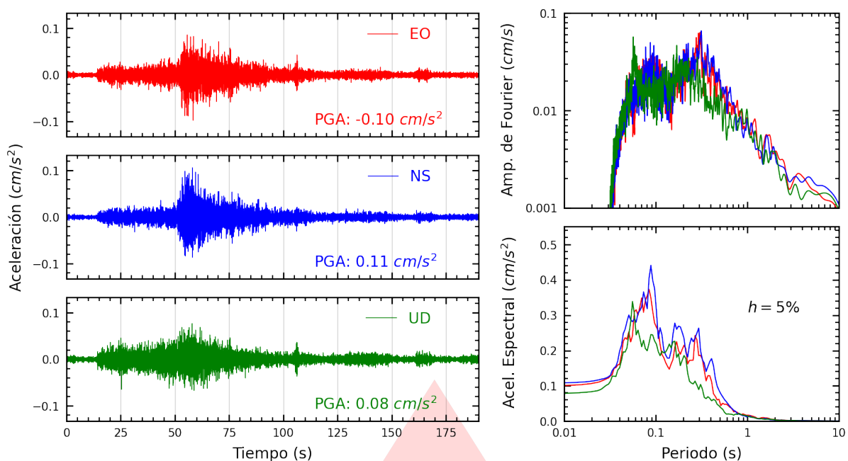
Figura A.7: Registros tiempo-historia, espectros de Fourier y de respuesta en las direcciones EO, NS y vertical de la estación UJBG2. Sismo de Ocoña, Camaná - Arequipa del 2025-11-13, 04:04:40 (Hora local)
