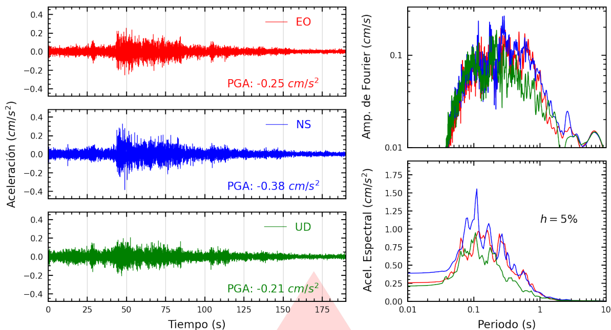
Figura A.3: Registros tiempo-historia, espectros de Fourier y de respuesta en las direcciones EO, NS y vertical de la estación UNICA. Sismo de Ocoña, Camaná - Arequipa del 2025-11-13, 04:04:40 (Hora local)
