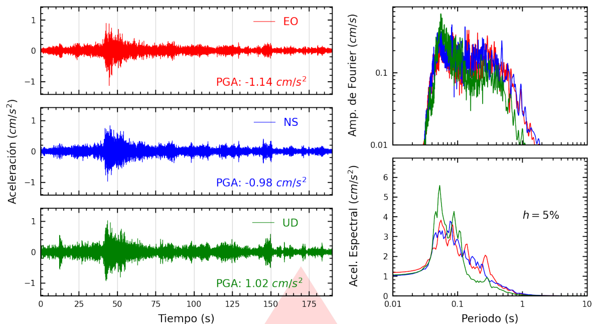
Figura A.1: Registros tiempo-historia, espectros de Fourier y de respuesta en las direcciones EO, NS y vertical de la estación SCAR2. Sismo de Ocoña, Camaná - Arequipa del 2025-11-13, 04:04:40 (Hora local)
