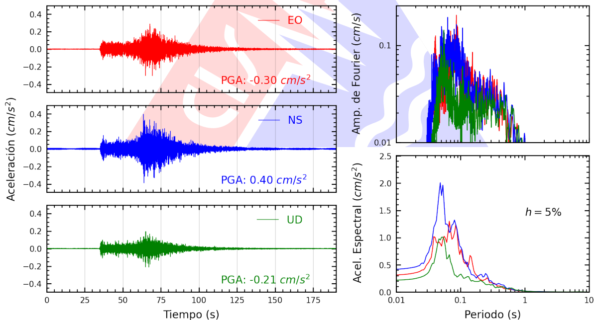
Figura A.2: Registros tiempo-historia, espectros de Fourier y de respuesta en las direcciones EO, NS y vertical de la estación UNAM. Sismo de Ocoña, Camaná - Arequipa del 2025-11-13, 04:04:40 (Hora local)
