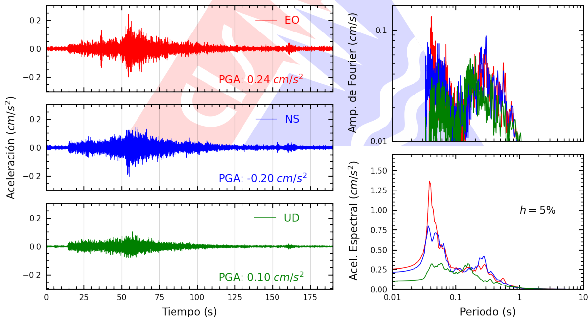
Figura A.4: Registros tiempo-historia, espectros de Fourier y de respuesta en las direcciones EO, NS y vertical de la estación UPTAC. Sismo de Ocoña, Camaná - Arequipa del 2025-11-13, 04:04:40 (Hora local)
