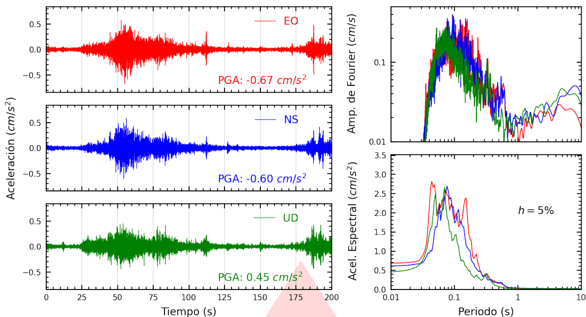
Figura A.13: Registros tiempo-historia, espectros de Fourier y de respuesta en las direcciones EO, NS y vertical de la estación SJLSV. Sismo de Huarney, Huarney - Áncash del 2025-11-16, 23:58:01 (Hora local)
