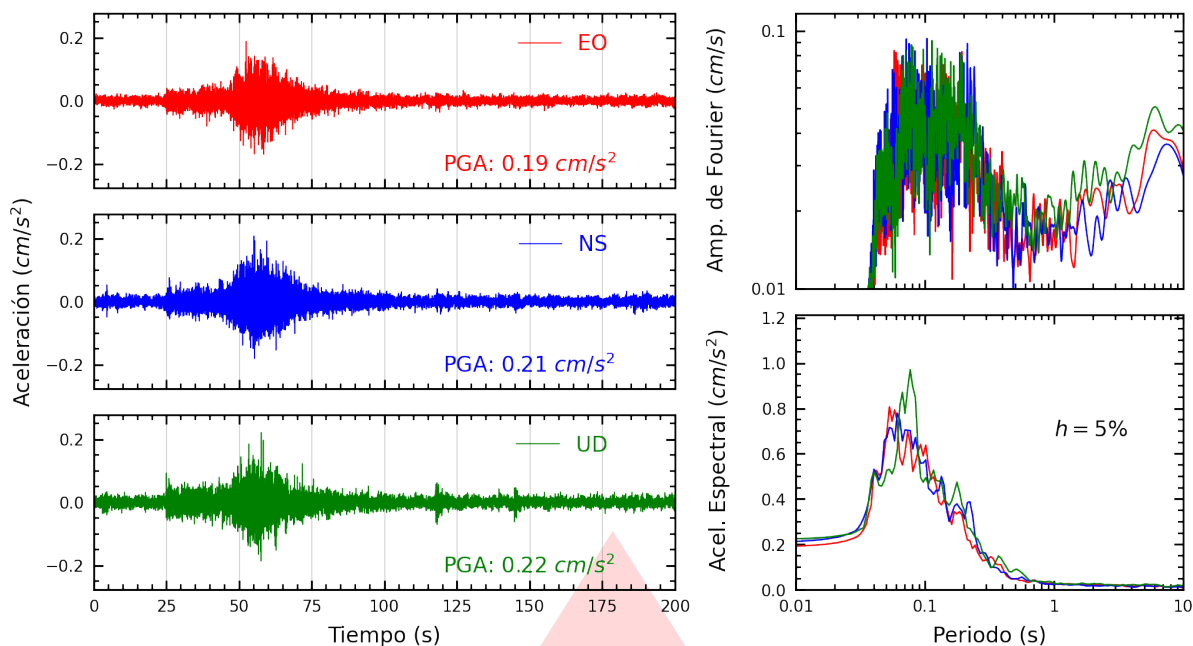
Figura A.33: Registros tiempo-historia, espectros de Fourier y de respuesta en las direcciones EO, NS y vertical de la estación UNFV. Sismo de Huarney, Huarney - Áncash del 2025-11-16, 23:58:01 (Hora local)
