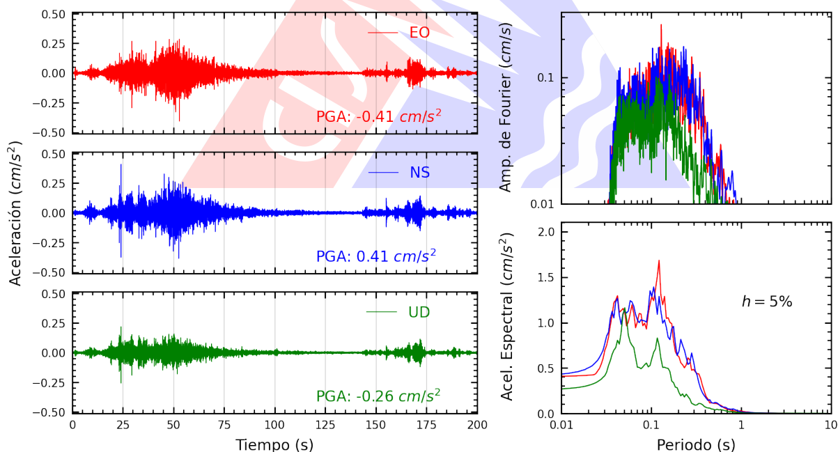
Figura A.24: Registros tiempo-historia, espectros de Fourier y de respuesta en las direcciones EO, NS y vertical de la estación BRISA. Sismo de Huarney, Huarney - Áncash del 2025-11-16, 23:58:01 (Hora local)
