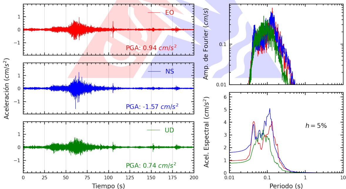
Figura A.2: Registros tiempo-historia, espectros de Fourier y de respuesta en las direcciones EO, NS y vertical de la estación CARAB. Sismo de Huarney, Huarney - Áncash del 2025-11-16, 23:58:01 (Hora local)
