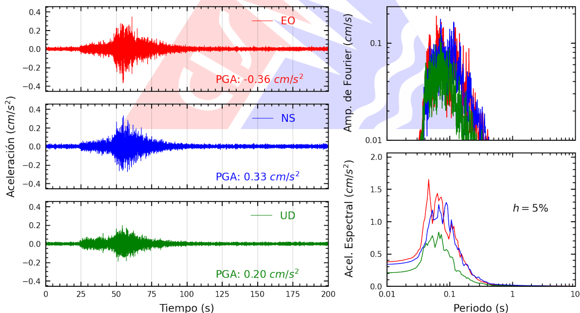
Figura A.26: Registros tiempo-historia, espectros de Fourier y de respuesta en las direcciones EO, NS y vertical de la estación ATARJ. Sismo de Huarney, Huarney - Áncash del 2025-11-16, 23:58:01 (Hora local)
