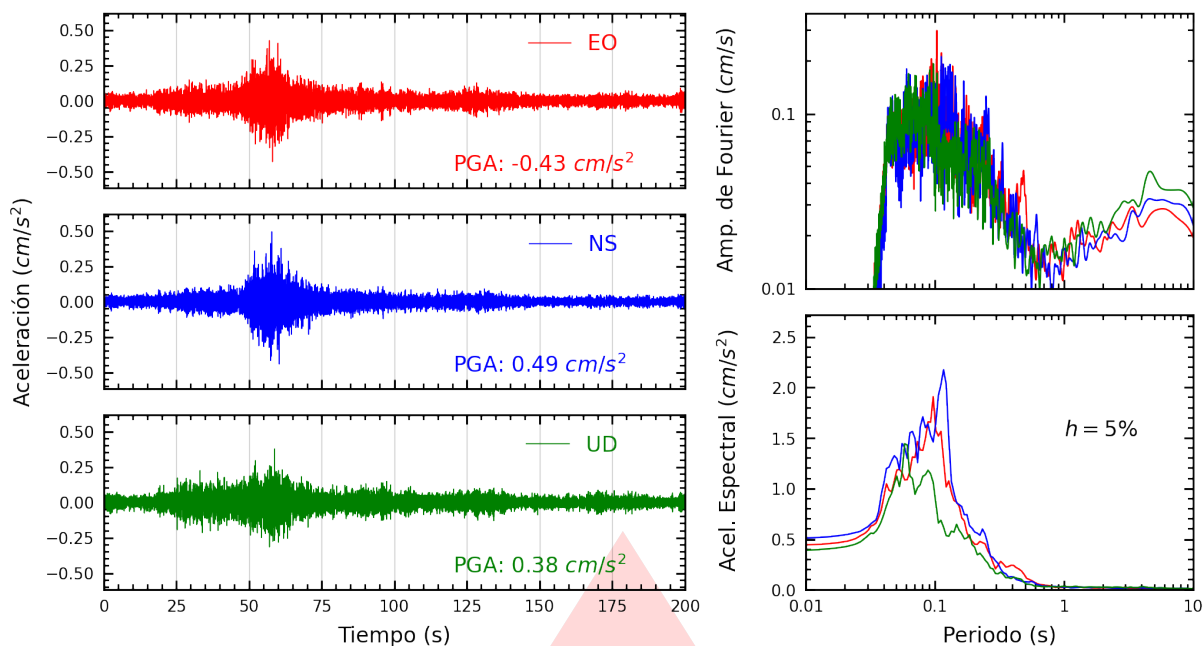
Figura A.17: Registros tiempo-historia, espectros de Fourier y de respuesta en las direcciones EO, NS y vertical de la estación URPPE. Sismo de Huarney, Huarney - Áncash del 2025-11-16, 23:58:01 (Hora local)
