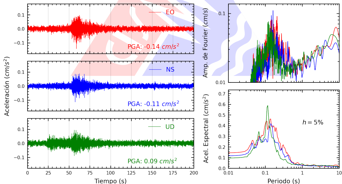
Figura A.38: Registros tiempo-historia, espectros de Fourier y de respuesta en las direcciones EO, NS y vertical de la estación UPAOT. Sismo de Huarney, Huarney - Áncash del 2025-11-16, 23:58:01 (Hora local)
