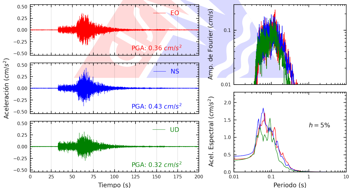
Figura A.22: Registros tiempo-historia, espectros de Fourier y de respuesta en las direcciones EO, NS y vertical de la estación JALV2. Sismo de Huarney, Huarney - Áncash del 2025-11-16, 23:58:01 (Hora local)
