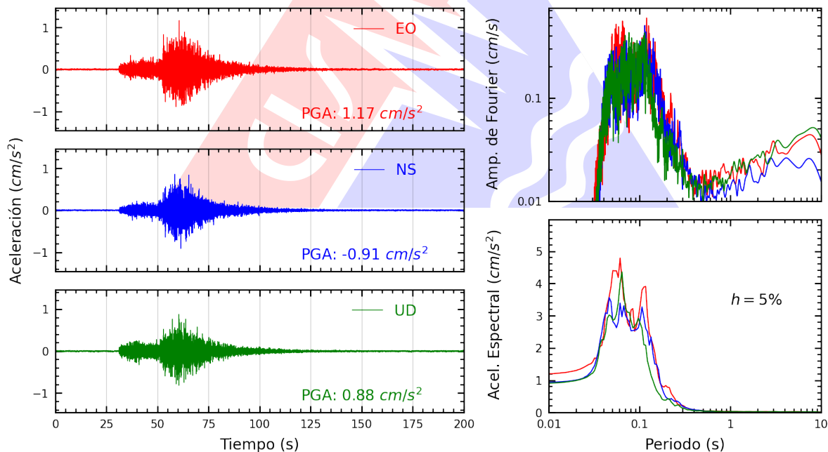
Figura A.6: Registros tiempo-historia, espectros de Fourier y de respuesta en las direcciones EO, NS y vertical de la estación AMORE. Sismo de Huarney, Huarney - Áncash del 2025-11-16, 23:58:01 (Hora local)
