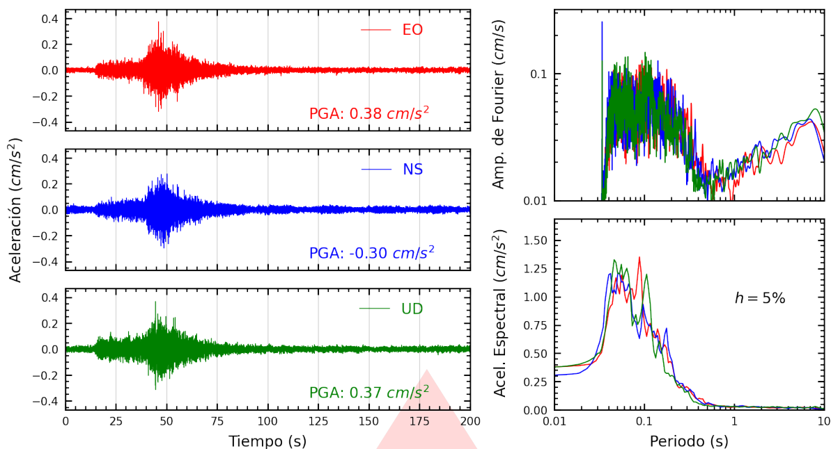
Figura A.25: Registros tiempo-historia, espectros de Fourier y de respuesta en las direcciones EO, NS y vertical de la estación USMP. Sismo de Huarney, Huarney - Áncash del 2025-11-16, 23:58:01 (Hora local)
