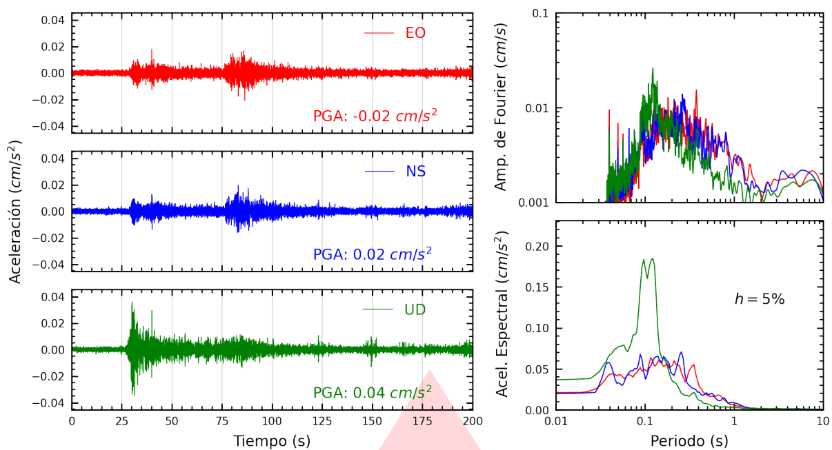
Figura A.39: Registros tiempo-historia, espectros de Fourier y de respuesta en las direcciones EO, NS y vertical de la estación UNIA. Sismo de Huarmey, Huarmey - Áncash del 2025-11-16, 23:58:01 (Hora local)
