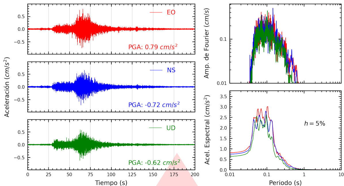
Figura A.9: Registros tiempo-historia, espectros de Fourier y de respuesta en las direcciones EO, NS y vertical de la estación PHERM. Sismo de Huarney, Huarney - Áncash del 2025-11-16, 23:58:01 (Hora local)
