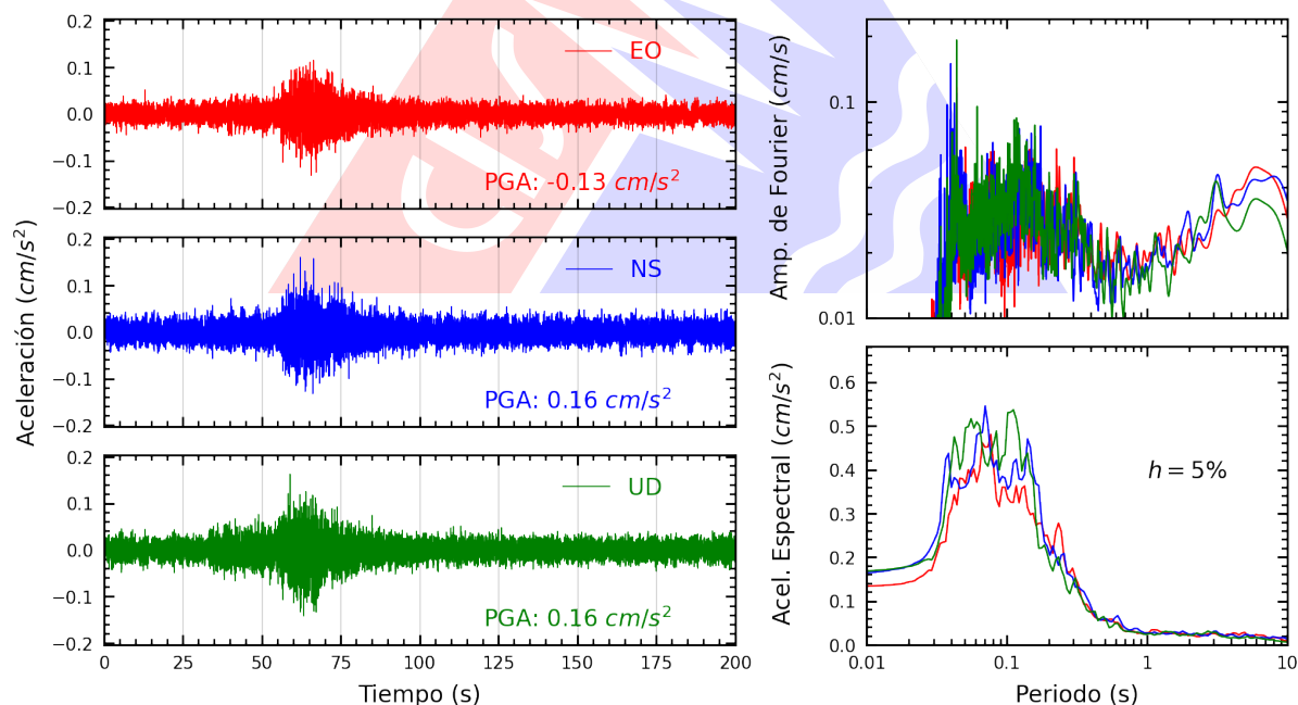
Figura A.36: Registros tiempo-historia, espectros de Fourier y de respuesta en las direcciones EO, NS y vertical de la estación BONDY. Sismo de Huarney, Huarney - Áncash del 2025-11-16, 23:58:01 (Hora local)
