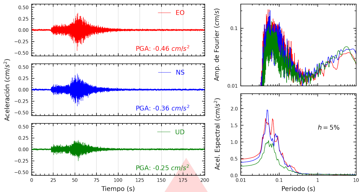
Figura A.19: Registros tiempo-historia, espectros de Fourier y de respuesta en las direcciones EO, NS y vertical de la estación UCSS. Sismo de Huarney, Huarney - Áncash del 2025-11-16, 23:58:01 (Hora local)
