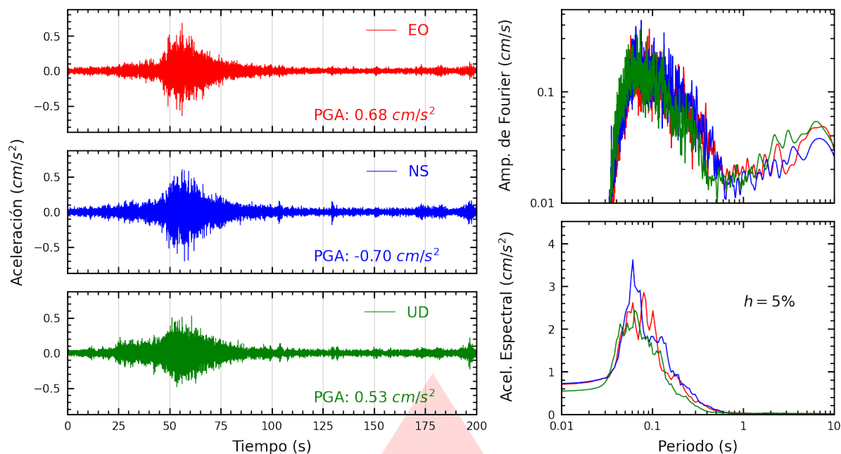
Figura A.11: Registros tiempo-historia, espectros de Fourier y de respuesta en las direcciones EO, NS y vertical de la estación SJLSC. Sismo de Huarney, Huarney - Áncash del 2025-11-16, 23:58:01 (Hora local)
