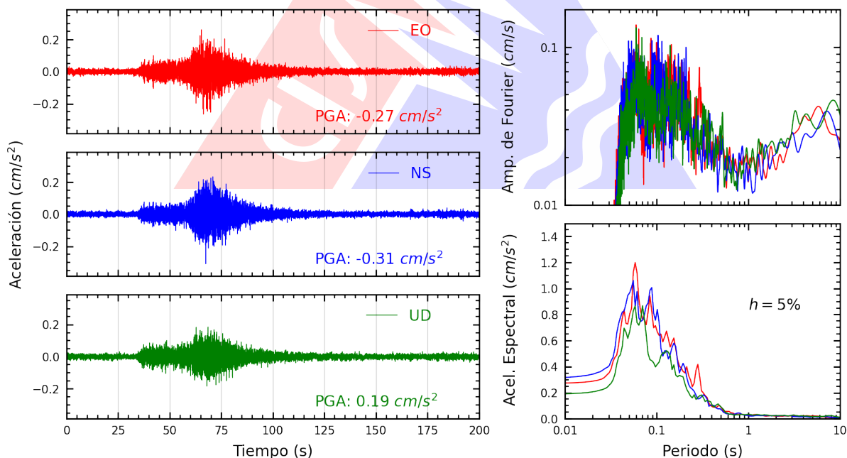
Figura A.30: Registros tiempo-historia, espectros de Fourier y de respuesta en las direcciones EO, NS y vertical de la estación IMCA. Sismo de Huarmey, Huarmey - Áncash del 2025-11-16, 23:58:01 (Hora local)
