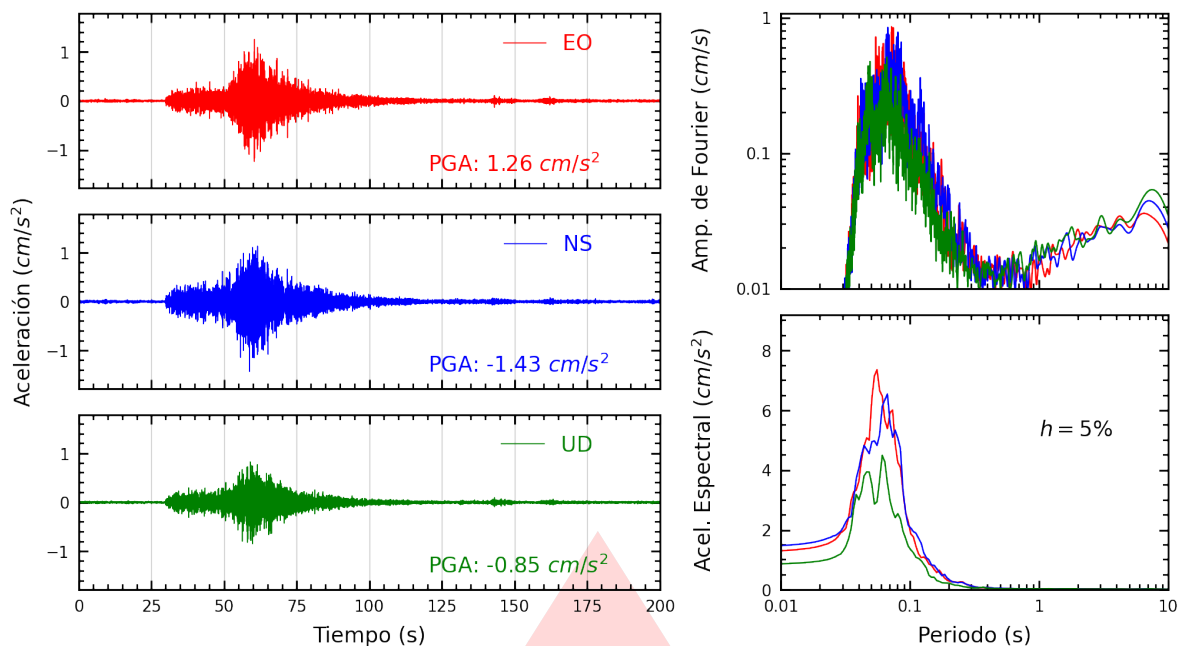
Figura A.3: Registros tiempo-historia, espectros de Fourier y de respuesta en las direcciones EO, NS y vertical de la estación JOSEO. Sismo de Huarney, Huarney - Áncash del 2025-11-16, 23:58:01 (Hora local)
