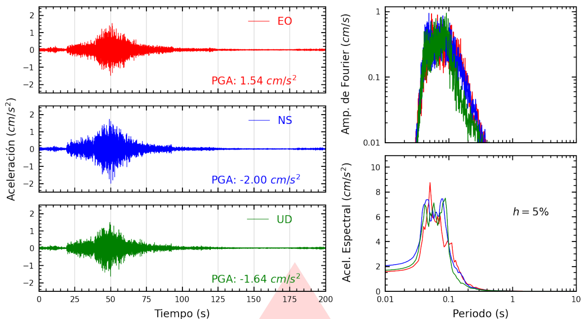
Figura A.1: Registros tiempo-historia, espectros de Fourier y de respuesta en las direcciones EO, NS y vertical de la estación SROSA. Sismo de Huarney, Huarney - Áncash del 2025-11-16, 23:58:01 (Hora local)
