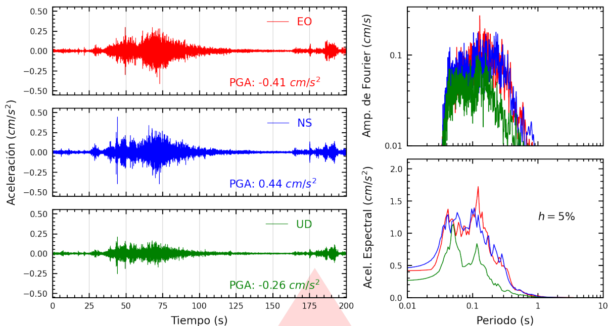
Figura A.21: Registros tiempo-historia, espectros de Fourier y de respuesta en las direcciones EO, NS y vertical de la estación BRIS2. Sismo de Huarney, Huarney - Áncash del 2025-11-16, 23:58:01 (Hora local)
