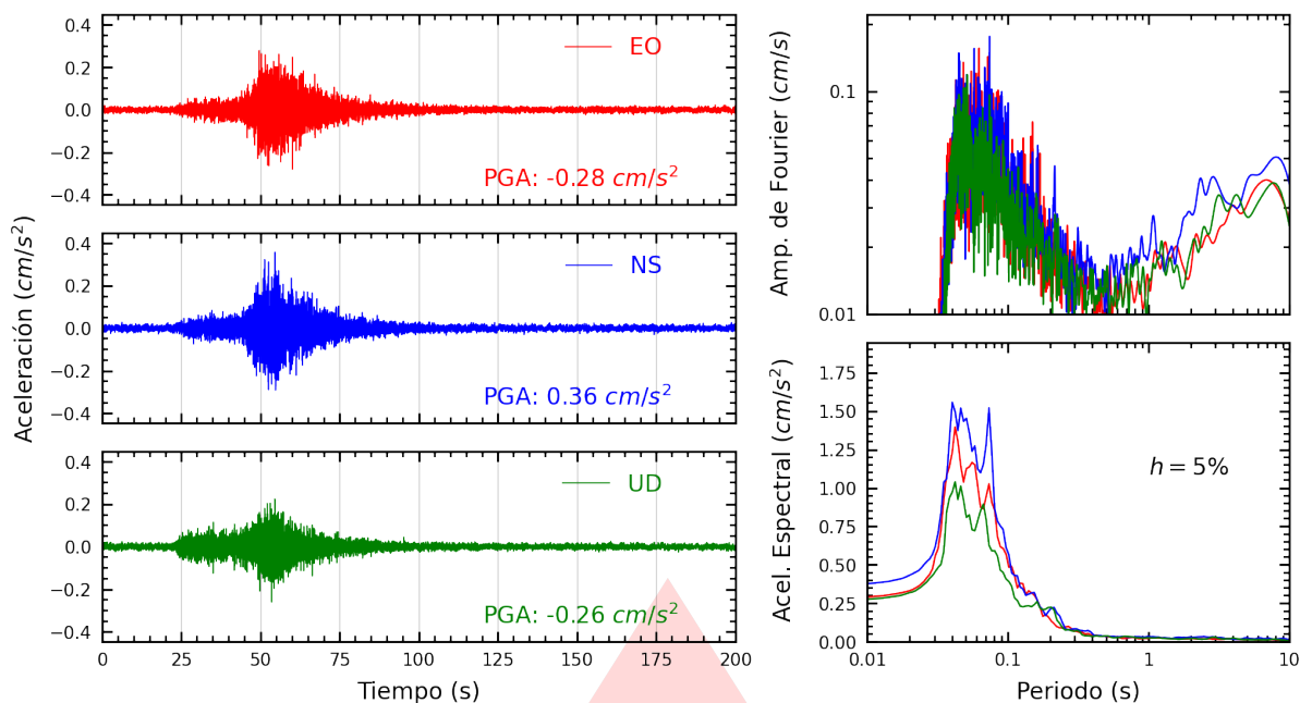
Figura A.27: Registros tiempo-historia, espectros de Fourier y de respuesta en las direcciones EO, NS y vertical de la estación SJLCE. Sismo de Huarney, Huarney - Áncash del 2025-11-16, 23:58:01 (Hora local)
