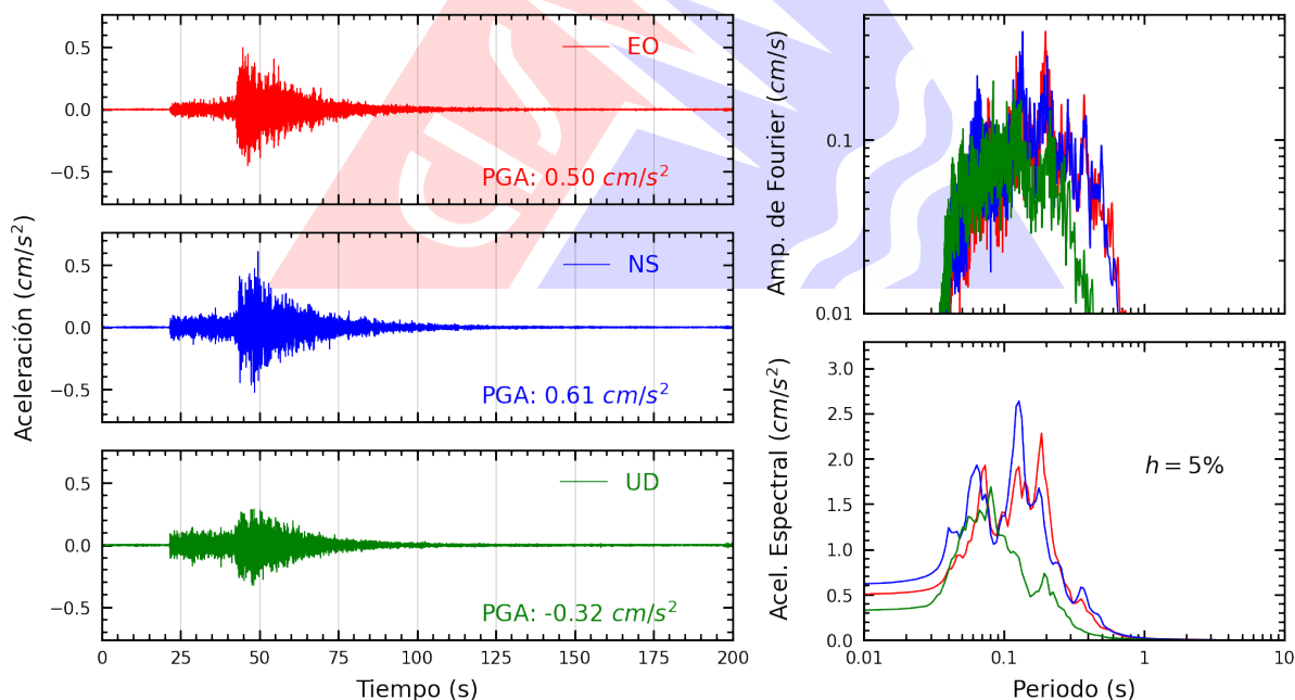
Figura A.14: Registros tiempo-historia, espectros de Fourier y de respuesta en las direcciones EO, NS y vertical de la estación VHAYA. Sismo de Huarney, Huarney - Áncash del 2025-11-16, 23:58:01 (Hora local)
