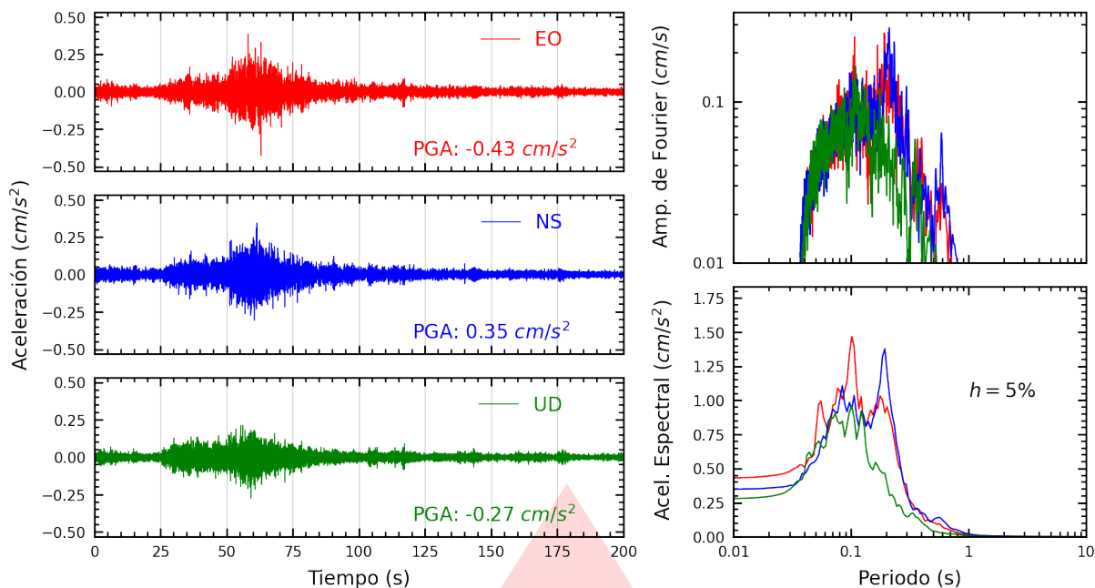
Figura A.23: Registros tiempo-historia, espectros de Fourier y de respuesta en las direcciones EO, NS y vertical de la estación SCCHO. Sismo de Huarney, Huarney - Áncash del 2025-11-16, 23:58:01 (Hora local)
