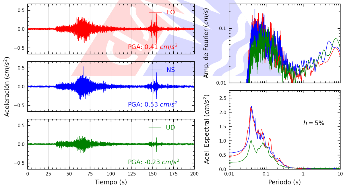
Figura A.16: Registros tiempo-historia, espectros de Fourier y de respuesta en las direcciones EO, NS y vertical de la estación CEPRE. Sismo de Huarney, Huarney - Áncash del 2025-11-16, 23:58:01 (Hora local)
