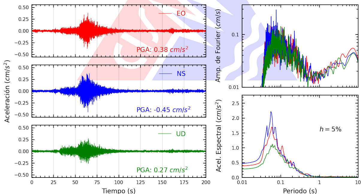
Figura A.20: Registros tiempo-historia, espectros de Fourier y de respuesta en las direcciones EO, NS y vertical de la estación COMAS. Sismo de Huarney, Huarney - Áncash del 2025-11-16, 23:58:01 (Hora local)
