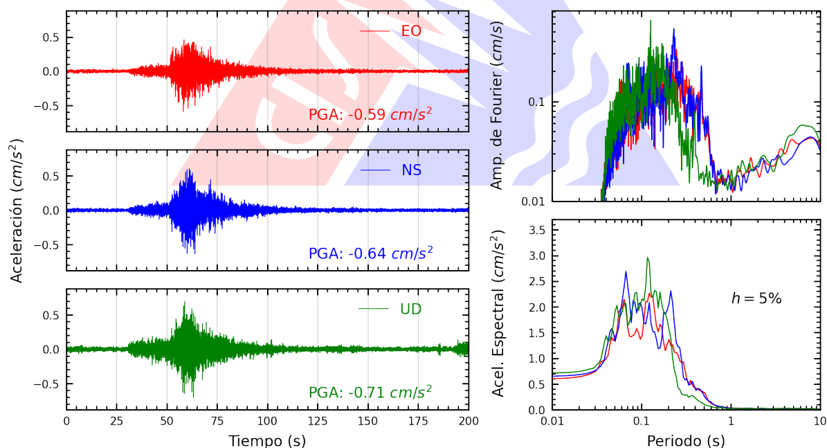
Figura A.10: Registros tiempo-historia, espectros de Fourier y de respuesta en las direcciones EO, NS y vertical de la estación MDPP. Sismo de Huarney, Huarney - Áncash del 2025-11-16, 23:58:01 (Hora local)
