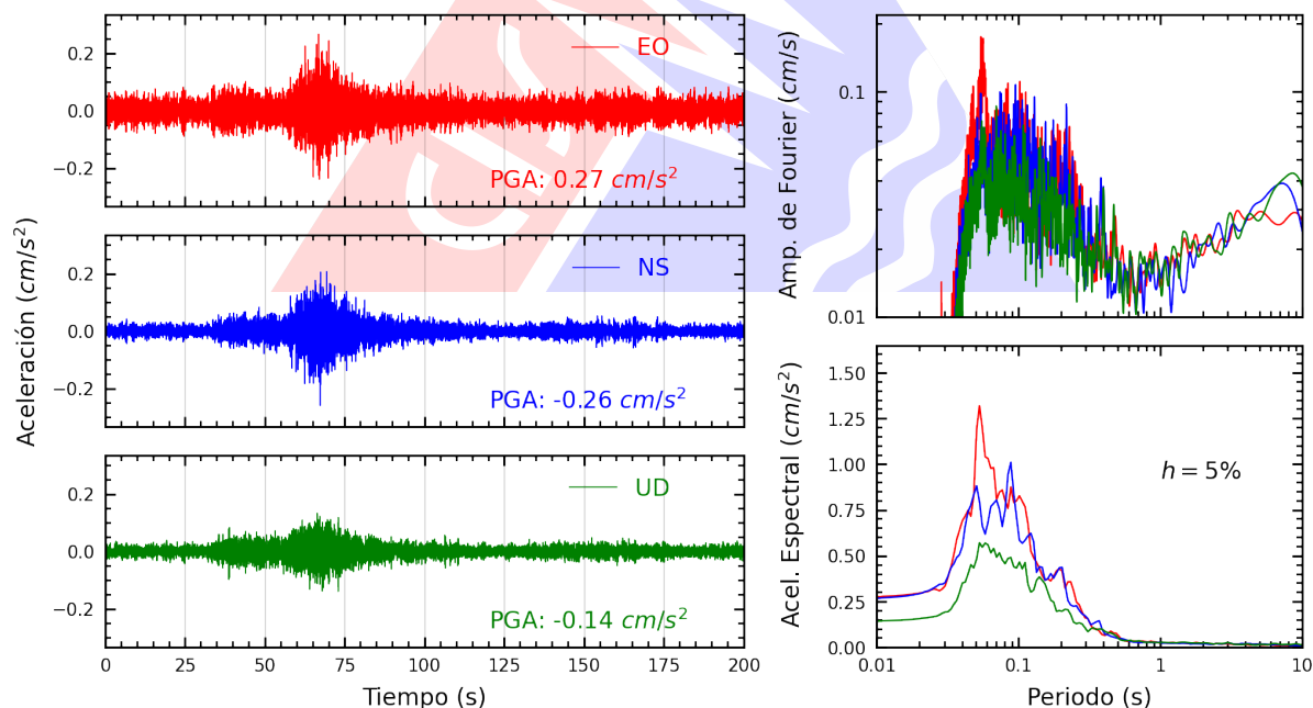
Figura A.32: Registros tiempo-historia, espectros de Fourier y de respuesta en las direcciones EO, NS y vertical de la estación INICT. Sismo de Huarney, Huarney - Áncash del 2025-11-16, 23:58:01 (Hora local)
