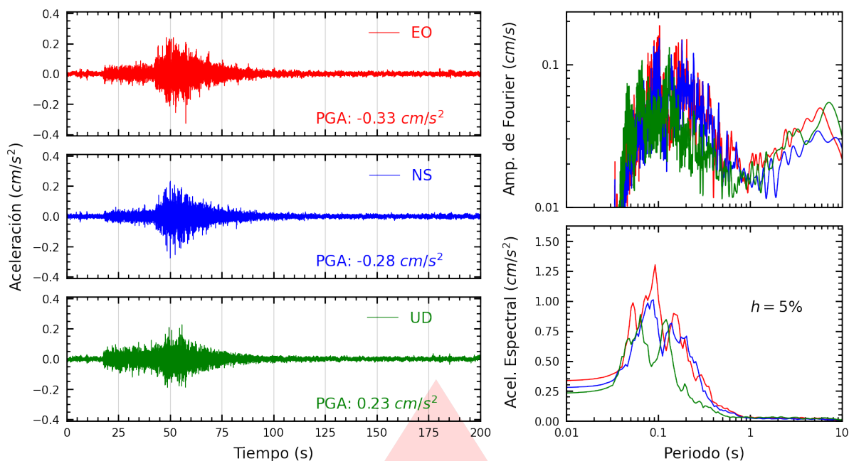
Figura A.29: Registros tiempo-historia, espectros de Fourier y de respuesta en las direcciones EO, NS y vertical de la estación USILP. Sismo de Huarmey, Huarmey - Áncash del 2025-11-16, 23:58:01 (Hora local)
