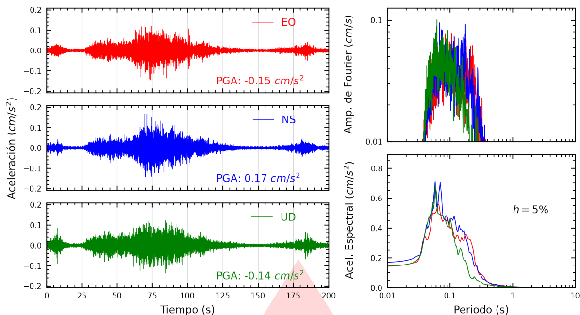
Figura A.35: Registros tiempo-historia, espectros de Fourier y de respuesta en las direcciones EO, NS y vertical de la estación ASIA. Sismo de Huarney, Huarney - Áncash del 2025-11-16, 23:58:01 (Hora local)
