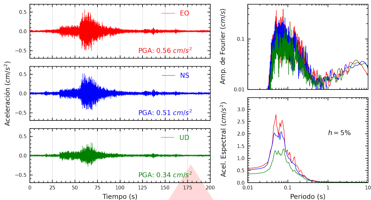
Figura A.15: Registros tiempo-historia, espectros de Fourier y de respuesta en las direcciones EO, NS y vertical de la estación FICPE. Sismo de Huarney, Huarney - Áncash del 2025-11-16, 23:58:01 (Hora local)
