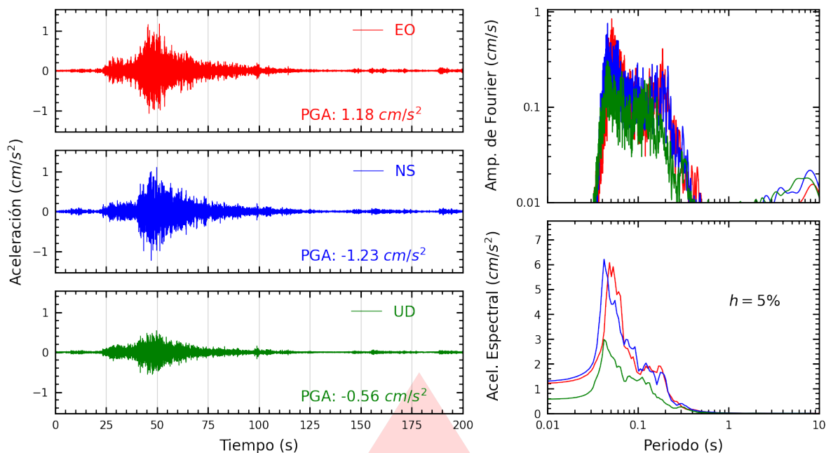
Figura A.5: Registros tiempo-historia, espectros de Fourier y de respuesta en las direcciones EO, NS y vertical de la estación UNS. Sismo de Huarney, Huarney - Áncash del 2025-11-16, 23:58:01 (Hora local)
