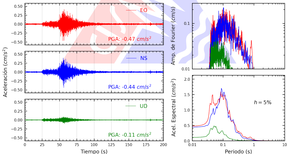
Figura A.18: Registros tiempo-historia, espectros de Fourier y de respuesta en las direcciones EO, NS y vertical de la estación UCVAT. Sismo de Huarney, Huarney - Áncash del 2025-11-16, 23:58:01 (Hora local)
