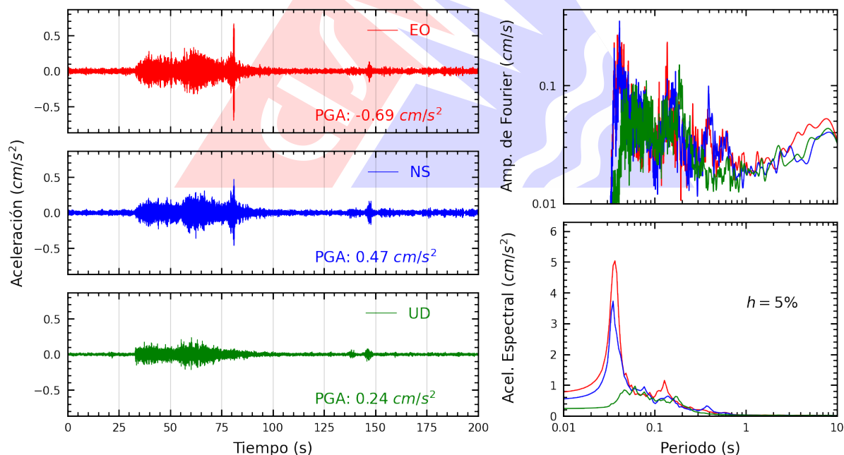
Figura A.12: Registros tiempo-historia, espectros de Fourier y de respuesta en las direcciones EO, NS y vertical de la estación DHNPE. Sismo de Huarney, Huarney - Áncash del 2025-11-16, 23:58:01 (Hora local)
