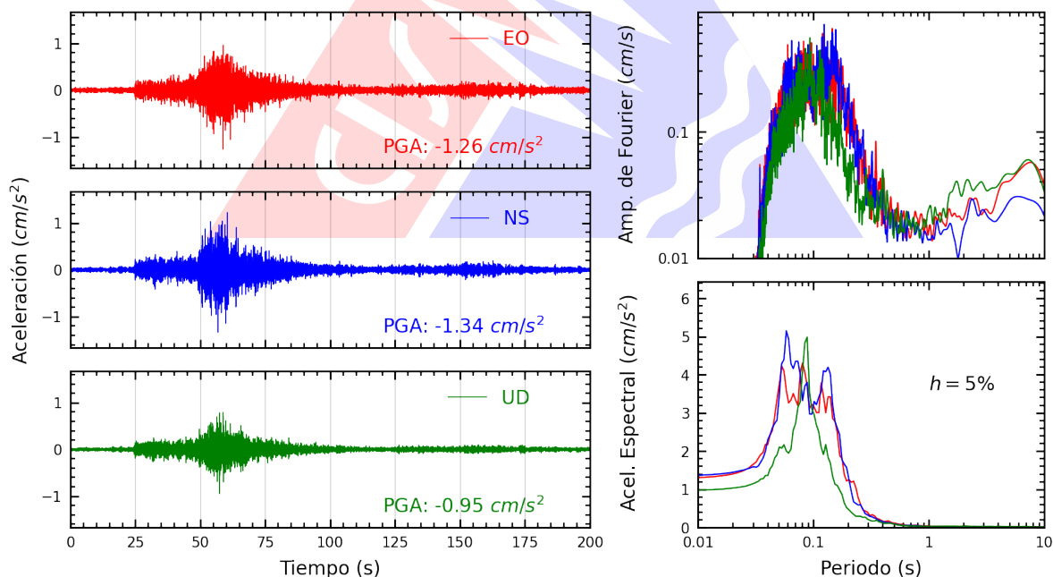
Figura A.4: Registros tiempo-historia, espectros de Fourier y de respuesta en las direcciones EO, NS y vertical de la estación USILM. Sismo de Huarney, Huarney - Áncash del 2025-11-16, 23:58:01 (Hora local)
