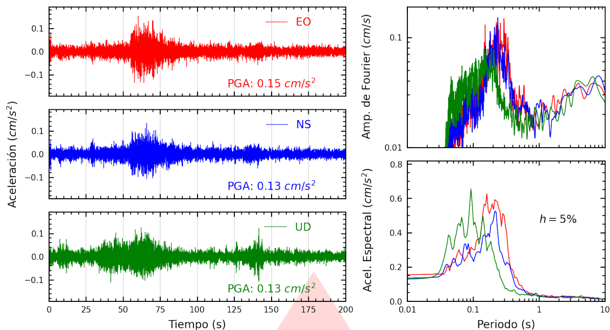
Figura A.37: Registros tiempo-historia, espectros de Fourier y de respuesta en las direcciones EO, NS y vertical de la estación DSML. Sismo de Huarney, Huarney - Áncash del 2025-11-16, 23:58:01 (Hora local)
