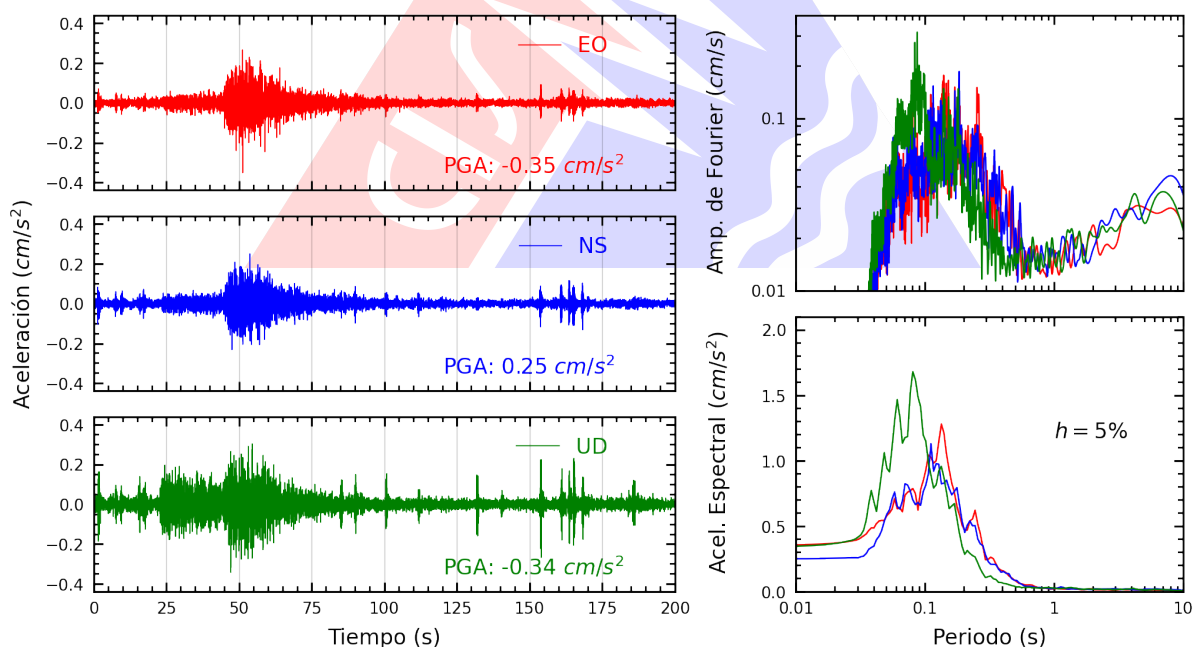
Figura A.28: Registros tiempo-historia, espectros de Fourier y de respuesta en las direcciones EO, NS y vertical de la estación RAMON. Sismo de Huarney, Huarney - Áncash del 2025-11-16, 23:58:01 (Hora local)
