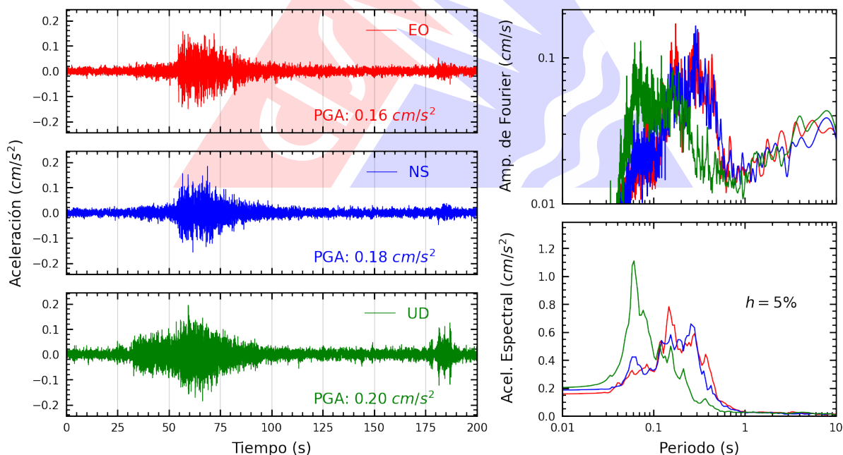
Figura A.34: Registros tiempo-historia, espectros de Fourier y de respuesta en las direcciones EO, NS y vertical de la estación ACAPU. Sismo de Huarney, Huarney - Áncash del 2025-11-16, 23:58:01 (Hora local)
