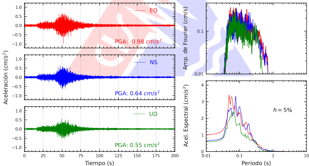
Figura A.8: Registros tiempo-historia, espectros de Fourier y de respuesta en las direcciones EO, NS y vertical de la estación UNTEL. Sismo de Huarmey, Huarmey - Áncash del 2025-11-16, 23:58:01 (Hora local)
