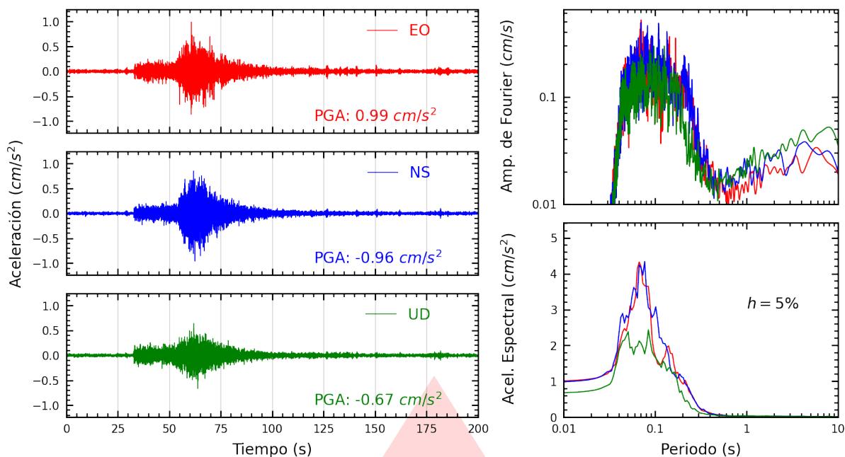
Figura A.7: Registros tiempo-historia, espectros de Fourier y de respuesta en las direcciones EO, NS y vertical de la estación INDEP. Sismo de Huarmey, Huarmey - Áncash del 2025-11-16, 23:58:01 (Hora local)
