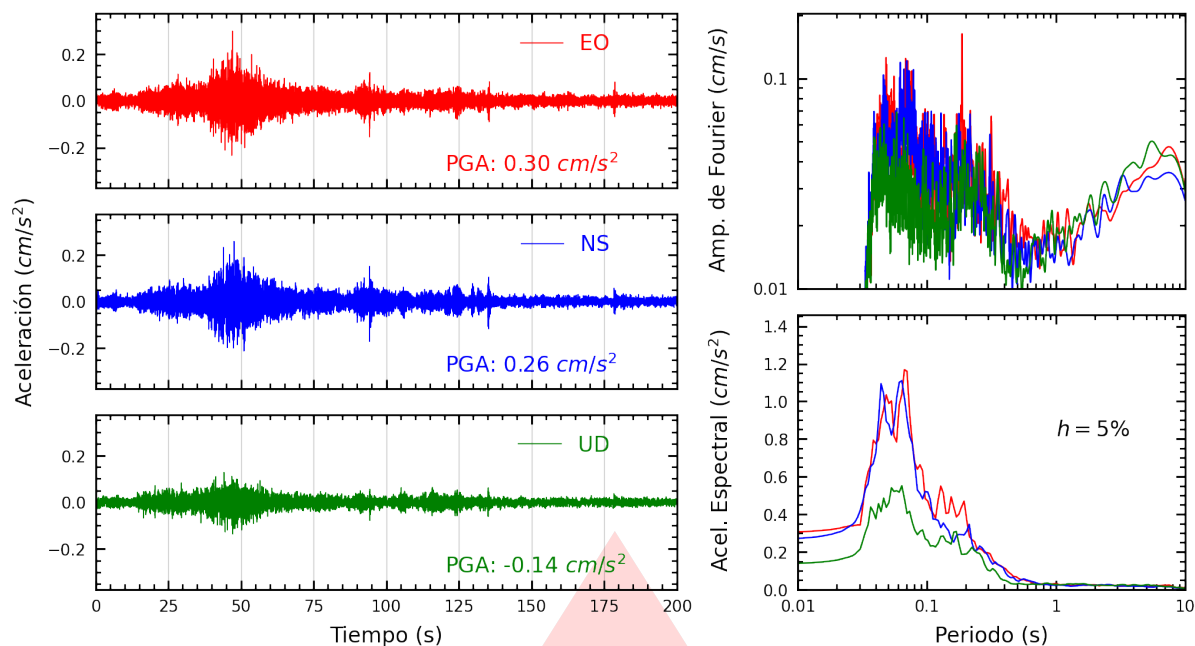
Figura A.31: Registros tiempo-historia, espectros de Fourier y de respuesta en las direcciones EO, NS y vertical de la estación UPCVI. Sismo de Huarney, Huarney - Áncash del 2025-11-16, 23:58:01 (Hora local)
