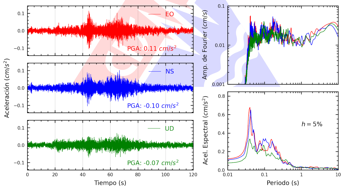
Figura A.24: Registros tiempo-historia, espectros de Fourier y de respuesta en las direcciones EO, NS y vertical de la estación COMAS. Sismo de Palpa, Palpa - Ica del 2025-11-25, 02:23:09 (Hora local)
