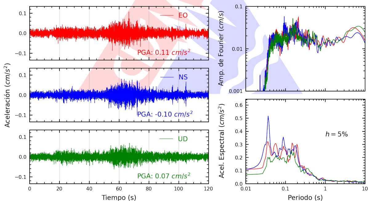
Figura A.26: Registros tiempo-historia, espectros de Fourier y de respuesta en las direcciones EO, NS y vertical de la estación IMCA. Sismo de Palpa, Palpa - Ica del 2025-11-25, 02:23:09 (Hora local)
