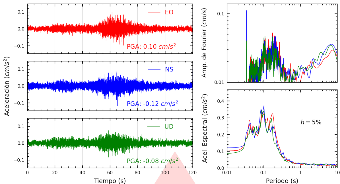
Figura A.23: Registros tiempo-historia, espectros de Fourier y de respuesta en las direcciones EO, NS y vertical de la estación USMP. Sismo de Palpa, Palpa - Ica del 2025-11-25, 02:23:09 (Hora local)
