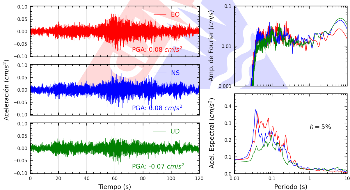
Figura A.30: Registros tiempo-historia, espectros de Fourier y de respuesta en las direcciones EO, NS y vertical de la estación CEPRE. Sismo de Palpa, Palpa - Ica del 2025-11-25, 02:23:09 (Hora local)
