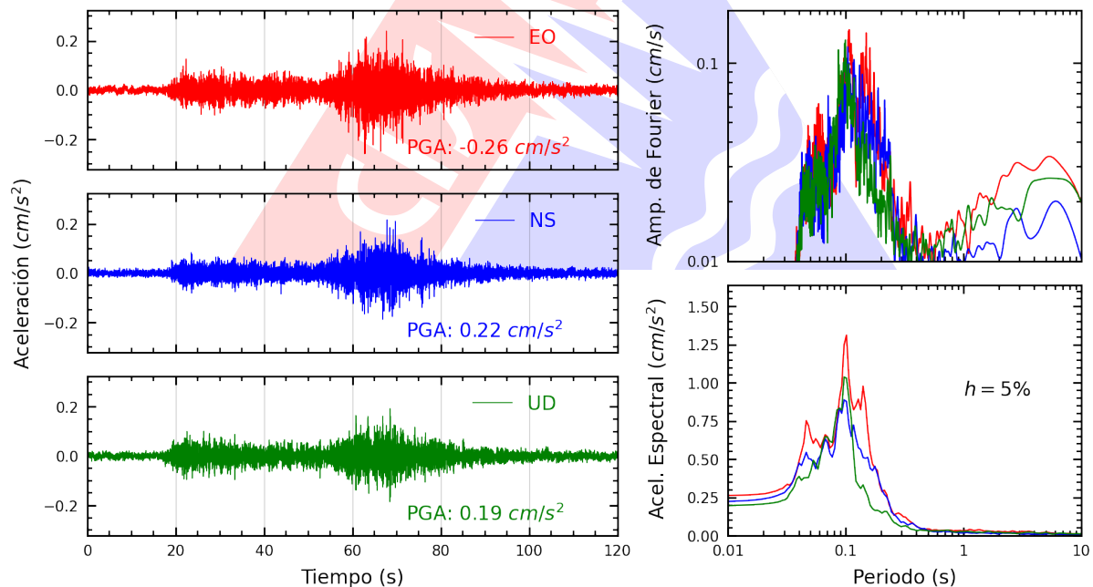
Figura A.12: Registros tiempo-historia, espectros de Fourier y de respuesta en las direcciones EO, NS y vertical de la estación AMORE. Sismo de Palpa, Palpa - Ica del 2025-11-25, 02:23:09 (Hora local)
