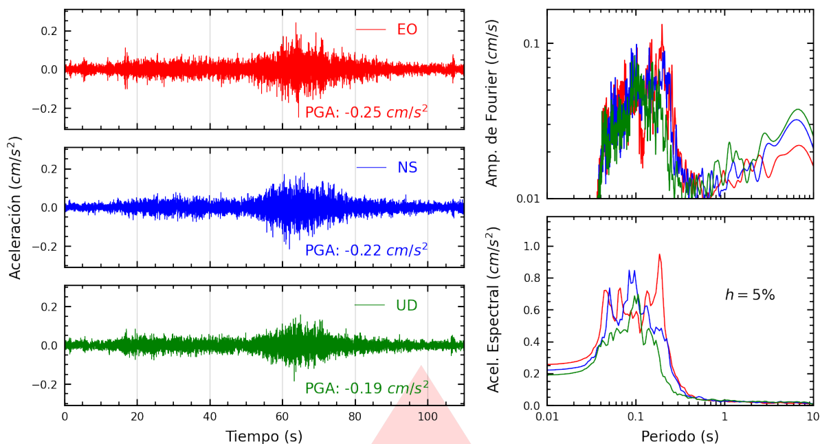
Figura A.13: Registros tiempo-historia, espectros de Fourier y de respuesta en las direcciones EO, NS y vertical de la estación INDEP. Sismo de Palpa, Palpa - Ica del 2025-11-25, 02:23:09 (Hora local)
