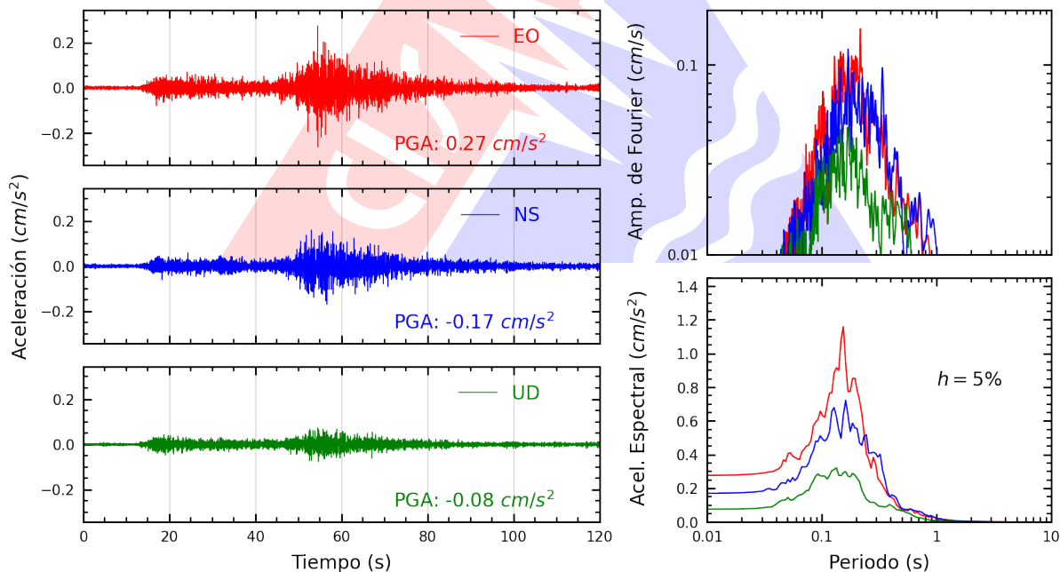
Figura A.8: Registros tiempo-historia, espectros de Fourier y de respuesta en las direcciones EO, NS y vertical de la estación BRIS2. Sismo de Palpa, Palpa - Ica del 2025-11-25, 02:23:09 (Hora local)
