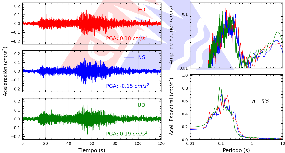
Figura A.16: Registros tiempo-historia, espectros de Fourier y de respuesta en las direcciones EO, NS y vertical de la estación SOVES. Sismo de Palpa, Palpa - Ica del 2025-11-25, 02:23:09 (Hora local)
