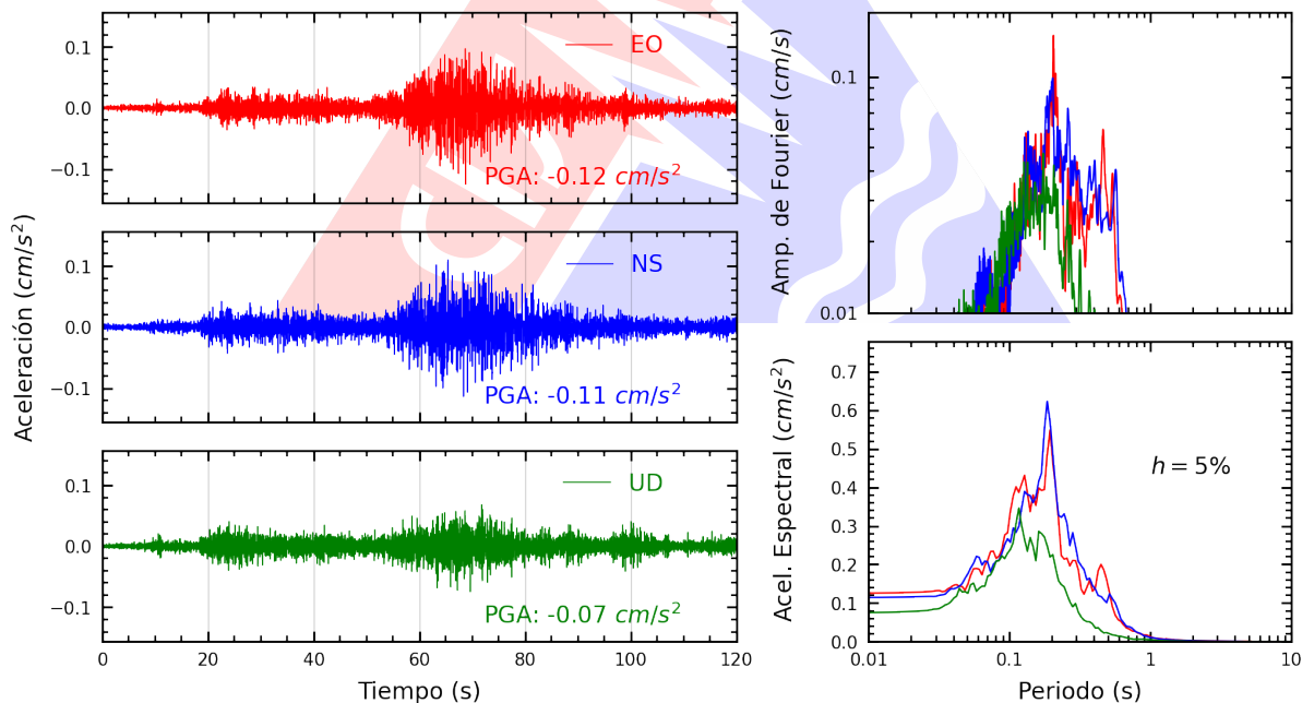
Figura A.22: Registros tiempo-historia, espectros de Fourier y de respuesta en las direcciones EO, NS y vertical de la estación VHAYA. Sismo de Palpa, Palpa - Ica del 2025-11-25, 02:23:09 (Hora local)
