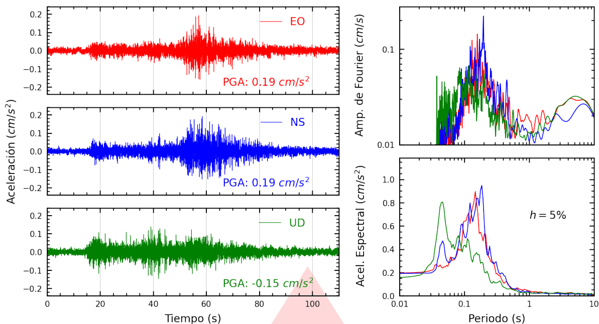
Figura A.15: Registros tiempo-historia, espectros de Fourier y de respuesta en las direcciones EO, NS y vertical de la estación SOCHO. Sismo de Palpa, Palpa - Ica del 2025-11-25, 02:23:09 (Hora local)
