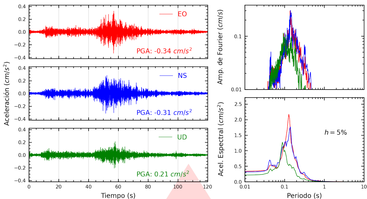
Figura A.7: Registros tiempo-historia, espectros de Fourier y de respuesta en las direcciones EO, NS y vertical de la estación CARAB. Sismo de Palpa, Palpa - Ica del 2025-11-25, 02:23:09 (Hora local)
