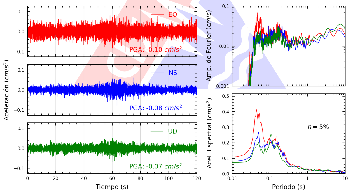
Figura A.28: Registros tiempo-historia, espectros de Fourier y de respuesta en las direcciones EO, NS y vertical de la estación INICT. Sismo de Palpa, Palpa - Ica del 2025-11-25, 02:23:09 (Hora local)
