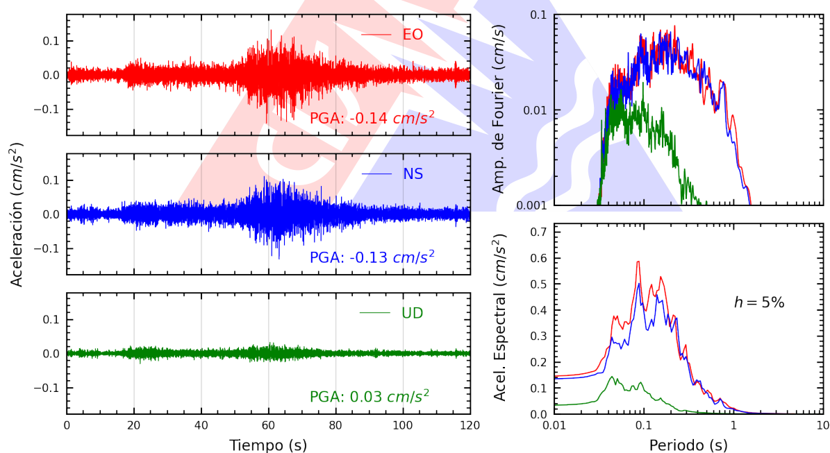
Figura A.20: Registros tiempo-historia, espectros de Fourier y de respuesta en las direcciones EO, NS y vertical de la estación UCVAT. Sismo de Palpa, Palpa - Ica del 2025-11-25, 02:23:09 (Hora local)
