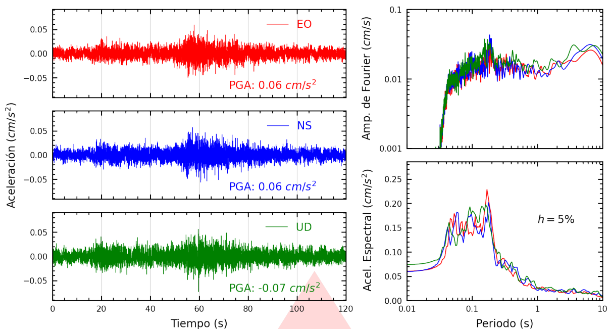
Figura A.33: Registros tiempo-historia, espectros de Fourier y de respuesta en las direcciones EO, NS y vertical de la estación UNFV. Sismo de Palpa, Palpa - Ica del 2025-11-25, 02:23:09 (Hora local)
