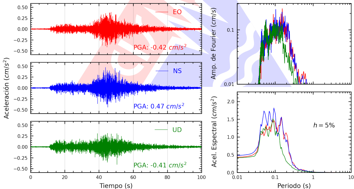
Figura A.2: Registros tiempo-historia, espectros de Fourier y de respuesta en las direcciones EO, NS y vertical de la estación ASIA. Sismo de Palpa, Palpa - Ica del 2025-11-25, 02:23:09 (Hora local)
