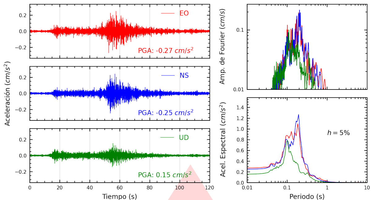
Figura A.9: Registros tiempo-historia, espectros de Fourier y de respuesta en las direcciones EO, NS y vertical de la estación SCCHO. Sismo de Palpa, Palpa - Ica del 2025-11-25, 02:23:09 (Hora local)
