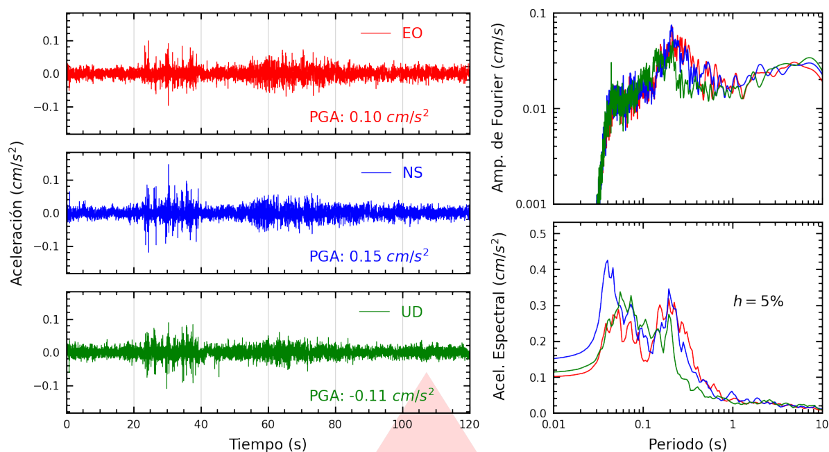
Figura A.19: Registros tiempo-historia, espectros de Fourier y de respuesta en las direcciones EO, NS y vertical de la estación DSML. Sismo de Palpa, Palpa - Ica del 2025-11-25, 02:23:09 (Hora local)
