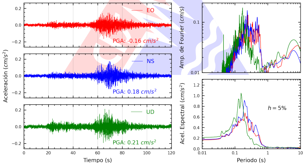
Figura A.14: Registros tiempo-historia, espectros de Fourier y de respuesta en las direcciones EO, NS y vertical de la estación MDPP. Sismo de Palpa, Palpa - Ica del 2025-11-25, 02:23:09 (Hora local)
