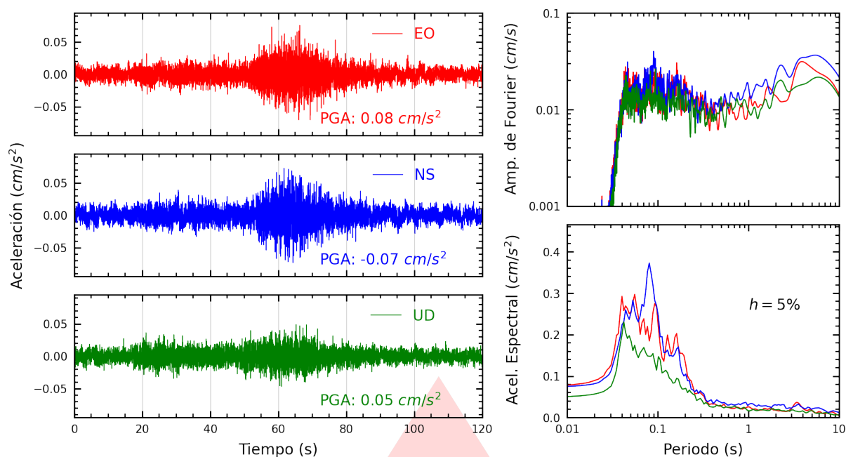
Figura A.31: Registros tiempo-historia, espectros de Fourier y de respuesta en las direcciones EO, NS y vertical de la estación SJLCE. Sismo de Palpa, Palpa - Ica del 2025-11-25, 02:23:09 (Hora local)
