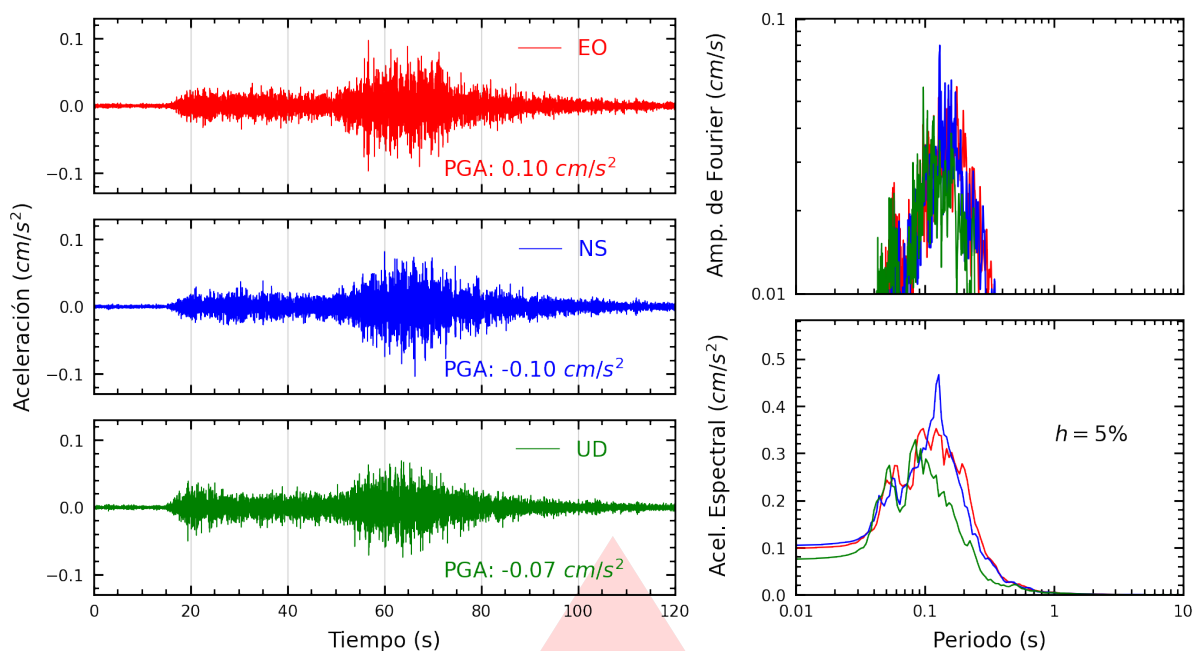
Figura A.27: Registros tiempo-historia, espectros de Fourier y de respuesta en las direcciones EO, NS y vertical de la estación JALV2. Sismo de Palpa, Palpa - Ica del 2025-11-25, 02:23:09 (Hora local)
