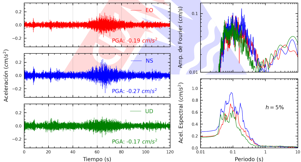
Figura A.10: Registros tiempo-historia, espectros de Fourier y de respuesta en las direcciones EO, NS y vertical de la estación SJLSC. Sismo de Palpa, Palpa - Ica del 2025-11-25, 02:23:09 (Hora local)
