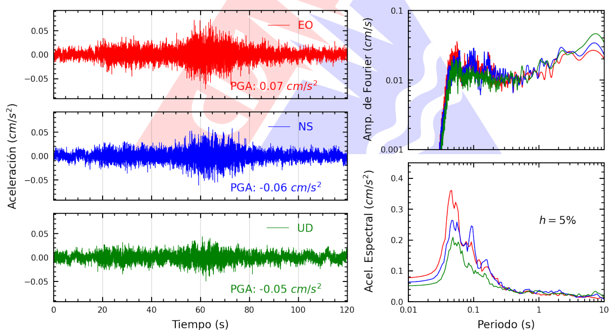
Figura A.32: Registros tiempo-historia, espectros de Fourier y de respuesta en las direcciones EO, NS y vertical de la estación UCSS. Sismo de Palpa, Palpa - Ica del 2025-11-25, 02:23:09 (Hora local)
