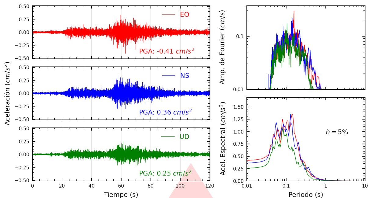
Figura A.3: Registros tiempo-historia, espectros de Fourier y de respuesta en las direcciones EO, NS y vertical de la estación PHERM. Sismo de Palpa, Palpa - Ica del 2025-11-25, 02:23:09 (Hora local)
