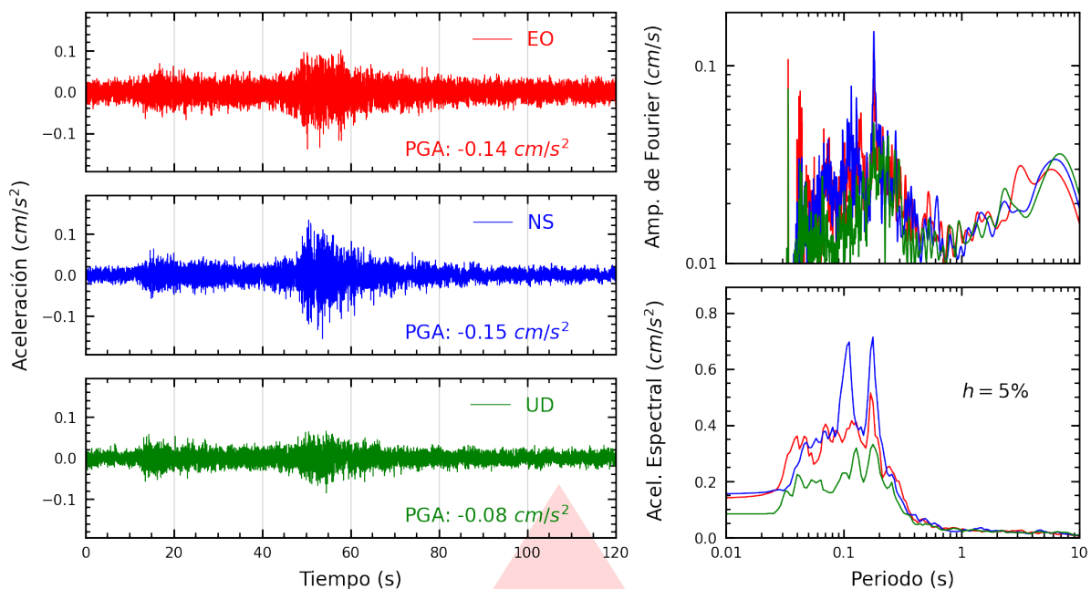
Figura A.17: Registros tiempo-historia, espectros de Fourier y de respuesta en las direcciones EO, NS y vertical de la estación UPCVI. Sismo de Palpa, Palpa - Ica del 2025-11-25, 02:23:09 (Hora local)
