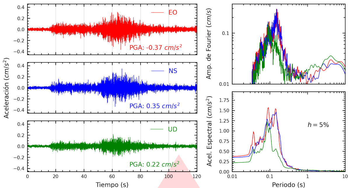
Figura A.5: Registros tiempo-historia, espectros de Fourier y de respuesta en las direcciones EO, NS y vertical de la estación USILM. Sismo de Palpa, Palpa - Ica del 2025-11-25, 02:23:09 (Hora local)
