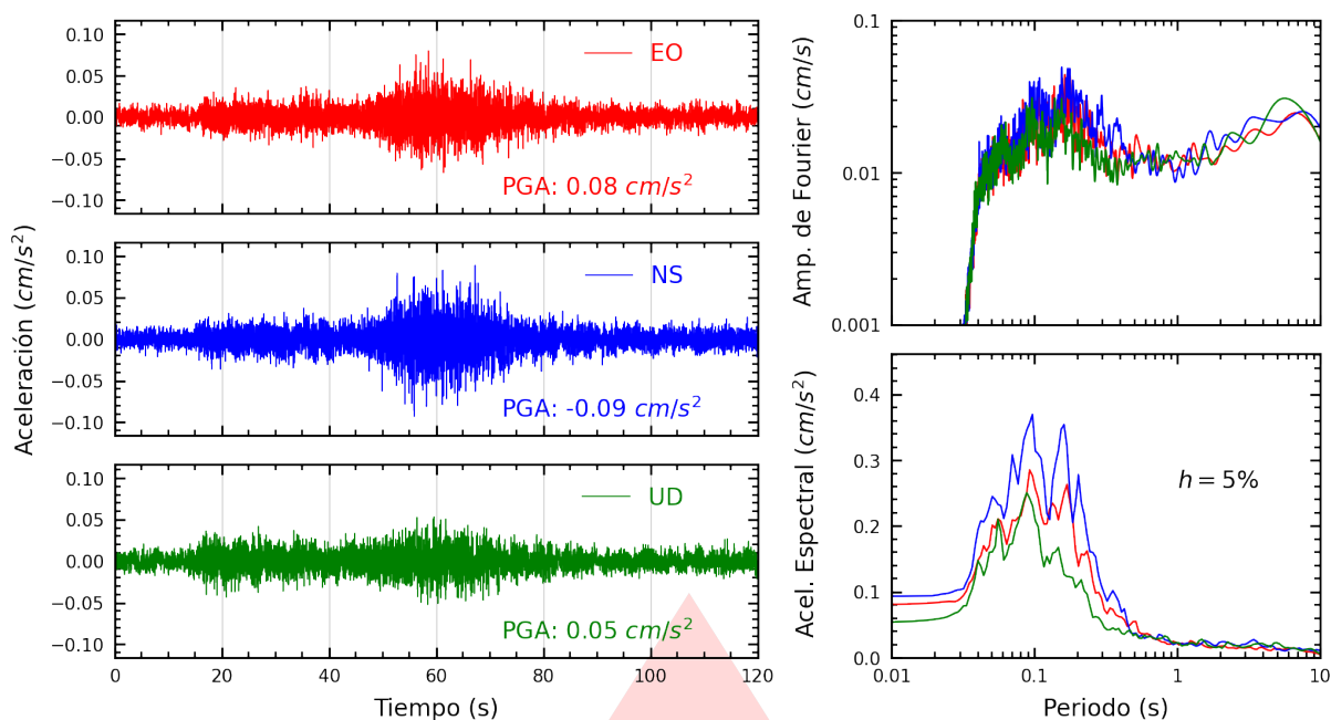
Figura A.29: Registros tiempo-historia, espectros de Fourier y de respuesta en las direcciones EO, NS y vertical de la estación SERVI. Sismo de Palpa, Palpa - Ica del 2025-11-25, 02:23:09 (Hora local)
