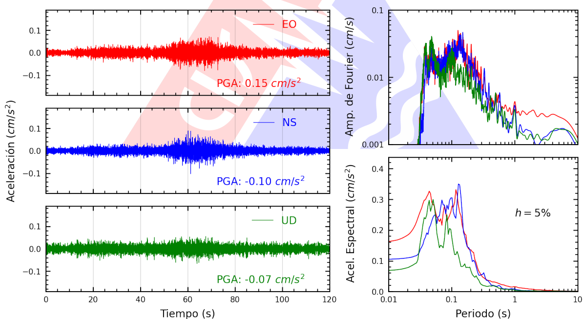
Figura A.18: Registros tiempo-historia, espectros de Fourier y de respuesta en las direcciones EO, NS y vertical de la estación ATARJ. Sismo de Palpa, Palpa - Ica del 2025-11-25, 02:23:09 (Hora local)
