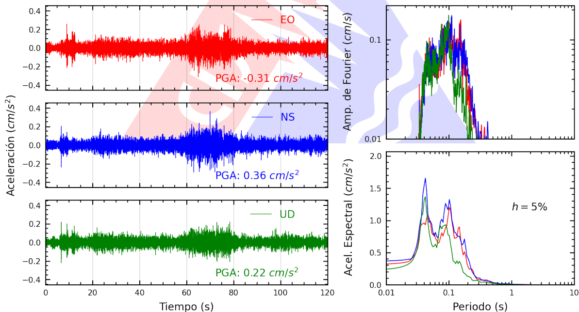
Figura A.6: Registros tiempo-historia, espectros de Fourier y de respuesta en las direcciones EO, NS y vertical de la estación SROSA. Sismo de Palpa, Palpa - Ica del 2025-11-25, 02:23:09 (Hora local)
