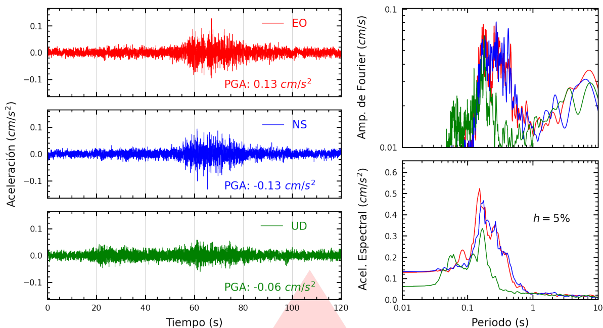
Figura A.21: Registros tiempo-historia, espectros de Fourier y de respuesta en las direcciones EO, NS y vertical de la estación ACAPU. Sismo de Palpa, Palpa - Ica del 2025-11-25, 02:23:09 (Hora local)
