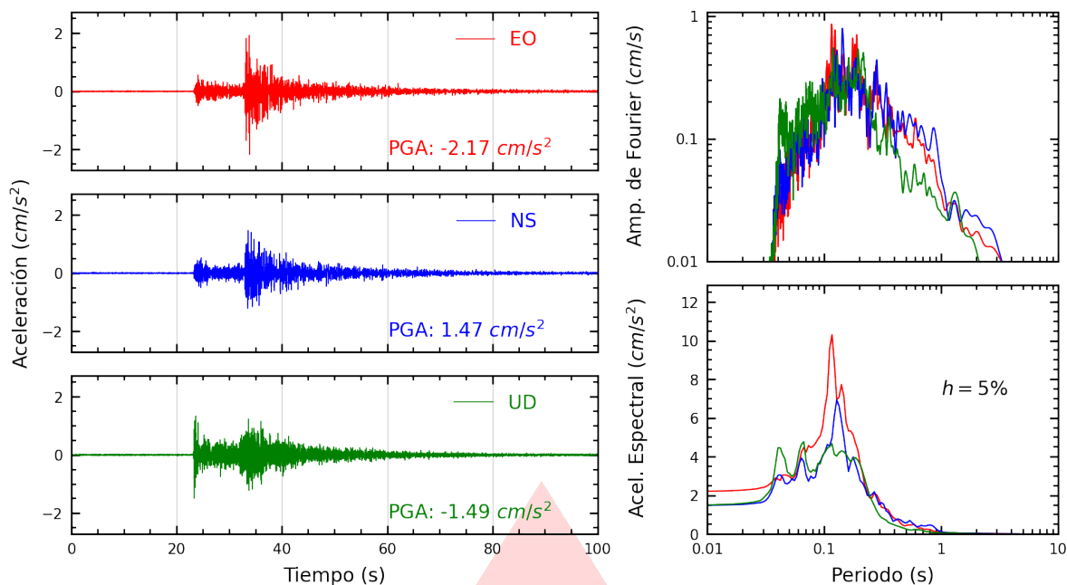
Figura A.1: Registros tiempo-historia, espectros de Fourier y de respuesta en las direcciones EO, NS y vertical de la estación UNICA. Sismo de Palpa, Palpa - Ica del 2025-11-25, 02:23:09 (Hora local)
