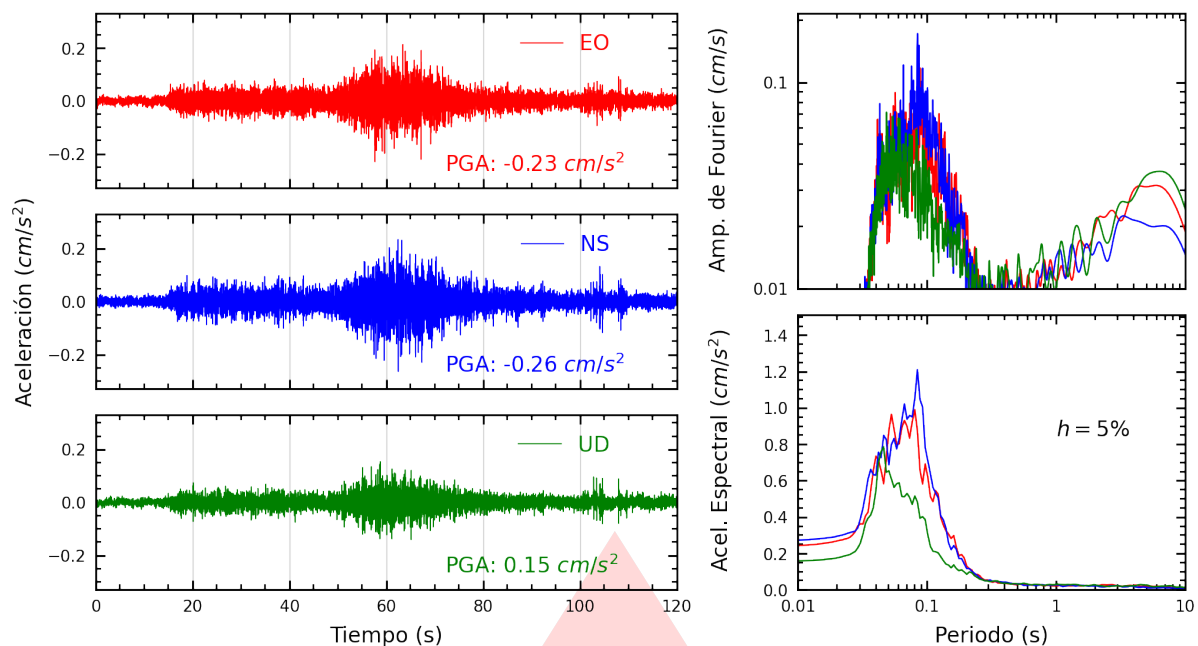
Figura A.11: Registros tiempo-historia, espectros de Fourier y de respuesta en las direcciones EO, NS y vertical de la estación JOSEO. Sismo de Palpa, Palpa - Ica del 2025-11-25, 02:23:09 (Hora local)
