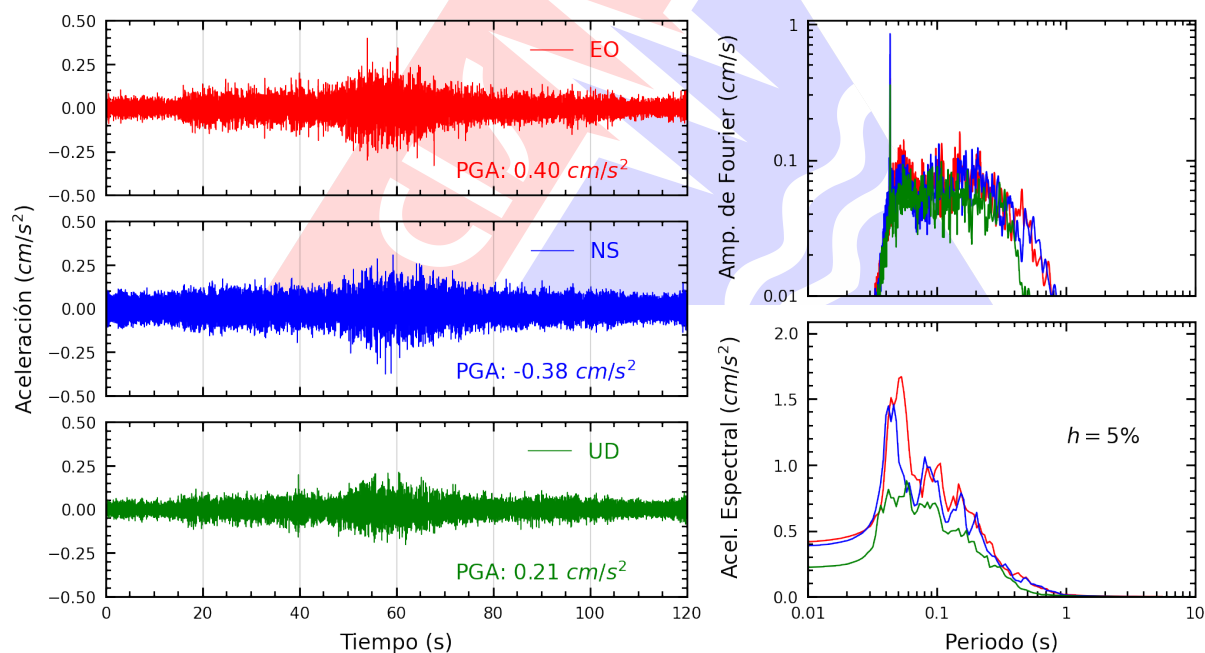
Figura A.4: Registros tiempo-historia, espectros de Fourier y de respuesta en las direcciones EO, NS y vertical de la estación UNTEL. Sismo de Palpa, Palpa - Ica del 2025-11-25, 02:23:09 (Hora local)
