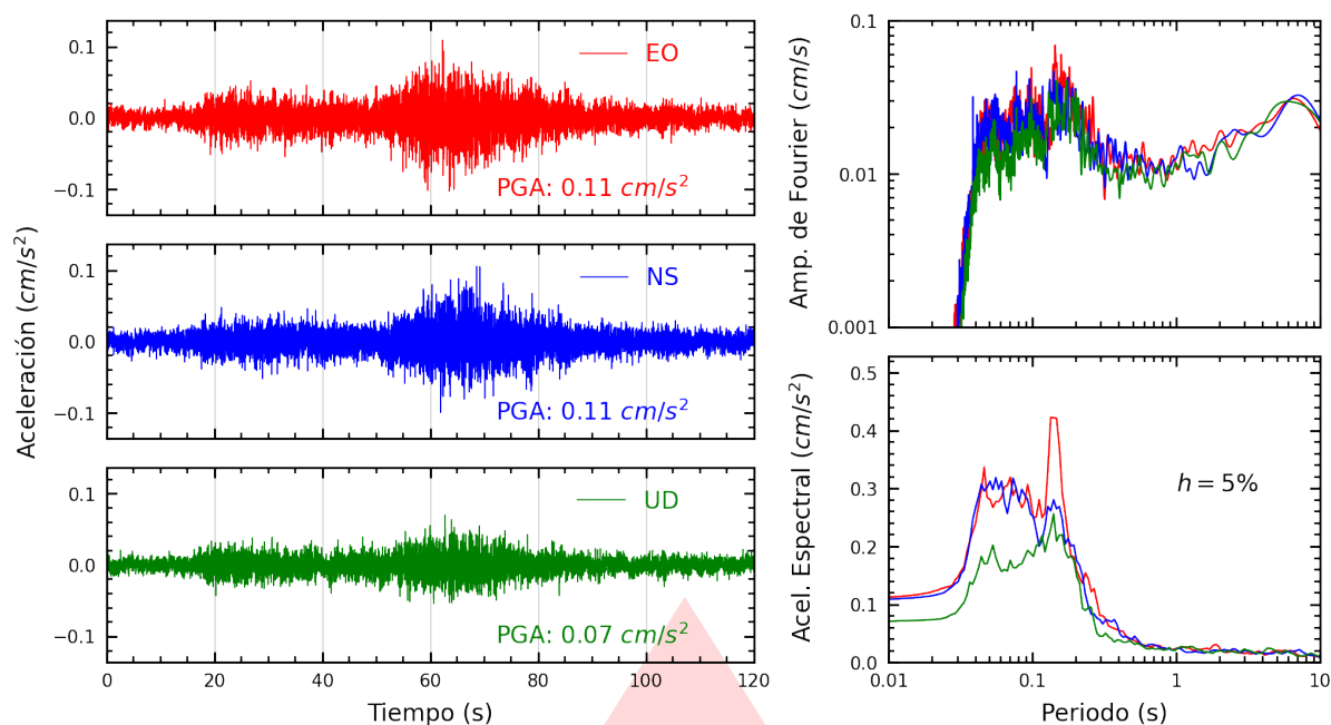
Figura A.25: Registros tiempo-historia, espectros de Fourier y de respuesta en las direcciones EO, NS y vertical de la estación FICPE. Sismo de Palpa, Palpa - Ica del 2025-11-25, 02:23:09 (Hora local)
