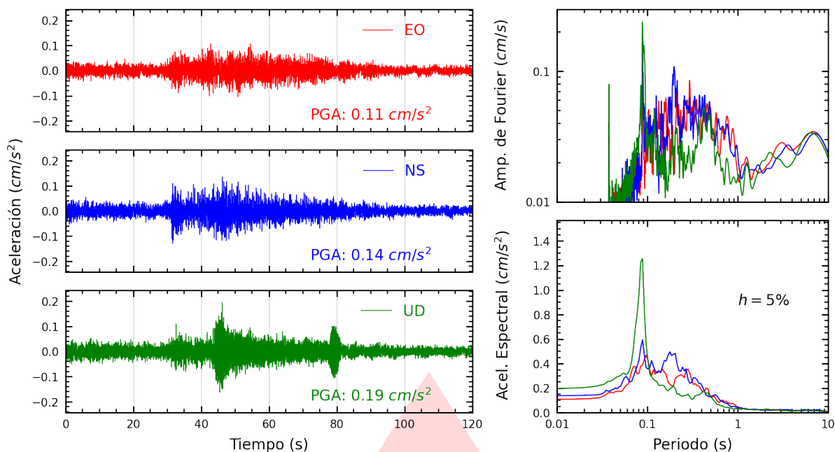
Figura A.7: Registros tiempo-historia, espectros de Fourier y de respuesta en las direcciones EO, NS y vertical de la estación SOCHO. Sismo de Atico, Caravelí - Arequipa del 2025-11-25, 04:57:04 (Hora local)
