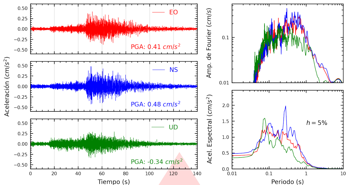
Figura A.1: Registros tiempo-historia, espectros de Fourier y de respuesta en las direcciones EO, NS y vertical de la estación UNICA. Sismo de Atico, Caravelí - Arequipa del 2025-11-25, 04:57:04 (Hora local)
