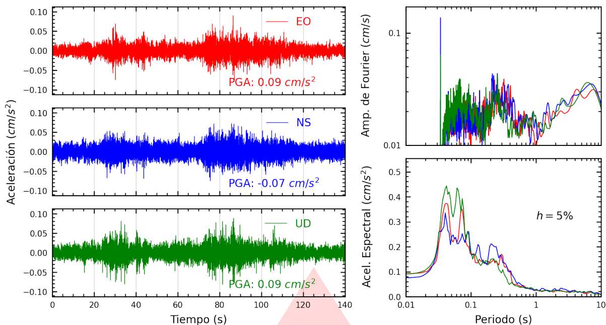
Figura A.13: Registros tiempo-historia, espectros de Fourier y de respuesta en las direcciones EO, NS y vertical de la estación USMP. Sismo de Atico, Caravelí - Arequipa del 2025-11-25, 04:57:04 (Hora local)
