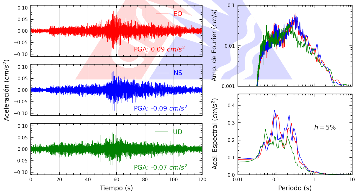
Figura A.14: Registros tiempo-historia, espectros de Fourier y de respuesta en las direcciones EO, NS y vertical de la estación UJB2. Sismo de Atico, Caravelí - Arequipa del 2025-11-25, 04:57:04 (Hora local)
