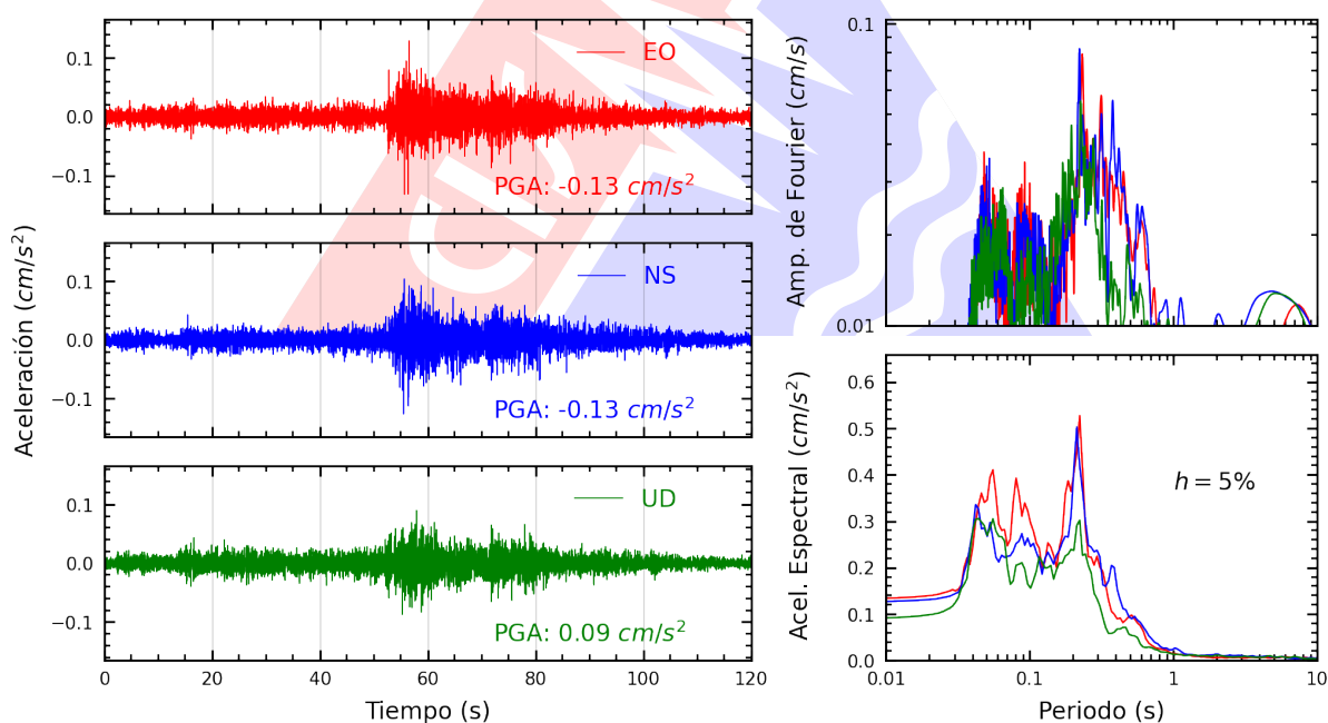
Figura A.10: Registros tiempo-historia, espectros de Fourier y de respuesta en las direcciones EO, NS y vertical de la estación CREY. Sismo de Atico, Caravelí - Arequipa del 2025-11-25, 04:57:04 (Hora local)
