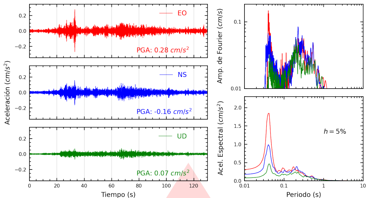
Figura A.3: Registros tiempo-historia, espectros de Fourier y de respuesta en las direcciones EO, NS y vertical de la estación UPTAC. Sismo de Atico, Caravelí - Arequipa del 2025-11-25, 04:57:04 (Hora local)
