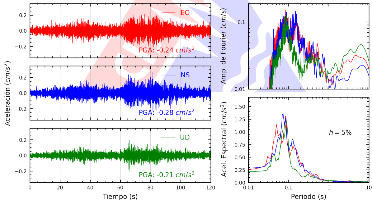
Figura A.2: Registros tiempo-historia, espectros de Fourier y de respuesta en las direcciones EO, NS y vertical de la estación USILM. Sismo de Atico, Caravelí - Arequipa del 2025-11-25, 04:57:04 (Hora local)
