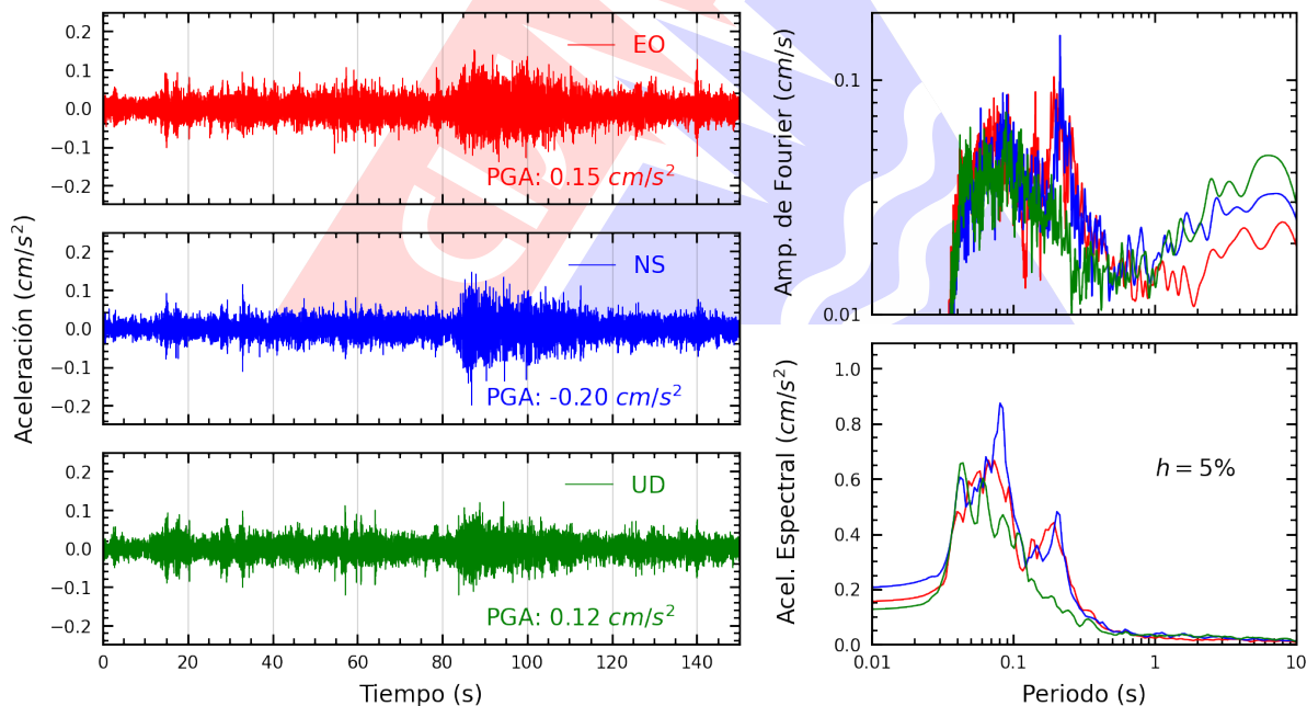
Figura A.6: Registros tiempo-historia, espectros de Fourier y de respuesta en las direcciones EO, NS y vertical de la estación INDEP. Sismo de Atico, Caravelí - Arequipa del 2025-11-25, 04:57:04 (Hora local)
