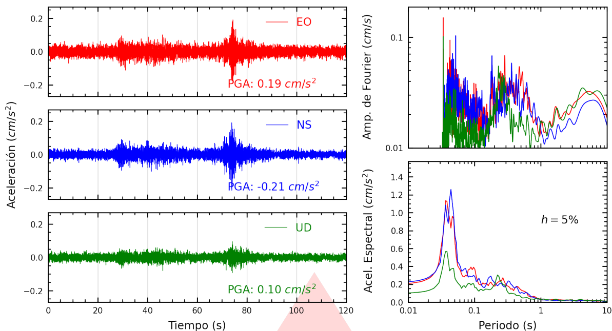
Figura A.5: Registros tiempo-historia, espectros de Fourier y de respuesta en las direcciones EO, NS y vertical de la estación UPCVI. Sismo de Atico, Caravelí - Arequipa del 2025-11-25, 04:57:04 (Hora local)
