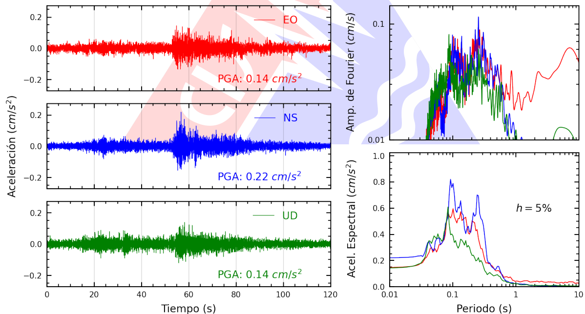
Figura A.4: Registros tiempo-historia, espectros de Fourier y de respuesta en las direcciones EO, NS y vertical de la estación UJB3. Sismo de Atico, Caravelí - Arequipa del 2025-11-25, 04:57:04 (Hora local)
