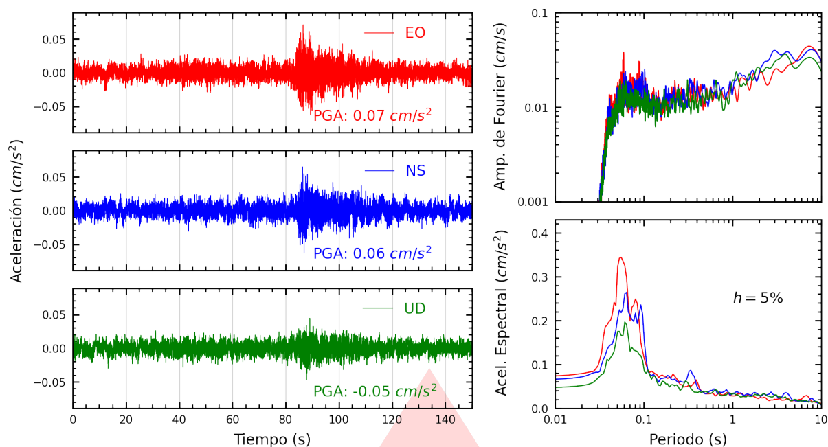
Figura A.15: Registros tiempo-historia, espectros de Fourier y de respuesta en las direcciones EO, NS y vertical de la estación UCSS. Sismo de Atico, Caravelí - Arequipa del 2025-11-25, 04:57:04 (Hora local)
