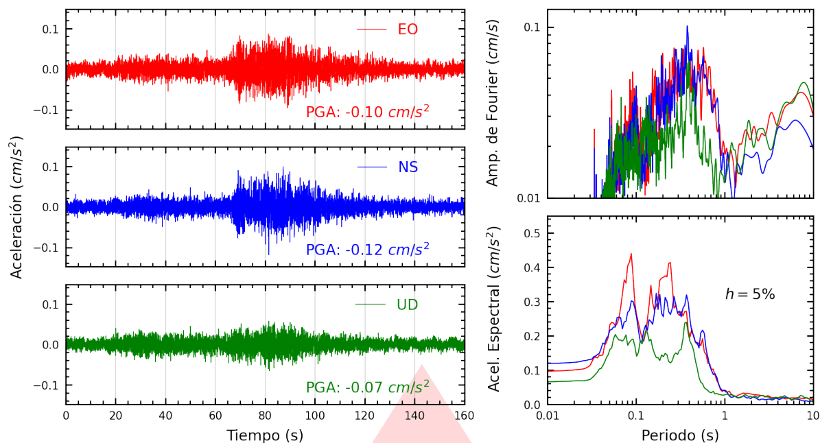
Figura A.11: Registros tiempo-historia, espectros de Fourier y de respuesta en las direcciones EO, NS y vertical de la estación USILP. Sismo de Atico, Caravelí - Arequipa del 2025-11-25, 04:57:04 (Hora local)
