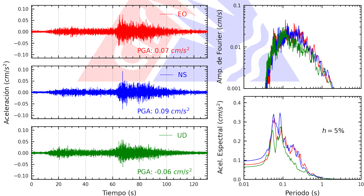
Figura A.12: Registros tiempo-historia, espectros de Fourier y de respuesta en las direcciones EO, NS y vertical de la estación JALV2. Sismo de Atico, Caravelí - Arequipa del 2025-11-25, 04:57:04 (Hora local)
