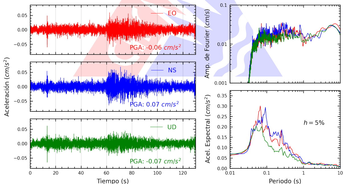
Figura A.16: Registros tiempo-historia, espectros de Fourier y de respuesta en las direcciones EO, NS y vertical de la estación SERVI. Sismo de Atico, Caravelí - Arequipa del 2025-11-25, 04:57:04 (Hora local)
