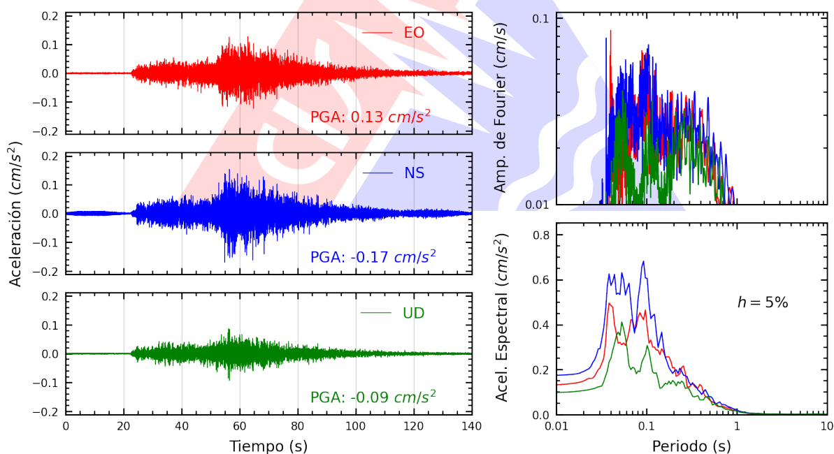
Figura A.8: Registros tiempo-historia, espectros de Fourier y de respuesta en las direcciones EO, NS y vertical de la estación UNAM. Sismo de Atico, Caravelí - Arequipa del 2025-11-25, 04:57:04 (Hora local)
