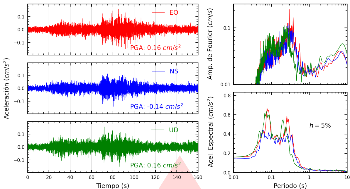
Figura A.9: Registros tiempo-historia, espectros de Fourier y de respuesta en las direcciones EO, NS y vertical de la estación SOVES. Sismo de Atico, Caravelí - Arequipa del 2025-11-25, 04:57:04 (Hora local)
