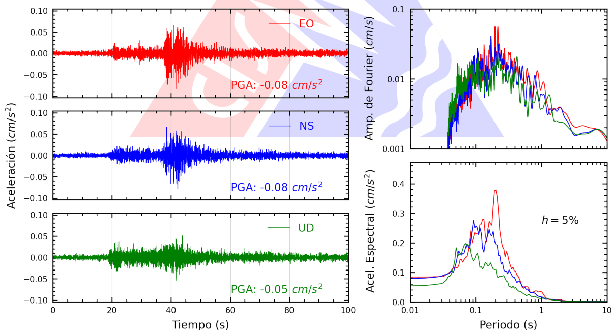
Figura A.4: Registros tiempo-historia, espectros de Fourier y de respuesta en las direcciones EO, NS y vertical de la estación UNC. Sismo de Ferreñafe, Ferreñafe - Lambayeque del 2025-12-01, 20:46:26 (Hora local)
