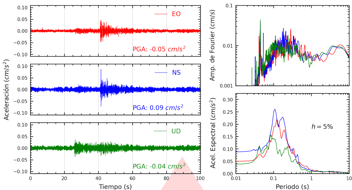
Figura A.3: Registros tiempo-historia, espectros de Fourier y de respuesta en las direcciones EO, NS y vertical de la estación UNJ. Sismo de Ferreñafe, Ferreñafe - Lambayeque del 2025-12-01, 20:46:26 (Hora local)
