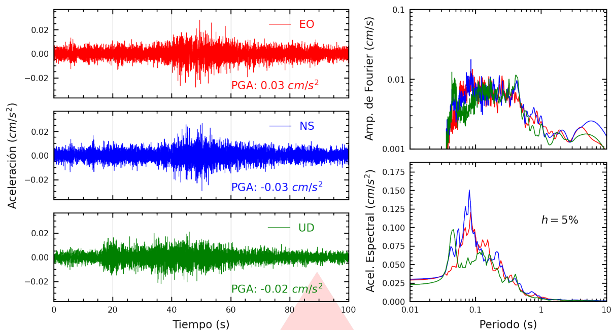
Figura A.5: Registros tiempo-historia, espectros de Fourier y de respuesta en las direcciones EO, NS y vertical de la estación UNF. Sismo de Ferreñafe, Ferreñafe - Lambayeque del 2025-12-01, 20:46:26 (Hora local)
