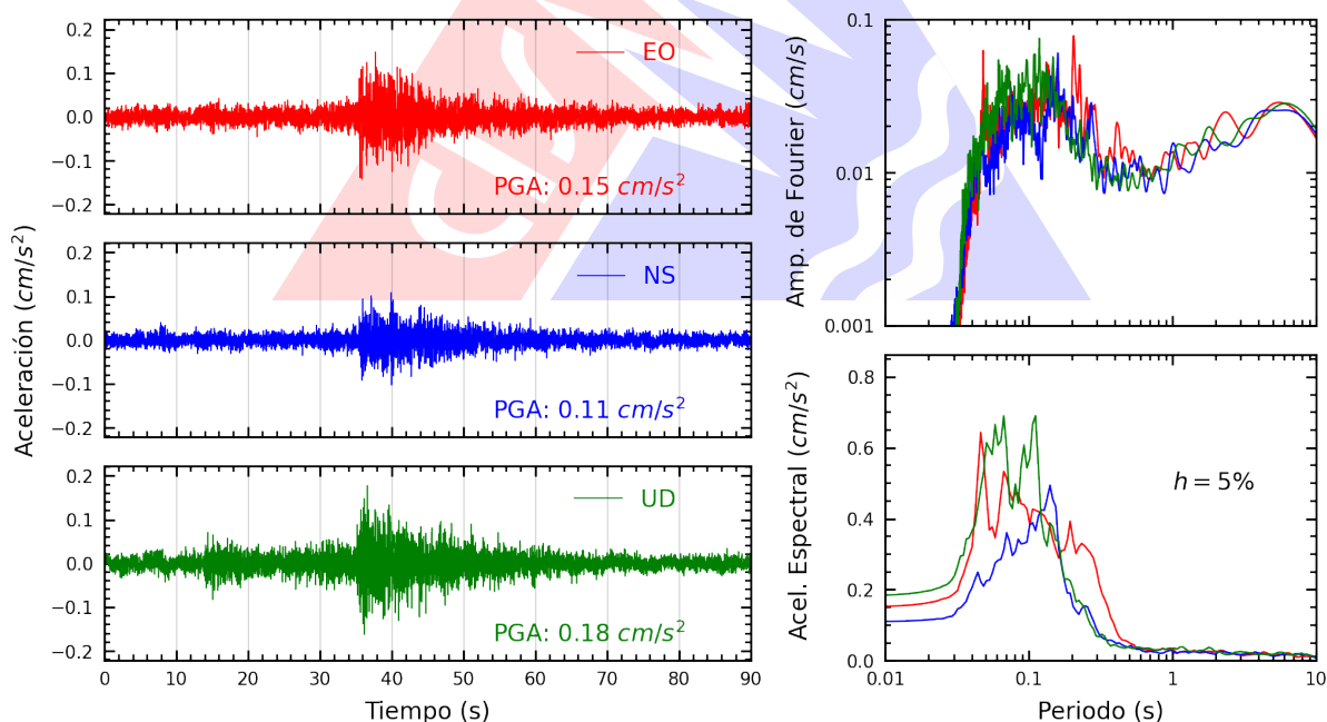
Figura A.2: Registros tiempo-historia, espectros de Fourier y de respuesta en las direcciones EO, NS y vertical de la estación UPAOT. Sismo de Ferreñafe, Ferreñafe - Lambayeque del 2025-12-01, 20:46:26 (Hora local)
