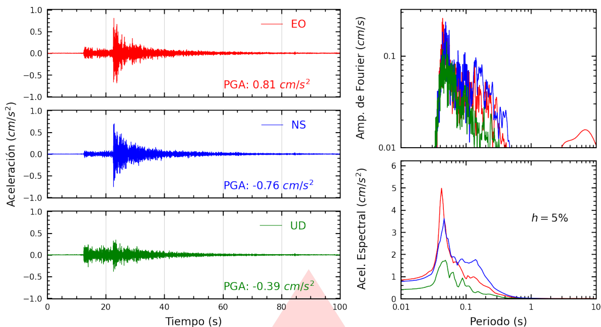
Figura A.1: Registros tiempo-historia, espectros de Fourier y de respuesta en las direcciones EO, NS y vertical de la estación SCCHI. Sismo de Ferreñafe, Ferreñafe - Lambayeque del 2025-12-01, 20:46:26 (Hora local)
