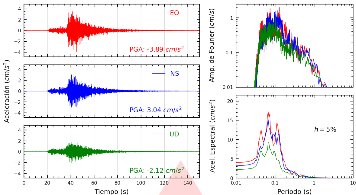
Figura A.25: Registros tiempo-historia, espectros de Fourier y de respuesta en las direcciones EO, NS y vertical de la estación ATARJ. Sismo de Supe Puerto, Barranca - Lima del 2025-12-26, 19:35:15 (Hora local)
