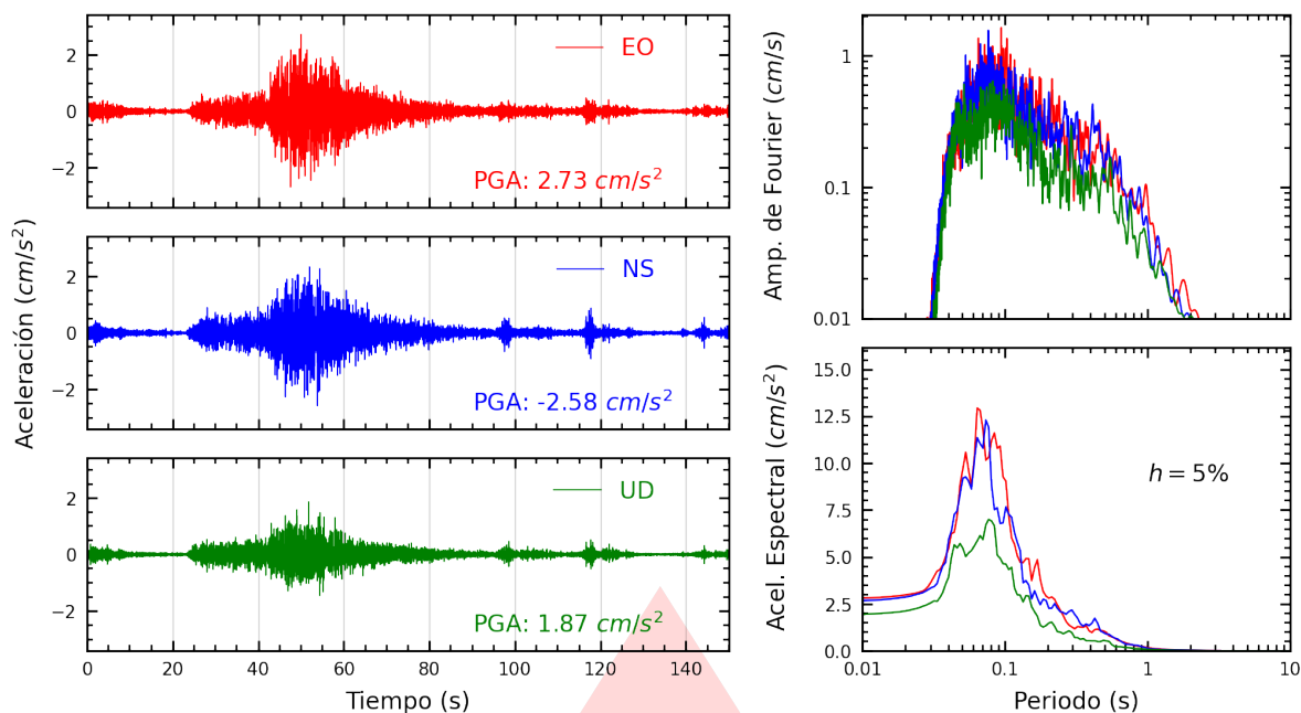
Figura A.33: Registros tiempo-historia, espectros de Fourier y de respuesta en las direcciones EO, NS y vertical de la estación PACHA. Sismo de Supe Puerto, Barranca - Lima del 2025-12-26, 19:35:15 (Hora local)
