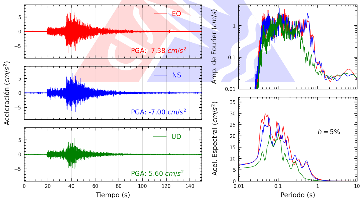
Figura A.10: Registros tiempo-historia, espectros de Fourier y de respuesta en las direcciones EO, NS y vertical de la estación OLIVO. Sismo de Supe Puerto, Barranca - Lima del 2025-12-26, 19:35:15 (Hora local)
