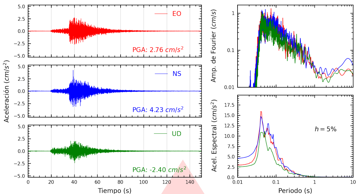
Figura A.21: Registros tiempo-historia, espectros de Fourier y de respuesta en las direcciones EO, NS y vertical de la estación SJLCE. Sismo de Supe Puerto, Barranca - Lima del 2025-12-26, 19:35:15 (Hora local)
