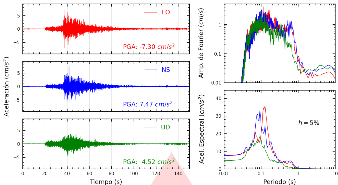
Figura A.9: Registros tiempo-historia, espectros de Fourier y de respuesta en las direcciones EO, NS y vertical de la estación SJLSV. Sismo de Supe Puerto, Barranca - Lima del 2025-12-26, 19:35:15 (Hora local)
