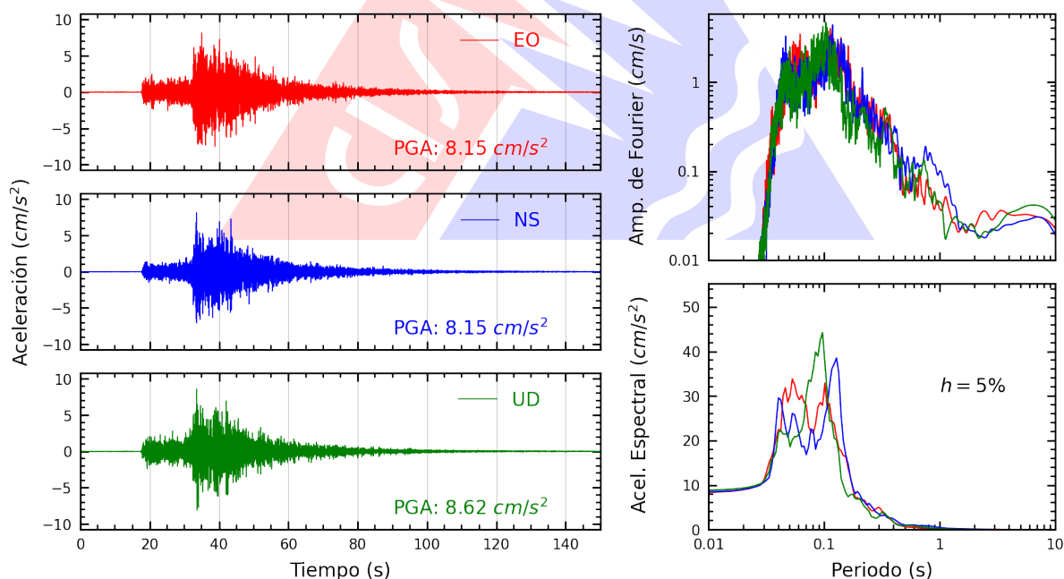
Figura A.6: Registros tiempo-historia, espectros de Fourier y de respuesta en las direcciones EO, NS y vertical de la estación AMORE. Sismo de Supe Puerto, Barranca - Lima del 2025-12-26, 19:35:15 (Hora local)
