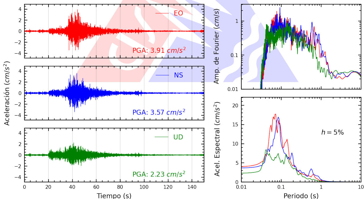
Figura A.24: Registros tiempo-historia, espectros de Fourier y de respuesta en las direcciones EO, NS y vertical de la estación UPCS. Sismo de Supe Puerto, Barranca - Lima del 2025-12-26, 19:35:15 (Hora local)
