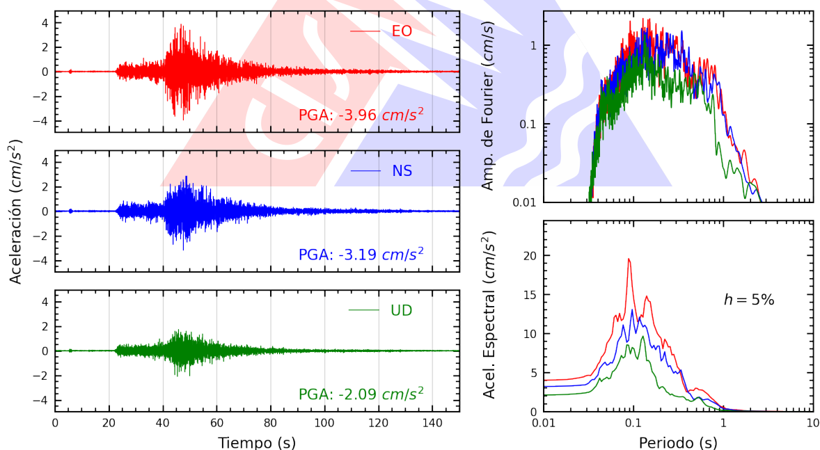
Figura A.22: Registros tiempo-historia, espectros de Fourier y de respuesta en las direcciones EO, NS y vertical de la estación BRISA. Sismo de Supe Puerto, Barranca - Lima del 2025-12-26, 19:35:15 (Hora local)
