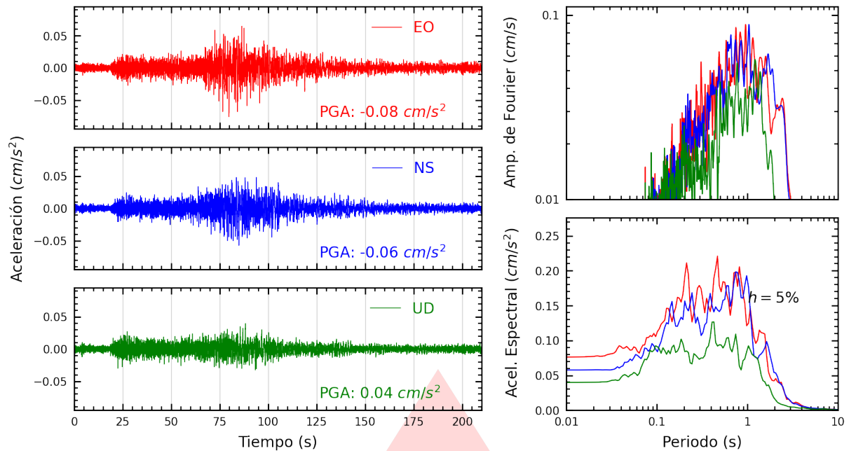
Figura A.45: Registros tiempo-historia, espectros de Fourier y de respuesta en las direcciones EO, NS y vertical de la estación UNC. Sismo de Supe Puerto, Barranca - Lima del 2025-12-26, 19:35:15 (Hora local)
