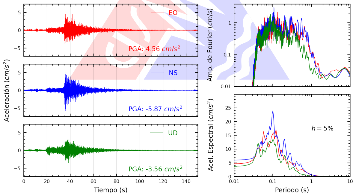
Figura A.12: Registros tiempo-historia, espectros de Fourier y de respuesta en las direcciones EO, NS y vertical de la estación MADRE. Sismo de Supe Puerto, Barranca - Lima del 2025-12-26, 19:35:15 (Hora local)
