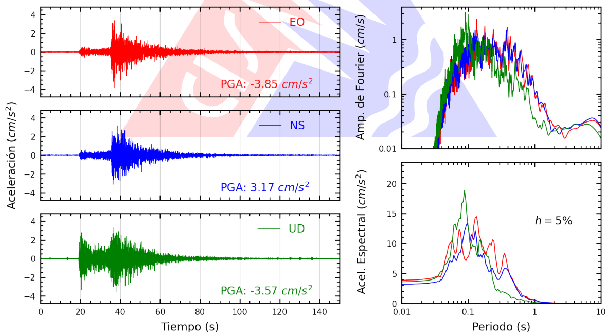
Figura A.26: Registros tiempo-historia, espectros de Fourier y de respuesta en las direcciones EO, NS y vertical de la estación RAMON. Sismo de Supe Puerto, Barranca - Lima del 2025-12-26, 19:35:15 (Hora local)
