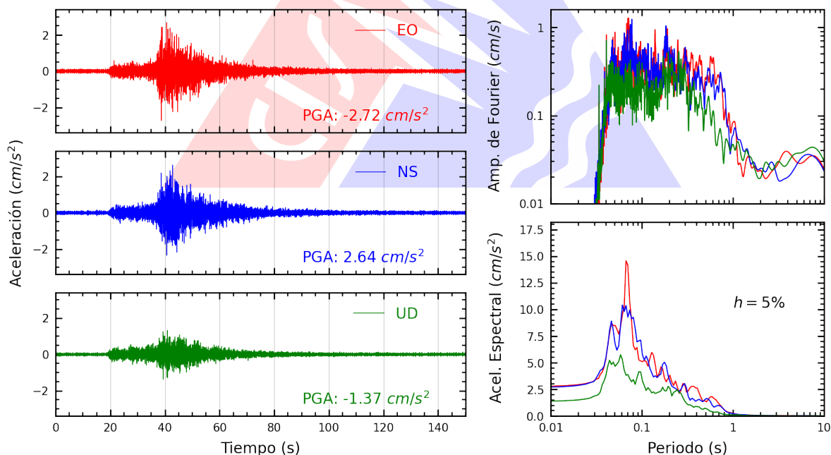
Figura A.34: Registros tiempo-historia, espectros de Fourier y de respuesta en las direcciones EO, NS y vertical de la estación UPCVI. Sismo de Supe Puerto, Barranca - Lima del 2025-12-26, 19:35:15 (Hora local)
