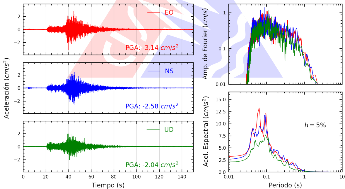
Figura A.32: Registros tiempo-historia, espectros de Fourier y de respuesta en las direcciones EO, NS y vertical de la estación BORJA. Sismo de Supe Puerto, Barranca - Lima del 2025-12-26, 19:35:15 (Hora local)
