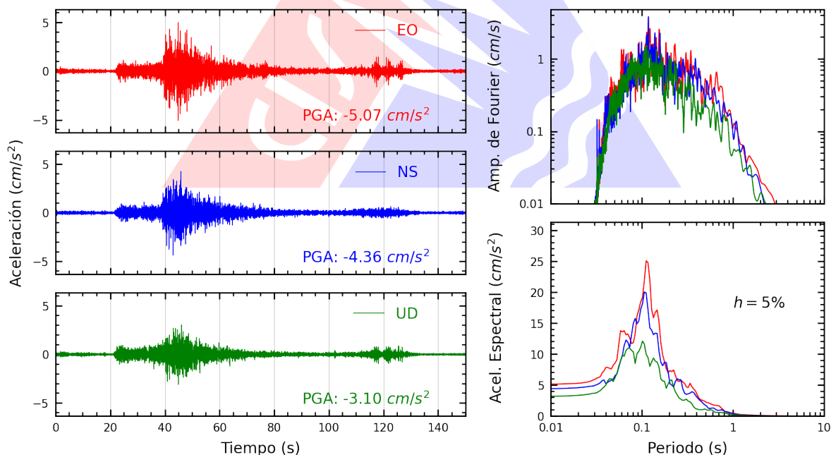
Figura A.14: Registros tiempo-historia, espectros de Fourier y de respuesta en las direcciones EO, NS y vertical de la estación SOBAR. Sismo de Supe Puerto, Barranca - Lima del 2025-12-26, 19:35:15 (Hora local)
