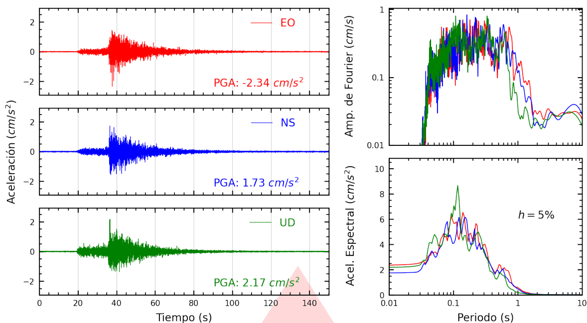
Figura A.39: Registros tiempo-historia, espectros de Fourier y de respuesta en las direcciones EO, NS y vertical de la estación BONDY. Sismo de Supe Puerto, Barranca - Lima del 2025-12-26, 19:35:15 (Hora local)
