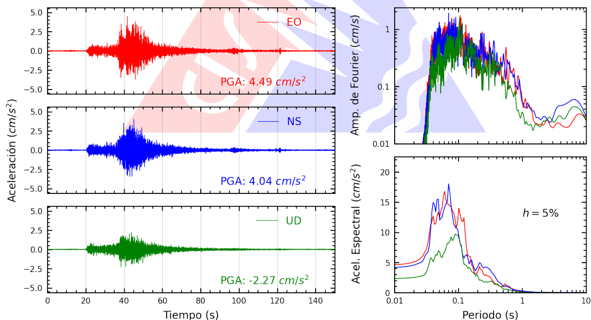
Figura A.18: Registros tiempo-historia, espectros de Fourier y de respuesta en las direcciones EO, NS y vertical de la estación CEPRE. Sismo de Supe Puerto, Barranca - Lima del 2025-12-26, 19:35:15 (Hora local)
