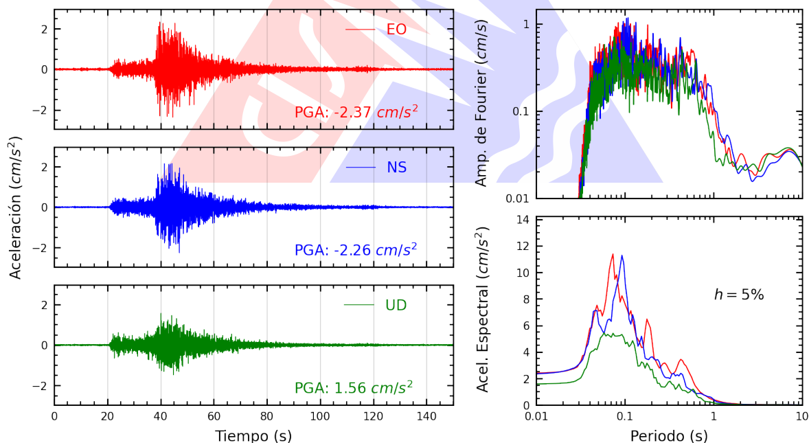
Figura A.38: Registros tiempo-historia, espectros de Fourier y de respuesta en las direcciones EO, NS y vertical de la estación INICT. Sismo de Supe Puerto, Barranca - Lima del 2025-12-26, 19:35:15 (Hora local)
