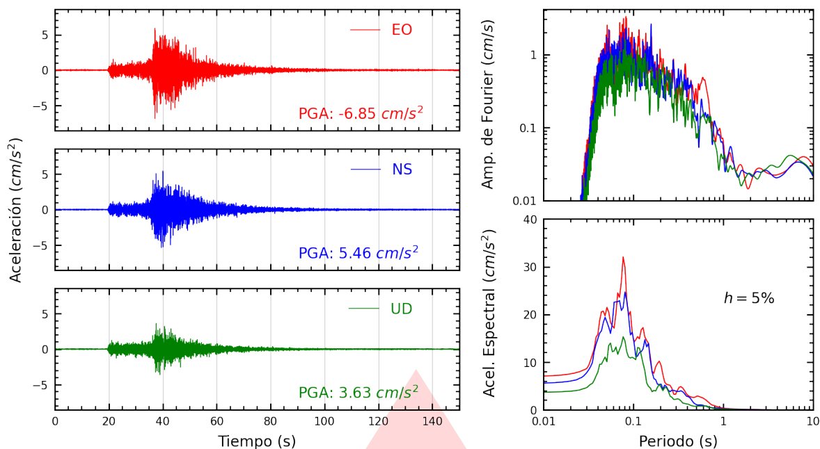
Figura A.11: Registros tiempo-historia, espectros de Fourier y de respuesta en las direcciones EO, NS y vertical de la estación FICPE. Sismo de Supe Puerto, Barranca - Lima del 2025-12-26, 19:35:15 (Hora local)
