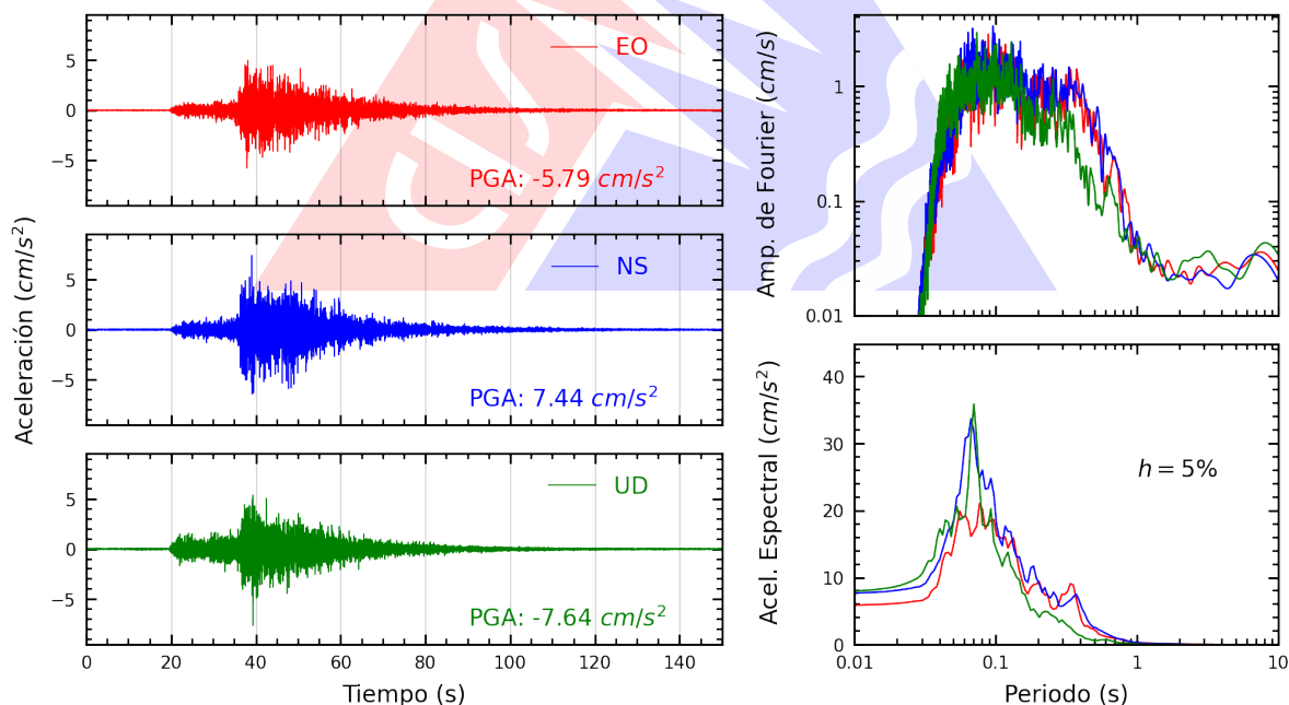
Figura A.8: Registros tiempo-historia, espectros de Fourier y de respuesta en las direcciones EO, NS y vertical de la estación SJLSC. Sismo de Supe Puerto, Barranca - Lima del 2025-12-26, 19:35:15 (Hora local)
