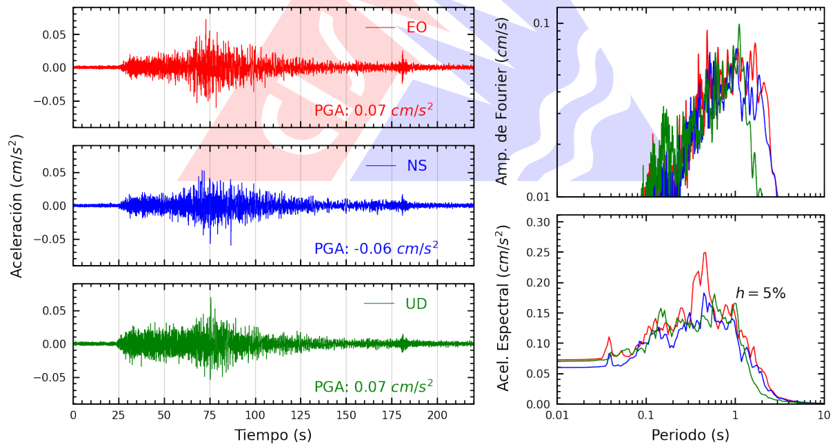
Figura A.46: Registros tiempo-historia, espectros de Fourier y de respuesta en las direcciones EO, NS y vertical de la estación UNCP. Sismo de Supe Puerto, Barranca - Lima del 2025-12-26, 19:35:15 (Hora local)
