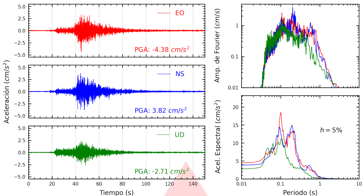
Figura A.19: Registros tiempo-historia, espectros de Fourier y de respuesta en las direcciones EO, NS y vertical de la estación SCCHO. Sismo de Supe Puerto, Barranca - Lima del 2025-12-26, 19:35:15 (Hora local)
