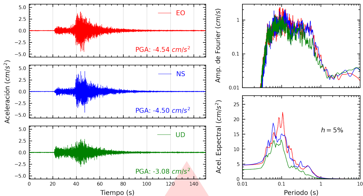
Figura A.17: Registros tiempo-historia, espectros de Fourier y de respuesta en las direcciones EO, NS y vertical de la estación URPE. Sismo de Supe Puerto, Barranca - Lima del 2025-12-26, 19:35:15 (Hora local)
