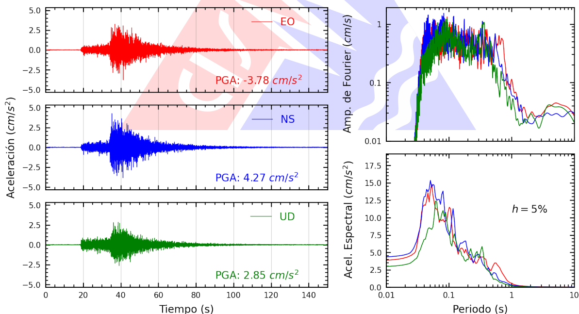
Figura A.20: Registros tiempo-historia, espectros de Fourier y de respuesta en las direcciones EO, NS y vertical de la estación COMAS. Sismo de Supe Puerto, Barranca - Lima del 2025-12-26, 19:35:15 (Hora local)
