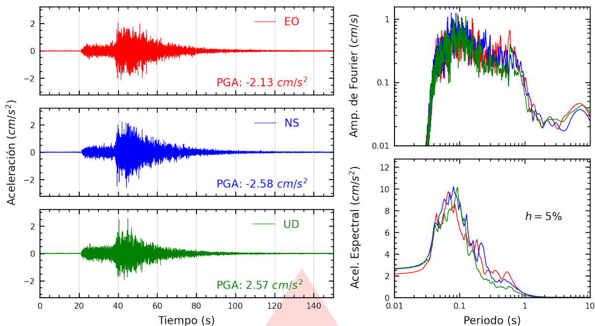
Figura A.37: Registros tiempo-historia, espectros de Fourier y de respuesta en las direcciones EO, NS y vertical de la estación SERVI. Sismo de Supe Puerto, Barranca - Lima del 2025-12-26, 19:35:15 (Hora local)
