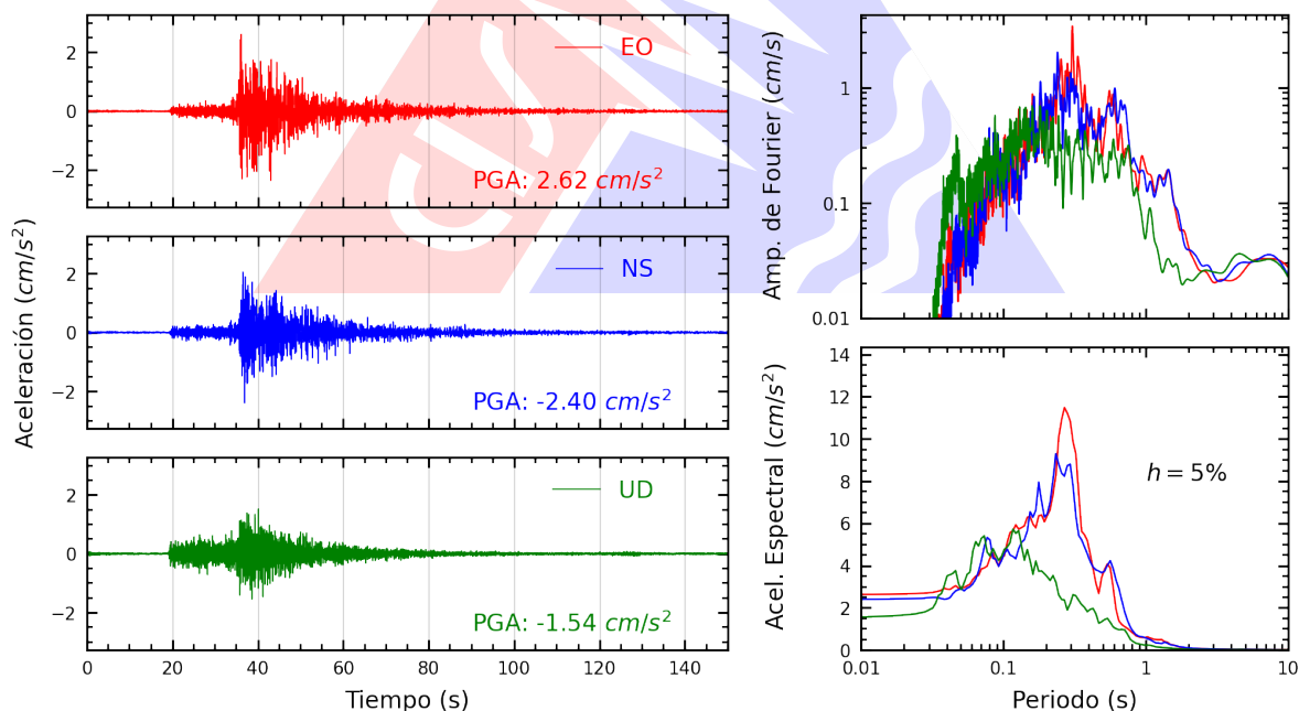
Figura A.36: Registros tiempo-historia, espectros de Fourier y de respuesta en las direcciones EO, NS y vertical de la estación DSMI. Sismo de Supe Puerto, Barranca - Lima del 2025-12-26, 19:35:15 (Hora local)
