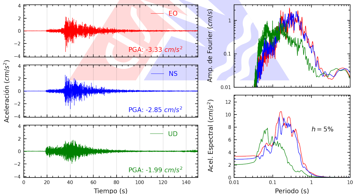
Figura A.30: Registros tiempo-historia, espectros de Fourier y de respuesta en las direcciones EO, NS y vertical de la estación ACAPU. Sismo de Supe Puerto, Barranca - Lima del 2025-12-26, 19:35:15 (Hora local)
