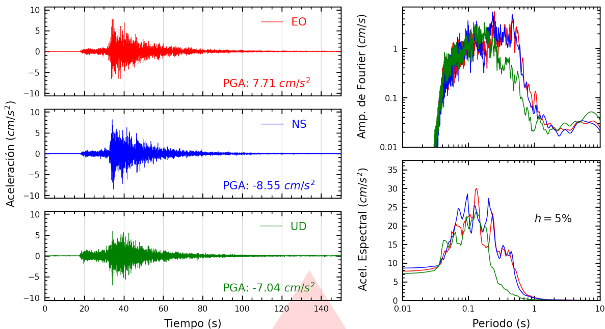
Figura A.7: Registros tiempo-historia, espectros de Fourier y de respuesta en las direcciones EO, NS y vertical de la estación MDPP. Sismo de Supe Puerto, Barranca - Lima del 2025-12-26, 19:35:15 (Hora local)
