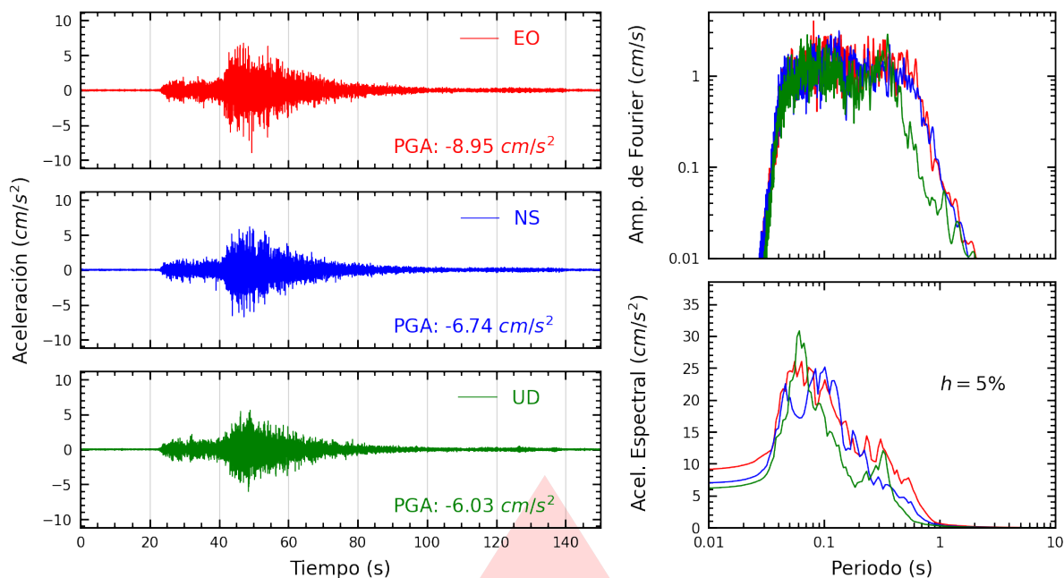
Figura A.5: Registros tiempo-historia, espectros de Fourier y de respuesta en las direcciones EO, NS y vertical de la estación UNTEL. Sismo de Supe Puerto, Barranca - Lima del 2025-12-26, 19:35:15 (Hora local)
