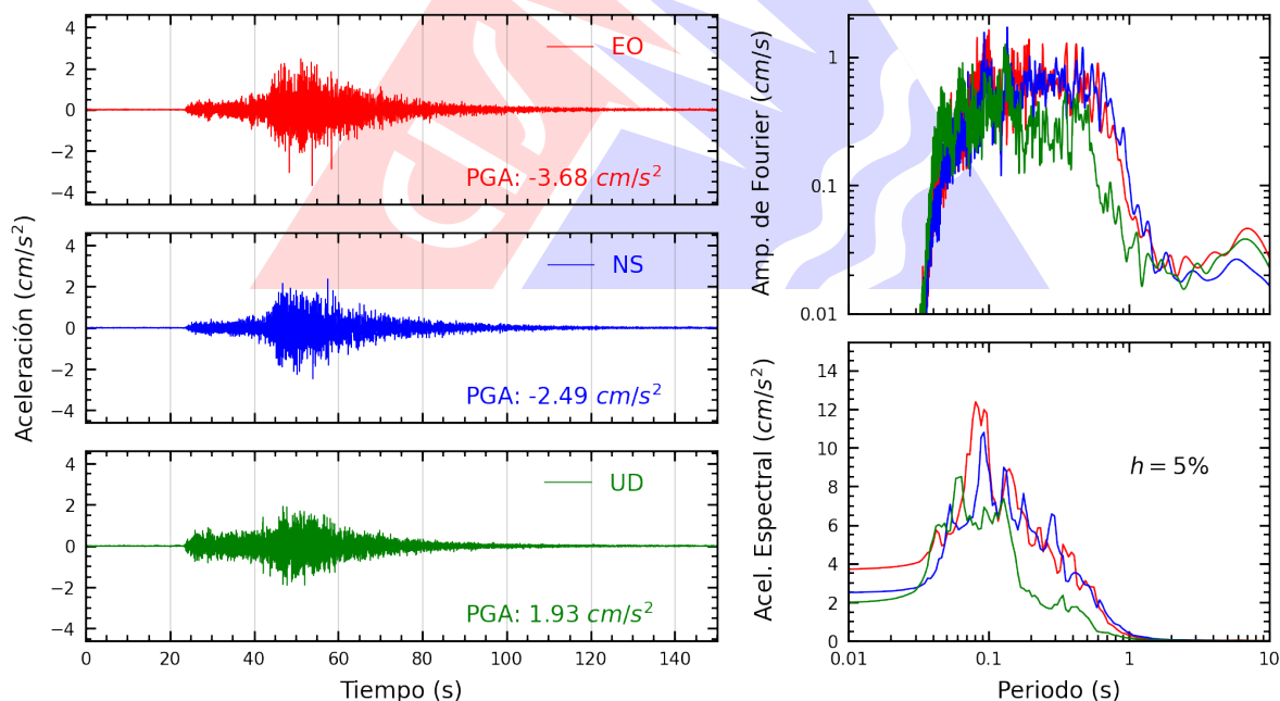
Figura A.28: Registros tiempo-historia, espectros de Fourier y de respuesta en las direcciones EO, NS y vertical de la estación USILP. Sismo de Supe Puerto, Barranca - Lima del 2025-12-26, 19:35:15 (Hora local)
