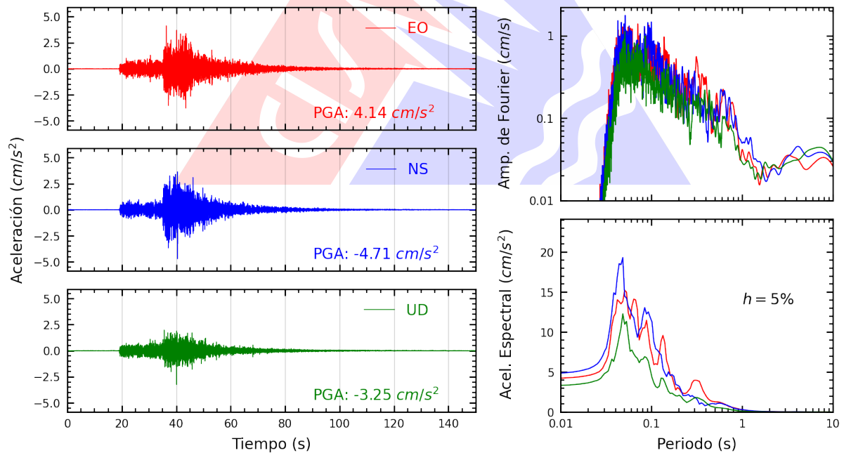
Figura A.16: Registros tiempo-historia, espectros de Fourier y de respuesta en las direcciones EO, NS y vertical de la estación UCSS. Sismo de Supe Puerto, Barranca - Lima del 2025-12-26, 19:35:15 (Hora local)
