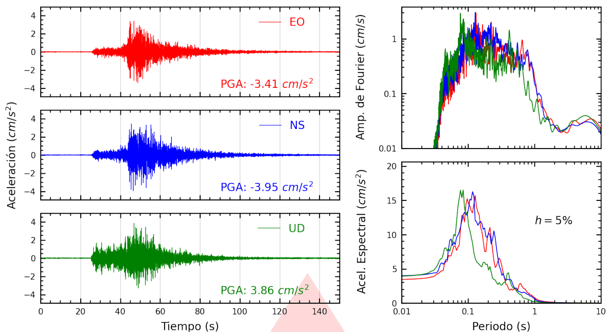
Figura A.23: Registros tiempo-historia, espectros de Fourier y de respuesta en las direcciones EO, NS y vertical de la estación SOCHO. Sismo de Supe Puerto, Barranca - Lima del 2025-12-26, 19:35:15 (Hora local)
