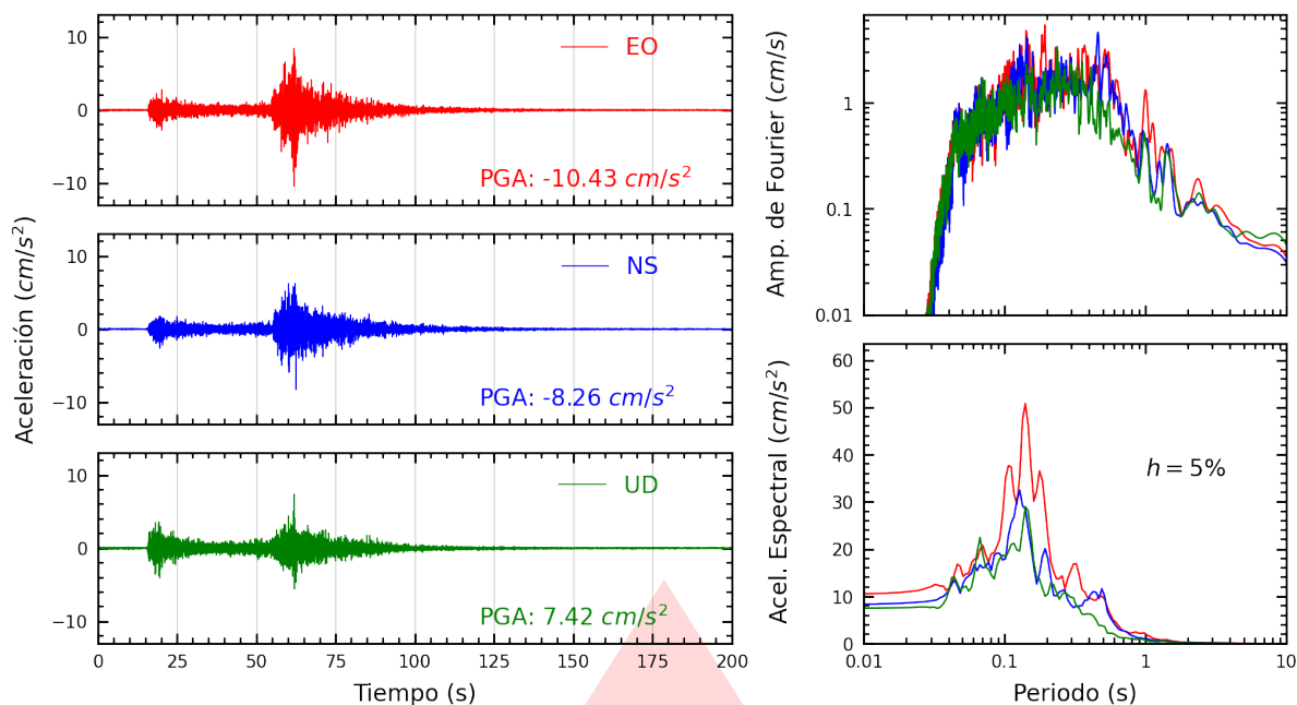
Figura A.15: Registros tiempo-historia, espectros de Fourier y de respuesta en las direcciones EO, NS y vertical de la estación URPE. Sismo de Chimbote, Santa - Áncash del 2025-12-27, 21:51:48 (Hora local)
