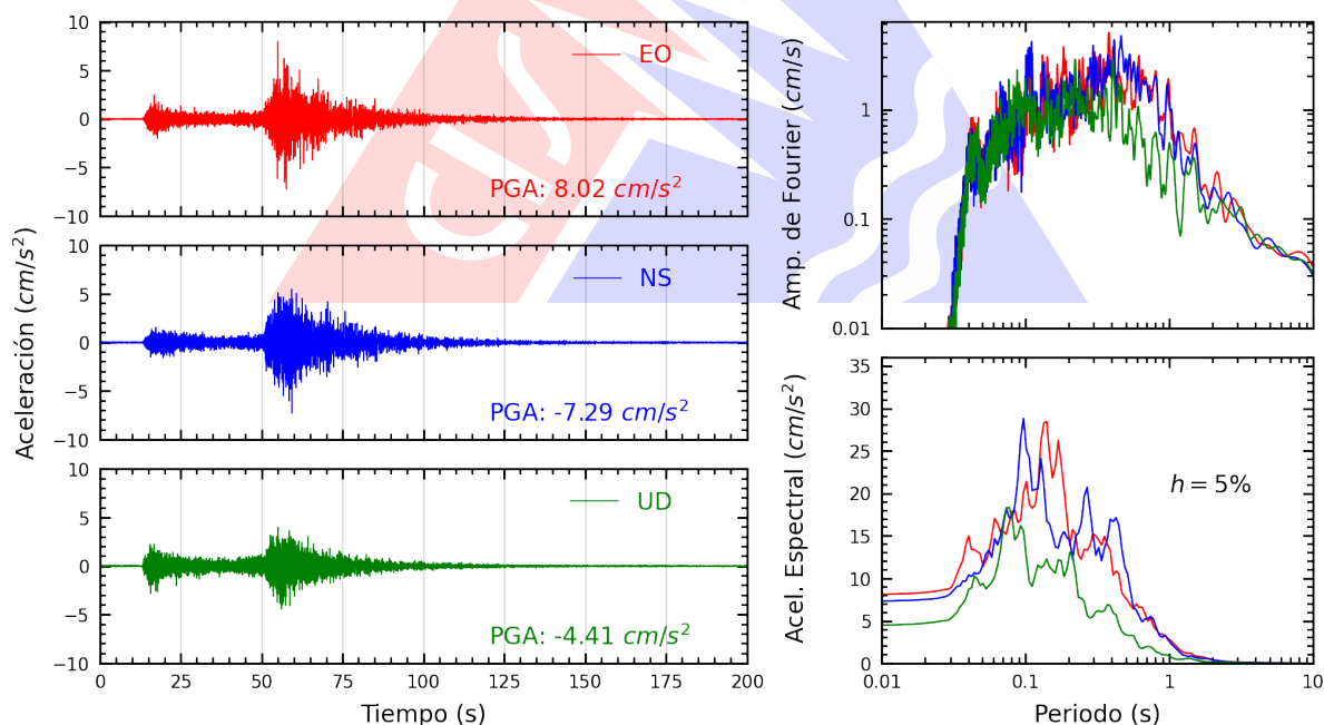
Figura A.20: Registros tiempo-historia, espectros de Fourier y de respuesta en las direcciones EO, NS y vertical de la estación MADRE. Sismo de Chimbote, Santa - Áncash del 2025-12-27, 21:51:48 (Hora local)
