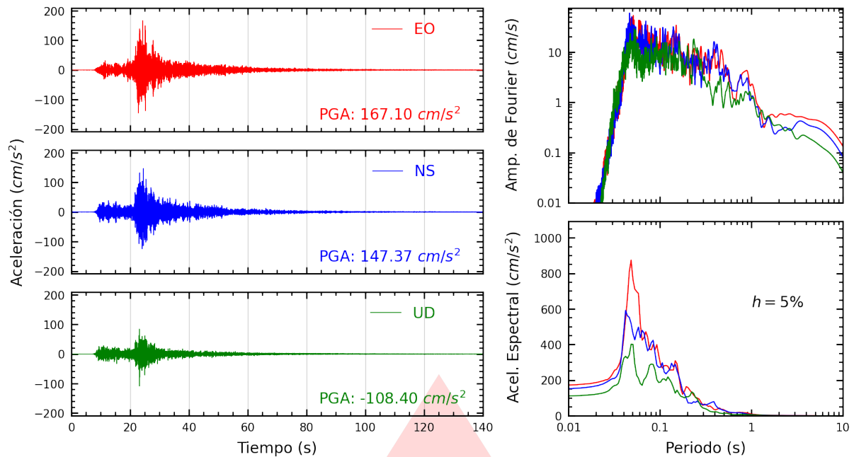
Figura A.3: Registros tiempo-historia, espectros de Fourier y de respuesta en las direcciones EO, NS y vertical de la estación SCTRU. Sismo de Chimbote, Santa - Áncash del 2025-12-27, 21:51:48 (Hora local)
