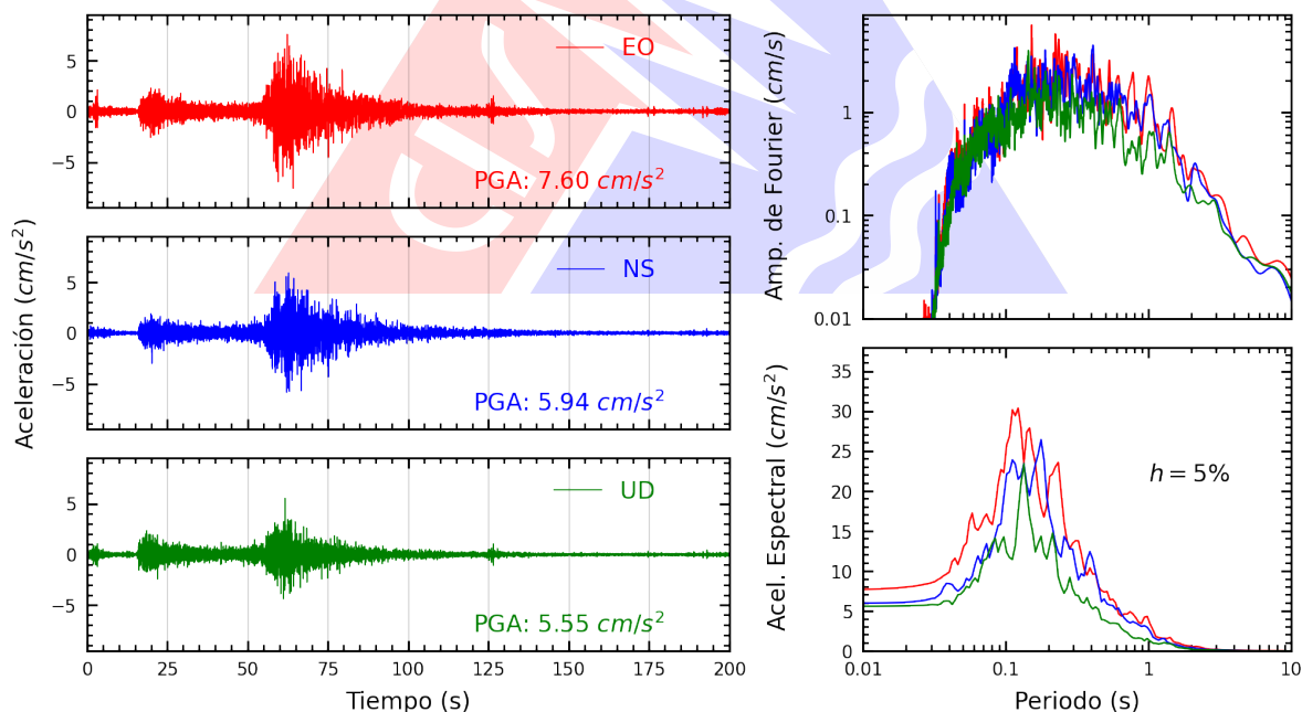
Figura A.22: Registros tiempo-historia, espectros de Fourier y de respuesta en las direcciones EO, NS y vertical de la estación SOBAR. Sismo de Chimbote, Santa - Áncash del 2025-12-27, 21:51:48 (Hora local)
