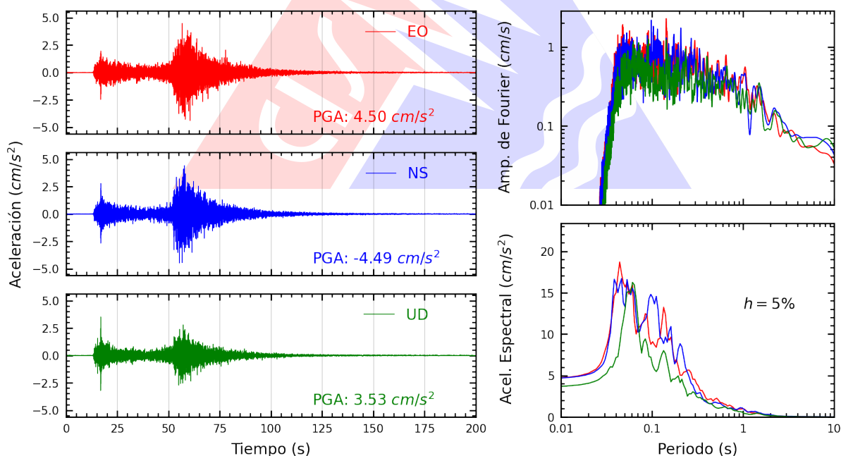
Figura A.38: Registros tiempo-historia, espectros de Fourier y de respuesta en las direcciones EO, NS y vertical de la estación UCSS. Sismo de Chimbote, Santa - Áncash del 2025-12-27, 21:51:48 (Hora local)
