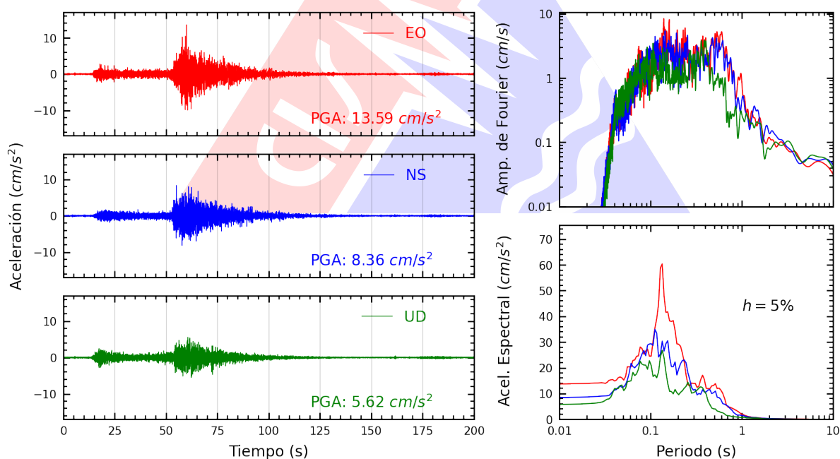
Figura A.10: Registros tiempo-historia, espectros de Fourier y de respuesta en las direcciones EO, NS y vertical de la estación SJLSV. Sismo de Chimbote, Santa - Áncash del 2025-12-27, 21:51:48 (Hora local)
