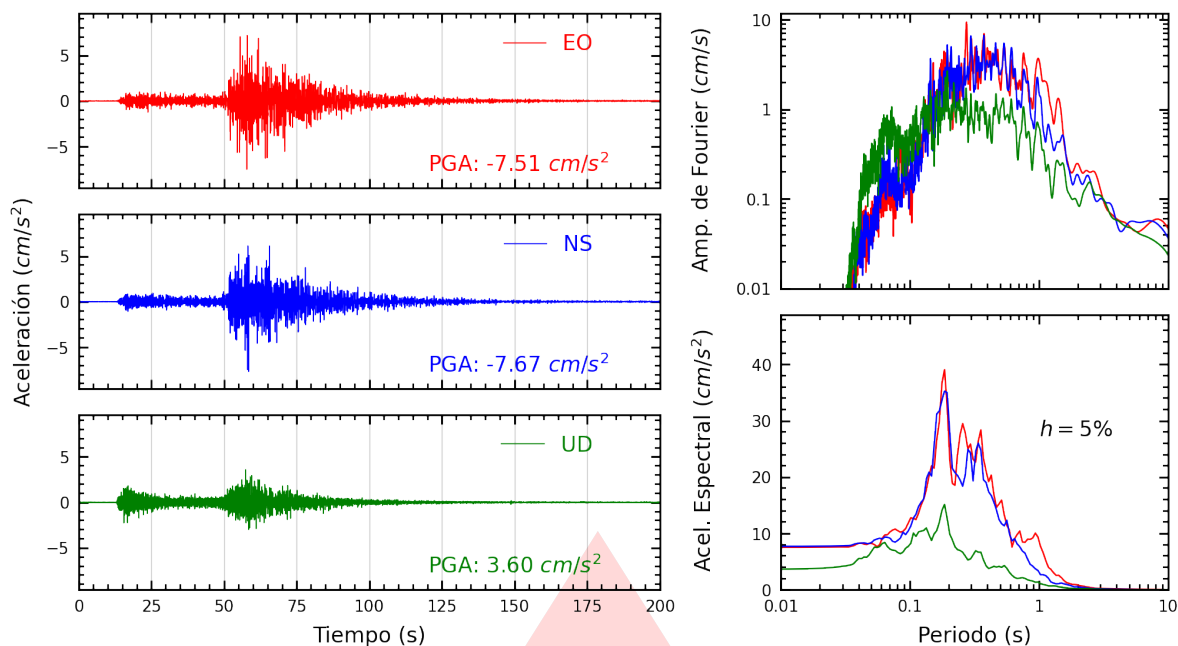
Figura A.21: Registros tiempo-historia, espectros de Fourier y de respuesta en las direcciones EO, NS y vertical de la estación ACAPU. Sismo de Chimbote, Santa - Áncash del 2025-12-27, 21:51:48 (Hora local)
