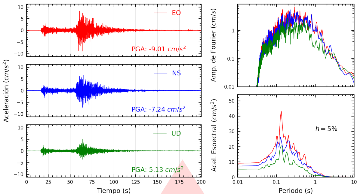
Figura A.17: Registros tiempo-historia, espectros de Fourier y de respuesta en las direcciones EO, NS y vertical de la estación BRISA. Sismo de Chimbote, Santa - Áncash del 2025-12-27, 21:51:48 (Hora local)
