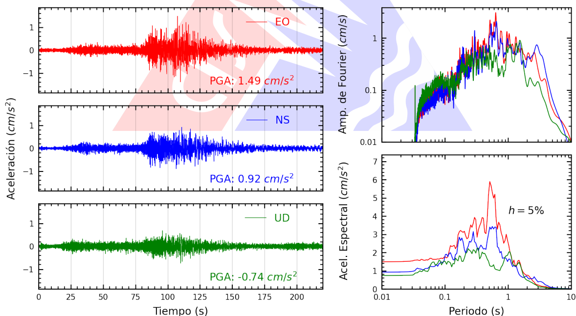
Figura A.48: Registros tiempo-historia, espectros de Fourier y de respuesta en las direcciones EO, NS y vertical de la estación SCICA. Sismo de Chimbote, Santa - Áncash del 2025-12-27, 21:51:48 (Hora local)
