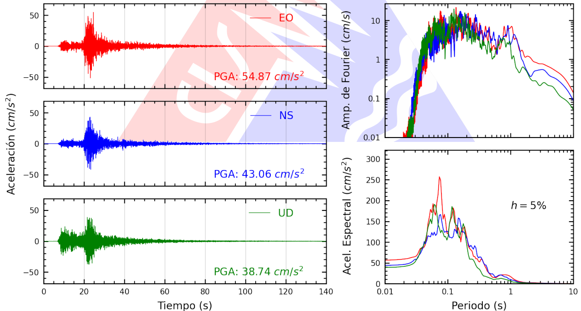
Figura A.4: Registros tiempo-historia, espectros de Fourier y de respuesta en las direcciones EO, NS y vertical de la estación UPAOT. Sismo de Chimbote, Santa - Áncash del 2025-12-27, 21:51:48 (Hora local)
