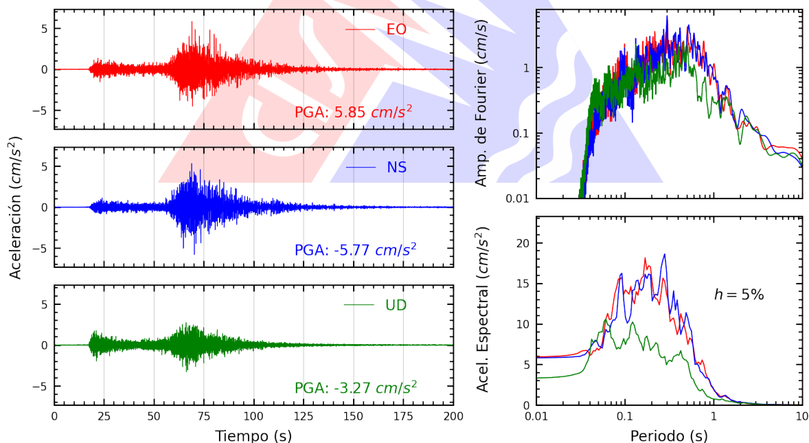
Figura A.30: Registros tiempo-historia, espectros de Fourier y de respuesta en las direcciones EO, NS y vertical de la estación USILP. Sismo de Chimbote, Santa - Áncash del 2025-12-27, 21:51:48 (Hora local)
