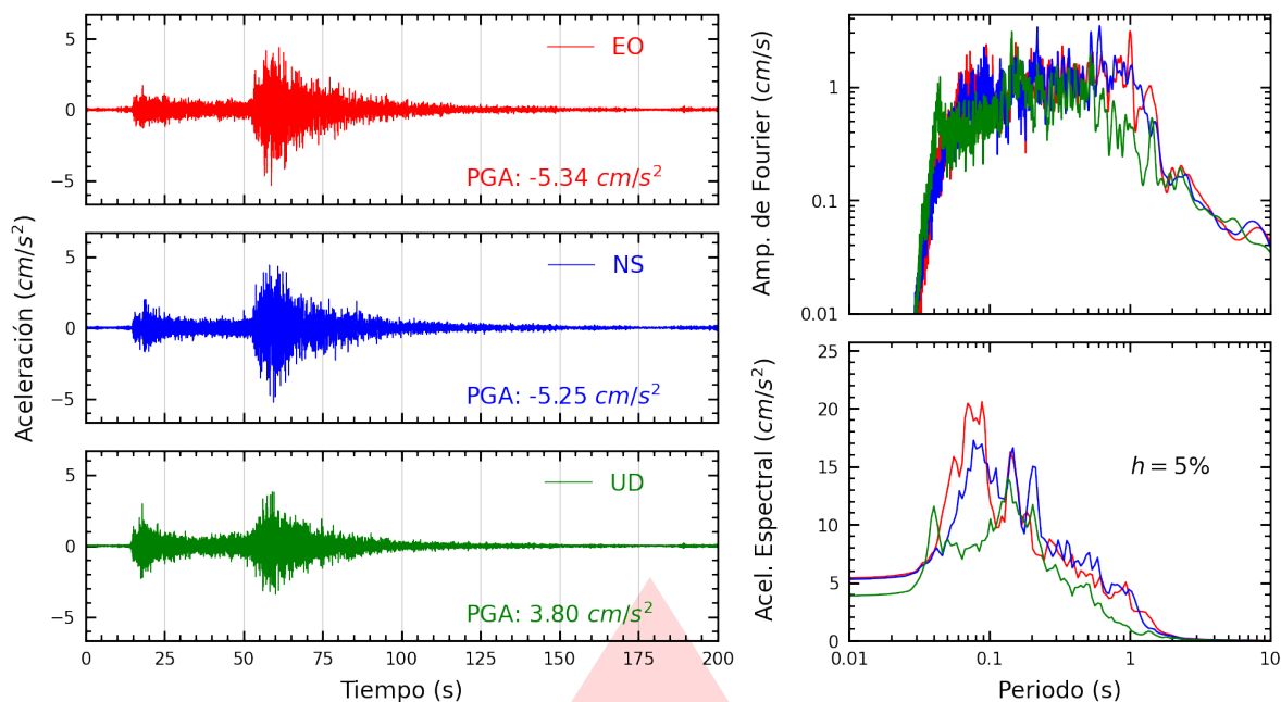
Figura A.31: Registros tiempo-historia, espectros de Fourier y de respuesta en las direcciones EO, NS y vertical de la estación UPCSM. Sismo de Chimbote, Santa - Áncash del 2025-12-27, 21:51:48 (Hora local)
