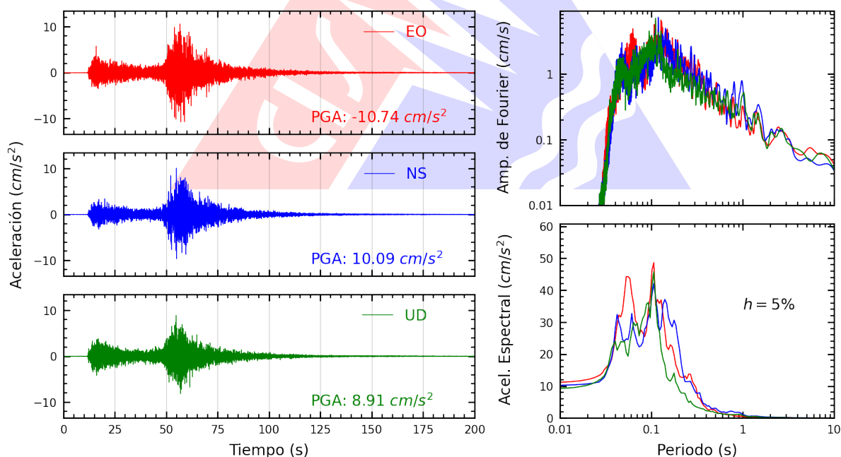
Figura A.14: Registros tiempo-historia, espectros de Fourier y de respuesta en las direcciones EO, NS y vertical de la estación AMORE. Sismo de Chimbote, Santa - Áncash del 2025-12-27, 21:51:48 (Hora local)
