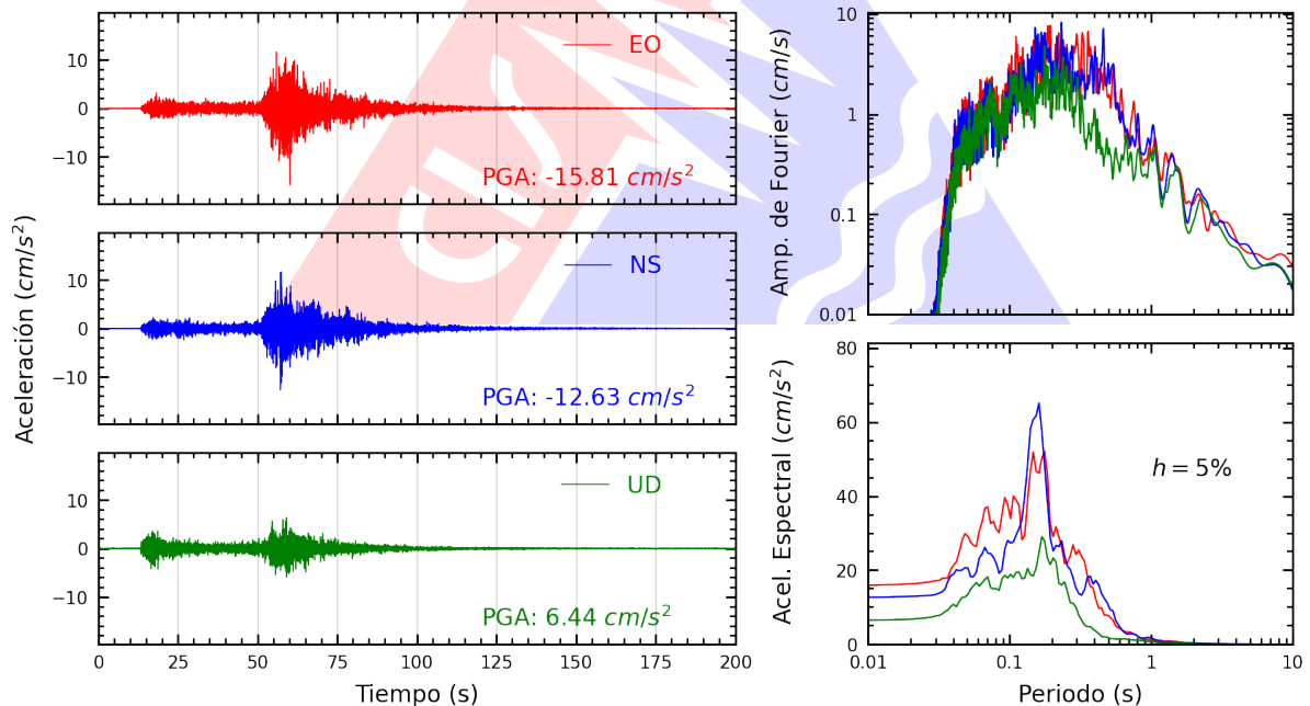
Figura A.8: Registros tiempo-historia, espectros de Fourier y de respuesta en las direcciones EO, NS y vertical de la estación SCOLI. Sismo de Chimbote, Santa - Áncash del 2025-12-27, 21:51:48 (Hora local)
