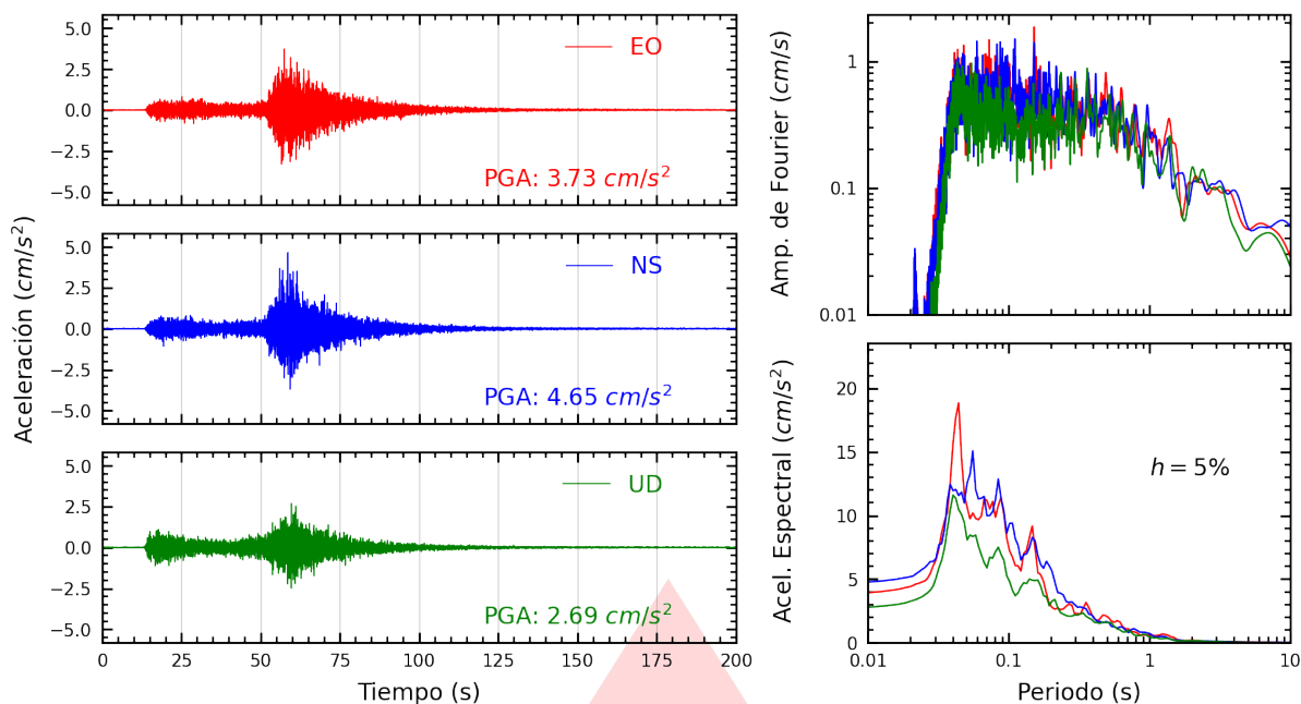
Figura A.37: Registros tiempo-historia, espectros de Fourier y de respuesta en las direcciones EO, NS y vertical de la estación SJLCE. Sismo de Chimbote, Santa - Áncash del 2025-12-27, 21:51:48 (Hora local)
