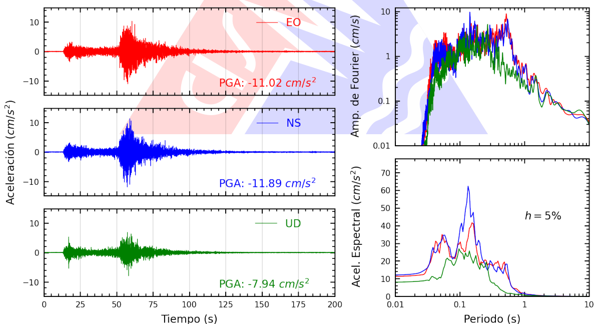
Figura A.12: Registros tiempo-historia, espectros de Fourier y de respuesta en las direcciones EO, NS y vertical de la estación OLIVO. Sismo de Chimbote, Santa - Áncash del 2025-12-27, 21:51:48 (Hora local)
