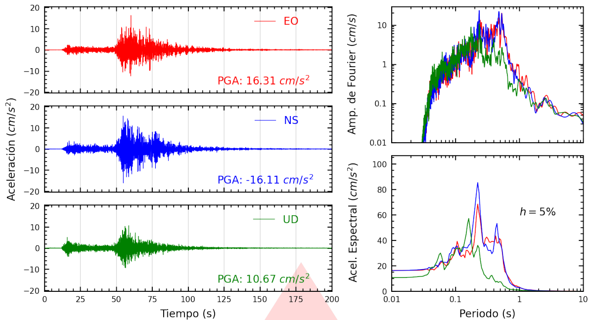
Figura A.7: Registros tiempo-historia, espectros de Fourier y de respuesta en las direcciones EO, NS y vertical de la estación MDP. Sismo de Chimbote, Santa - Áncash del 2025-12-27, 21:51:48 (Hora local)
