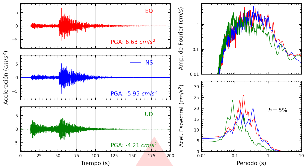
Figura A.25: Registros tiempo-historia, espectros de Fourier y de respuesta en las direcciones EO, NS y vertical de la estación RAMON. Sismo de Chimbote, Santa - Áncash del 2025-12-27, 21:51:48 (Hora local)
