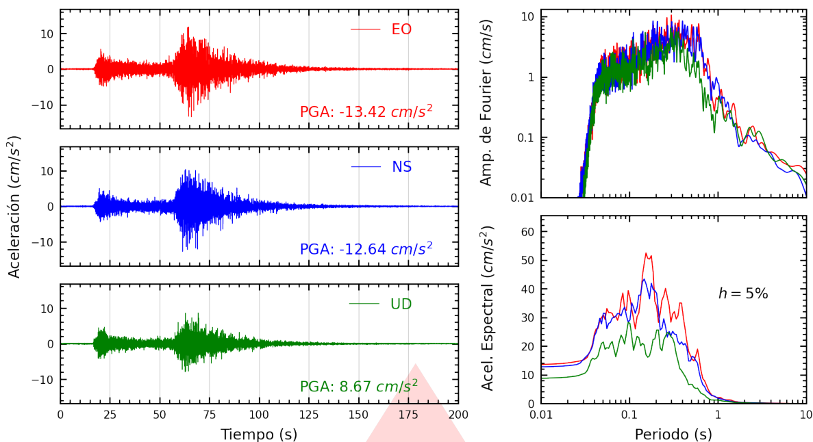
Figura A.11: Registros tiempo-historia, espectros de Fourier y de respuesta en las direcciones EO, NS y vertical de la estación UNTEL. Sismo de Chimbote, Santa - Áncash del 2025-12-27, 21:51:48 (Hora local)
