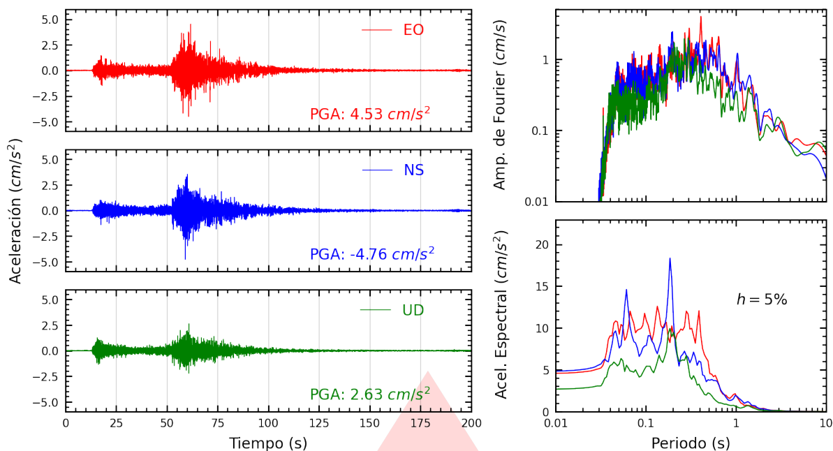
Figura A.35: Registros tiempo-historia, espectros de Fourier y de respuesta en las direcciones EO, NS y vertical de la estación UPCVI. Sismo de Chimbote, Santa - Áncash del 2025-12-27, 21:51:48 (Hora local)
