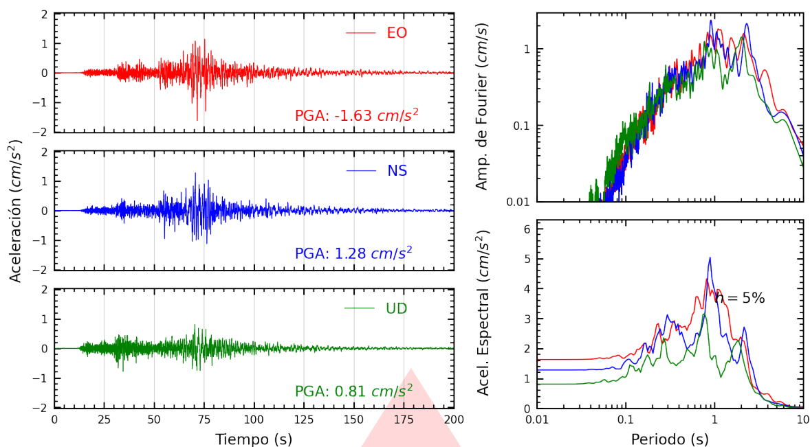
Figura A.47: Registros tiempo-historia, espectros de Fourier y de respuesta en las direcciones EO, NS y vertical de la estación UNJ. Sismo de Chimbote, Santa - Áncash del 2025-12-27, 21:51:48 (Hora local)
