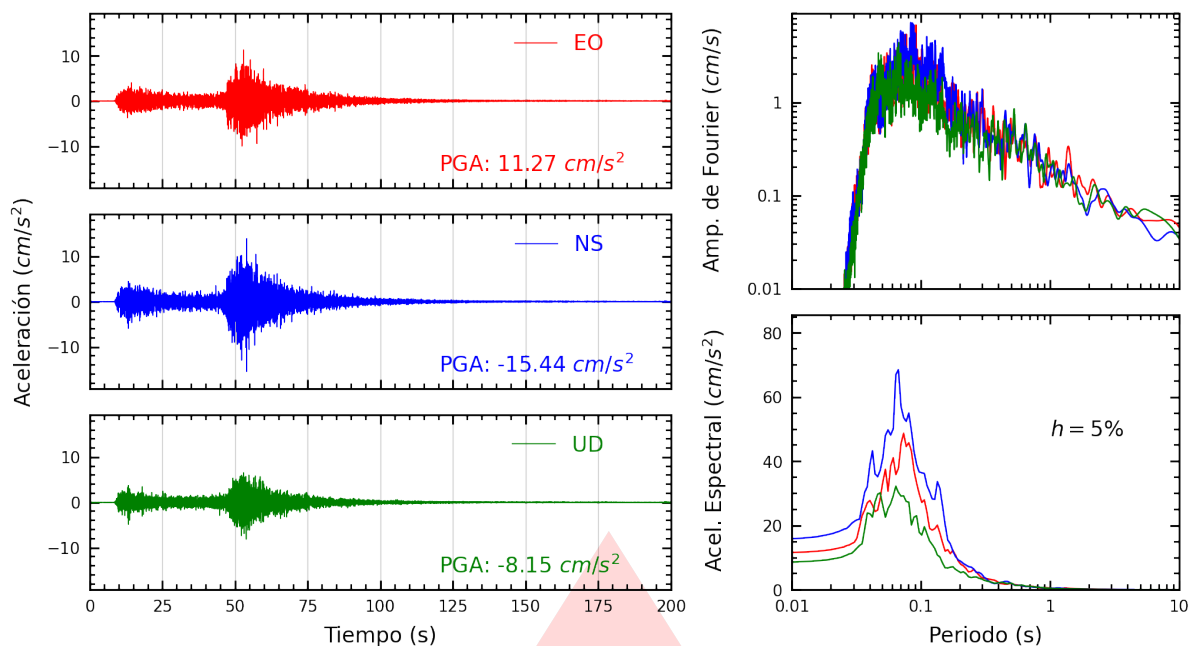
Figura A.9: Registros tiempo-historia, espectros de Fourier y de respuesta en las direcciones EO, NS y vertical de la estación JOSEO. Sismo de Chimbote, Santa - Áncash del 2025-12-27, 21:51:48 (Hora local)
