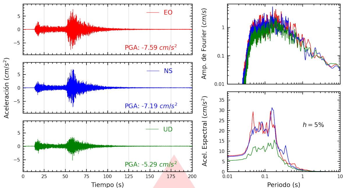
Figura A.23: Registros tiempo-historia, espectros de Fourier y de respuesta en las direcciones EO, NS y vertical de la estación FICPE. Sismo de Chimbote, Santa - Áncash del 2025-12-27, 21:51:48 (Hora local)
