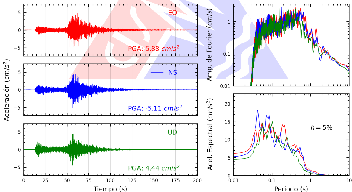
Figura A.28: Registros tiempo-historia, espectros de Fourier y de respuesta en las direcciones EO, NS y vertical de la estación COMAS. Sismo de Chimbote, Santa - Áncash del 2025-12-27, 21:51:48 (Hora local)
