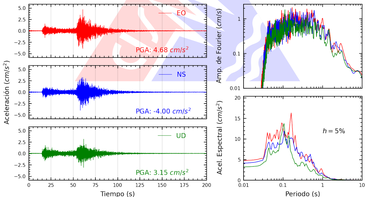
Figura A.36: Registros tiempo-historia, espectros de Fourier y de respuesta en las direcciones EO, NS y vertical de la estación BORJA. Sismo de Chimbote, Santa - Áncash del 2025-12-27, 21:51:48 (Hora local)
