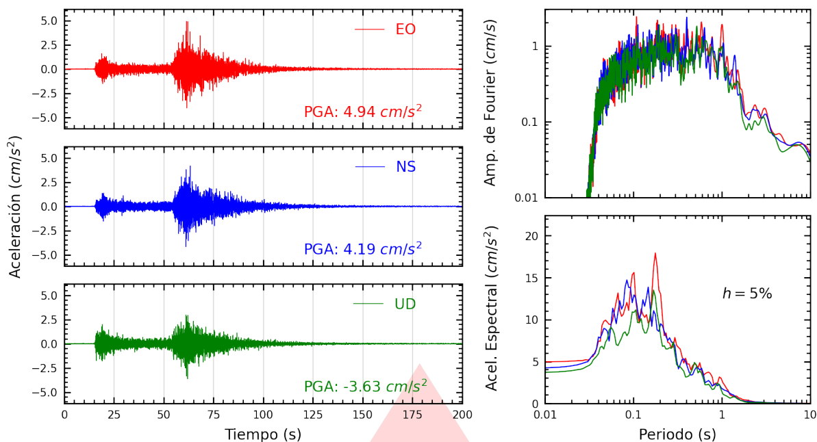
Figura A.33: Registros tiempo-historia, espectros de Fourier y de respuesta en las direcciones EO, NS y vertical de la estación SERVI. Sismo de Chimbote, Santa - Áncash del 2025-12-27, 21:51:48 (Hora local)
