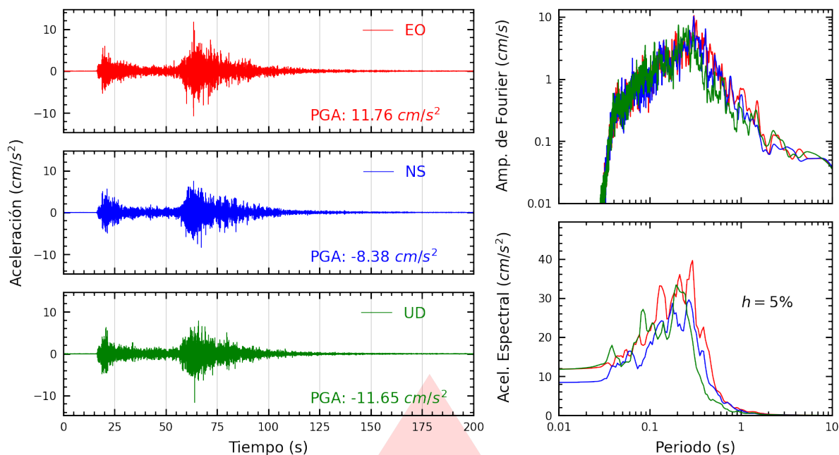
Figura A.13: Registros tiempo-historia, espectros de Fourier y de respuesta en las direcciones EO, NS y vertical de la estación SOVES. Sismo de Chimbote, Santa - Áncash del 2025-12-27, 21:51:48 (Hora local)
