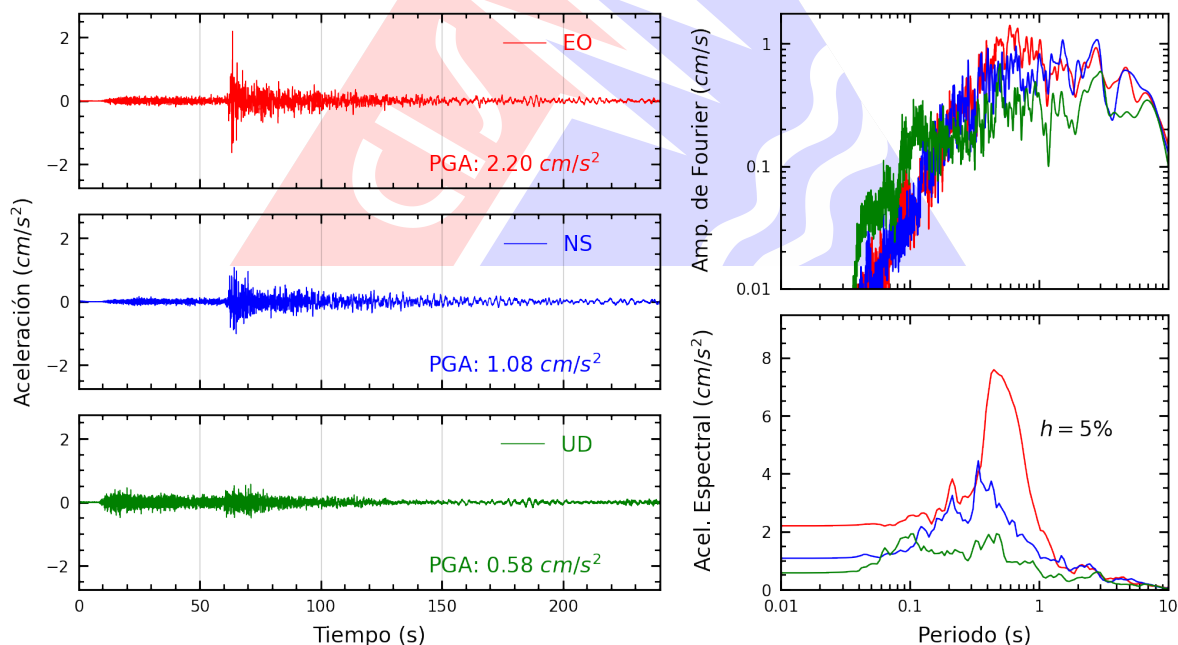
Figura A.46: Registros tiempo-historia, espectros de Fourier y de respuesta en las direcciones EO, NS y vertical de la estación SCPUC. Sismo de Chimbote, Santa - Áncash del 2025-12-27, 21:51:48 (Hora local)
