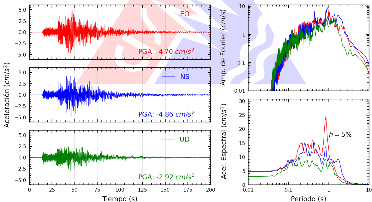
Figura A.34: Registros tiempo-historia, espectros de Fourier y de respuesta en las direcciones EO, NS y vertical de la estación UNC. Sismo de Chimbote, Santa - Áncash del 2025-12-27, 21:51:48 (Hora local)
