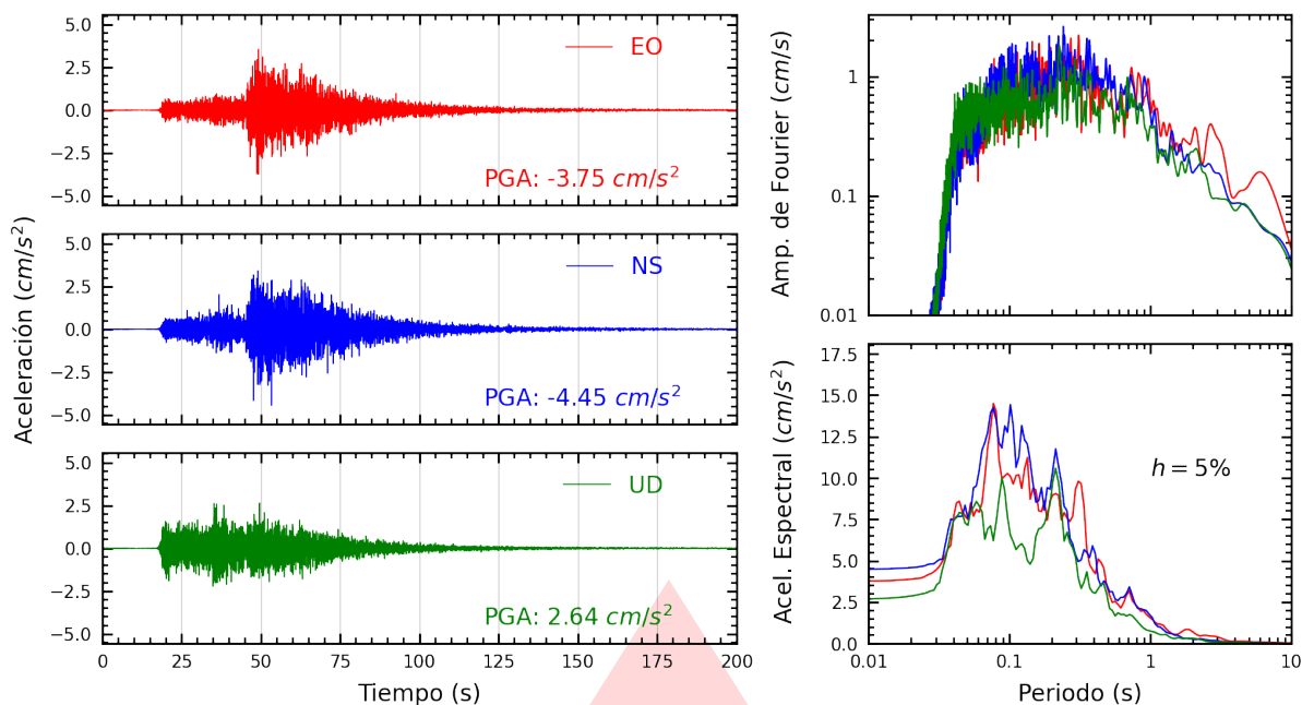
Figura A.39: Registros tiempo-historia, espectros de Fourier y de respuesta en las direcciones EO, NS y vertical de la estación SCCHI. Sismo de Chimbote, Santa - Áncash del 2025-12-27, 21:51:48 (Hora local)
