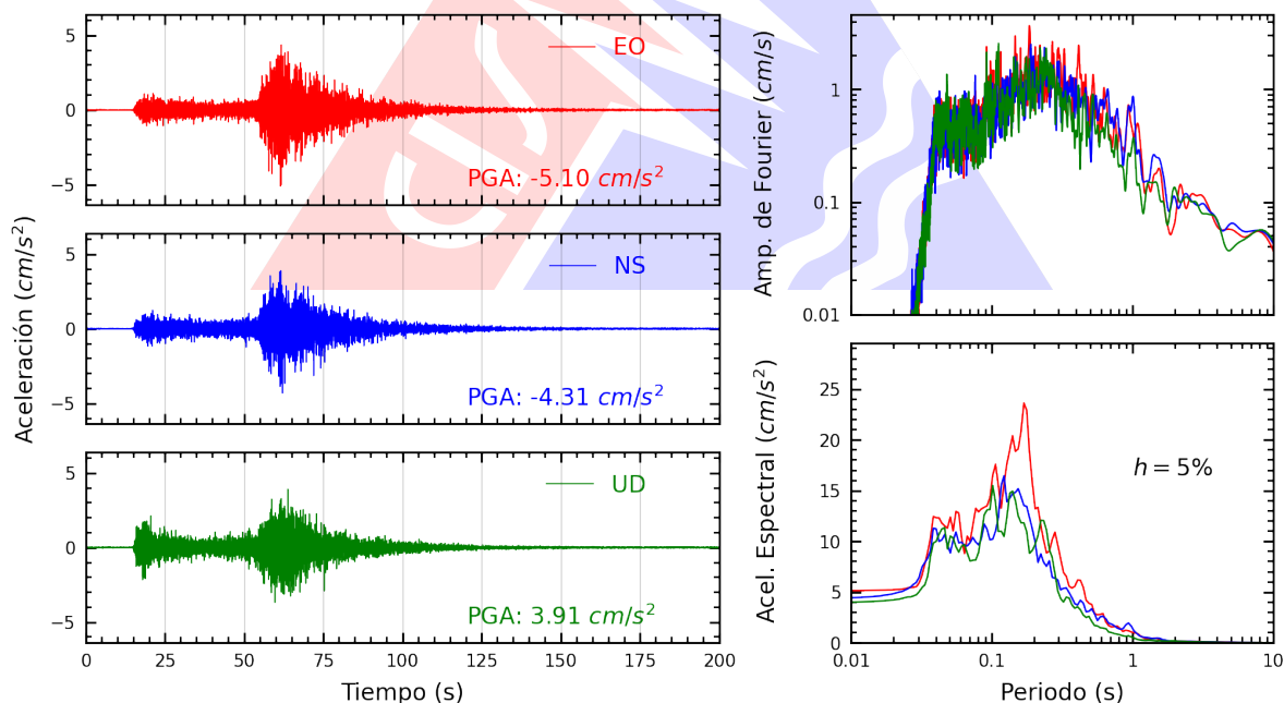
Figura A.32: Registros tiempo-historia, espectros de Fourier y de respuesta en las direcciones EO, NS y vertical de la estación USMP. Sismo de Chimbote, Santa - Áncash del 2025-12-27, 21:51:48 (Hora local)
