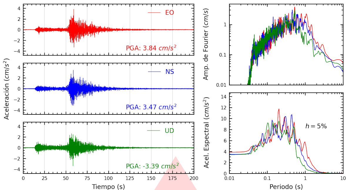
Figura A.43: Registros tiempo-historia, espectros de Fourier y de respuesta en las direcciones EO, NS y vertical de la estación BONDY. Sismo de Chimbote, Santa - Áncash del 2025-12-27, 21:51:48 (Hora local)
