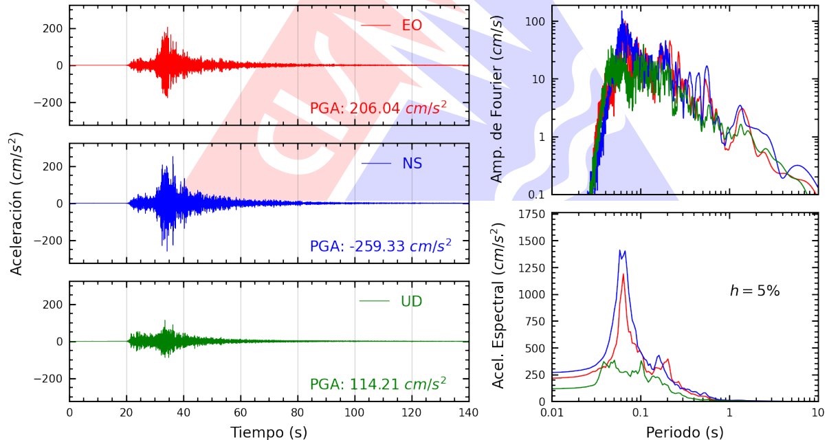
Figura A.2: Registros tiempo-historia, espectros de Fourier y de respuesta en las direcciones EO, NS y vertical de la estación UNS. Sismo de Chimbote, Santa - Áncash del 2025-12-27, 21:51:48 (Hora local)
