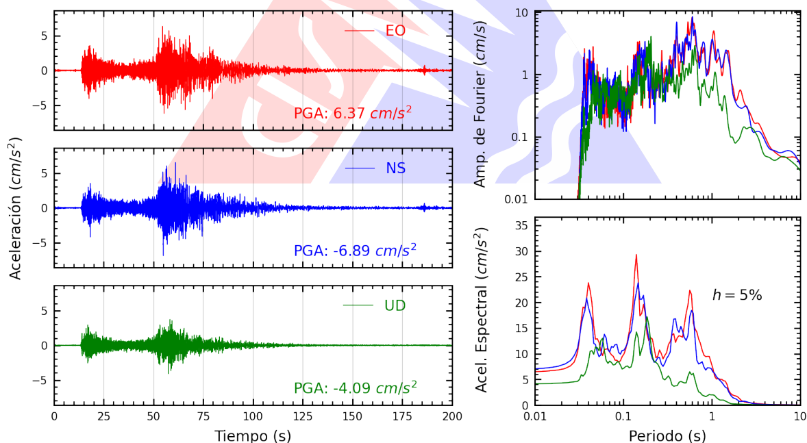
Figura A.24: Registros tiempo-historia, espectros de Fourier y de respuesta en las direcciones EO, NS y vertical de la estación DHNPE. Sismo de Chimbote, Santa - Áncash del 2025-12-27, 21:51:48 (Hora local)
