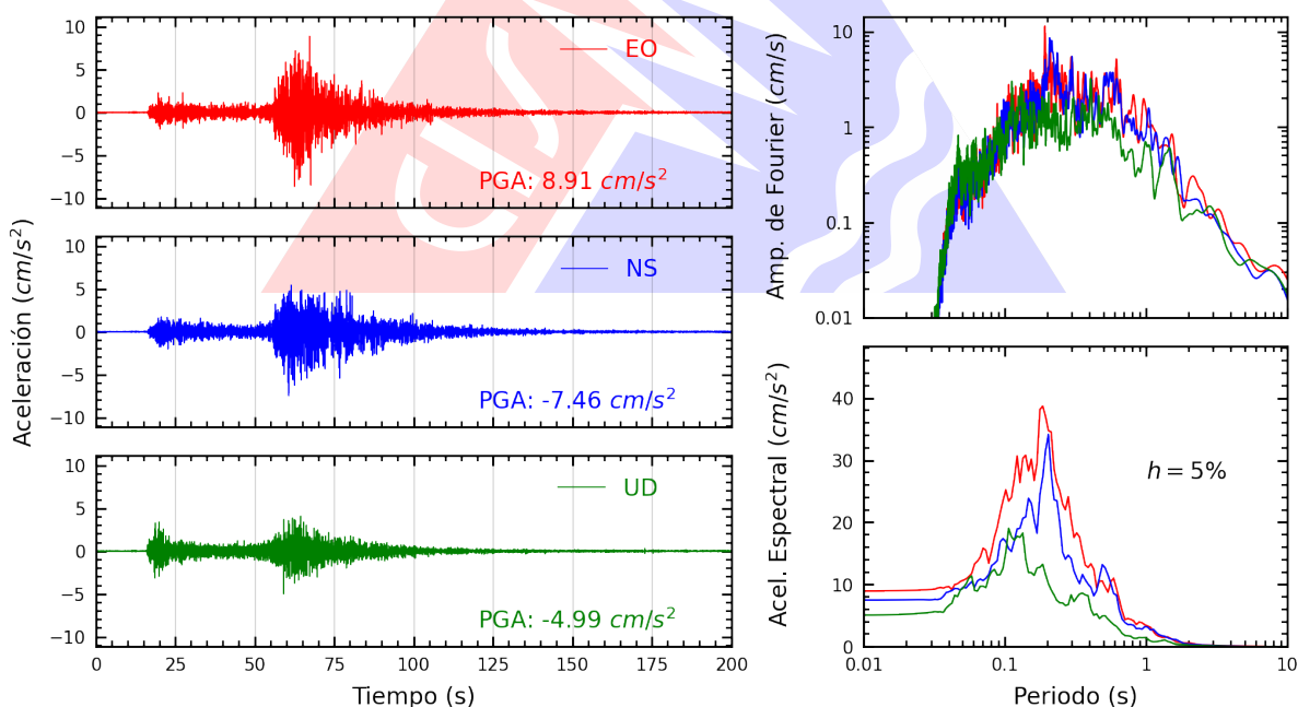
Figura A.18: Registros tiempo-historia, espectros de Fourier y de respuesta en las direcciones EO, NS y vertical de la estación SCCHO. Sismo de Chimbote, Santa - Áncash del 2025-12-27, 21:51:48 (Hora local)
