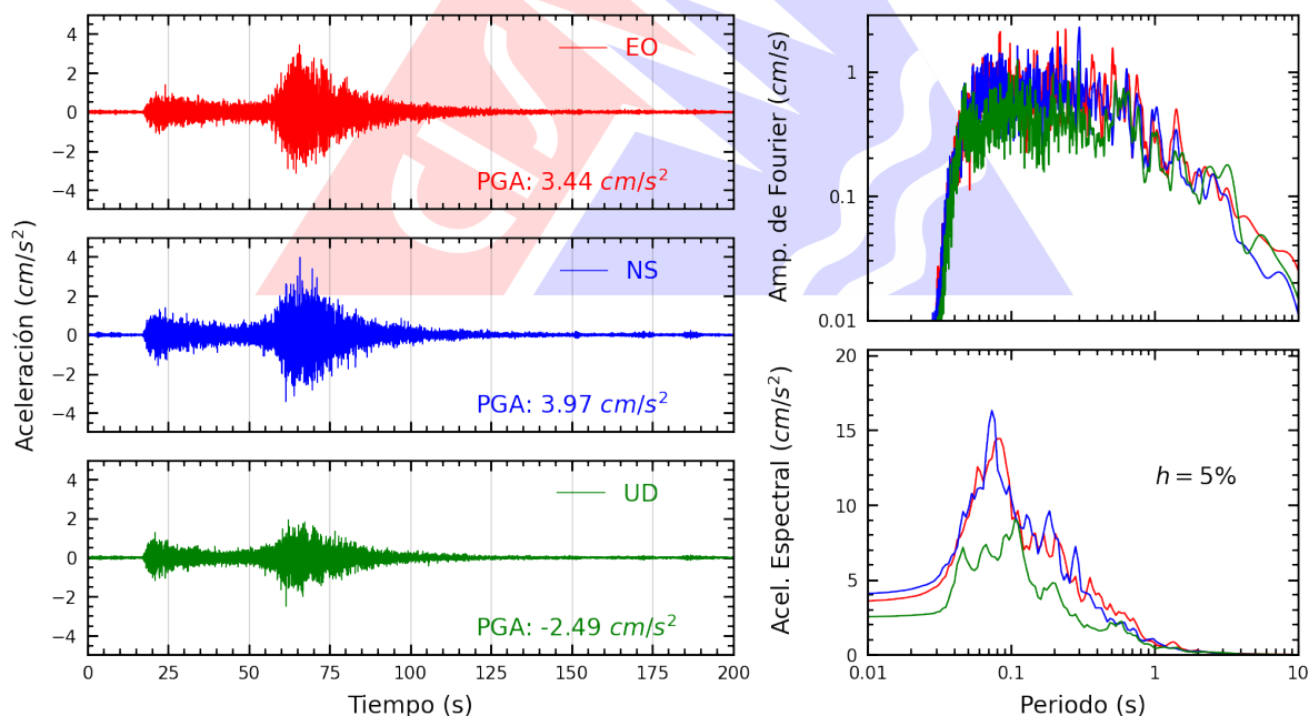
Figura A.42: Registros tiempo-historia, espectros de Fourier y de respuesta en las direcciones EO, NS y vertical de la estación PACHA. Sismo de Chimbote, Santa - Áncash del 2025-12-27, 21:51:48 (Hora local)
