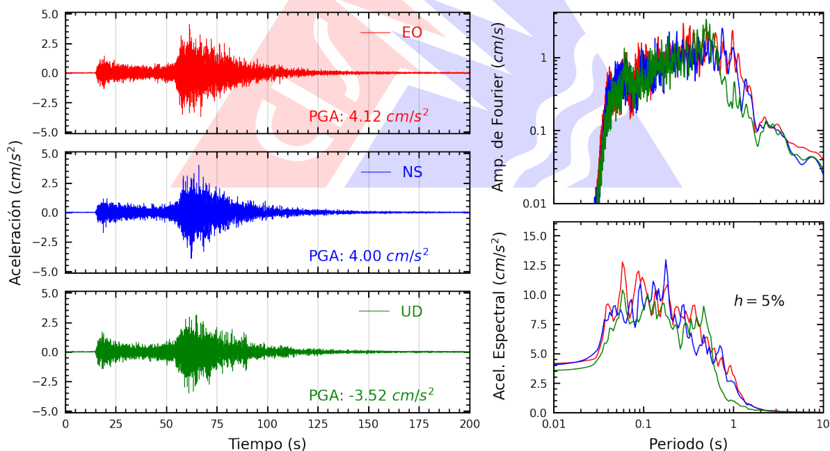
Figura A.40: Registros tiempo-historia, espectros de Fourier y de respuesta en las direcciones EO, NS y vertical de la estación IMCA. Sismo de Chimbote, Santa - Áncash del 2025-12-27, 21:51:48 (Hora local)
