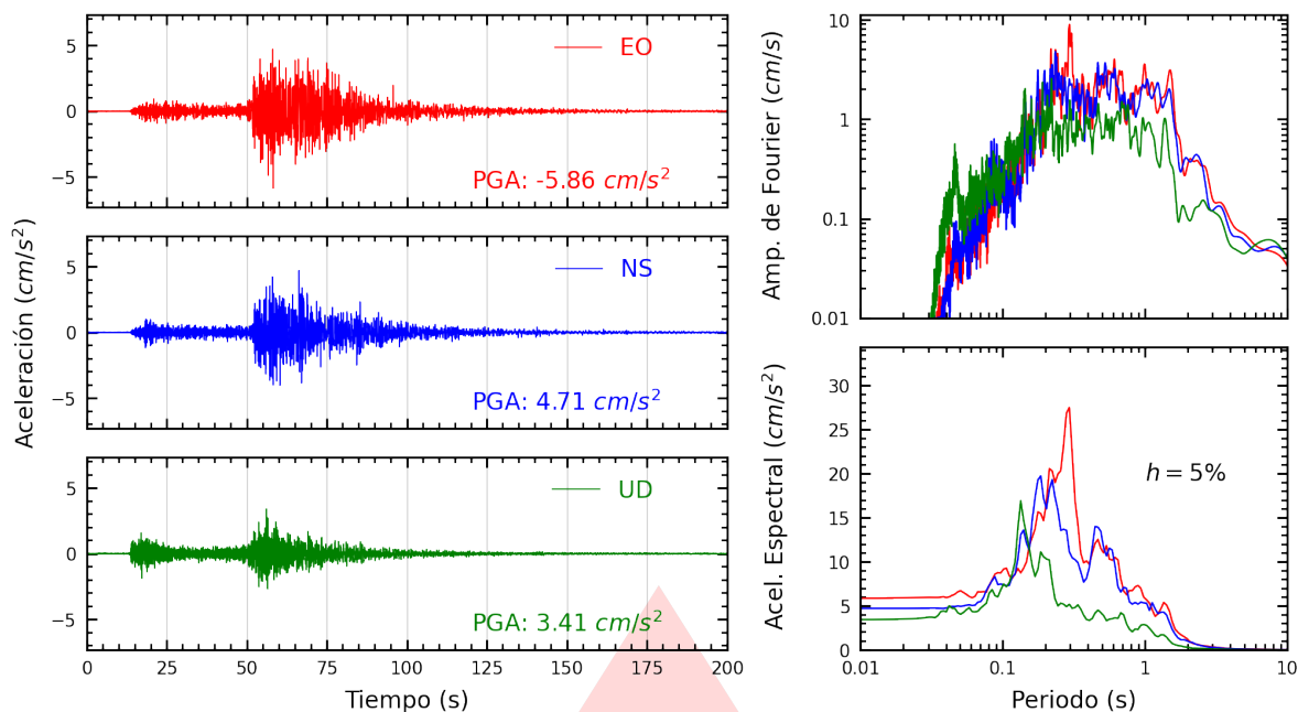
Figura A.29: Registros tiempo-historia, espectros de Fourier y de respuesta en las direcciones EO, NS y vertical de la estación DDMI. Sismo de Chimbote, Santa - Áncash del 2025-12-27, 21:51:48 (Hora local)
