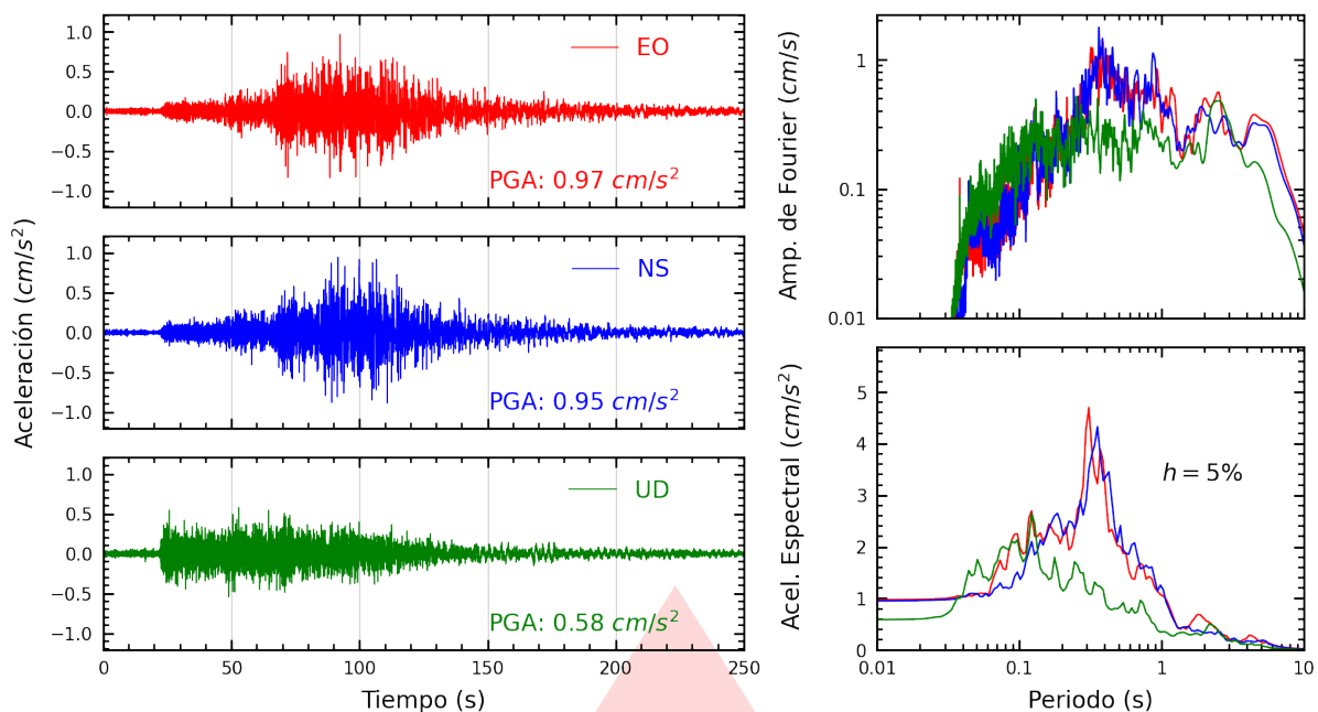
Figura A.49: Registros tiempo-historia, espectros de Fourier y de respuesta en las direcciones EO, NS y vertical de la estación SCPIU. Sismo de Chimbote, Santa - Áncash del 2025-12-27, 21:51:48 (Hora local)
