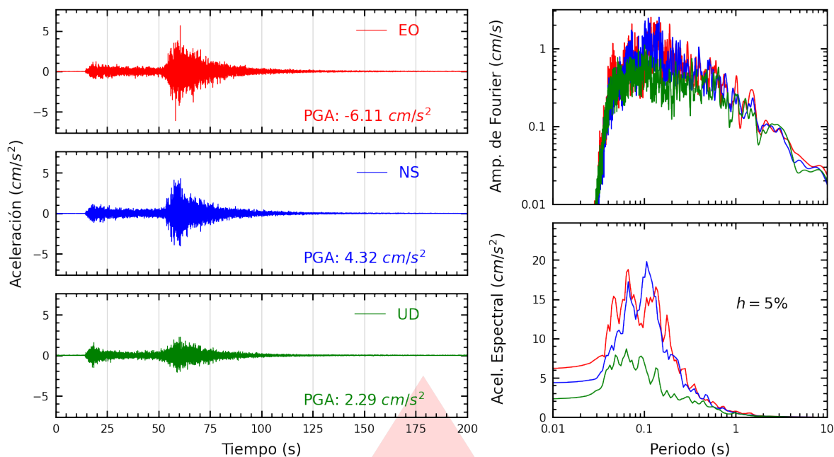
Figura A.27: Registros tiempo-historia, espectros de Fourier y de respuesta en las direcciones EO, NS y vertical de la estación ATARJ. Sismo de Chimbote, Santa - Áncash del 2025-12-27, 21:51:48 (Hora local)
