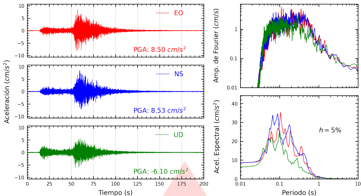
Figura A.19: Registros tiempo-historia, espectros de Fourier y de respuesta en las direcciones EO, NS y vertical de la estación SJLSC. Sismo de Chimbote, Santa - Áncash del 2025-12-27, 21:51:48 (Hora local)
