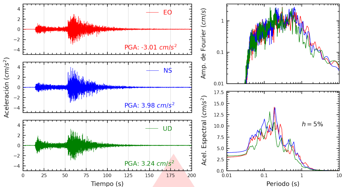
Figura A.41: Registros tiempo-historia, espectros de Fourier y de respuesta en las direcciones EO, NS y vertical de la estación UNFV. Sismo de Chimbote, Santa - Áncash del 2025-12-27, 21:51:48 (Hora local)
