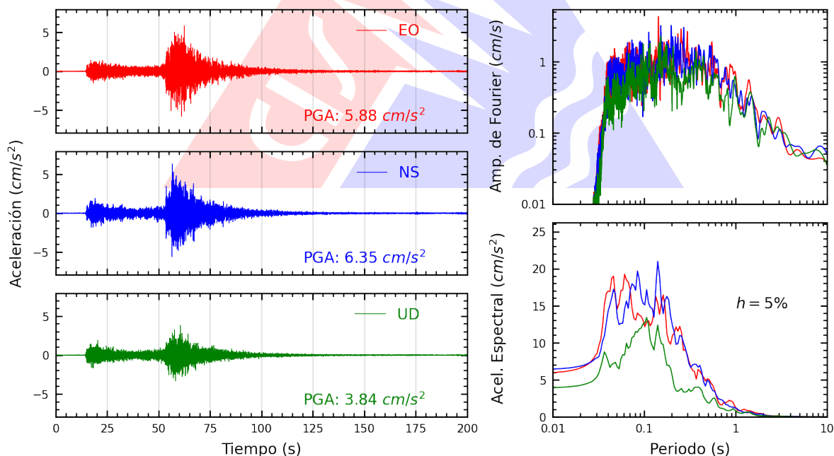
Figura A.26: Registros tiempo-historia, espectros de Fourier y de respuesta en las direcciones EO, NS y vertical de la estación CEPRE. Sismo de Chimbote, Santa - Áncash del 2025-12-27, 21:51:48 (Hora local)
