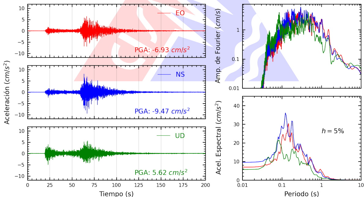
Figura A.16: Registros tiempo-historia, espectros de Fourier y de respuesta en las direcciones EO, NS y vertical de la estación SOCHO. Sismo de Chimbote, Santa - Áncash del 2025-12-27, 21:51:48 (Hora local)
