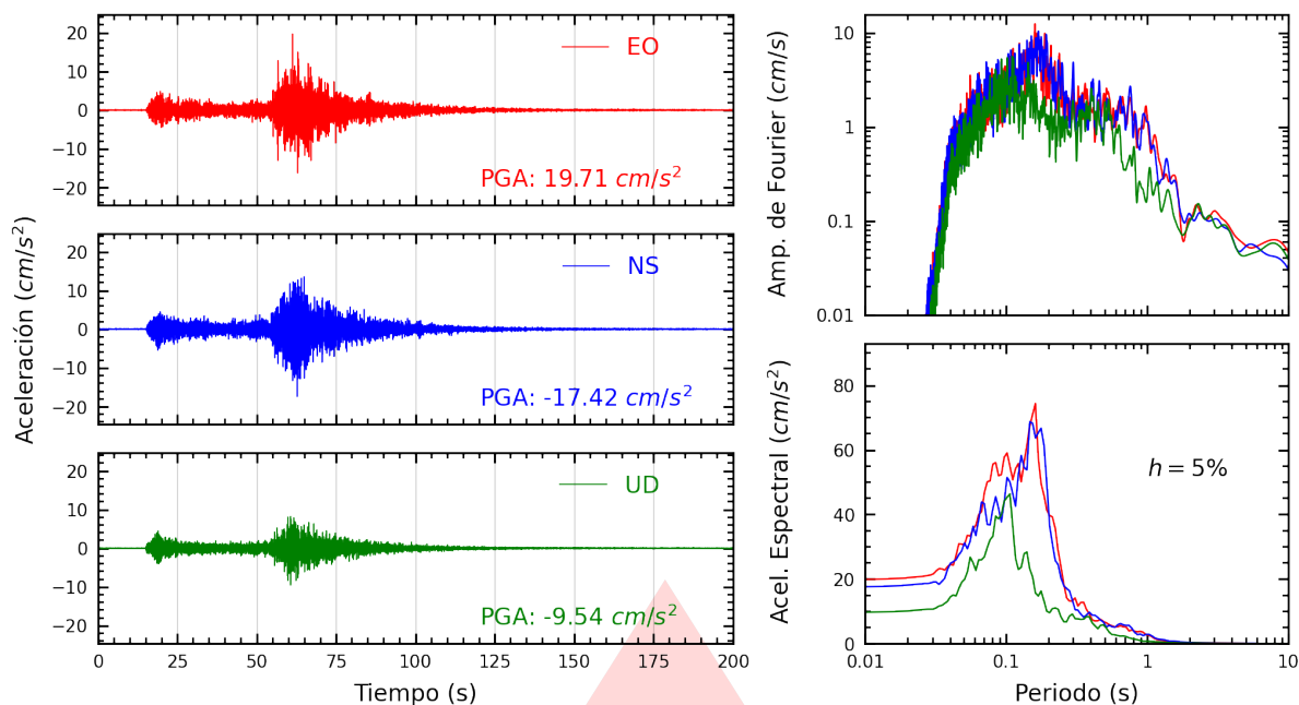
Figura A.5: Registros tiempo-historia, espectros de Fourier y de respuesta en las direcciones EO, NS y vertical de la estación USILM. Sismo de Chimbote, Santa - Áncash del 2025-12-27, 21:51:48 (Hora local)
