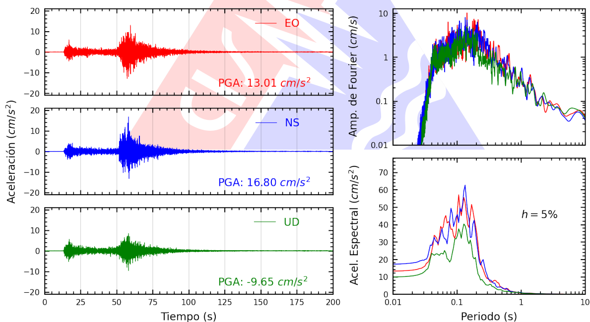
Figura A.6: Registros tiempo-historia, espectros de Fourier y de respuesta en las direcciones EO, NS y vertical de la estación INDEP. Sismo de Chimbote, Santa - Áncash del 2025-12-27, 21:51:48 (Hora local)
