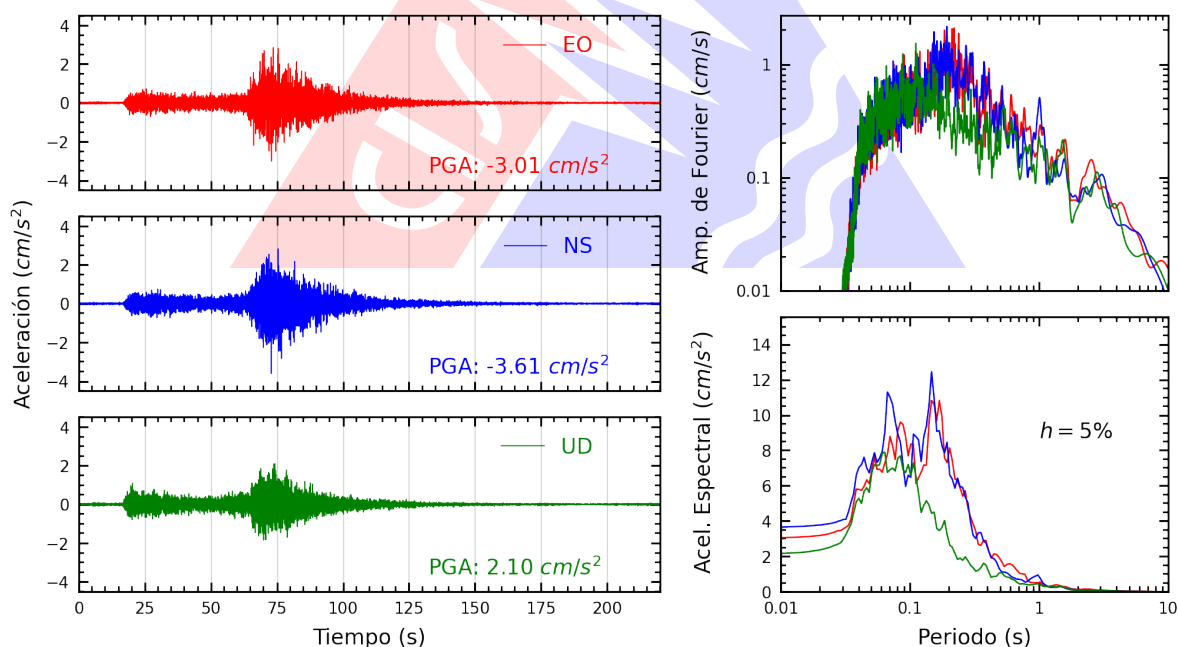
Figura A.44: Registros tiempo-historia, espectros de Fourier y de respuesta en las direcciones EO, NS y vertical de la estación ASIA. Sismo de Chimbote, Santa - Áncash del 2025-12-27, 21:51:48 (Hora local)
