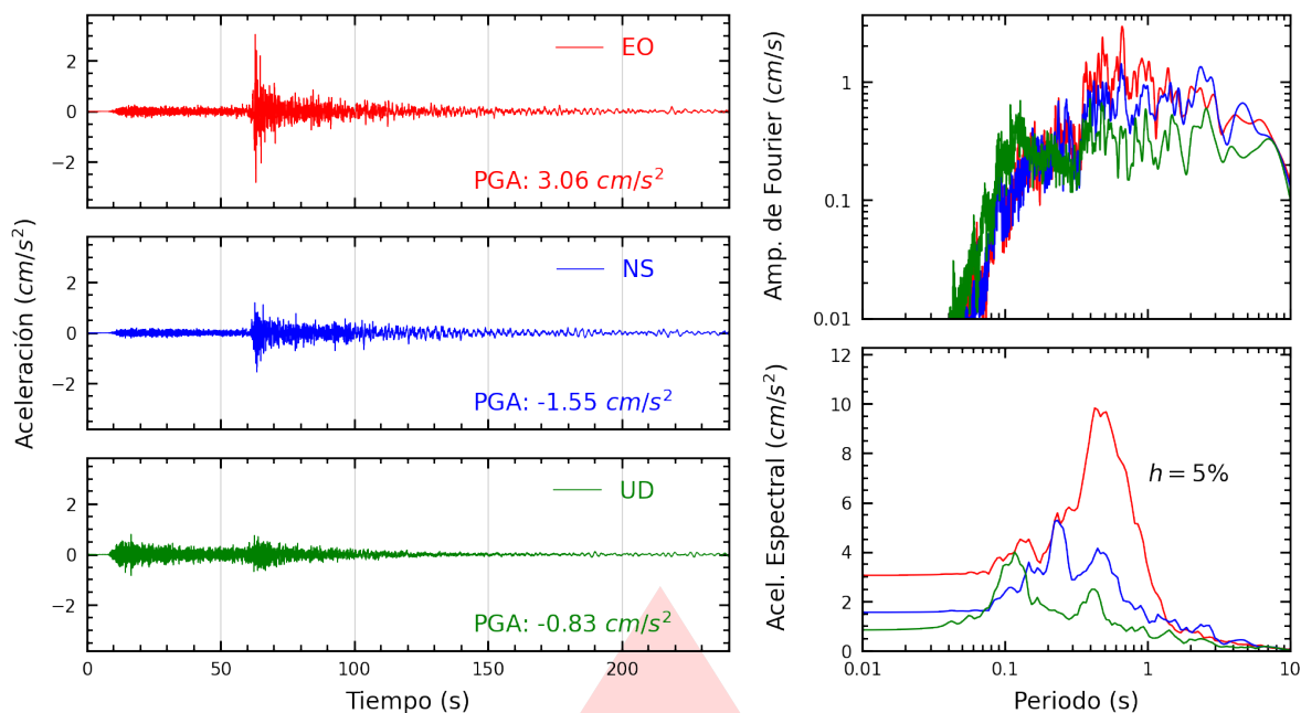
Figura A.45: Registros tiempo-historia, espectros de Fourier y de respuesta en las direcciones EO, NS y vertical de la estación UNIA. Sismo de Chimbote, Santa - Áncash del 2025-12-27, 21:51:48 (Hora local)
