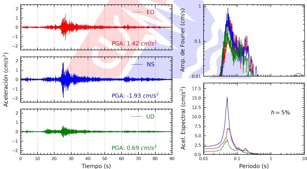
Figura A.2: Registros tiempo-historia, espectros de Fourier y de respuesta en las direcciones EO, NS y vertical de la estación UNS. Sismo de Chimbote, Santa - Áncash del 2025-12-27, 22:51:28 (Hora local)
