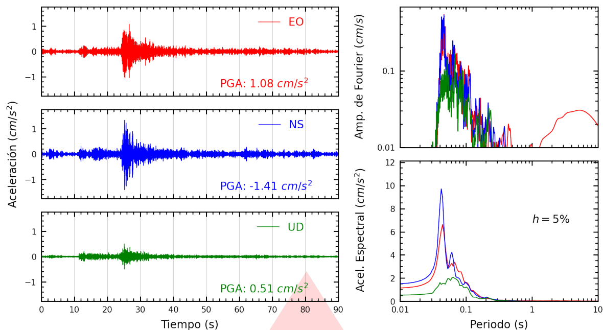
Figura A.3: Registros tiempo-historia, espectros de Fourier y de respuesta en las direcciones EO, NS y vertical de la estación SCTRU. Sismo de Chimbote, Santa - Áncash del 2025-12-27, 22:51:28 (Hora local)
