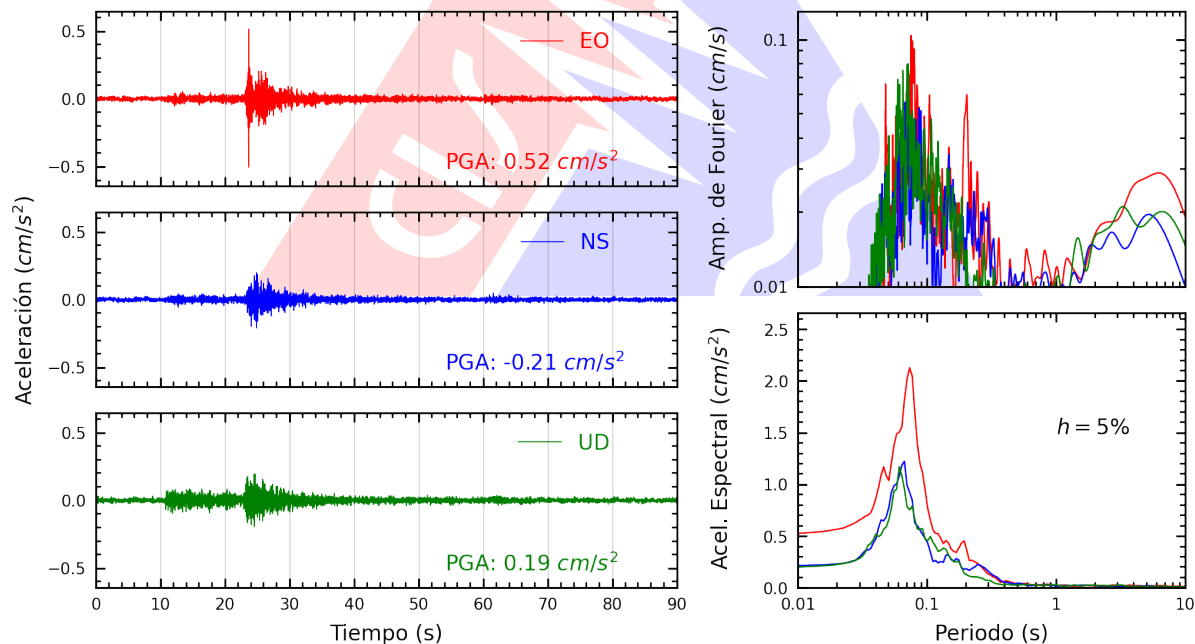
Figura A.4: Registros tiempo-historia, espectros de Fourier y de respuesta en las direcciones EO, NS y vertical de la estación UPAOT. Sismo de Chimbote, Santa - Áncash del 2025-12-27, 22:51:28 (Hora local)
