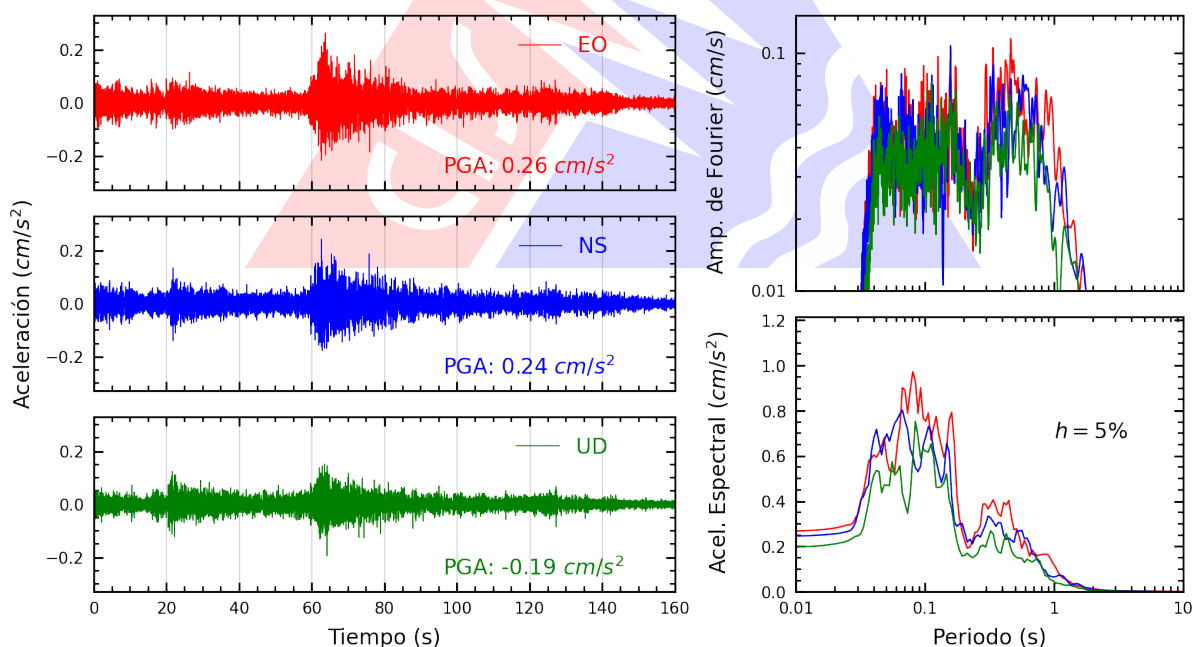
Figura A.36: Registros tiempo-historia, espectros de Fourier y de respuesta en las direcciones EO, NS y vertical de la estación BORJA. Sismo de Chimbote, Santa - Áncash del 2025-12-28, 18:19:55 (Hora local)
