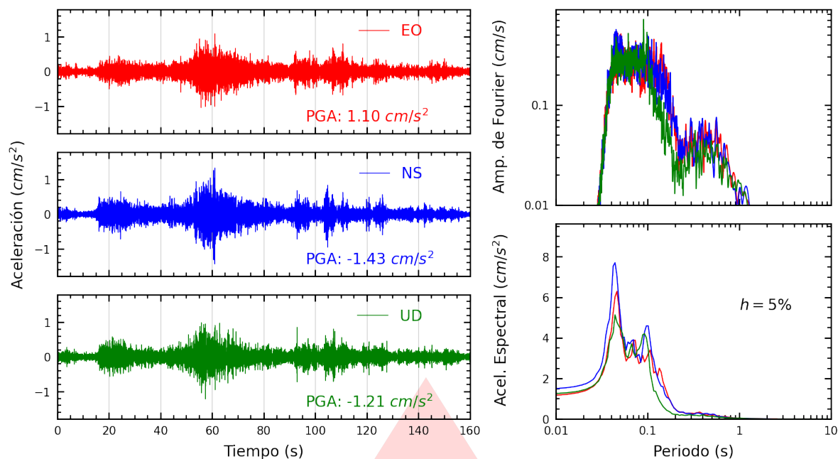
Figura A.5: Registros tiempo-historia, espectros de Fourier y de respuesta en las direcciones EO, NS y vertical de la estación SROSA. Sismo de Chimbote, Santa - Áncash del 2025-12-28, 18:19:55 (Hora local)
