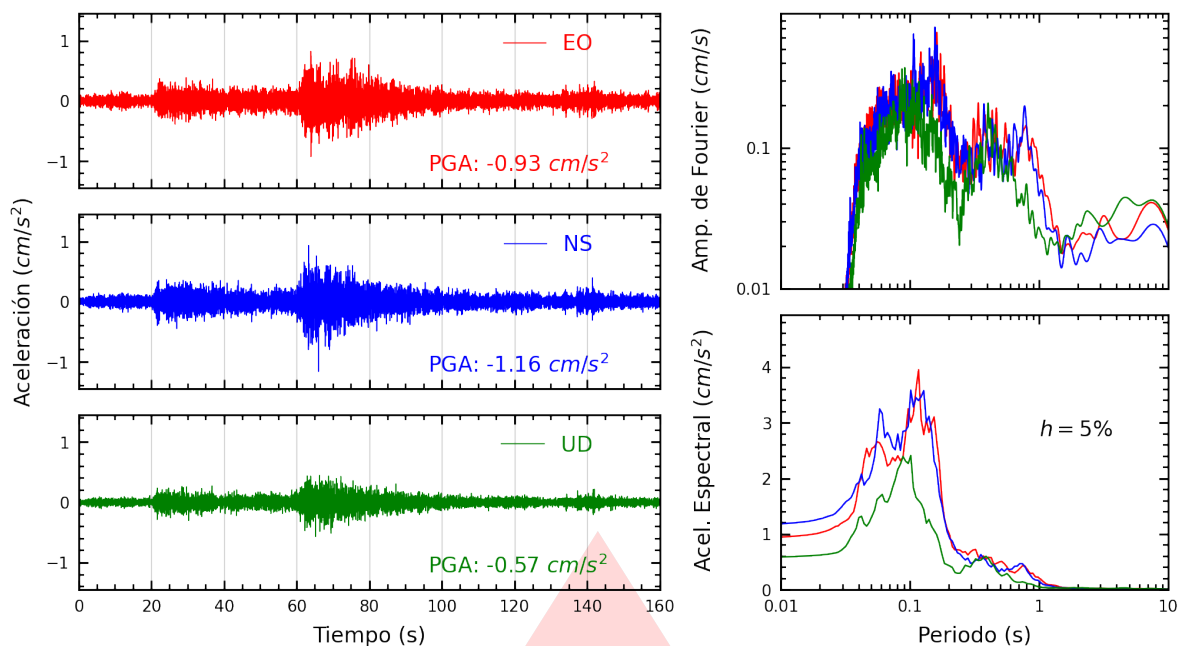
Figura A.7: Registros tiempo-historia, espectros de Fourier y de respuesta en las direcciones EO, NS y vertical de la estación USILM. Sismo de Chimbote, Santa - Áncash del 2025-12-28, 18:19:55 (Hora local)
