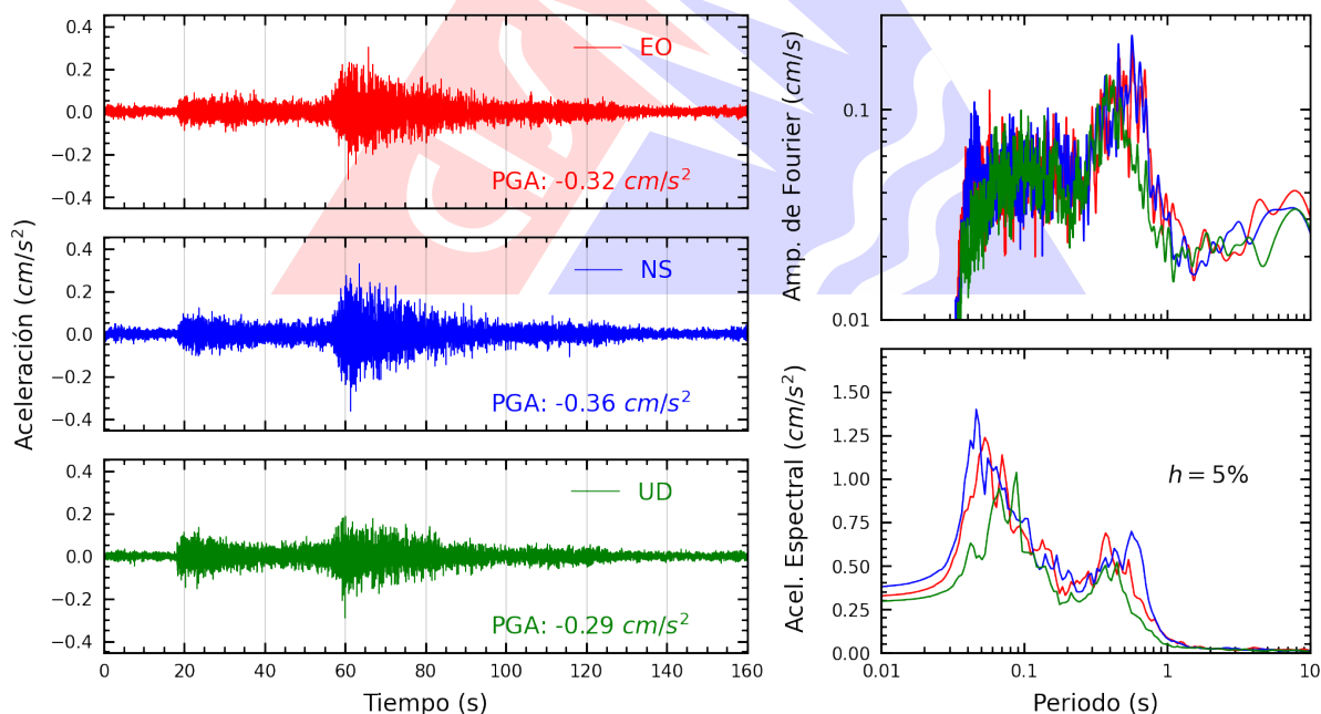
Figura A.26: Registros tiempo-historia, espectros de Fourier y de respuesta en las direcciones EO, NS y vertical de la estación COMAS. Sismo de Chimbote, Santa - Áncash del 2025-12-28, 18:19:55 (Hora local)
