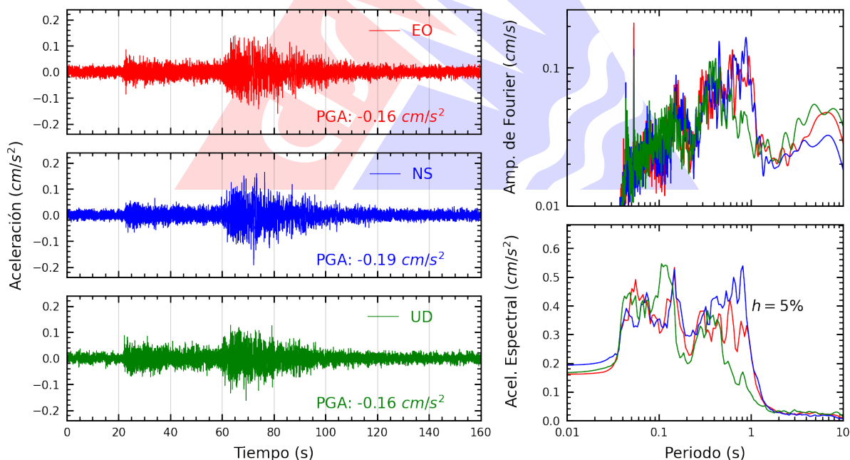
Figura A.40: Registros tiempo-historia, espectros de Fourier y de respuesta en las direcciones EO, NS y vertical de la estación UNMSM. Sismo de Chimbote, Santa - Áncash del 2025-12-28, 18:19:55 (Hora local)
