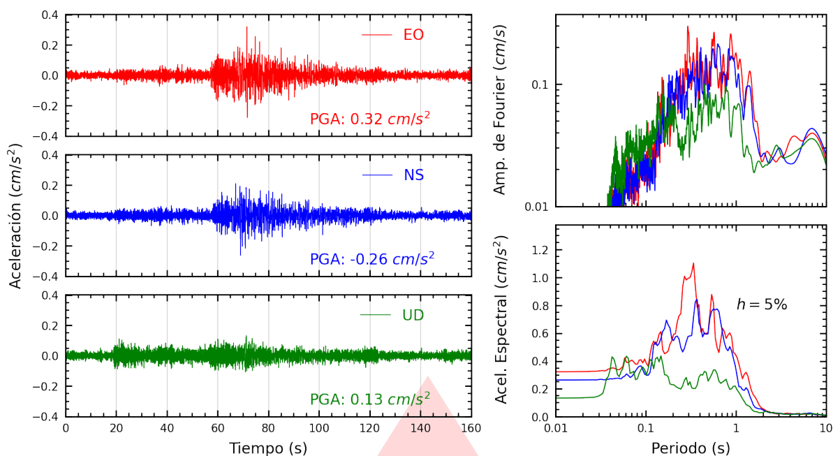
Figura A.29: Registros tiempo-historia, espectros de Fourier y de respuesta en las direcciones EO, NS y vertical de la estación DSMI. Sismo de Chimbote, Santa - Áncash del 2025-12-28, 18:19:55 (Hora local)
