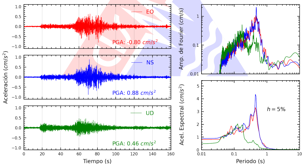
Figura A.10: Registros tiempo-historia, espectros de Fourier y de respuesta en las direcciones EO, NS y vertical de la estación MDPP. Sismo de Chimbote, Santa - Áncash del 2025-12-28, 18:19:55 (Hora local)
