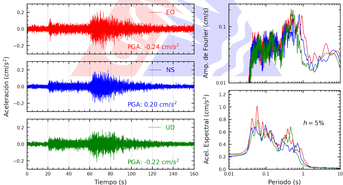
Figura A.38: Registros tiempo-historia, espectros de Fourier y de respuesta en las direcciones EO, NS y vertical de la estación IMCA. Sismo de Chimbote, Santa - Áncash del 2025-12-28, 18:19:55 (Hora local)
