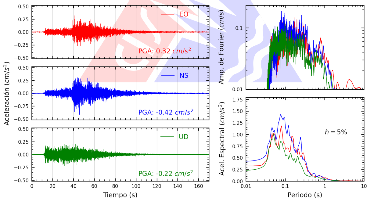
Figura A.24: Registros tiempo-historia, espectros de Fourier y de respuesta en las direcciones EO, NS y vertical de la estación SCCHI. Sismo de Chimbote, Santa - Áncash del 2025-12-28, 18:19:55 (Hora local)
