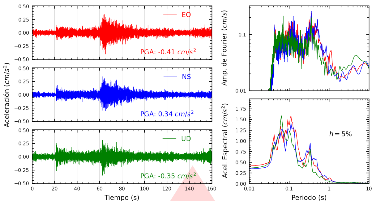
Figura A.25: Registros tiempo-historia, espectros de Fourier y de respuesta en las direcciones EO, NS y vertical de la estación URPE. Sismo de Chimbote, Santa - Áncash del 2025-12-28, 18:19:55 (Hora local)
