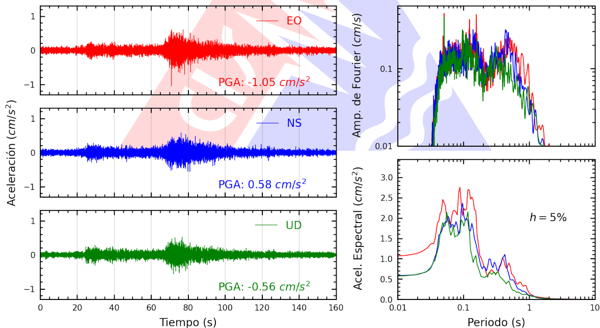
Figura A.8: Registros tiempo-historia, espectros de Fourier y de respuesta en las direcciones EO, NS y vertical de la estación PHERM. Sismo de Chimbote, Santa - Áncash del 2025-12-28, 18:19:55 (Hora local)
