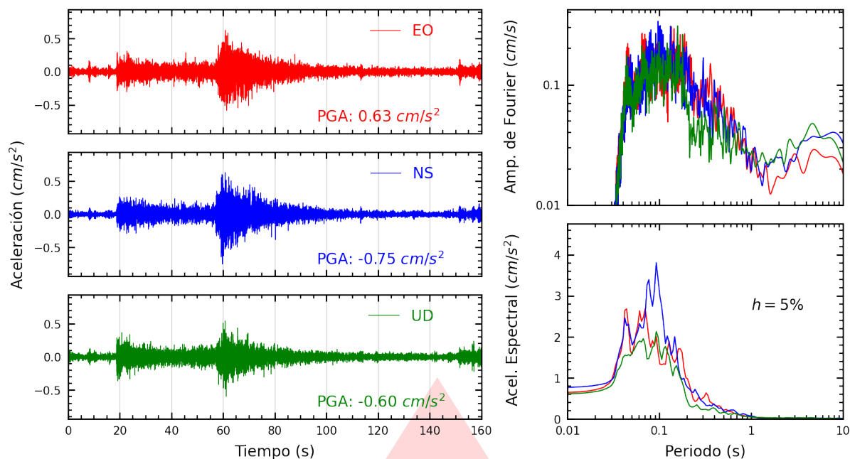
Figura A.11: Registros tiempo-historia, espectros de Fourier y de respuesta en las direcciones EO, NS y vertical de la estación INDEP. Sismo de Chimbote, Santa - Áncash del 2025-12-28, 18:19:55 (Hora local)
