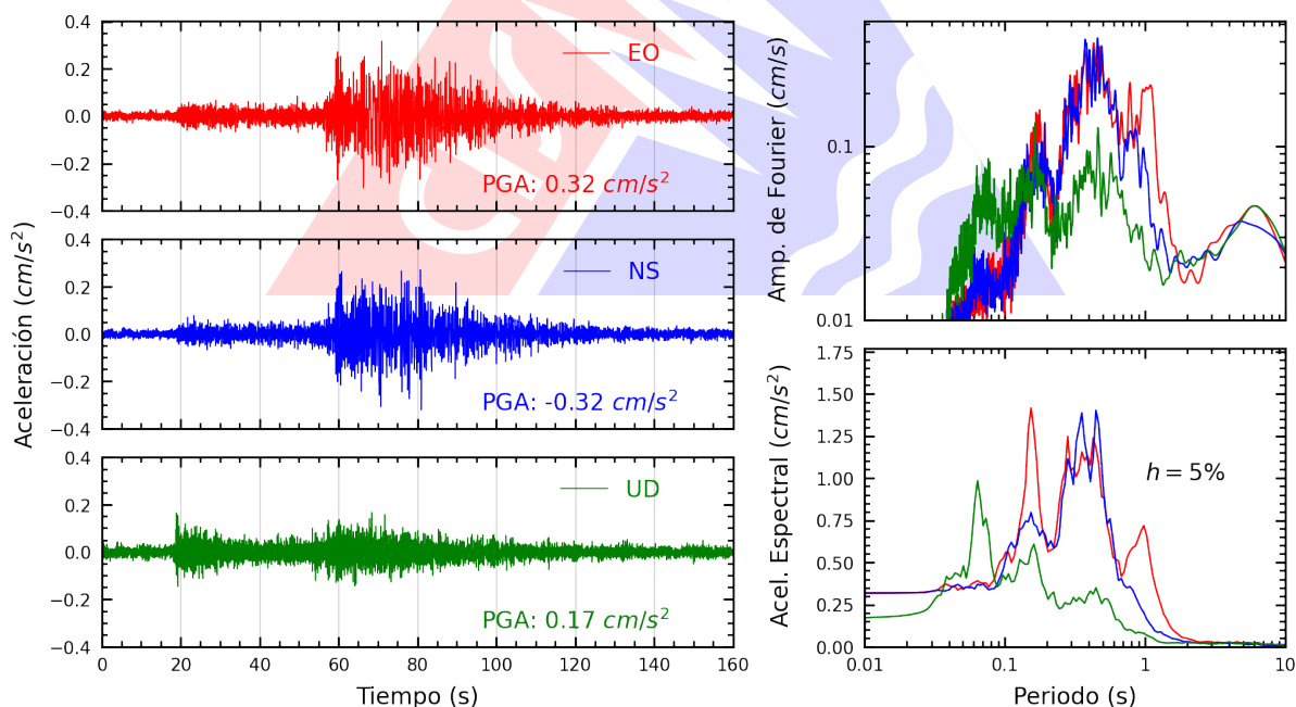
Figura A.30: Registros tiempo-historia, espectros de Fourier y de respuesta en las direcciones EO, NS y vertical de la estación ACAPU. Sismo de Chimbote, Santa - Áncash del 2025-12-28, 18:19:55 (Hora local)
