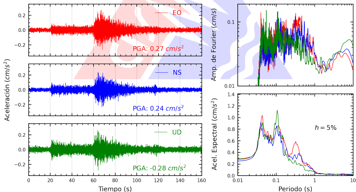
Figura A.34: Registros tiempo-historia, espectros de Fourier y de respuesta en las direcciones EO, NS y vertical de la estación USMP. Sismo de Chimbote, Santa - Áncash del 2025-12-28, 18:19:55 (Hora local)
