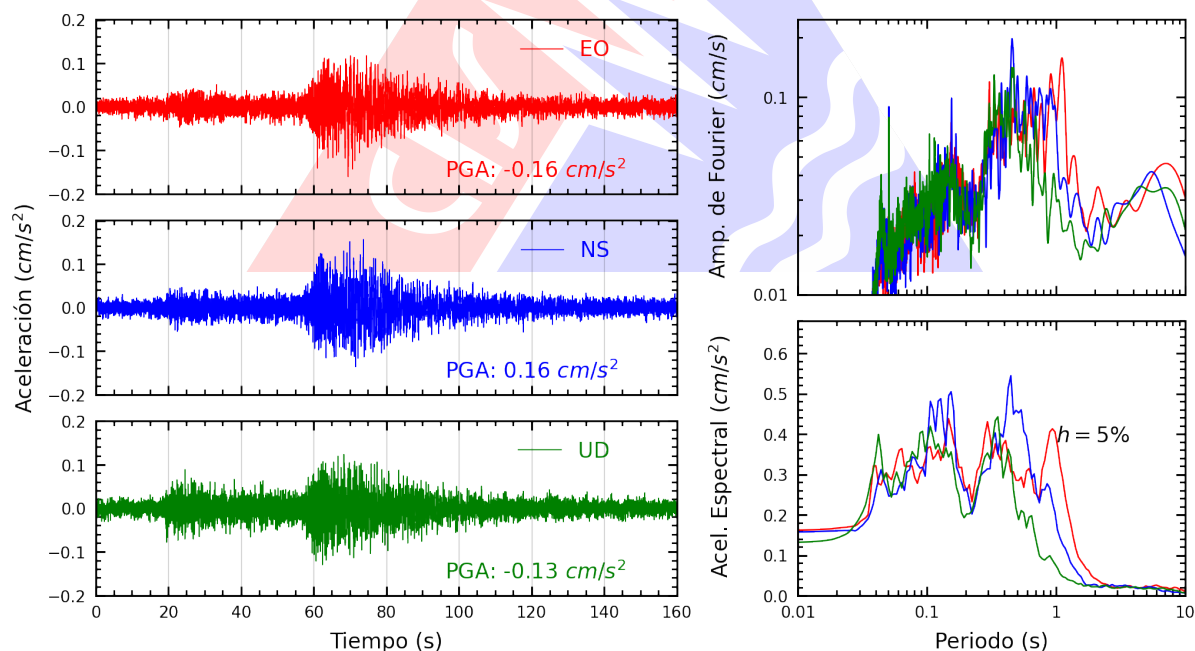
Figura A.42: Registros tiempo-historia, espectros de Fourier y de respuesta en las direcciones EO, NS y vertical de la estación BONDY. Sismo de Chimbote, Santa - Áncash del 2025-12-28, 18:19:55 (Hora local)
