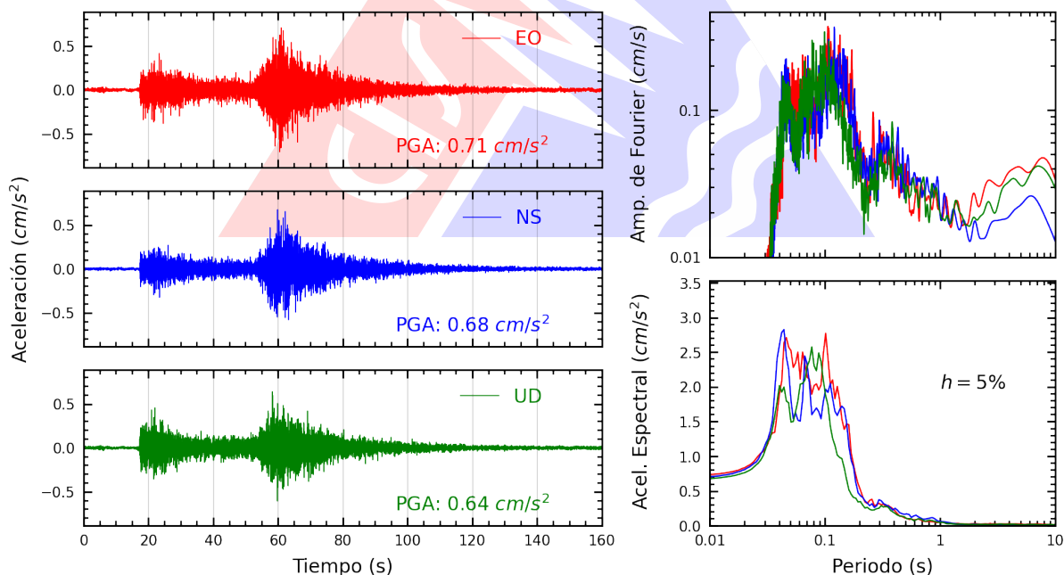
Figura A.14: Registros tiempo-historia, espectros de Fourier y de respuesta en las direcciones EO, NS y vertical de la estación AMORE. Sismo de Chimbote, Santa - Áncash del 2025-12-28, 18:19:55 (Hora local)
