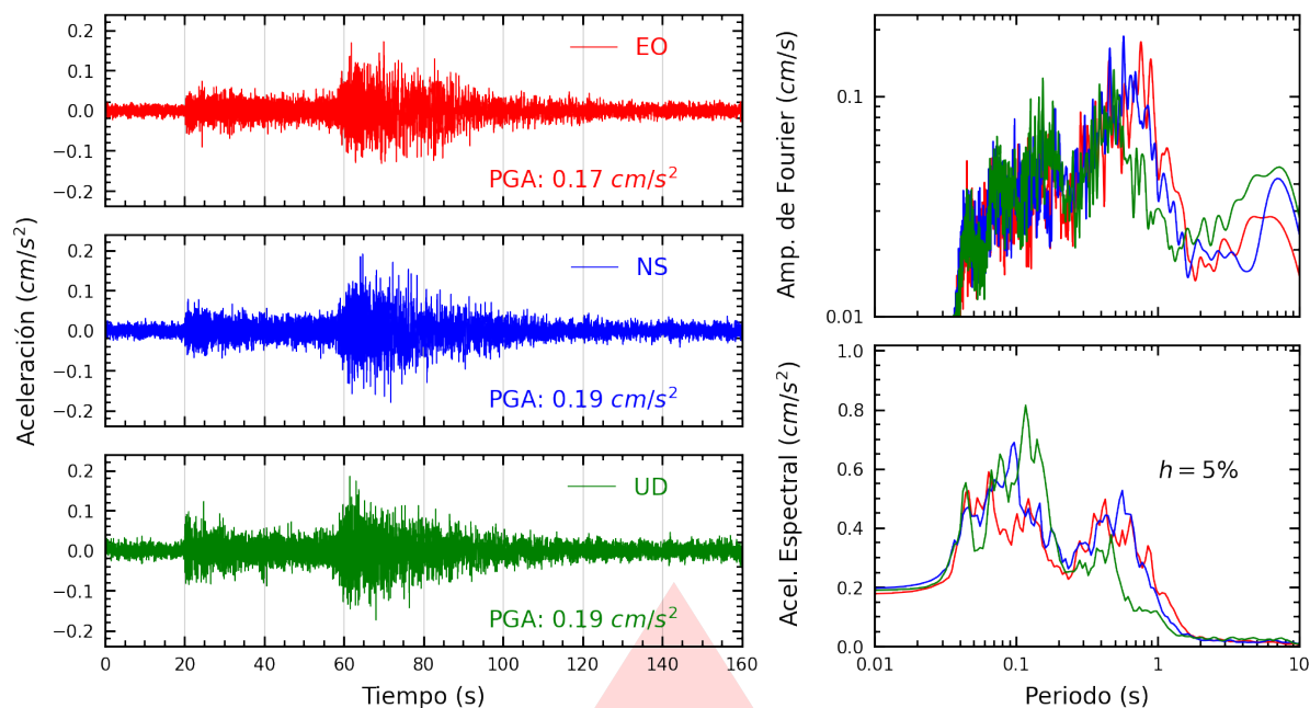
Figura A.41: Registros tiempo-historia, espectros de Fourier y de respuesta en las direcciones EO, NS y vertical de la estación UNFV. Sismo de Chimbote, Santa - Áncash del 2025-12-28, 18:19:55 (Hora local)
