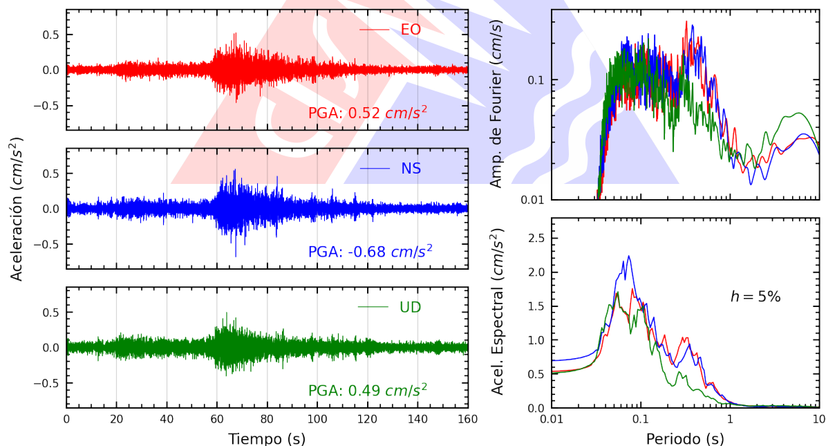
Figura A.16: Registros tiempo-historia, espectros de Fourier y de respuesta en las direcciones EO, NS y vertical de la estación SJLSC. Sismo de Chimbote, Santa - Áncash del 2025-12-28, 18:19:55 (Hora local)
