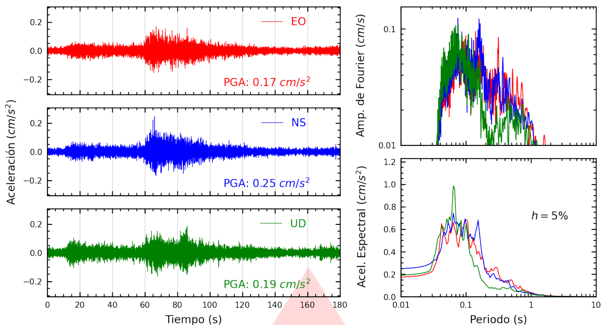
Figura A.37: Registros tiempo-historia, espectros de Fourier y de respuesta en las direcciones EO, NS y vertical de la estación ASIA. Sismo de Chimbote, Santa - Áncash del 2025-12-28, 18:19:55 (Hora local)
