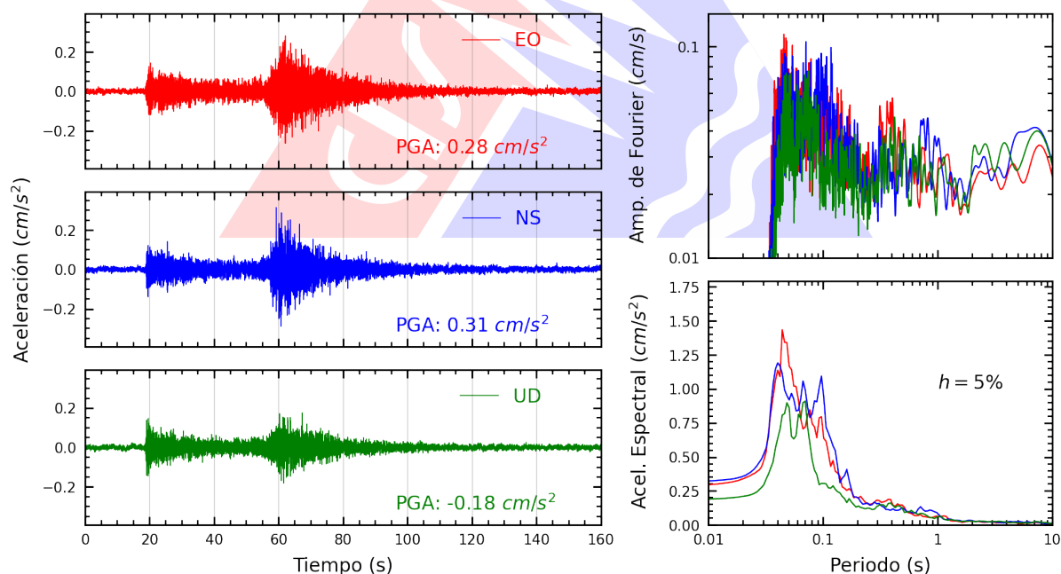
Figura A.32: Registros tiempo-historia, espectros de Fourier y de respuesta en las direcciones EO, NS y vertical de la estación UCSS. Sismo de Chimbote, Santa - Áncash del 2025-12-28, 18:19:55 (Hora local)
