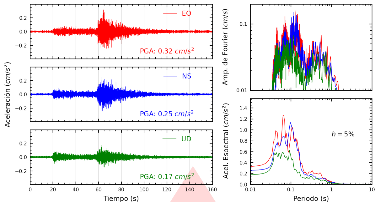
Figura A.31: Registros tiempo-historia, espectros de Fourier y de respuesta en las direcciones EO, NS y vertical de la estación ATARJ. Sismo de Chimbote, Santa - Áncash del 2025-12-28, 18:19:55 (Hora local)
