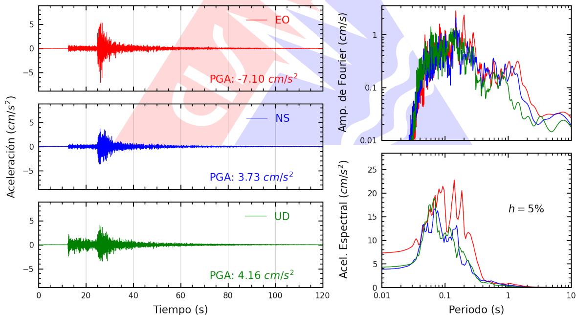
Figura A.4: Registros tiempo-historia, espectros de Fourier y de respuesta en las direcciones EO, NS y vertical de la estación UPAOT. Sismo de Chimbote, Santa - Áncash del 2025-12-28, 18:19:55 (Hora local)
