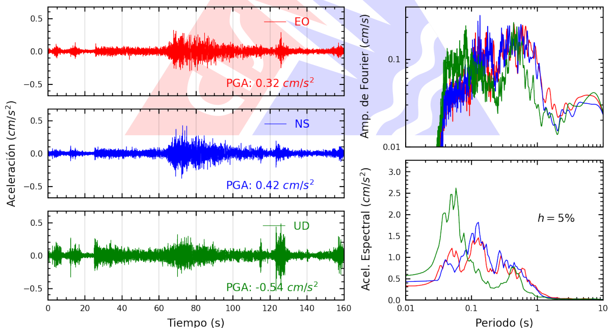
Figura A.18: Registros tiempo-historia, espectros de Fourier y de respuesta en las direcciones EO, NS y vertical de la estación SOCHO. Sismo de Chimbote, Santa - Áncash del 2025-12-28, 18:19:55 (Hora local)
