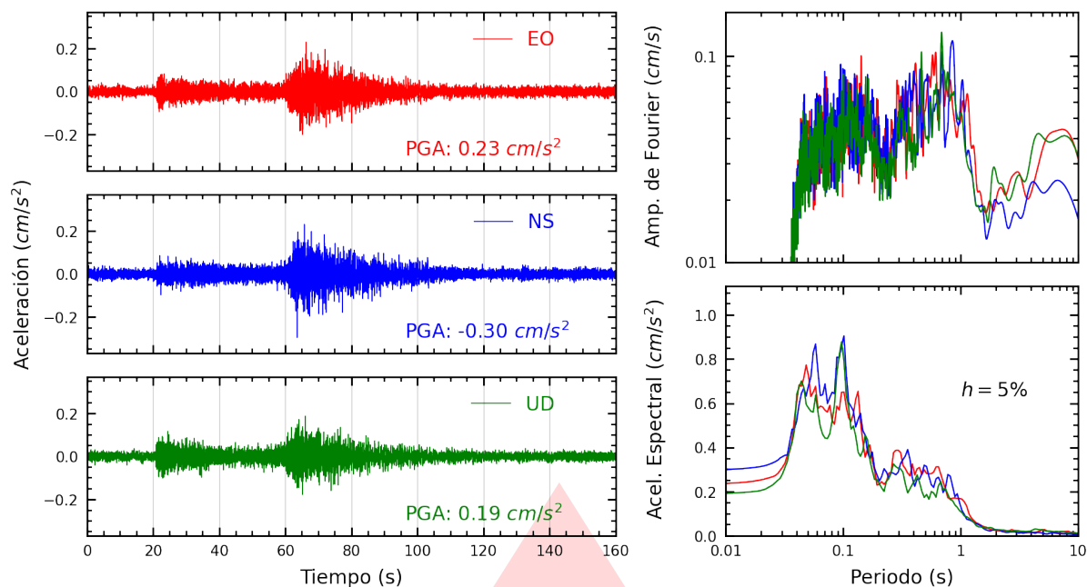
Figura A.33: Registros tiempo-historia, espectros de Fourier y de respuesta en las direcciones EO, NS y vertical de la estación SERVI. Sismo de Chimbote, Santa - Áncash del 2025-12-28, 18:19:55 (Hora local)
