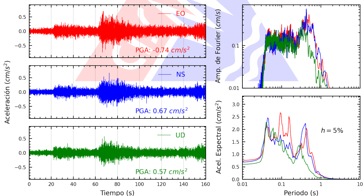
Figura A.12: Registros tiempo-historia, espectros de Fourier y de respuesta en las direcciones EO, NS y vertical de la estación UNTEL. Sismo de Chimbote, Santa - Áncash del 2025-12-28, 18:19:55 (Hora local)
