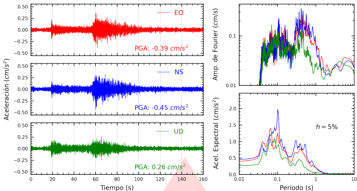
Figura A.23: Registros tiempo-historia, espectros de Fourier y de respuesta en las direcciones EO, NS y vertical de la estación MADRE. Sismo de Chimbote, Santa - Áncash del 2025-12-28, 18:19:55 (Hora local)
