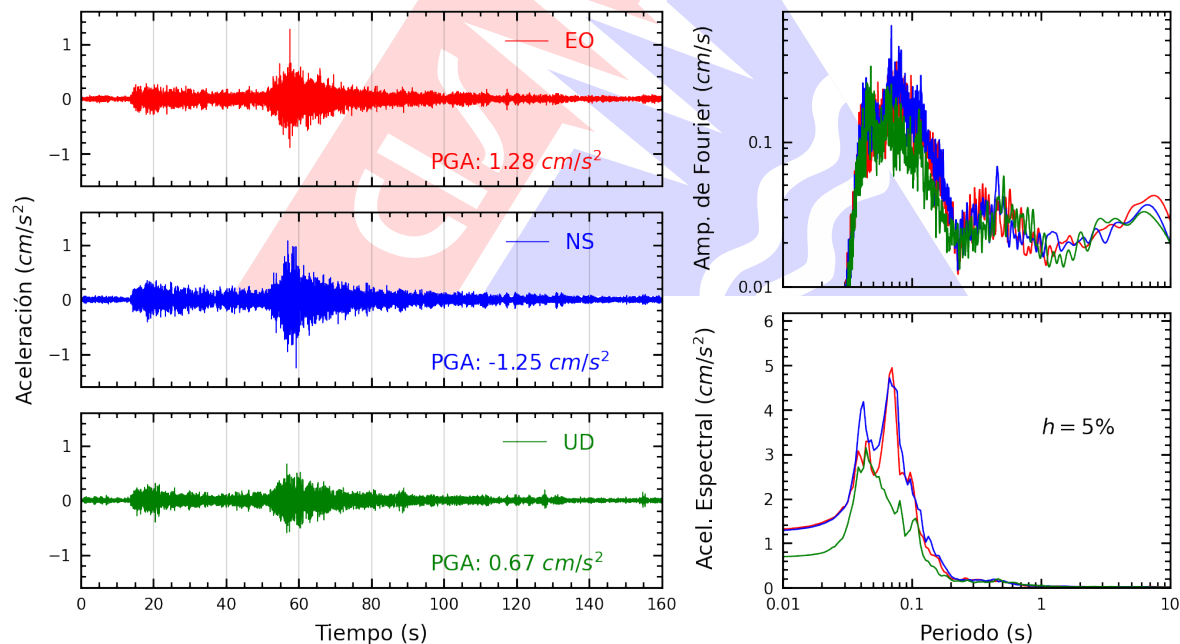
Figura A.6: Registros tiempo-historia, espectros de Fourier y de respuesta en las direcciones EO, NS y vertical de la estación JOSEO. Sismo de Chimbote, Santa - Áncash del 2025-12-28, 18:19:55 (Hora local)
