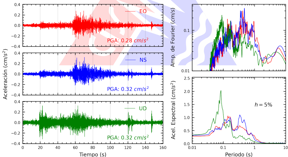
Figura A.28: Registros tiempo-historia, espectros de Fourier y de respuesta en las direcciones EO, NS y vertical de la estación RAMON. Sismo de Chimbote, Santa - Áncash del 2025-12-28, 18:19:55 (Hora local)
