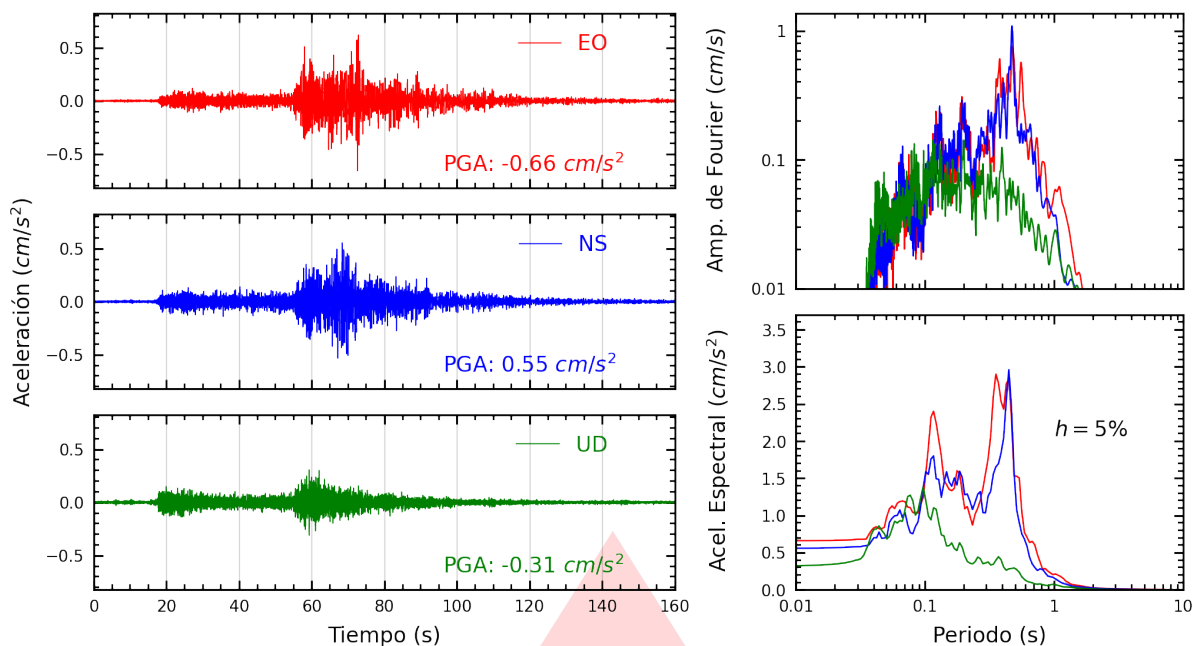
Figura A.17: Registros tiempo-historia, espectros de Fourier y de respuesta en las direcciones EO, NS y vertical de la estación VHAYA. Sismo de Chimbote, Santa - Áncash del 2025-12-28, 18:19:55 (Hora local)
