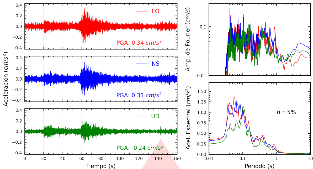
Figura A.27: Registros tiempo-historia, espectros de Fourier y de respuesta en las direcciones EO, NS y vertical de la estación CEPRE. Sismo de Chimbote, Santa - Áncash del 2025-12-28, 18:19:55 (Hora local)
