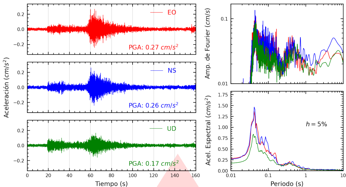
Figura A.35: Registros tiempo-historia, espectros de Fourier y de respuesta en las direcciones EO, NS y vertical de la estación SJLCE. Sismo de Chimbote, Santa - Áncash del 2025-12-28, 18:19:55 (Hora local)
