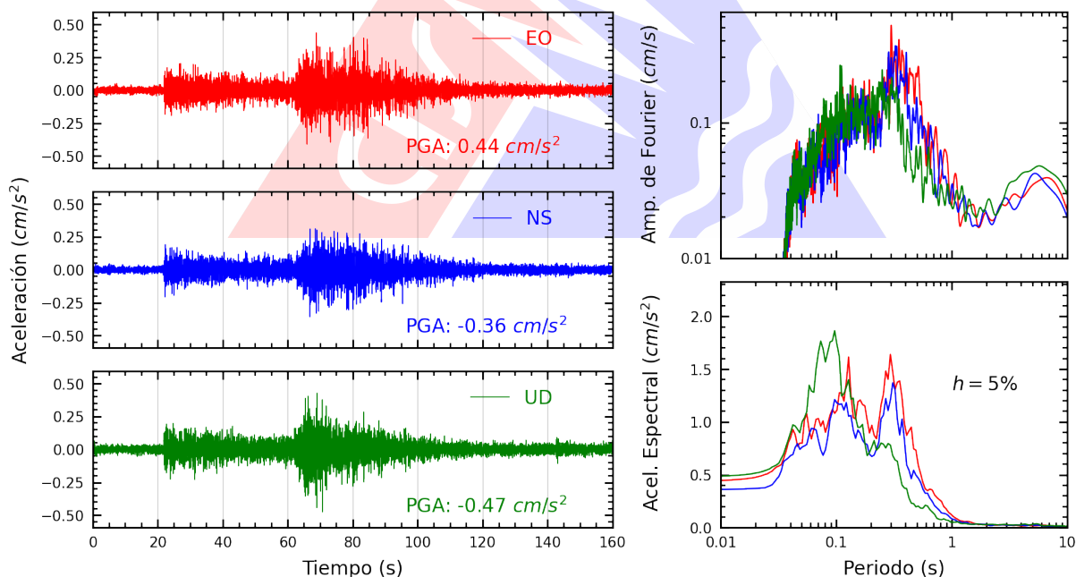
Figura A.20: Registros tiempo-historia, espectros de Fourier y de respuesta en las direcciones EO, NS y vertical de la estación SOVES. Sismo de Chimbote, Santa - Áncash del 2025-12-28, 18:19:55 (Hora local)
