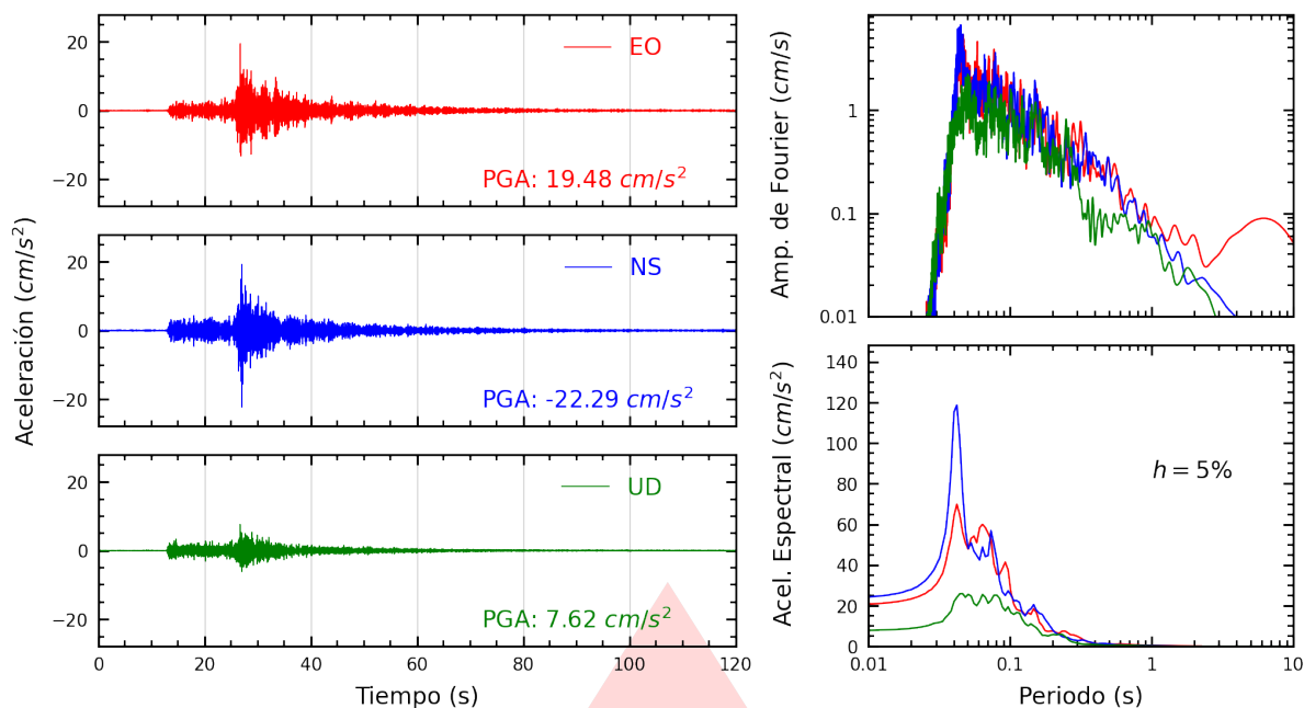
Figura A.3: Registros tiempo-historia, espectros de Fourier y de respuesta en las direcciones EO, NS y vertical de la estación SCTRU. Sismo de Chimbote, Santa - Áncash del 2025-12-28, 18:19:55 (Hora local)
