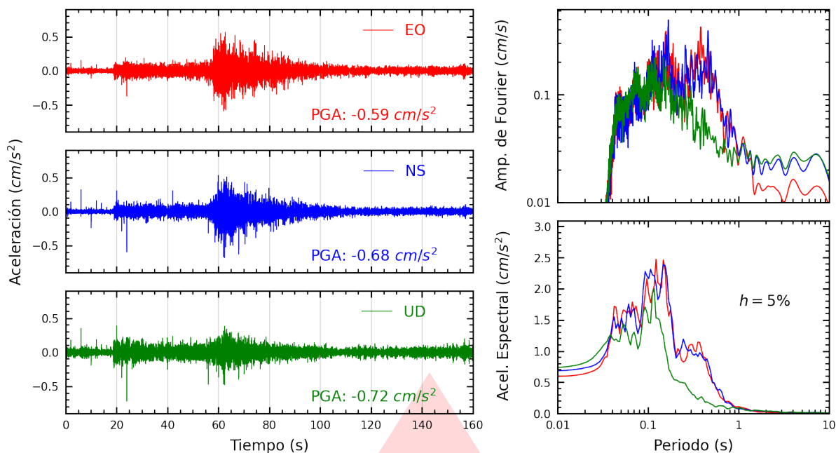
Figura A.13: Registros tiempo-historia, espectros de Fourier y de respuesta en las direcciones EO, NS y vertical de la estación SCOLI. Sismo de Chimbote, Santa - Áncash del 2025-12-28, 18:19:55 (Hora local)
