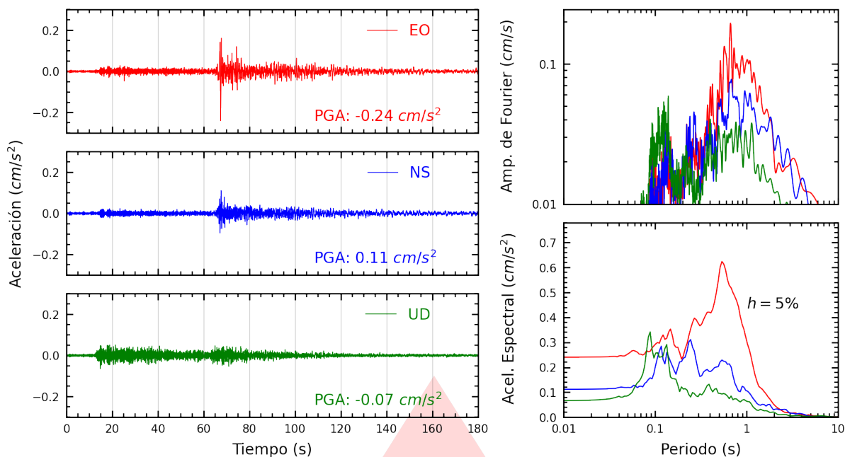
Figura A.39: Registros tiempo-historia, espectros de Fourier y de respuesta en las direcciones EO, NS y vertical de la estación UNIA. Sismo de Chimbote, Santa - Áncash del 2025-12-28, 18:19:55 (Hora local)
