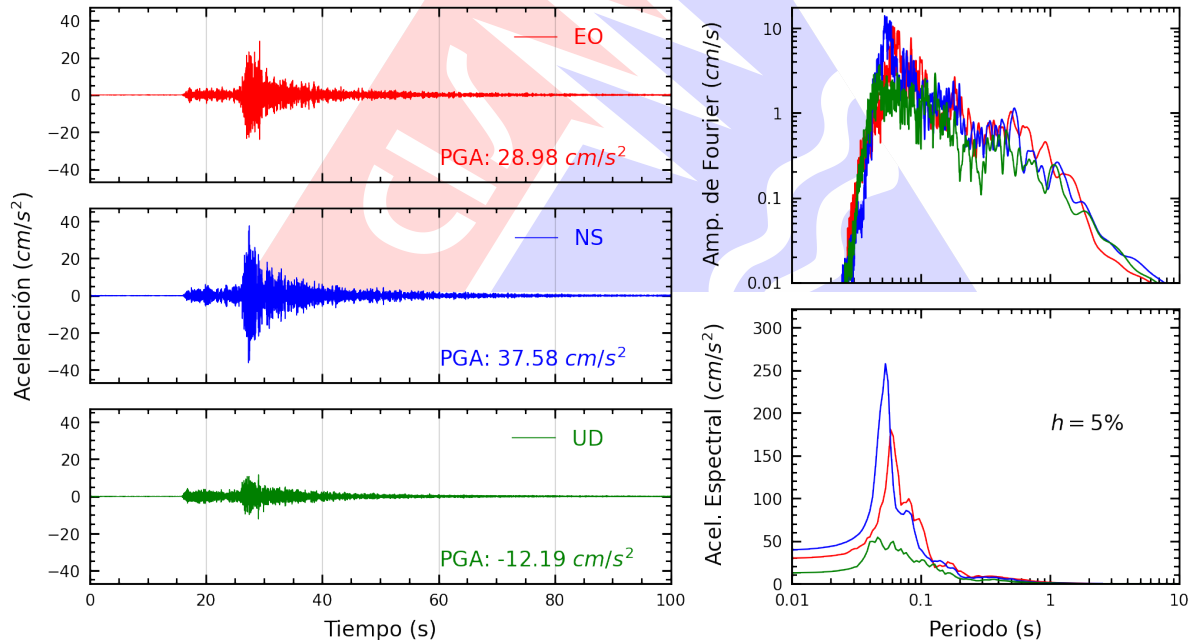
Figura A.2: Registros tiempo-historia, espectros de Fourier y de respuesta en las direcciones EO, NS y vertical de la estación UNS. Sismo de Chimbote, Santa - Áncash del 2025-12-28, 18:19:55 (Hora local)
