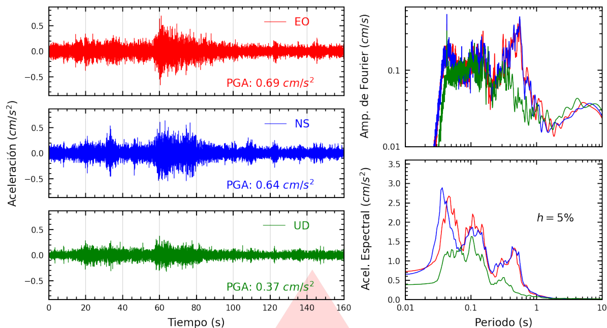
Figura A.15: Registros tiempo-historia, espectros de Fourier y de respuesta en las direcciones EO, NS y vertical de la estación OLIVO. Sismo de Chimbote, Santa - Áncash del 2025-12-28, 18:19:55 (Hora local)
