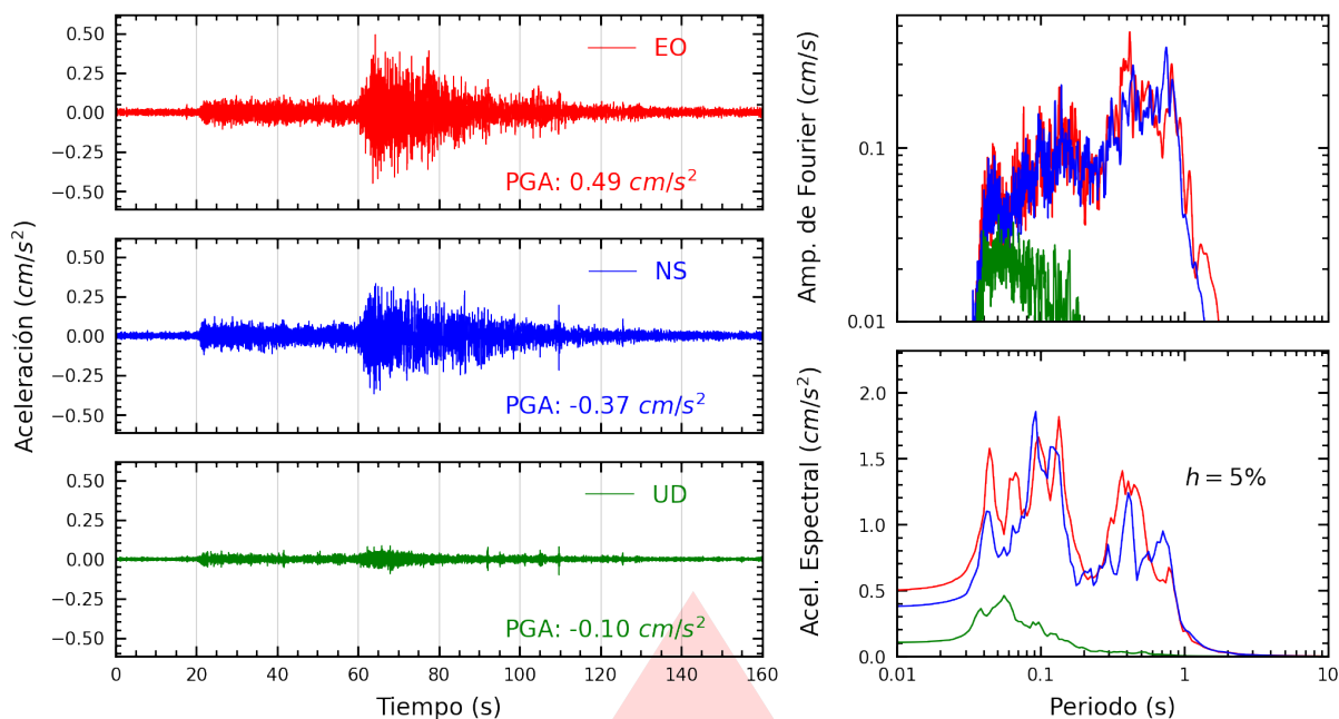
Figura A.19: Registros tiempo-historia, espectros de Fourier y de respuesta en las direcciones EO, NS y vertical de la estación UCVAT. Sismo de Chimbote, Santa - Áncash del 2025-12-28, 18:19:55 (Hora local)
