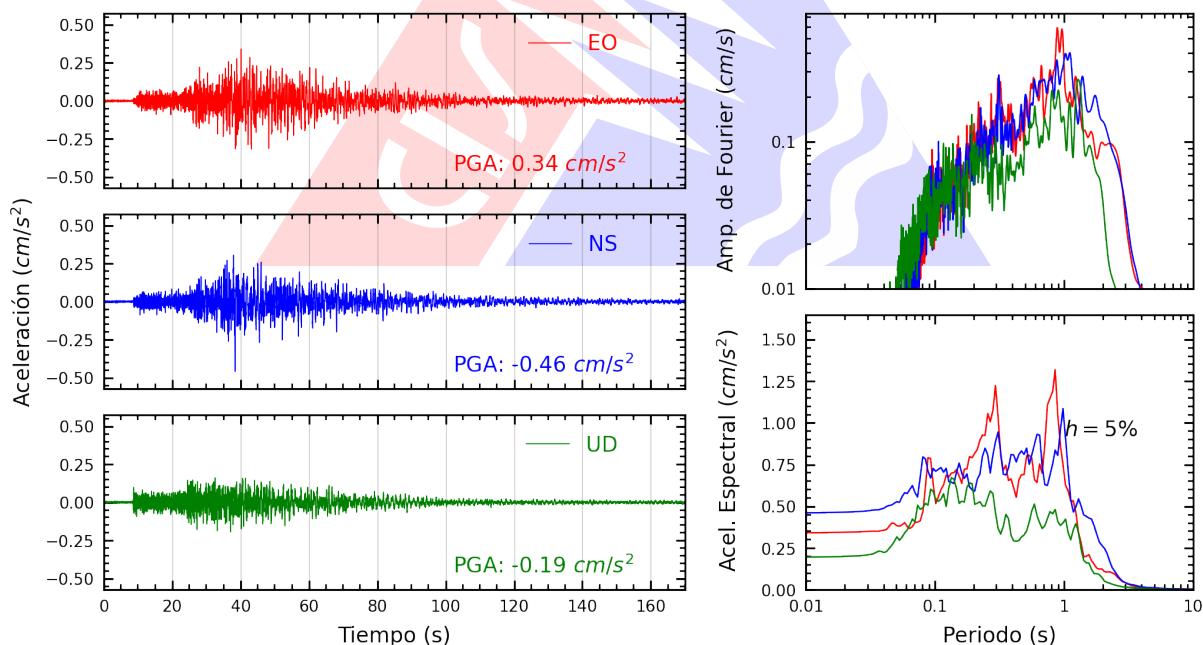
Figura A.22: Registros tiempo-historia, espectros de Fourier y de respuesta en las direcciones EO, NS y vertical de la estación UNC. Sismo de Chimbote, Santa - Áncash del 2025-12-28, 18:19:55 (Hora local)
