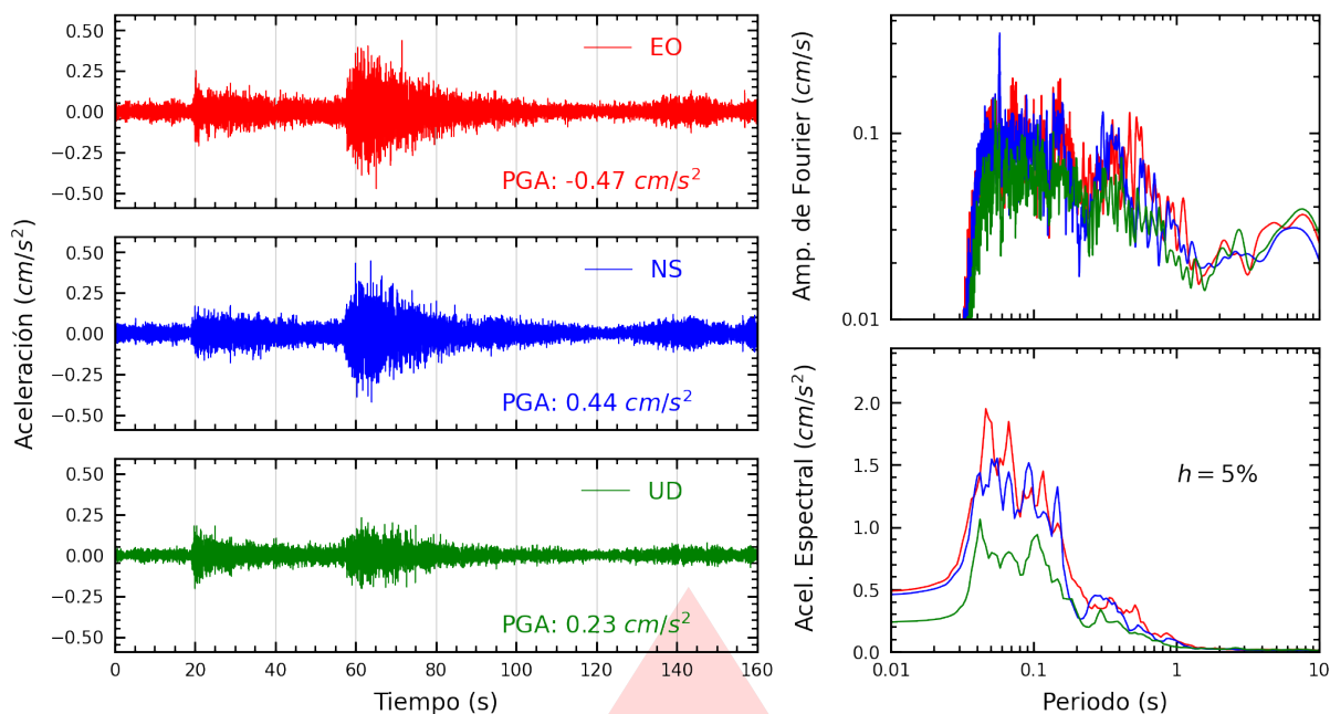
Figura A.21: Registros tiempo-historia, espectros de Fourier y de respuesta en las direcciones EO, NS y vertical de la estación FICPE. Sismo de Chimbote, Santa - Áncash del 2025-12-28, 18:19:55 (Hora local)
