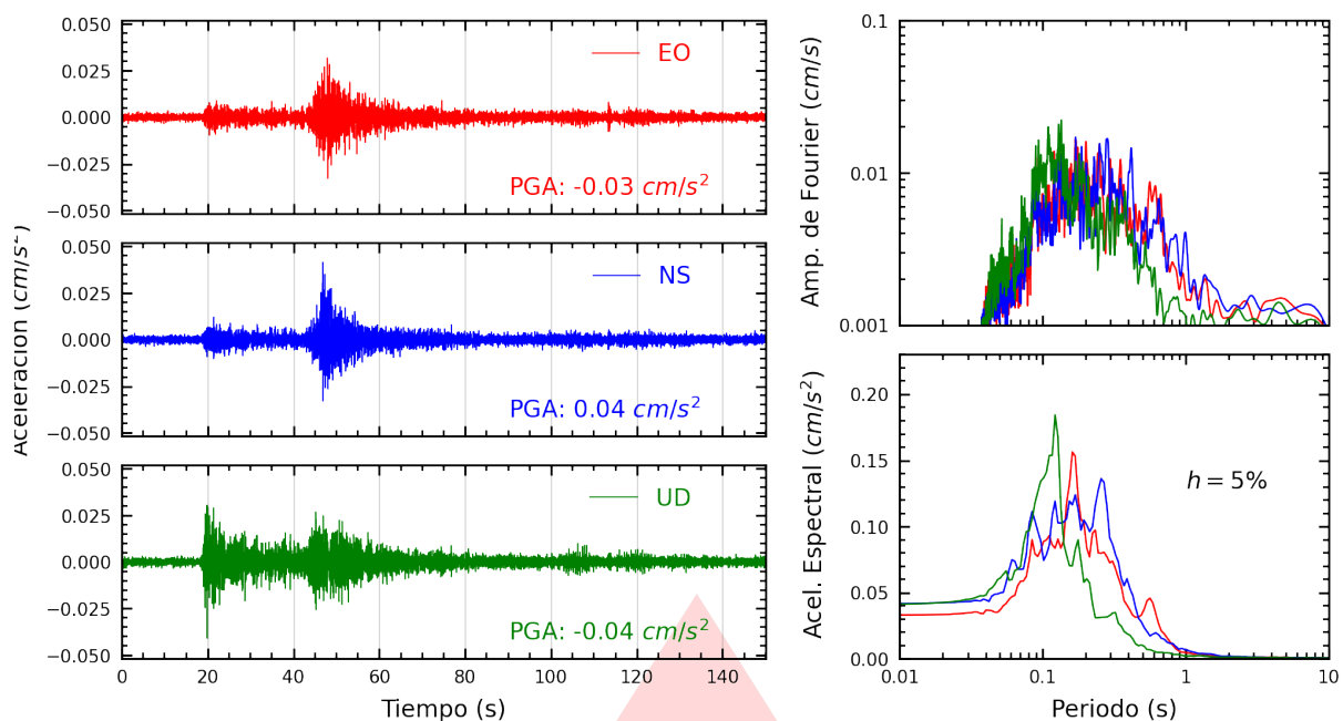
Figura A.1: Registros tiempo-historia, espectros de Fourier y de respuesta en las direcciones EO, NS y vertical de la estación UNIA. Sismo de Codo del Pozuzo, Puerto Inca - Huánuco del 2025-12-30, 20:28:16 (Hora local)
